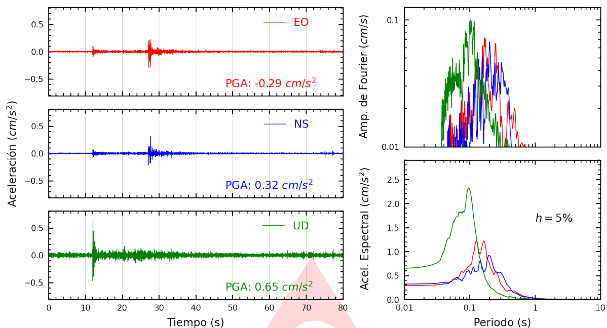
Figura A.1: Registros tiempo-historia, espectros de Fourier y de respuesta en las direcciones EO, NS y vertical de la estación SCPUC. Sismo de Pucallpa, Coronel Portillo - Ucayali del 2023-05-04, 20:06:05 (Hora local)
