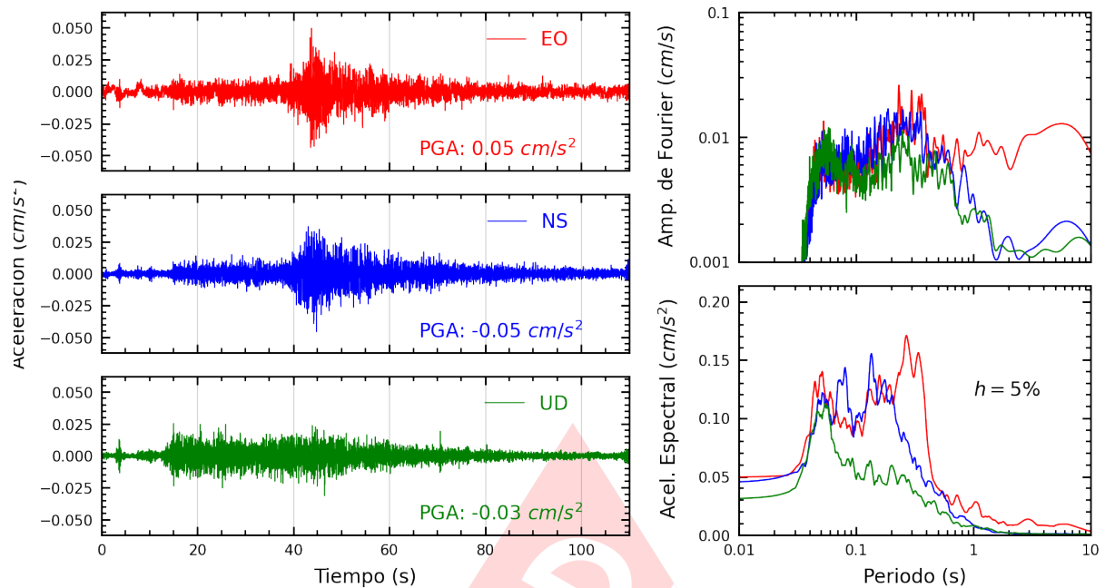
Figura A.9: Registros tiempo-historia, espectros de Fourier y de respuesta en las direcciones EO, NS y vertical de la estación SCCHI. Sismo de Salaverry, Trujillo - La Libertad del 2023-05-11, 01:29:14 (Hora local)
