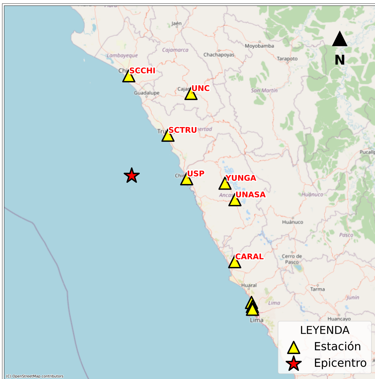
Figura 2: Mapa de ubicación de la(s) estación(es) acelerográfica(s) a nivel nacional correspondiente(s) al Sismo de Salaverry, Trujillo - La Libertad del 11 de mayo de 2023 a las 01:29:14 (hora local)
