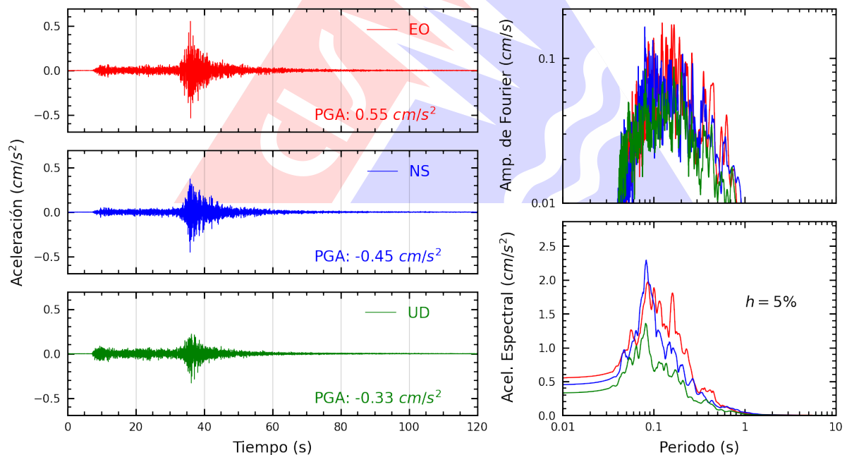
Figura A.2: Registros tiempo-historia, espectros de Fourier y de respuesta en las direcciones EO, NS y vertical de la estación YUNGA. Sismo de Salaverry, Trujillo - La Libertad del 2023-05-11, 01:29:14 (Hora local)
