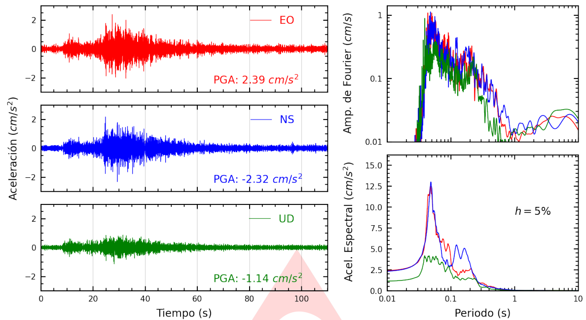
Figura A.1: Registros tiempo-historia, espectros de Fourier y de respuesta en las direcciones EO, NS y vertical de la estación USP. Sismo de Salaverry, Trujillo - La Libertad del 2023-05-11, 01:29:14 (Hora local)
