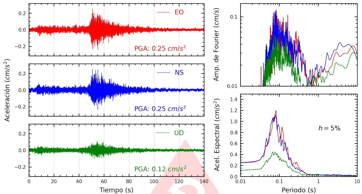
Figura A.5: Registros tiempo-historia, espectros de Fourier y de respuesta en las direcciones EO, NS y vertical de la estación DEFEN. Sismo de Salaverry, Trujillo - La Libertad del 2023-05-11, 01:29:14 (Hora local)
