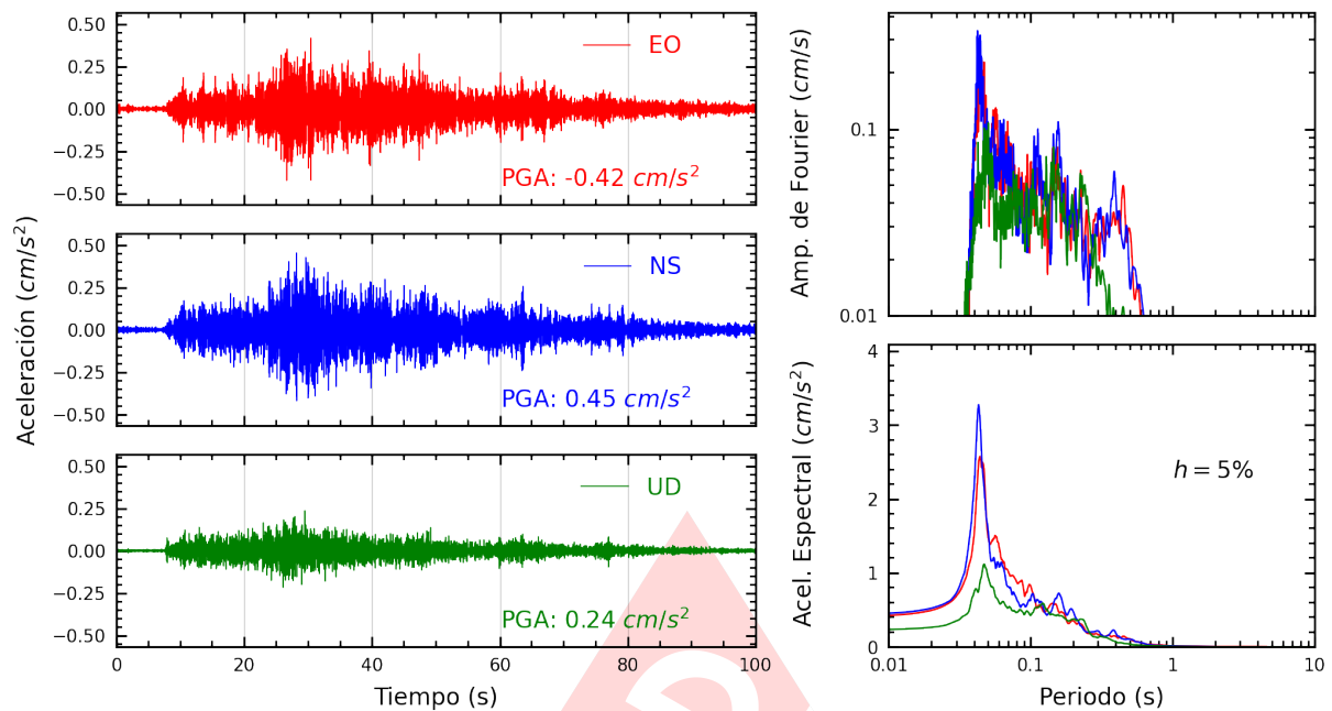
Figura A.3: Registros tiempo-historia, espectros de Fourier y de respuesta en las direcciones EO, NS y vertical de la estación SCTRU. Sismo de Salaverry, Trujillo - La Libertad del 2023-05-11, 01:29:14 (Hora local)
