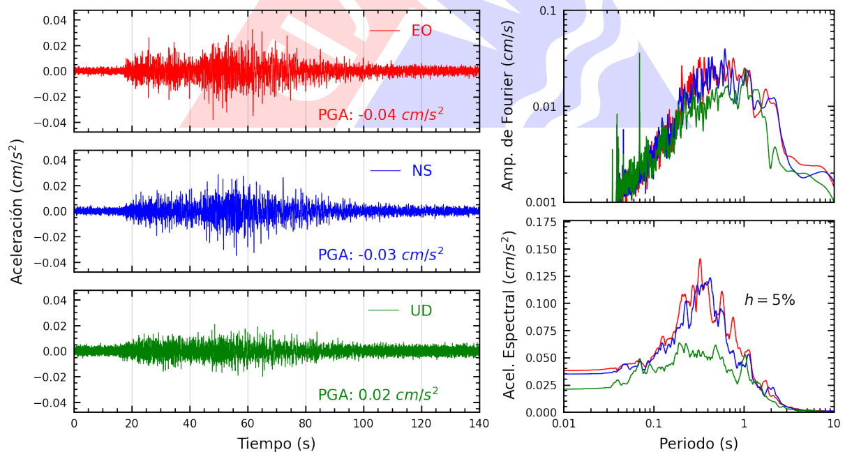
Figura A.10: Registros tiempo-historia, espectros de Fourier y de respuesta en las direcciones EO, NS y vertical de la estación UNC. Sismo de Salaverry, Trujillo - La Libertad del 2023-05-11, 01:29:14 (Hora local)
