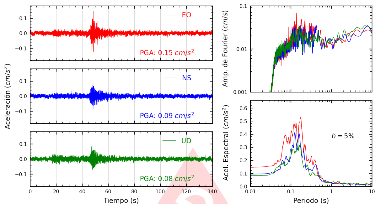
Figura A.7: Registros tiempo-historia, espectros de Fourier y de respuesta en las direcciones EO, NS y vertical de la estación UNASA. Sismo de Salaverry, Trujillo - La Libertad del 2023-05-11, 01:29:14 (Hora local)
