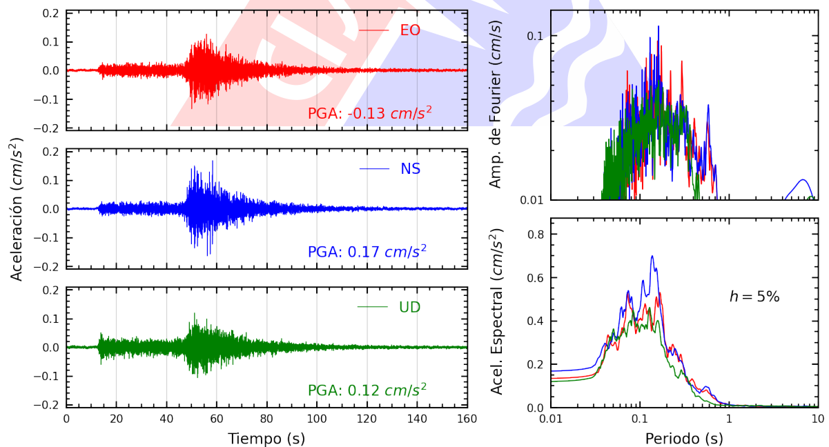
Figura A.6: Registros tiempo-historia, espectros de Fourier y de respuesta en las direcciones EO, NS y vertical de la estación CARAL. Sismo de Salaverry, Trujillo - La Libertad del 2023-05-11, 01:29:14 (Hora local)
