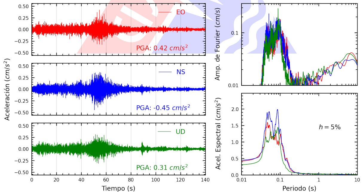
Figura A.4: Registros tiempo-historia, espectros de Fourier y de respuesta en las direcciones EO, NS y vertical de la estación SROSA. Sismo de Salaverry, Trujillo - La Libertad del 2023-05-11, 01:29:14 (Hora local)
