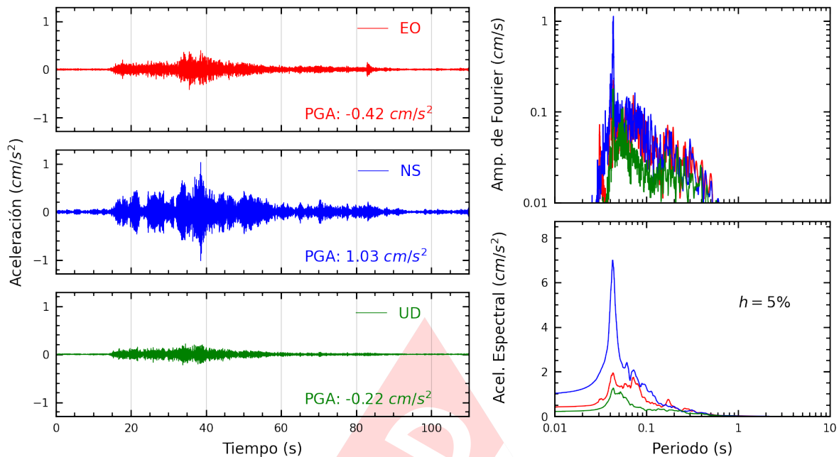
Figura A.5: Registros tiempo-historia, espectros de Fourier y de respuesta en las direcciones EO, NS y vertical de la estación UNAM. Sismo de Tacna, Tacna - Tacna del 2023-06-05, 11:54:51 (Hora local)
