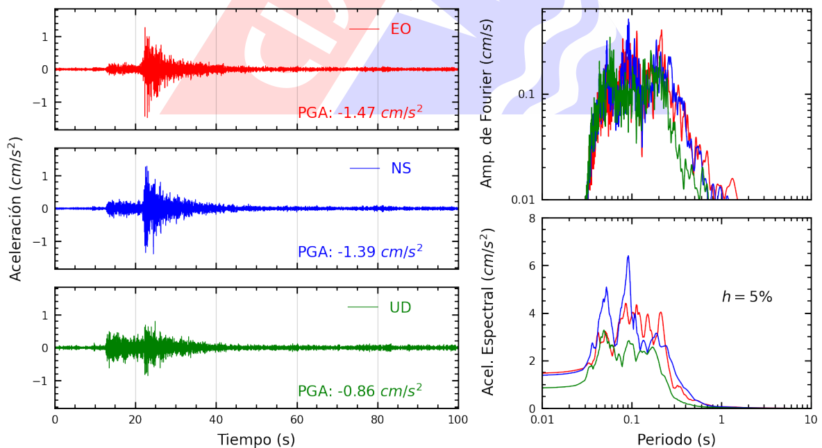
Figura A.4: Registros tiempo-historia, espectros de Fourier y de respuesta en las direcciones EO, NS y vertical de la estación UJBG2. Sismo de Tacna, Tacna - Tacna del 2023-06-05, 11:54:51 (Hora local)
