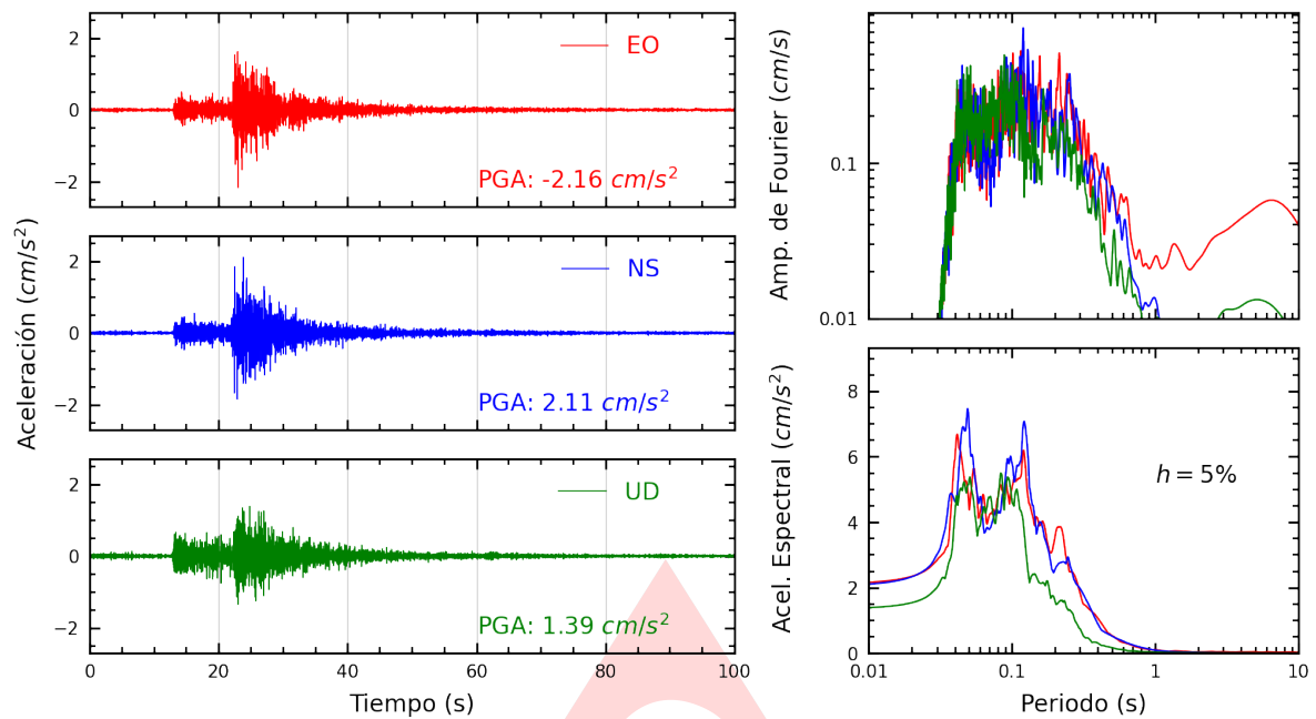
Figura A.1: Registros tiempo-historia, espectros de Fourier y de respuesta en las direcciones EO, NS y vertical de la estación UJBG3. Sismo de Tacna, Tacna - Tacna del 2023-06-05, 11:54:51 (Hora local)
