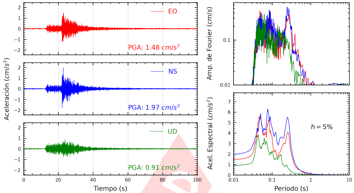
Figura A.3: Registros tiempo-historia, espectros de Fourier y de respuesta en las direcciones EO, NS y vertical de la estación CREY. Sismo de Tacna, Tacna - Tacna del 2023-06-05, 11:54:51 (Hora local)
