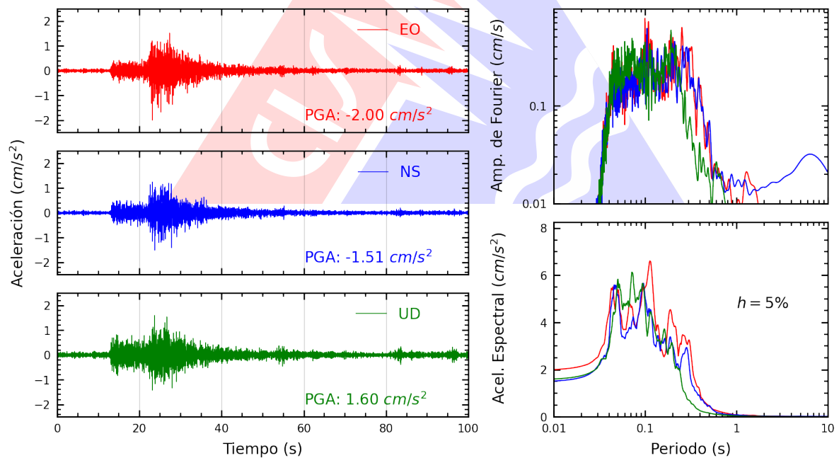
Figura A.2: Registros tiempo-historia, espectros de Fourier y de respuesta en las direcciones EO, NS y vertical de la estación SCTAC. Sismo de Tacna, Tacna - Tacna del 2023-06-05, 11:54:51 (Hora local)
