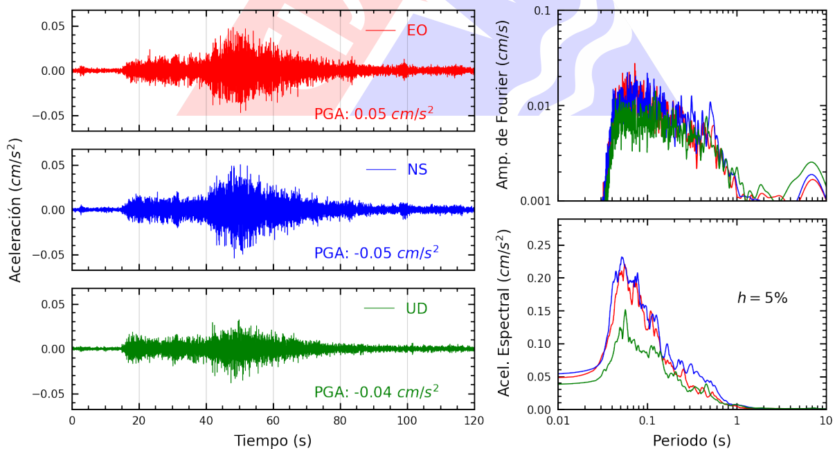
Figura A.6: Registros tiempo-historia, espectros de Fourier y de respuesta en las direcciones EO, NS y vertical de la estación UNSA. Sismo de Tacna, Tacna - Tacna del 2023-06-05, 11:54:51 (Hora local)
