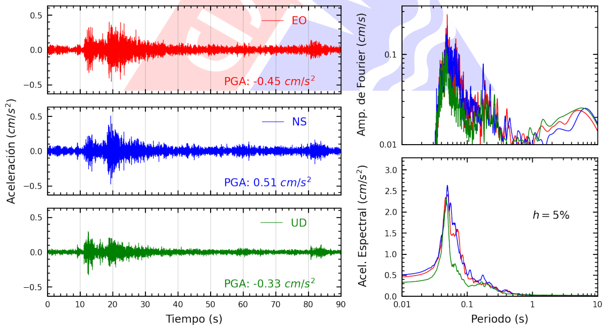
Figura A.28: Registros tiempo-historia, espectros de Fourier y de respuesta en las direcciones EO, NS y vertical de la estación UPCVI. Sismo de Provincia Constitucional del Callao , Callao - Lima del 2023-06-12, 06:20:30 (Hora local)
