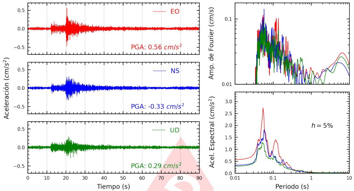
Figura A.25: Registros tiempo-historia, espectros de Fourier y de respuesta en las direcciones EO, NS y vertical de la estación IMCA. Sismo de Provincia Constitucional del Callao , Callao - Lima del 2023-06-12, 06:20:30 (Hora local)
