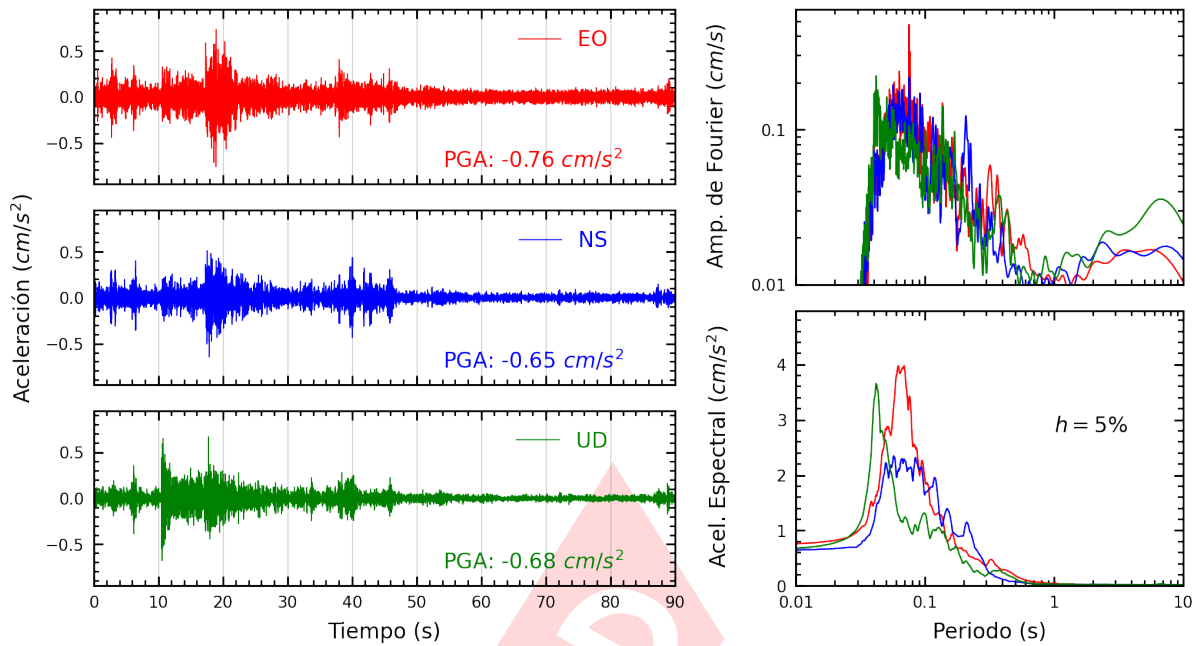
Figura A.21: Registros tiempo-historia, espectros de Fourier y de respuesta en las direcciones EO, NS y vertical de la estación UPCSM. Sismo de Provincia Constitucional del Callao , Callao - Lima del 2023-06-12, 06:20:30 (Hora local)
