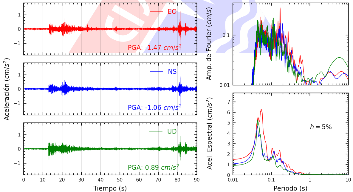
Figura A.14: Registros tiempo-historia, espectros de Fourier y de respuesta en las direcciones EO, NS y vertical de la estación PRADO. Sismo de Provincia Constitucional del Callao , Callao - Lima del 2023-06-12, 06:20:30 (Hora local)
