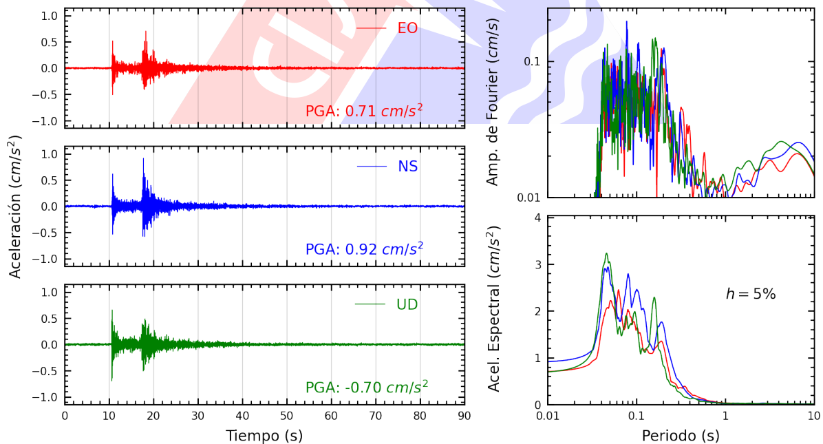
Figura A.20: Registros tiempo-historia, espectros de Fourier y de respuesta en las direcciones EO, NS y vertical de la estación UNFV. Sismo de Provincia Constitucional del Callao , Callao - Lima del 2023-06-12, 06:20:30 (Hora local)
