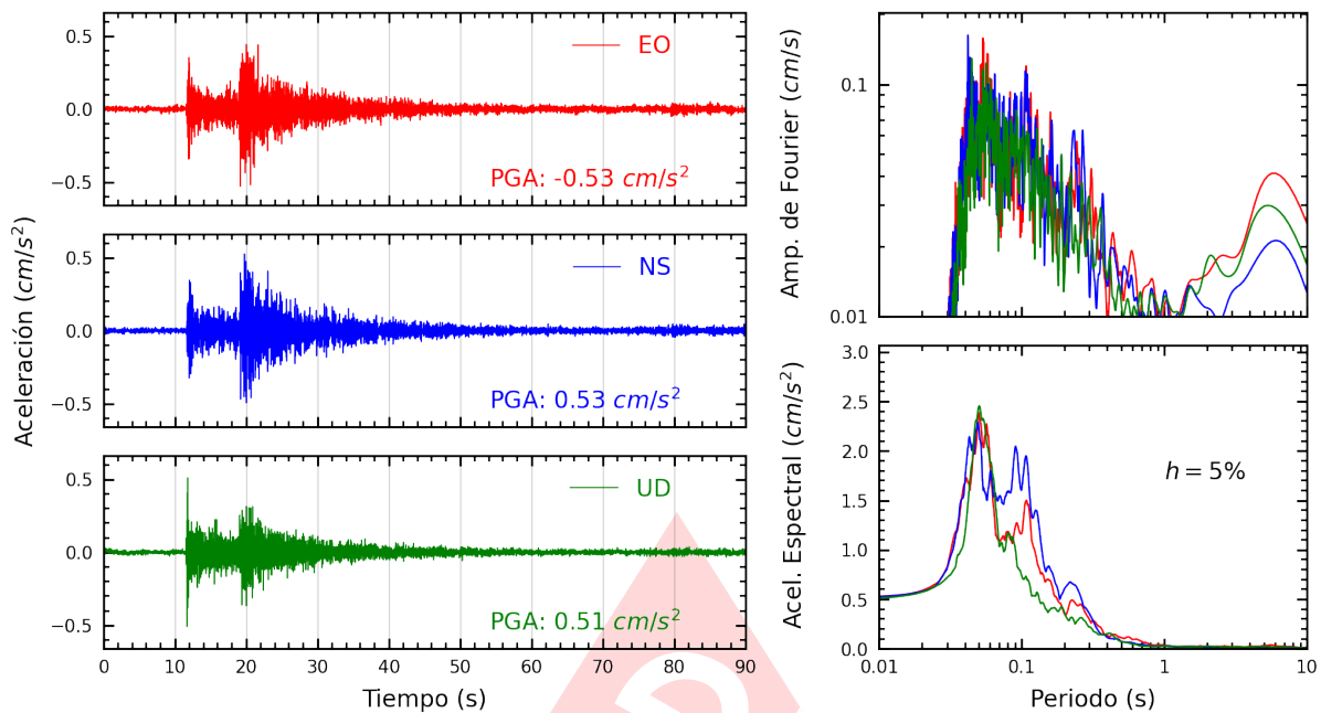
Figura A.27: Registros tiempo-historia, espectros de Fourier y de respuesta en las direcciones EO, NS y vertical de la estación COMAS. Sismo de Provincia Constitucional del Callao , Callao - Lima del 2023-06-12, 06:20:30 (Hora local)
