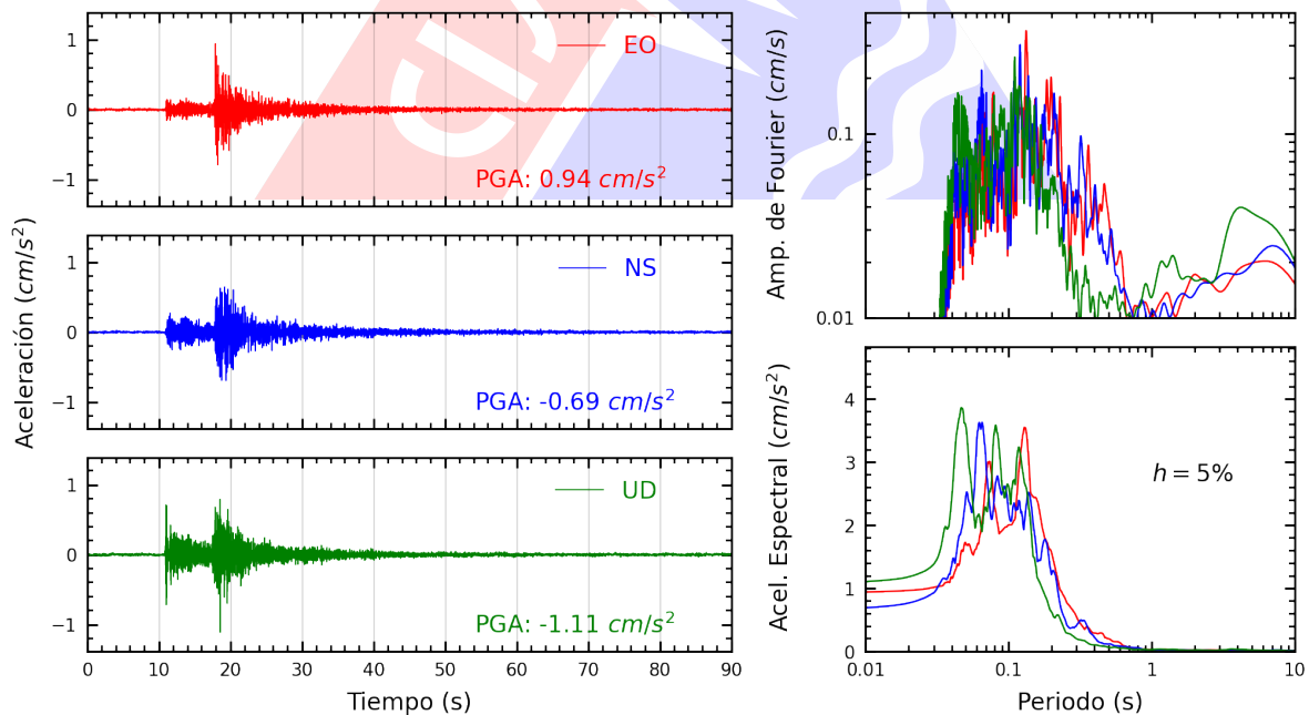
Figura A.16: Registros tiempo-historia, espectros de Fourier y de respuesta en las direcciones EO, NS y vertical de la estación VHAYA. Sismo de Provincia Constitucional del Callao , Callao - Lima del 2023-06-12, 06:20:30 (Hora local)
