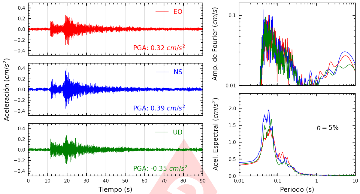
Figura A.31: Registros tiempo-historia, espectros de Fourier y de respuesta en las direcciones EO, NS y vertical de la estación SERVI. Sismo de Provincia Constitucional del Callao , Callao - Lima del 2023-06-12, 06:20:30 (Hora local)
