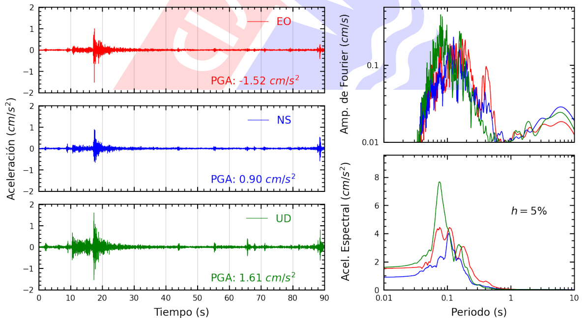
Figura A.12: Registros tiempo-historia, espectros de Fourier y de respuesta en las direcciones EO, NS y vertical de la estación RAMON. Sismo de Provincia Constitucional del Callao , Callao - Lima del 2023-06-12, 06:20:30 (Hora local)
