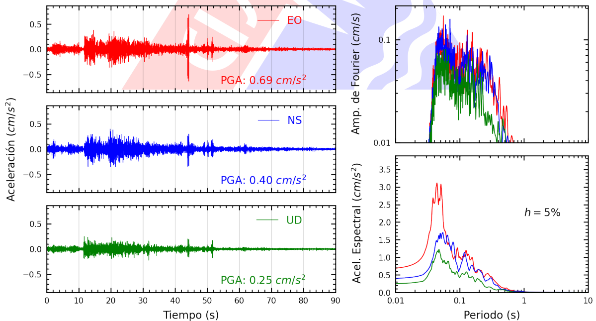
Figura A.24: Registros tiempo-historia, espectros de Fourier y de respuesta en las direcciones EO, NS y vertical de la estación BRISA. Sismo de Provincia Constitucional del Callao , Callao - Lima del 2023-06-12, 06:20:30 (Hora local)
