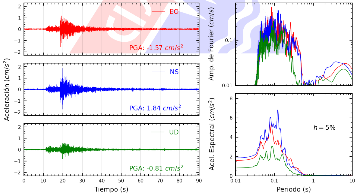
Figura A.8: Registros tiempo-historia, espectros de Fourier y de respuesta en las direcciones EO, NS y vertical de la estación DEFEN. Sismo de Provincia Constitucional del Callao , Callao - Lima del 2023-06-12, 06:20:30 (Hora local)
