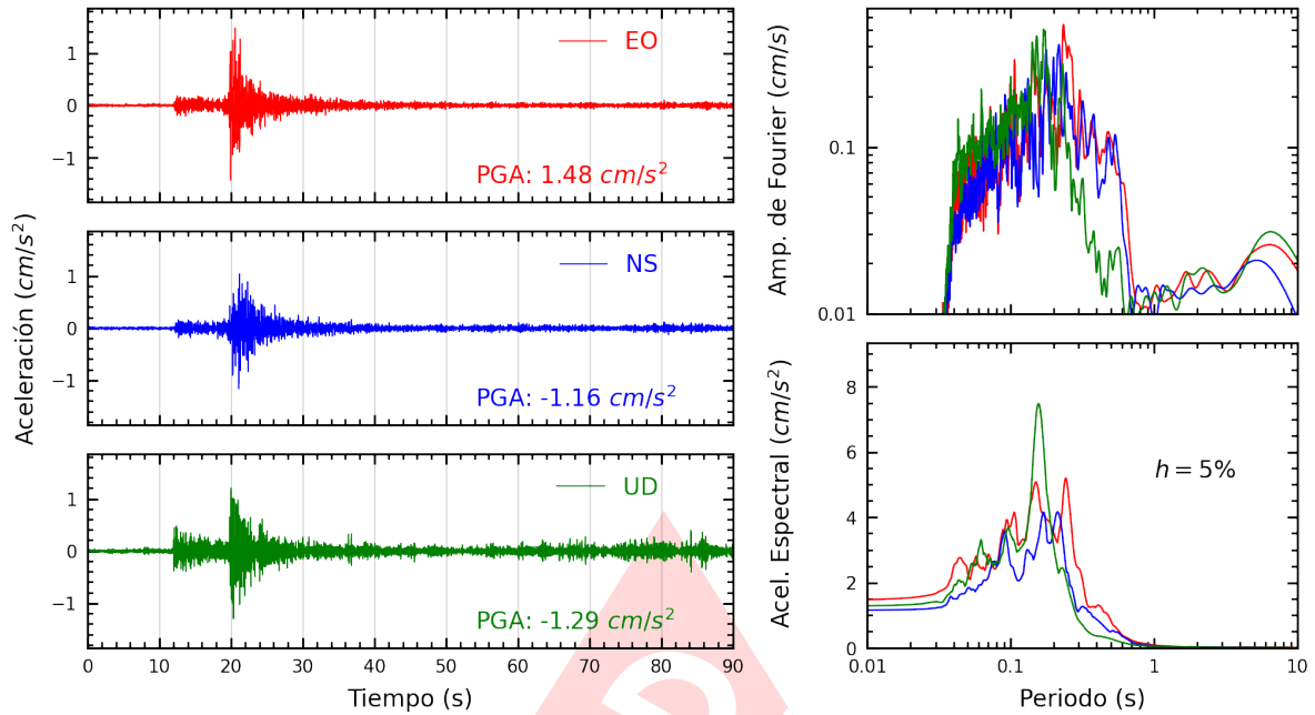
Figura A.13: Registros tiempo-historia, espectros de Fourier y de respuesta en las direcciones EO, NS y vertical de la estación MDPP. Sismo de Provincia Constitucional del Callao , Callao - Lima del 2023-06-12, 06:20:30 (Hora local)
