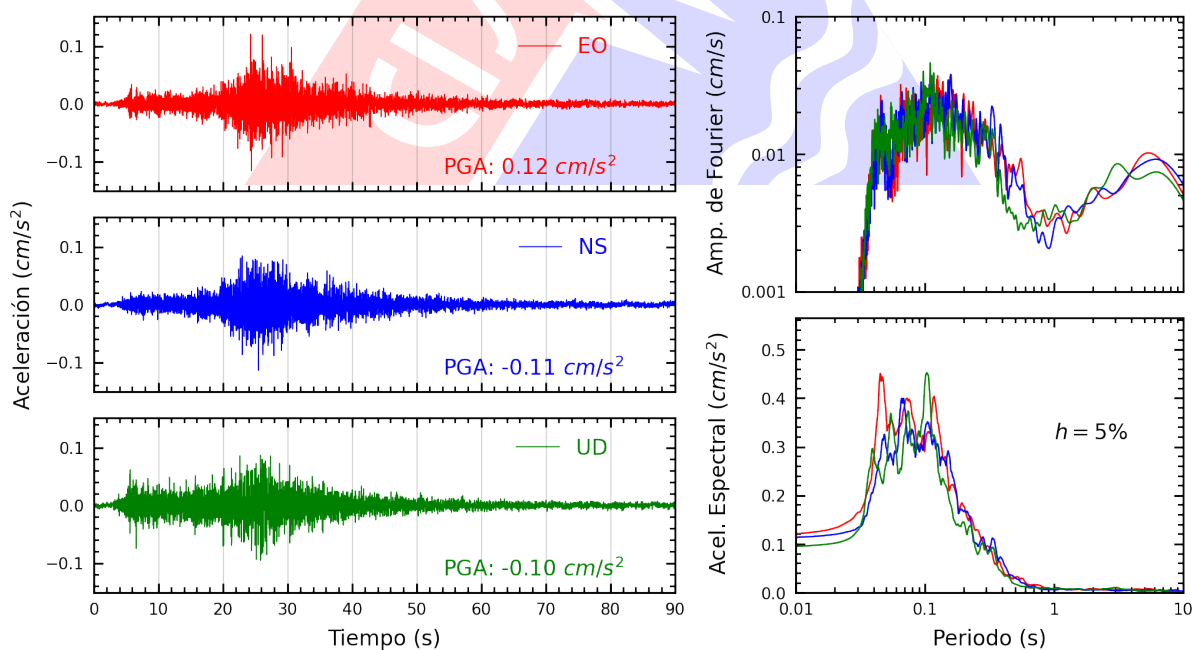
Figura A.34: Registros tiempo-historia, espectros de Fourier y de respuesta en las direcciones EO, NS y vertical de la estación CARAL. Sismo de Provincia Constitucional del Callao , Callao - Lima del 2023-06-12, 06:20:30 (Hora local)
