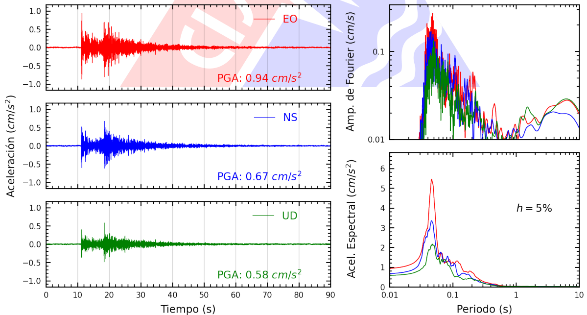
Figura A.18: Registros tiempo-historia, espectros de Fourier y de respuesta en las direcciones EO, NS y vertical de la estación UCSS. Sismo de Provincia Constitucional del Callao , Callao - Lima del 2023-06-12, 06:20:30 (Hora local)
