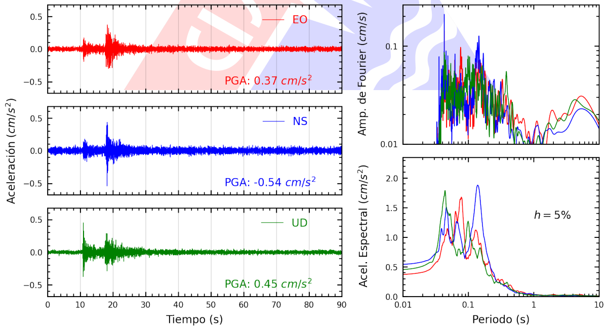
Figura A.26: Registros tiempo-historia, espectros de Fourier y de respuesta en las direcciones EO, NS y vertical de la estación BONDY. Sismo de Provincia Constitucional del Callao , Callao - Lima del 2023-06-12, 06:20:30 (Hora local)
