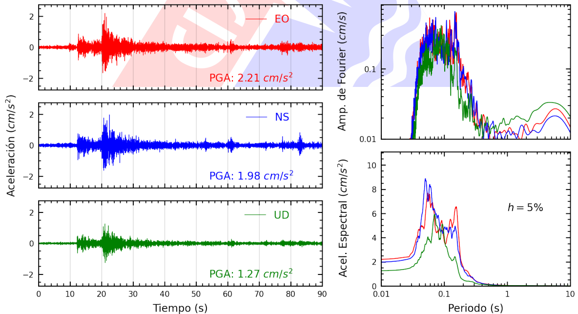
Figura A.6: Registros tiempo-historia, espectros de Fourier y de respuesta en las direcciones EO, NS y vertical de la estación USILM. Sismo de Provincia Constitucional del Callao , Callao - Lima del 2023-06-12, 06:20:30 (Hora local)
