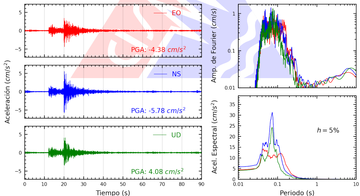
Figura A.2: Registros tiempo-historia, espectros de Fourier y de respuesta en las direcciones EO, NS y vertical de la estación SROSA. Sismo de Provincia Constitucional del Callao , Callao - Lima del 2023-06-12, 06:20:30 (Hora local)
