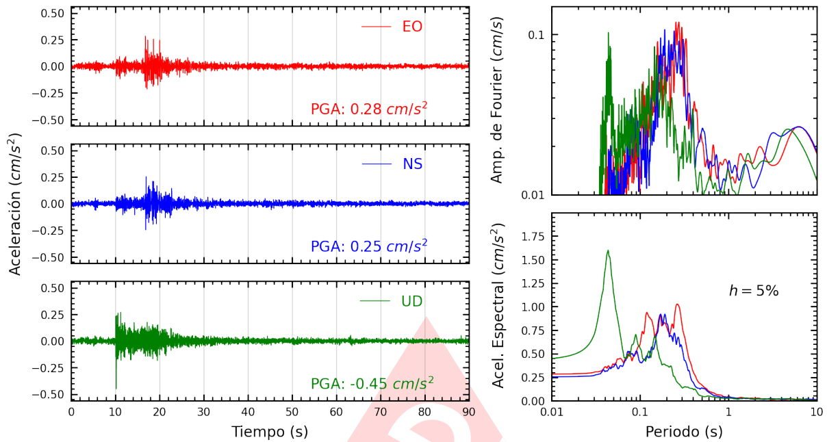
Figura A.29: Registros tiempo-historia, espectros de Fourier y de respuesta en las direcciones EO, NS y vertical de la estación DSMI. Sismo de Provincia Constitucional del Callao , Callao - Lima del 2023-06-12, 06:20:30 (Hora local)
