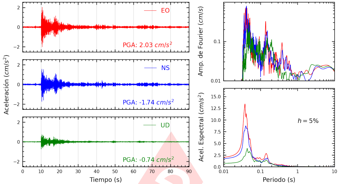
Figura A.7: Registros tiempo-historia, espectros de Fourier y de respuesta en las direcciones EO, NS y vertical de la estación DHNPE. Sismo de Provincia Constitucional del Callao , Callao - Lima del 2023-06-12, 06:20:30 (Hora local)
