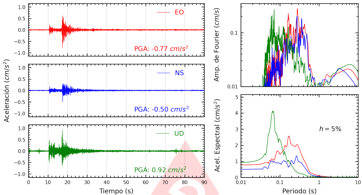
Figura A.19: Registros tiempo-historia, espectros de Fourier y de respuesta en las direcciones EO, NS y vertical de la estación ACAPU. Sismo de Provincia Constitucional del Callao , Callao - Lima del 2023-06-12, 06:20:30 (Hora local)
