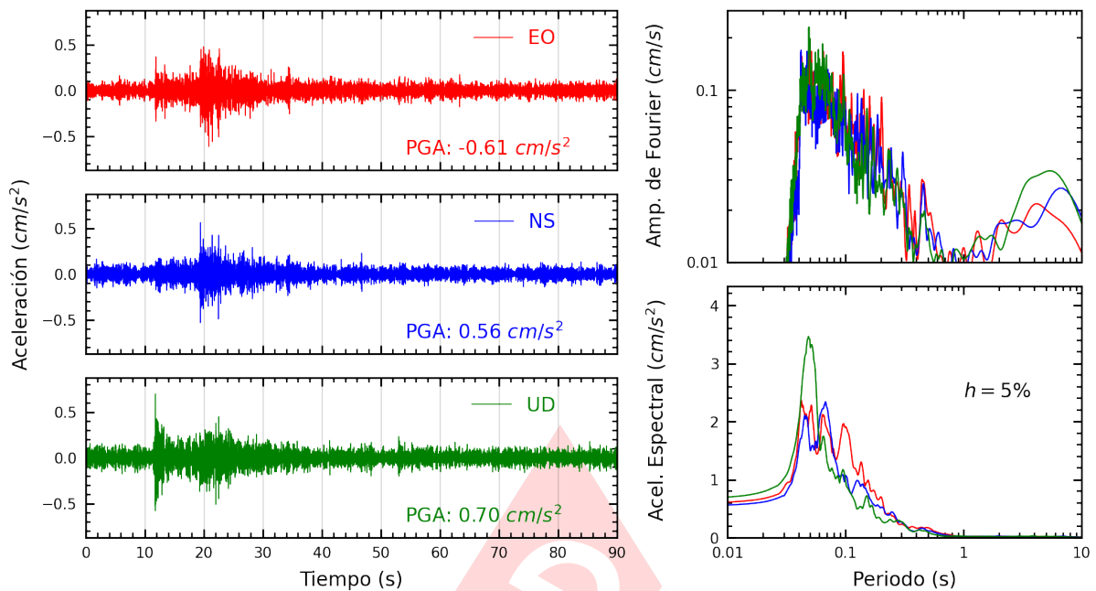
Figura A.23: Registros tiempo-historia, espectros de Fourier y de respuesta en las direcciones EO, NS y vertical de la estación URPE. Sismo de Provincia Constitucional del Callao , Callao - Lima del 2023-06-12, 06:20:30 (Hora local)
