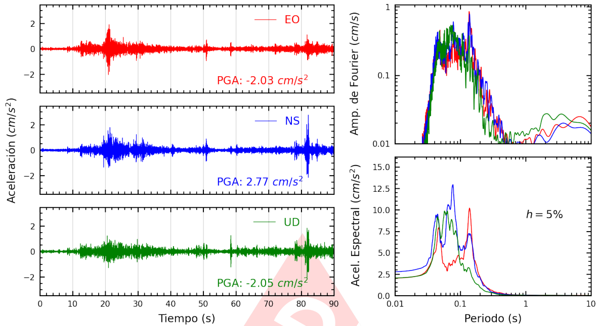
Figura A.3: Registros tiempo-historia, espectros de Fourier y de respuesta en las direcciones EO, NS y vertical de la estación CARAB. Sismo de Provincia Constitucional del Callao , Callao - Lima del 2023-06-12, 06:20:30 (Hora local)
