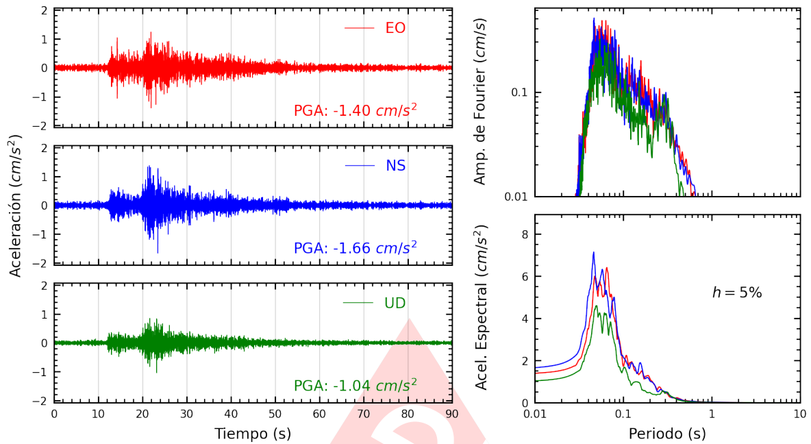
Figura A.11: Registros tiempo-historia, espectros de Fourier y de respuesta en las direcciones EO, NS y vertical de la estación UNTEL. Sismo de Provincia Constitucional del Callao , Callao - Lima del 2023-06-12, 06:20:30 (Hora local)
