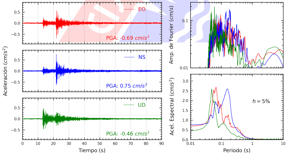
Figura A.22: Registros tiempo-historia, espectros de Fourier y de respuesta en las direcciones EO, NS y vertical de la estación USILP. Sismo de Provincia Constitucional del Callao , Callao - Lima del 2023-06-12, 06:20:30 (Hora local)
