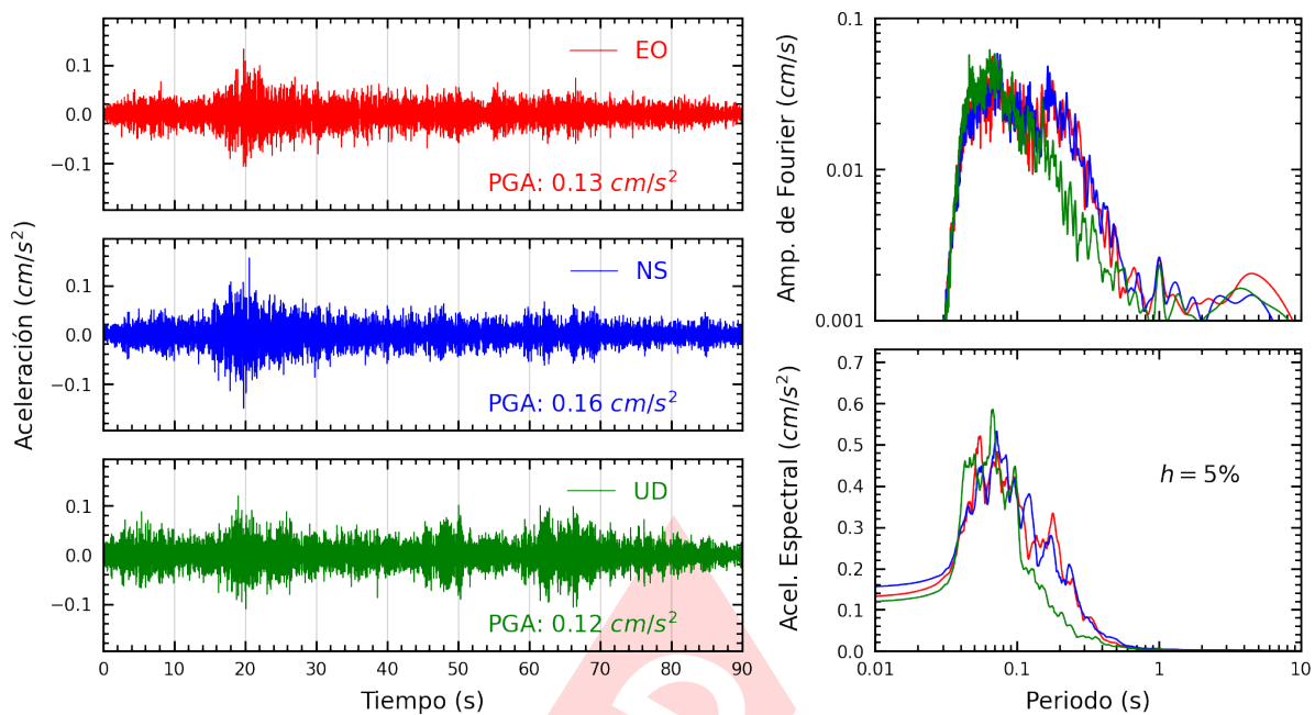
Figura A.33: Registros tiempo-historia, espectros de Fourier y de respuesta en las direcciones EO, NS y vertical de la estación ASIA. Sismo de Provincia Constitucional del Callao , Callao - Lima del 2023-06-12, 06:20:30 (Hora local)
