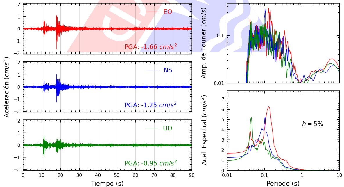
Figura A.10: Registros tiempo-historia, espectros de Fourier y de respuesta en las direcciones EO, NS y vertical de la estación MADRE. Sismo de Provincia Constitucional del Callao , Callao - Lima del 2023-06-12, 06:20:30 (Hora local)
