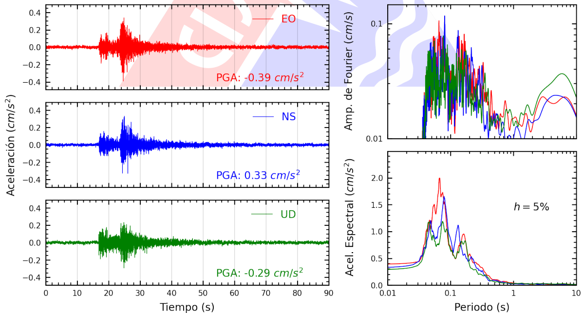
Figura A.32: Registros tiempo-historia, espectros de Fourier y de respuesta en las direcciones EO, NS y vertical de la estación UNMSM. Sismo de Provincia Constitucional del Callao , Callao - Lima del 2023-06-12, 06:20:30 (Hora local)
