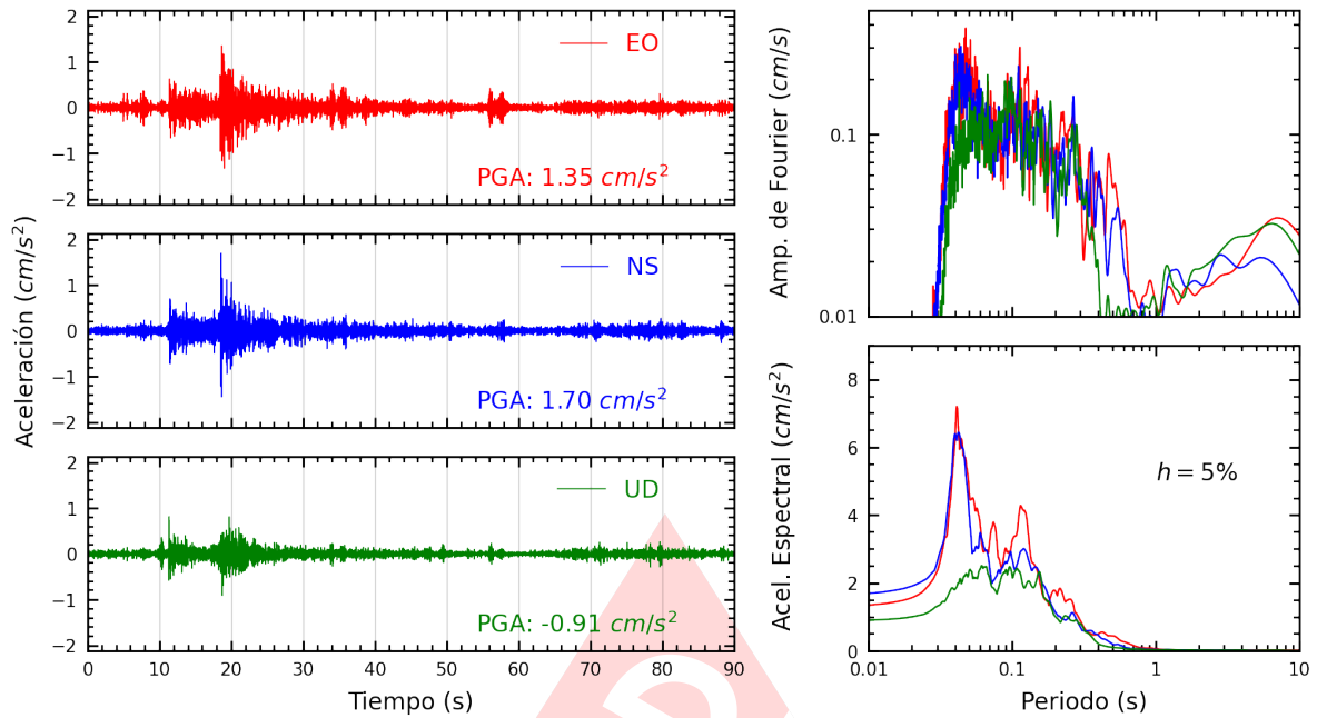
Figura A.9: Registros tiempo-historia, espectros de Fourier y de respuesta en las direcciones EO, NS y vertical de la estación OLIVO. Sismo de Provincia Constitucional del Callao , Callao - Lima del 2023-06-12, 06:20:30 (Hora local)
