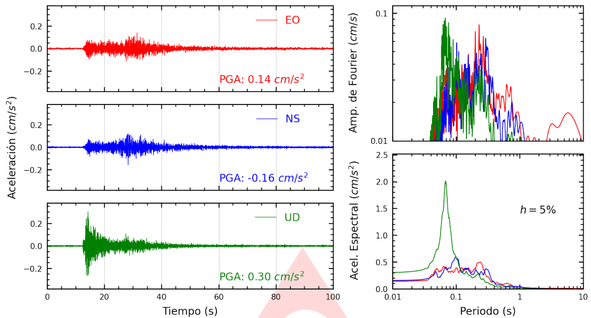
Figura A.1: Registros tiempo-historia, espectros de Fourier y de respuesta en las direcciones EO, NS y vertical de la estación SCCHI. Sismo de Sechura, Sechura - Piura del 2023-07-13, 14:33:12 (Hora local)
