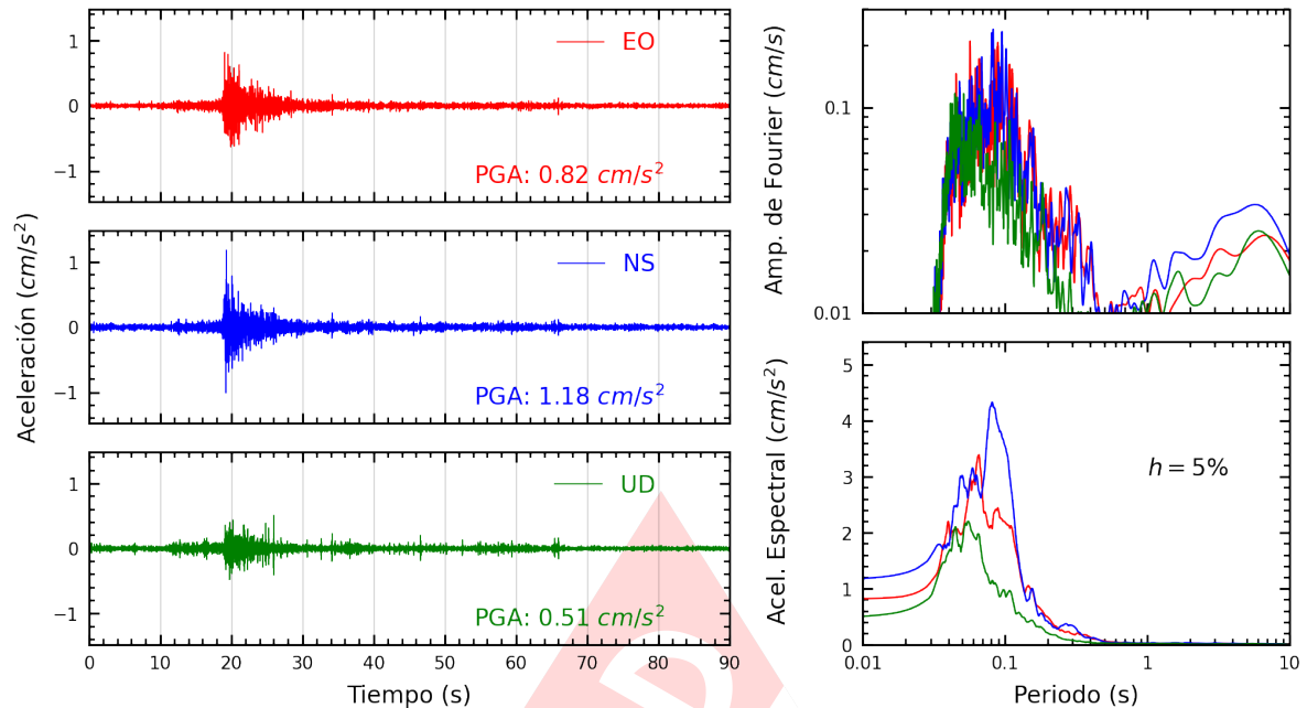
Figura A.3: Registros tiempo-historia, espectros de Fourier y de respuesta en las direcciones EO, NS y vertical de la estación DEFEN. Sismo de Ancon, Lima - Lima del 2023-07-13, 19:48:31 (Hora local)
