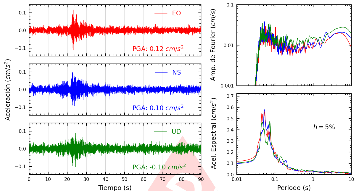
Figura A.17: Registros tiempo-historia, espectros de Fourier y de respuesta en las direcciones EO, NS y vertical de la estación UNFV. Sismo de Ancon, Lima - Lima del 2023-07-13, 19:48:31 (Hora local)
