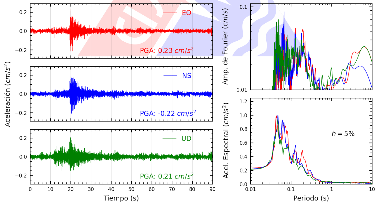
Figura A.14: Registros tiempo-historia, espectros de Fourier y de respuesta en las direcciones EO, NS y vertical de la estación VHAYA. Sismo de Ancon, Lima - Lima del 2023-07-13, 19:48:31 (Hora local)
