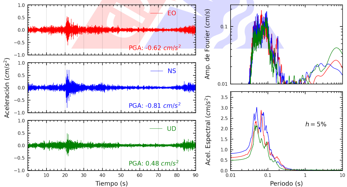
Figura A.4: Registros tiempo-historia, espectros de Fourier y de respuesta en las direcciones EO, NS y vertical de la estación INDEP. Sismo de Ancon, Lima - Lima del 2023-07-13, 19:48:31 (Hora local)
