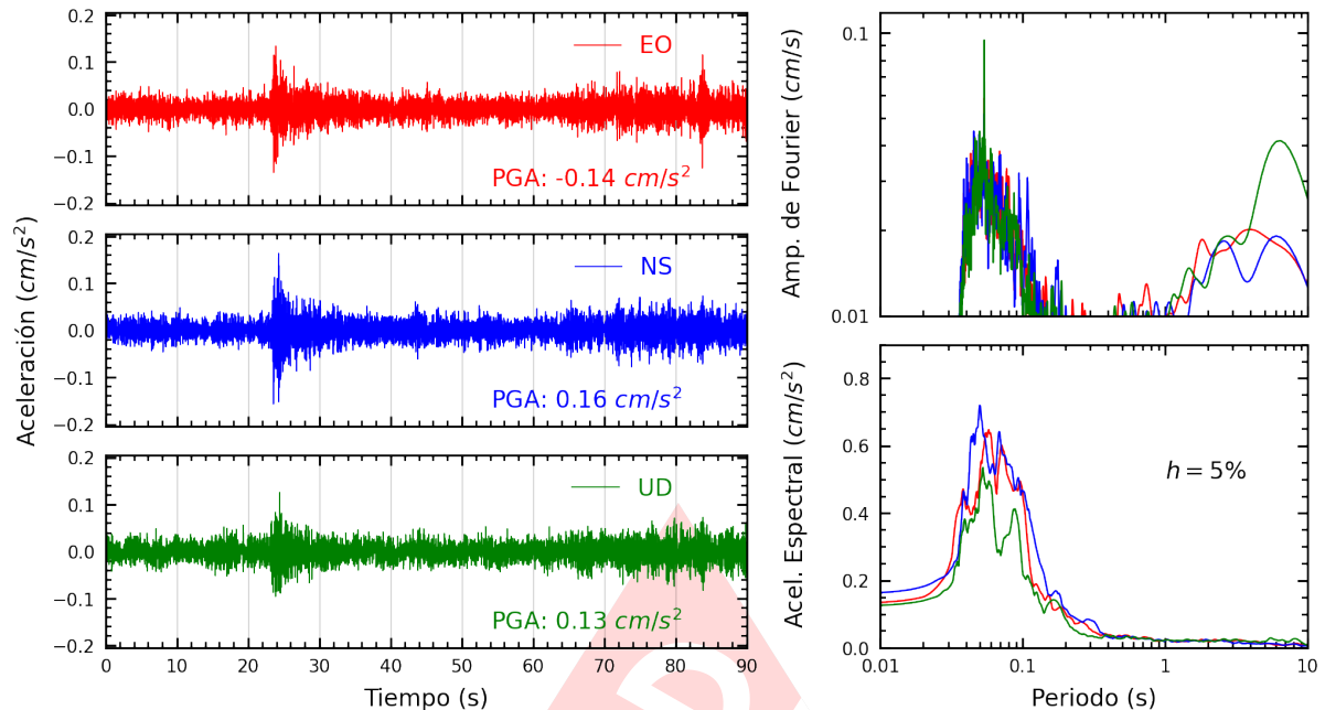
Figura A.15: Registros tiempo-historia, espectros de Fourier y de respuesta en las direcciones EO, NS y vertical de la estación SERVI. Sismo de Ancon, Lima - Lima del 2023-07-13, 19:48:31 (Hora local)
