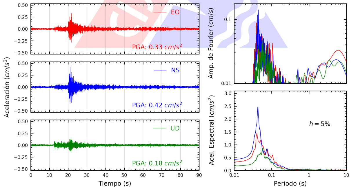
Figura A.8: Registros tiempo-historia, espectros de Fourier y de respuesta en las direcciones EO, NS y vertical de la estación COMAS. Sismo de Ancon, Lima - Lima del 2023-07-13, 19:48:31 (Hora local)
