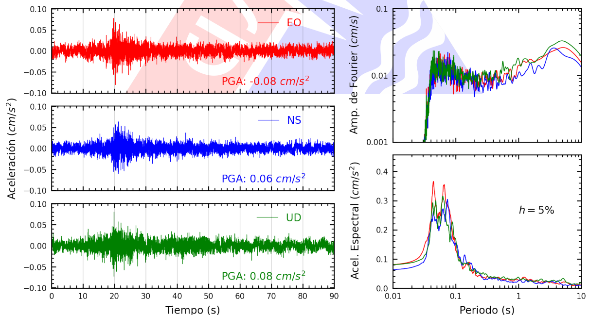
Figura A.18: Registros tiempo-historia, espectros de Fourier y de respuesta en las direcciones EO, NS y vertical de la estación UNMSM. Sismo de Ancon, Lima - Lima del 2023-07-13, 19:48:31 (Hora local)
