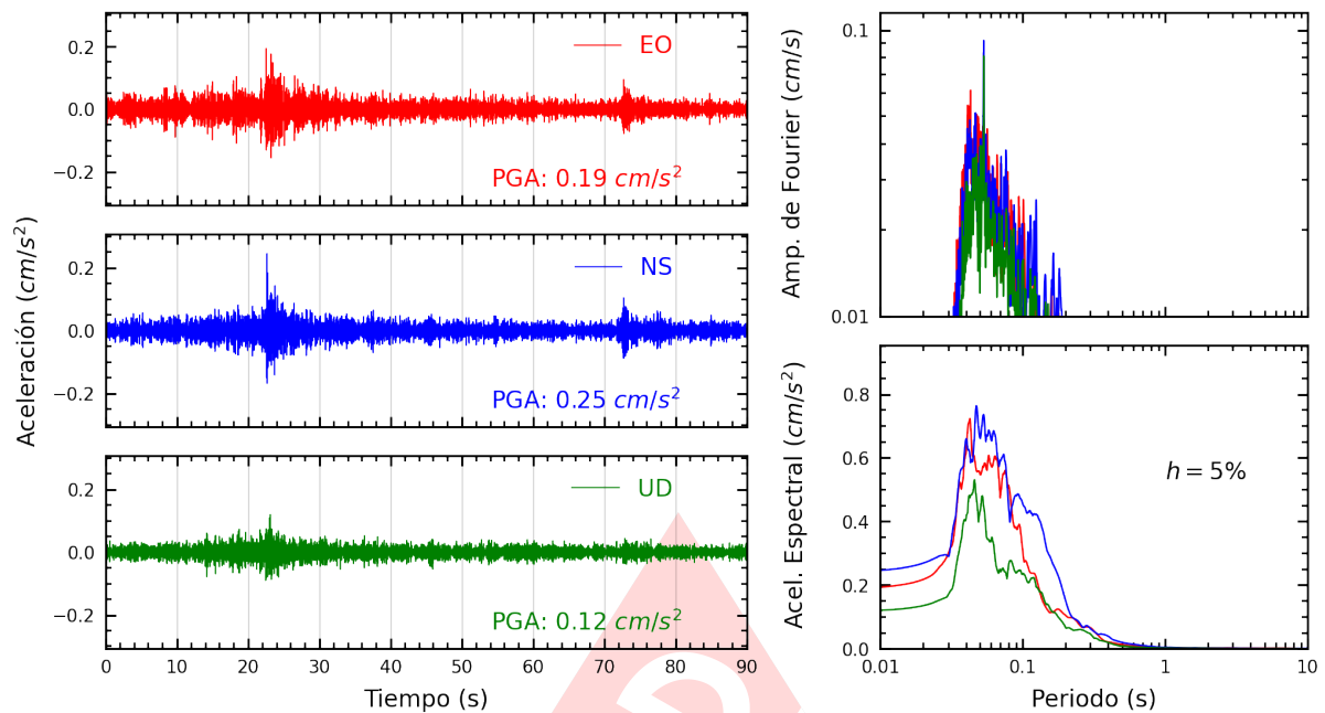
Figura A.13: Registros tiempo-historia, espectros de Fourier y de respuesta en las direcciones EO, NS y vertical de la estación BORJA. Sismo de Ancon, Lima - Lima del 2023-07-13, 19:48:31 (Hora local)
