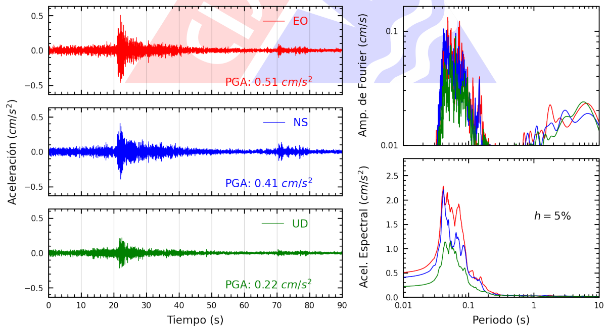
Figura A.6: Registros tiempo-historia, espectros de Fourier y de respuesta en las direcciones EO, NS y vertical de la estación FICPE. Sismo de Ancon, Lima - Lima del 2023-07-13, 19:48:31 (Hora local)
