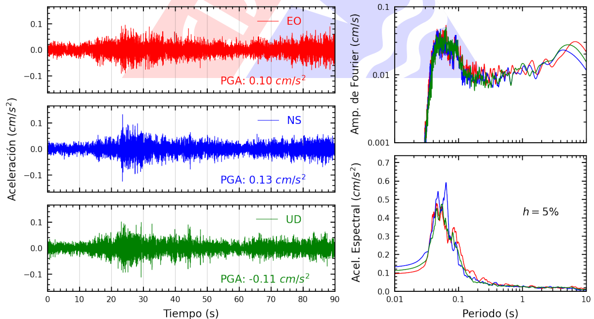
Figura A.16: Registros tiempo-historia, espectros de Fourier y de respuesta en las direcciones EO, NS y vertical de la estación IMCA. Sismo de Ancon, Lima - Lima del 2023-07-13, 19:48:31 (Hora local)
