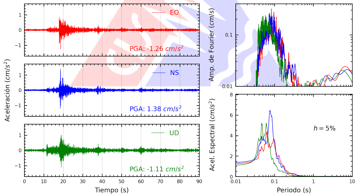
Figura A.2: Registros tiempo-historia, espectros de Fourier y de respuesta en las direcciones EO, NS y vertical de la estación ANCON. Sismo de Ancon, Lima - Lima del 2023-07-13, 19:48:31 (Hora local)
