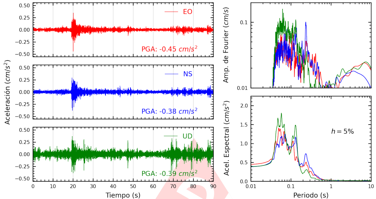
Figura A.7: Registros tiempo-historia, espectros de Fourier y de respuesta en las direcciones EO, NS y vertical de la estación MDPP. Sismo de Ancon, Lima - Lima del 2023-07-13, 19:48:31 (Hora local)
