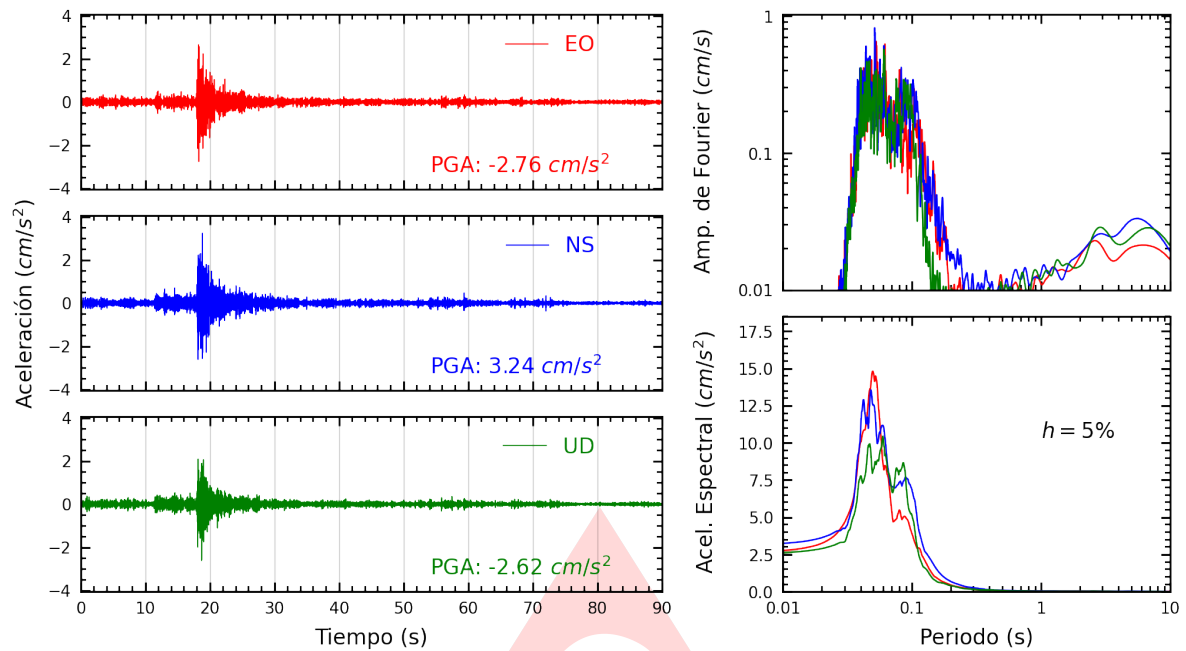
Figura A.1: Registros tiempo-historia, espectros de Fourier y de respuesta en las direcciones EO, NS y vertical de la estación SROSA. Sismo de Ancon, Lima - Lima del 2023-07-13, 19:48:31 (Hora local)
