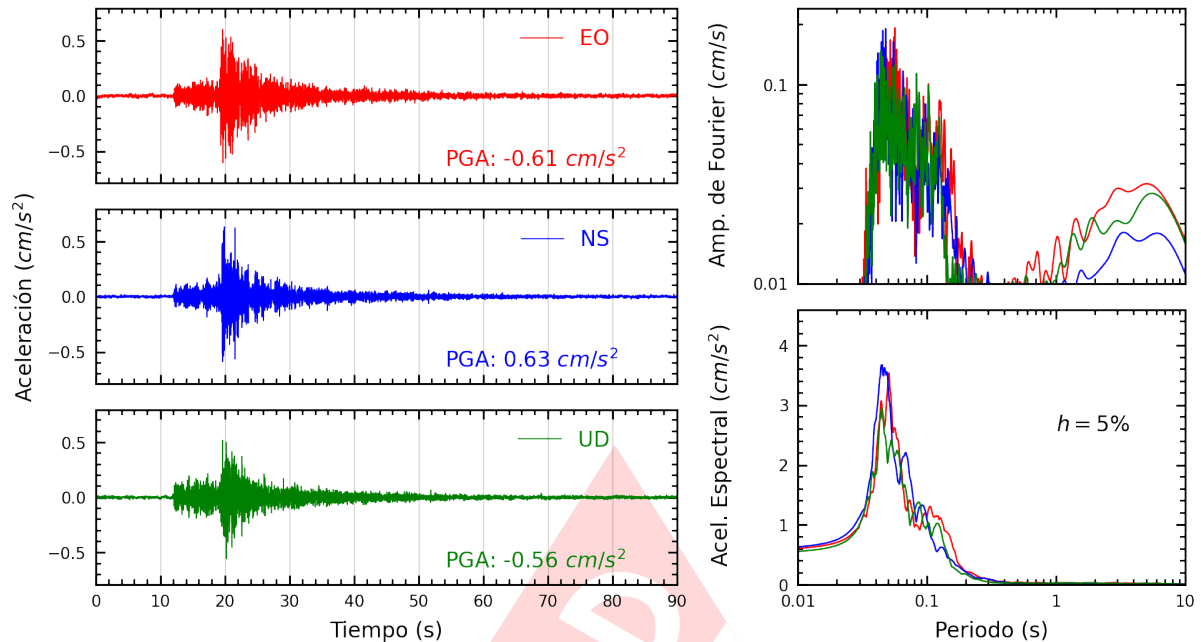
Figura A.5: Registros tiempo-historia, espectros de Fourier y de respuesta en las direcciones EO, NS y vertical de la estación AMORE. Sismo de Ancon, Lima - Lima del 2023-07-13, 19:48:31 (Hora local)
