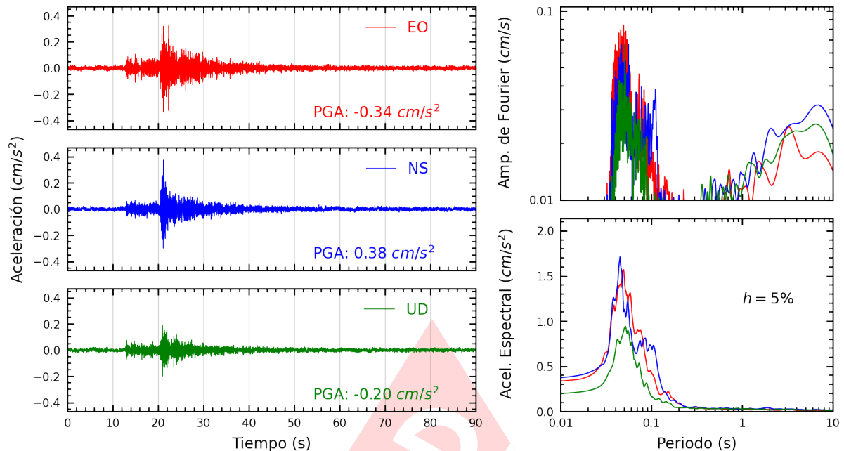
Figura A.9: Registros tiempo-historia, espectros de Fourier y de respuesta en las direcciones EO, NS y vertical de la estación UCSS. Sismo de Ancon, Lima - Lima del 2023-07-13, 19:48:31 (Hora local)
