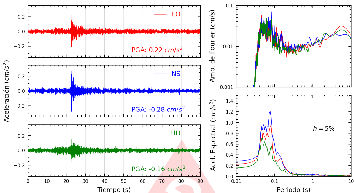
Figura A.11: Registros tiempo-historia, espectros de Fourier y de respuesta en las direcciones EO, NS y vertical de la estación CENEP. Sismo de Ancon, Lima - Lima del 2023-07-13, 19:48:31 (Hora local)
