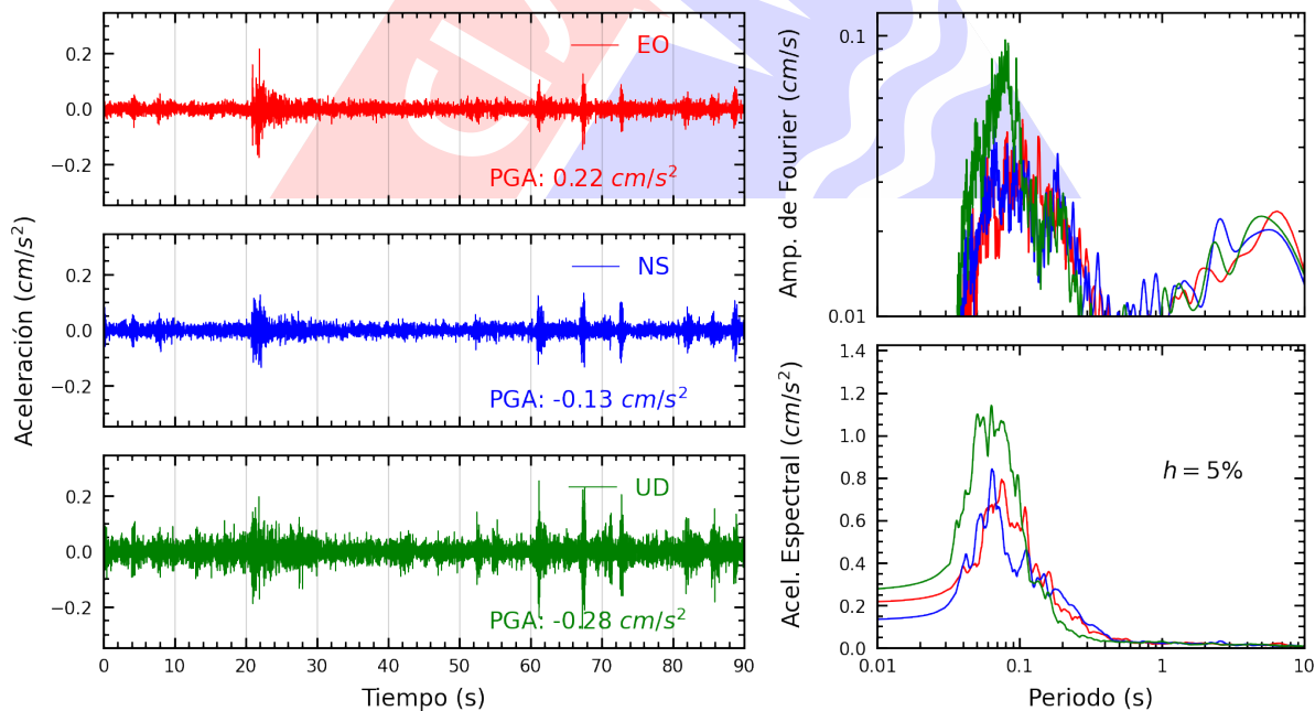
Figura A.12: Registros tiempo-historia, espectros de Fourier y de respuesta en las direcciones EO, NS y vertical de la estación RAMON. Sismo de Ancon, Lima - Lima del 2023-07-13, 19:48:31 (Hora local)
