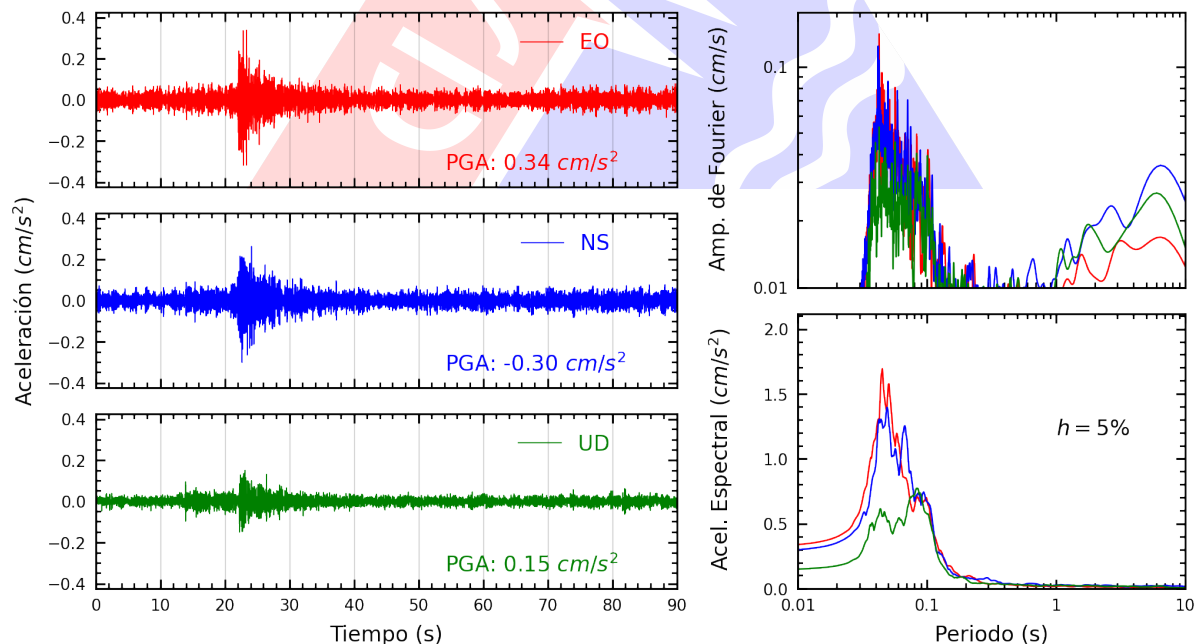
Figura A.10: Registros tiempo-historia, espectros de Fourier y de respuesta en las direcciones EO, NS y vertical de la estación CEPRE. Sismo de Ancon, Lima - Lima del 2023-07-13, 19:48:31 (Hora local)
