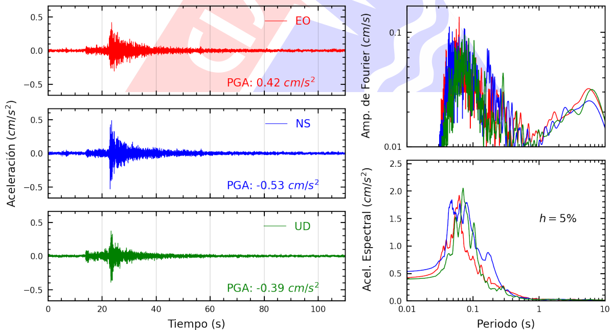
Figura A.16: Registros tiempo-historia, espectros de Fourier y de respuesta en las direcciones EO, NS y vertical de la estación COMAS. Sismo de Ancon, Lima - Lima del 2023-07-20, 23:08:50 (Hora local)
