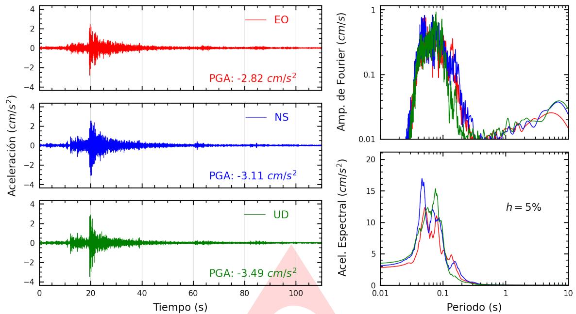
Figura A.1: Registros tiempo-historia, espectros de Fourier y de respuesta en las direcciones EO, NS y vertical de la estación SROSA. Sismo de Ancon, Lima - Lima del 2023-07-20, 23:08:50 (Hora local)
