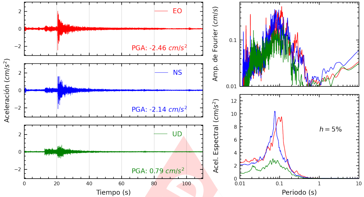
Figura A.3: Registros tiempo-historia, espectros de Fourier y de respuesta en las direcciones EO, NS y vertical de la estación DEFEN. Sismo de Ancon, Lima - Lima del 2023-07-20, 23:08:50 (Hora local)
