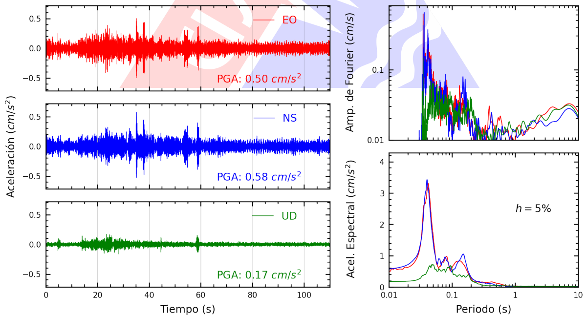
Figura A.14: Registros tiempo-historia, espectros de Fourier y de respuesta en las direcciones EO, NS y vertical de la estación DHNPE. Sismo de Ancon, Lima - Lima del 2023-07-20, 23:08:50 (Hora local)
