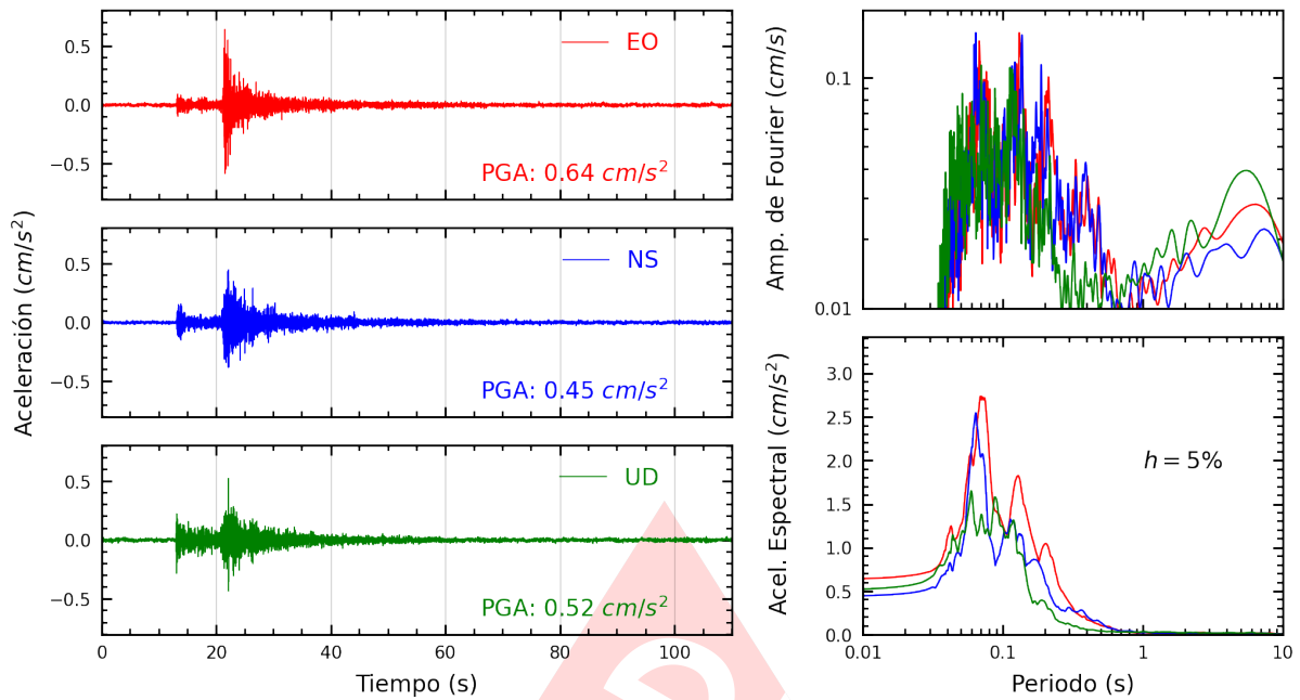
Figura A.11: Registros tiempo-historia, espectros de Fourier y de respuesta en las direcciones EO, NS y vertical de la estación VHAYA. Sismo de Ancon, Lima - Lima del 2023-07-20, 23:08:50 (Hora local)
