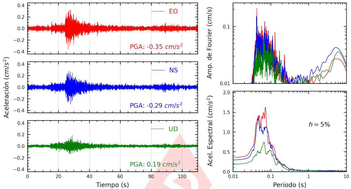
Figura A.21: Registros tiempo-historia, espectros de Fourier y de respuesta en las direcciones EO, NS y vertical de la estación CEPRE. Sismo de Ancon, Lima - Lima del 2023-07-20, 23:08:50 (Hora local)
