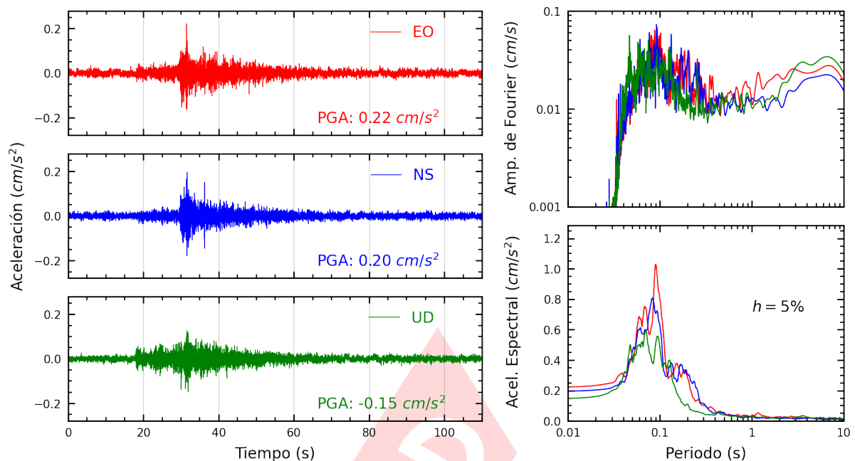
Figura A.29: Registros tiempo-historia, espectros de Fourier y de respuesta en las direcciones EO, NS y vertical de la estación USILP. Sismo de Ancon, Lima - Lima del 2023-07-20, 23:08:50 (Hora local)
