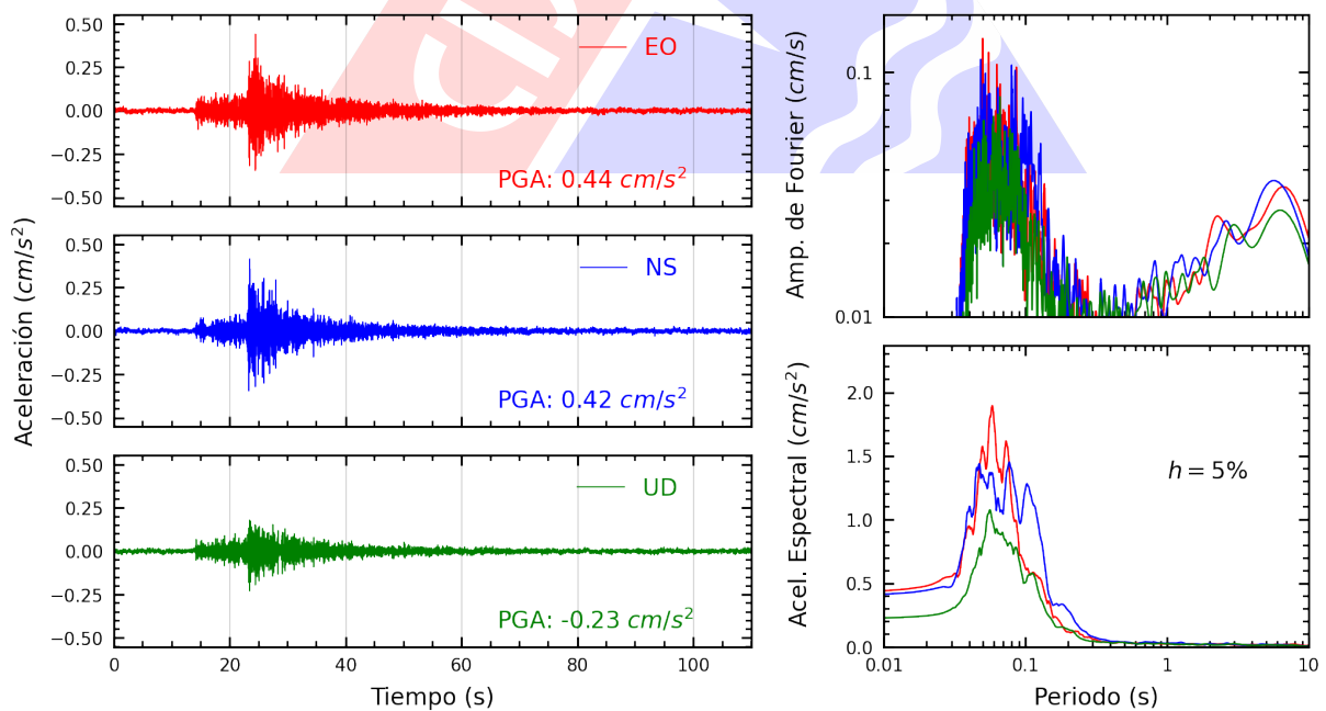
Figura A.18: Registros tiempo-historia, espectros de Fourier y de respuesta en las direcciones EO, NS y vertical de la estación UCSS. Sismo de Ancon, Lima - Lima del 2023-07-20, 23:08:50 (Hora local)
