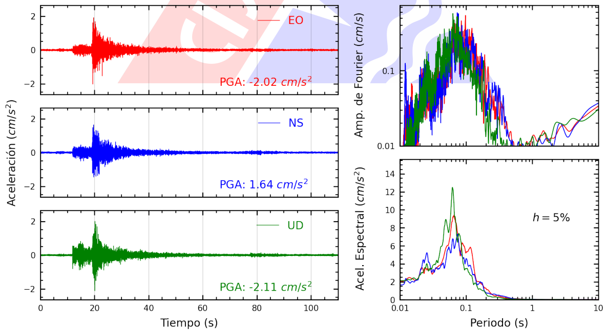
Figura A.4: Registros tiempo-historia, espectros de Fourier y de respuesta en las direcciones EO, NS y vertical de la estación ANCON. Sismo de Ancon, Lima - Lima del 2023-07-20, 23:08:50 (Hora local)
