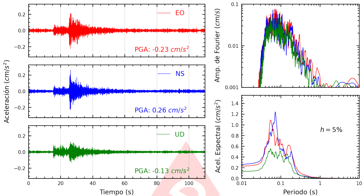
Figura A.27: Registros tiempo-historia, espectros de Fourier y de respuesta en las direcciones EO, NS y vertical de la estación BORJA. Sismo de Ancon, Lima - Lima del 2023-07-20, 23:08:50 (Hora local)
