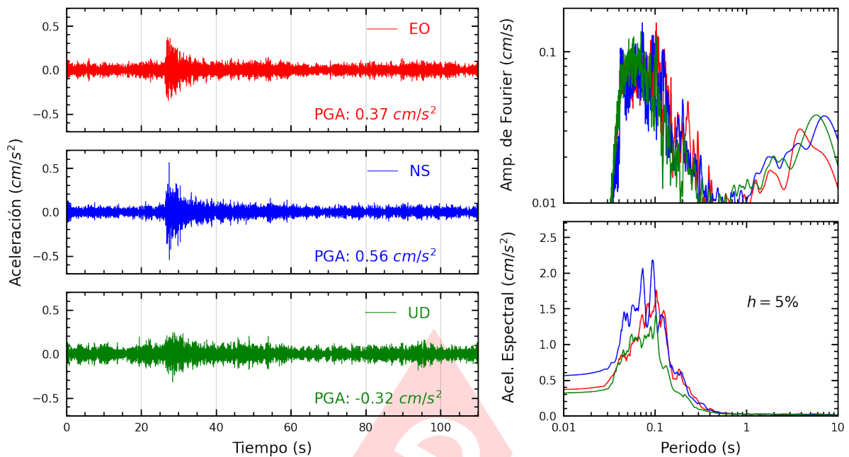
Figura A.15: Registros tiempo-historia, espectros de Fourier y de respuesta en las direcciones EO, NS y vertical de la estación URPE. Sismo de Ancon, Lima - Lima del 2023-07-20, 23:08:50 (Hora local)
