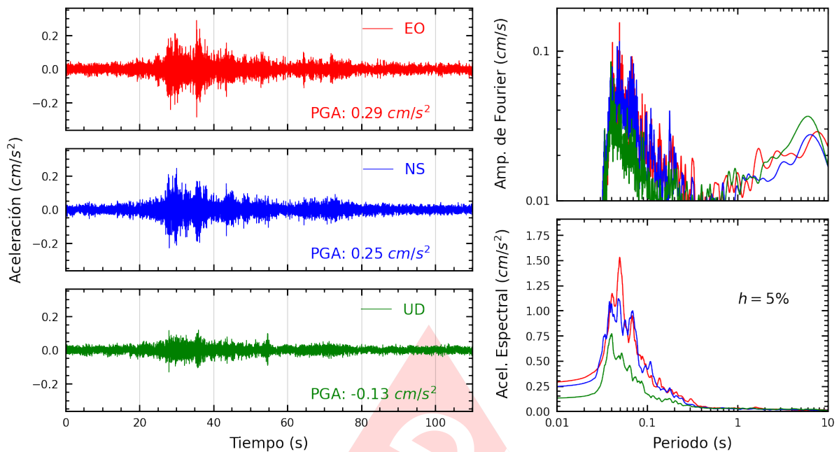
Figura A.25: Registros tiempo-historia, espectros de Fourier y de respuesta en las direcciones EO, NS y vertical de la estación UPCVI. Sismo de Ancon, Lima - Lima del 2023-07-20, 23:08:50 (Hora local)
