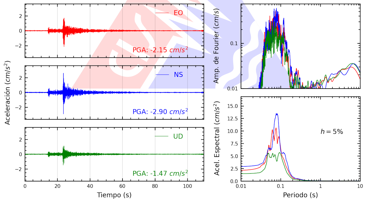
Figura A.2: Registros tiempo-historia, espectros de Fourier y de respuesta en las direcciones EO, NS y vertical de la estación JOSEO. Sismo de Ancon, Lima - Lima del 2023-07-20, 23:08:50 (Hora local)
