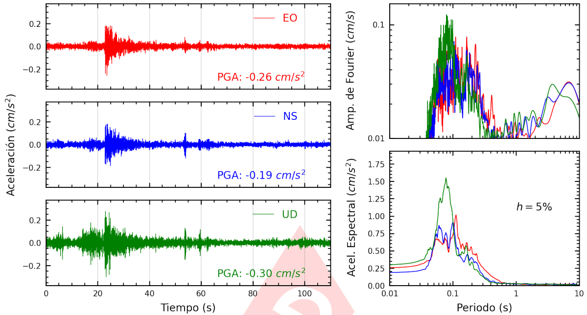
Figura A.23: Registros tiempo-historia, espectros de Fourier y de respuesta en las direcciones EO, NS y vertical de la estación RAMON. Sismo de Ancon, Lima - Lima del 2023-07-20, 23:08:50 (Hora local)
