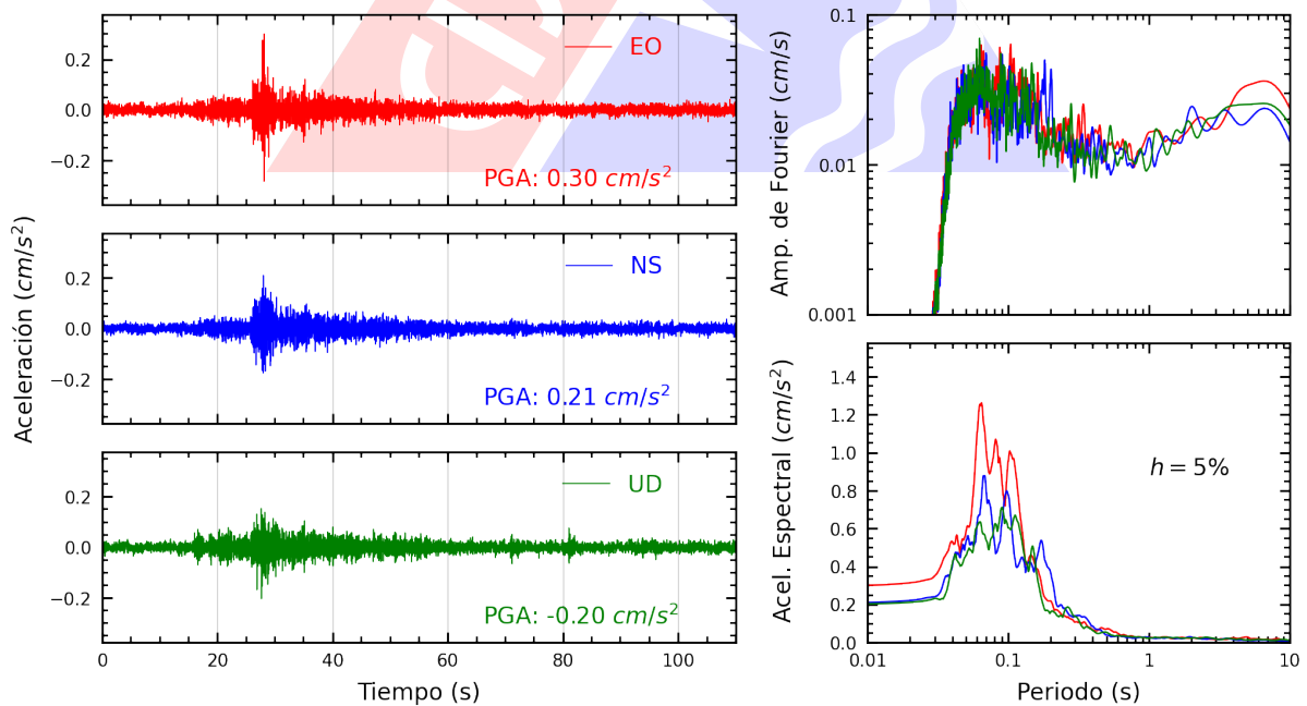
Figura A.22: Registros tiempo-historia, espectros de Fourier y de respuesta en las direcciones EO, NS y vertical de la estación IMCA. Sismo de Ancon, Lima - Lima del 2023-07-20, 23:08:50 (Hora local)
