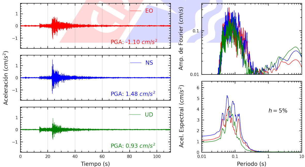
Figura A.6: Registros tiempo-historia, espectros de Fourier y de respuesta en las direcciones EO, NS y vertical de la estación INDEP. Sismo de Ancon, Lima - Lima del 2023-07-20, 23:08:50 (Hora local)
