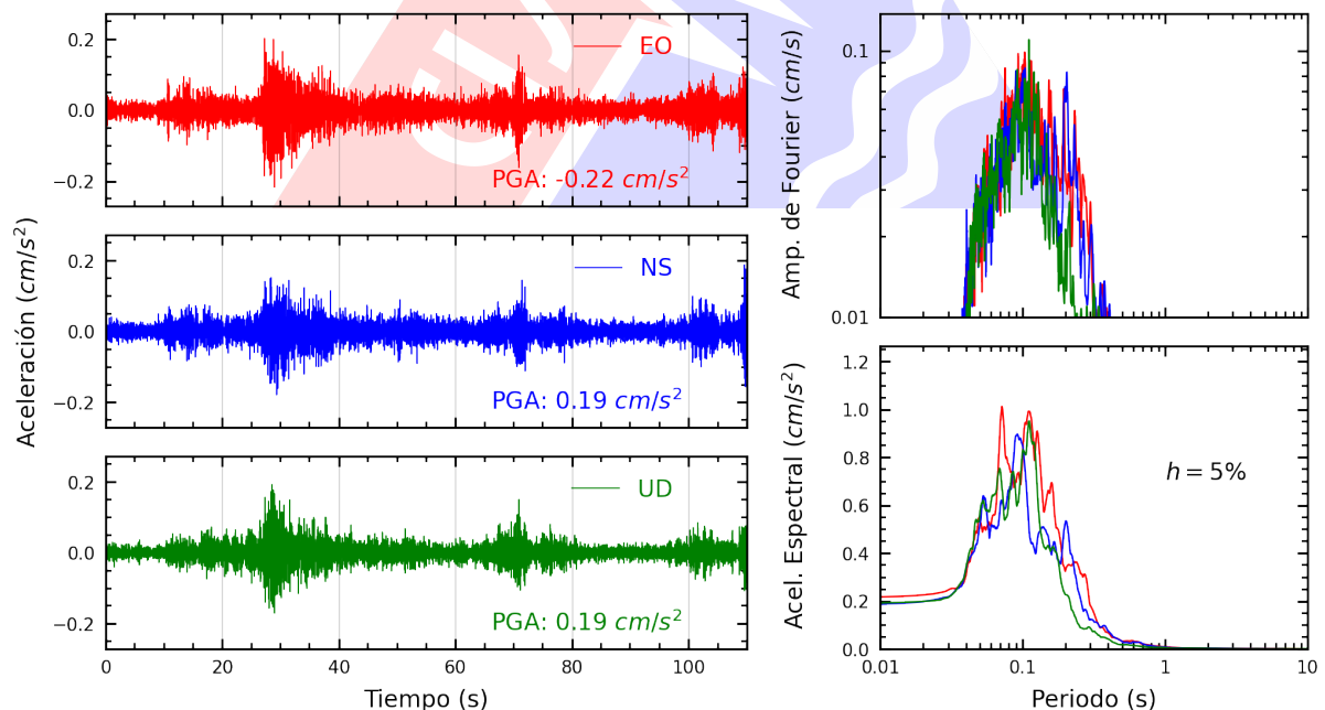
Figura A.30: Registros tiempo-historia, espectros de Fourier y de respuesta en las direcciones EO, NS y vertical de la estación SCCHO. Sismo de Ancon, Lima - Lima del 2023-07-20, 23:08:50 (Hora local)
