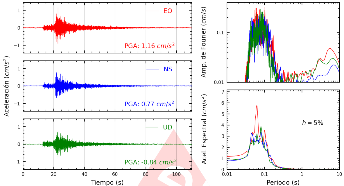
Figura A.7: Registros tiempo-historia, espectros de Fourier y de respuesta en las direcciones EO, NS y vertical de la estación AMORE. Sismo de Ancon, Lima - Lima del 2023-07-20, 23:08:50 (Hora local)
