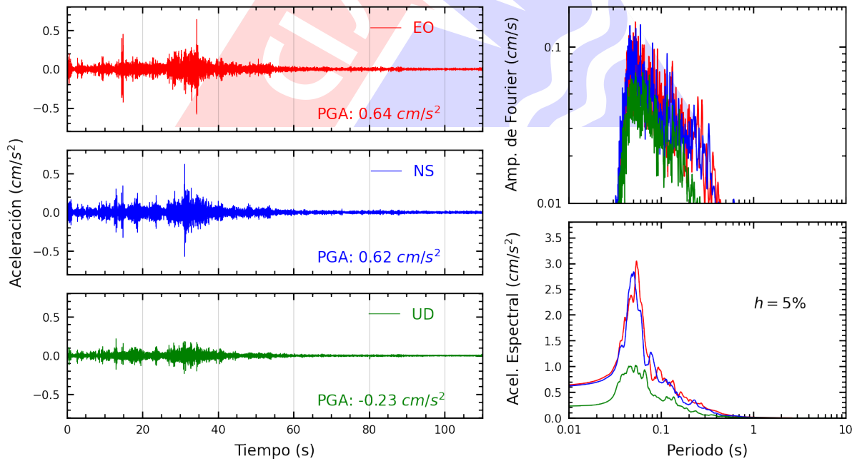
Figura A.12: Registros tiempo-historia, espectros de Fourier y de respuesta en las direcciones EO, NS y vertical de la estación BRISA. Sismo de Ancon, Lima - Lima del 2023-07-20, 23:08:50 (Hora local)
