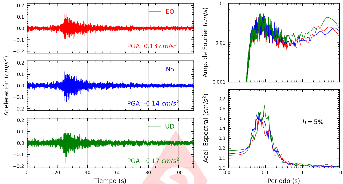
Figura A.31: Registros tiempo-historia, espectros de Fourier y de respuesta en las direcciones EO, NS y vertical de la estación UNFV. Sismo de Ancon, Lima - Lima del 2023-07-20, 23:08:50 (Hora local)
