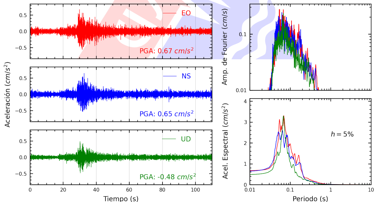
Figura A.10: Registros tiempo-historia, espectros de Fourier y de respuesta en las direcciones EO, NS y vertical de la estación UNTEL. Sismo de Ancon, Lima - Lima del 2023-07-20, 23:08:50 (Hora local)
