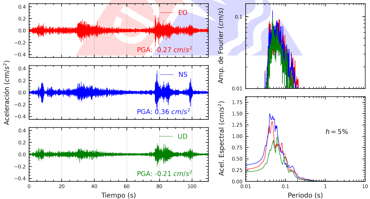
Figura A.20: Registros tiempo-historia, espectros de Fourier y de respuesta en las direcciones EO, NS y vertical de la estación PACHA. Sismo de Ancon, Lima - Lima del 2023-07-20, 23:08:50 (Hora local)
