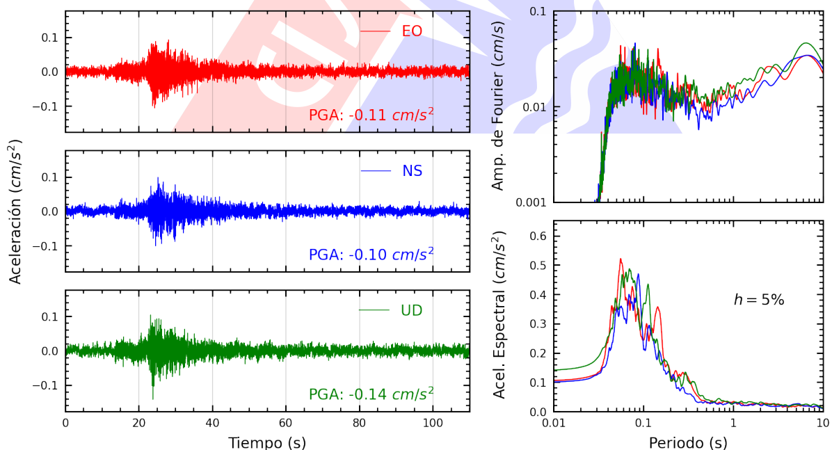
Figura A.32: Registros tiempo-historia, espectros de Fourier y de respuesta en las direcciones EO, NS y vertical de la estación UNMSM. Sismo de Ancon, Lima - Lima del 2023-07-20, 23:08:50 (Hora local)
