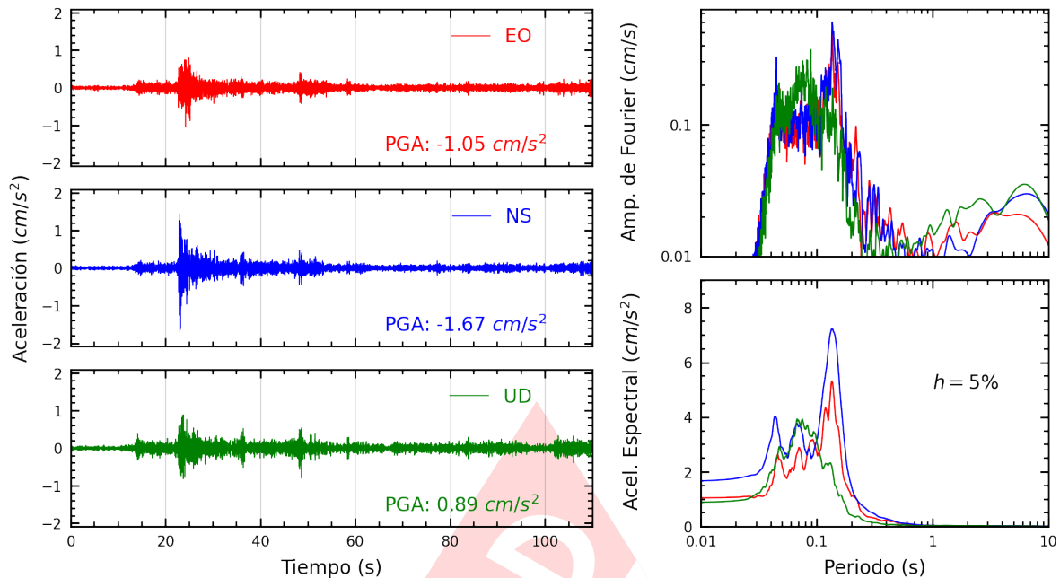
Figura A.5: Registros tiempo-historia, espectros de Fourier y de respuesta en las direcciones EO, NS y vertical de la estación CARAB. Sismo de Ancon, Lima - Lima del 2023-07-20, 23:08:50 (Hora local)
