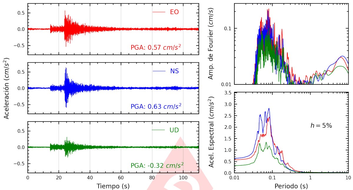
Figura A.13: Registros tiempo-historia, espectros de Fourier y de respuesta en las direcciones EO, NS y vertical de la estación FICPE. Sismo de Ancon, Lima - Lima del 2023-07-20, 23:08:50 (Hora local)
