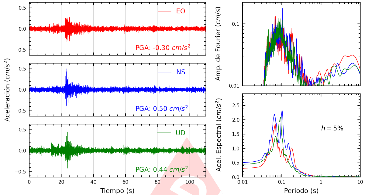
Figura A.17: Registros tiempo-historia, espectros de Fourier y de respuesta en las direcciones EO, NS y vertical de la estación MADRE. Sismo de Ancon, Lima - Lima del 2023-07-20, 23:08:50 (Hora local)
