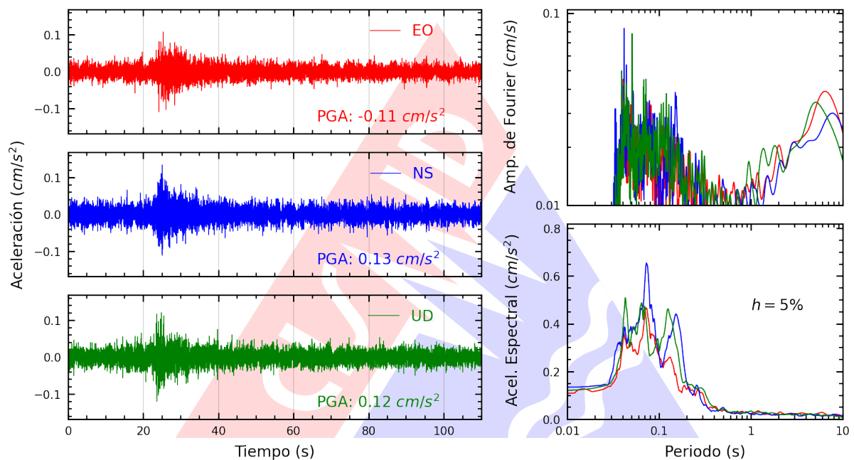
Figura A.33: Registros tiempo-historia, espectros de Fourier y de respuesta en las direcciones EO, NS y vertical de la estación BONDY. Sismo de Ancon, Lima - Lima del 2023-07-20, 23:08:50 (Hora local)
