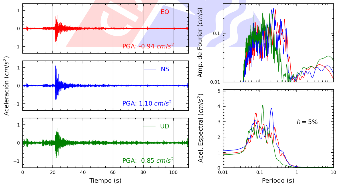
Figura A.8: Registros tiempo-historia, espectros de Fourier y de respuesta en las direcciones EO, NS y vertical de la estación MDPP. Sismo de Ancon, Lima - Lima del 2023-07-20, 23:08:50 (Hora local)
