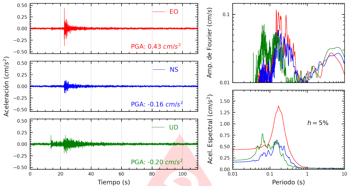
Figura A.19: Registros tiempo-historia, espectros de Fourier y de respuesta en las direcciones EO, NS y vertical de la estación ACAPU. Sismo de Ancon, Lima - Lima del 2023-07-20, 23:08:50 (Hora local)
