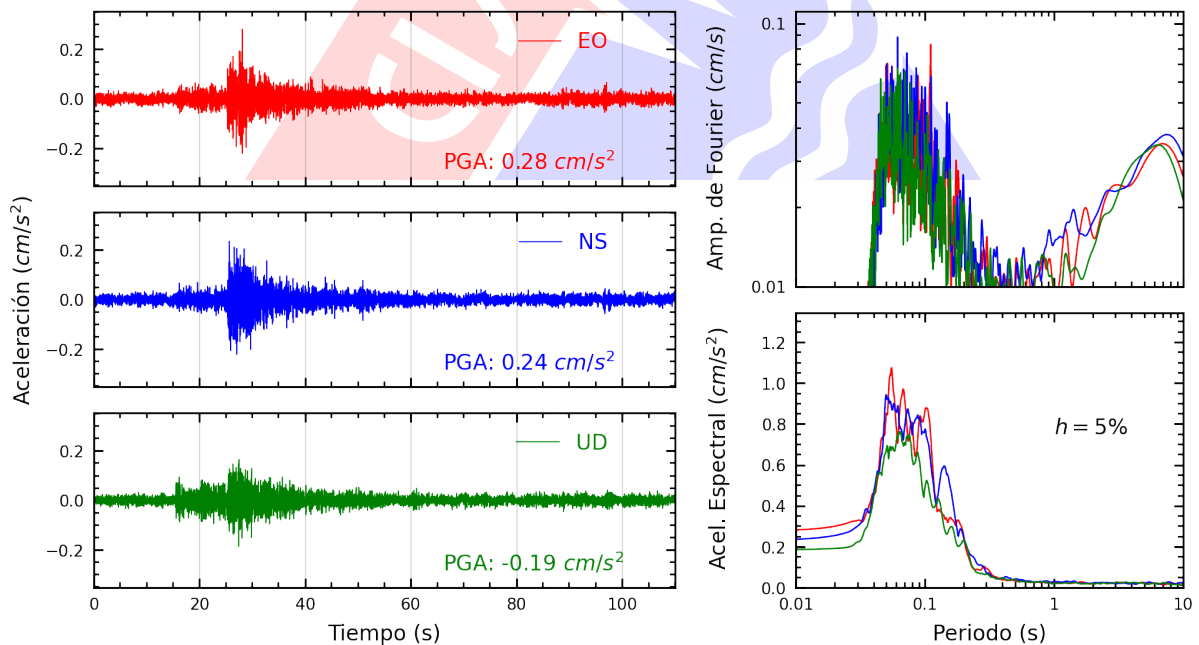
Figura A.26: Registros tiempo-historia, espectros de Fourier y de respuesta en las direcciones EO, NS y vertical de la estación CENEP. Sismo de Ancon, Lima - Lima del 2023-07-20, 23:08:50 (Hora local)
