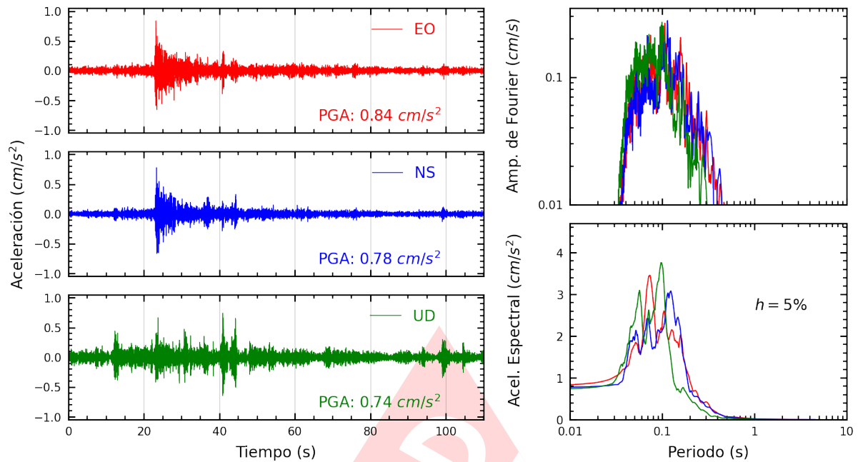
Figura A.9: Registros tiempo-historia, espectros de Fourier y de respuesta en las direcciones EO, NS y vertical de la estación SCOLI. Sismo de Ancon, Lima - Lima del 2023-07-20, 23:08:50 (Hora local)
