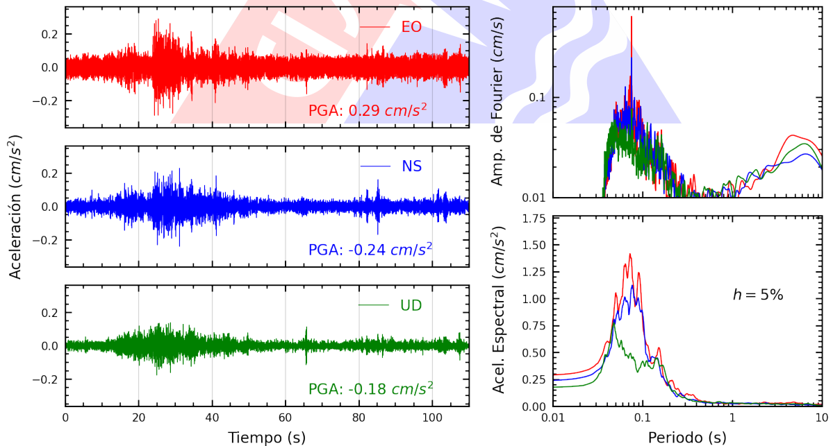
Figura A.24: Registros tiempo-historia, espectros de Fourier y de respuesta en las direcciones EO, NS y vertical de la estación UPCSM. Sismo de Ancon, Lima - Lima del 2023-07-20, 23:08:50 (Hora local)
