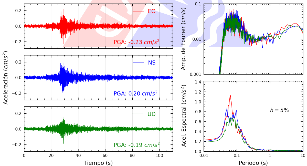
Figura A.28: Registros tiempo-historia, espectros de Fourier y de respuesta en las direcciones EO, NS y vertical de la estación SERVI. Sismo de Ancon, Lima - Lima del 2023-07-20, 23:08:50 (Hora local)
