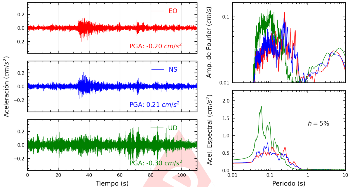
Figura A.5: Registros tiempo-historia, espectros de Fourier y de respuesta en las direcciones EO, NS y vertical de la estación MDPP. Sismo de Cajacay, Bolognesi - Ancash del 2023-07-23, 16:17:22 (Hora local)
