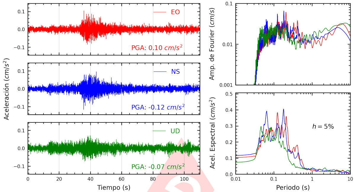
Figura A.9: Registros tiempo-historia, espectros de Fourier y de respuesta en las direcciones EO, NS y vertical de la estación VHAYA. Sismo de Cajacay, Bolognesi - Ancash del 2023-07-23, 16:17:22 (Hora local)
