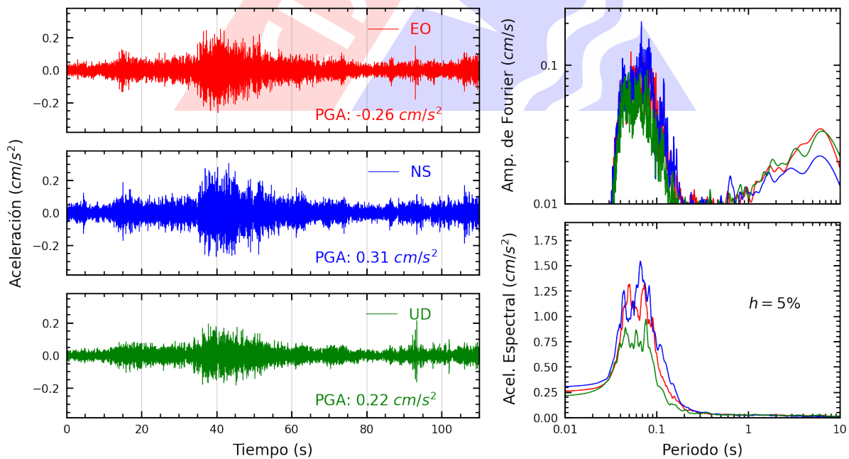
Figura A.4: Registros tiempo-historia, espectros de Fourier y de respuesta en las direcciones EO, NS y vertical de la estación JOSEO. Sismo de Cajacay, Bolognesi - Ancash del 2023-07-23, 16:17:22 (Hora local)
