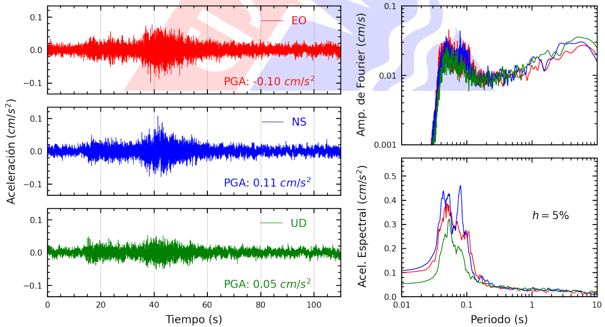
Figura A.10: Registros tiempo-historia, espectros de Fourier y de respuesta en las direcciones EO, NS y vertical de la estación UCSS. Sismo de Cajacay, Bolognesi - Ancash del 2023-07-23, 16:17:22 (Hora local)
