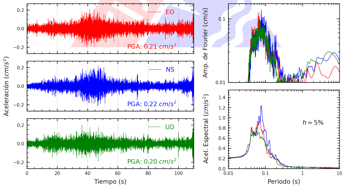
Figura A.6: Registros tiempo-historia, espectros de Fourier y de respuesta en las direcciones EO, NS y vertical de la estación INDEP. Sismo de Cajacay, Bolognesi - Ancash del 2023-07-23, 16:17:22 (Hora local)
