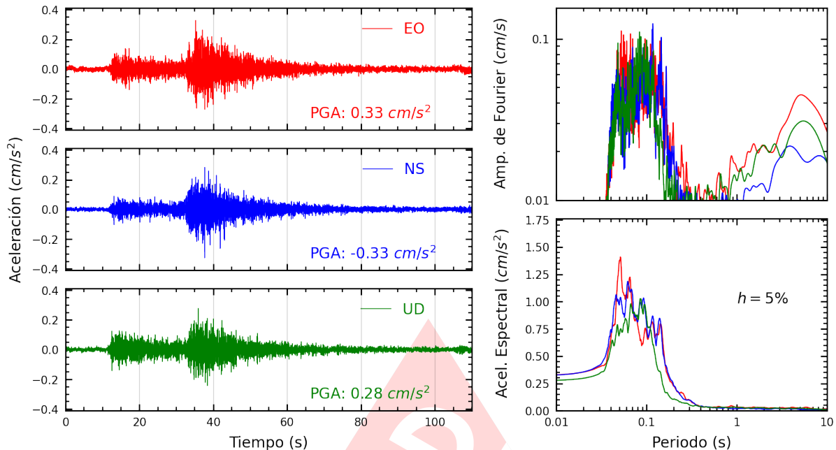
Figura A.3: Registros tiempo-historia, espectros de Fourier y de respuesta en las direcciones EO, NS y vertical de la estación AMORE. Sismo de Cajacay, Bolognesi - Ancash del 2023-07-23, 16:17:22 (Hora local)
