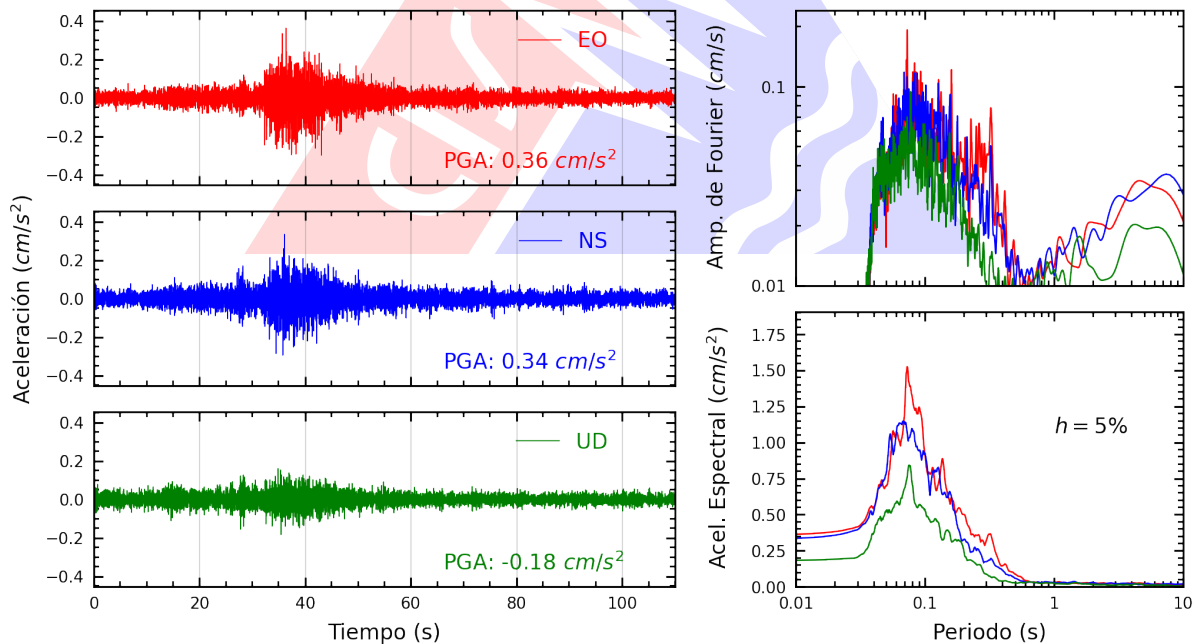
Figura A.2: Registros tiempo-historia, espectros de Fourier y de respuesta en las direcciones EO, NS y vertical de la estación DEFEN. Sismo de Cajacay, Bolognesi - Ancash del 2023-07-23, 16:17:22 (Hora local)
