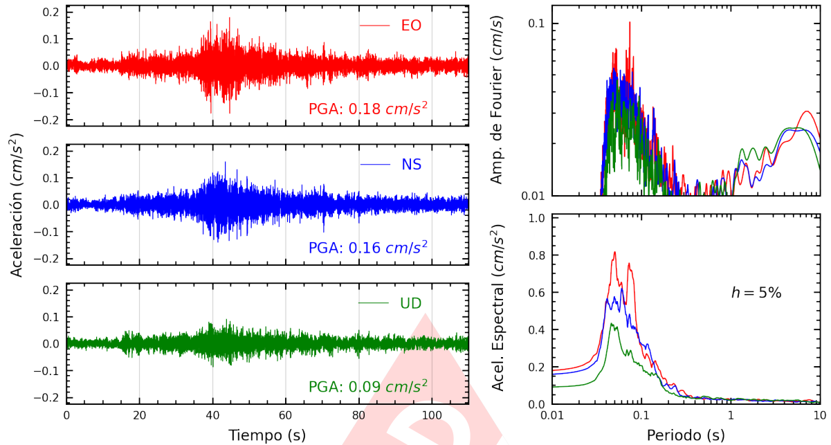
Figura A.7: Registros tiempo-historia, espectros de Fourier y de respuesta en las direcciones EO, NS y vertical de la estación FICPE. Sismo de Cajacay, Bolognesi - Ancash del 2023-07-23, 16:17:22 (Hora local)
