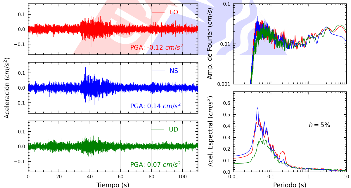
Figura A.8: Registros tiempo-historia, espectros de Fourier y de respuesta en las direcciones EO, NS y vertical de la estación COMAS. Sismo de Cajacay, Bolognesi - Ancash del 2023-07-23, 16:17:22 (Hora local)
