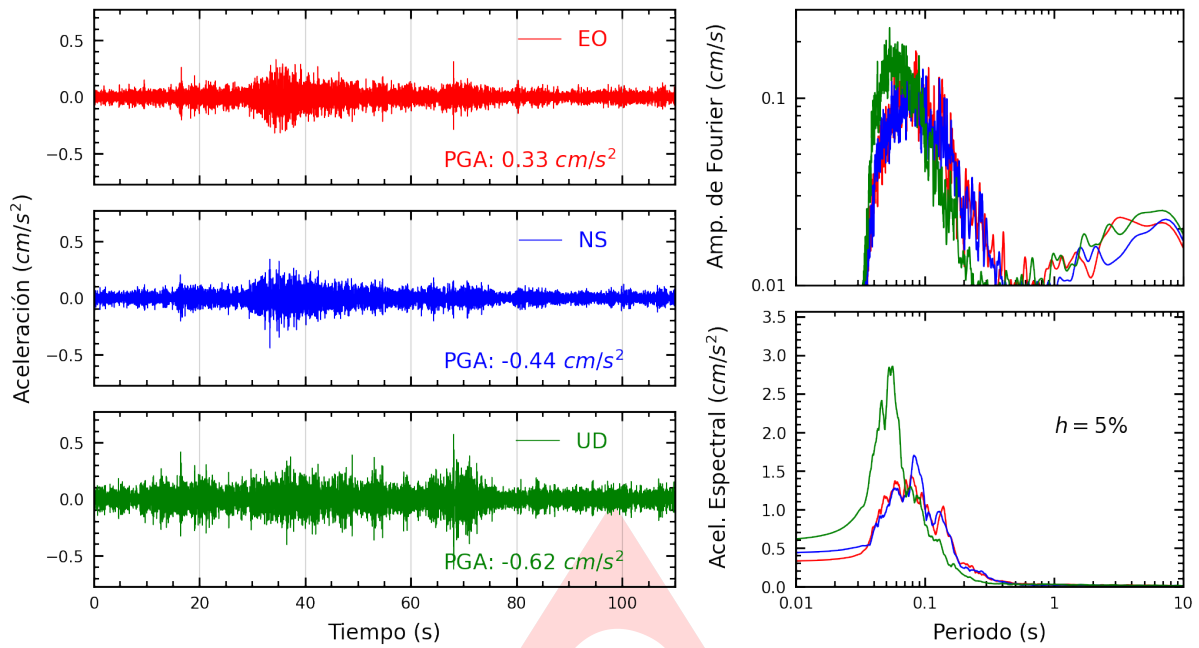
Figura A.1: Registros tiempo-historia, espectros de Fourier y de respuesta en las direcciones EO, NS y vertical de la estación ANCON. Sismo de Cajacay, Bolognesi - Ancash del 2023-07-23, 16:17:22 (Hora local)
