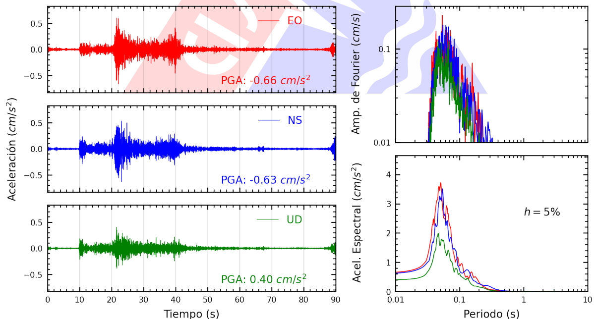
Figura A.26: Registros tiempo-historia, espectros de Fourier y de respuesta en las direcciones EO, NS y vertical de la estación PACHA. Sismo de Ancon, Lima - Lima del 2023-08-03, 01:47:23 (Hora local)
