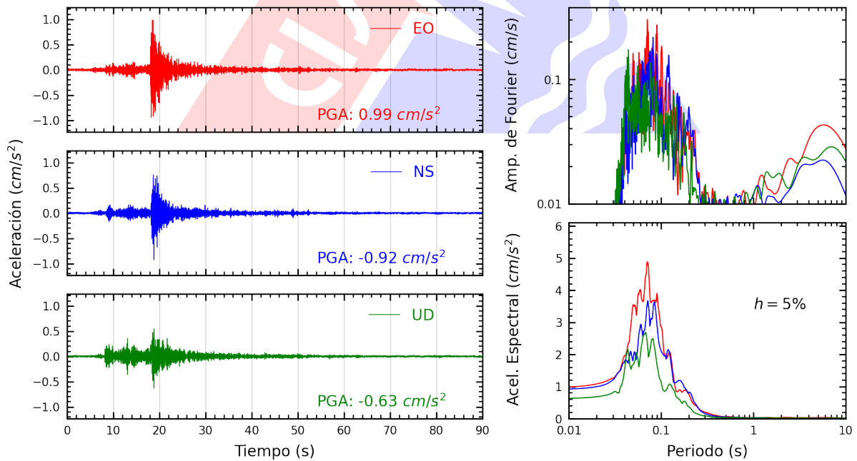
Figura A.18: Registros tiempo-historia, espectros de Fourier y de respuesta en las direcciones EO, NS y vertical de la estación UPCSM. Sismo de Ancon, Lima - Lima del 2023-08-03, 01:47:23 (Hora local)
