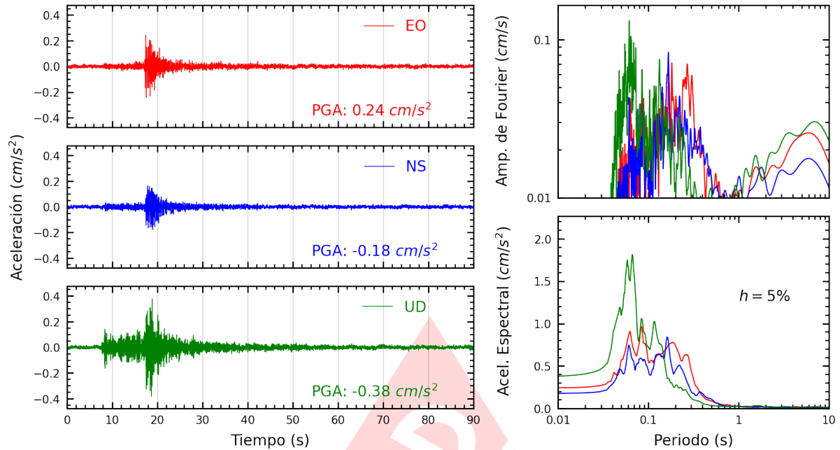
Figura A.35: Registros tiempo-historia, espectros de Fourier y de respuesta en las direcciones EO, NS y vertical de la estación ACAPU. Sismo de Ancon, Lima - Lima del 2023-08-03, 01:47:23 (Hora local)
