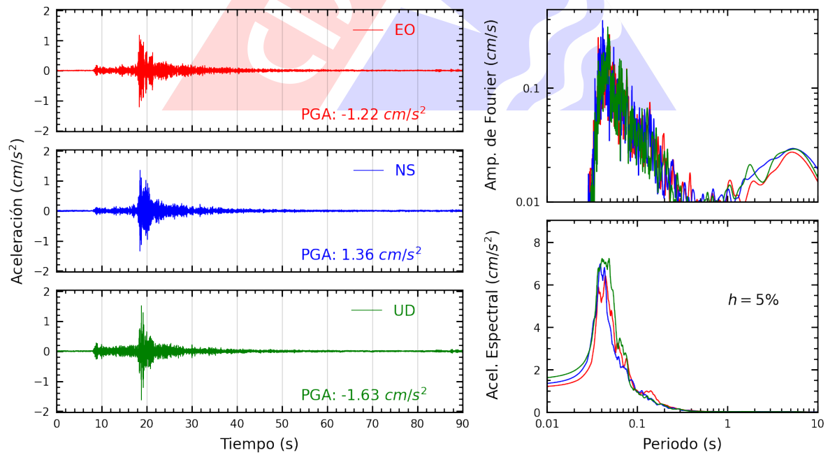
Figura A.14: Registros tiempo-historia, espectros de Fourier y de respuesta en las direcciones EO, NS y vertical de la estación USMP. Sismo de Ancon, Lima - Lima del 2023-08-03, 01:47:23 (Hora local)
