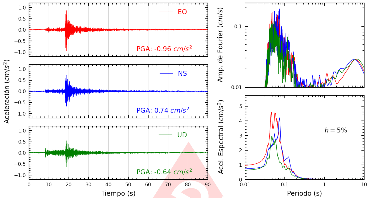
Figura A.19: Registros tiempo-historia, espectros de Fourier y de respuesta en las direcciones EO, NS y vertical de la estación CENEP. Sismo de Ancon, Lima - Lima del 2023-08-03, 01:47:23 (Hora local)
