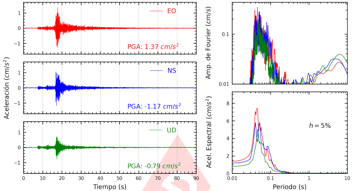
Figura A.15: Registros tiempo-historia, espectros de Fourier y de respuesta en las direcciones EO, NS y vertical de la estación UCSS. Sismo de Ancon, Lima - Lima del 2023-08-03, 01:47:23 (Hora local)
