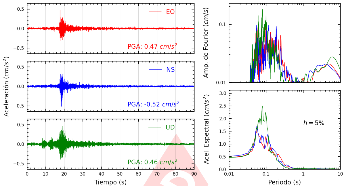
Figura A.31: Registros tiempo-historia, espectros de Fourier y de respuesta en las direcciones EO, NS y vertical de la estación RAMON. Sismo de Ancon, Lima - Lima del 2023-08-03, 01:47:23 (Hora local)
