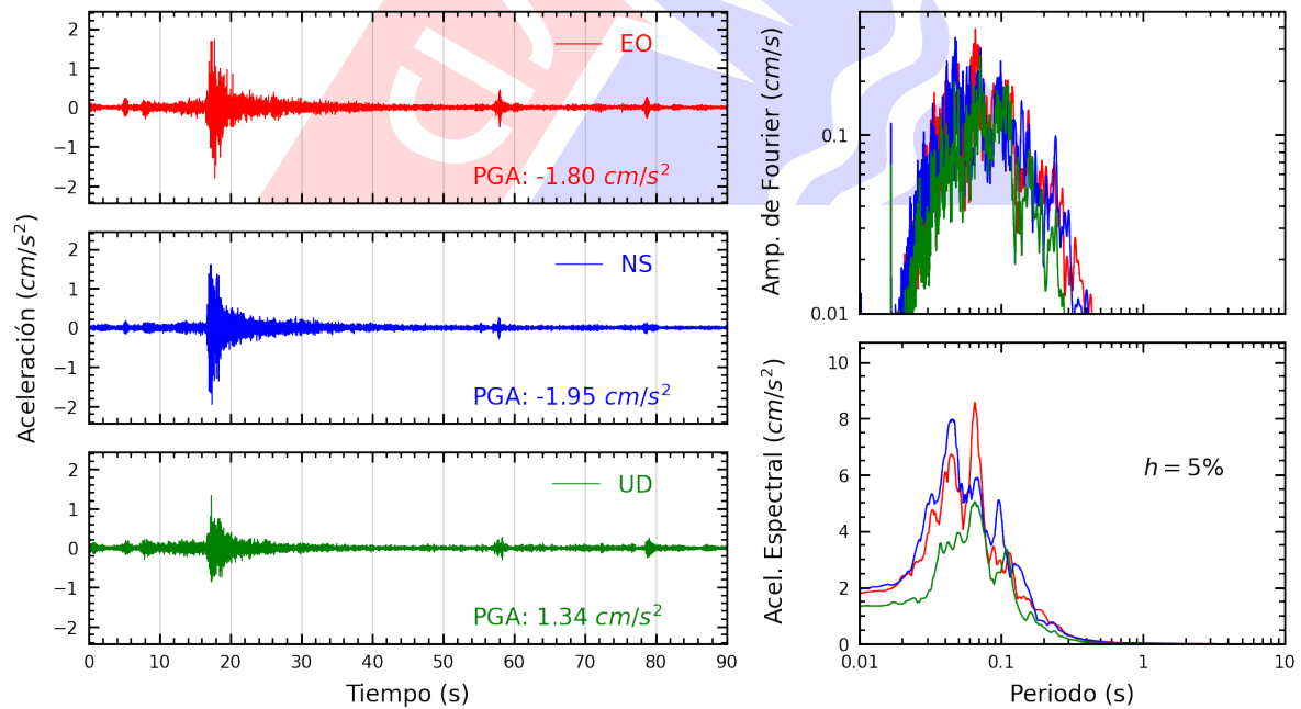
Figura A.10: Registros tiempo-historia, espectros de Fourier y de respuesta en las direcciones EO, NS y vertical de la estación SCOLI. Sismo de Ancon, Lima - Lima del 2023-08-03, 01:47:23 (Hora local)
