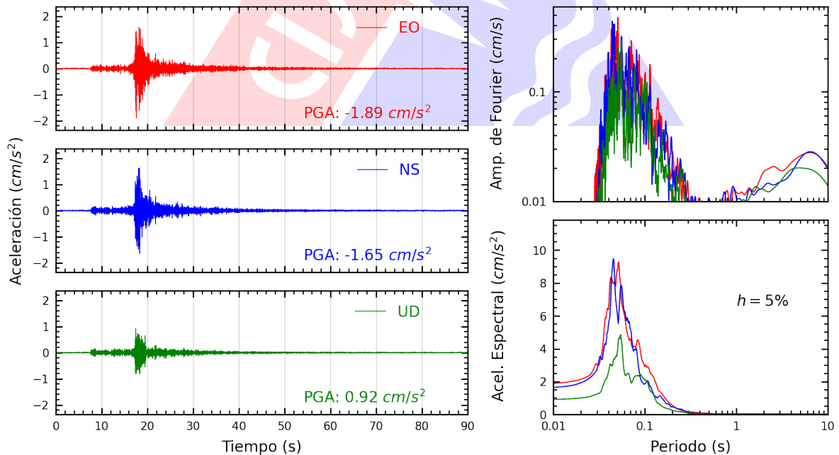
Figura A.12: Registros tiempo-historia, espectros de Fourier y de respuesta en las direcciones EO, NS y vertical de la estación FICPE. Sismo de Ancon, Lima - Lima del 2023-08-03, 01:47:23 (Hora local)
