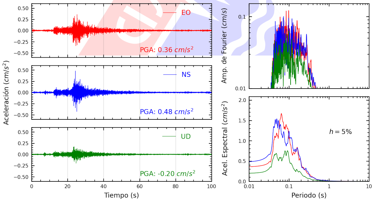
Figura A.32: Registros tiempo-historia, espectros de Fourier y de respuesta en las direcciones EO, NS y vertical de la estación BRISA. Sismo de Ancon, Lima - Lima del 2023-08-03, 01:47:23 (Hora local)
