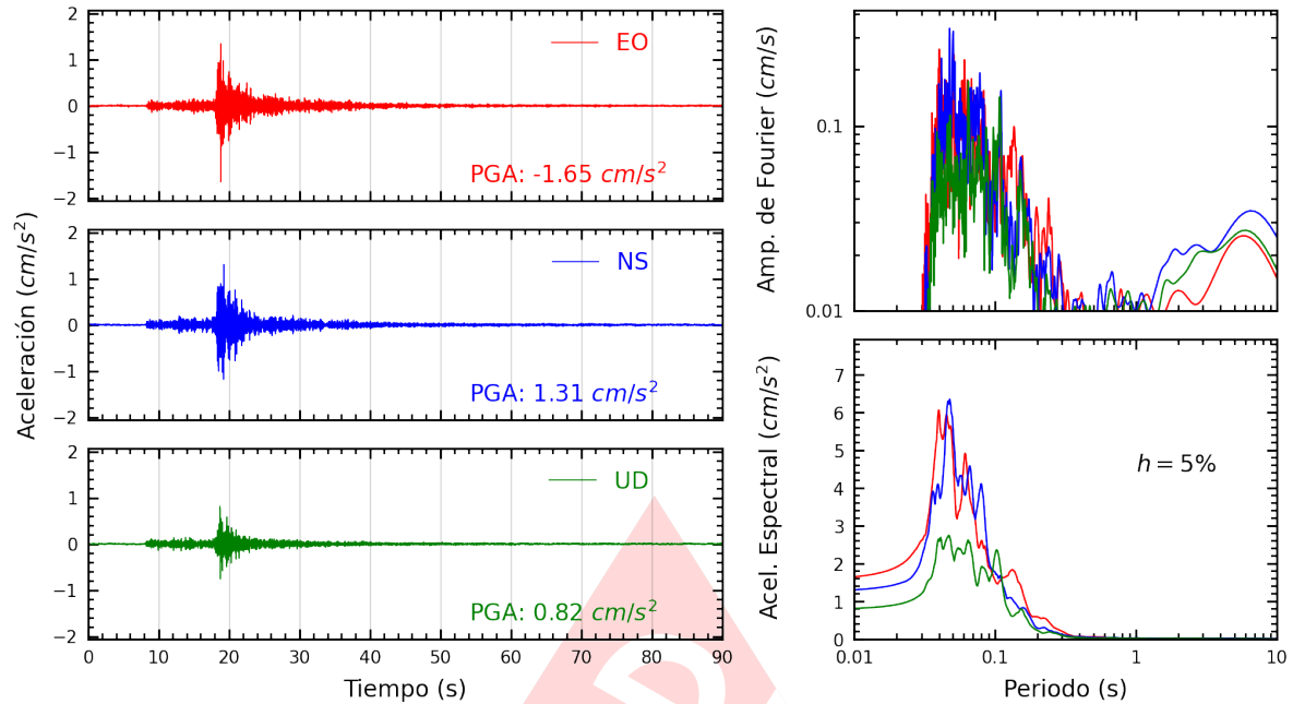
Figura A.13: Registros tiempo-historia, espectros de Fourier y de respuesta en las direcciones EO, NS y vertical de la estación CEPRE. Sismo de Ancon, Lima - Lima del 2023-08-03, 01:47:23 (Hora local)
