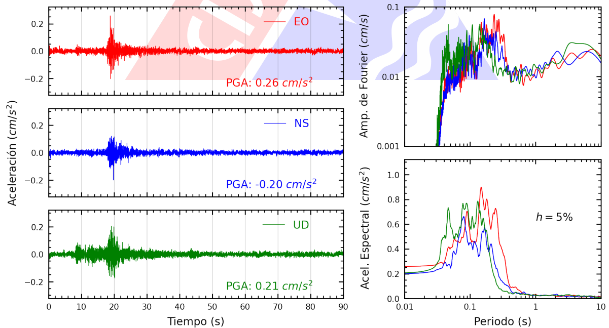
Figura A.36: Registros tiempo-historia, espectros de Fourier y de respuesta en las direcciones EO, NS y vertical de la estación DSMI. Sismo de Ancon, Lima - Lima del 2023-08-03, 01:47:23 (Hora local)
