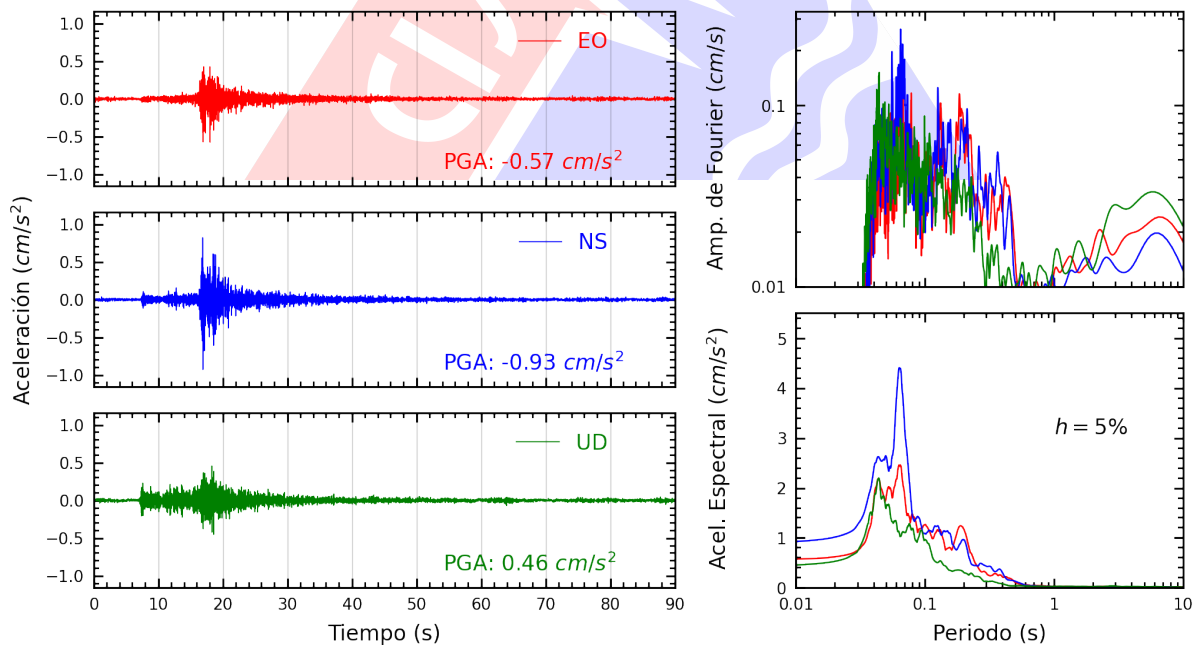
Figura A.20: Registros tiempo-historia, espectros de Fourier y de respuesta en las direcciones EO, NS y vertical de la estación VHAYA. Sismo de Ancon, Lima - Lima del 2023-08-03, 01:47:23 (Hora local)
