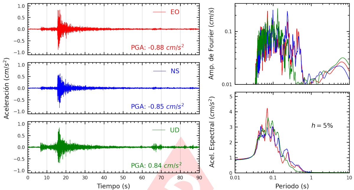
Figura A.21: Registros tiempo-historia, espectros de Fourier y de respuesta en las direcciones EO, NS y vertical de la estación MDPP. Sismo de Ancon, Lima - Lima del 2023-08-03, 01:47:23 (Hora local)
