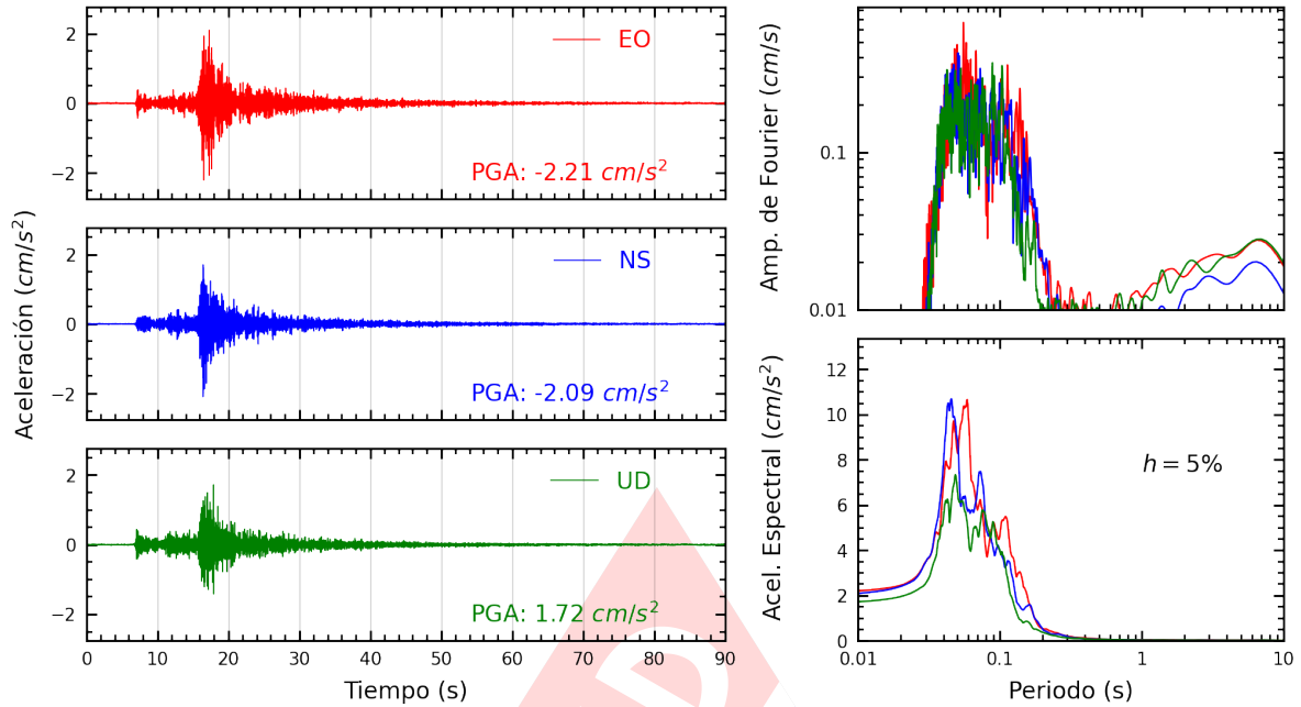
Figura A.7: Registros tiempo-historia, espectros de Fourier y de respuesta en las direcciones EO, NS y vertical de la estación AMORE. Sismo de Ancon, Lima - Lima del 2023-08-03, 01:47:23 (Hora local)
