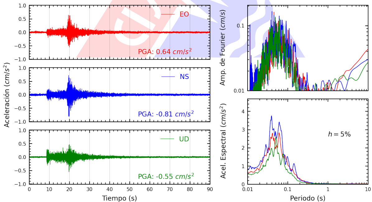
Figura A.24: Registros tiempo-historia, espectros de Fourier y de respuesta en las direcciones EO, NS y vertical de la estación SERVI. Sismo de Ancon, Lima - Lima del 2023-08-03, 01:47:23 (Hora local)
