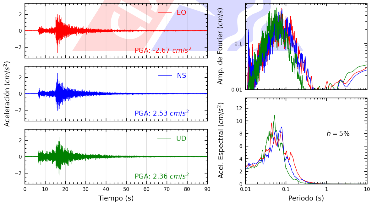
Figura A.4: Registros tiempo-historia, espectros de Fourier y de respuesta en las direcciones EO, NS y vertical de la estación ANCON. Sismo de Ancon, Lima - Lima del 2023-08-03, 01:47:23 (Hora local)
