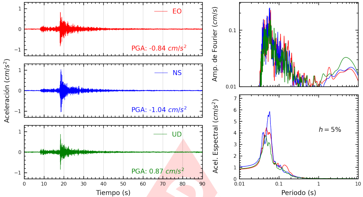
Figura A.17: Registros tiempo-historia, espectros de Fourier y de respuesta en las direcciones EO, NS y vertical de la estación IMCA. Sismo de Ancon, Lima - Lima del 2023-08-03, 01:47:23 (Hora local)
