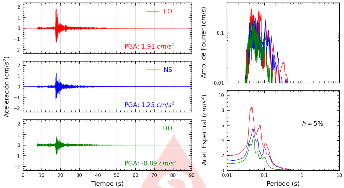
Figura A.11: Registros tiempo-historia, espectros de Fourier y de respuesta en las direcciones EO, NS y vertical de la estación ATARJ. Sismo de Ancon, Lima - Lima del 2023-08-03, 01:47:23 (Hora local)
