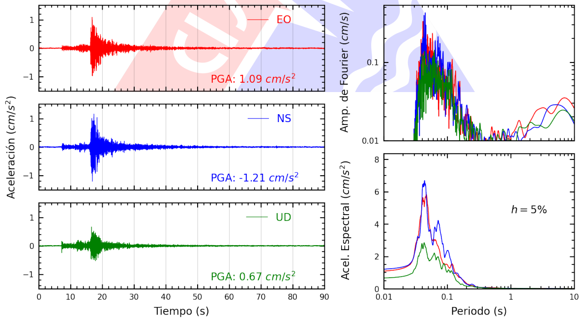
Figura A.16: Registros tiempo-historia, espectros de Fourier y de respuesta en las direcciones EO, NS y vertical de la estación COMAS. Sismo de Ancon, Lima - Lima del 2023-08-03, 01:47:23 (Hora local)
