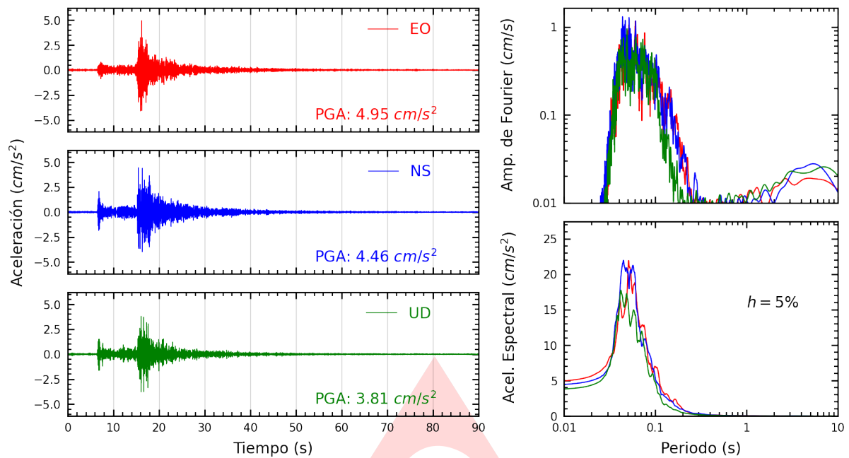
Figura A.1: Registros tiempo-historia, espectros de Fourier y de respuesta en las direcciones EO, NS y vertical de la estación SROSA. Sismo de Ancon, Lima - Lima del 2023-08-03, 01:47:23 (Hora local)
