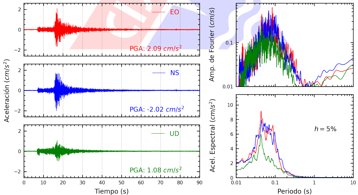
Figura A.8: Registros tiempo-historia, espectros de Fourier y de respuesta en las direcciones EO, NS y vertical de la estación DEFEN. Sismo de Ancon, Lima - Lima del 2023-08-03, 01:47:23 (Hora local)
