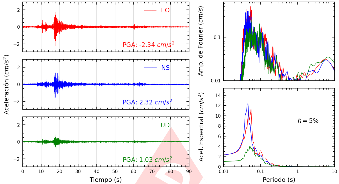
Figura A.5: Registros tiempo-historia, espectros de Fourier y de respuesta en las direcciones EO, NS y vertical de la estación OLIVO. Sismo de Ancon, Lima - Lima del 2023-08-03, 01:47:23 (Hora local)
