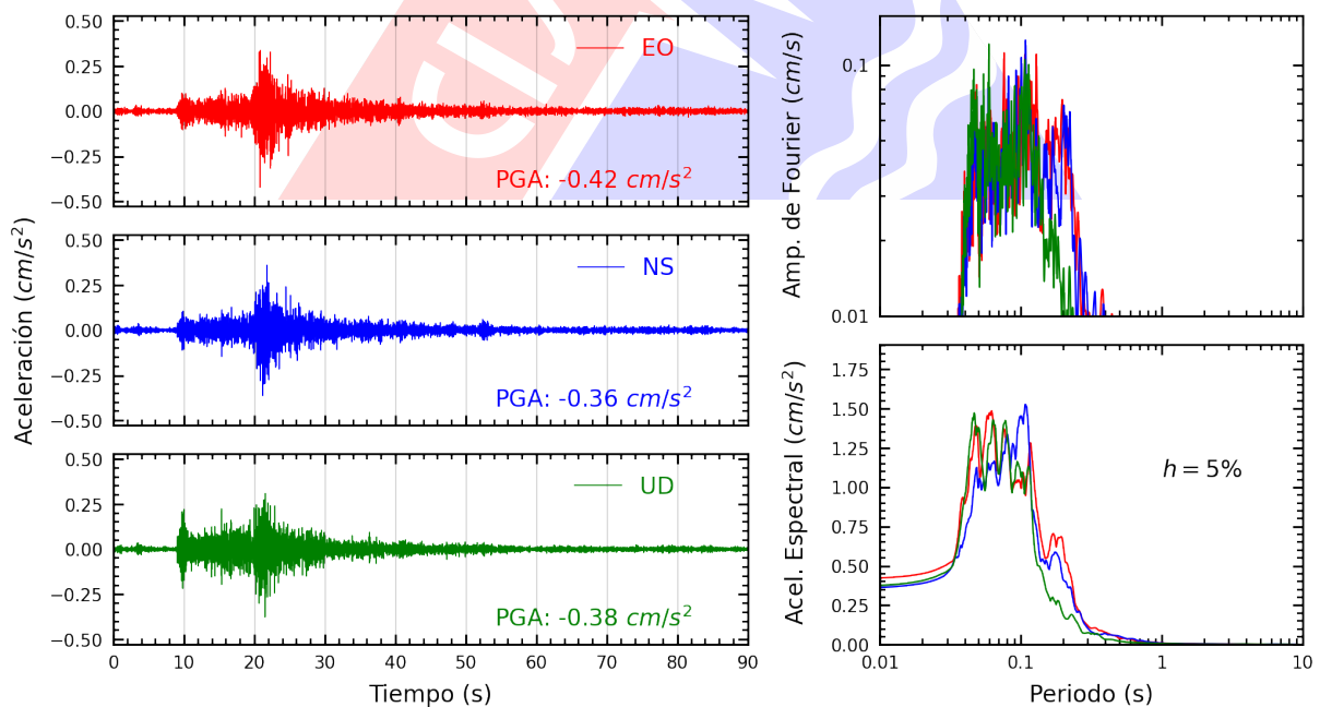
Figura A.34: Registros tiempo-historia, espectros de Fourier y de respuesta en las direcciones EO, NS y vertical de la estación SCCHO. Sismo de Ancon, Lima - Lima del 2023-08-03, 01:47:23 (Hora local)
