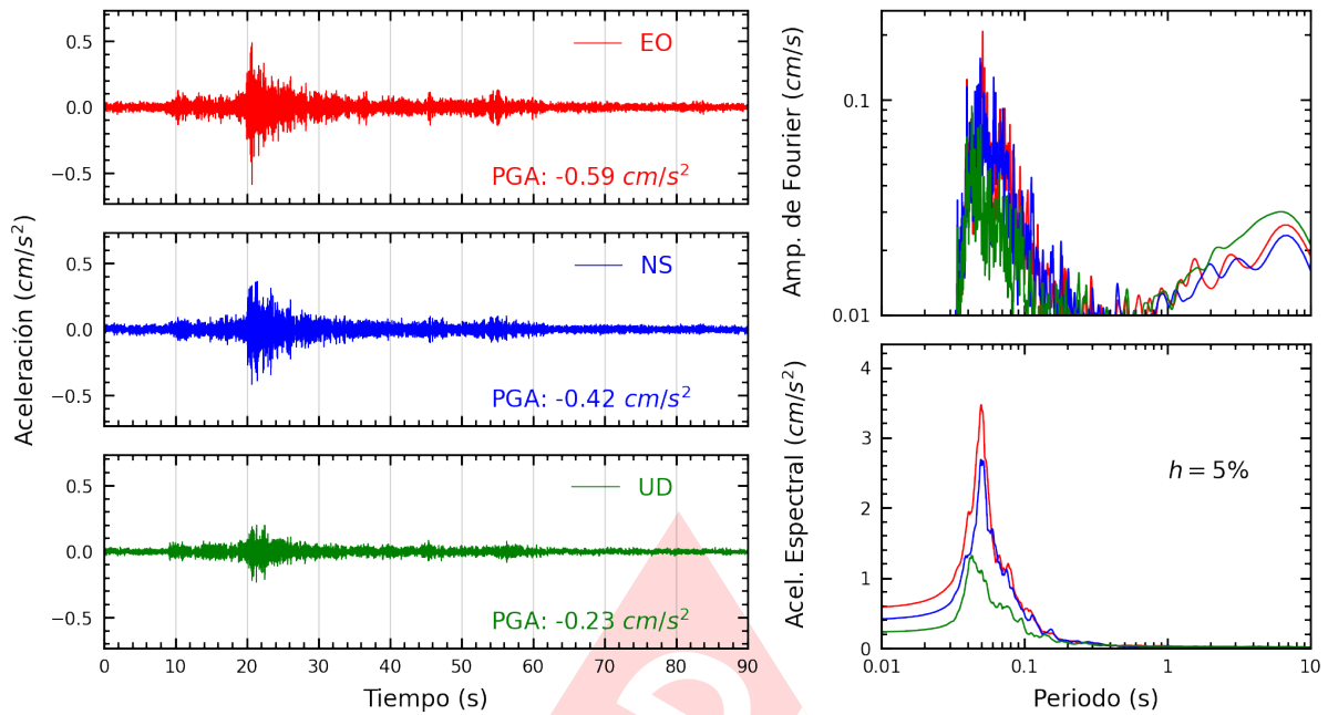
Figura A.27: Registros tiempo-historia, espectros de Fourier y de respuesta en las direcciones EO, NS y vertical de la estación UPCVI. Sismo de Ancon, Lima - Lima del 2023-08-03, 01:47:23 (Hora local)
