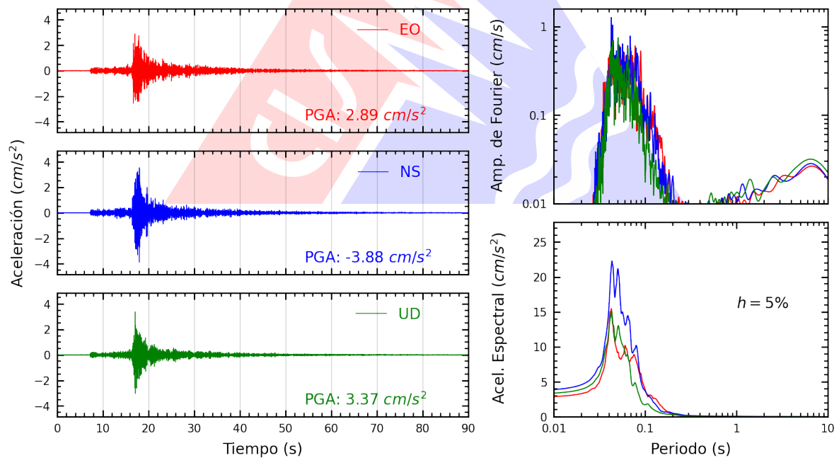
Figura A.2: Registros tiempo-historia, espectros de Fourier y de respuesta en las direcciones EO, NS y vertical de la estación JOSEO. Sismo de Ancon, Lima - Lima del 2023-08-03, 01:47:23 (Hora local)
