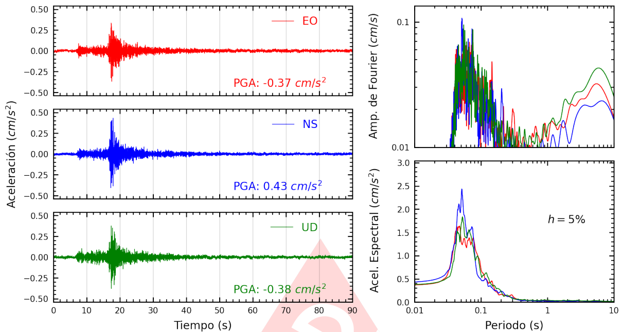
Figura A.33: Registros tiempo-historia, espectros de Fourier y de respuesta en las direcciones EO, NS y vertical de la estación UNMSM. Sismo de Ancon, Lima - Lima del 2023-08-03, 01:47:23 (Hora local)
