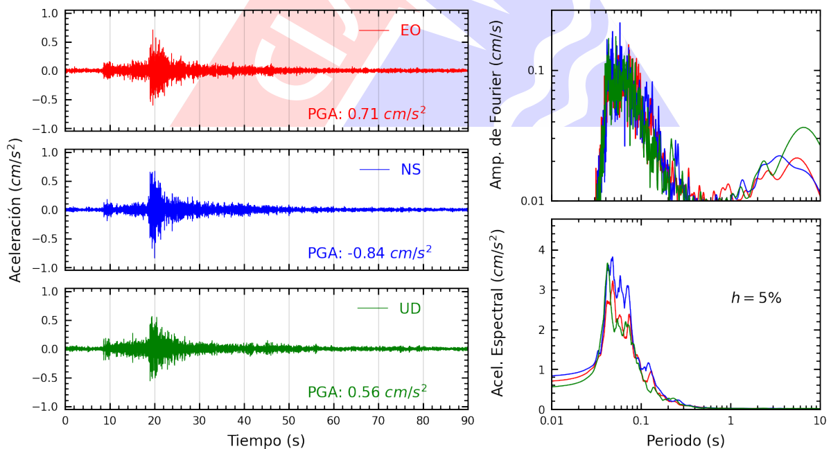
Figura A.22: Registros tiempo-historia, espectros de Fourier y de respuesta en las direcciones EO, NS y vertical de la estación URPE. Sismo de Ancon, Lima - Lima del 2023-08-03, 01:47:23 (Hora local)
