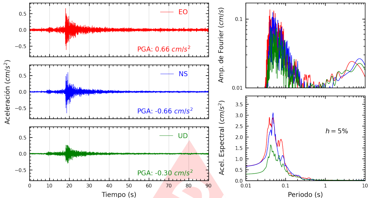
Figura A.25: Registros tiempo-historia, espectros de Fourier y de respuesta en las direcciones EO, NS y vertical de la estación INICT. Sismo de Ancon, Lima - Lima del 2023-08-03, 01:47:23 (Hora local)
