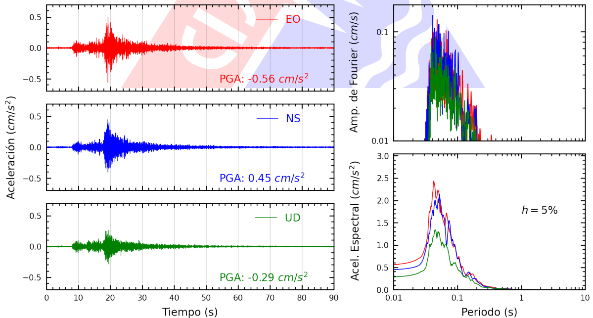
Figura A.28: Registros tiempo-historia, espectros de Fourier y de respuesta en las direcciones EO, NS y vertical de la estación BORJA. Sismo de Ancon, Lima - Lima del 2023-08-03, 01:47:23 (Hora local)
