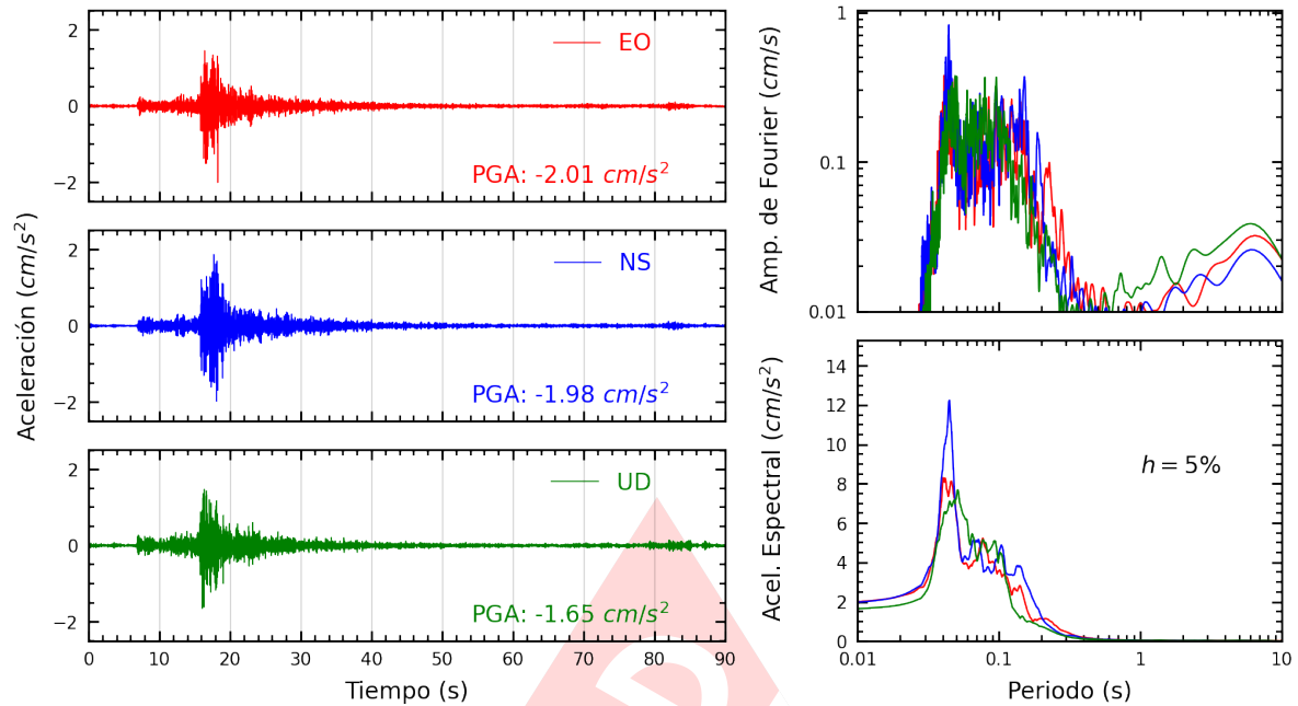
Figura A.9: Registros tiempo-historia, espectros de Fourier y de respuesta en las direcciones EO, NS y vertical de la estación CARAB. Sismo de Ancon, Lima - Lima del 2023-08-03, 01:47:23 (Hora local)
