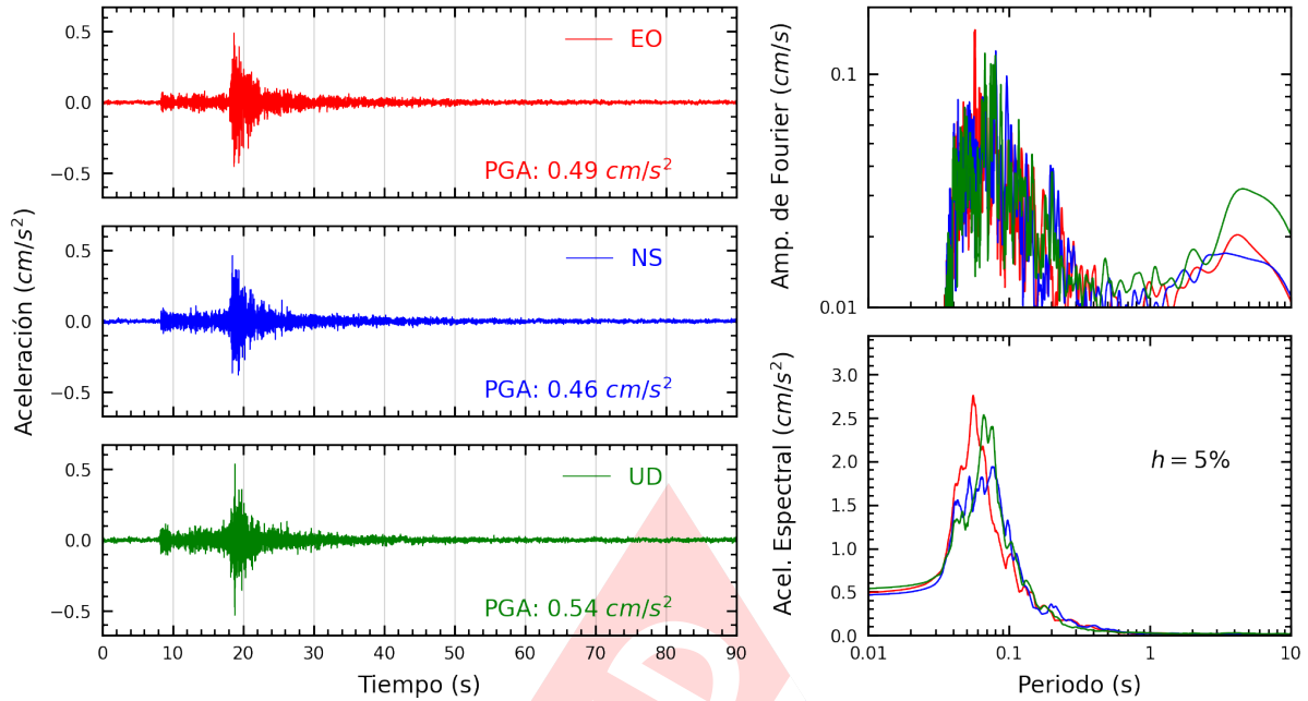
Figura A.29: Registros tiempo-historia, espectros de Fourier y de respuesta en las direcciones EO, NS y vertical de la estación UNFV. Sismo de Ancon, Lima - Lima del 2023-08-03, 01:47:23 (Hora local)
