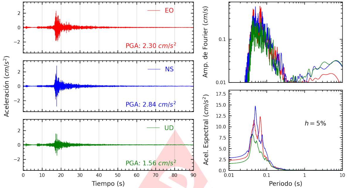
Figura A.3: Registros tiempo-historia, espectros de Fourier y de respuesta en las direcciones EO, NS y vertical de la estación INDEP. Sismo de Ancon, Lima - Lima del 2023-08-03, 01:47:23 (Hora local)
