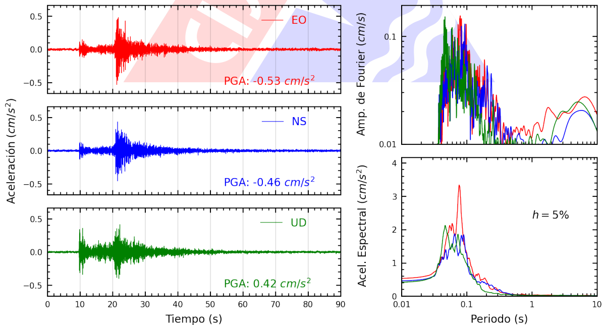
Figura A.30: Registros tiempo-historia, espectros de Fourier y de respuesta en las direcciones EO, NS y vertical de la estación USILP. Sismo de Ancon, Lima - Lima del 2023-08-03, 01:47:23 (Hora local)
