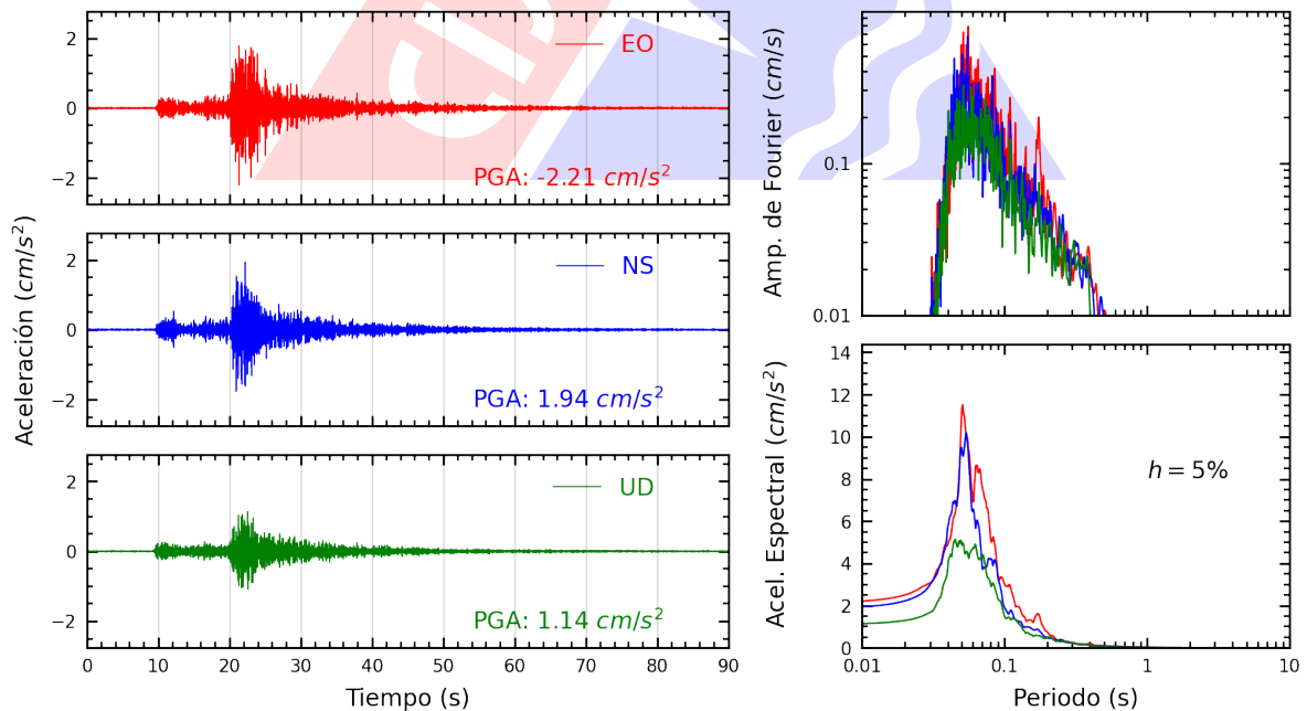
Figura A.6: Registros tiempo-historia, espectros de Fourier y de respuesta en las direcciones EO, NS y vertical de la estación UNTEL. Sismo de Ancon, Lima - Lima del 2023-08-03, 01:47:23 (Hora local)
