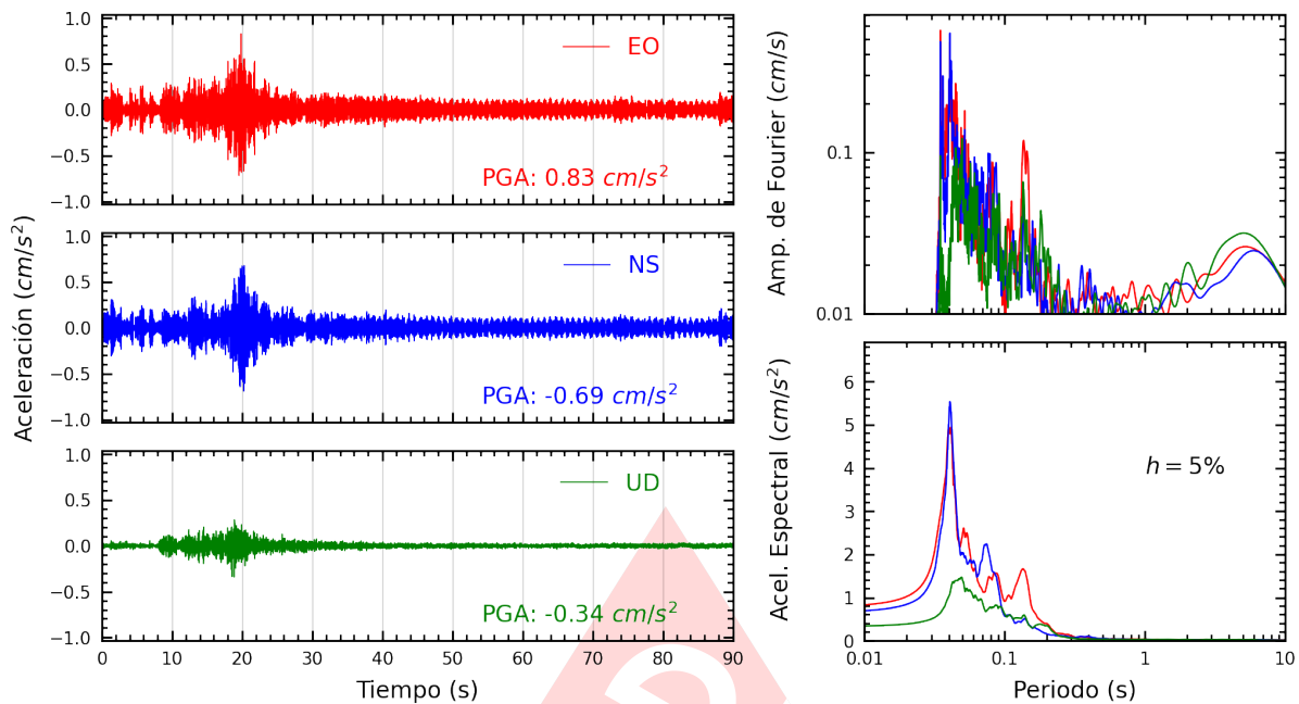
Figura A.23: Registros tiempo-historia, espectros de Fourier y de respuesta en las direcciones EO, NS y vertical de la estación DHNPE. Sismo de Ancon, Lima - Lima del 2023-08-03, 01:47:23 (Hora local)
