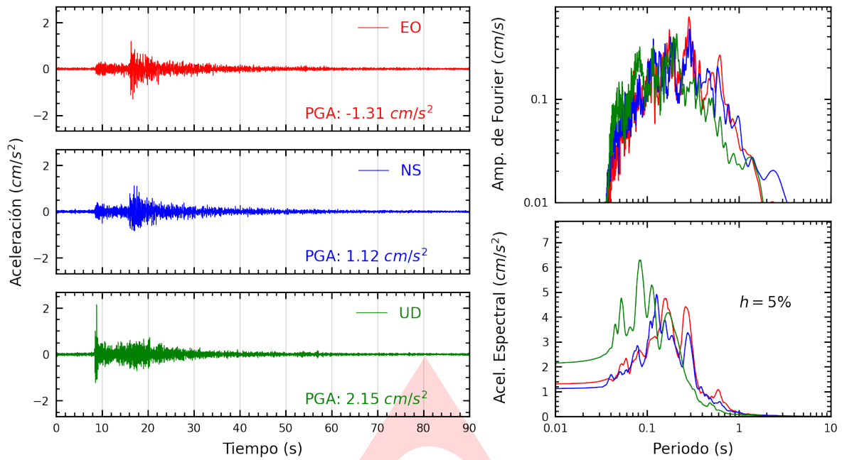
Figura A.1: Registros tiempo-historia, espectros de Fourier y de respuesta en las direcciones EO, NS y vertical de la estación UNICA. Sismo de Ica, Ica - Ica del 2023-10-02, 11:24:02 (Hora local)
