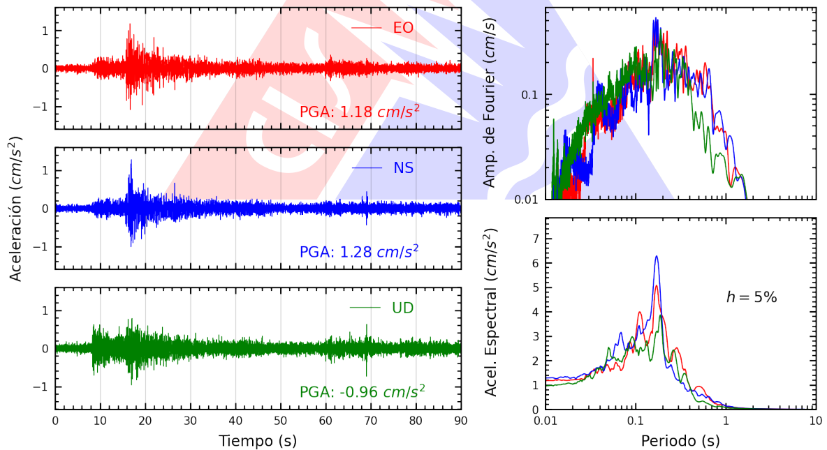
Figura A.2: Registros tiempo-historia, espectros de Fourier y de respuesta en las direcciones EO, NS y vertical de la estación SCICA. Sismo de Ica, Ica - Ica del 2023-10-02, 11:24:02 (Hora local)
