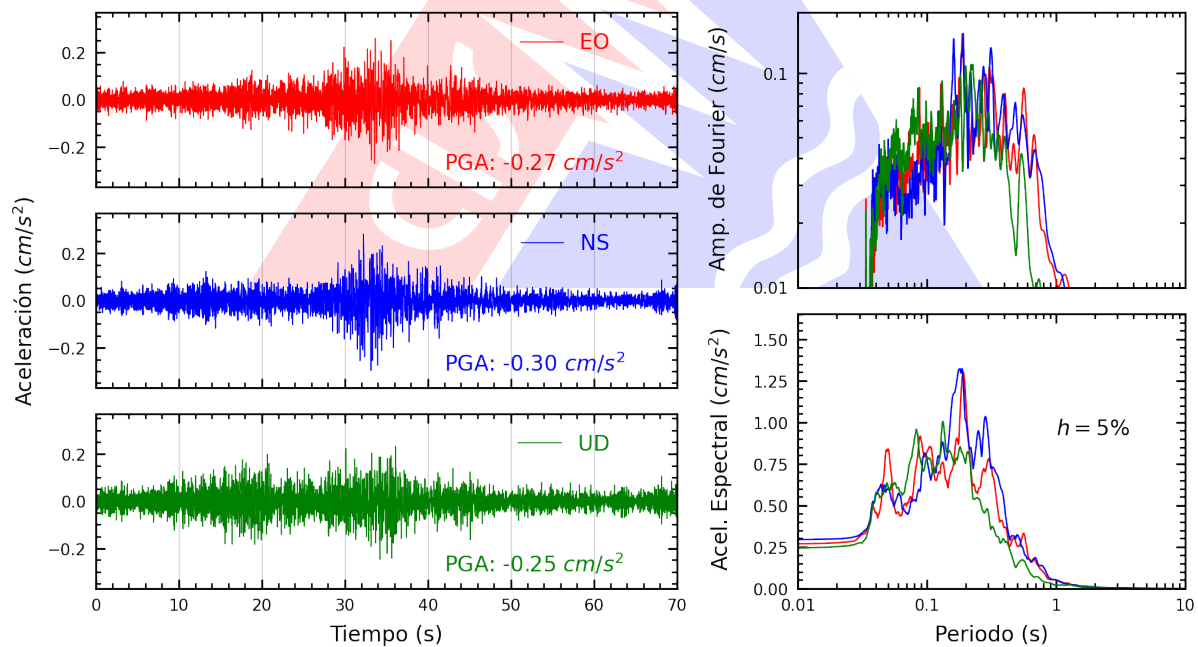
Figura A.2: Registros tiempo-historia, espectros de Fourier y de respuesta en las direcciones EO, NS y vertical de la estación SCICA. Sismo de Marcona, Nazca - Ica del 2023-10-15, 22:49:31 (Hora local)
