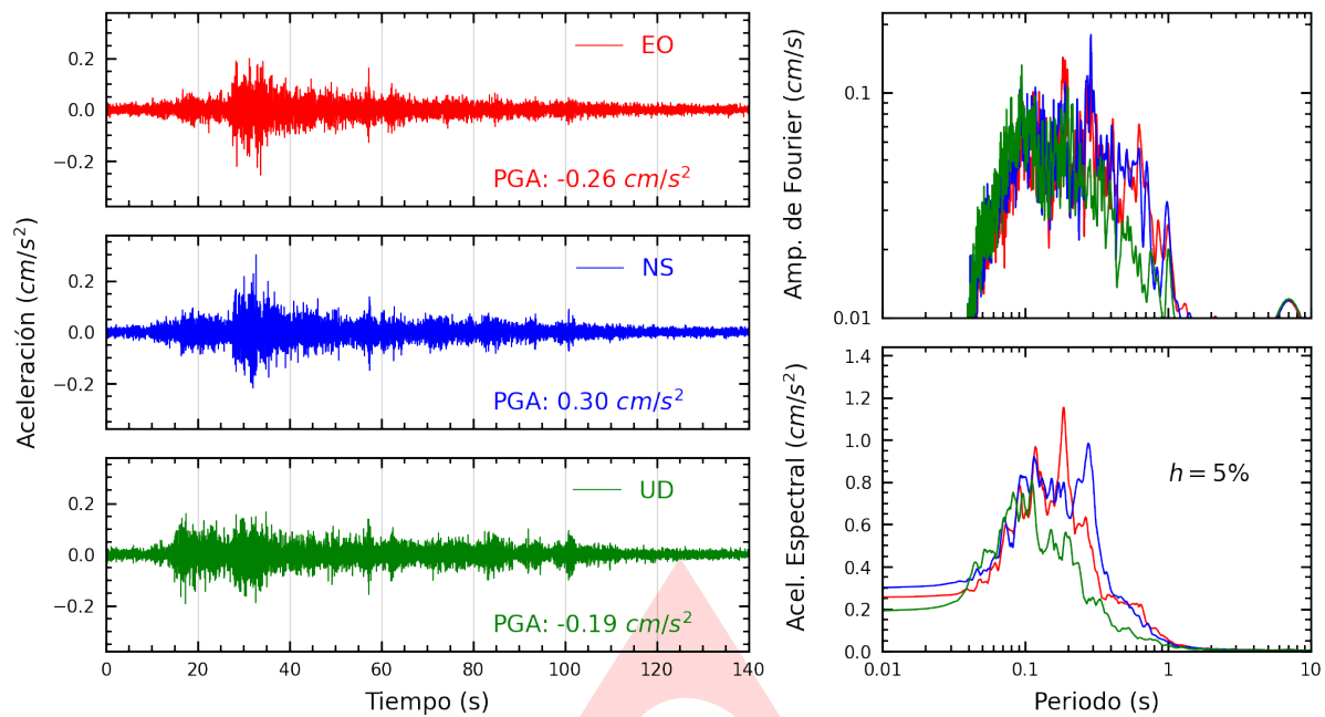
Figura A.1: Registros tiempo-historia, espectros de Fourier y de respuesta en las direcciones EO, NS y vertical de la estación UNICA. Sismo de Marcona, Nazca - Ica del 2023-10-15, 22:49:31 (Hora local)
