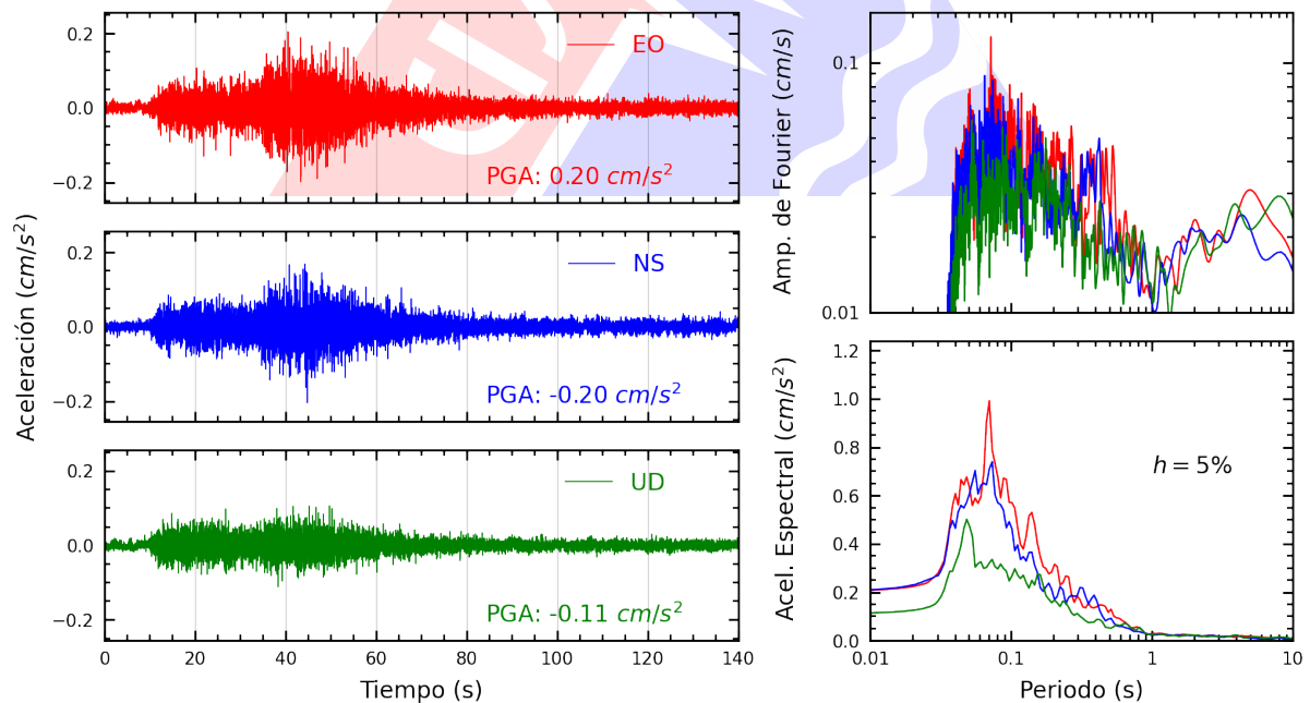
Figura A.18: Registros tiempo-historia, espectros de Fourier y de respuesta en las direcciones EO, NS y vertical de la estación FICPE. Sismo de Huarney, Huarney - Ancash del 2023-11-01, 01:47:05 (Hora local)
