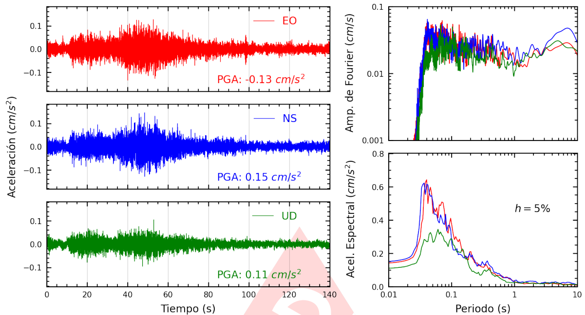
Figura A.21: Registros tiempo-historia, espectros de Fourier y de respuesta en las direcciones EO, NS y vertical de la estación CEPRE. Sismo de Huarney, Huarney - Ancash del 2023-11-01, 01:47:05 (Hora local)
