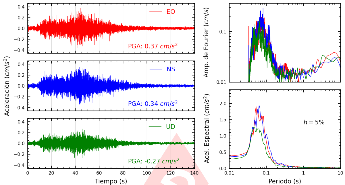
Figura A.11: Registros tiempo-historia, espectros de Fourier y de respuesta en las direcciones EO, NS y vertical de la estación JOSEO. Sismo de Huarney, Huarney - Ancash del 2023-11-01, 01:47:05 (Hora local)
