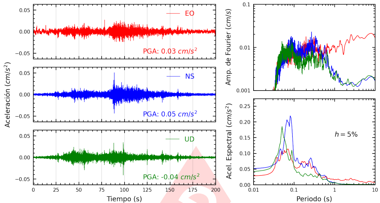
Figura A.31: Registros tiempo-historia, espectros de Fourier y de respuesta en las direcciones EO, NS y vertical de la estación SCCHL. Sismo de Huarney, Huarney - Ancash del 2023-11-01, 01:47:05 (Hora local)
