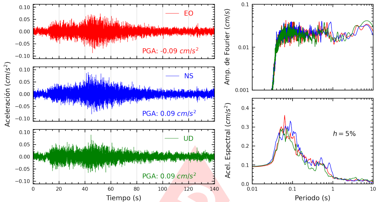
Figura A.29: Registros tiempo-historia, espectros de Fourier y de respuesta en las direcciones EO, NS y vertical de la estación SERVI. Sismo de Huarney, Huarney - Ancash del 2023-11-01, 01:47:05 (Hora local)
