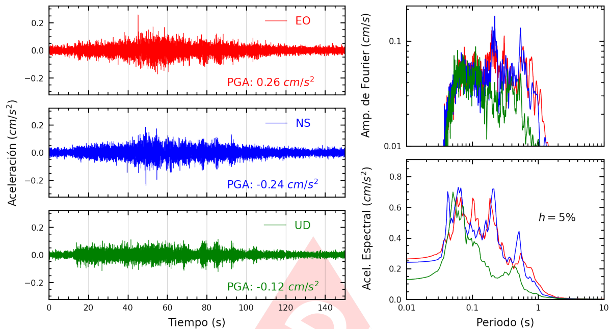
Figura A.15: Registros tiempo-historia, espectros de Fourier y de respuesta en las direcciones EO, NS y vertical de la estación SCCHO. Sismo de Huarney, Huarney - Ancash del 2023-11-01, 01:47:05 (Hora local)
