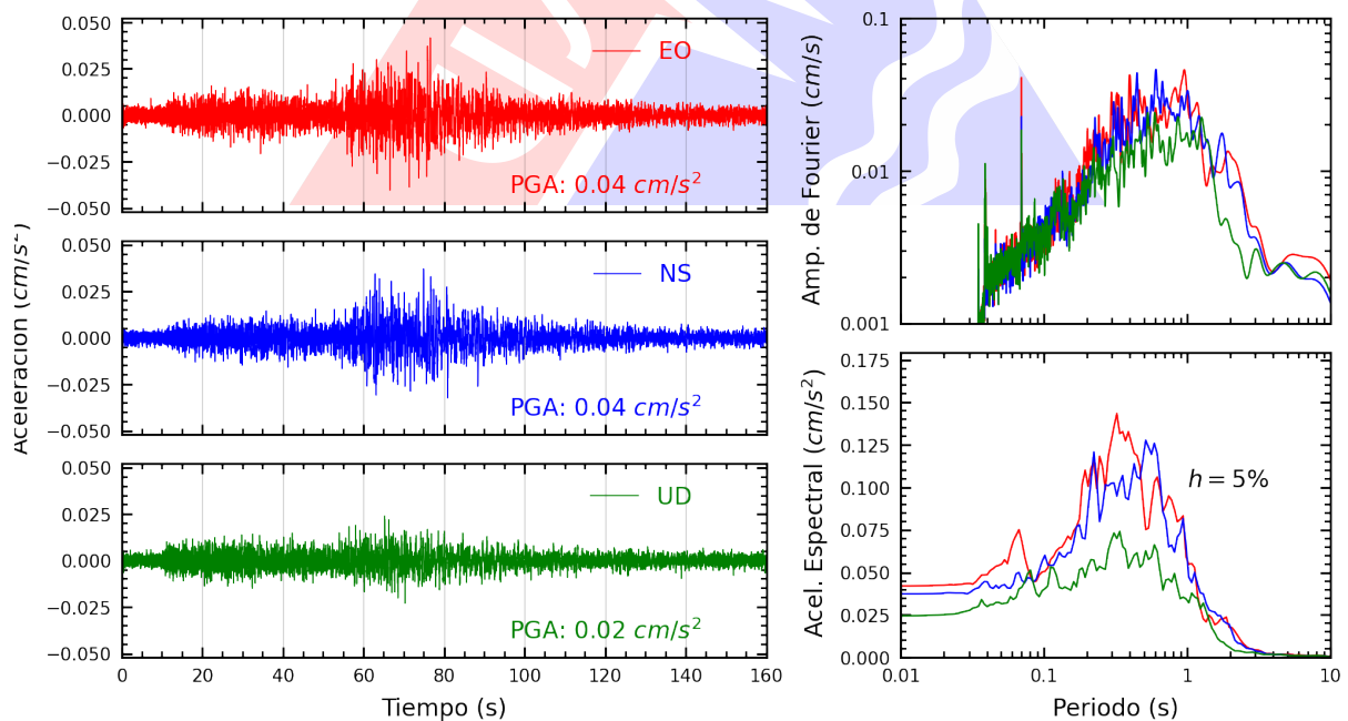
Figura A.32: Registros tiempo-historia, espectros de Fourier y de respuesta en las direcciones EO, NS y vertical de la estación UNC. Sismo de Huarney, Huarney - Ancash del 2023-11-01, 01:47:05 (Hora local)
