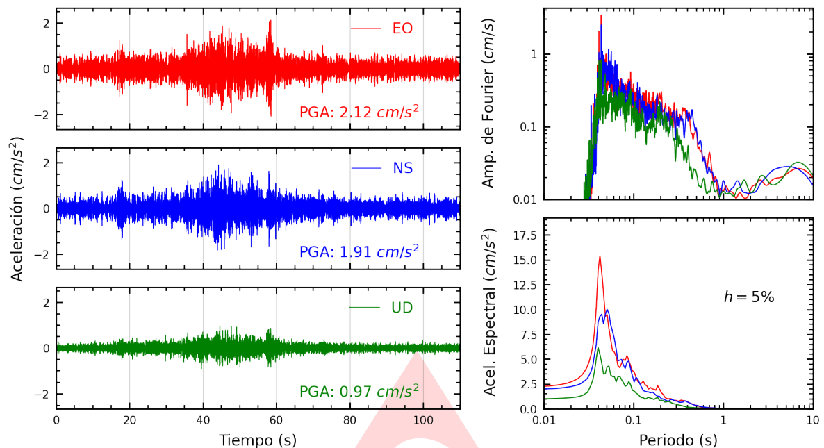
Figura A.1: Registros tiempo-historia, espectros de Fourier y de respuesta en las direcciones EO, NS y vertical de la estación USP. Sismo de Huarney, Huarney - Ancash del 2023-11-01, 01:47:05 (Hora local)
