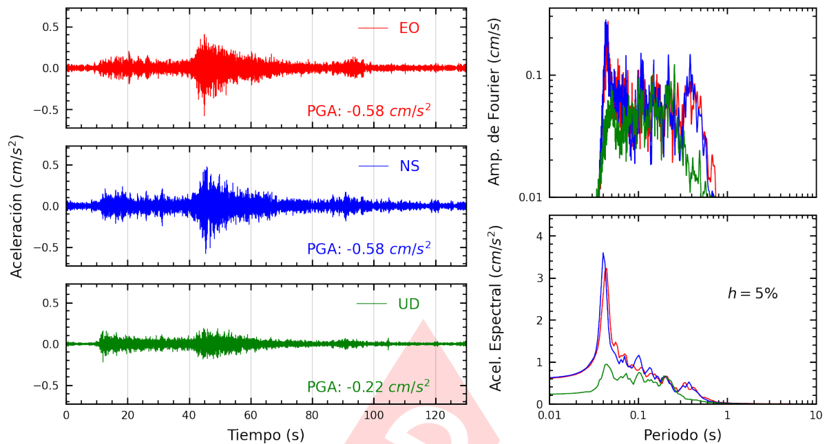
Figura A.7: Registros tiempo-historia, espectros de Fourier y de respuesta en las direcciones EO, NS y vertical de la estación SCTRU. Sismo de Huarney, Huarney - Ancash del 2023-11-01, 01:47:05 (Hora local)
