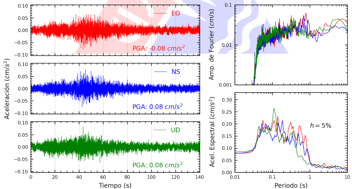
Figura A.30: Registros tiempo-historia, espectros de Fourier y de respuesta en las direcciones EO, NS y vertical de la estación UNMSM. Sismo de Huarney, Huarney - Ancash del 2023-11-01, 01:47:05 (Hora local)
