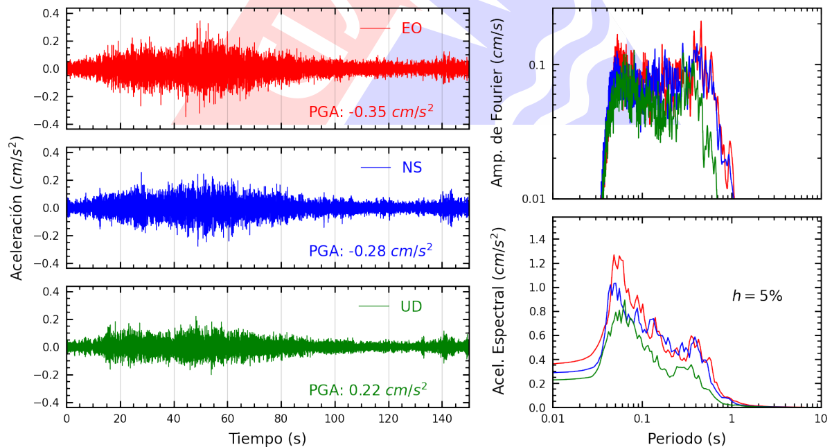
Figura A.12: Registros tiempo-historia, espectros de Fourier y de respuesta en las direcciones EO, NS y vertical de la estación UNTEL. Sismo de Huarney, Huarney - Ancash del 2023-11-01, 01:47:05 (Hora local)
