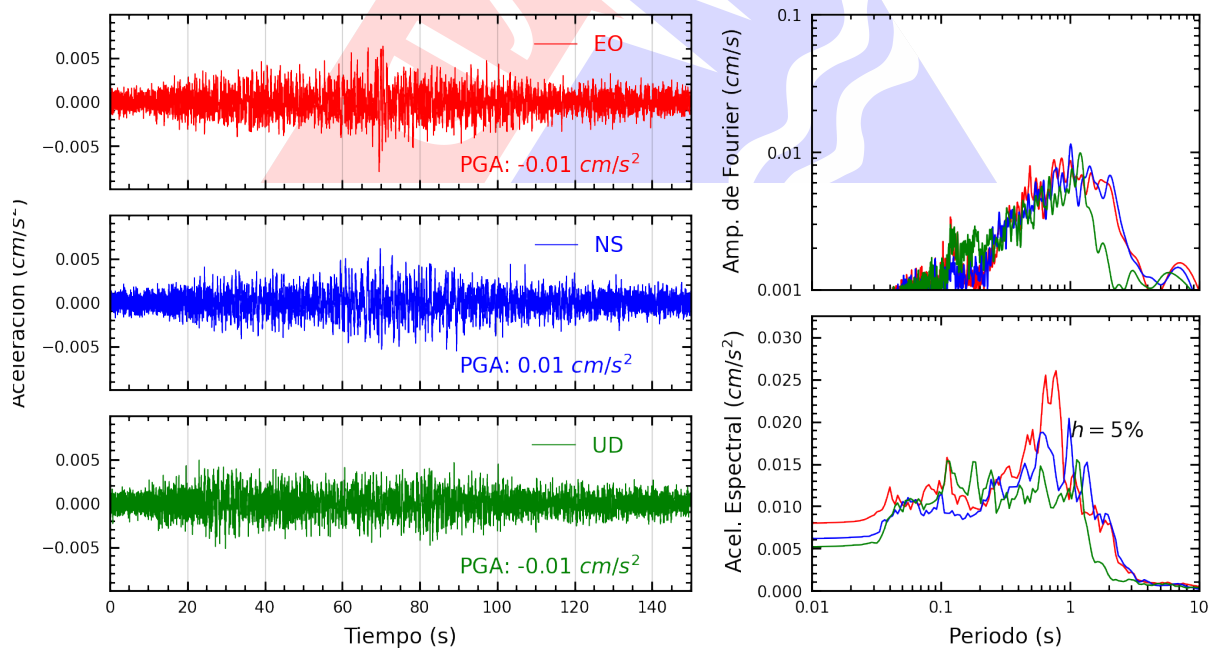
Figura A.34: Registros tiempo-historia, espectros de Fourier y de respuesta en las direcciones EO, NS y vertical de la estación UNCP. Sismo de Huarney, Huarney - Ancash del 2023-11-01, 01:47:05 (Hora local)
