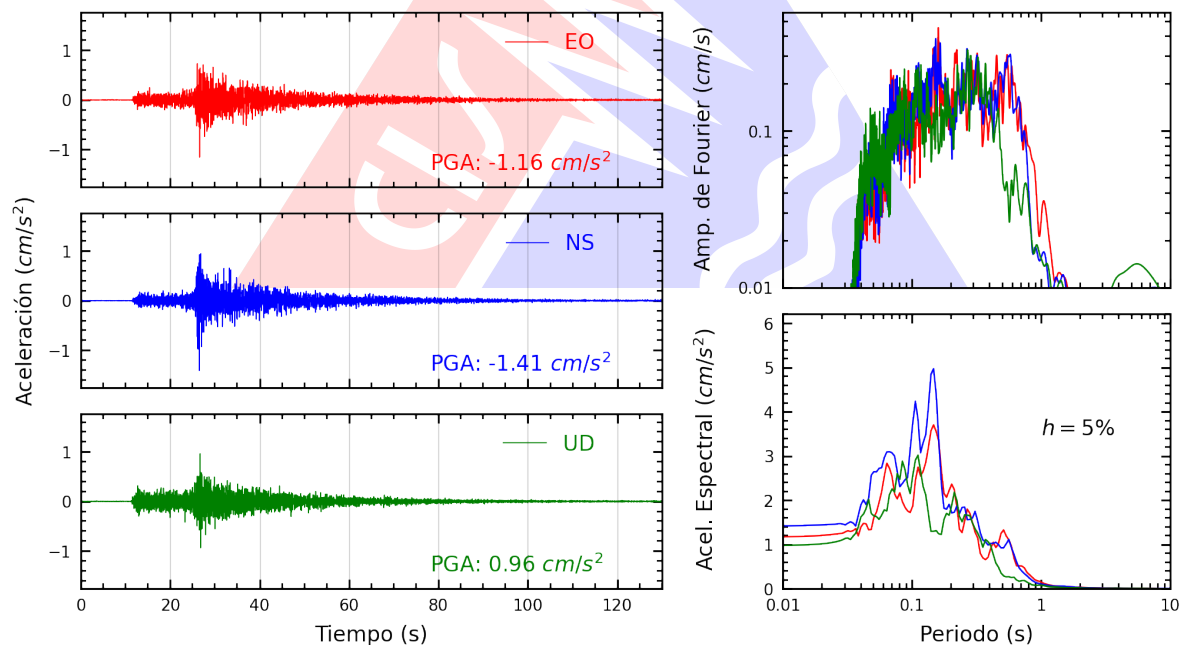
Figura A.2: Registros tiempo-historia, espectros de Fourier y de respuesta en las direcciones EO, NS y vertical de la estación CARAL. Sismo de Huarney, Huarney - Ancash del 2023-11-01, 01:47:05 (Hora local)
