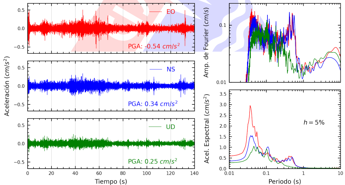
Figura A.8: Registros tiempo-historia, espectros de Fourier y de respuesta en las direcciones EO, NS y vertical de la estación OLIVO. Sismo de Huarney, Huarney - Ancash del 2023-11-01, 01:47:05 (Hora local)
