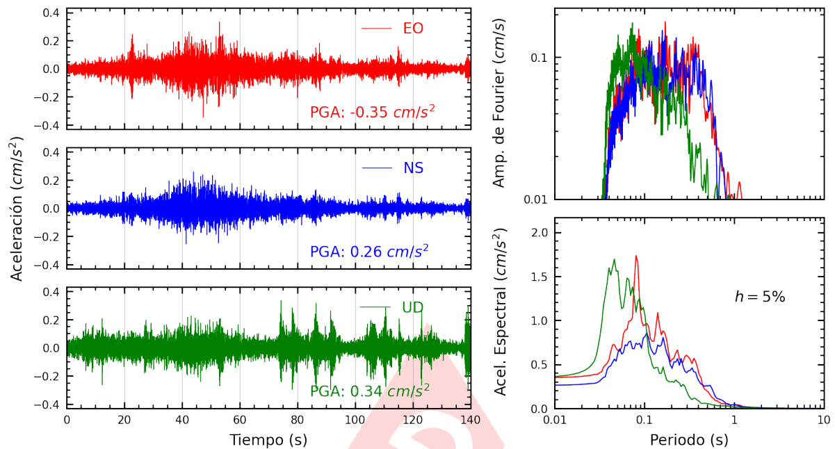
Figura A.13: Registros tiempo-historia, espectros de Fourier y de respuesta en las direcciones EO, NS y vertical de la estación SCOLI. Sismo de Huarney, Huarney - Ancash del 2023-11-01, 01:47:05 (Hora local)
