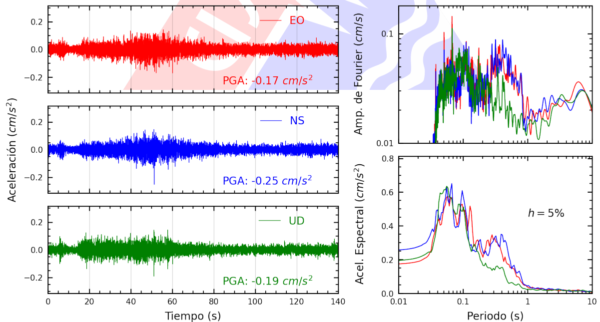
Figura A.16: Registros tiempo-historia, espectros de Fourier y de respuesta en las direcciones EO, NS y vertical de la estación MADRE. Sismo de Huarney, Huarney - Ancash del 2023-11-01, 01:47:05 (Hora local)
