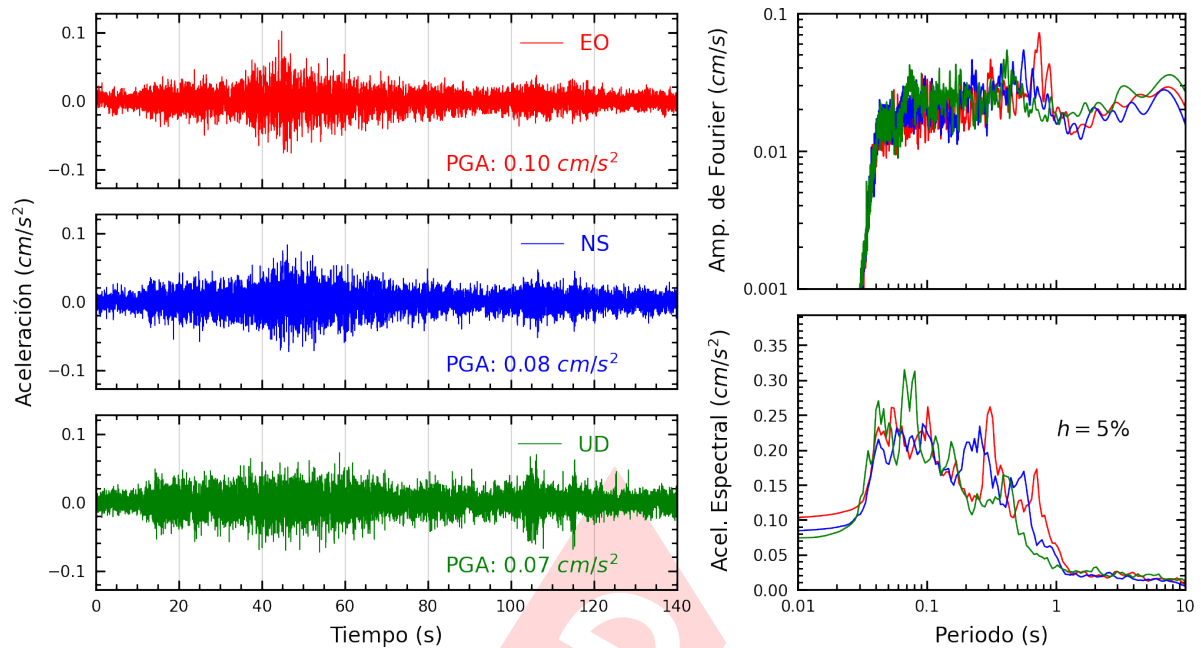
Figura A.27: Registros tiempo-historia, espectros de Fourier y de respuesta en las direcciones EO, NS y vertical de la estación UNFV. Sismo de Huarney, Huarney - Ancash del 2023-11-01, 01:47:05 (Hora local)
