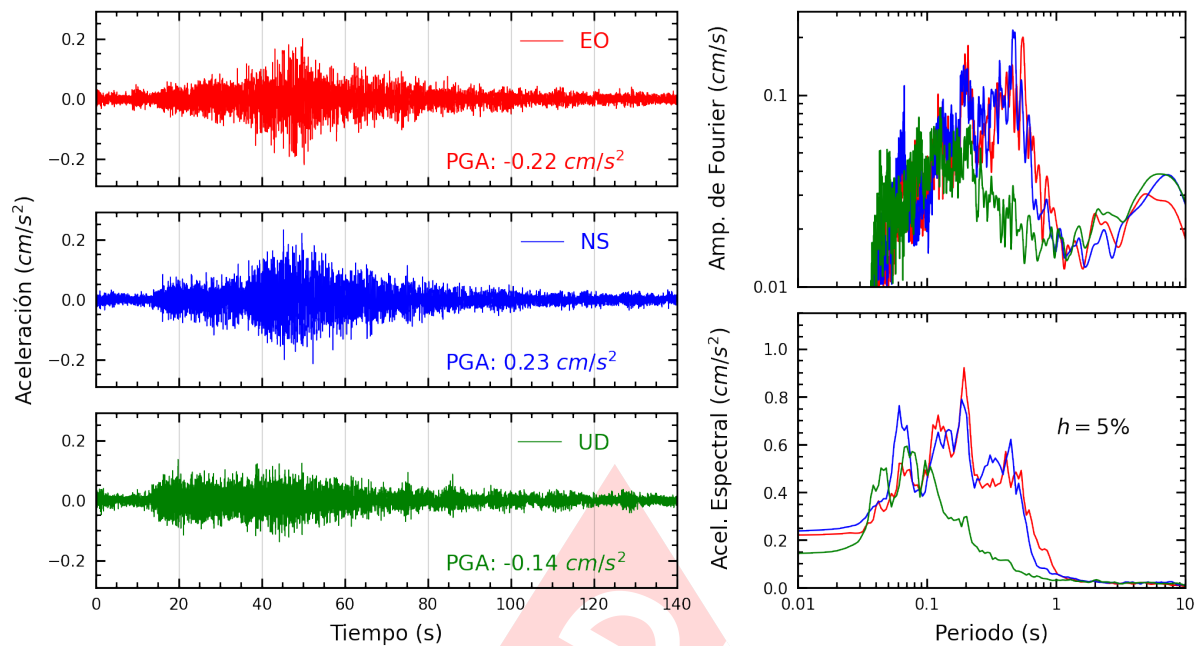
Figura A.17: Registros tiempo-historia, espectros de Fourier y de respuesta en las direcciones EO, NS y vertical de la estación VHAYA. Sismo de Huarney, Huarney - Ancash del 2023-11-01, 01:47:05 (Hora local)
