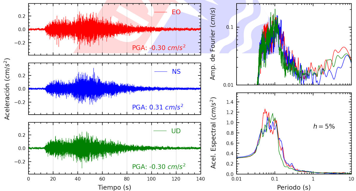
Figura A.14: Registros tiempo-historia, espectros de Fourier y de respuesta en las direcciones EO, NS y vertical de la estación AMORE. Sismo de Huarney, Huarney - Ancash del 2023-11-01, 01:47:05 (Hora local)
