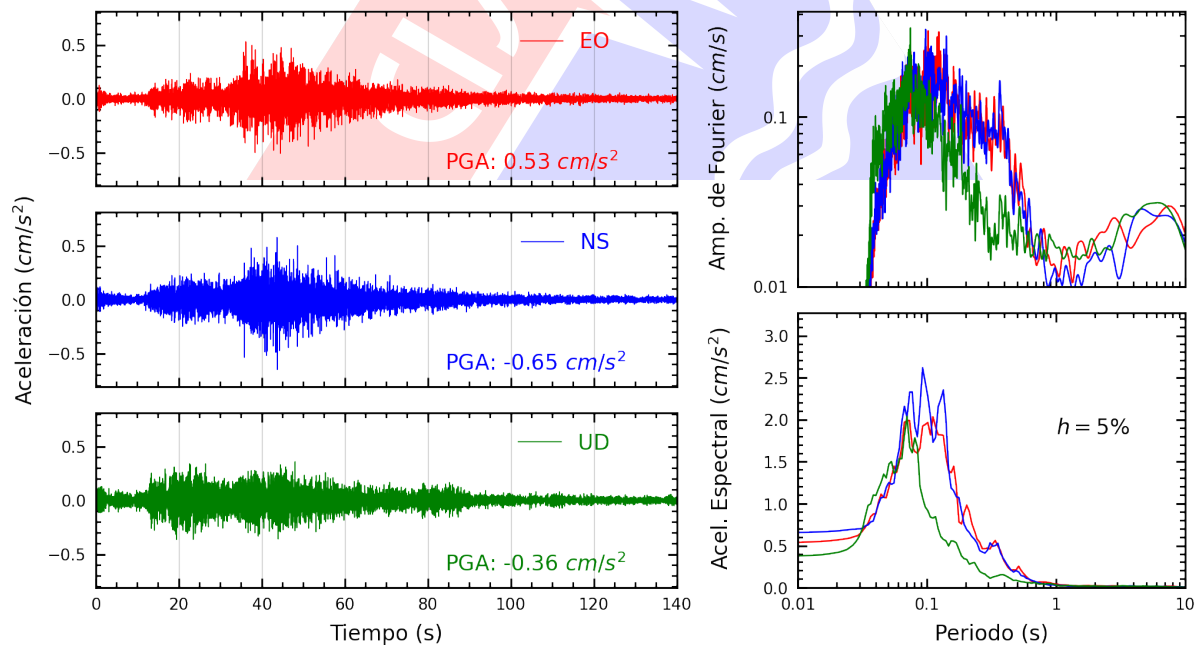
Figura A.4: Registros tiempo-historia, espectros de Fourier y de respuesta en las direcciones EO, NS y vertical de la estación ANCON. Sismo de Huarmey, Huarmey - Ancash del 2023-11-01, 01:47:05 (Hora local)
