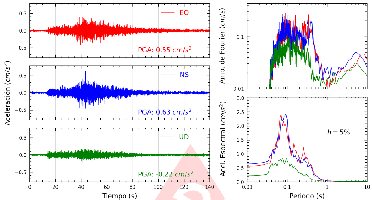
Figura A.5: Registros tiempo-historia, espectros de Fourier y de respuesta en las direcciones EO, NS y vertical de la estación DEFEN. Sismo de Huarney, Huarney - Ancash del 2023-11-01, 01:47:05 (Hora local)
