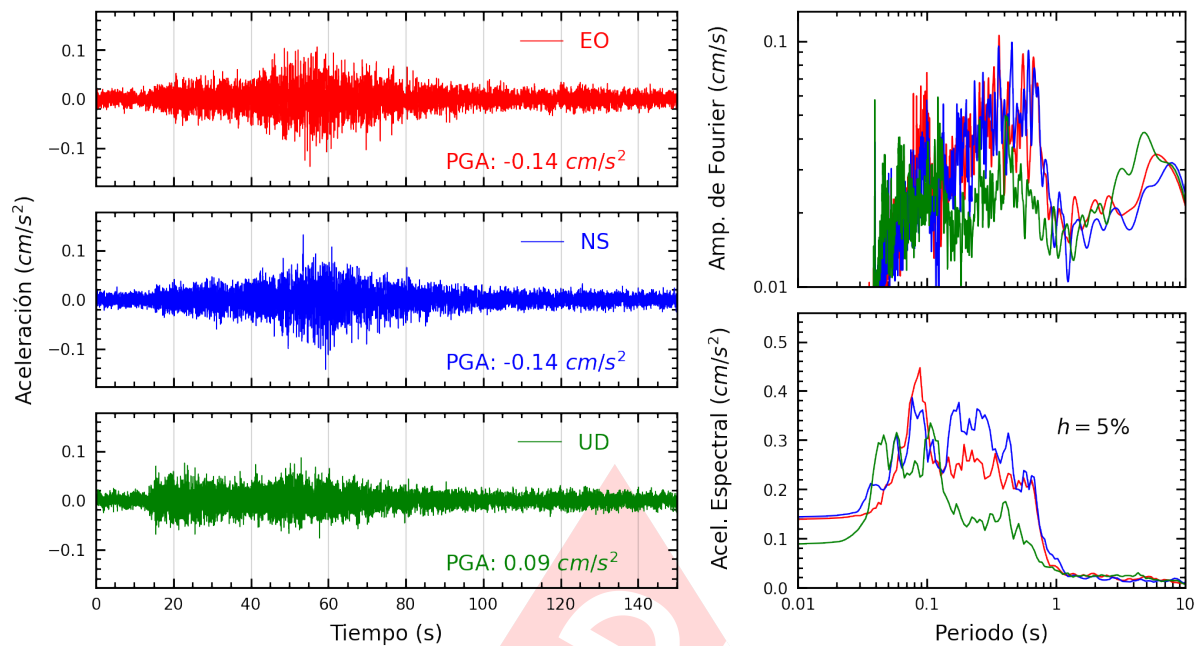
Figura A.23: Registros tiempo-historia, espectros de Fourier y de respuesta en las direcciones EO, NS y vertical de la estación USILP. Sismo de Huarmey, Huarmey - Ancash del 2023-11-01, 01:47:05 (Hora local)
