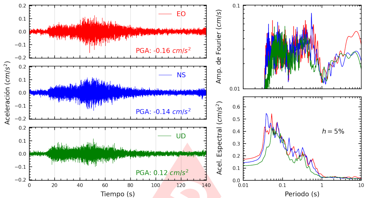
Figura A.19: Registros tiempo-historia, espectros de Fourier y de respuesta en las direcciones EO, NS y vertical de la estación COMAS. Sismo de Huarney, Huarney - Ancash del 2023-11-01, 01:47:05 (Hora local)
