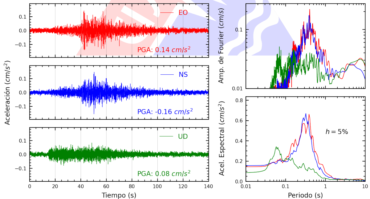
Figura A.20: Registros tiempo-historia, espectros de Fourier y de respuesta en las direcciones EO, NS y vertical de la estación ACAPU. Sismo de Huarney, Huarney - Ancash del 2023-11-01, 01:47:05 (Hora local)
