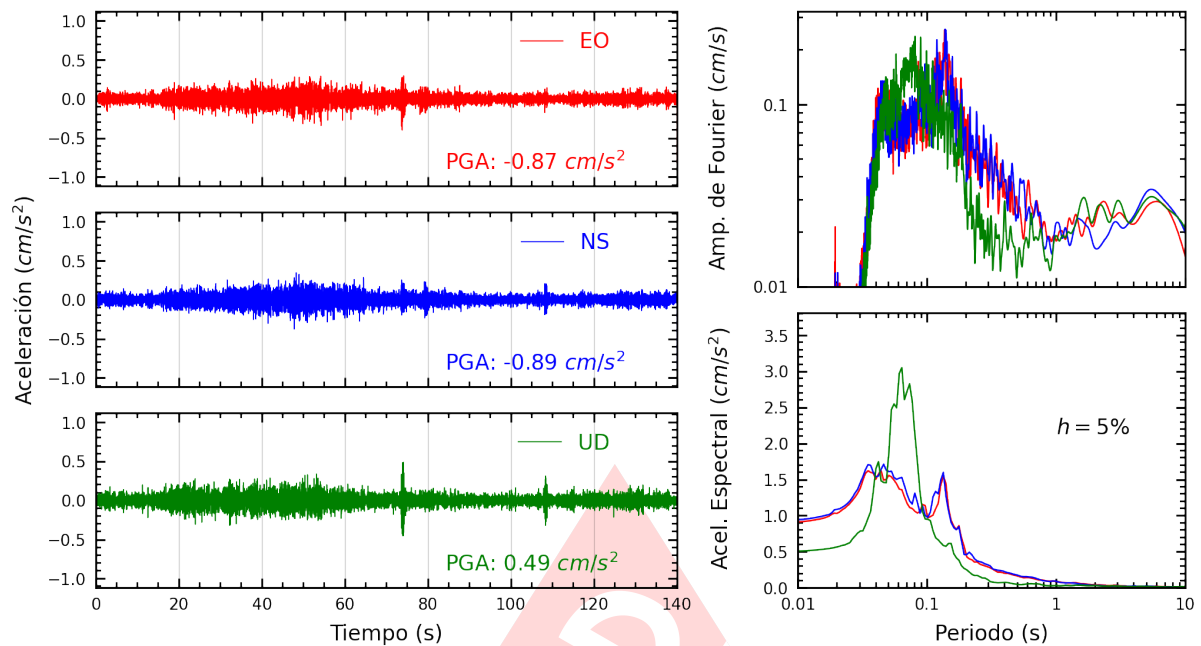
Figura A.3: Registros tiempo-historia, espectros de Fourier y de respuesta en las direcciones EO, NS y vertical de la estación CARAB. Sismo de Huarmey, Huarmey - Ancash del 2023-11-01, 01:47:05 (Hora local)
