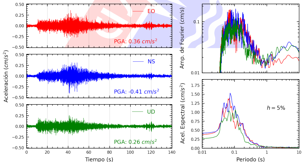
Figura A.10: Registros tiempo-historia, espectros de Fourier y de respuesta en las direcciones EO, NS y vertical de la estación INDEP. Sismo de Huarmey, Huarmey - Ancash del 2023-11-01, 01:47:05 (Hora local)
