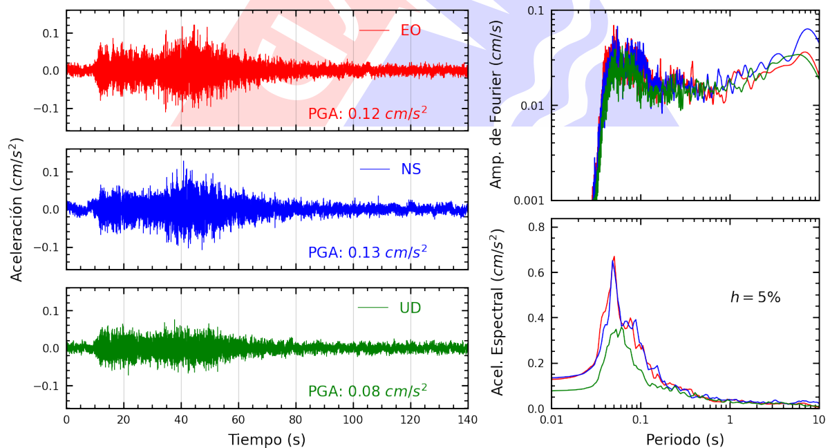
Figura A.24: Registros tiempo-historia, espectros de Fourier y de respuesta en las direcciones EO, NS y vertical de la estación UCSS. Sismo de Huarmey, Huarmey - Ancash del 2023-11-01, 01:47:05 (Hora local)
