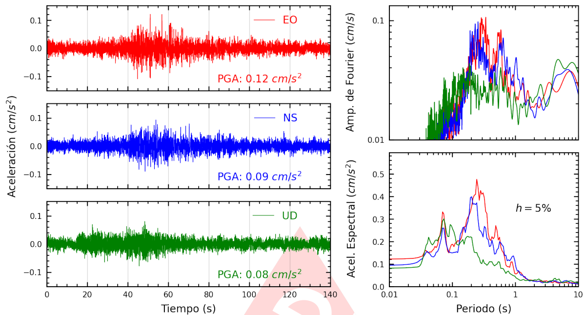
Figura A.25: Registros tiempo-historia, espectros de Fourier y de respuesta en las direcciones EO, NS y vertical de la estación DSML. Sismo de Huarney, Huarney - Ancash del 2023-11-01, 01:47:05 (Hora local)
