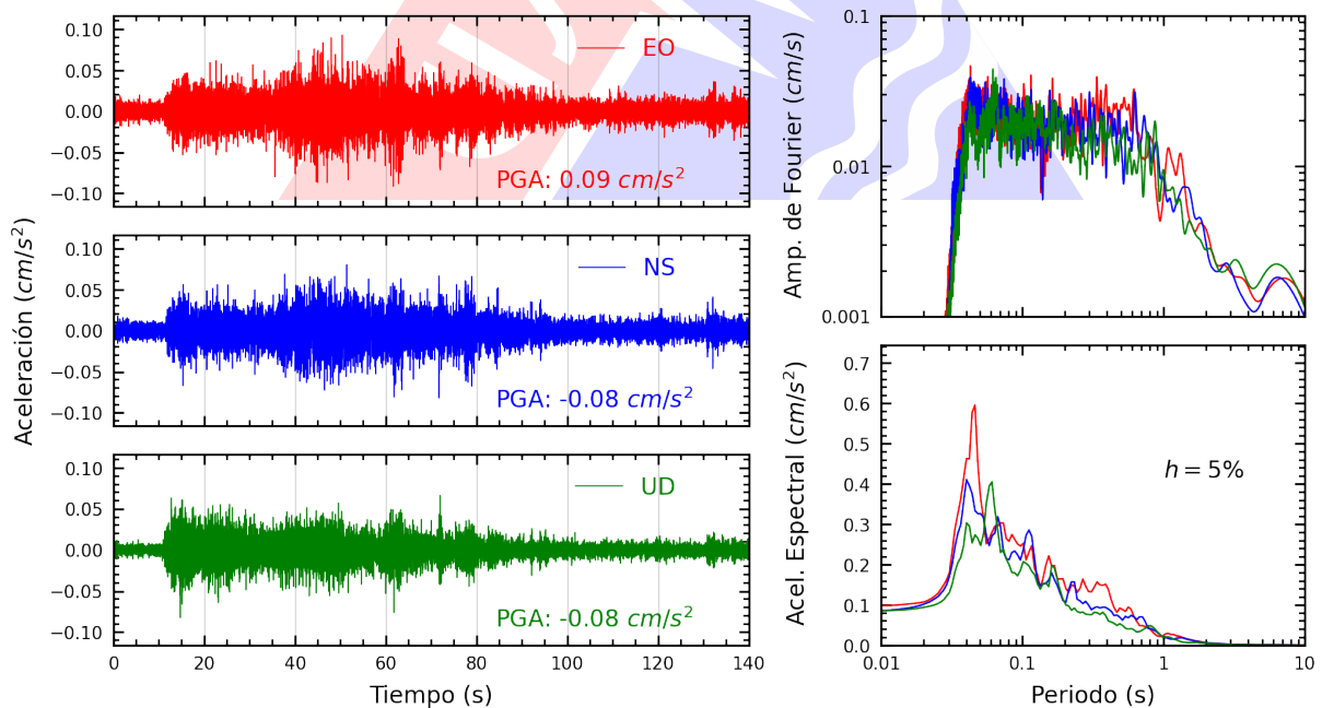
Figura A.28: Registros tiempo-historia, espectros de Fourier y de respuesta en las direcciones EO, NS y vertical de la estación BORJA. Sismo de Huarney, Huarney - Ancash del 2023-11-01, 01:47:05 (Hora local)
