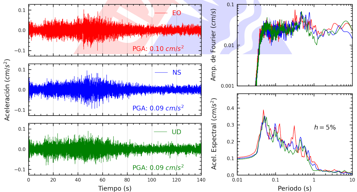
Figura A.26: Registros tiempo-historia, espectros de Fourier y de respuesta en las direcciones EO, NS y vertical de la estación IMCA. Sismo de Huarney, Huarney - Ancash del 2023-11-01, 01:47:05 (Hora local)
