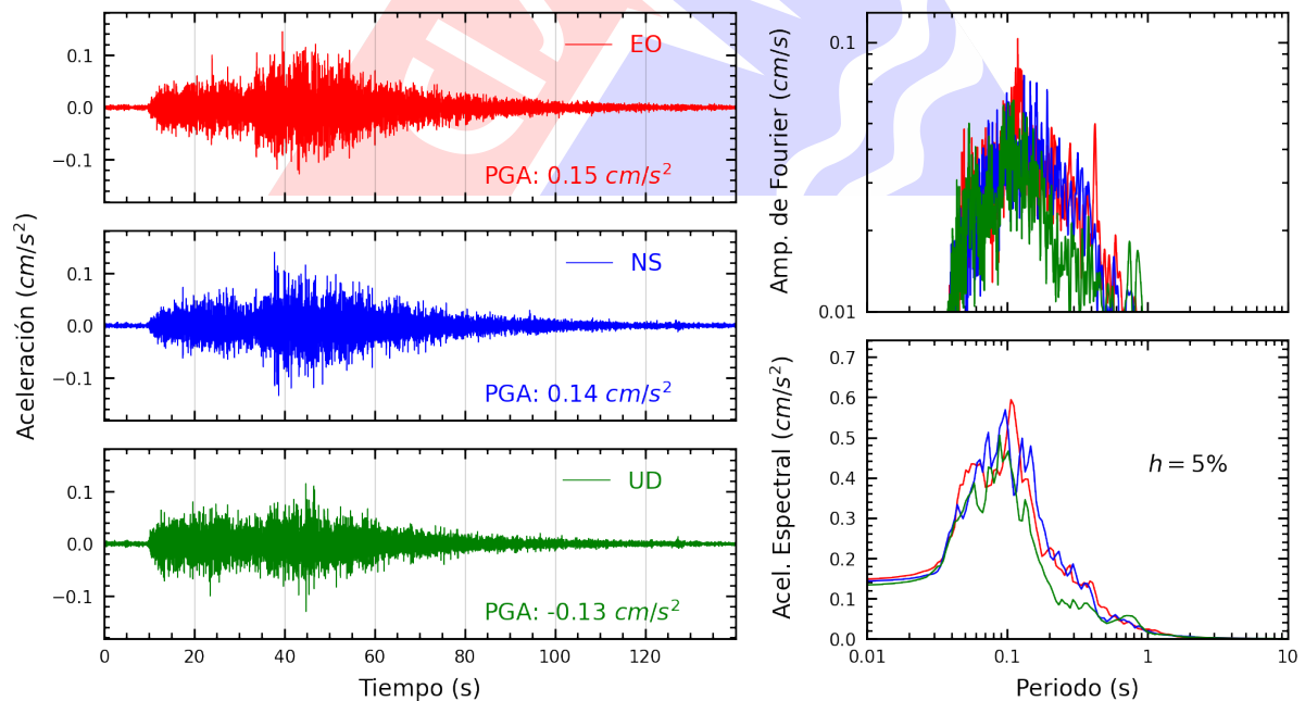
Figura A.22: Registros tiempo-historia, espectros de Fourier y de respuesta en las direcciones EO, NS y vertical de la estación JALV2. Sismo de Huarney, Huarney - Ancash del 2023-11-01, 01:47:05 (Hora local)
