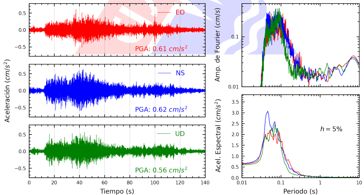
Figura A.6: Registros tiempo-historia, espectros de Fourier y de respuesta en las direcciones EO, NS y vertical de la estación SROSA. Sismo de Huarney, Huarney - Ancash del 2023-11-01, 01:47:05 (Hora local)
