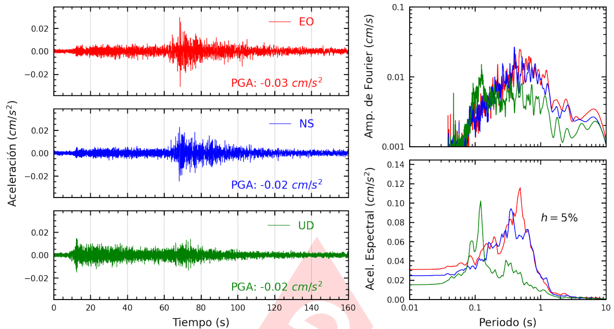
Figura A.33: Registros tiempo-historia, espectros de Fourier y de respuesta en las direcciones EO, NS y vertical de la estación UNIA. Sismo de Huarney, Huarney - Ancash del 2023-11-01, 01:47:05 (Hora local)
