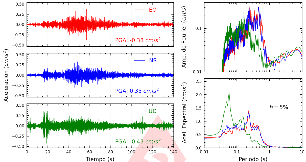
Figura A.9: Registros tiempo-historia, espectros de Fourier y de respuesta en las direcciones EO, NS y vertical de la estación MDPP. Sismo de Huarmey, Huarmey - Ancash del 2023-11-01, 01:47:05 (Hora local)
