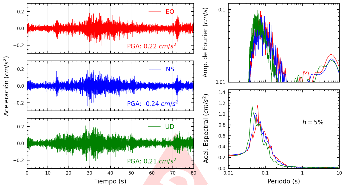
Figura A.15: Registros tiempo-historia, espectros de Fourier y de respuesta en las direcciones EO, NS y vertical de la estación ANCON. Sismo de Chilca, Cañete - Lima del 2023-12-08, 00:06:48 (Hora local)
