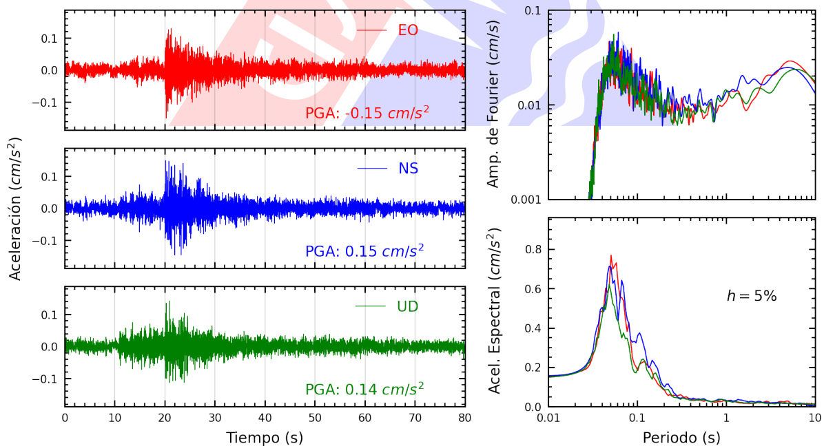
Figura A.24: Registros tiempo-historia, espectros de Fourier y de respuesta en las direcciones EO, NS y vertical de la estación CENEP. Sismo de Chilca, Cañete - Lima del 2023-12-08, 00:06:48 (Hora local)
