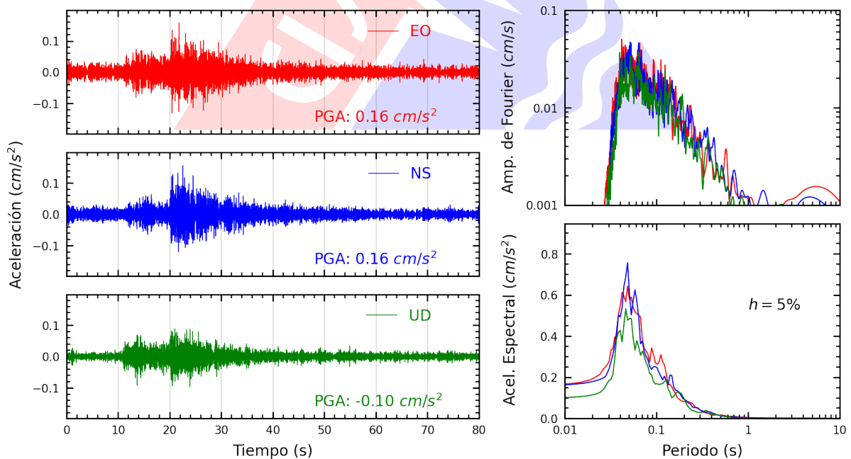
Figura A.22: Registros tiempo-historia, espectros de Fourier y de respuesta en las direcciones EO, NS y vertical de la estación BORJA. Sismo de Chilca, Cañete - Lima del 2023-12-08, 00:06:48 (Hora local)
