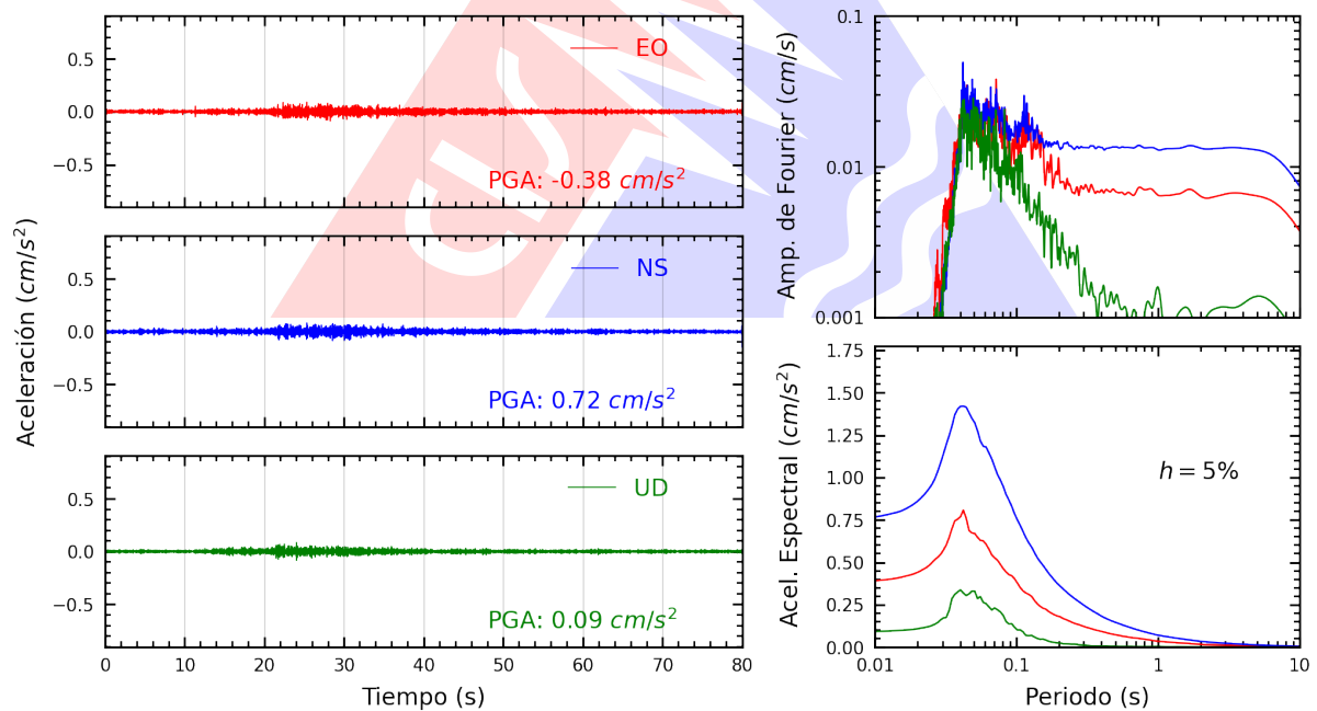
Figura A.2: Registros tiempo-historia, espectros de Fourier y de respuesta en las direcciones EO, NS y vertical de la estación ATARJ. Sismo de Chilca, Cañete - Lima del 2023-12-08, 00:06:48 (Hora local)
