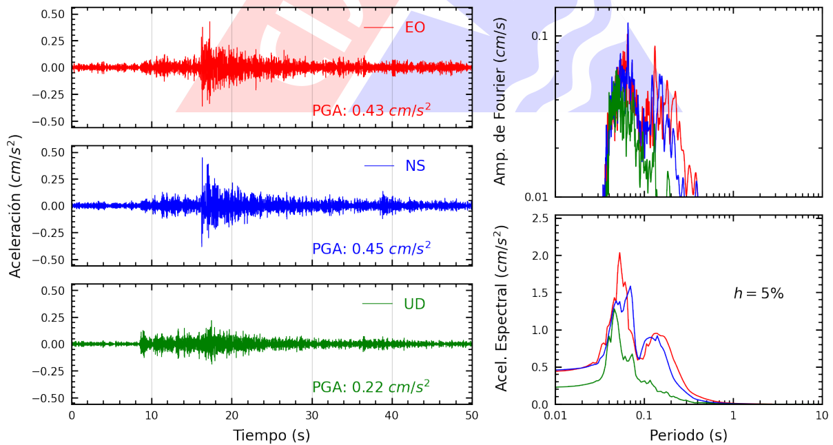
Figura A.8: Registros tiempo-historia, espectros de Fourier y de respuesta en las direcciones EO, NS y vertical de la estación PACHA. Sismo de Chilca, Cañete - Lima del 2023-12-08, 00:06:48 (Hora local)
