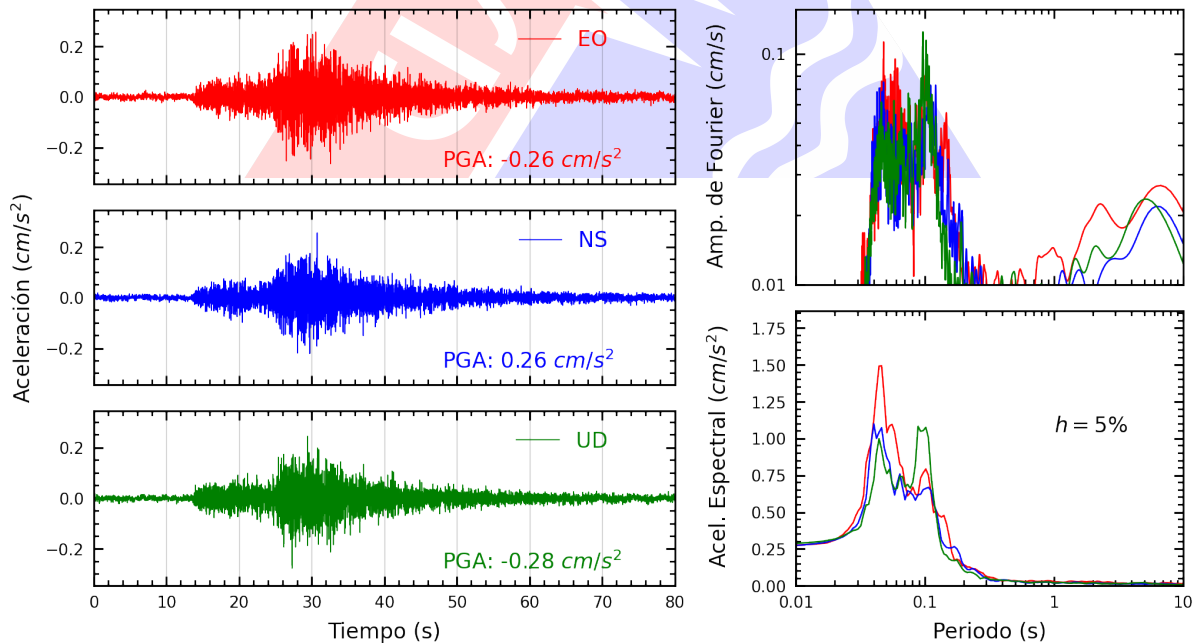
Figura A.12: Registros tiempo-historia, espectros de Fourier y de respuesta en las direcciones EO, NS y vertical de la estación AMORE. Sismo de Chilca, Cañete - Lima del 2023-12-08, 00:06:48 (Hora local)
