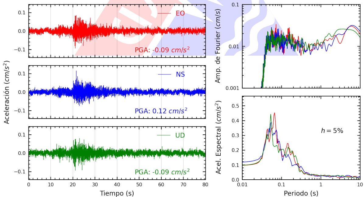
Figura A.26: Registros tiempo-historia, espectros de Fourier y de respuesta en las direcciones EO, NS y vertical de la estación UNMSM. Sismo de Chilca, Cañete - Lima del 2023-12-08, 00:06:48 (Hora local)
