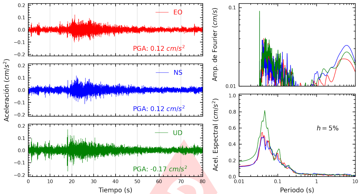
Figura A.21: Registros tiempo-historia, espectros de Fourier y de respuesta en las direcciones EO, NS y vertical de la estación USMP. Sismo de Chilca, Cañete - Lima del 2023-12-08, 00:06:48 (Hora local)
