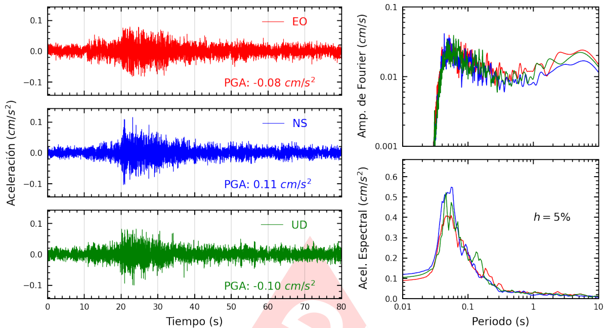
Figura A.27: Registros tiempo-historia, espectros de Fourier y de respuesta en las direcciones EO, NS y vertical de la estación IMCA. Sismo de Chilca, Cañete - Lima del 2023-12-08, 00:06:48 (Hora local)
