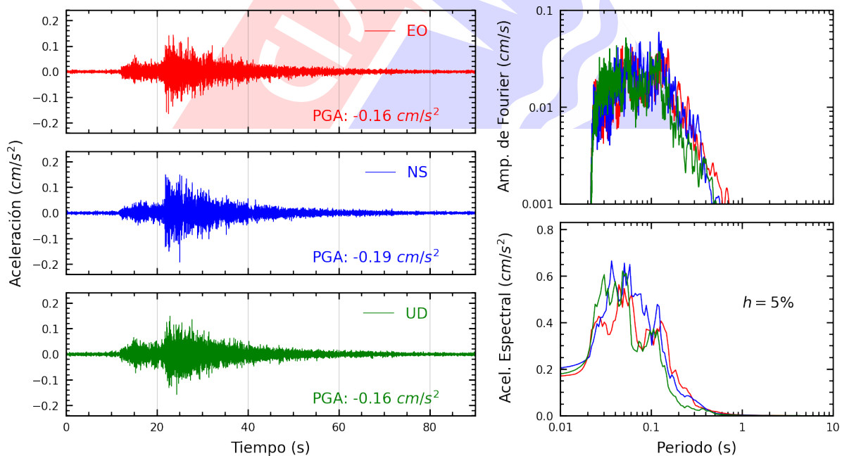
Figura A.20: Registros tiempo-historia, espectros de Fourier y de respuesta en las direcciones EO, NS y vertical de la estación JALV2. Sismo de Chilca, Cañete - Lima del 2023-12-08, 00:06:48 (Hora local)
