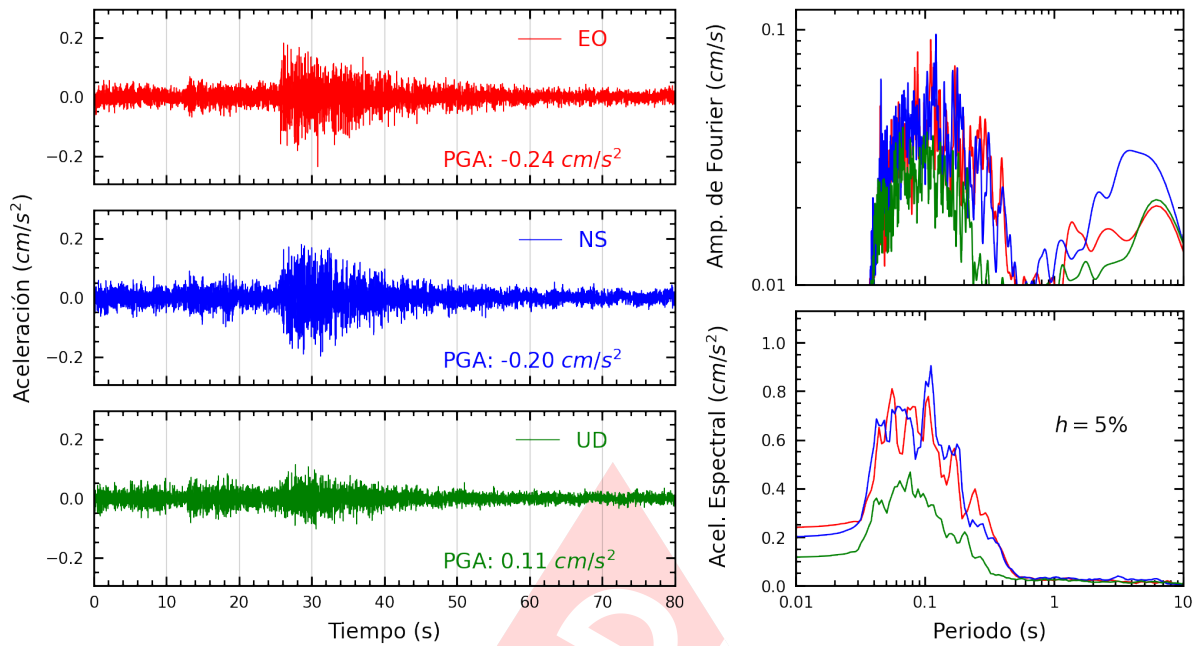
Figura A.17: Registros tiempo-historia, espectros de Fourier y de respuesta en las direcciones EO, NS y vertical de la estación DEFEN. Sismo de Chilca, Cañete - Lima del 2023-12-08, 00:06:48 (Hora local)
