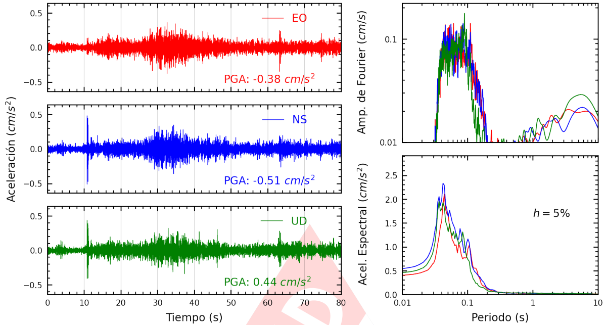
Figura A.5: Registros tiempo-historia, espectros de Fourier y de respuesta en las direcciones EO, NS y vertical de la estación SROSA. Sismo de Chilca, Cañete - Lima del 2023-12-08, 00:06:48 (Hora local)
