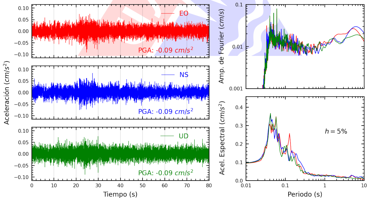
Figura A.28: Registros tiempo-historia, espectros de Fourier y de respuesta en las direcciones EO, NS y vertical de la estación BONDY. Sismo de Chilca, Cañete - Lima del 2023-12-08, 00:06:48 (Hora local)
