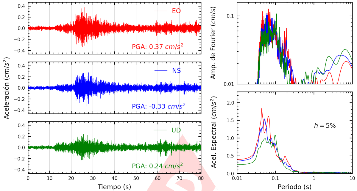
Figura A.9: Registros tiempo-historia, espectros de Fourier y de respuesta en las direcciones EO, NS y vertical de la estación INDEP. Sismo de Chilca, Cañete - Lima del 2023-12-08, 00:06:48 (Hora local)
