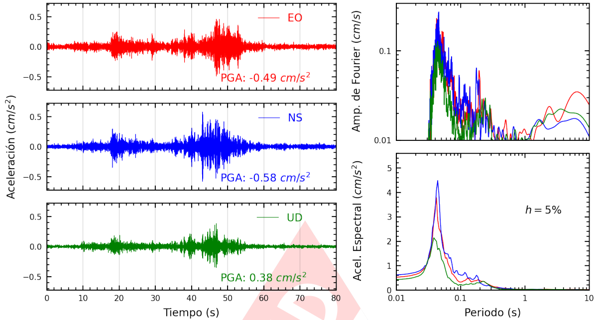
Figura A.3: Registros tiempo-historia, espectros de Fourier y de respuesta en las direcciones EO, NS y vertical de la estación UPCVI. Sismo de Chilca, Cañete - Lima del 2023-12-08, 00:06:48 (Hora local)
