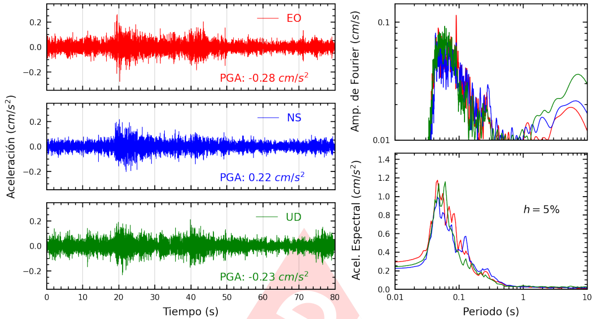
Figura A.11: Registros tiempo-historia, espectros de Fourier y de respuesta en las direcciones EO, NS y vertical de la estación URPE. Sismo de Chilca, Cañete - Lima del 2023-12-08, 00:06:48 (Hora local)
