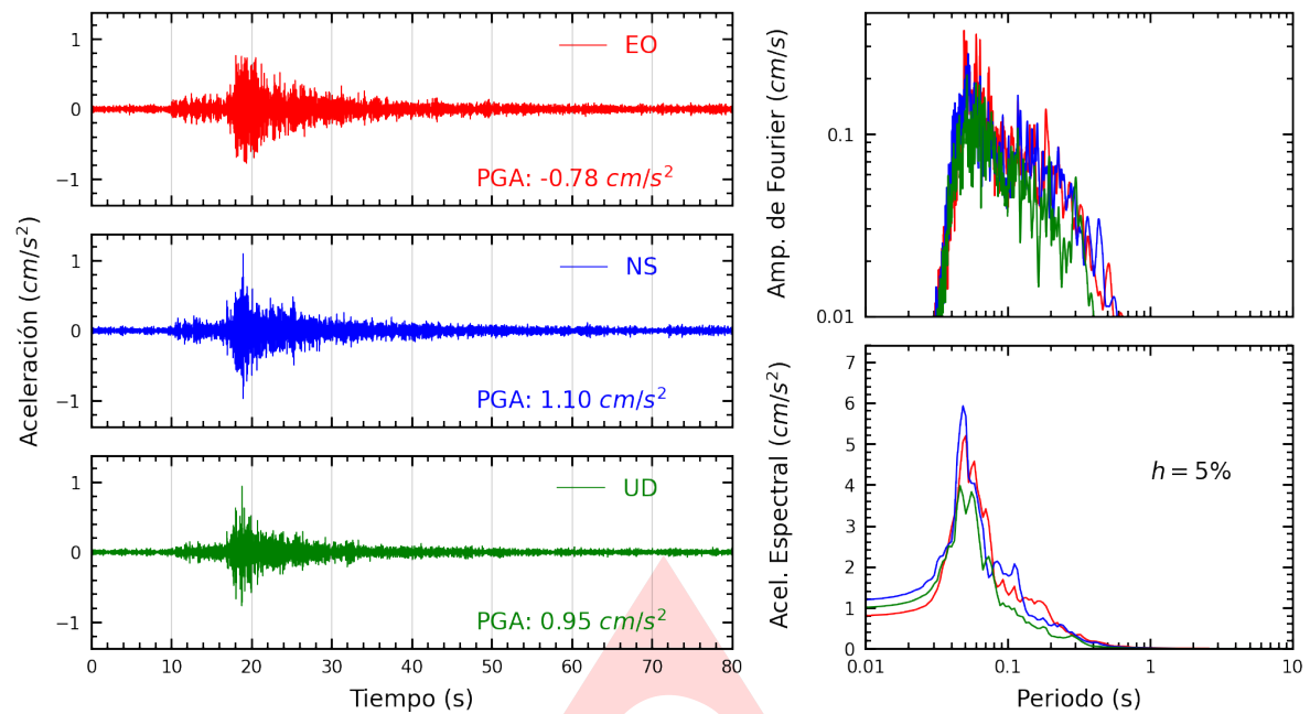
Figura A.1: Registros tiempo-historia, espectros de Fourier y de respuesta en las direcciones EO, NS y vertical de la estación UNTEL. Sismo de Chilca, Cañete - Lima del 2023-12-08, 00:06:48 (Hora local)
