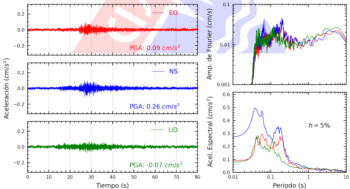
Figura A.14: Registros tiempo-historia, espectros de Fourier y de respuesta en las direcciones EO, NS y vertical de la estación VHAYA. Sismo de Chilca, Cañete - Lima del 2023-12-08, 00:06:48 (Hora local)
