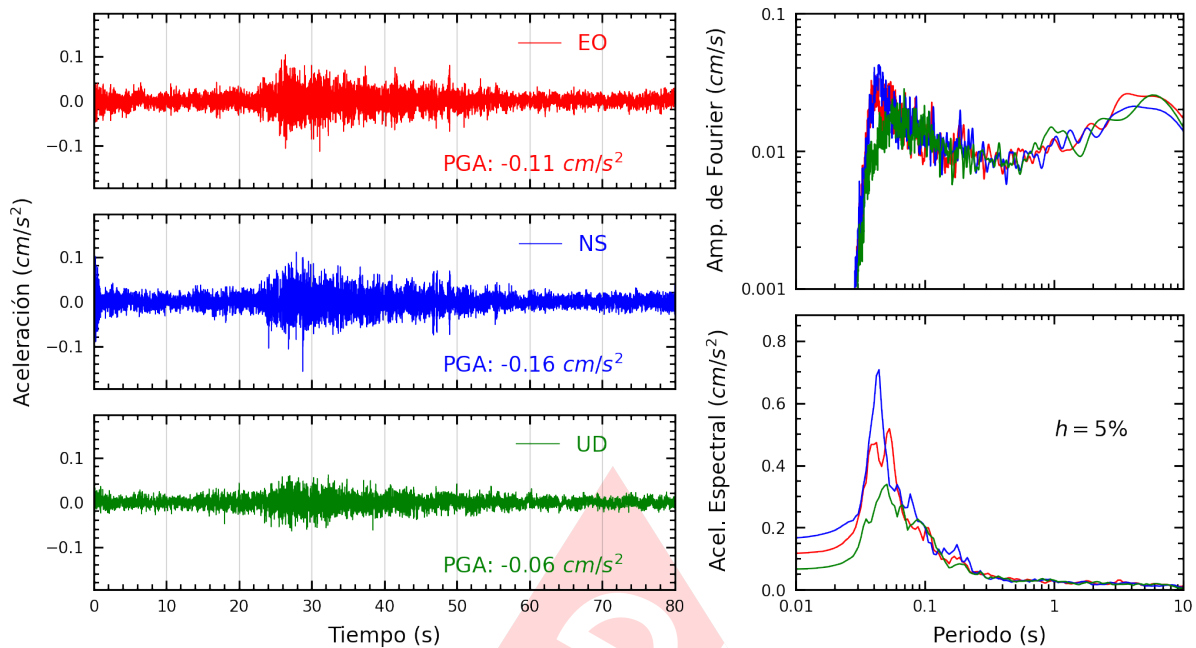
Figura A.23: Registros tiempo-historia, espectros de Fourier y de respuesta en las direcciones EO, NS y vertical de la estación COMAS. Sismo de Chilca, Cañete - Lima del 2023-12-08, 00:06:48 (Hora local)
