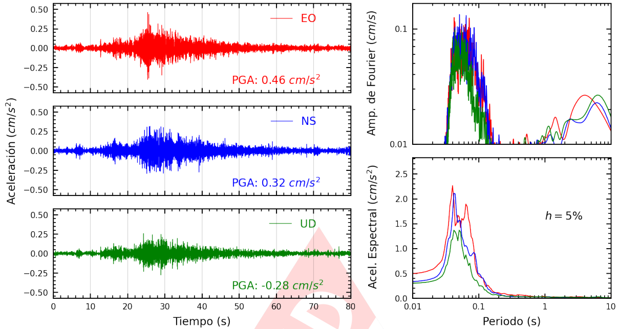
Figura A.7: Registros tiempo-historia, espectros de Fourier y de respuesta en las direcciones EO, NS y vertical de la estación JOSEO. Sismo de Chilca, Cañete - Lima del 2023-12-08, 00:06:48 (Hora local)
