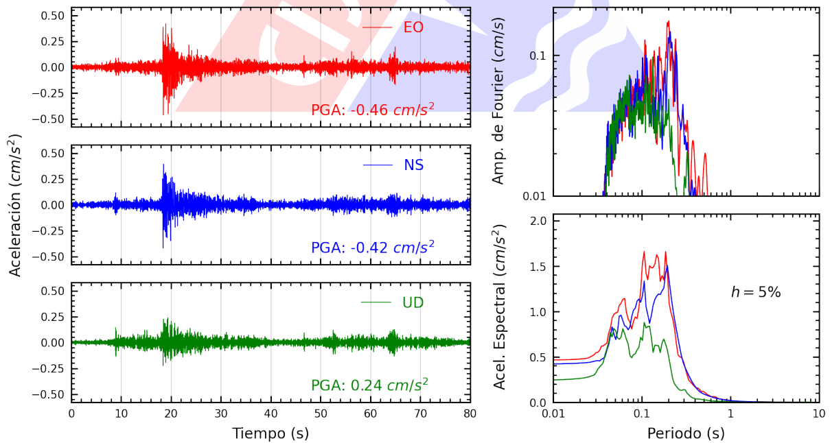
Figura A.6: Registros tiempo-historia, espectros de Fourier y de respuesta en las direcciones EO, NS y vertical de la estación SCCHO. Sismo de Chilca, Cañete - Lima del 2023-12-08, 00:06:48 (Hora local)
