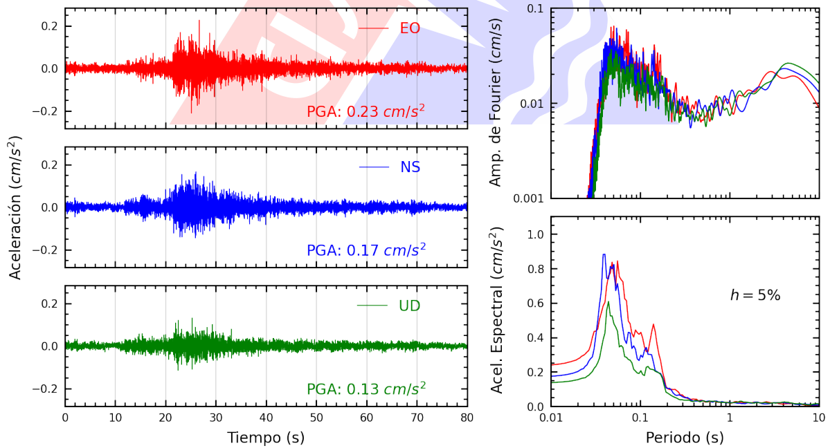
Figura A.18: Registros tiempo-historia, espectros de Fourier y de respuesta en las direcciones EO, NS y vertical de la estación FICPE. Sismo de Chilca, Cañete - Lima del 2023-12-08, 00:06:48 (Hora local)
