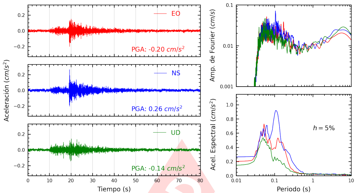
Figura A.13: Registros tiempo-historia, espectros de Fourier y de respuesta en las direcciones EO, NS y vertical de la estación SERVI. Sismo de Chilca, Cañete - Lima del 2023-12-08, 00:06:48 (Hora local)
