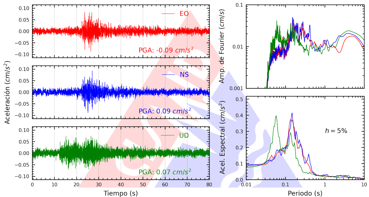
Figura A.29: Registros tiempo-historia, espectros de Fourier y de respuesta en las direcciones EO, NS y vertical de la estación ACAPU. Sismo de Chilca, Cañete - Lima del 2023-12-08, 00:06:48 (Hora local)
