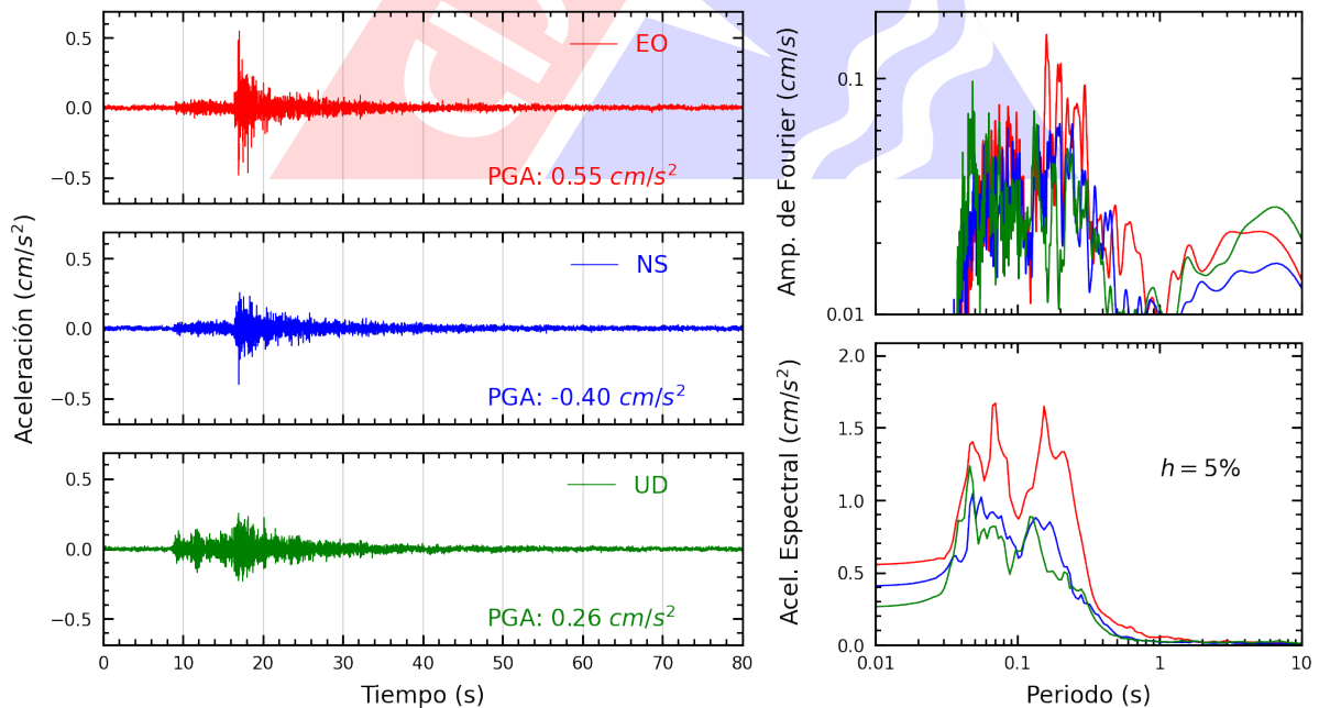
Figura A.4: Registros tiempo-historia, espectros de Fourier y de respuesta en las direcciones EO, NS y vertical de la estación USILP. Sismo de Chilca, Cañete - Lima del 2023-12-08, 00:06:48 (Hora local)
