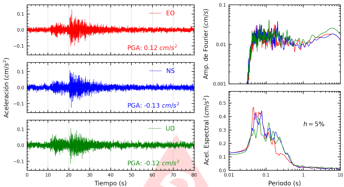
Figura A.25: Registros tiempo-historia, espectros de Fourier y de respuesta en las direcciones EO, NS y vertical de la estación UNFV. Sismo de Chilca, Cañete - Lima del 2023-12-08, 00:06:48 (Hora local)
