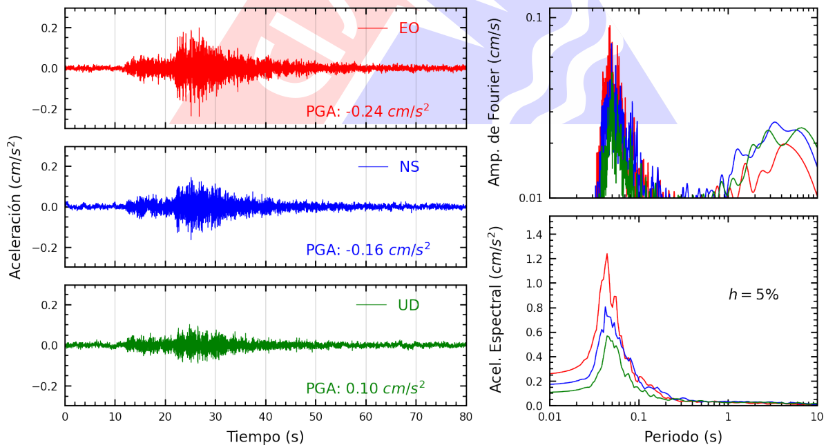
Figura A.16: Registros tiempo-historia, espectros de Fourier y de respuesta en las direcciones EO, NS y vertical de la estación UCSS. Sismo de Chilca, Cañete - Lima del 2023-12-08, 00:06:48 (Hora local)
