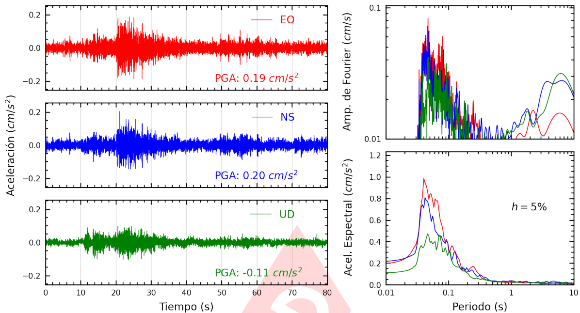
Figura A.19: Registros tiempo-historia, espectros de Fourier y de respuesta en las direcciones EO, NS y vertical de la estación CEPRE. Sismo de Chilca, Cañete - Lima del 2023-12-08, 00:06:48 (Hora local)
