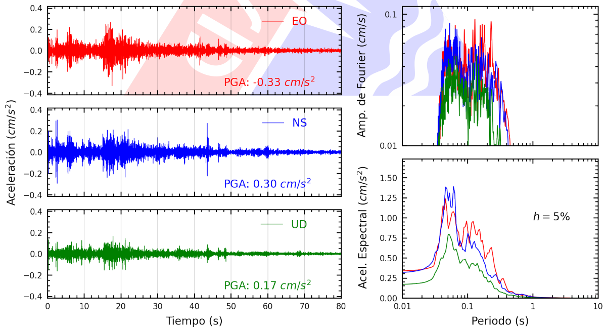
Figura A.10: Registros tiempo-historia, espectros de Fourier y de respuesta en las direcciones EO, NS y vertical de la estación BRISA. Sismo de Chilca, Cañete - Lima del 2023-12-08, 00:06:48 (Hora local)
