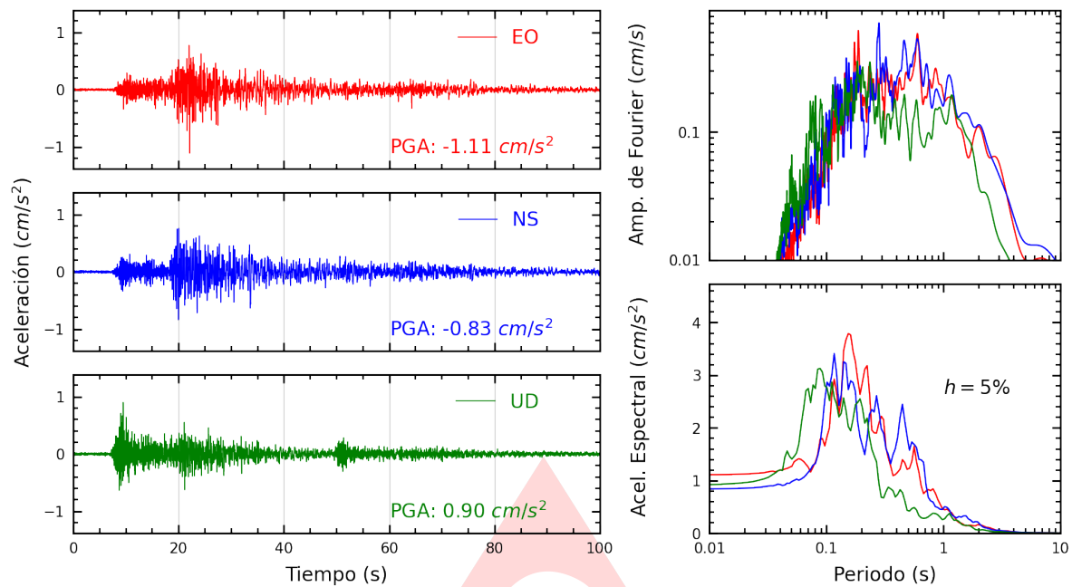
Figura A.1: Registros tiempo-historia, espectros de Fourier y de respuesta en las direcciones EO, NS y vertical de la estación UNICA. Sismo de Pisco, Pisco - Ica del 2023-12-09, 22:38:19 (Hora local)
