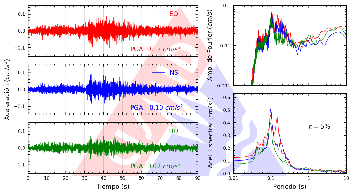
Figura A.5: Registros tiempo-historia, espectros de Fourier y de respuesta en las direcciones EO, NS y vertical de la estación AMORE. Sismo de Pisco, Pisco - Ica del 2023-12-09, 22:38:19 (Hora local)
