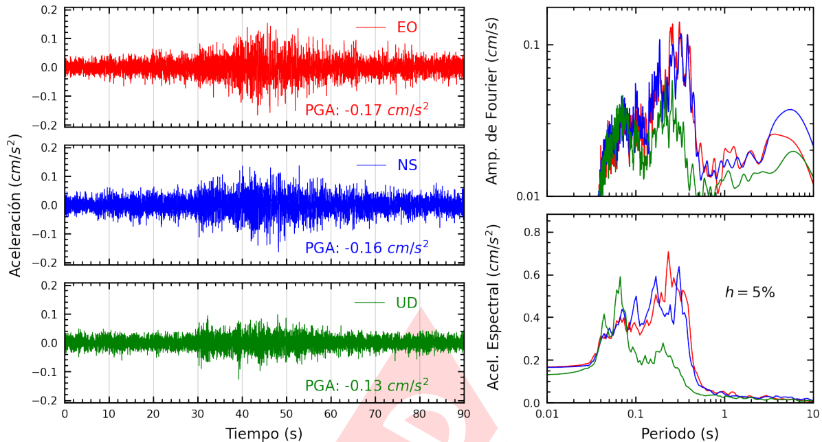
Figura A.3: Registros tiempo-historia, espectros de Fourier y de respuesta en las direcciones EO, NS y vertical de la estación DEFEN. Sismo de Pisco, Pisco - Ica del 2023-12-09, 22:38:19 (Hora local)
