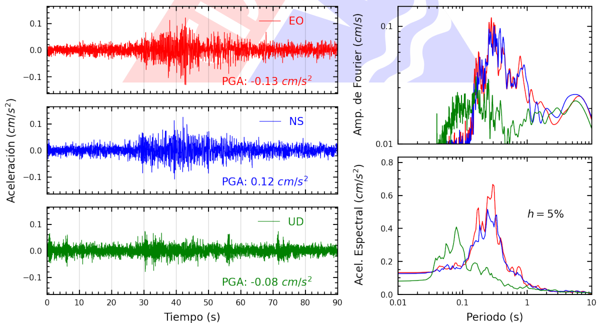
Figura A.4: Registros tiempo-historia, espectros de Fourier y de respuesta en las direcciones EO, NS y vertical de la estación ACAPU. Sismo de Pisco, Pisco - Ica del 2023-12-09, 22:38:19 (Hora local)
