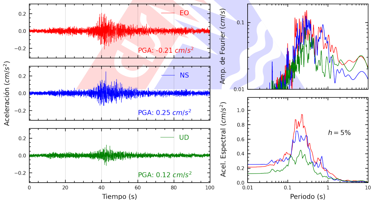
Figura A.2: Registros tiempo-historia, espectros de Fourier y de respuesta en las direcciones EO, NS y vertical de la estación USILP. Sismo de Pisco, Pisco - Ica del 2023-12-09, 22:38:19 (Hora local)
