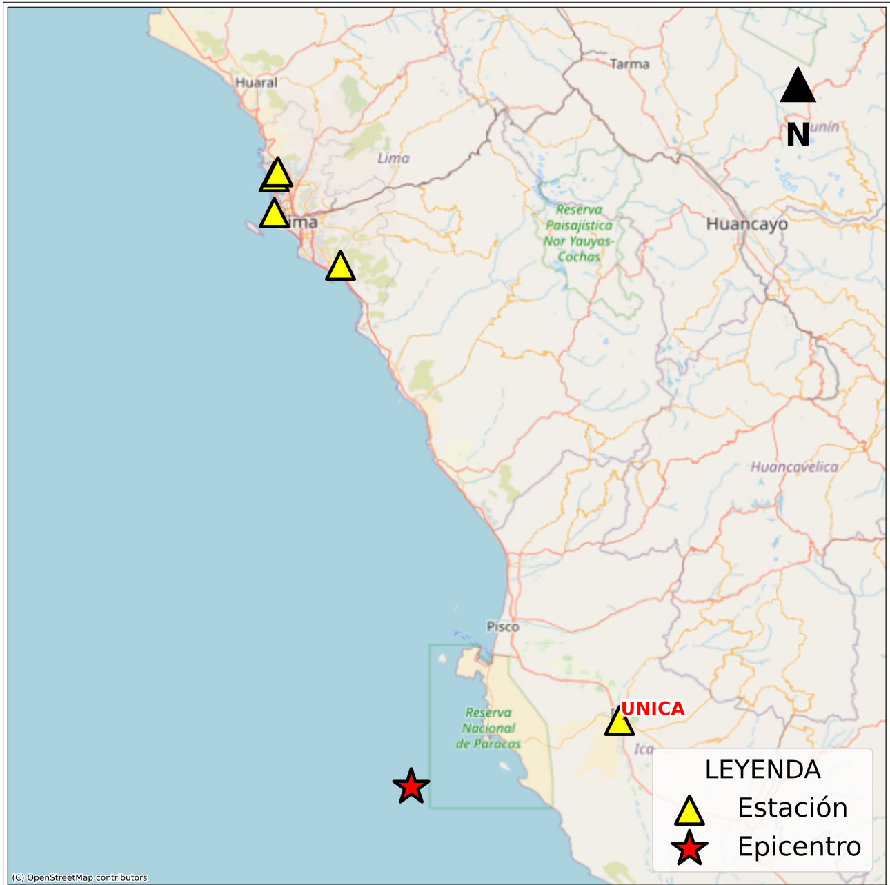
Figura 2: Mapa de ubicación de la(s) estación(es) acelerográfica(s) a nivel nacional correspondiente(s) al Sismo de Pisco, Pisco - Ica del 09 de diciembre de 2023 a las 22:38:19 (hora local)
