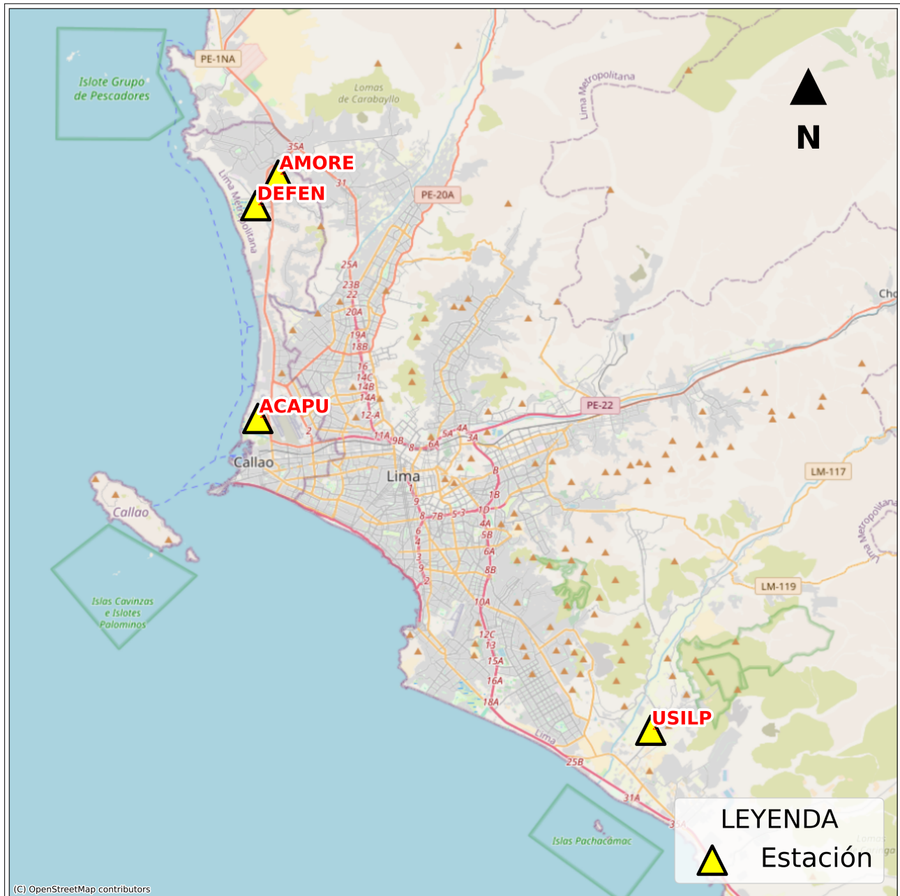
Figura 3: Mapa de ubicación de la(s) estación(es) acelerográfica(s) en Lima Metropolitana correspondiente(s) al Sismo de Pisco, Pisco - Ica del 09 de diciembre de 2023 a las 22:38:19 (hora local)
