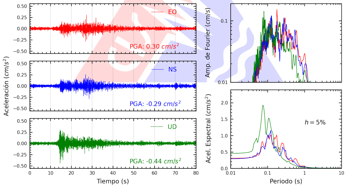
Figura A.2: Registros tiempo-historia, espectros de Fourier y de respuesta en las direcciones EO, NS y vertical de la estación UNICA. Sismo de Pisco, Pisco - Ica del 2023-12-10, 07:14:12 (Hora local)
