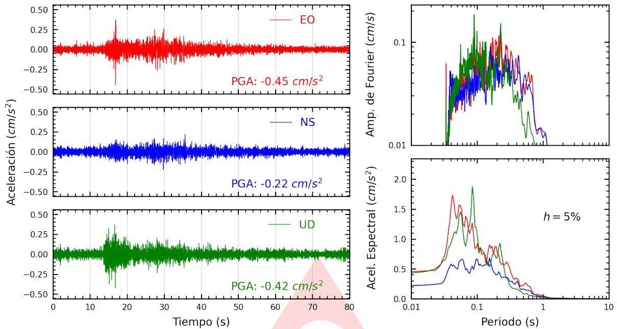
Figura A.1: Registros tiempo-historia, espectros de Fourier y de respuesta en las direcciones EO, NS y vertical de la estación SCICA. Sismo de Pisco, Pisco - Ica del 2023-12-10, 07:14:12 (Hora local)
