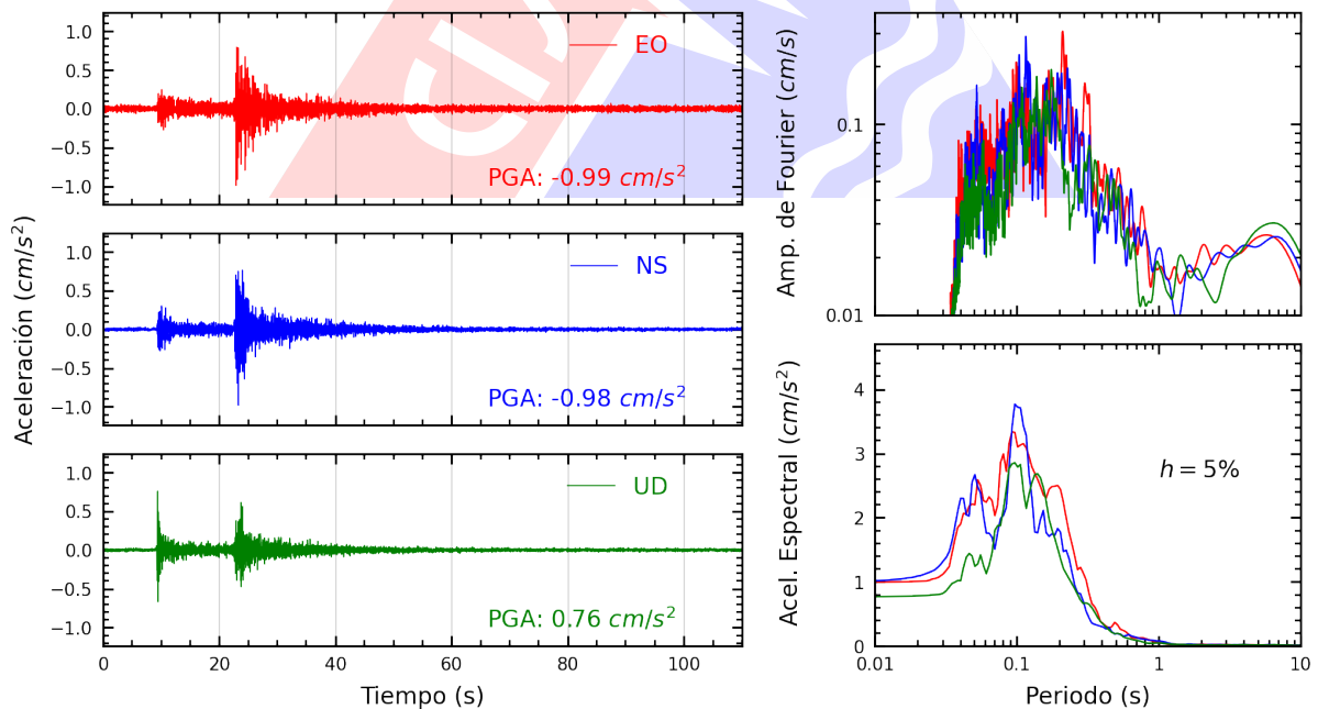
Figura A.24: Registros tiempo-historia, espectros de Fourier y de respuesta en las direcciones EO, NS y vertical de la estación INICT. Sismo de Canta, Canta - Lima del 2023-12-13, 02:38:49 (Hora local)
