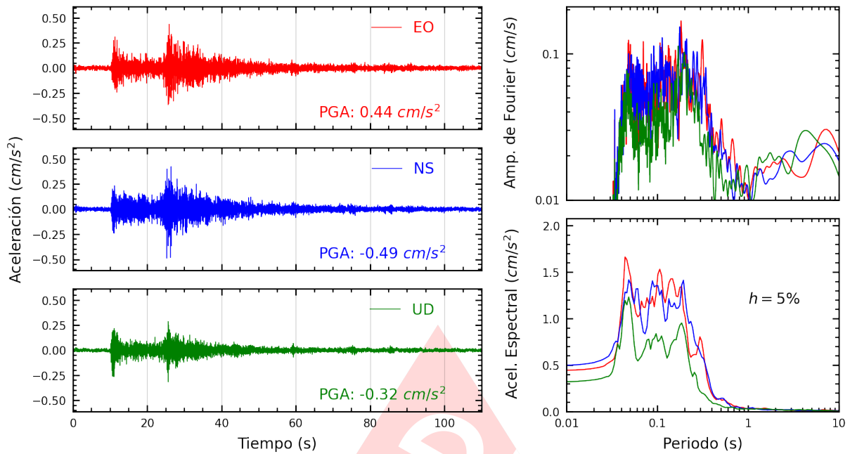
Figura A.35: Registros tiempo-historia, espectros de Fourier y de respuesta en las direcciones EO, NS y vertical de la estación UPCVI. Sismo de Canta, Canta - Lima del 2023-12-13, 02:38:49 (Hora local)
