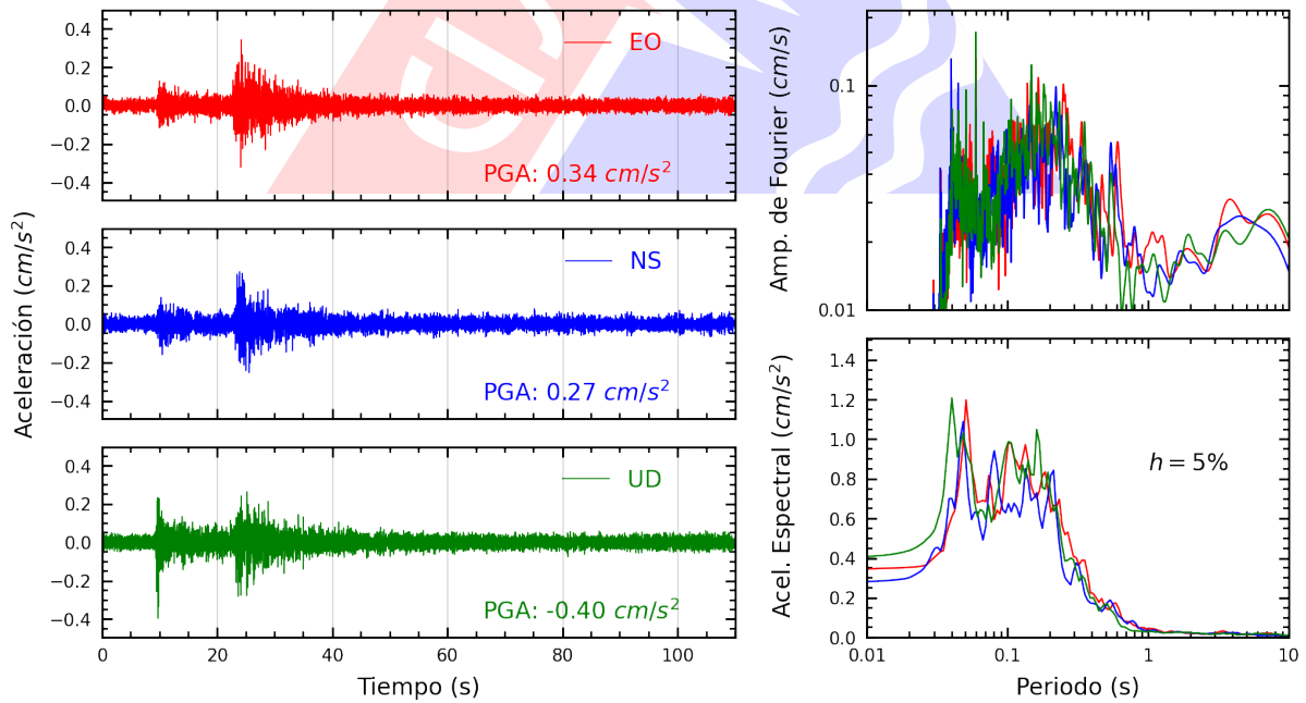
Figura A.36: Registros tiempo-historia, espectros de Fourier y de respuesta en las direcciones EO, NS y vertical de la estación BONDY. Sismo de Canta, Canta - Lima del 2023-12-13, 02:38:49 (Hora local)
