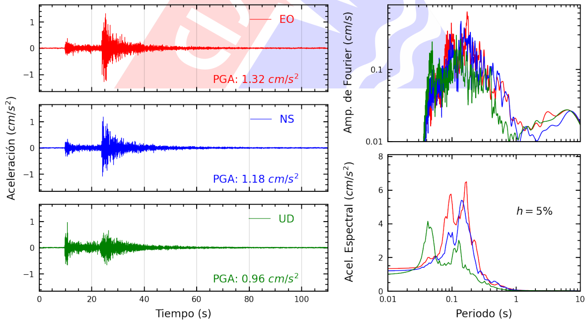
Figura A.16: Registros tiempo-historia, espectros de Fourier y de respuesta en las direcciones EO, NS y vertical de la estación USILP. Sismo de Canta, Canta - Lima del 2023-12-13, 02:38:49 (Hora local)
