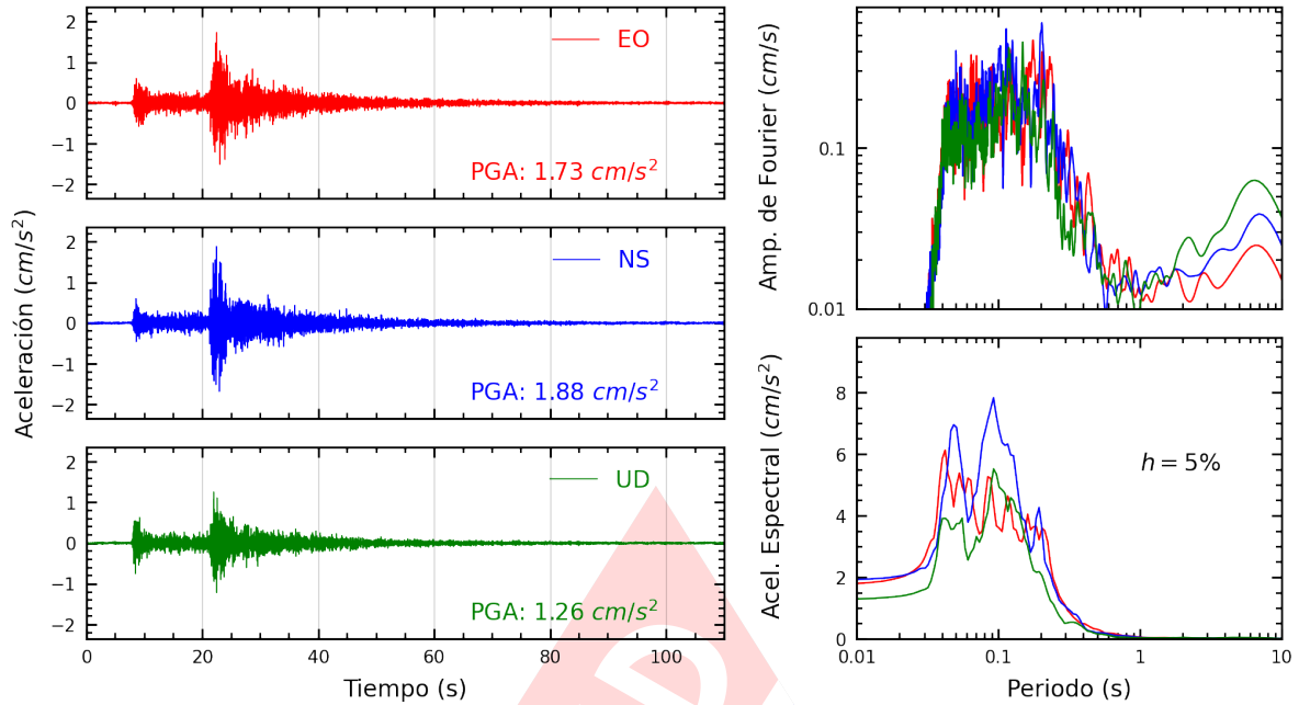
Figura A.7: Registros tiempo-historia, espectros de Fourier y de respuesta en las direcciones EO, NS y vertical de la estación INDEP. Sismo de Canta, Canta - Lima del 2023-12-13, 02:38:49 (Hora local)
