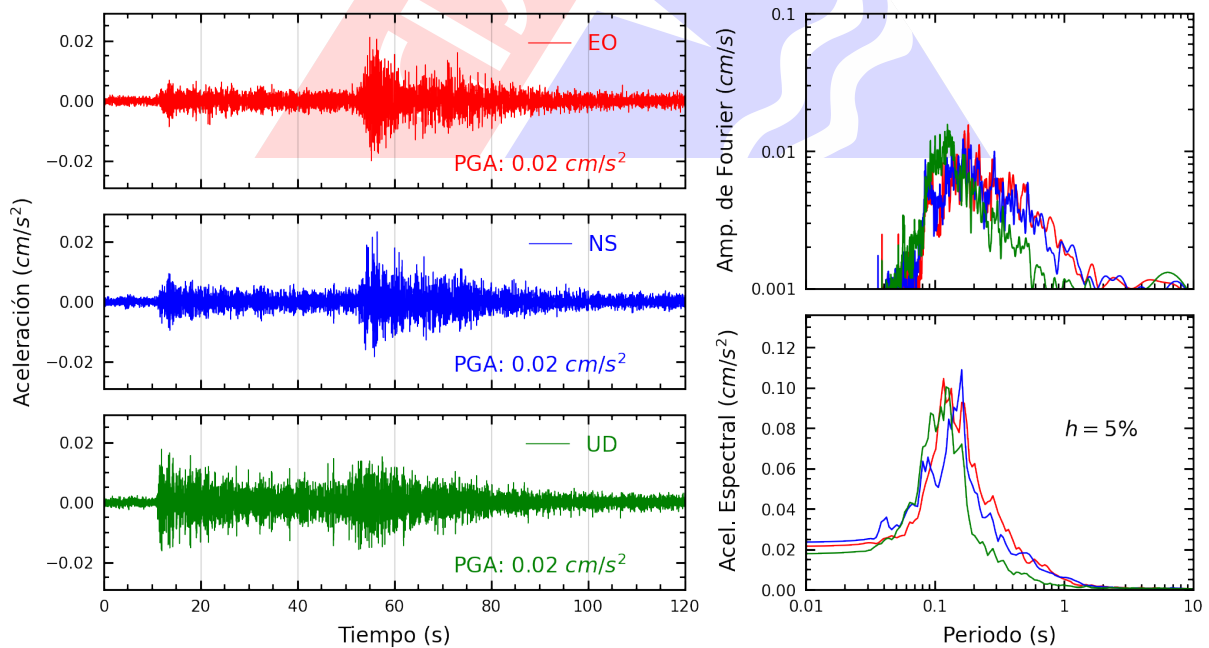
Figura A.38: Registros tiempo-historia, espectros de Fourier y de respuesta en las direcciones EO, NS y vertical de la estación UNIA. Sismo de Canta, Canta - Lima del 2023-12-13, 02:38:49 (Hora local)
