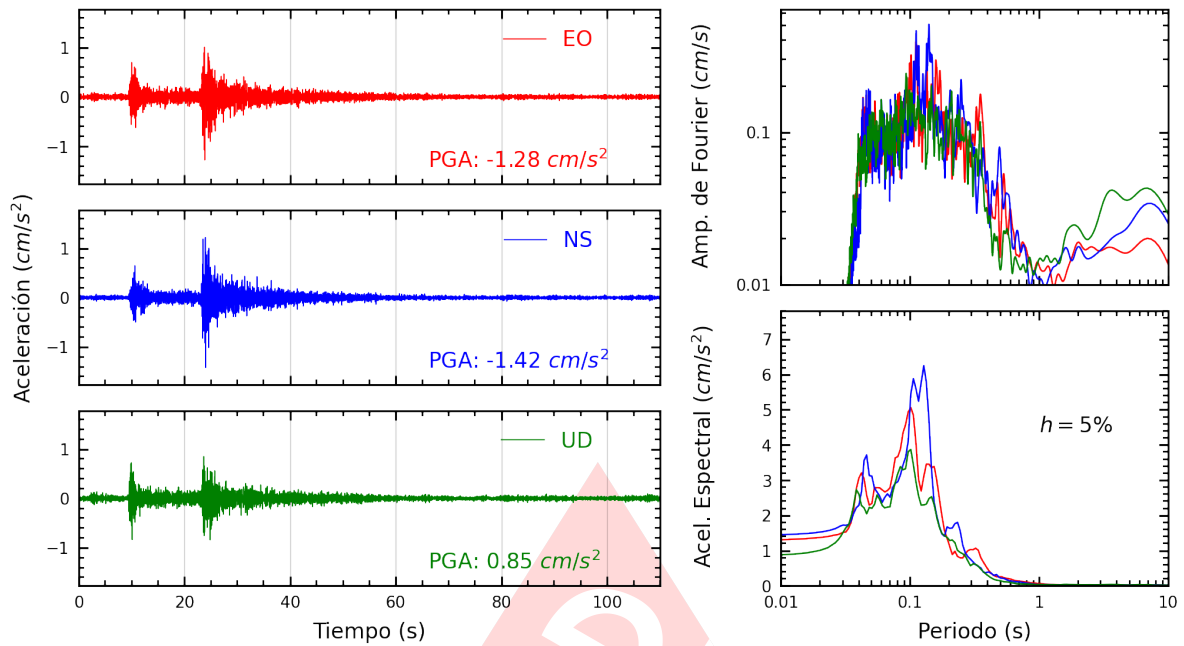
Figura A.15: Registros tiempo-historia, espectros de Fourier y de respuesta en las direcciones EO, NS y vertical de la estación URPE. Sismo de Canta, Canta - Lima del 2023-12-13, 02:38:49 (Hora local)
