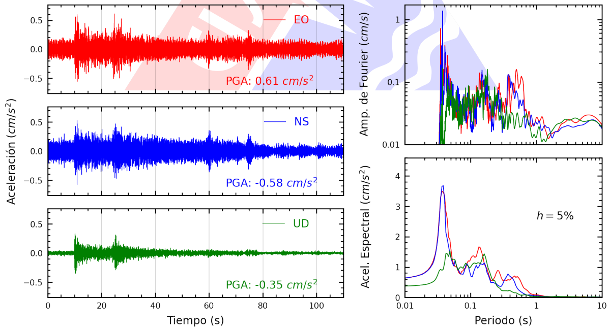
Figura A.30: Registros tiempo-historia, espectros de Fourier y de respuesta en las direcciones EO, NS y vertical de la estación DHNPE. Sismo de Canta, Canta - Lima del 2023-12-13, 02:38:49 (Hora local)
