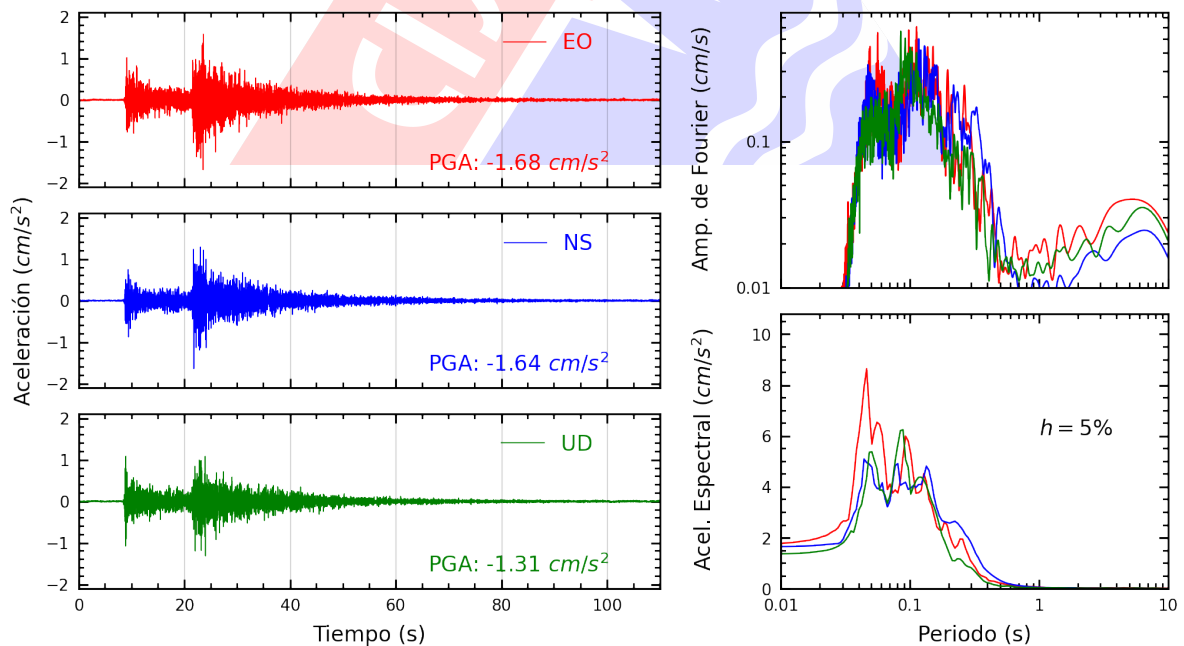
Figura A.8: Registros tiempo-historia, espectros de Fourier y de respuesta en las direcciones EO, NS y vertical de la estación AMORE. Sismo de Canta, Canta - Lima del 2023-12-13, 02:38:49 (Hora local)
