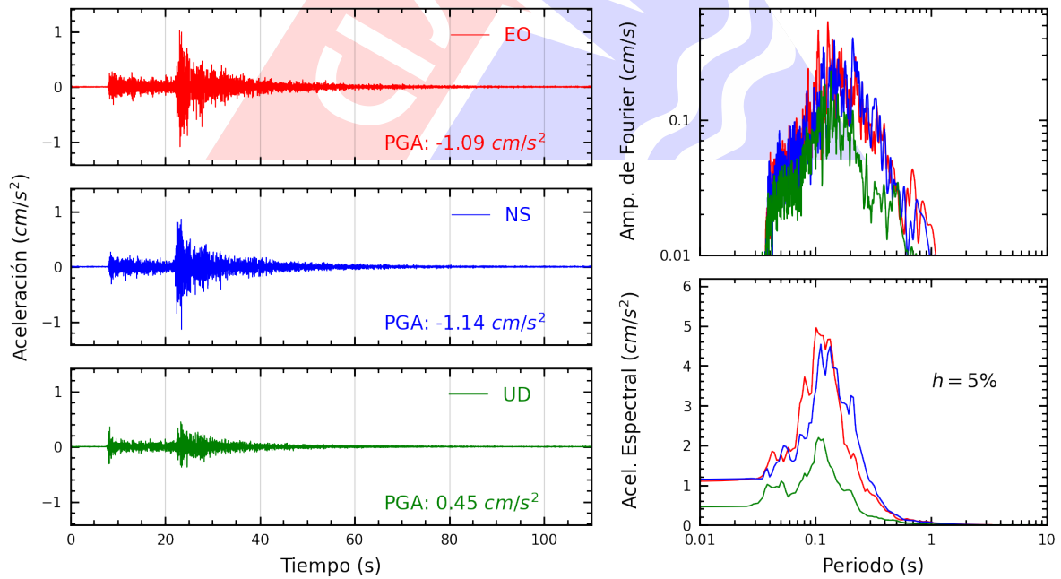
Figura A.22: Registros tiempo-historia, espectros de Fourier y de respuesta en las direcciones EO, NS y vertical de la estación BRISA. Sismo de Canta, Canta - Lima del 2023-12-13, 02:38:49 (Hora local)
