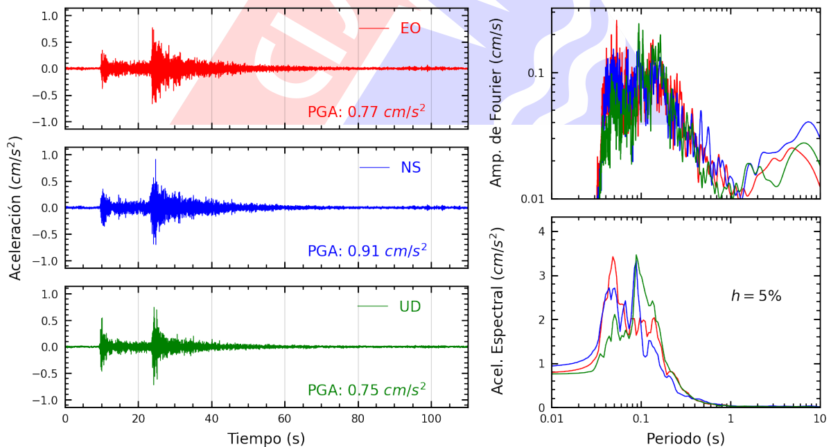
Figura A.26: Registros tiempo-historia, espectros de Fourier y de respuesta en las direcciones EO, NS y vertical de la estación CEPRE. Sismo de Canta, Canta - Lima del 2023-12-13, 02:38:49 (Hora local)
