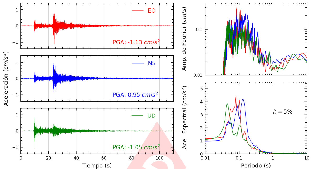
Figura A.23: Registros tiempo-historia, espectros de Fourier y de respuesta en las direcciones EO, NS y vertical de la estación CENEP. Sismo de Canta, Canta - Lima del 2023-12-13, 02:38:49 (Hora local)
