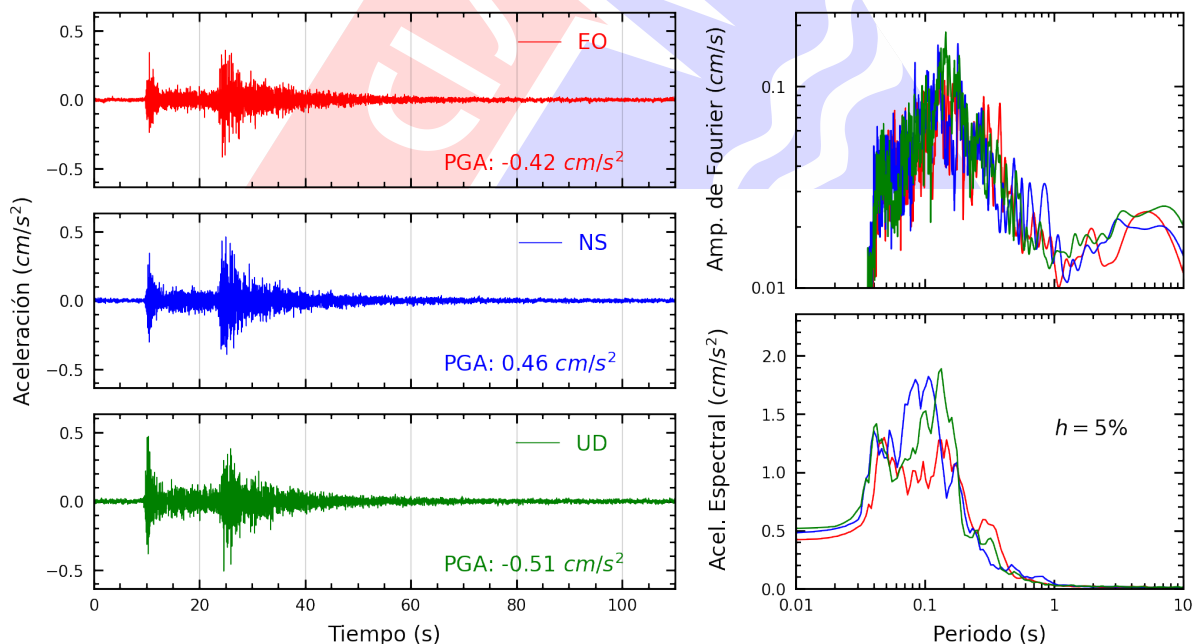
Figura A.34: Registros tiempo-historia, espectros de Fourier y de respuesta en las direcciones EO, NS y vertical de la estación UNFV. Sismo de Canta, Canta - Lima del 2023-12-13, 02:38:49 (Hora local)
