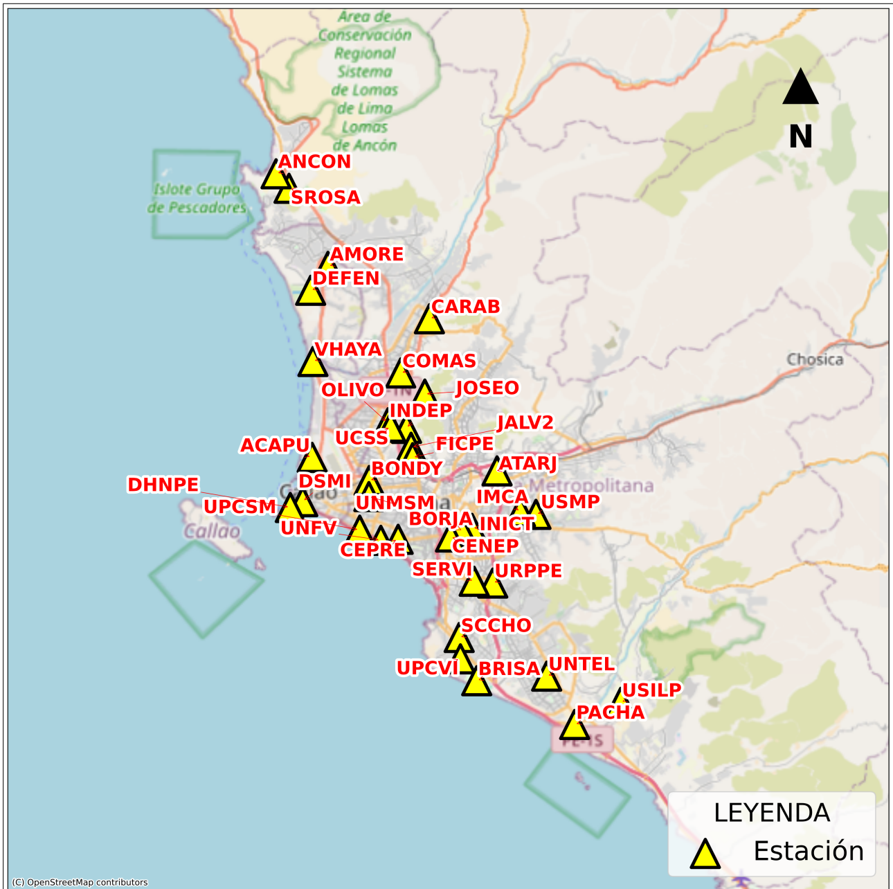
Figura 3: Mapa de ubicación de la(s) estación(es) acelerográfica(s) en Lima Metropolitana correspondiente(s) al Sismo de Canta, Canta - Lima del 13 de diciembre de 2023 a las 02:38:49 (hora local)
