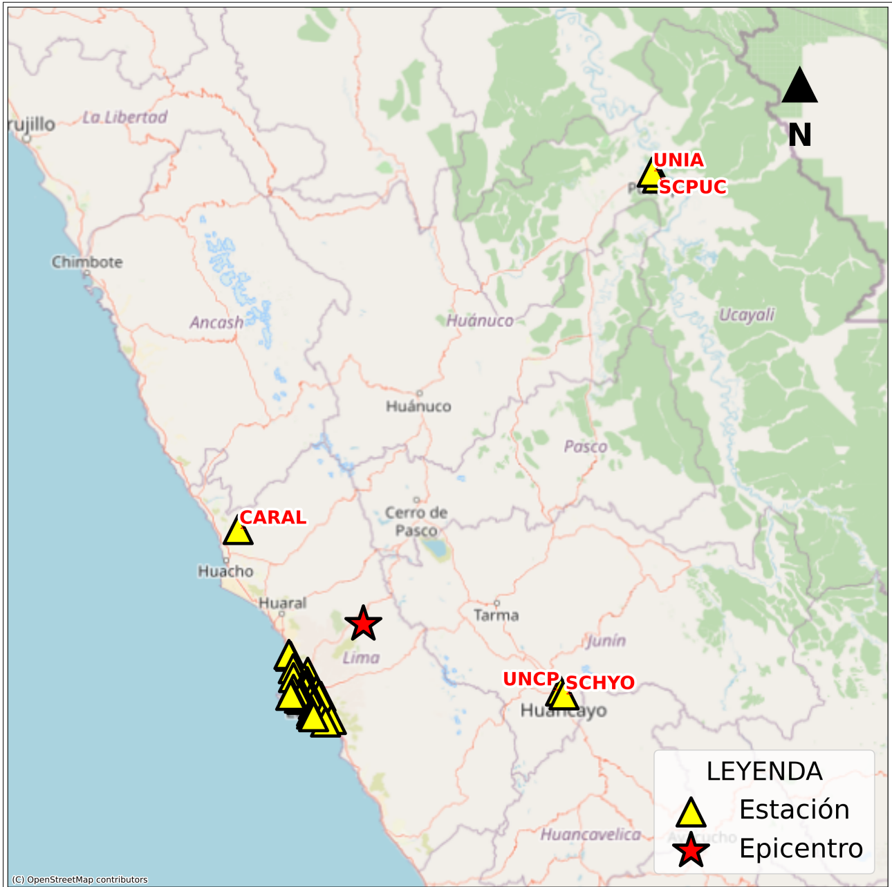
Figura 2: Mapa de ubicación de la(s) estación(es) acelerográfica(s) a nivel nacional correspondiente(s) al Sismo de Canta, Canta - Lima del 13 de diciembre de 2023 a las 02:38:49 (hora local)
