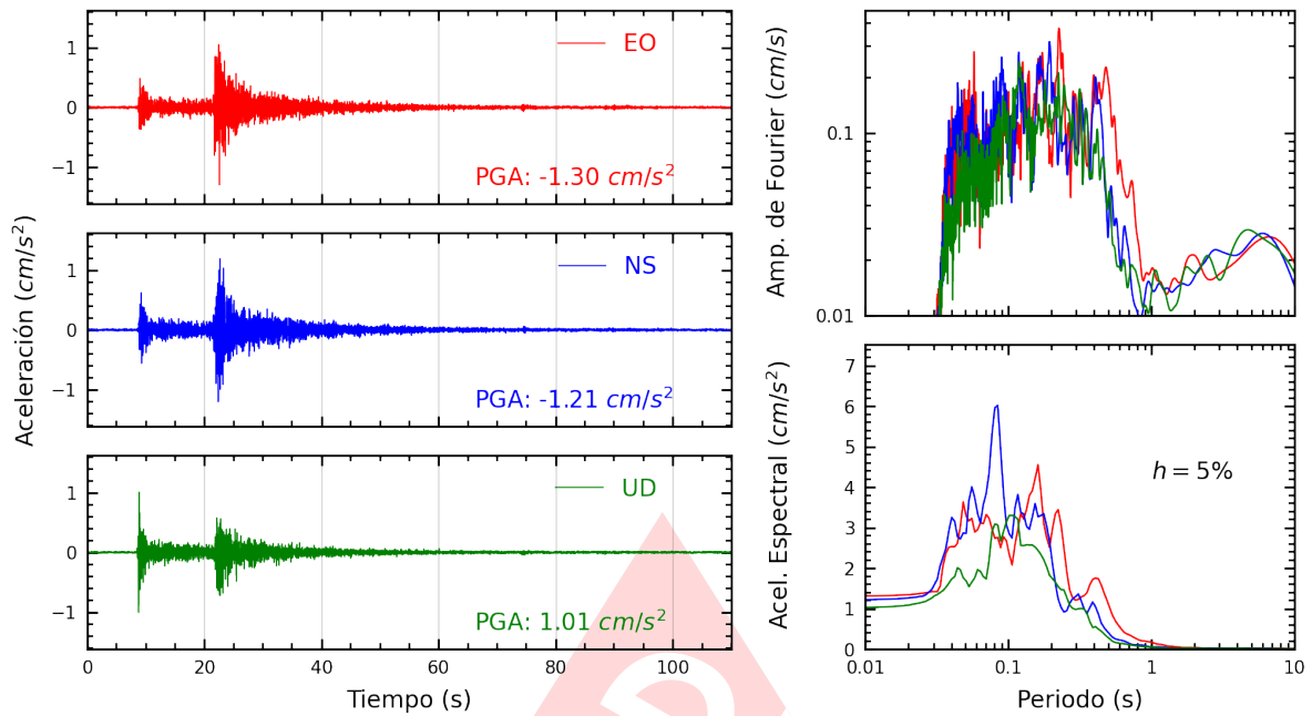
Figura A.17: Registros tiempo-historia, espectros de Fourier y de respuesta en las direcciones EO, NS y vertical de la estación COMAS. Sismo de Canta, Canta - Lima del 2023-12-13, 02:38:49 (Hora local)
