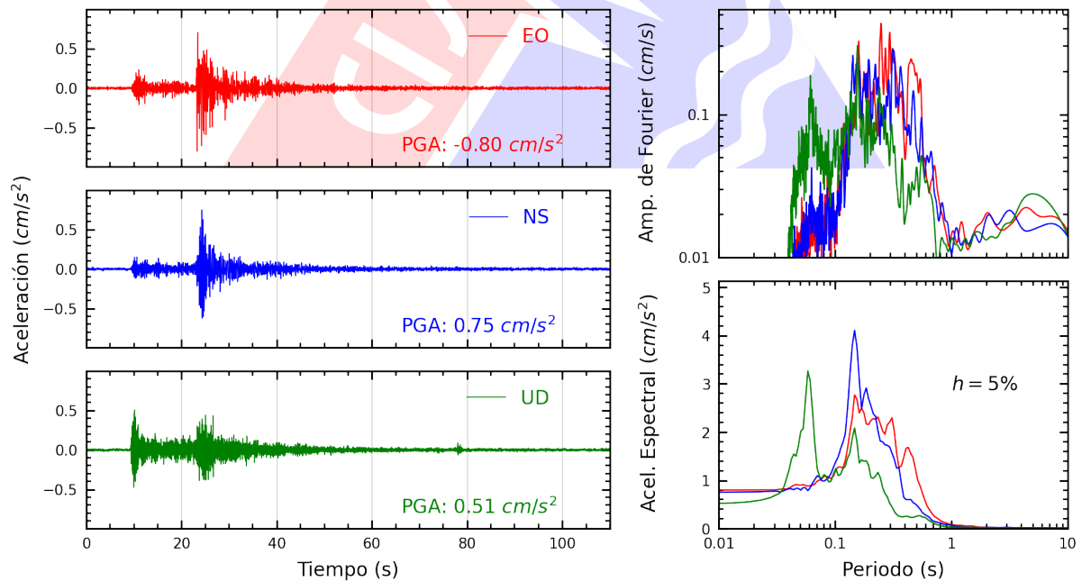
Figura A.28: Registros tiempo-historia, espectros de Fourier y de respuesta en las direcciones EO, NS y vertical de la estación ACAPU. Sismo de Canta, Canta - Lima del 2023-12-13, 02:38:49 (Hora local)
