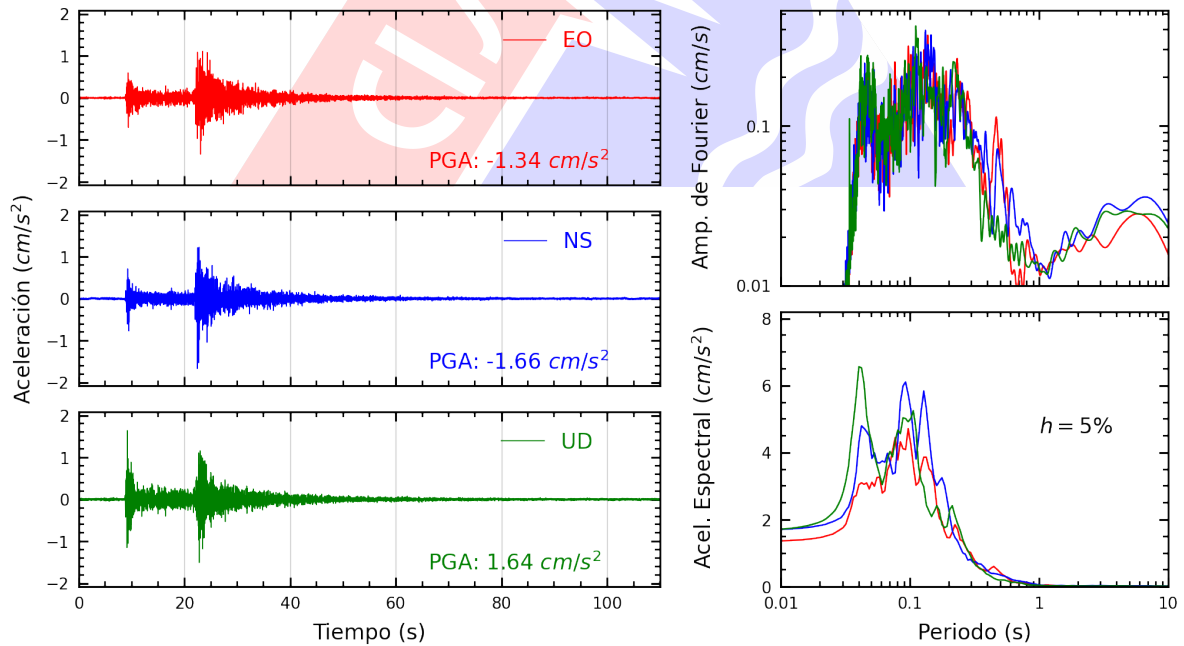
Figura A.10: Registros tiempo-historia, espectros de Fourier y de respuesta en las direcciones EO, NS y vertical de la estación USMP. Sismo de Canta, Canta - Lima del 2023-12-13, 02:38:49 (Hora local)
