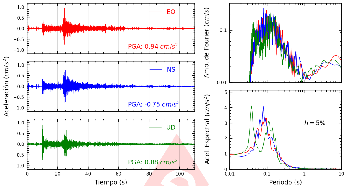
Figura A.25: Registros tiempo-historia, espectros de Fourier y de respuesta en las direcciones EO, NS y vertical de la estación UPCSM. Sismo de Canta, Canta - Lima del 2023-12-13, 02:38:49 (Hora local)
