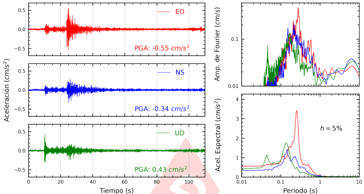
Figura A.33: Registros tiempo-historia, espectros de Fourier y de respuesta en las direcciones EO, NS y vertical de la estación DSML. Sismo de Canta, Canta - Lima del 2023-12-13, 02:38:49 (Hora local)
