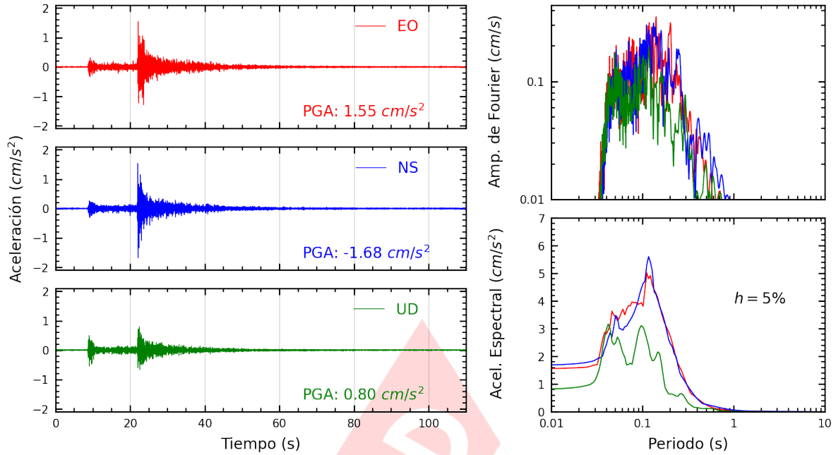
Figura A.9: Registros tiempo-historia, espectros de Fourier y de respuesta en las direcciones EO, NS y vertical de la estación ATARJ. Sismo de Canta, Canta - Lima del 2023-12-13, 02:38:49 (Hora local)
