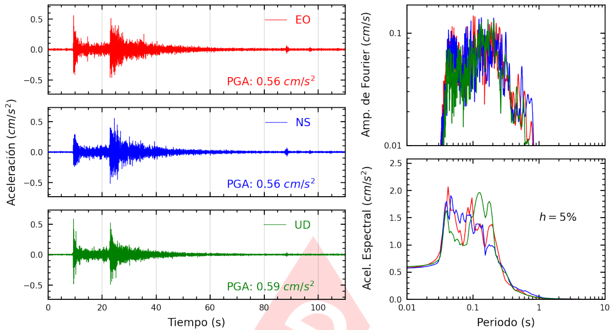
Figura A.31: Registros tiempo-historia, espectros de Fourier y de respuesta en las direcciones EO, NS y vertical de la estación BORJA. Sismo de Canta, Canta - Lima del 2023-12-13, 02:38:49 (Hora local)
