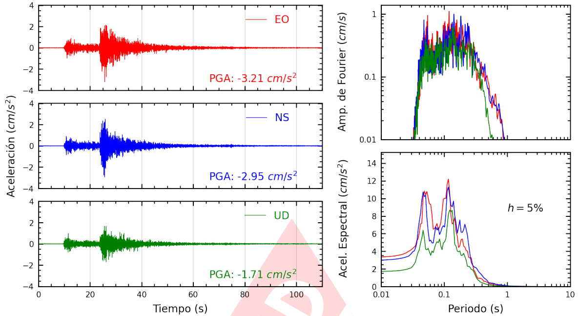
Figura A.3: Registros tiempo-historia, espectros de Fourier y de respuesta en las direcciones EO, NS y vertical de la estación UNTEL. Sismo de Canta, Canta - Lima del 2023-12-13, 02:38:49 (Hora local)
