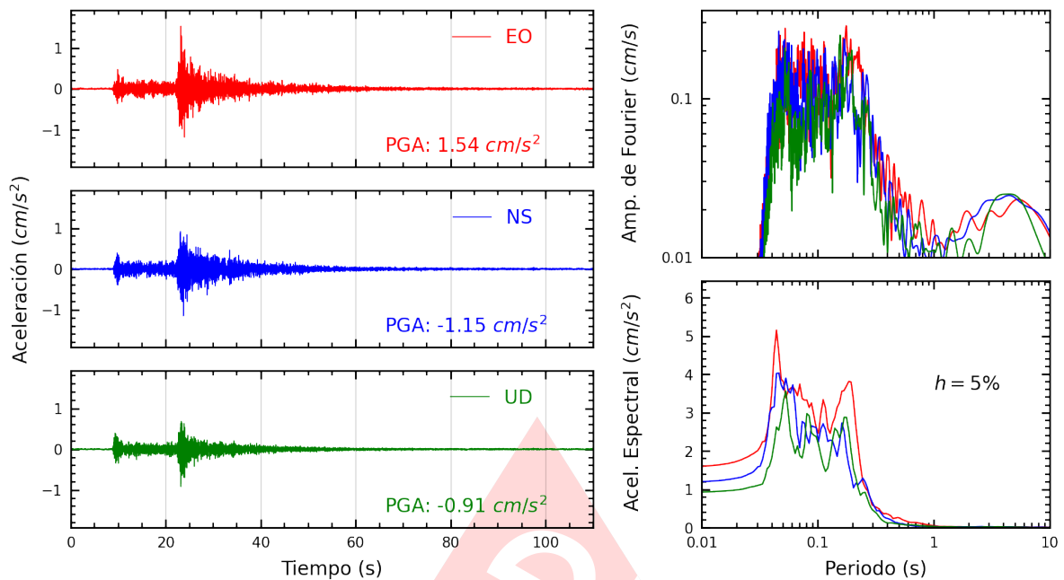
Figura A.13: Registros tiempo-historia, espectros de Fourier y de respuesta en las direcciones EO, NS y vertical de la estación FICPE. Sismo de Canta, Canta - Lima del 2023-12-13, 02:38:49 (Hora local)
