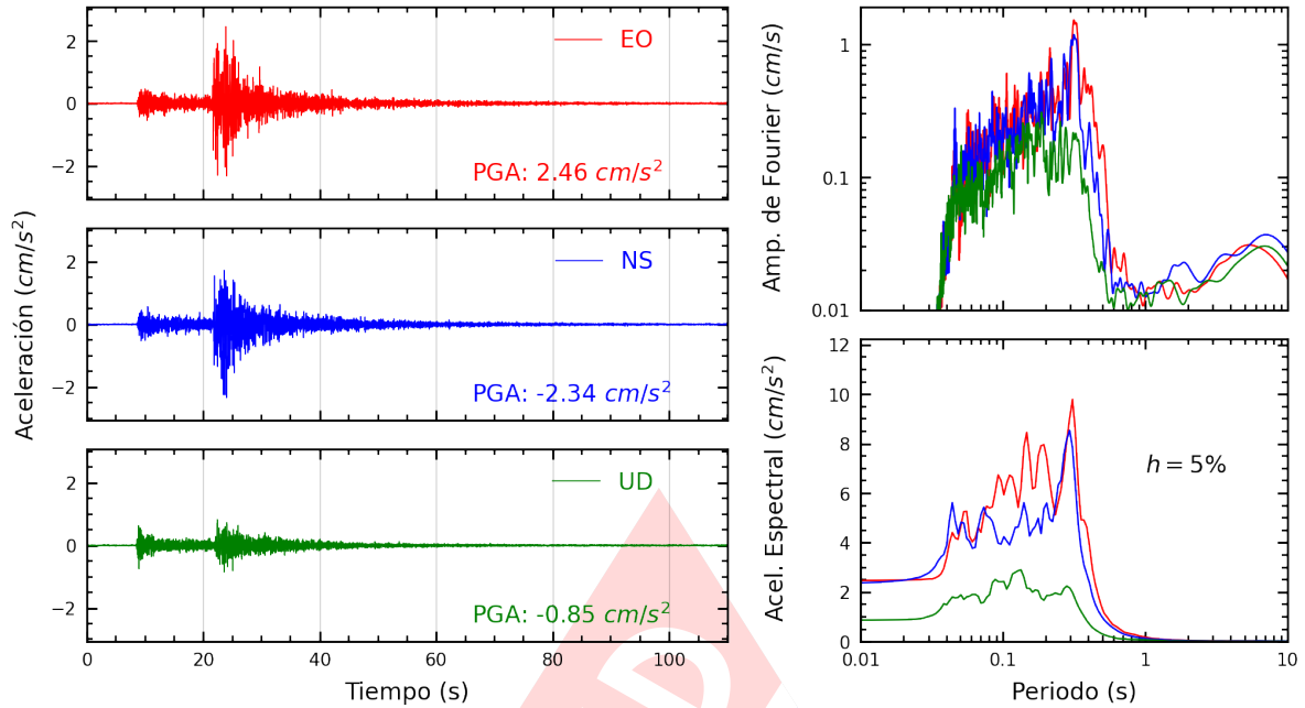
Figura A.5: Registros tiempo-historia, espectros de Fourier y de respuesta en las direcciones EO, NS y vertical de la estación DEFEN. Sismo de Canta, Canta - Lima del 2023-12-13, 02:38:49 (Hora local)
