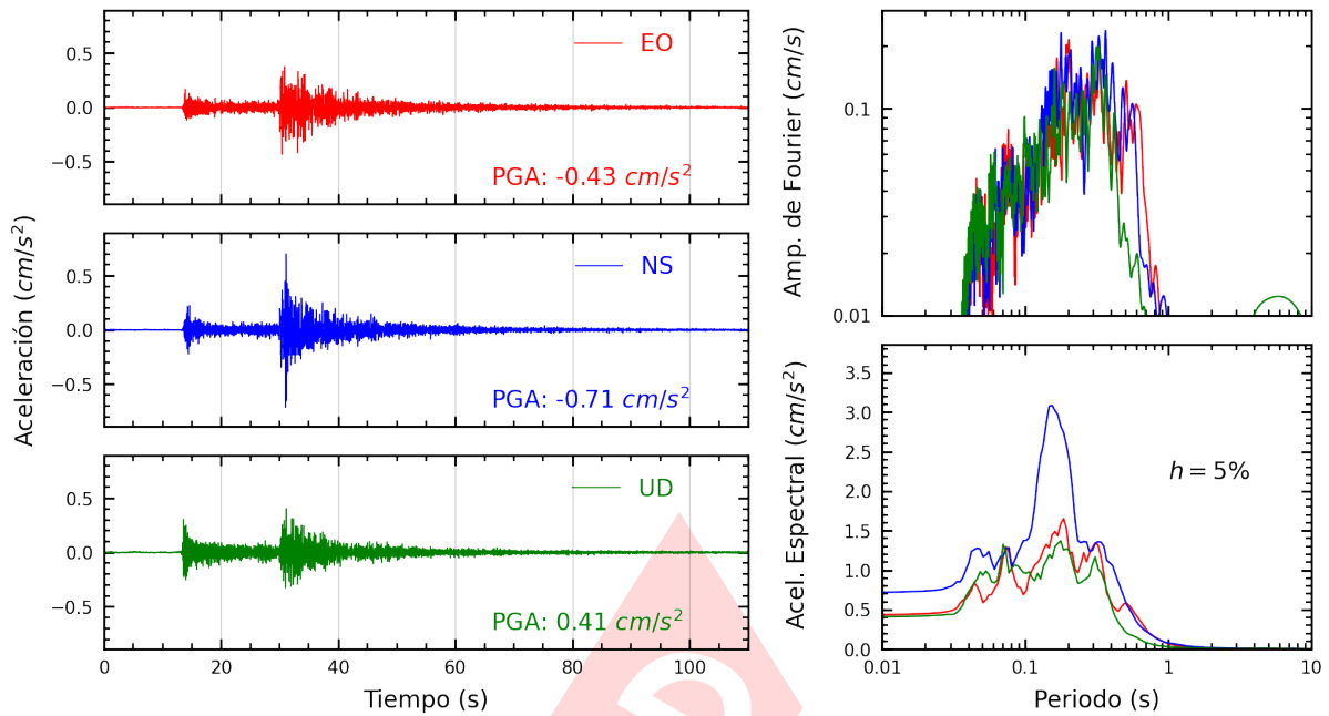
Figura A.29: Registros tiempo-historia, espectros de Fourier y de respuesta en las direcciones EO, NS y vertical de la estación CARAL. Sismo de Canta, Canta - Lima del 2023-12-13, 02:38:49 (Hora local)
