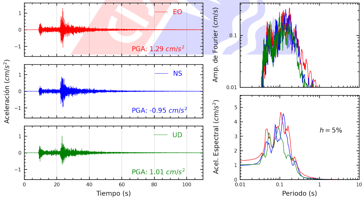
Figura A.18: Registros tiempo-historia, espectros de Fourier y de respuesta en las direcciones EO, NS y vertical de la estación JALV2. Sismo de Canta, Canta - Lima del 2023-12-13, 02:38:49 (Hora local)
