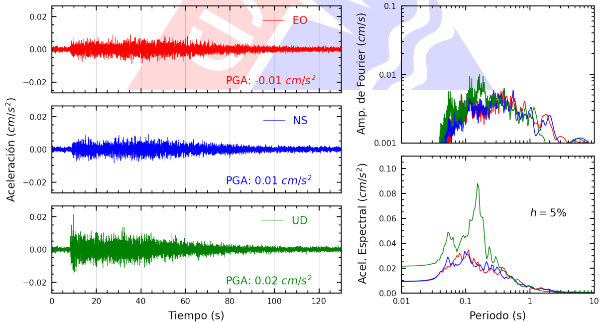
Figura A.40: Registros tiempo-historia, espectros de Fourier y de respuesta en las direcciones EO, NS y vertical de la estación UNCP. Sismo de Canta, Canta - Lima del 2023-12-13, 02:38:49 (Hora local)
