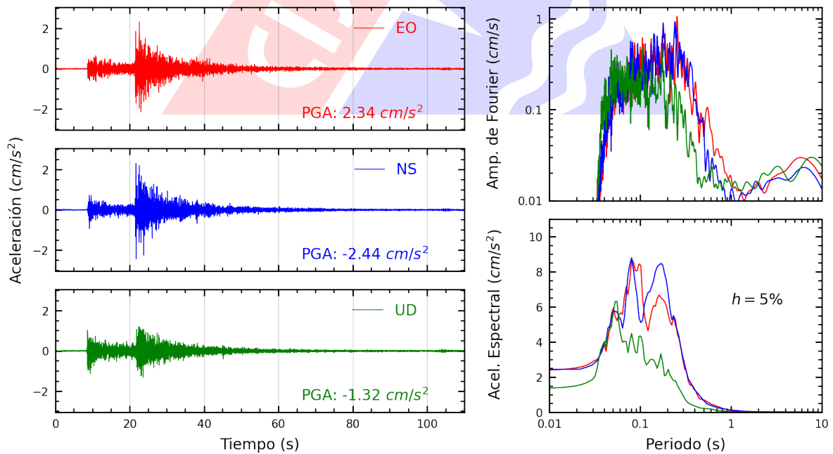
Figura A.6: Registros tiempo-historia, espectros de Fourier y de respuesta en las direcciones EO, NS y vertical de la estación ANCON. Sismo de Canta, Canta - Lima del 2023-12-13, 02:38:49 (Hora local)
