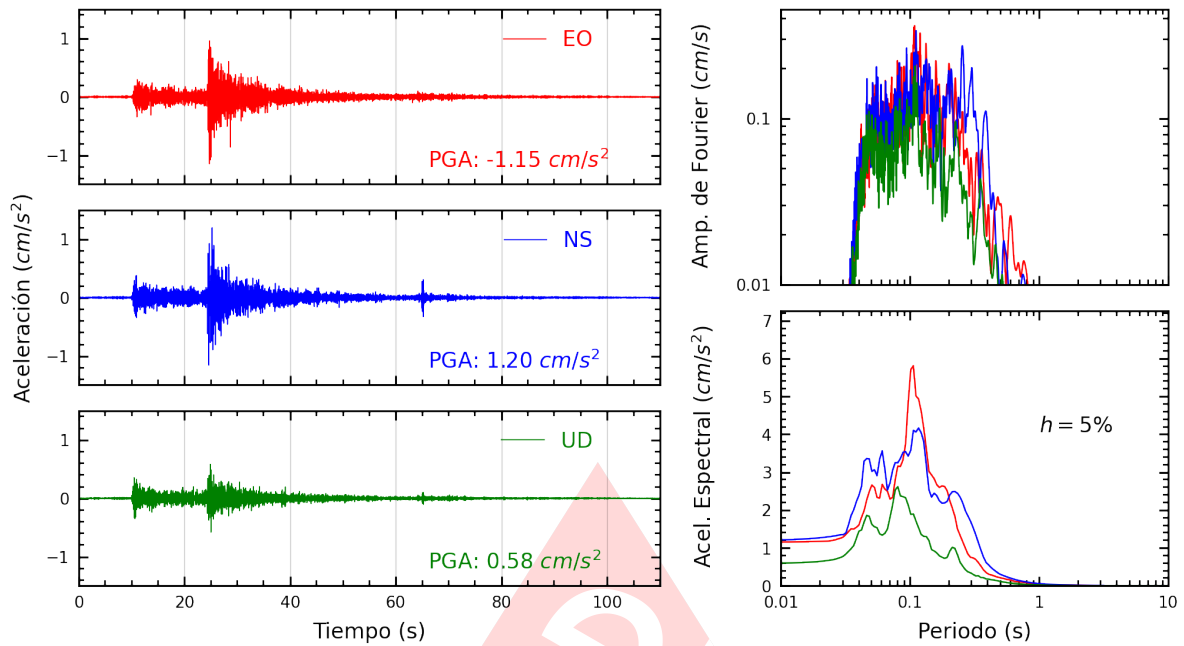
Figura A.21: Registros tiempo-historia, espectros de Fourier y de respuesta en las direcciones EO, NS y vertical de la estación PACHA. Sismo de Canta, Canta - Lima del 2023-12-13, 02:38:49 (Hora local)
