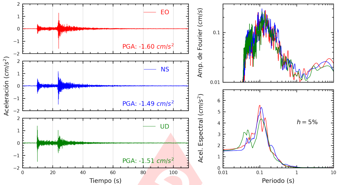
Figura A.11: Registros tiempo-historia, espectros de Fourier y de respuesta en las direcciones EO, NS y vertical de la estación SERVI. Sismo de Canta, Canta - Lima del 2023-12-13, 02:38:49 (Hora local)
