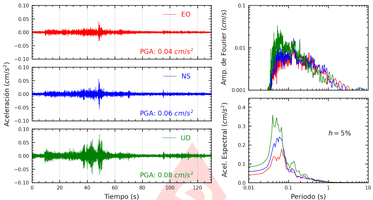
Figura A.37: Registros tiempo-historia, espectros de Fourier y de respuesta en las direcciones EO, NS y vertical de la estación SCHYO. Sismo de Canta, Canta - Lima del 2023-12-13, 02:38:49 (Hora local)
