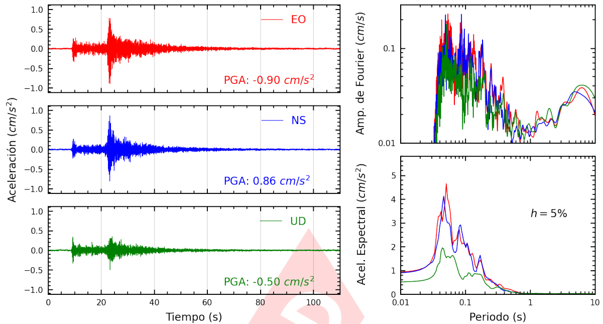
Figura A.27: Registros tiempo-historia, espectros de Fourier y de respuesta en las direcciones EO, NS y vertical de la estación UCSS. Sismo de Canta, Canta - Lima del 2023-12-13, 02:38:49 (Hora local)
