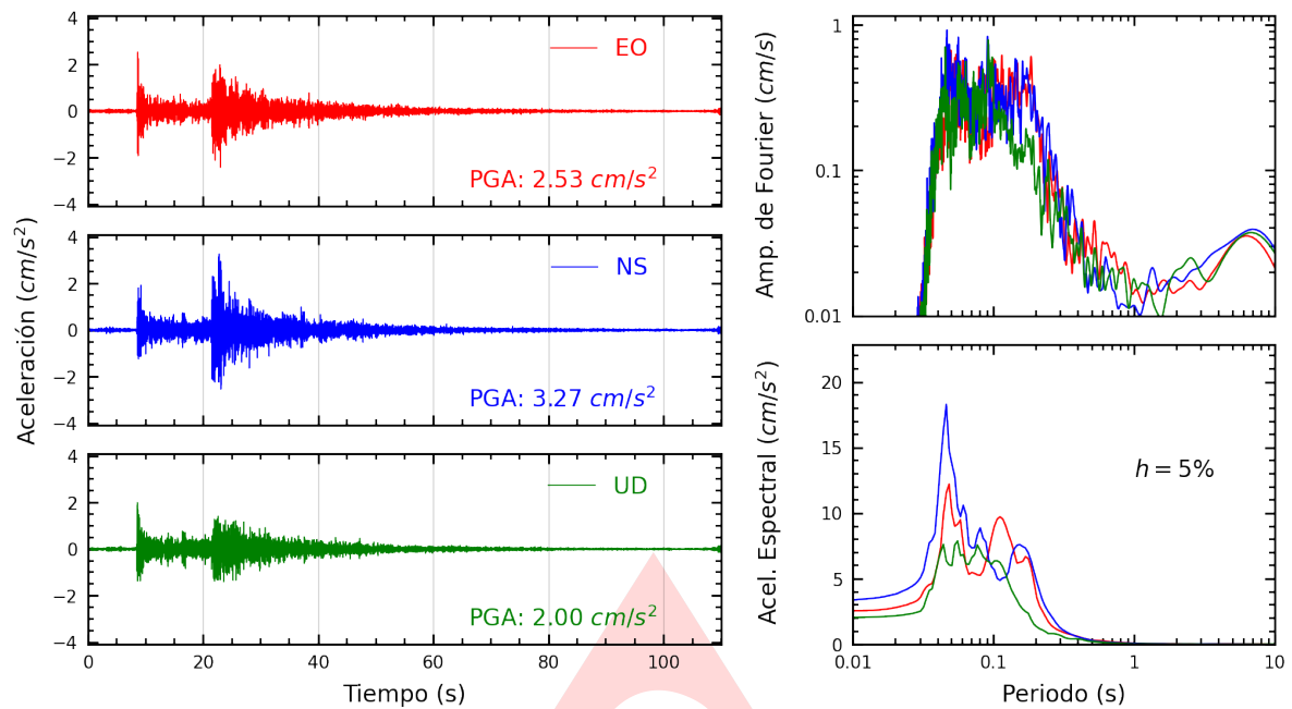
Figura A.1: Registros tiempo-historia, espectros de Fourier y de respuesta en las direcciones EO, NS y vertical de la estación SROSA. Sismo de Canta, Canta - Lima del 2023-12-13, 02:38:49 (Hora local)
