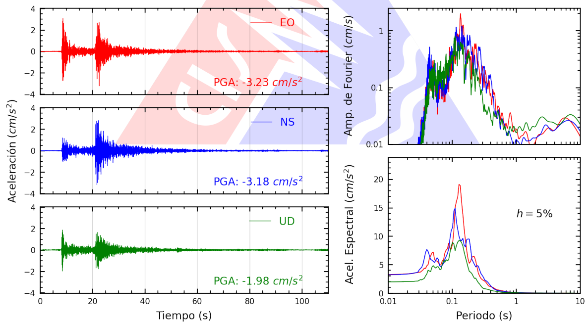
Figura A.2: Registros tiempo-historia, espectros de Fourier y de respuesta en las direcciones EO, NS y vertical de la estación CARAB. Sismo de Canta, Canta - Lima del 2023-12-13, 02:38:49 (Hora local)
