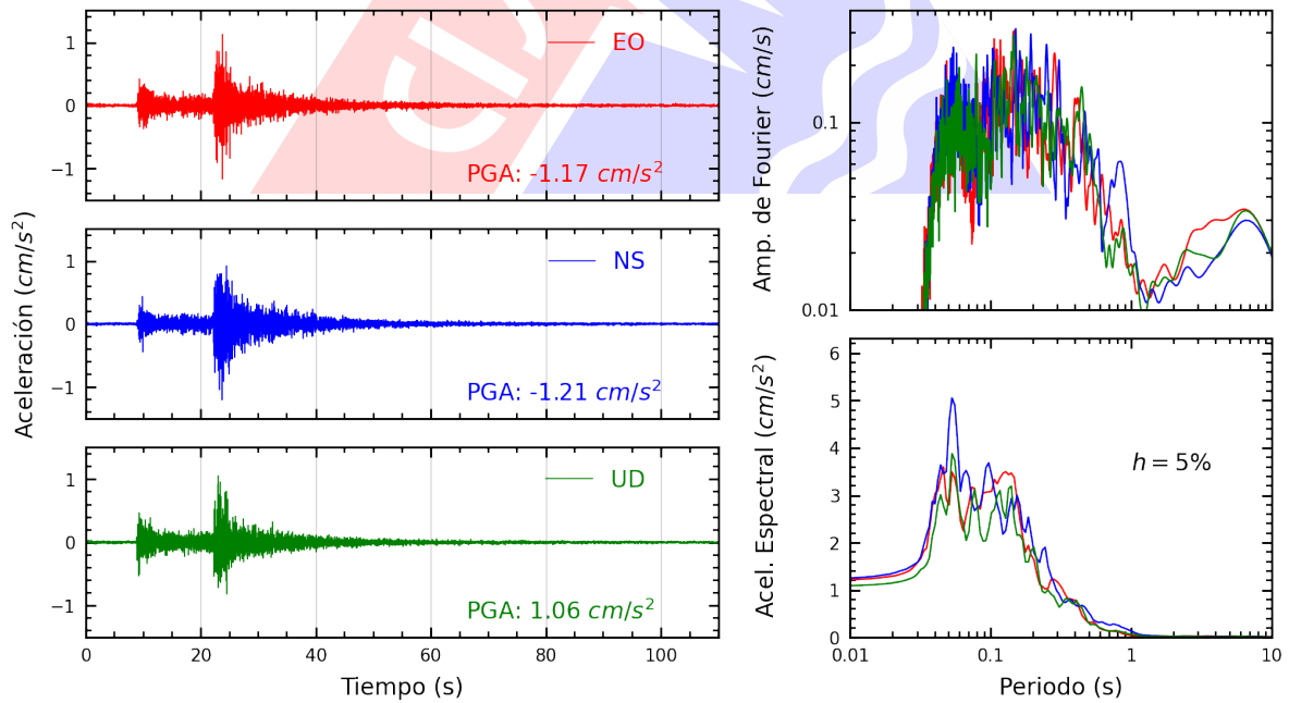
Figura A.20: Registros tiempo-historia, espectros de Fourier y de respuesta en las direcciones EO, NS y vertical de la estación IMCA. Sismo de Canta, Canta - Lima del 2023-12-13, 02:38:49 (Hora local)
