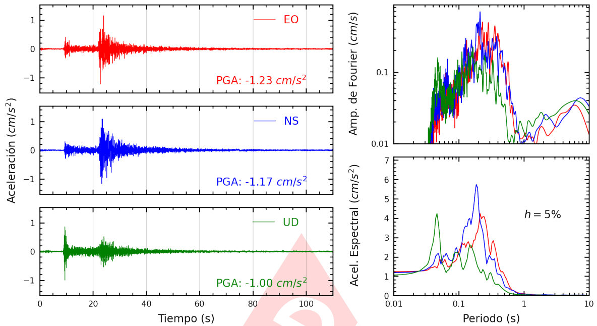
Figura A.19: Registros tiempo-historia, espectros de Fourier y de respuesta en las direcciones EO, NS y vertical de la estación VHAYA. Sismo de Canta, Canta - Lima del 2023-12-13, 02:38:49 (Hora local)
