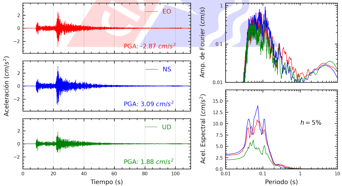
Figura A.4: Registros tiempo-historia, espectros de Fourier y de respuesta en las direcciones EO, NS y vertical de la estación JOSEO. Sismo de Canta, Canta - Lima del 2023-12-13, 02:38:49 (Hora local)
