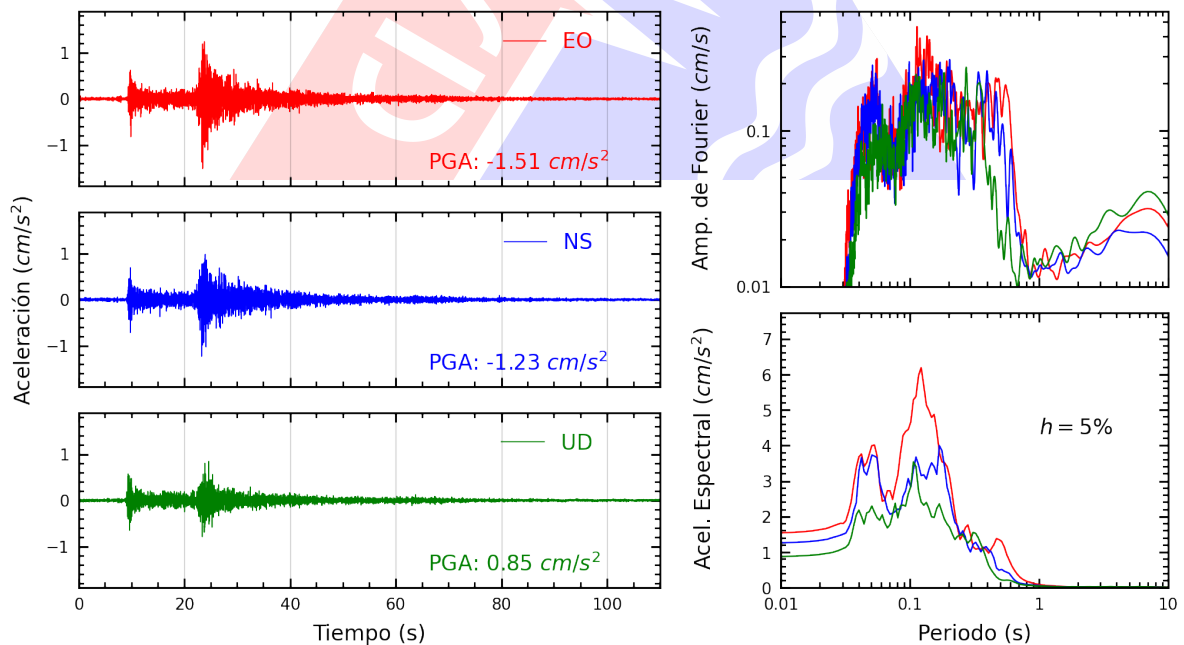
Figura A.14: Registros tiempo-historia, espectros de Fourier y de respuesta en las direcciones EO, NS y vertical de la estación OLIVO. Sismo de Canta, Canta - Lima del 2023-12-13, 02:38:49 (Hora local)
