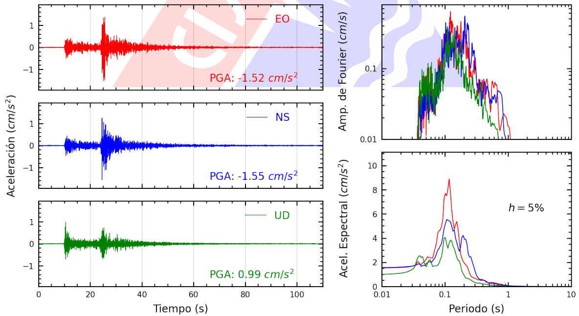
Figura A.12: Registros tiempo-historia, espectros de Fourier y de respuesta en las direcciones EO, NS y vertical de la estación SCCHO. Sismo de Canta, Canta - Lima del 2023-12-13, 02:38:49 (Hora local)
