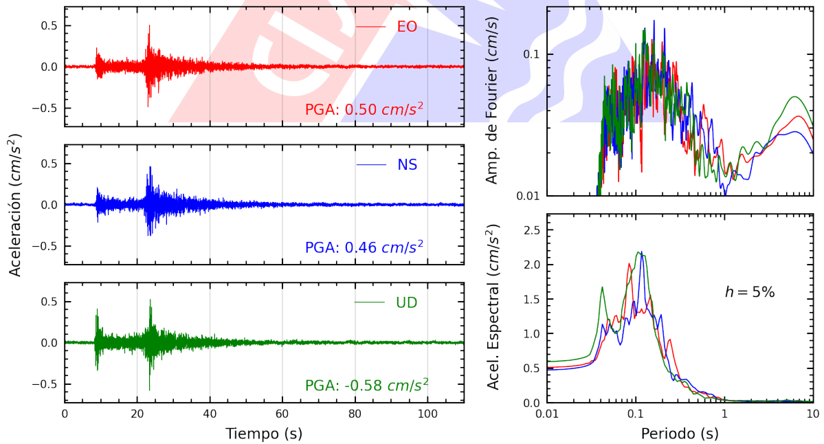
Figura A.32: Registros tiempo-historia, espectros de Fourier y de respuesta en las direcciones EO, NS y vertical de la estación UNMSM. Sismo de Canta, Canta - Lima del 2023-12-13, 02:38:49 (Hora local)
