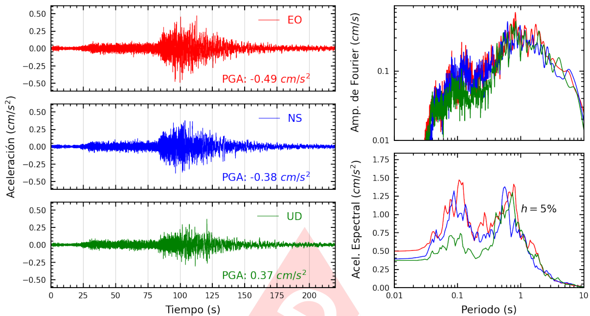
Figura A.33: Registros tiempo-historia, espectros de Fourier y de respuesta en las direcciones EO, NS y vertical de la estación ATARJ. Sismo de Aplao, Castilla - Arequipa del 2023-12-20, 07:11:20 (Hora local)
