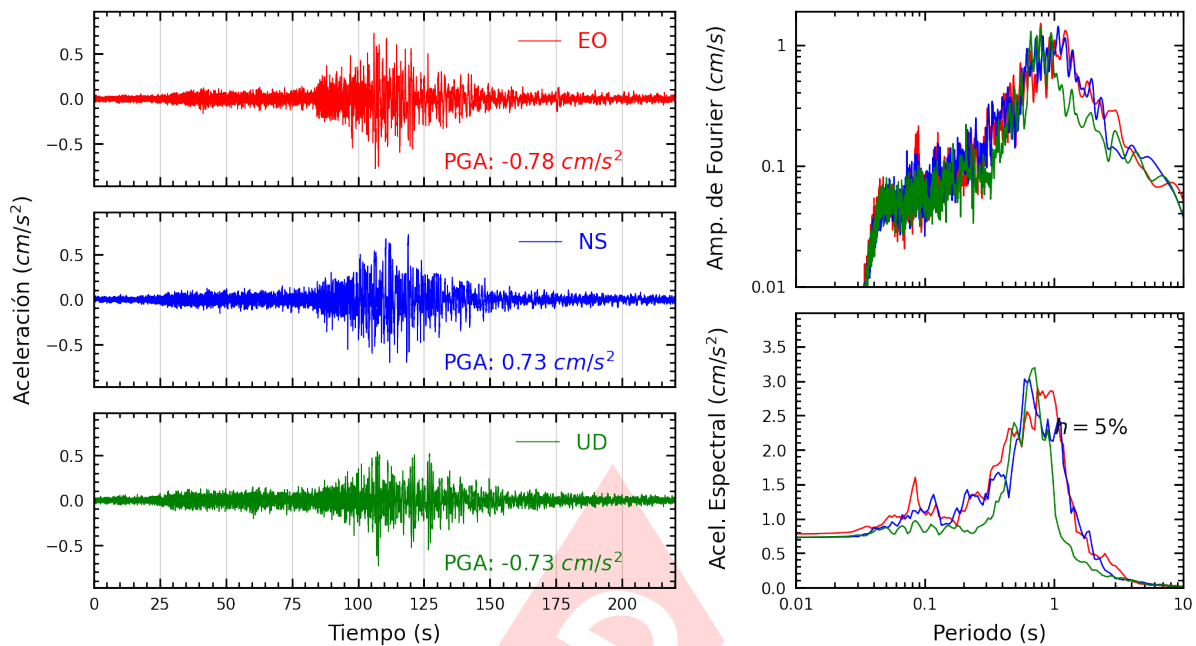
Figura A.27: Registros tiempo-historia, espectros de Fourier y de respuesta en las direcciones EO, NS y vertical de la estación CENEP. Sismo de Aplao, Castilla - Arequipa del 2023-12-20, 07:11:20 (Hora local)
