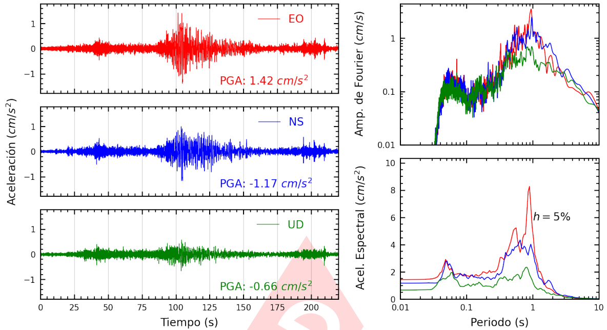
Figura A.15: Registros tiempo-historia, espectros de Fourier y de respuesta en las direcciones EO, NS y vertical de la estación UPCSM. Sismo de Aplao, Castilla - Arequipa del 2023-12-20, 07:11:20 (Hora local)
