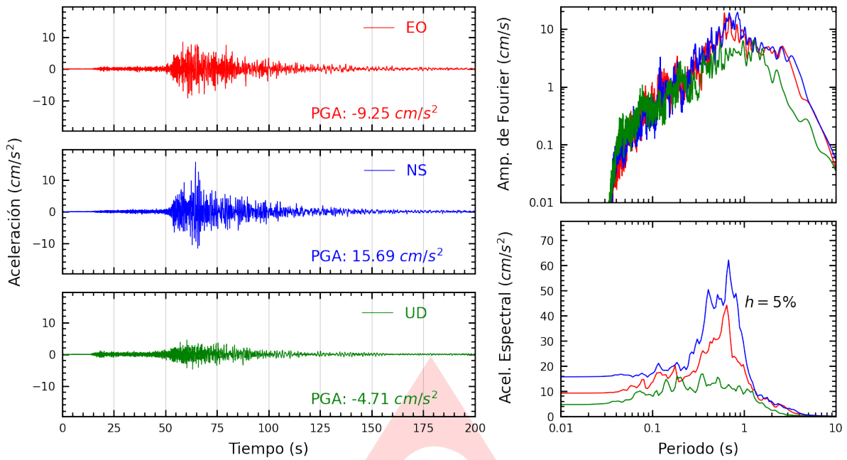
Figura A.1: Registros tiempo-historia, espectros de Fourier y de respuesta en las direcciones EO, NS y vertical de la estación UNICA. Sismo de Aplao, Castilla - Arequipa del 2023-12-20, 07:11:20 (Hora local)
