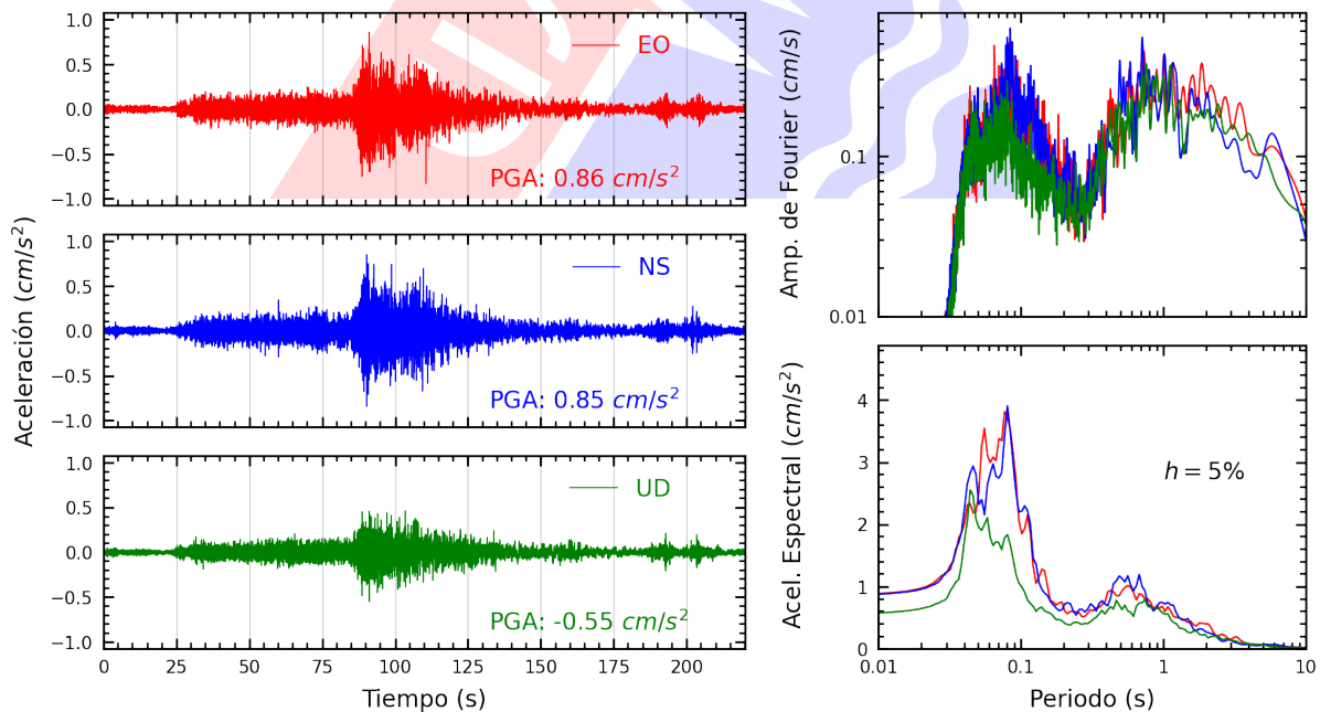
Figura A.24: Registros tiempo-historia, espectros de Fourier y de respuesta en las direcciones EO, NS y vertical de la estación JOSEO. Sismo de Aplao, Castilla - Arequipa del 2023-12-20, 07:11:20 (Hora local)
