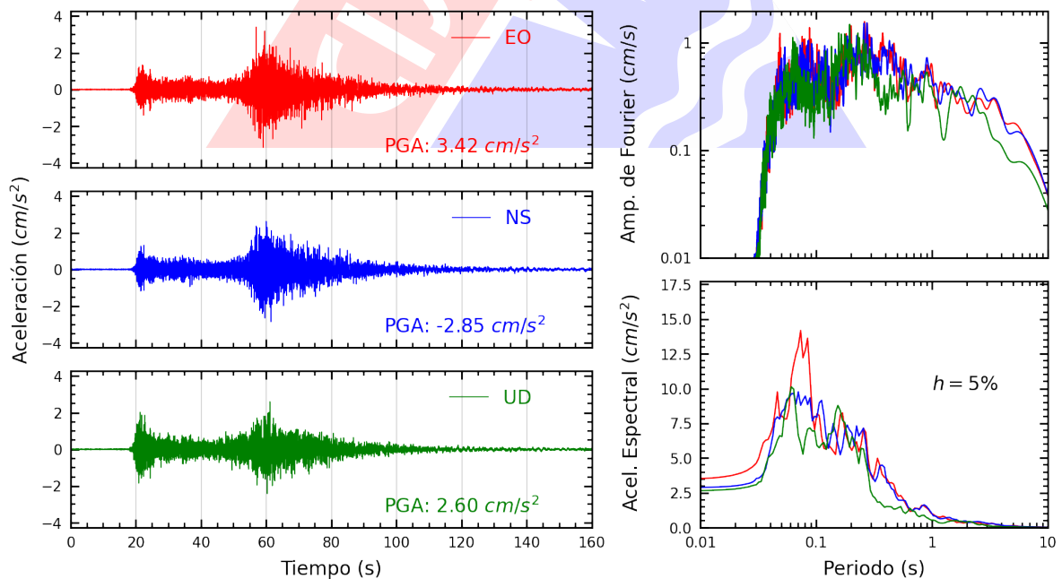
Figura A.6: Registros tiempo-historia, espectros de Fourier y de respuesta en las direcciones EO, NS y vertical de la estación CREY. Sismo de Aplao, Castilla - Arequipa del 2023-12-20, 07:11:20 (Hora local)
