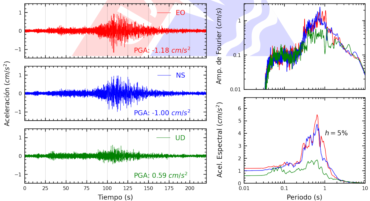
Figura A.18: Registros tiempo-historia, espectros de Fourier y de respuesta en las direcciones EO, NS y vertical de la estación MADRE. Sismo de Aplao, Castilla - Arequipa del 2023-12-20, 07:11:20 (Hora local)
