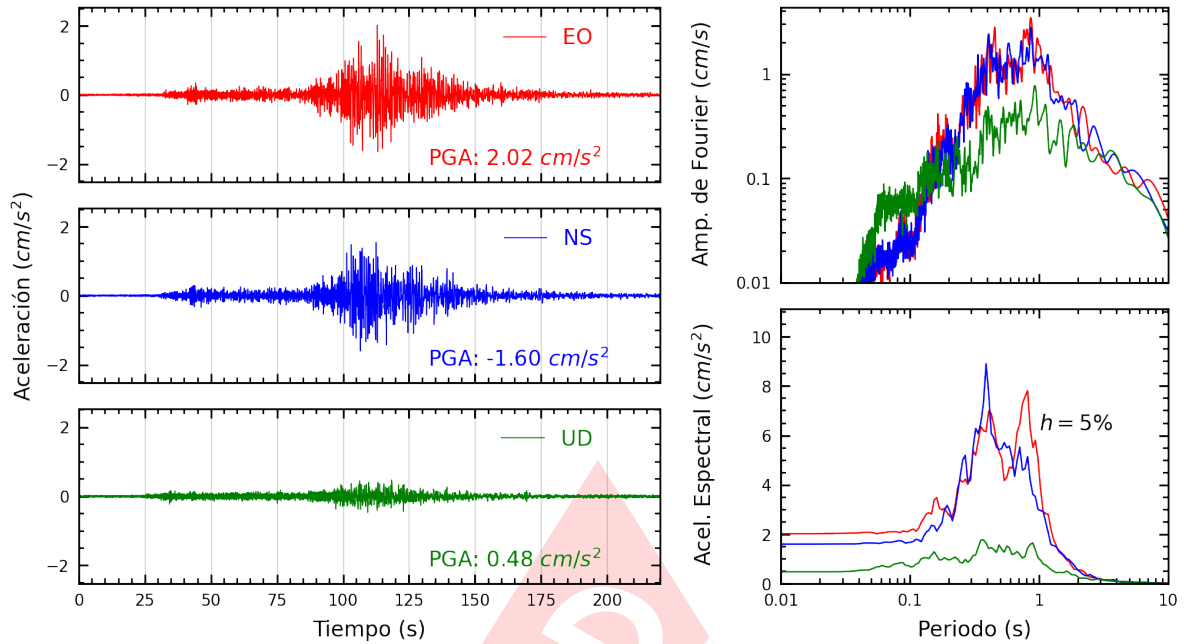
Figura A.13: Registros tiempo-historia, espectros de Fourier y de respuesta en las direcciones EO, NS y vertical de la estación ACAPU. Sismo de Aplao, Castilla - Arequipa del 2023-12-20, 07:11:20 (Hora local)
