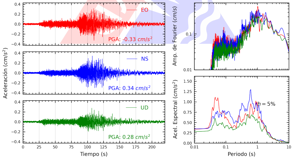
Figura A.34: Registros tiempo-historia, espectros de Fourier y de respuesta en las direcciones EO, NS y vertical de la estación UCSS. Sismo de Aplao, Castilla - Arequipa del 2023-12-20, 07:11:20 (Hora local)
