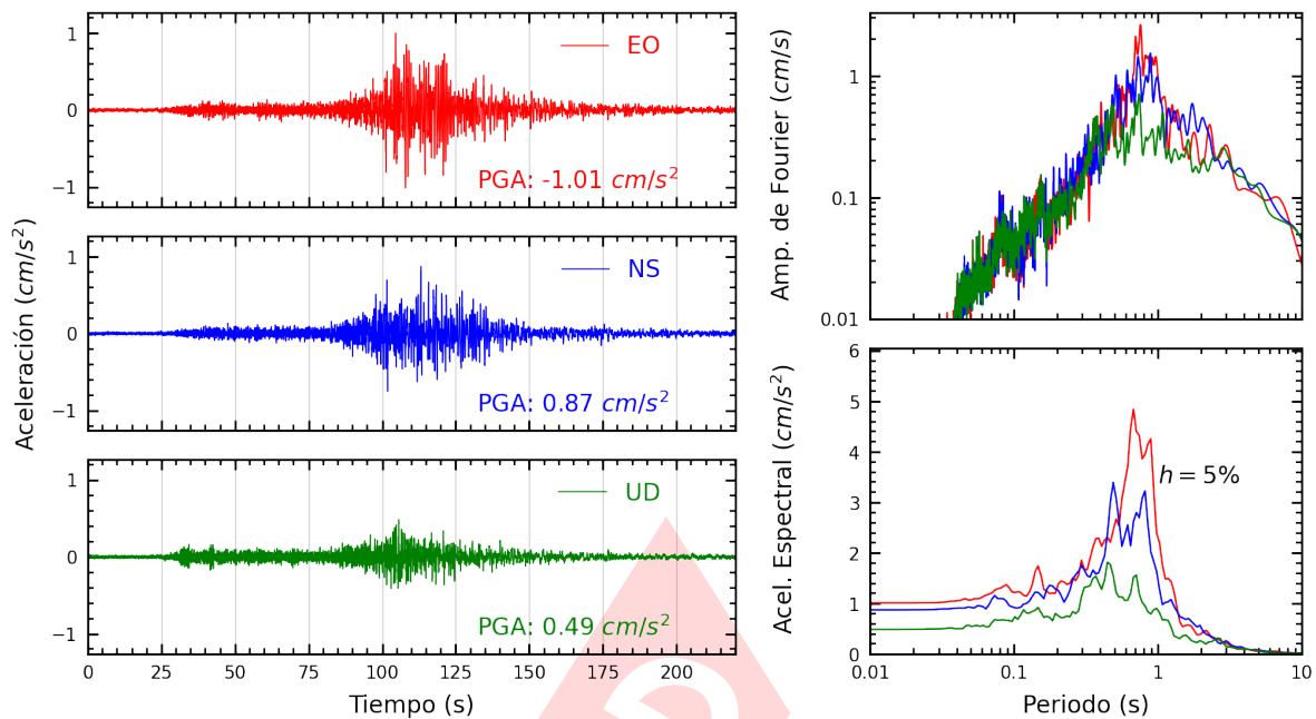
Figura A.21: Registros tiempo-historia, espectros de Fourier y de respuesta en las direcciones EO, NS y vertical de la estación UNMSM. Sismo de Aplao, Castilla - Arequipa del 2023-12-20, 07:11:20 (Hora local)
