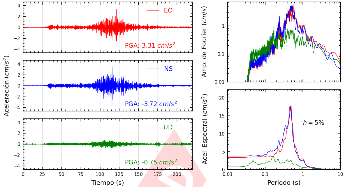
Figura A.5: Registros tiempo-historia, espectros de Fourier y de respuesta en las direcciones EO, NS y vertical de la estación MDPP. Sismo de Aplao, Castilla - Arequipa del 2023-12-20, 07:11:20 (Hora local)
