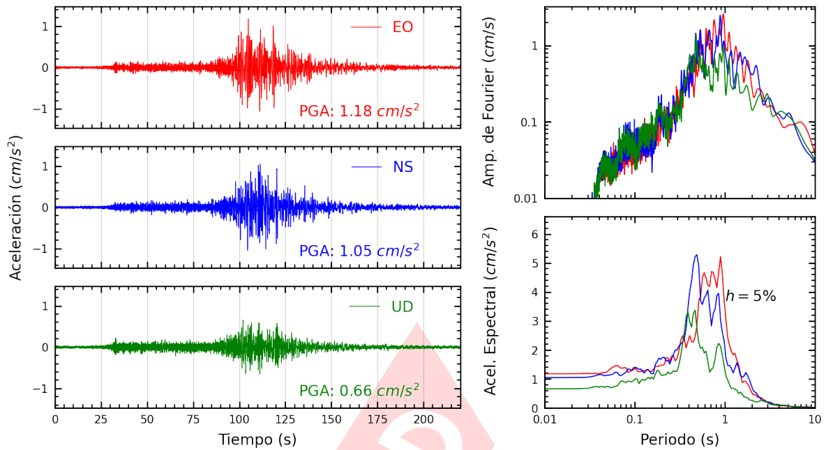
Figura A.19: Registros tiempo-historia, espectros de Fourier y de respuesta en las direcciones EO, NS y vertical de la estación UNFV. Sismo de Aplao, Castilla - Arequipa del 2023-12-20, 07:11:20 (Hora local)
