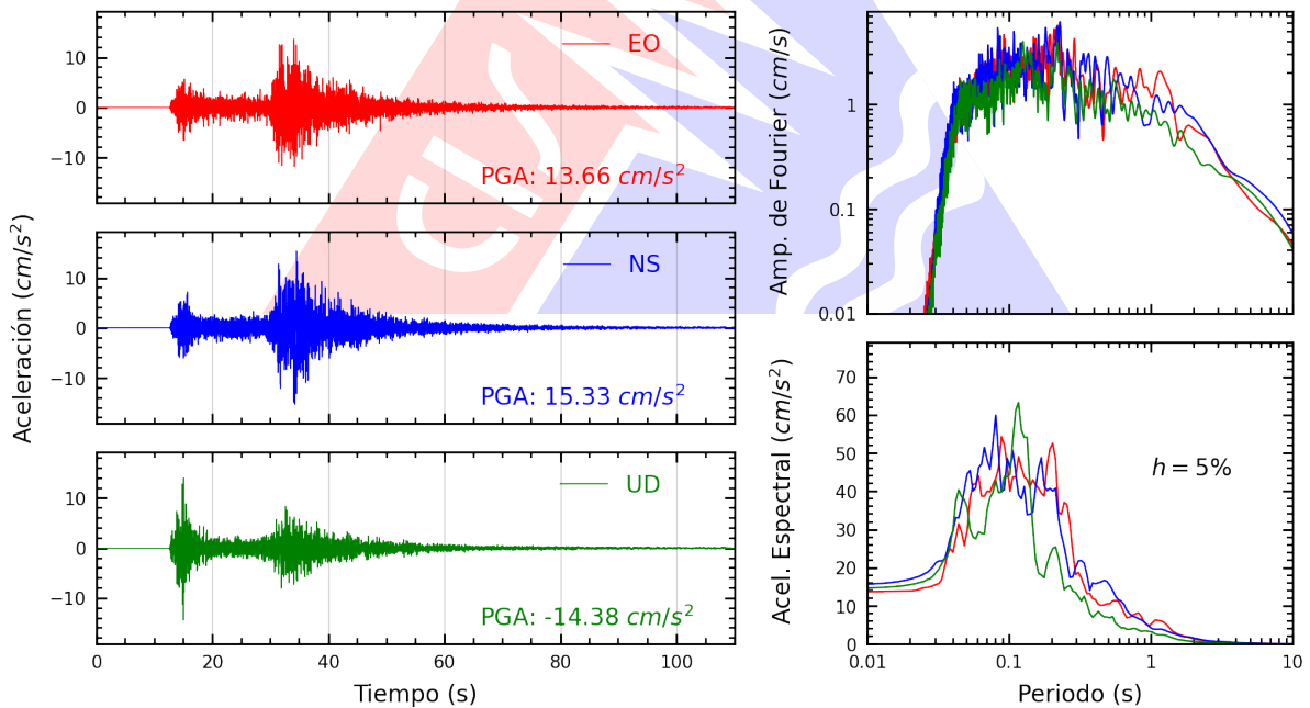
Figura A.2: Registros tiempo-historia, espectros de Fourier y de respuesta en las direcciones EO, NS y vertical de la estación UNSA. Sismo de Aplao, Castilla - Arequipa del 2023-12-20, 07:11:20 (Hora local)
