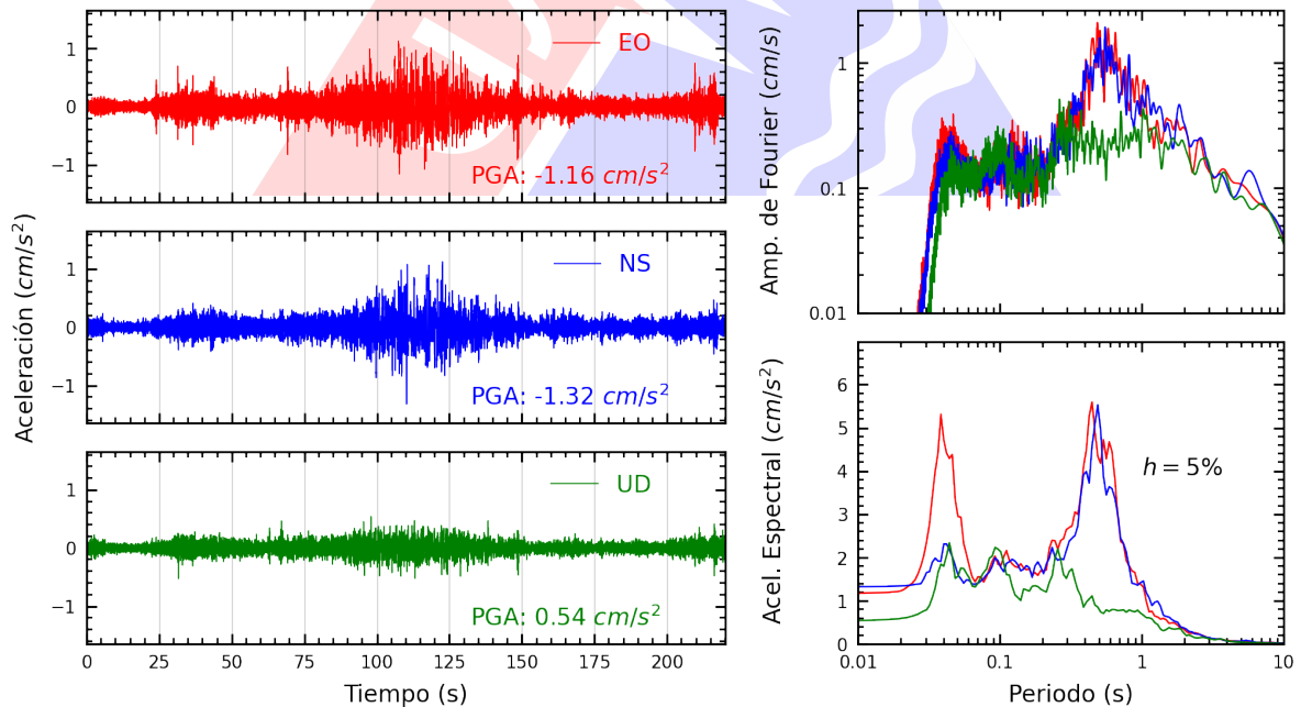
Figura A.16: Registros tiempo-historia, espectros de Fourier y de respuesta en las direcciones EO, NS y vertical de la estación OLIVO. Sismo de Aplao, Castilla - Arequipa del 2023-12-20, 07:11:20 (Hora local)
