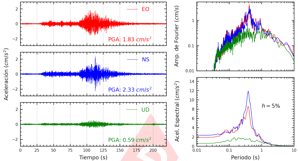
Figura A.9: Registros tiempo-historia, espectros de Fourier y de respuesta en las direcciones EO, NS y vertical de la estación DEFEN. Sismo de Aplao, Castilla - Arequipa del 2023-12-20, 07:11:20 (Hora local)
