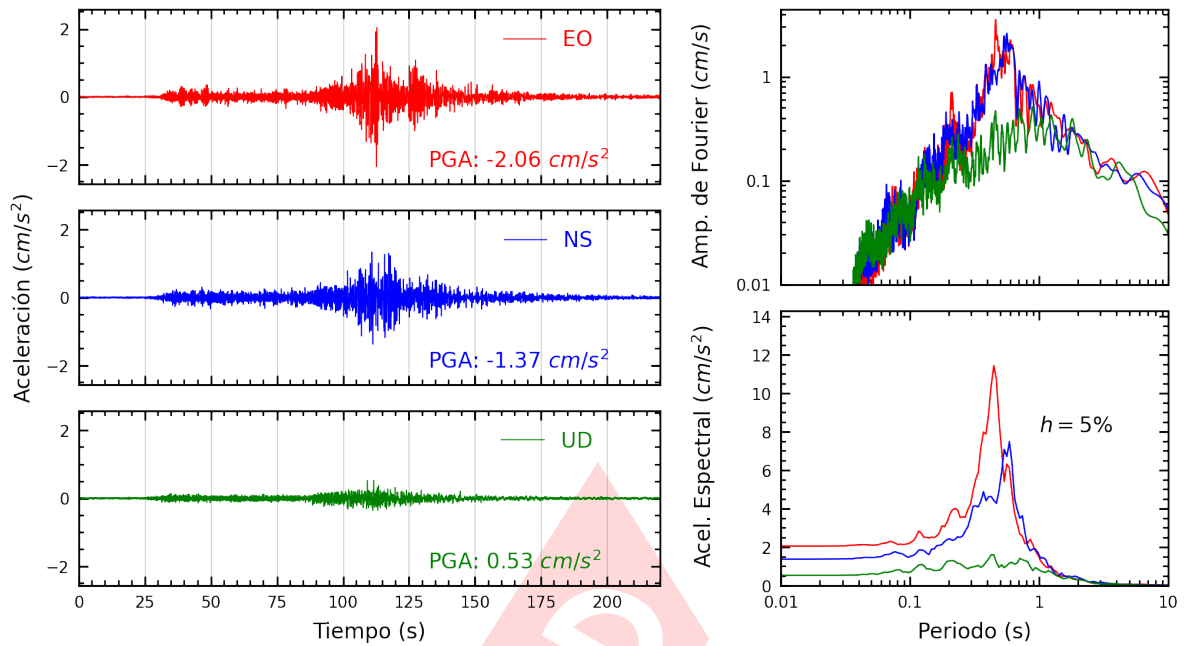
Figura A.11: Registros tiempo-historia, espectros de Fourier y de respuesta en las direcciones EO, NS y vertical de la estación VHAYA. Sismo de Aplao, Castilla - Arequipa del 2023-12-20, 07:11:20 (Hora local)
