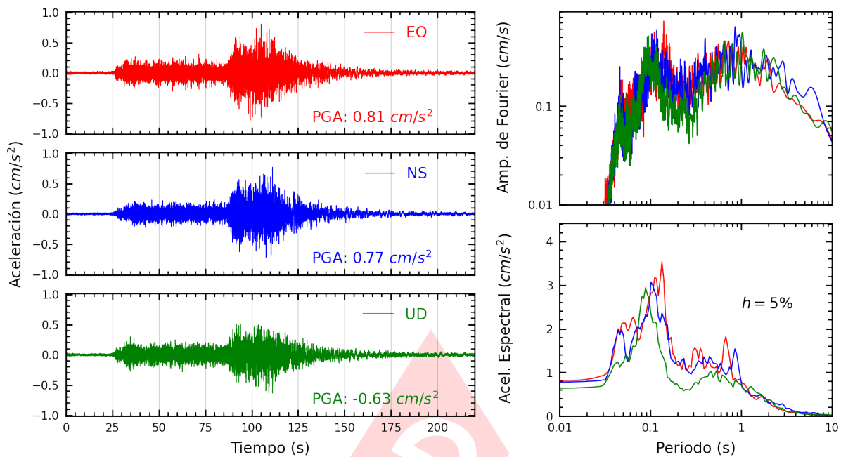
Figura A.25: Registros tiempo-historia, espectros de Fourier y de respuesta en las direcciones EO, NS y vertical de la estación AMORE. Sismo de Aplao, Castilla - Arequipa del 2023-12-20, 07:11:20 (Hora local)
