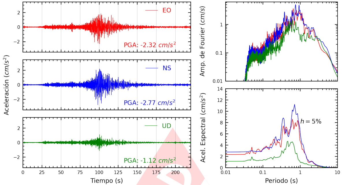
Figura A.7: Registros tiempo-historia, espectros de Fourier y de respuesta en las direcciones EO, NS y vertical de la estación BRISA. Sismo de Aplao, Castilla - Arequipa del 2023-12-20, 07:11:20 (Hora local)
