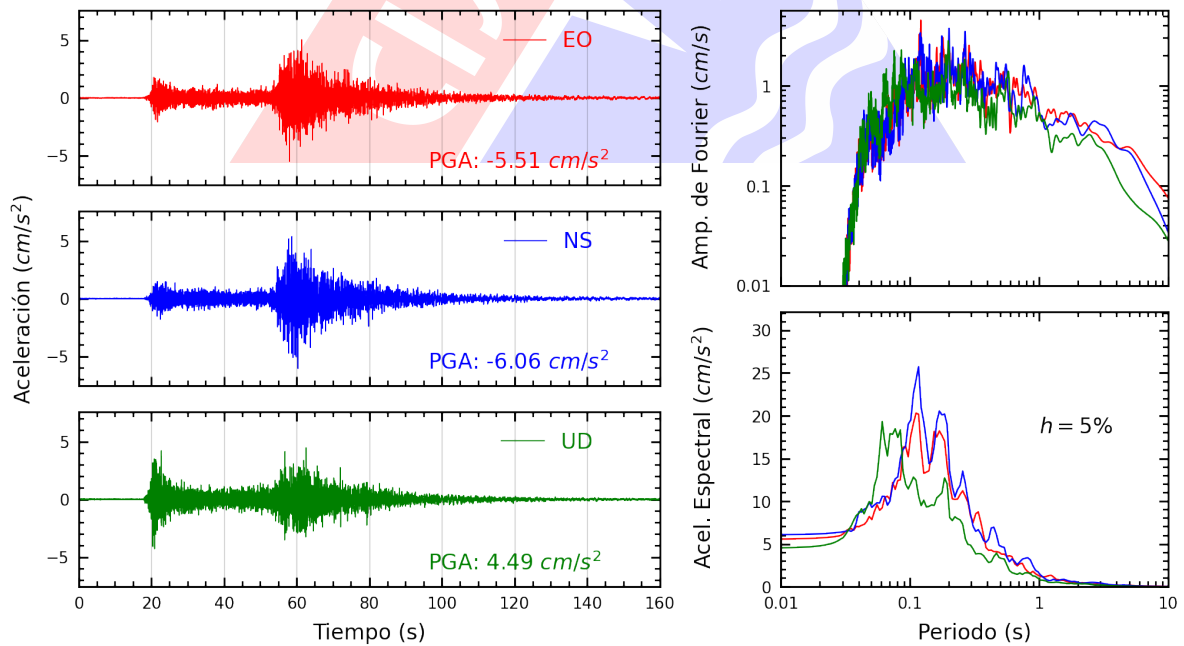
Figura A.4: Registros tiempo-historia, espectros de Fourier y de respuesta en las direcciones EO, NS y vertical de la estación UJBG3. Sismo de Aplao, Castilla - Arequipa del 2023-12-20, 07:11:20 (Hora local)
