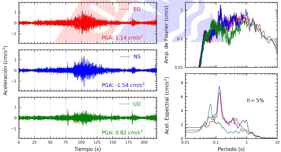
Figura A.14: Registros tiempo-historia, espectros de Fourier y de respuesta en las direcciones EO, NS y vertical de la estación CARAB. Sismo de Aplao, Castilla - Arequipa del 2023-12-20, 07:11:20 (Hora local)
