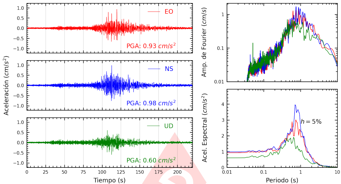
Figura A.23: Registros tiempo-historia, espectros de Fourier y de respuesta en las direcciones EO, NS y vertical de la estación BONDY. Sismo de Aplao, Castilla - Arequipa del 2023-12-20, 07:11:20 (Hora local)
