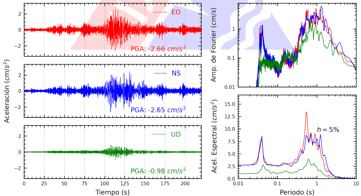
Figura A.8: Registros tiempo-historia, espectros de Fourier y de respuesta en las direcciones EO, NS y vertical de la estación DHNPE. Sismo de Aplao, Castilla - Arequipa del 2023-12-20, 07:11:20 (Hora local)
