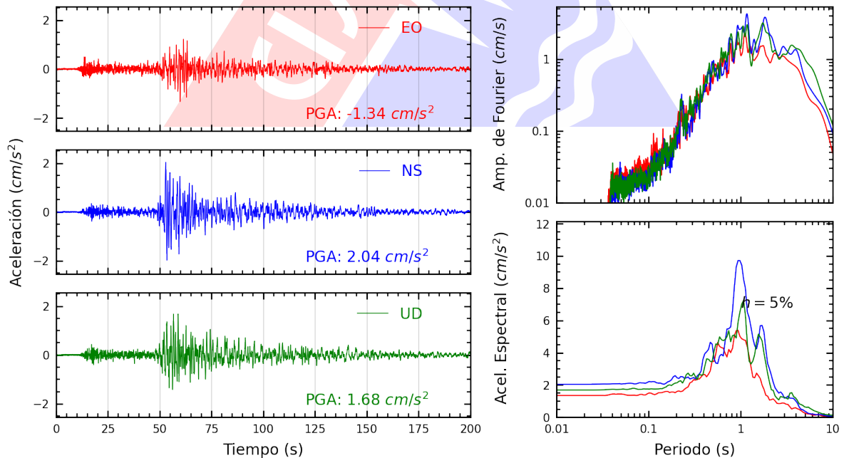
Figura A.12: Registros tiempo-historia, espectros de Fourier y de respuesta en las direcciones EO, NS y vertical de la estación UNSCH. Sismo de Aplao, Castilla - Arequipa del 2023-12-20, 07:11:20 (Hora local)
