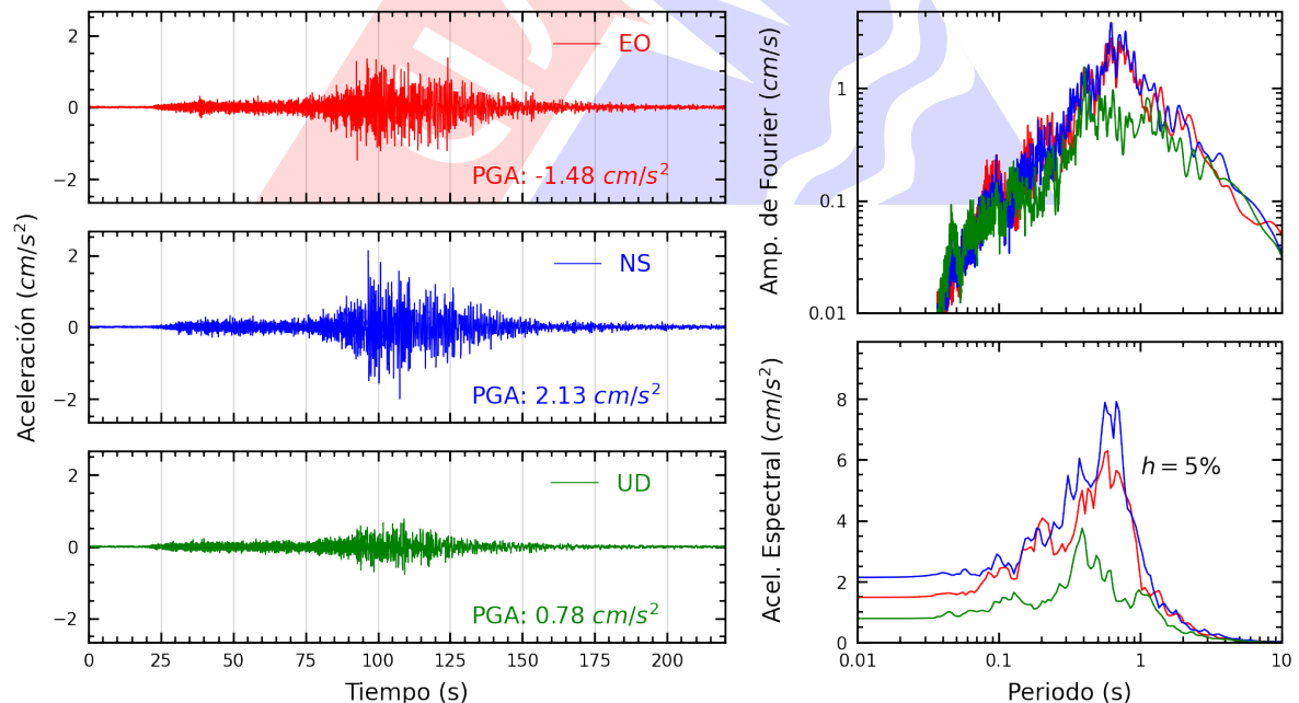
Figura A.10: Registros tiempo-historia, espectros de Fourier y de respuesta en las direcciones EO, NS y vertical de la estación USILP. Sismo de Aplao, Castilla - Arequipa del 2023-12-20, 07:11:20 (Hora local)
