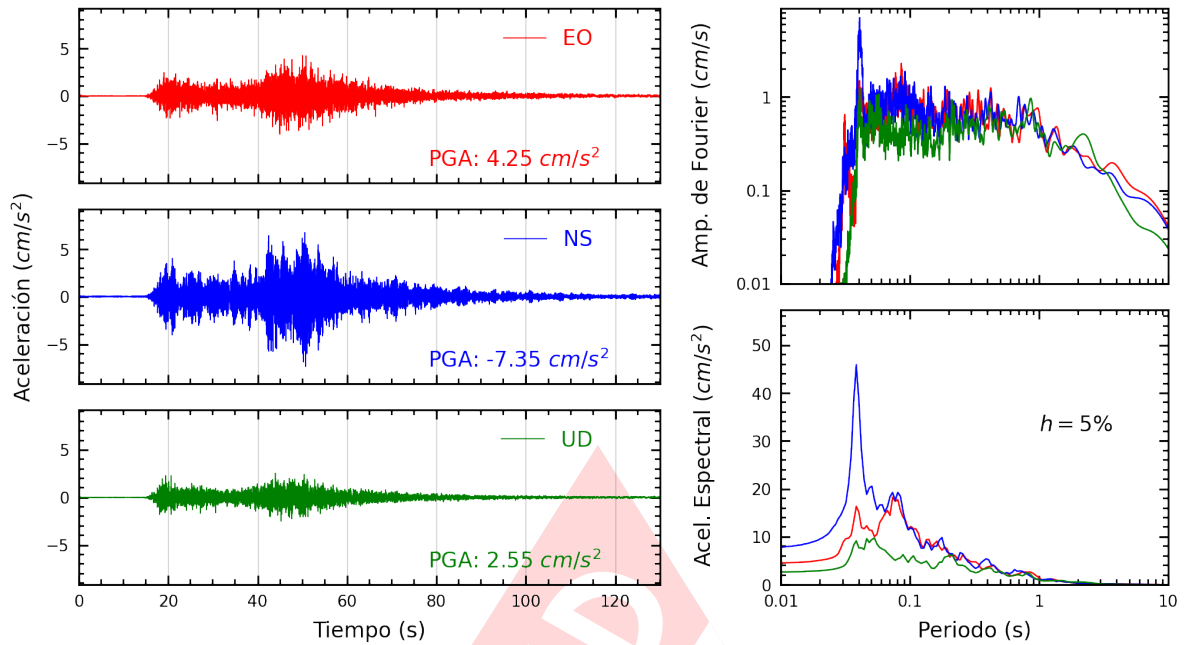
Figura A.3: Registros tiempo-historia, espectros de Fourier y de respuesta en las direcciones EO, NS y vertical de la estación UNAM. Sismo de Aplao, Castilla - Arequipa del 2023-12-20, 07:11:20 (Hora local)
