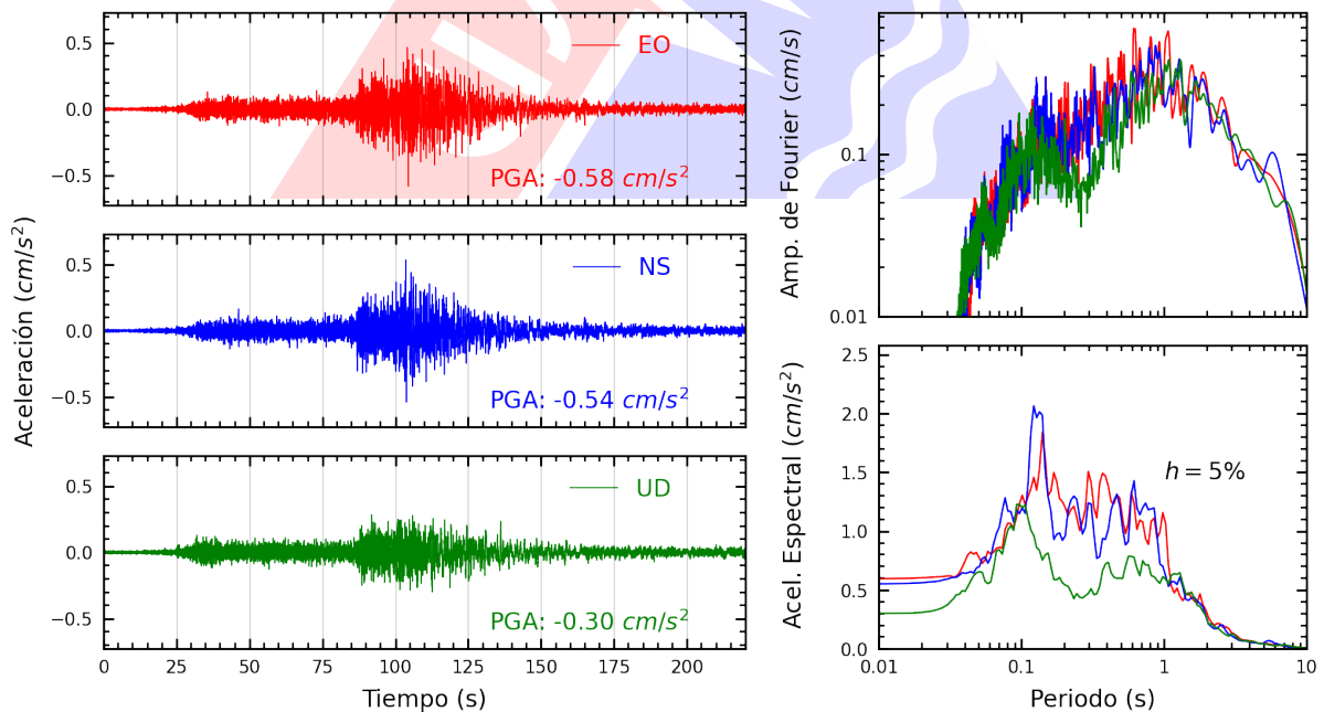
Figura A.32: Registros tiempo-historia, espectros de Fourier y de respuesta en las direcciones EO, NS y vertical de la estación JALV2. Sismo de Aplao, Castilla - Arequipa del 2023-12-20, 07:11:20 (Hora local)
