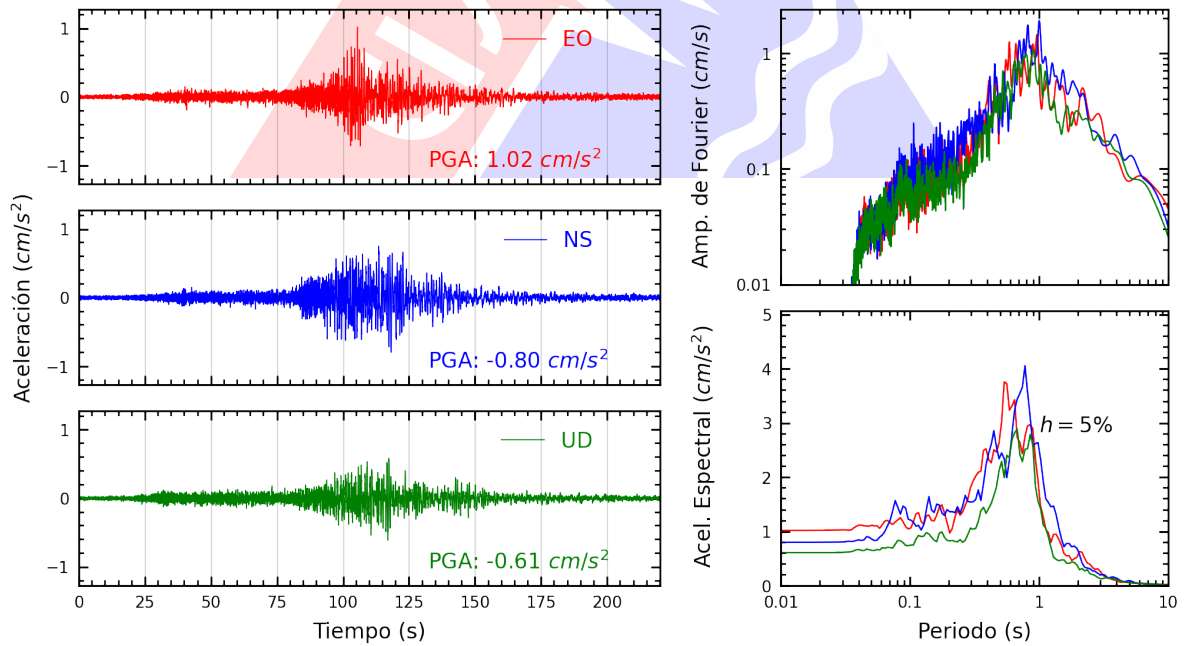
Figura A.20: Registros tiempo-historia, espectros de Fourier y de respuesta en las direcciones EO, NS y vertical de la estación SERVI. Sismo de Aplao, Castilla - Arequipa del 2023-12-20, 07:11:20 (Hora local)
