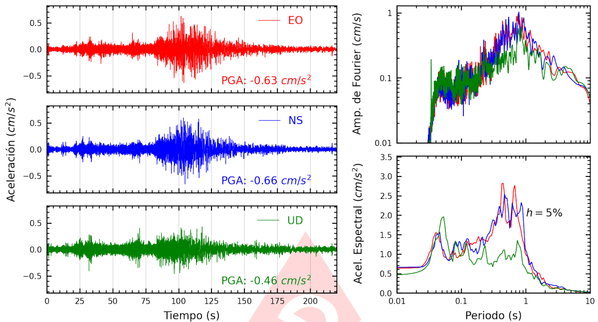
Figura A.29: Registros tiempo-historia, espectros de Fourier y de respuesta en las direcciones EO, NS y vertical de la estación USMP. Sismo de Aplao, Castilla - Arequipa del 2023-12-20, 07:11:20 (Hora local)
