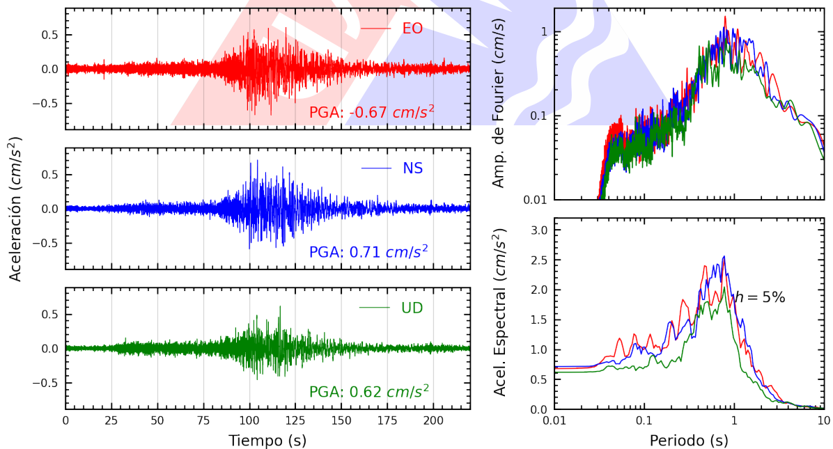
Figura A.28: Registros tiempo-historia, espectros de Fourier y de respuesta en las direcciones EO, NS y vertical de la estación INICT. Sismo de Aplao, Castilla - Arequipa del 2023-12-20, 07:11:20 (Hora local)
