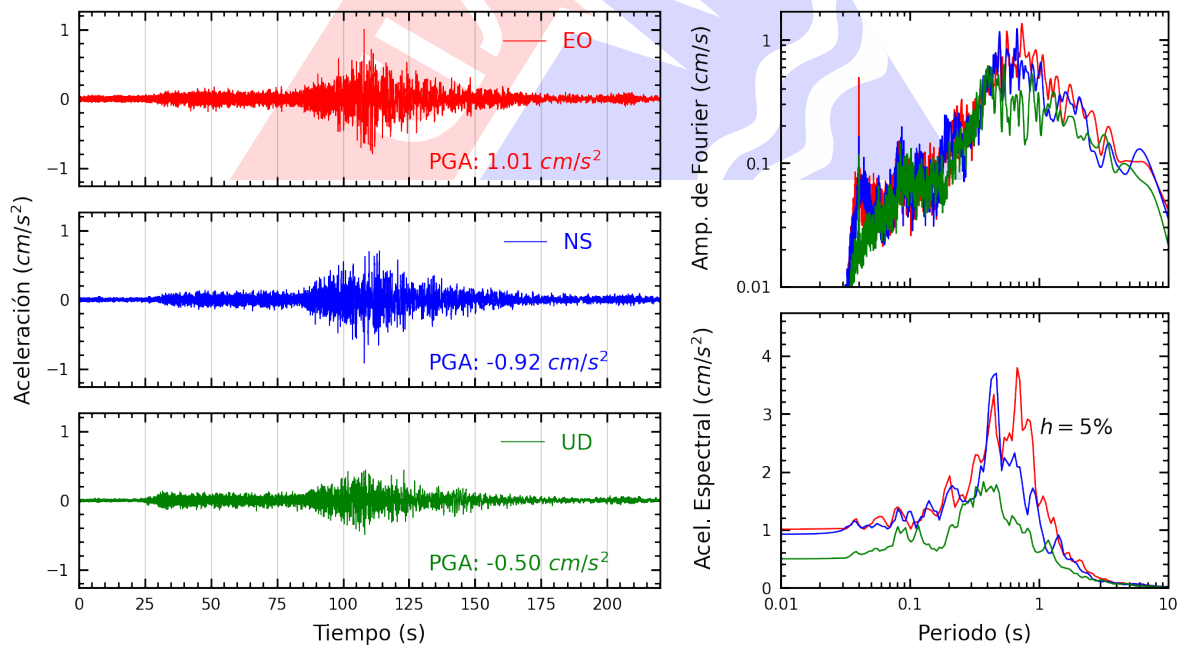
Figura A.22: Registros tiempo-historia, espectros de Fourier y de respuesta en las direcciones EO, NS y vertical de la estación COMAS. Sismo de Aplao, Castilla - Arequipa del 2023-12-20, 07:11:20 (Hora local)
