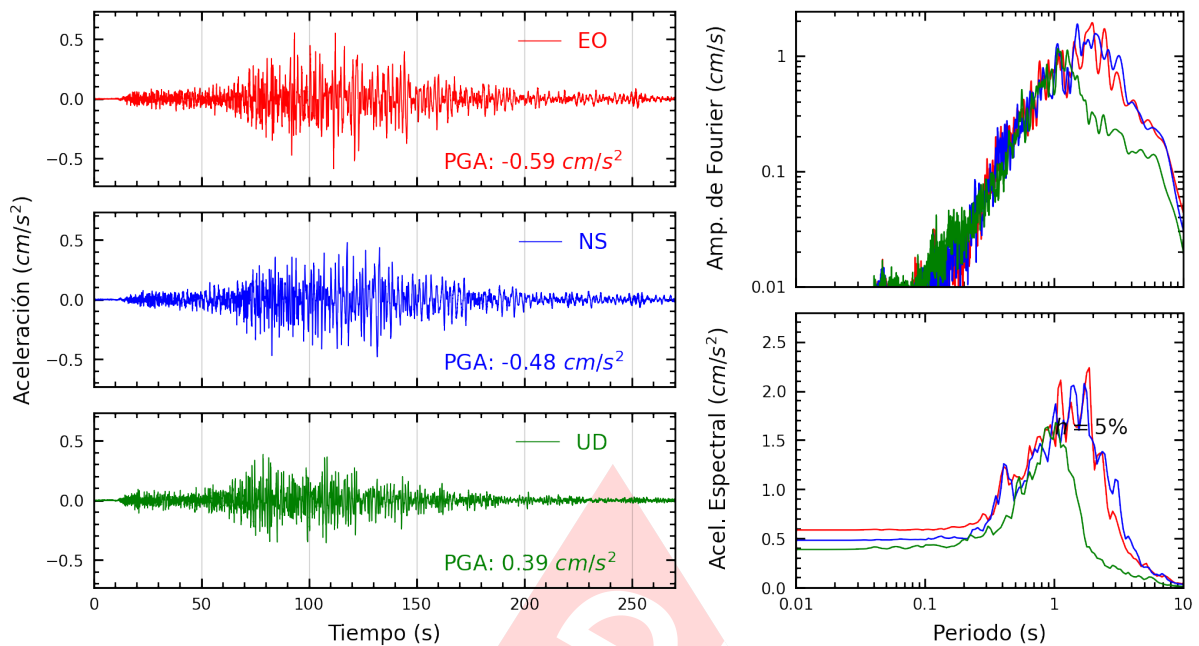
Figura A.31: Registros tiempo-historia, espectros de Fourier y de respuesta en las direcciones EO, NS y vertical de la estación UNCP. Sismo de Aplao, Castilla - Arequipa del 2023-12-20, 07:11:20 (Hora local)
