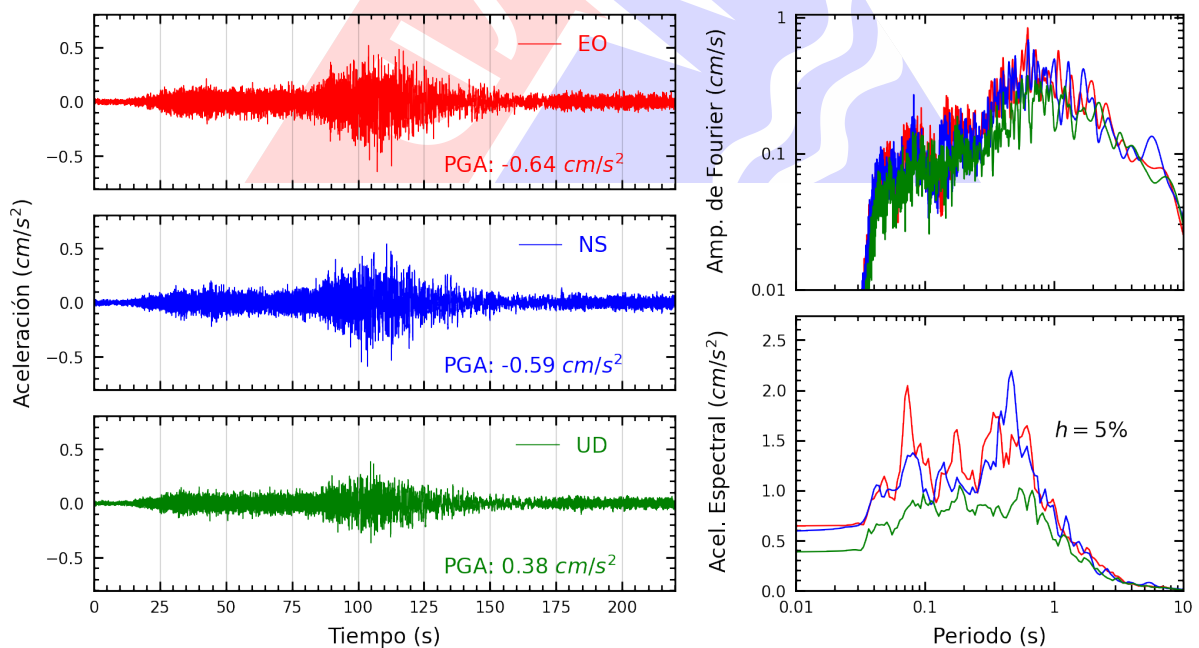
Figura A.30: Registros tiempo-historia, espectros de Fourier y de respuesta en las direcciones EO, NS y vertical de la estación FICPE. Sismo de Aplao, Castilla - Arequipa del 2023-12-20, 07:11:20 (Hora local)
