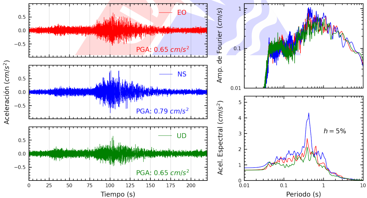
Figura A.26: Registros tiempo-historia, espectros de Fourier y de respuesta en las direcciones EO, NS y vertical de la estación URPPPE. Sismo de Aplao, Castilla - Arequipa del 2023-12-20, 07:11:20 (Hora local)
