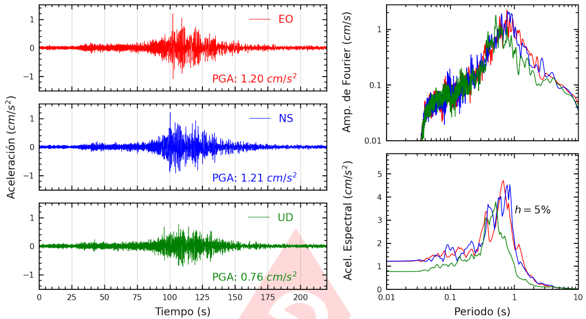
Figura A.17: Registros tiempo-historia, espectros de Fourier y de respuesta en las direcciones EO, NS y vertical de la estación IMCA. Sismo de Aplao, Castilla - Arequipa del 2023-12-20, 07:11:20 (Hora local)
