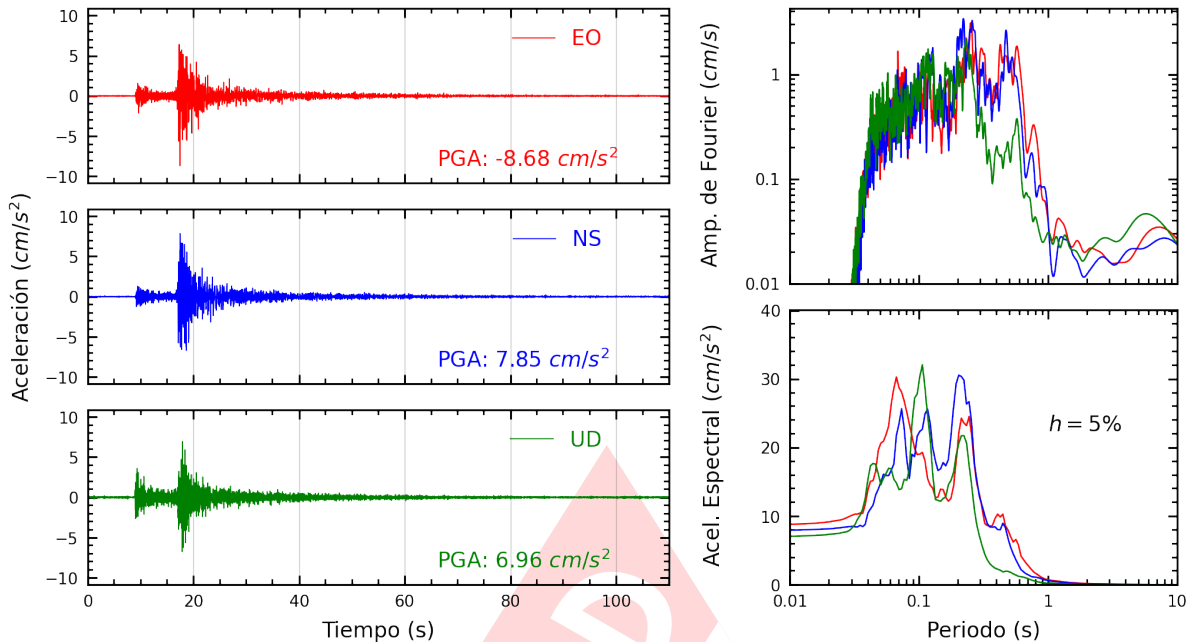
Figura A.5: Registros tiempo-historia, espectros de Fourier y de respuesta en las direcciones EO, NS y vertical de la estación MDPP. Sismo de Ancon, Lima - Lima del 2023-12-29, 09:49:46 (Hora local)
