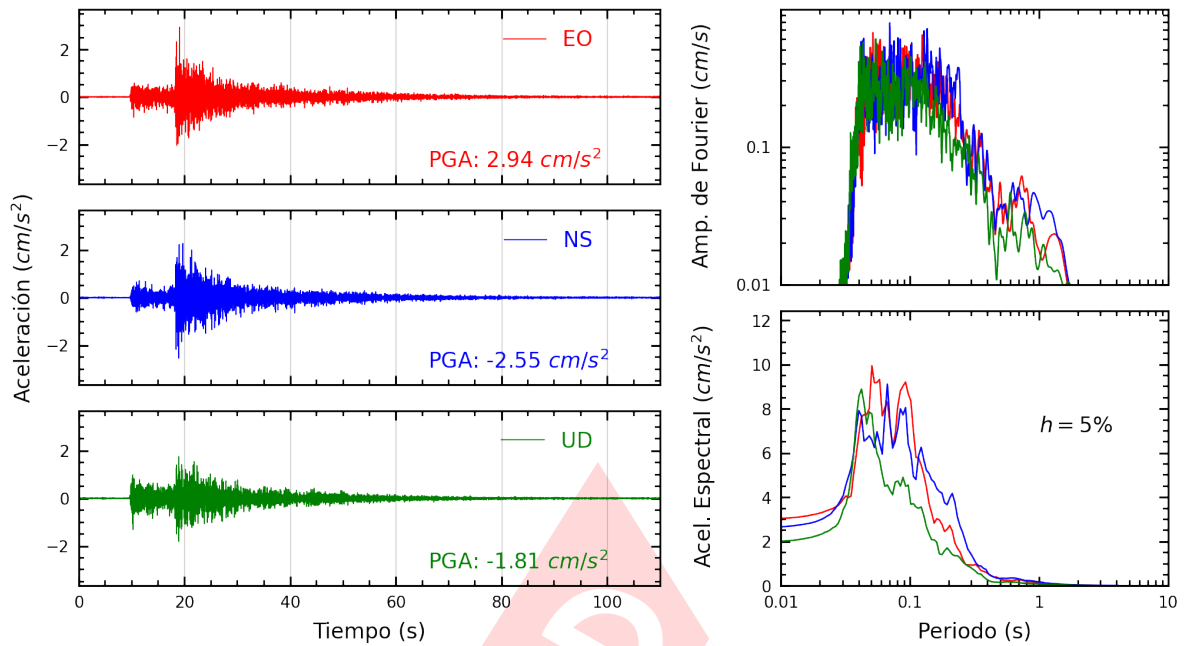
Figura A.17: Registros tiempo-historia, espectros de Fourier y de respuesta en las direcciones EO, NS y vertical de la estación JALV2. Sismo de Ancon, Lima - Lima del 2023-12-29, 09:49:46 (Hora local)
