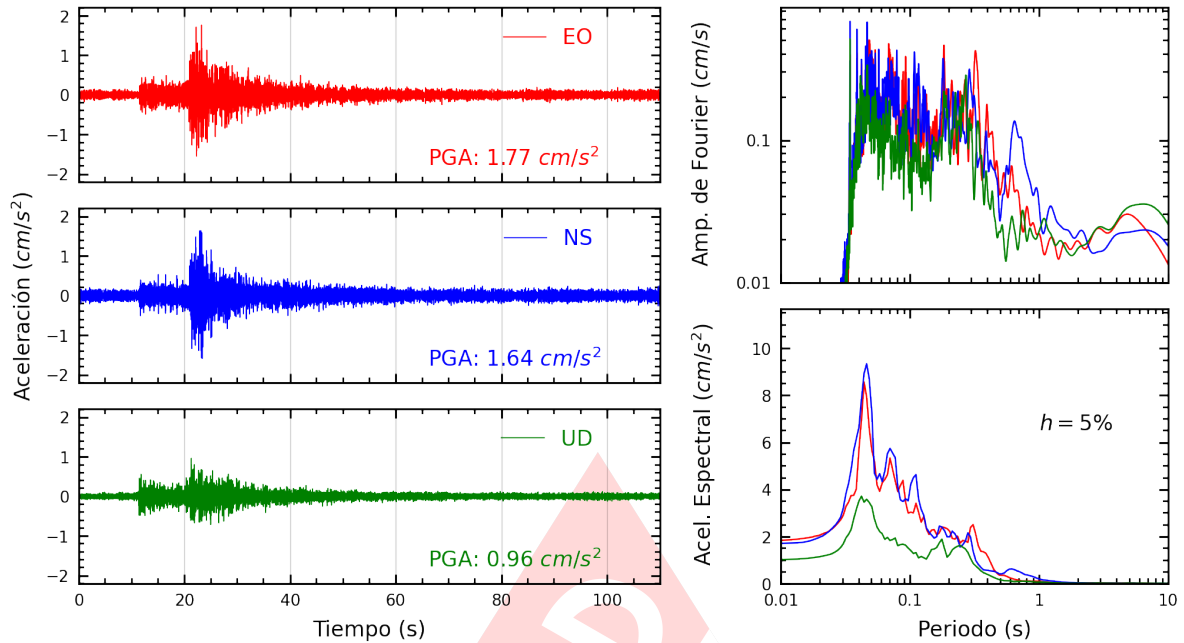
Figura A.25: Registros tiempo-historia, espectros de Fourier y de respuesta en las direcciones EO, NS y vertical de la estación UPCVI. Sismo de Ancon, Lima - Lima del 2023-12-29, 09:49:46 (Hora local)
