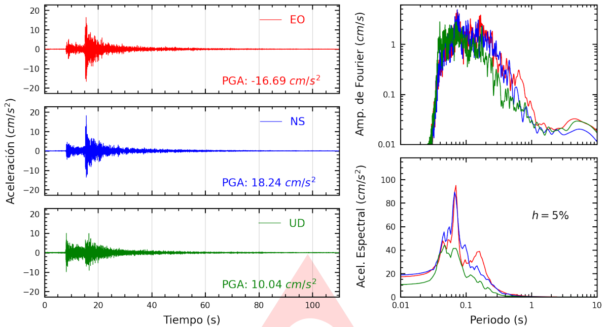
Figura A.1: Registros tiempo-historia, espectros de Fourier y de respuesta en las direcciones EO, NS y vertical de la estación ANCON. Sismo de Ancon, Lima - Lima del 2023-12-29, 09:49:46 (Hora local)
