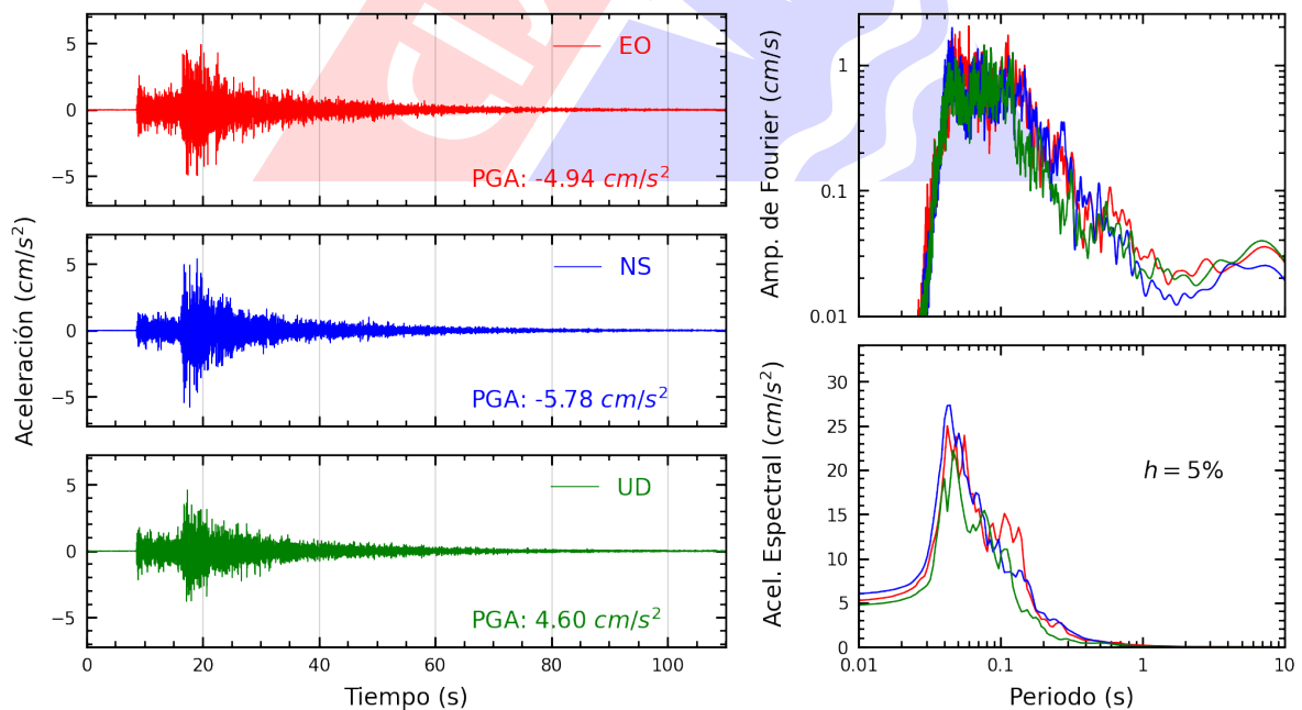
Figura A.8: Registros tiempo-historia, espectros de Fourier y de respuesta en las direcciones EO, NS y vertical de la estación AMORE. Sismo de Ancon, Lima - Lima del 2023-12-29, 09:49:46 (Hora local)
