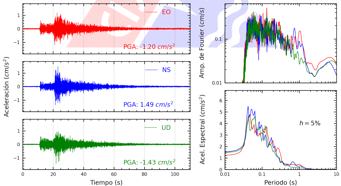
Figura A.30: Registros tiempo-historia, espectros de Fourier y de respuesta en las direcciones EO, NS y vertical de la estación IMCA. Sismo de Ancon, Lima - Lima del 2023-12-29, 09:49:46 (Hora local)
