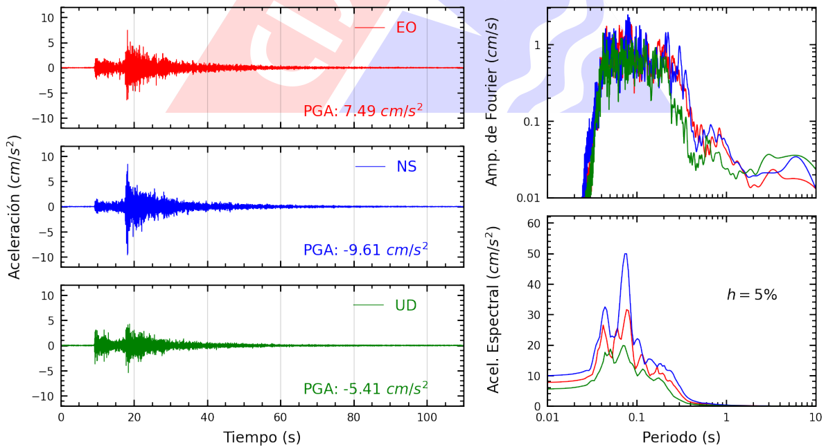
Figura A.4: Registros tiempo-historia, espectros de Fourier y de respuesta en las direcciones EO, NS y vertical de la estación INDEP. Sismo de Ancon, Lima - Lima del 2023-12-29, 09:49:46 (Hora local)
