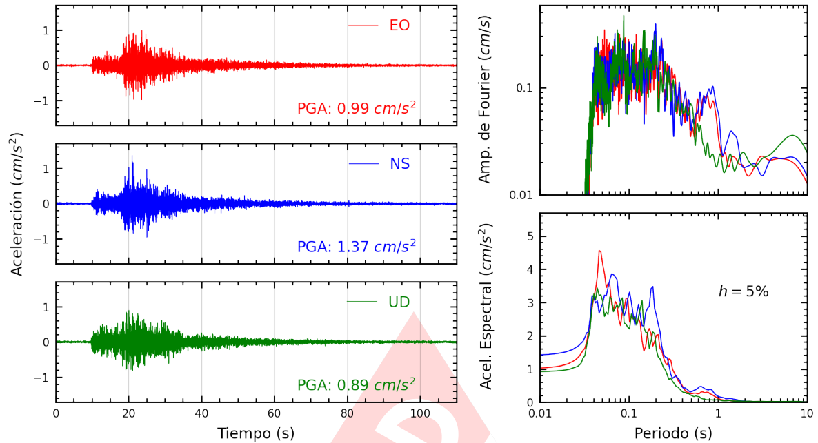
Figura A.31: Registros tiempo-historia, espectros de Fourier y de respuesta en las direcciones EO, NS y vertical de la estación UNFV. Sismo de Ancon, Lima - Lima del 2023-12-29, 09:49:46 (Hora local)
