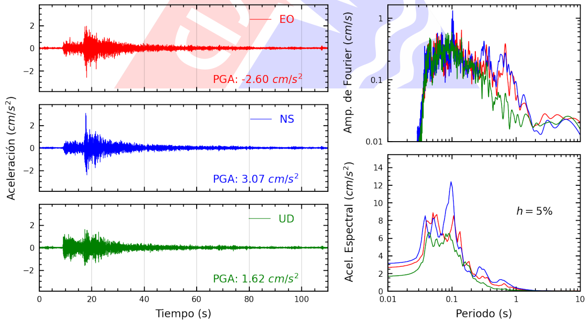
Figura A.14: Registros tiempo-historia, espectros de Fourier y de respuesta en las direcciones EO, NS y vertical de la estación MADRE. Sismo de Ancon, Lima - Lima del 2023-12-29, 09:49:46 (Hora local)
