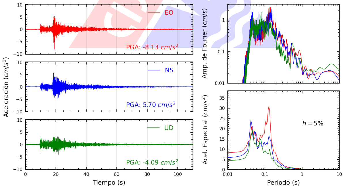
Figura A.6: Registros tiempo-historia, espectros de Fourier y de respuesta en las direcciones EO, NS y vertical de la estación CARAB. Sismo de Ancon, Lima - Lima del 2023-12-29, 09:49:46 (Hora local)
