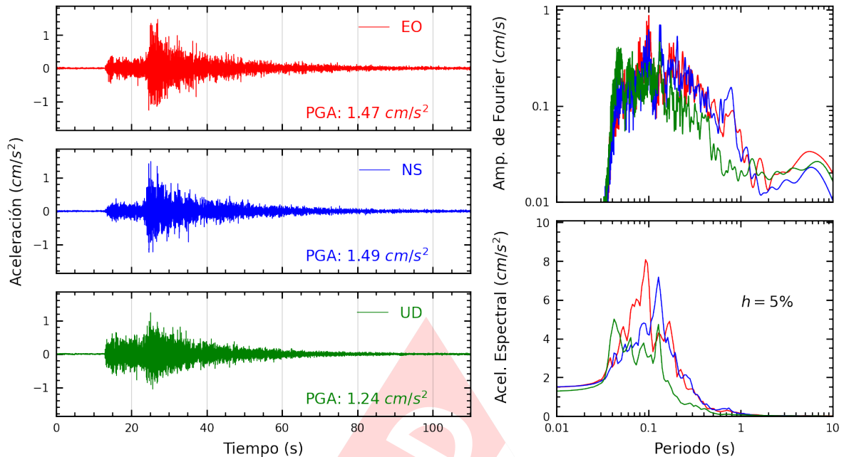
Figura A.29: Registros tiempo-historia, espectros de Fourier y de respuesta en las direcciones EO, NS y vertical de la estación USILP. Sismo de Ancon, Lima - Lima del 2023-12-29, 09:49:46 (Hora local)
