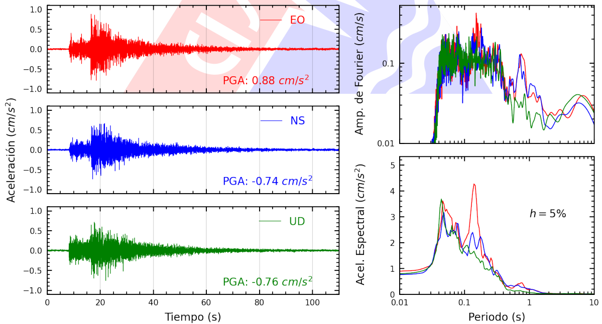
Figura A.34: Registros tiempo-historia, espectros de Fourier y de respuesta en las direcciones EO, NS y vertical de la estación UNMSM. Sismo de Ancon, Lima - Lima del 2023-12-29, 09:49:46 (Hora local)
