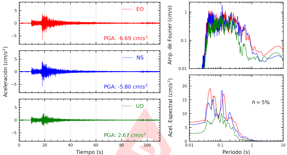
Figura A.7: Registros tiempo-historia, espectros de Fourier y de respuesta en las direcciones EO, NS y vertical de la estación OLIVO. Sismo de Ancon, Lima - Lima del 2023-12-29, 09:49:46 (Hora local)
