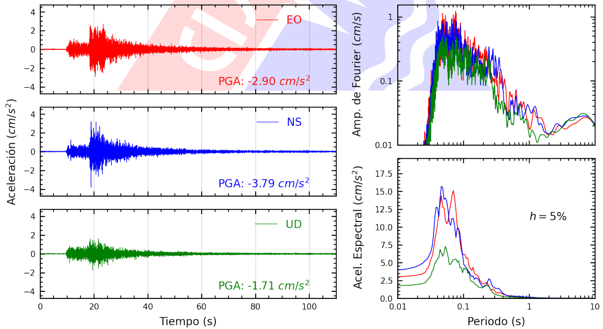
Figura A.12: Registros tiempo-historia, espectros de Fourier y de respuesta en las direcciones EO, NS y vertical de la estación FICPE. Sismo de Ancon, Lima - Lima del 2023-12-29, 09:49:46 (Hora local)
