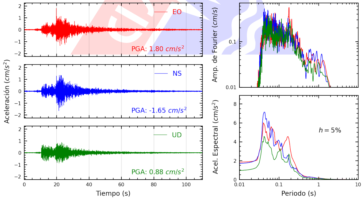
Figura A.24: Registros tiempo-historia, espectros de Fourier y de respuesta en las direcciones EO, NS y vertical de la estación BORJA. Sismo de Ancon, Lima - Lima del 2023-12-29, 09:49:46 (Hora local)
