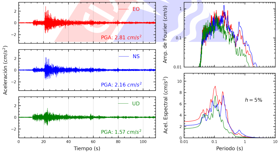
Figura A.18: Registros tiempo-historia, espectros de Fourier y de respuesta en las direcciones EO, NS y vertical de la estación SCCHO. Sismo de Ancon, Lima - Lima del 2023-12-29, 09:49:46 (Hora local)
