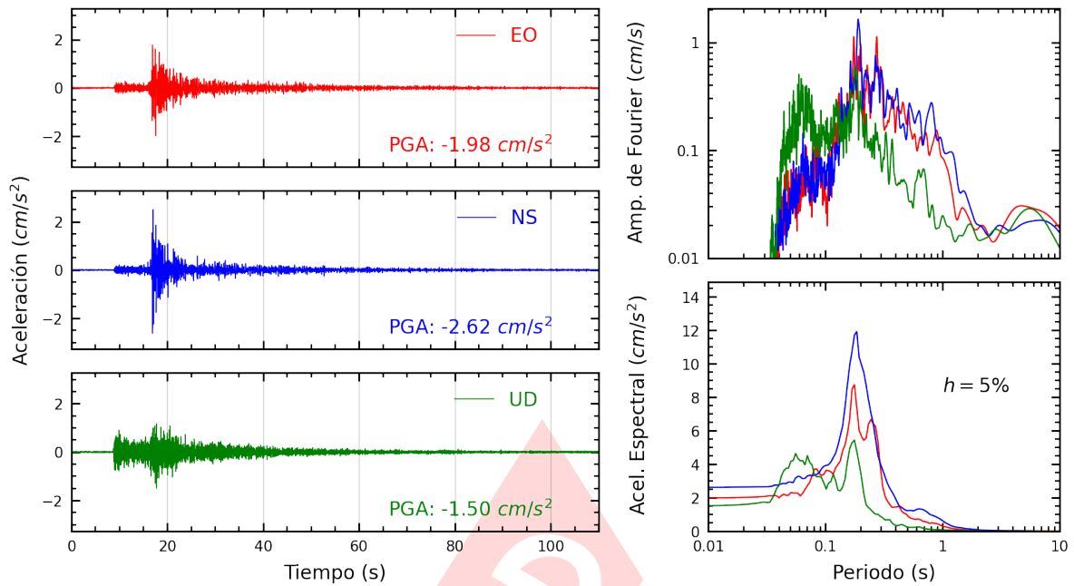
Figura A.19: Registros tiempo-historia, espectros de Fourier y de respuesta en las direcciones EO, NS y vertical de la estación ACAPU. Sismo de Ancon, Lima - Lima del 2023-12-29, 09:49:46 (Hora local)
