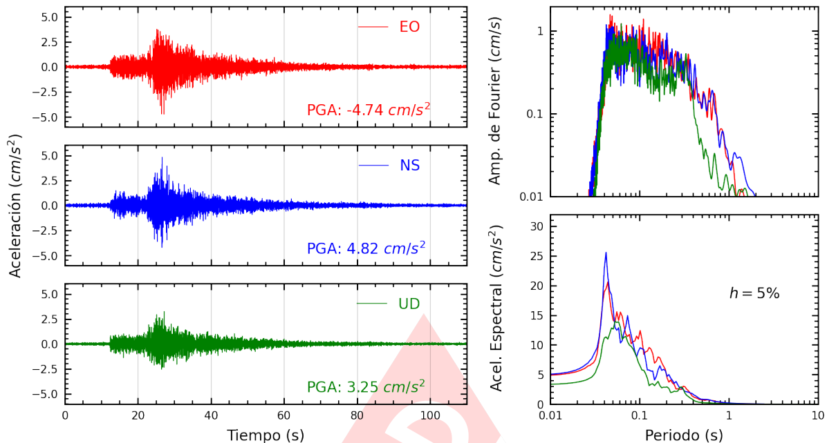
Figura A.9: Registros tiempo-historia, espectros de Fourier y de respuesta en las direcciones EO, NS y vertical de la estación UNTEL. Sismo de Ancon, Lima - Lima del 2023-12-29, 09:49:46 (Hora local)
