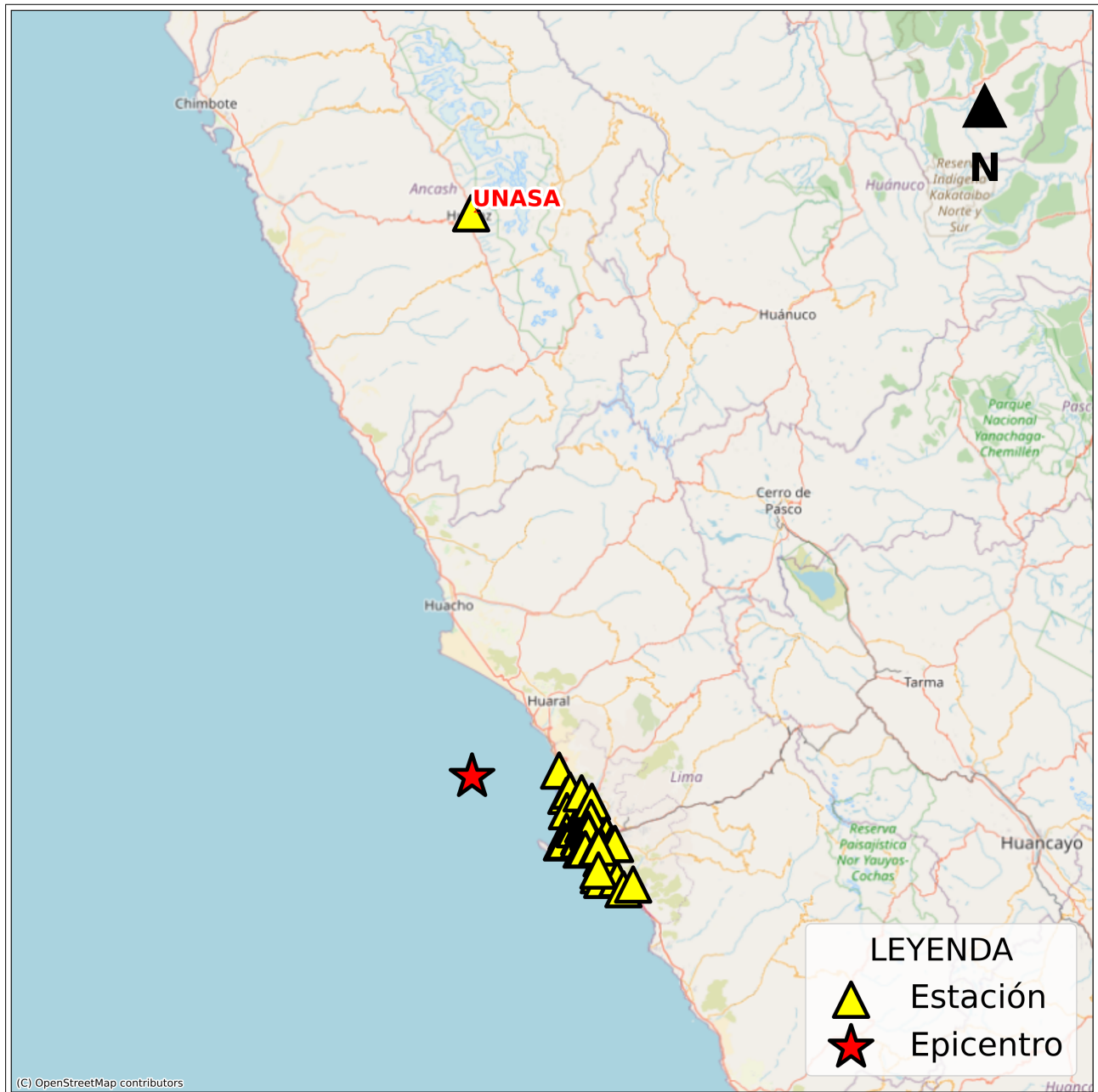
Figura 2: Mapa de ubicación de la(s) estación(es) acelerográfica(s) a nivel nacional correspondiente(s) al Sismo de Ancon, Lima - Lima del 29 de diciembre de 2023 a las 09:49:46 (hora local)
