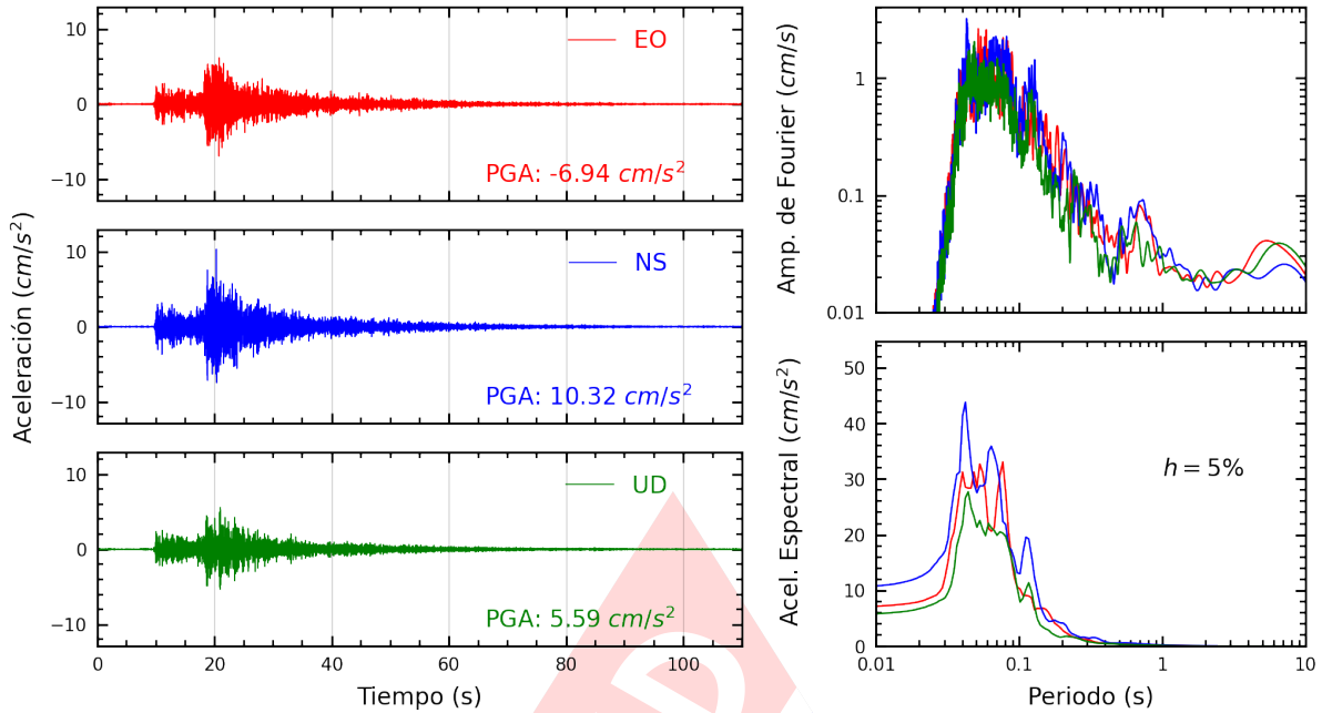
Figura A.3: Registros tiempo-historia, espectros de Fourier y de respuesta en las direcciones EO, NS y vertical de la estación JOSEO. Sismo de Ancon, Lima - Lima del 2023-12-29, 09:49:46 (Hora local)
