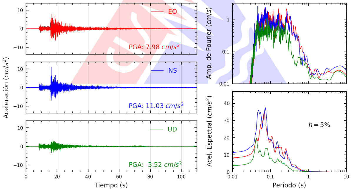
Figura A.2: Registros tiempo-historia, espectros de Fourier y de respuesta en las direcciones EO, NS y vertical de la estación DEFEN. Sismo de Ancon, Lima - Lima del 2023-12-29, 09:49:46 (Hora local)
