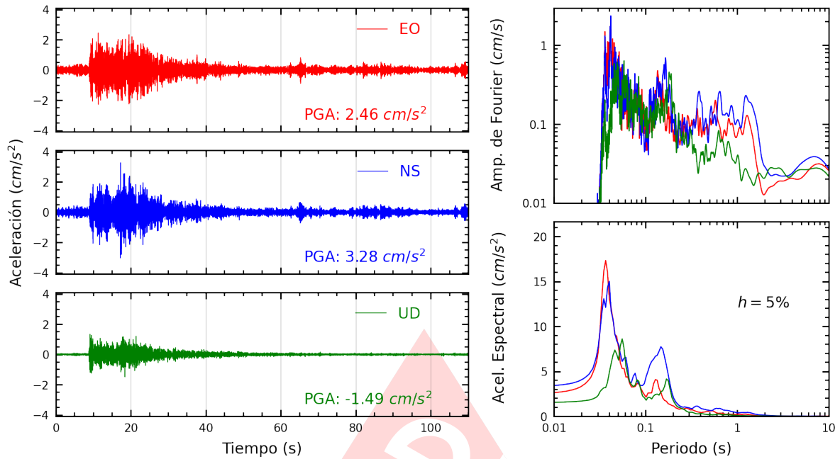
Figura A.13: Registros tiempo-historia, espectros de Fourier y de respuesta en las direcciones EO, NS y vertical de la estación DHNPE. Sismo de Ancon, Lima - Lima del 2023-12-29, 09:49:46 (Hora local)
