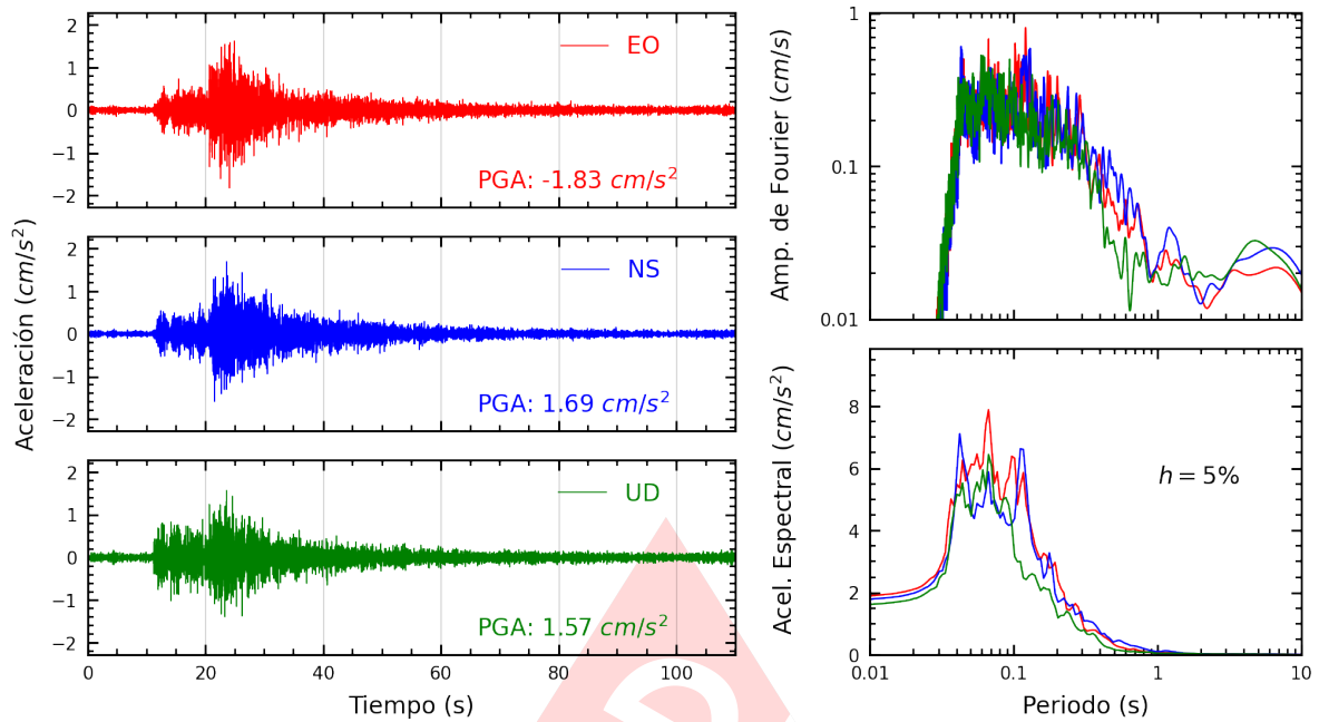
Figura A.23: Registros tiempo-historia, espectros de Fourier y de respuesta en las direcciones EO, NS y vertical de la estación URPE. Sismo de Ancon, Lima - Lima del 2023-12-29, 09:49:46 (Hora local)
