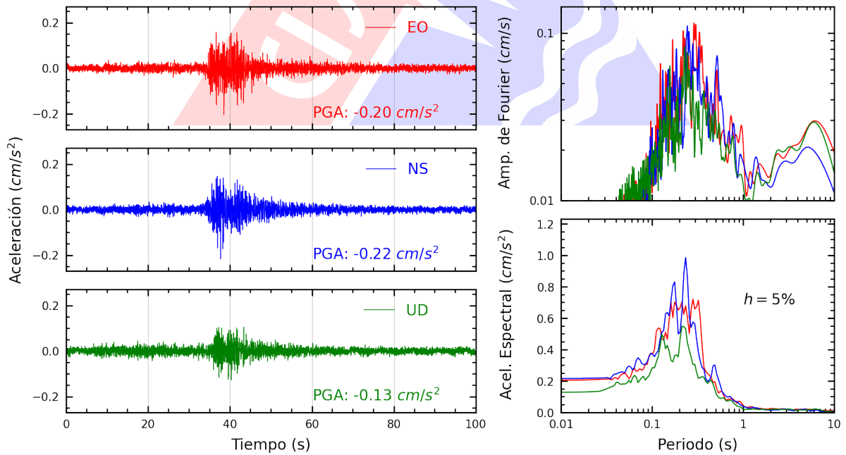
Figura A.36: Registros tiempo-historia, espectros de Fourier y de respuesta en las direcciones EO, NS y vertical de la estación UNASA. Sismo de Ancon, Lima - Lima del 2023-12-29, 09:49:46 (Hora local)
