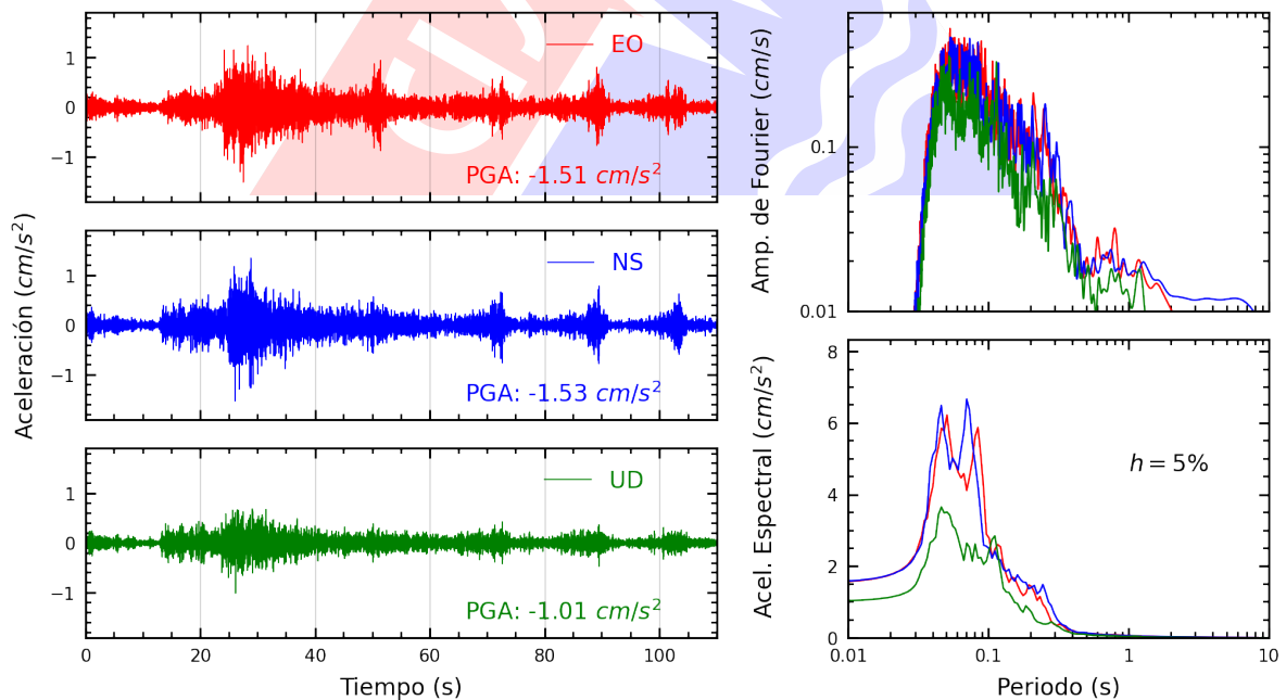
Figura A.28: Registros tiempo-historia, espectros de Fourier y de respuesta en las direcciones EO, NS y vertical de la estación PACHA. Sismo de Ancon, Lima - Lima del 2023-12-29, 09:49:46 (Hora local)
