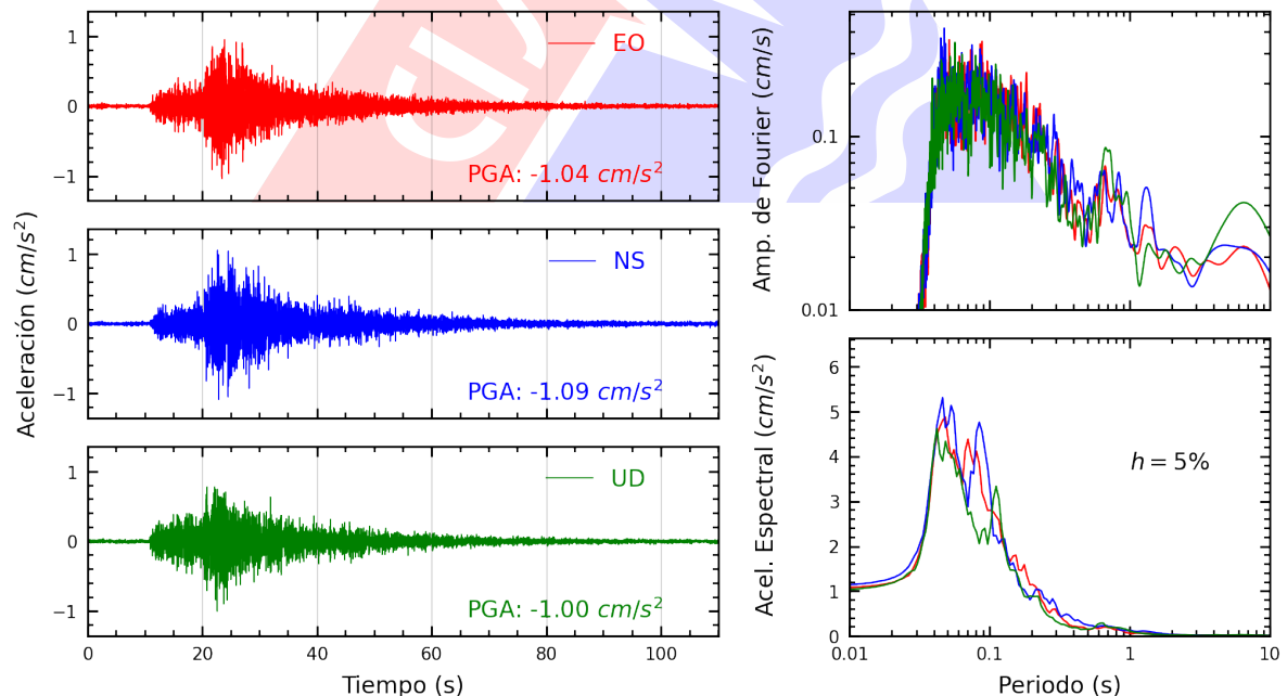
Figura A.32: Registros tiempo-historia, espectros de Fourier y de respuesta en las direcciones EO, NS y vertical de la estación SERVI. Sismo de Ancon, Lima - Lima del 2023-12-29, 09:49:46 (Hora local)
