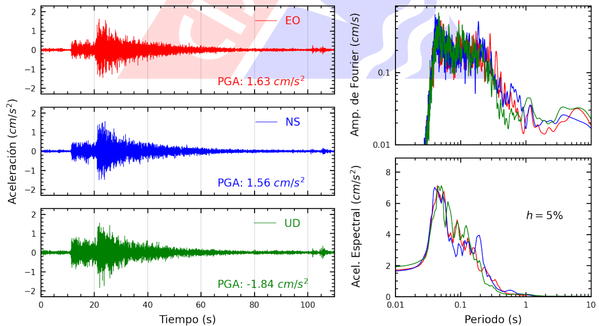
Figura A.22: Registros tiempo-historia, espectros de Fourier y de respuesta en las direcciones EO, NS y vertical de la estación USMP. Sismo de Ancon, Lima - Lima del 2023-12-29, 09:49:46 (Hora local)
