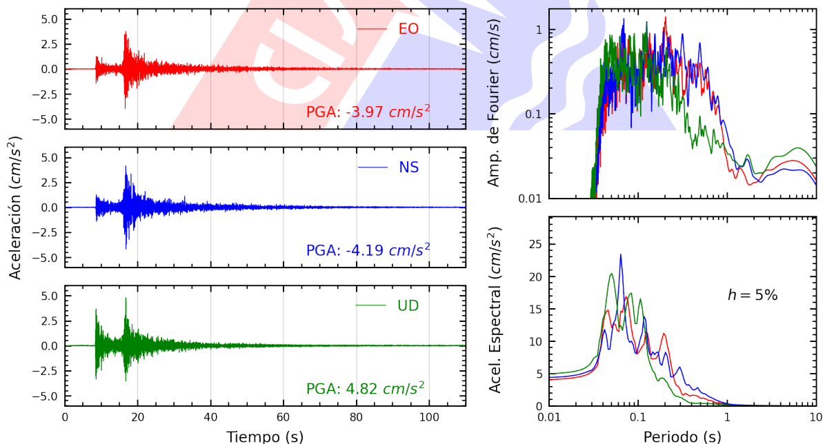
Figura A.10: Registros tiempo-historia, espectros de Fourier y de respuesta en las direcciones EO, NS y vertical de la estación VHAYA. Sismo de Ancon, Lima - Lima del 2023-12-29, 09:49:46 (Hora local)
