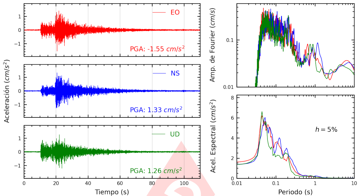
Figura A.27: Registros tiempo-historia, espectros de Fourier y de respuesta en las direcciones EO, NS y vertical de la estación CENEP. Sismo de Ancon, Lima - Lima del 2023-12-29, 09:49:46 (Hora local)
