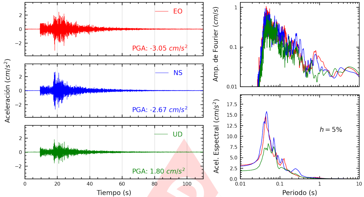
Figura A.15: Registros tiempo-historia, espectros de Fourier y de respuesta en las direcciones EO, NS y vertical de la estación UCSS. Sismo de Ancon, Lima - Lima del 2023-12-29, 09:49:46 (Hora local)
