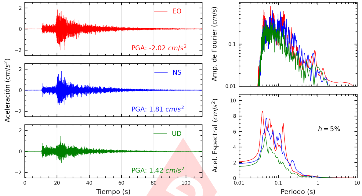
Figura A.21: Registros tiempo-historia, espectros de Fourier y de respuesta en las direcciones EO, NS y vertical de la estación ATARJ. Sismo de Ancon, Lima - Lima del 2023-12-29, 09:49:46 (Hora local)
