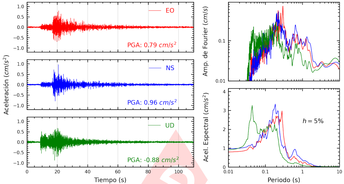
Figura A.33: Registros tiempo-historia, espectros de Fourier y de respuesta en las direcciones EO, NS y vertical de la estación DSML. Sismo de Ancon, Lima - Lima del 2023-12-29, 09:49:46 (Hora local)
