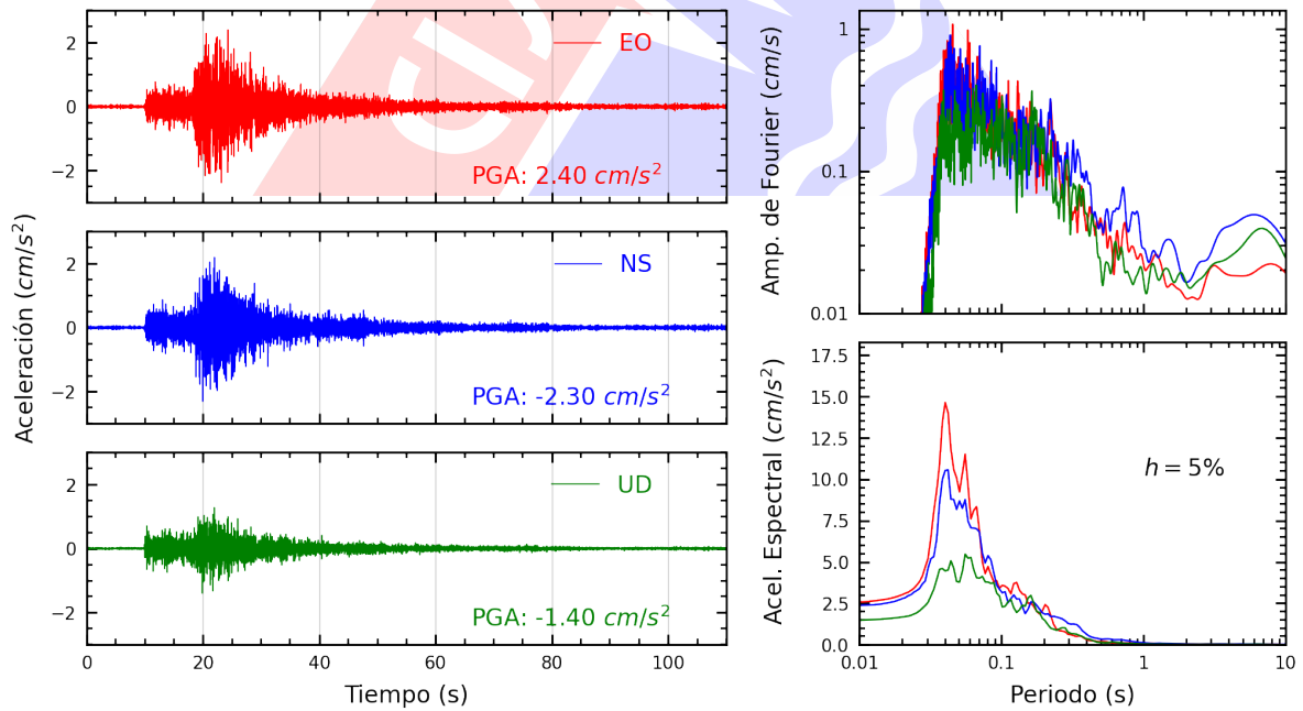
Figura A.20: Registros tiempo-historia, espectros de Fourier y de respuesta en las direcciones EO, NS y vertical de la estación CEPRE. Sismo de Ancon, Lima - Lima del 2023-12-29, 09:49:46 (Hora local)
