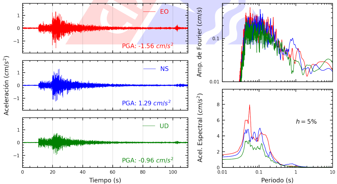
Figura A.26: Registros tiempo-historia, espectros de Fourier y de respuesta en las direcciones EO, NS y vertical de la estación INICT. Sismo de Ancon, Lima - Lima del 2023-12-29, 09:49:46 (Hora local)
