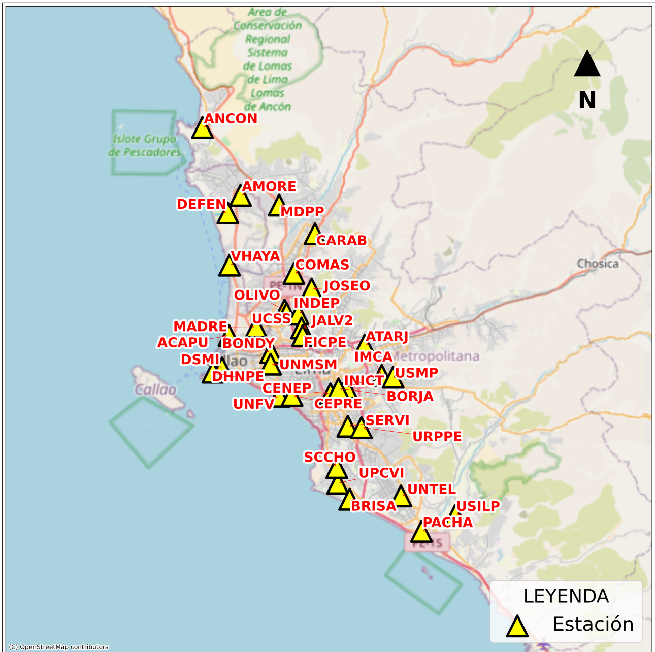
Figura 3: Mapa de ubicación de la(s) estación(es) acelerográfica(s) en Lima Metropolitana correspondiente(s) al Sismo de Ancon, Lima - Lima del 29 de diciembre de 2023 a las 09:49:46 (hora local)
