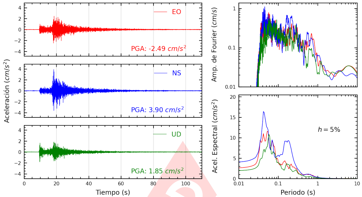
Figura A.11: Registros tiempo-historia, espectros de Fourier y de respuesta en las direcciones EO, NS y vertical de la estación COMAS. Sismo de Ancon, Lima - Lima del 2023-12-29, 09:49:46 (Hora local)
