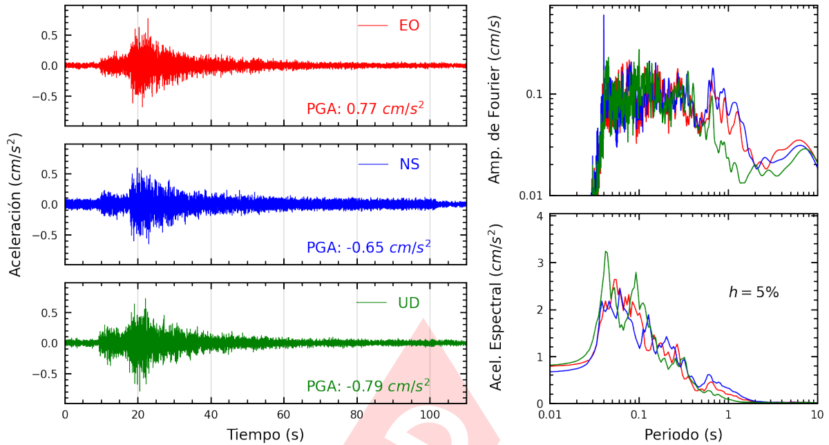
Figura A.35: Registros tiempo-historia, espectros de Fourier y de respuesta en las direcciones EO, NS y vertical de la estación BONDY. Sismo de Ancon, Lima - Lima del 2023-12-29, 09:49:46 (Hora local)
