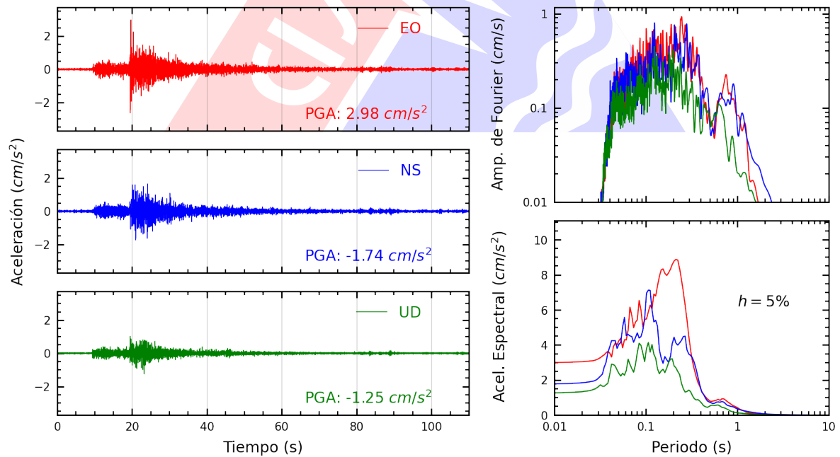
Figura A.16: Registros tiempo-historia, espectros de Fourier y de respuesta en las direcciones EO, NS y vertical de la estación BRISA. Sismo de Ancon, Lima - Lima del 2023-12-29, 09:49:46 (Hora local)
