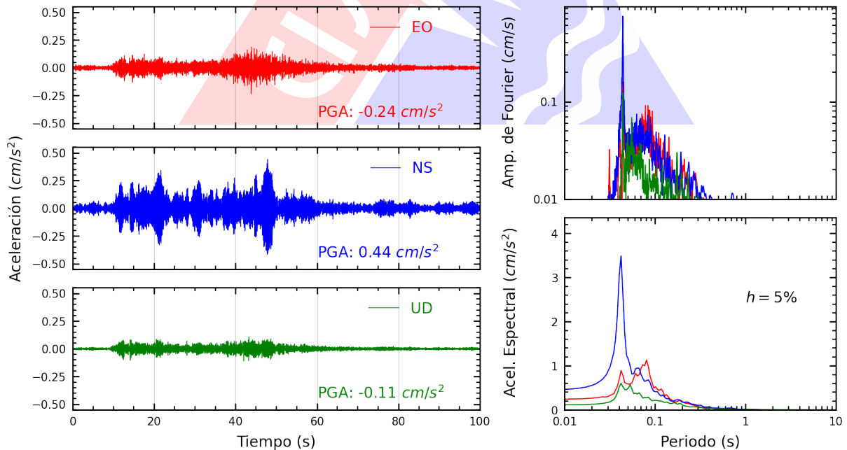
Figura A.4: Registros tiempo-historia, espectros de Fourier y de respuesta en las direcciones EO, NS y vertical de la estación UNAM. Sismo de Chuquibamba, Condesuyos - Arequipa del 2024-01-22, 13:34:38 (Hora local)
