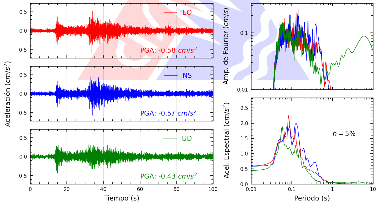
Figura A.2: Registros tiempo-historia, espectros de Fourier y de respuesta en las direcciones EO, NS y vertical de la estación SCARQ. Sismo de Chuquibamba, Condesuyos - Arequipa del 2024-01-22, 13:34:38 (Hora local)
