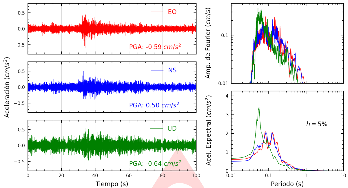
Figura A.1: Registros tiempo-historia, espectros de Fourier y de respuesta en las direcciones EO, NS y vertical de la estación SCAR2. Sismo de Chuquibamba, Condesuyos - Arequipa del 2024-01-22, 13:34:38 (Hora local)
