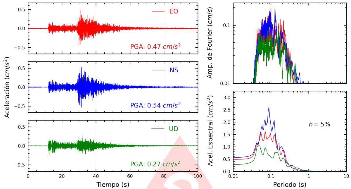
Figura A.3: Registros tiempo-historia, espectros de Fourier y de respuesta en las direcciones EO, NS y vertical de la estación UNSA. Sismo de Chuquibamba, Condesuyos - Arequipa del 2024-01-22, 13:34:38 (Hora local)
