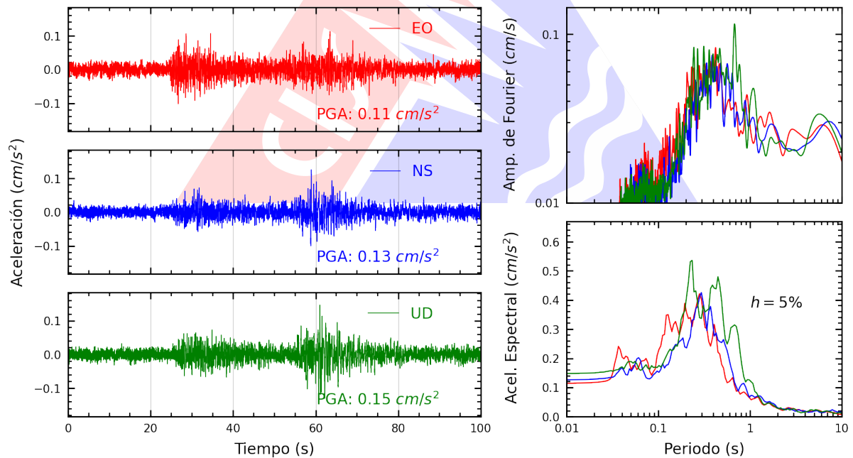
Figura A.2: Registros tiempo-historia, espectros de Fourier y de respuesta en las direcciones EO, NS y vertical de la estación UNSCH. Sismo de Atalaya, Atalaya - Ucayali del 2024-01-25, 14:15:19 (Hora local)
