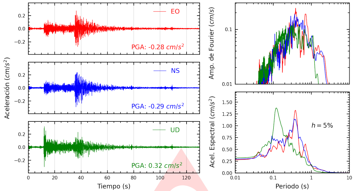
Figura A.1: Registros tiempo-historia, espectros de Fourier y de respuesta en las direcciones EO, NS y vertical de la estación UNCP. Sismo de Atalaya, Atalaya - Ucayali del 2024-01-25, 14:15:19 (Hora local)
