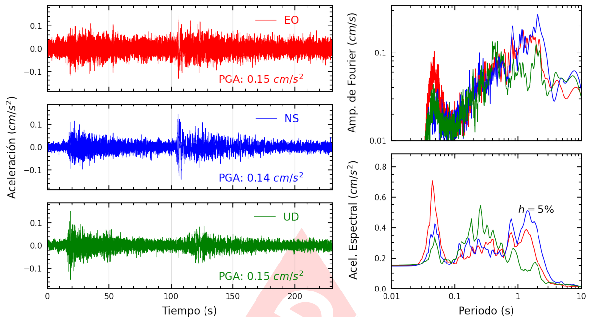
Figura A.25: Registros tiempo-historia, espectros de Fourier y de respuesta en las direcciones EO, NS y vertical de la estación INICT. Sismo de Esperanza, Purus - Ucayali del 2024-01-28, 04:38:50 (Hora local)
