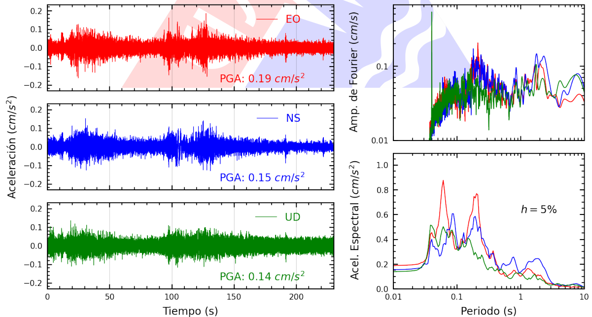
Figura A.20: Registros tiempo-historia, espectros de Fourier y de respuesta en las direcciones EO, NS y vertical de la estación INDEP. Sismo de Esperanza, Purus - Ucayali del 2024-01-28, 04:38:50 (Hora local)
