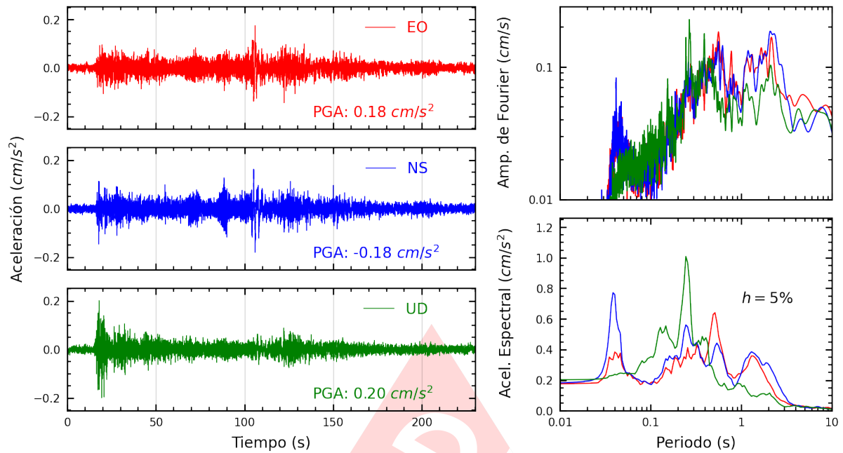
Figura A.19: Registros tiempo-historia, espectros de Fourier y de respuesta en las direcciones EO, NS y vertical de la estación COMAS. Sismo de Esperanza, Purus - Ucayali del 2024-01-28, 04:38:50 (Hora local)
