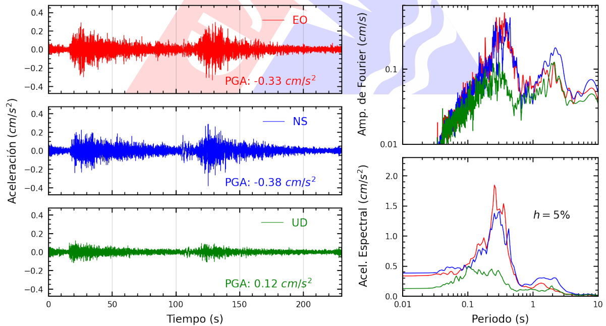
Figura A.10: Registros tiempo-historia, espectros de Fourier y de respuesta en las direcciones EO, NS y vertical de la estación DEFEN. Sismo de Esperanza, Purus - Ucayali del 2024-01-28, 04:38:50 (Hora local)
