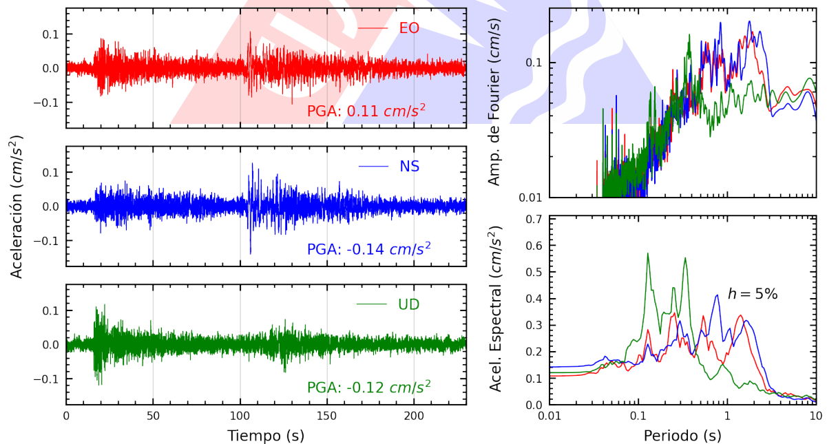
Figura A.26: Registros tiempo-historia, espectros de Fourier y de respuesta en las direcciones EO, NS y vertical de la estación UNMSM. Sismo de Esperanza, Purus - Ucayali del 2024-01-28, 04:38:50 (Hora local)
