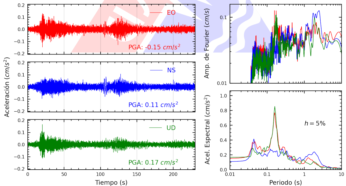
Figura A.22: Registros tiempo-historia, espectros de Fourier y de respuesta en las direcciones EO, NS y vertical de la estación FICPE. Sismo de Esperanza, Purus - Ucayali del 2024-01-28, 04:38:50 (Hora local)
