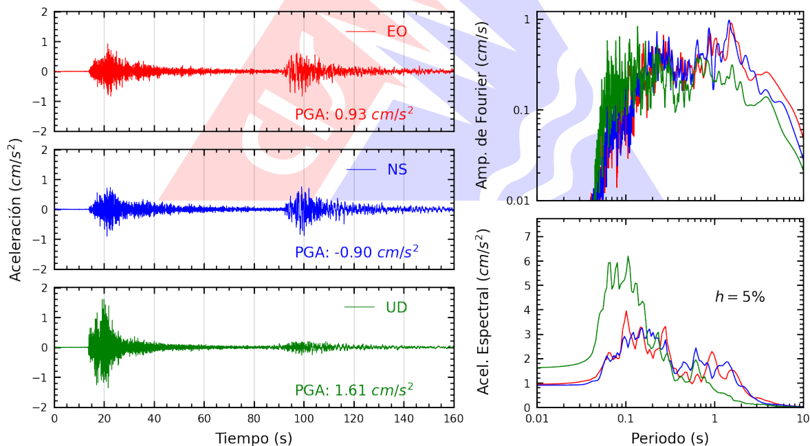
Figura A.2: Registros tiempo-historia, espectros de Fourier y de respuesta en las direcciones EO, NS y vertical de la estación UNAAA. Sismo de Esperanza, Purus - Ucayali del 2024-01-28, 04:38:50 (Hora local)
