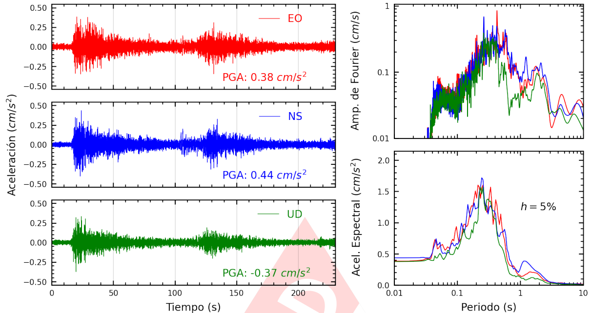
Figura A.7: Registros tiempo-historia, espectros de Fourier y de respuesta en las direcciones EO, NS y vertical de la estación UNTEL. Sismo de Esperanza, Purus - Ucayali del 2024-01-28, 04:38:50 (Hora local)
