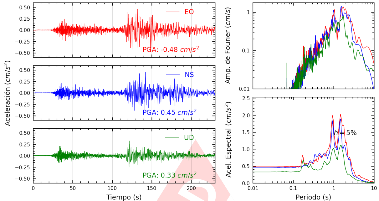
Figura A.5: Registros tiempo-historia, espectros de Fourier y de respuesta en las direcciones EO, NS y vertical de la estación UNC. Sismo de Esperanza, Purus - Ucayali del 2024-01-28, 04:38:50 (Hora local)
