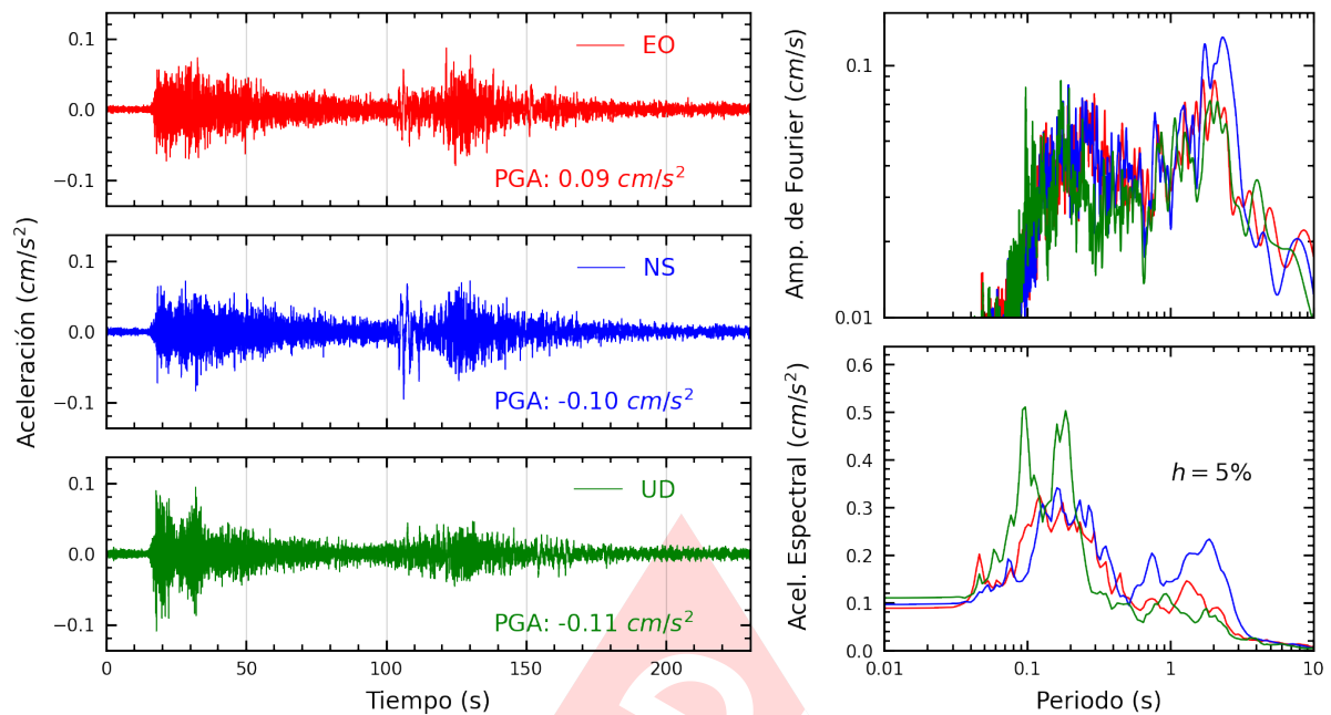
Figura A.29: Registros tiempo-historia, espectros de Fourier y de respuesta en las direcciones EO, NS y vertical de la estación JALV2. Sismo de Esperanza, Purus - Ucayali del 2024-01-28, 04:38:50 (Hora local)
