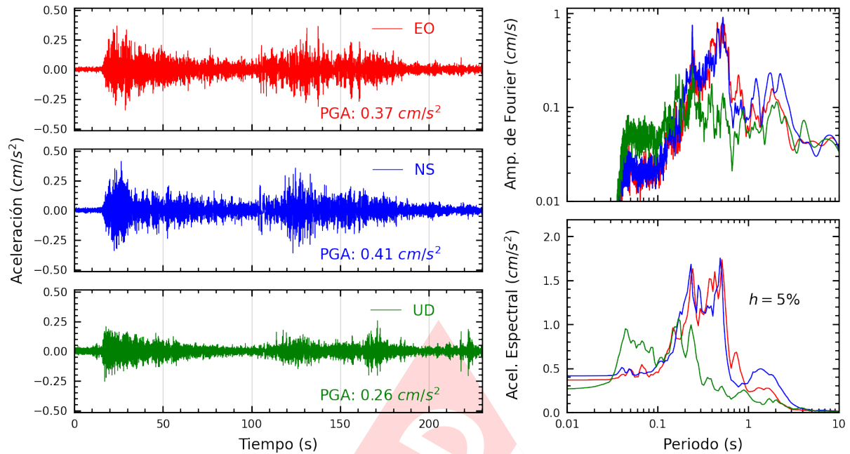
Figura A.9: Registros tiempo-historia, espectros de Fourier y de respuesta en las direcciones EO, NS y vertical de la estación MDPP. Sismo de Esperanza, Purus - Ucayali del 2024-01-28, 04:38:50 (Hora local)
