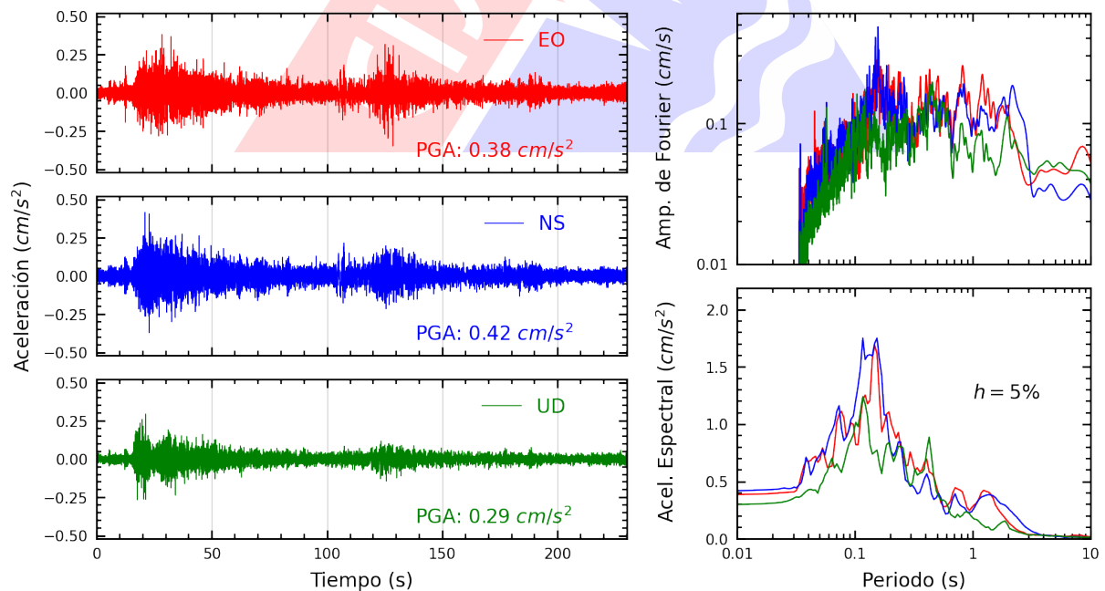
Figura A.8: Registros tiempo-historia, espectros de Fourier y de respuesta en las direcciones EO, NS y vertical de la estación USILM. Sismo de Esperanza, Purus - Ucayali del 2024-01-28, 04:38:50 (Hora local)
