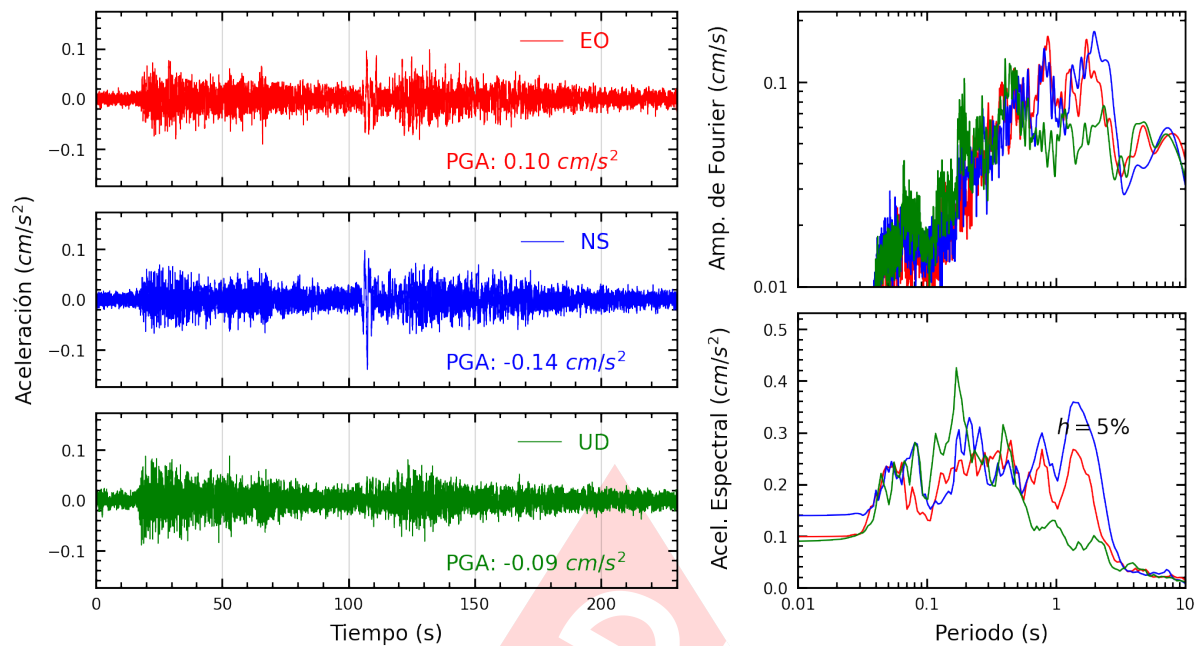
Figura A.27: Registros tiempo-historia, espectros de Fourier y de respuesta en las direcciones EO, NS y vertical de la estación UNFV. Sismo de Esperanza, Purus - Ucayali del 2024-01-28, 04:38:50 (Hora local)
