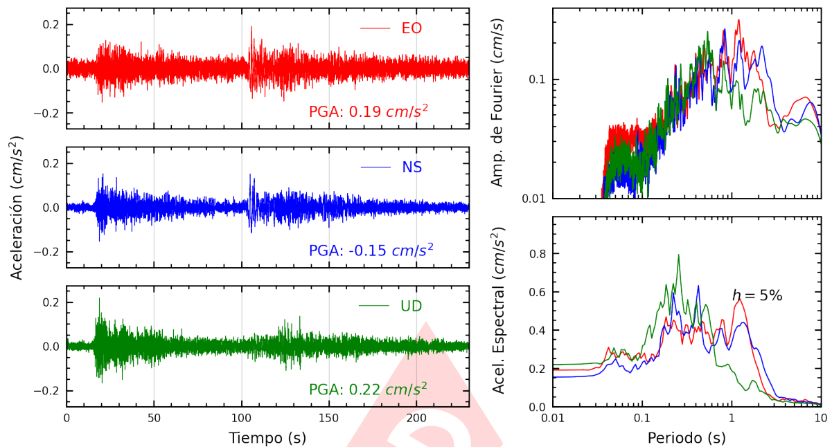
Figura A.17: Registros tiempo-historia, espectros de Fourier y de respuesta en las direcciones EO, NS y vertical de la estación IMCA. Sismo de Esperanza, Purus - Ucayali del 2024-01-28, 04:38:50 (Hora local)
