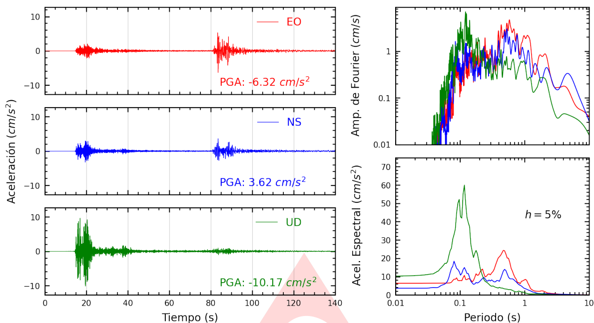
Figura A.1: Registros tiempo-historia, espectros de Fourier y de respuesta en las direcciones EO, NS y vertical de la estación UNIA. Sismo de Esperanza, Purus - Ucayali del 2024-01-28, 04:38:50 (Hora local)
