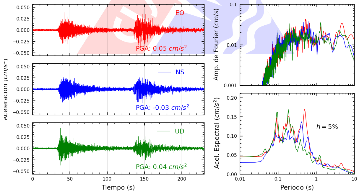
Figura A.30: Registros tiempo-historia, espectros de Fourier y de respuesta en las direcciones EO, NS y vertical de la estación UNSA. Sismo de Esperanza, Purus - Ucayali del 2024-01-28, 04:38:50 (Hora local)
