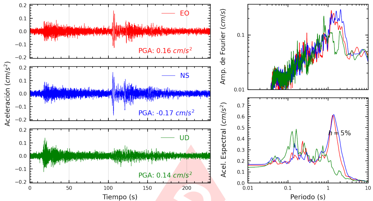
Figura A.21: Registros tiempo-historia, espectros de Fourier y de respuesta en las direcciones EO, NS y vertical de la estación CENEP. Sismo de Esperanza, Purus - Ucayali del 2024-01-28, 04:38:50 (Hora local)
