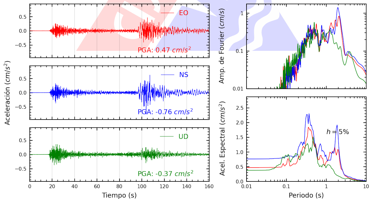
Figura A.4: Registros tiempo-historia, espectros de Fourier y de respuesta en las direcciones EO, NS y vertical de la estación UNCP. Sismo de Esperanza, Purus - Ucayali del 2024-01-28, 04:38:50 (Hora local)
