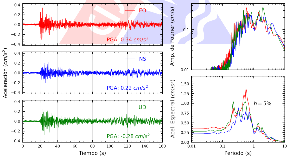
Figura A.12: Registros tiempo-historia, espectros de Fourier y de respuesta en las direcciones EO, NS y vertical de la estación UNSCH. Sismo de Esperanza, Purus - Ucayali del 2024-01-28, 04:38:50 (Hora local)
