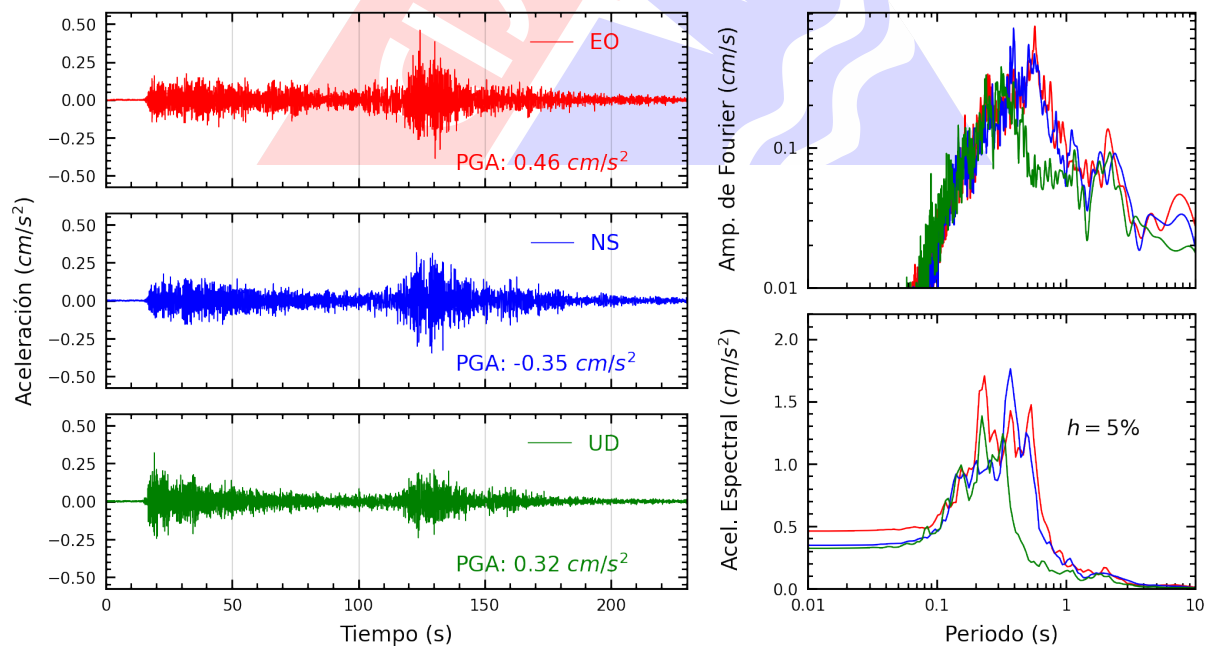
Figura A.6: Registros tiempo-historia, espectros de Fourier y de respuesta en las direcciones EO, NS y vertical de la estación CARAL. Sismo de Esperanza, Purus - Ucayali del 2024-01-28, 04:38:50 (Hora local)
