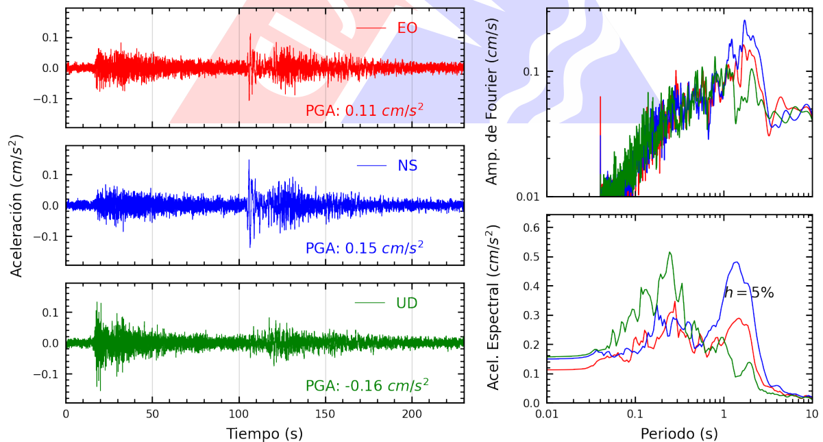
Figura A.24: Registros tiempo-historia, espectros de Fourier y de respuesta en las direcciones EO, NS y vertical de la estación SERVI. Sismo de Esperanza, Purus - Ucayali del 2024-01-28, 04:38:50 (Hora local)
