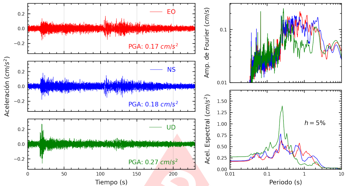
Figura A.15: Registros tiempo-historia, espectros de Fourier y de respuesta en las direcciones EO, NS y vertical de la estación MADRE. Sismo de Esperanza, Purus - Ucayali del 2024-01-28, 04:38:50 (Hora local)
