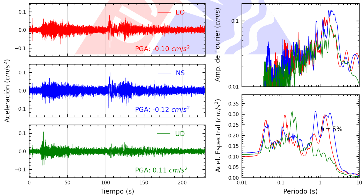
Figura A.28: Registros tiempo-historia, espectros de Fourier y de respuesta en las direcciones EO, NS y vertical de la estación ATARJ. Sismo de Esperanza, Purus - Ucayali del 2024-01-28, 04:38:50 (Hora local)
