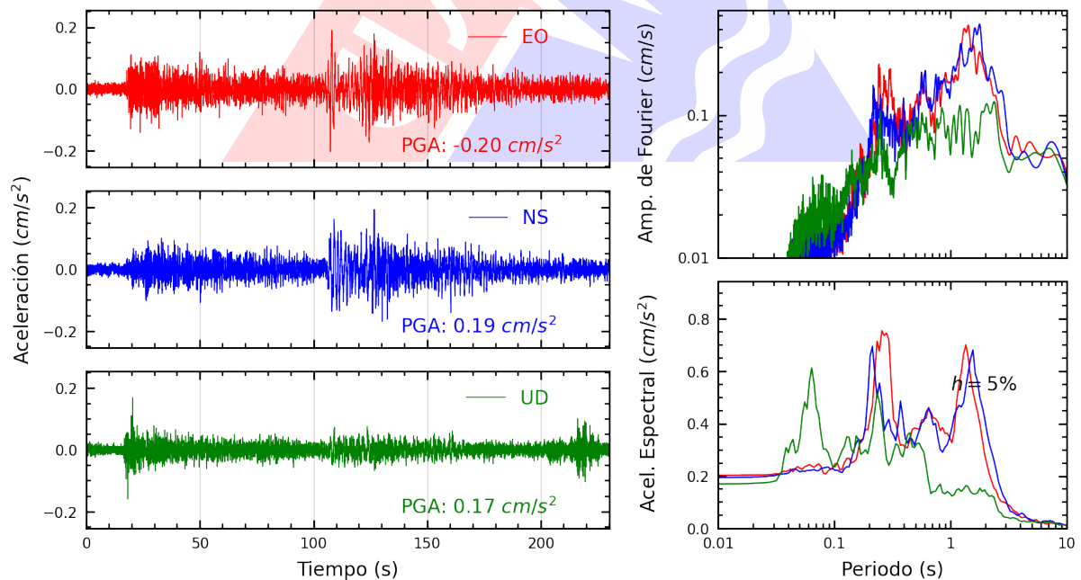
Figura A.18: Registros tiempo-historia, espectros de Fourier y de respuesta en las direcciones EO, NS y vertical de la estación DSMI. Sismo de Esperanza, Purus - Ucayali del 2024-01-28, 04:38:50 (Hora local)
