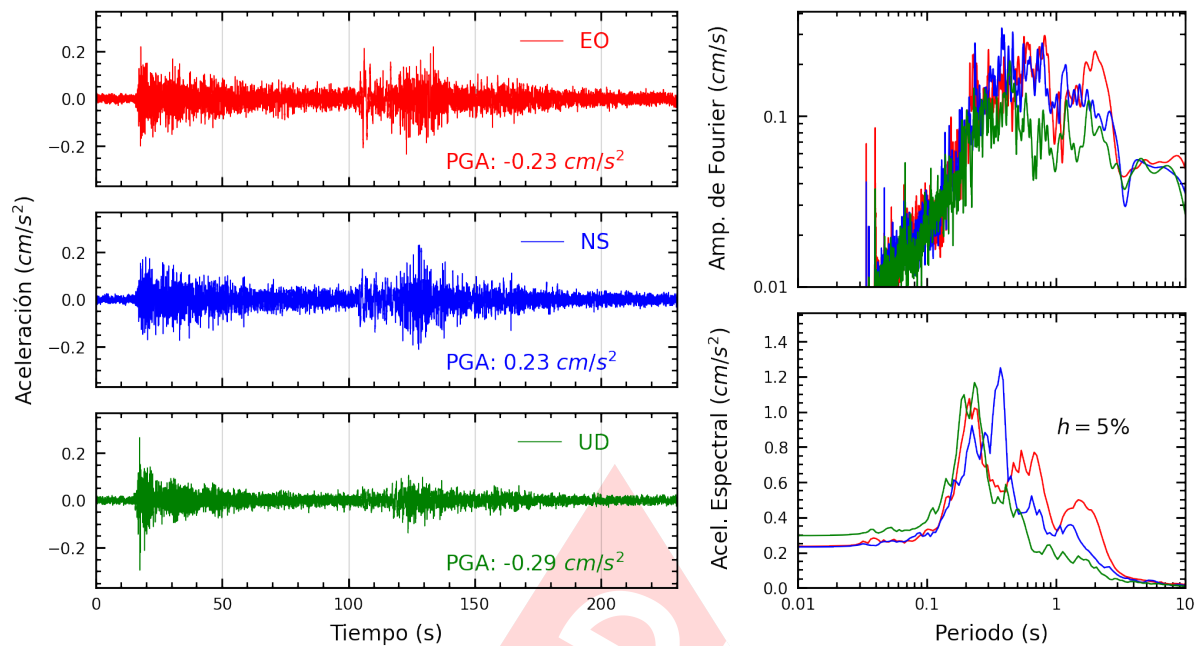
Figura A.13: Registros tiempo-historia, espectros de Fourier y de respuesta en las direcciones EO, NS y vertical de la estación USILP. Sismo de Esperanza, Purus - Ucayali del 2024-01-28, 04:38:50 (Hora local)
