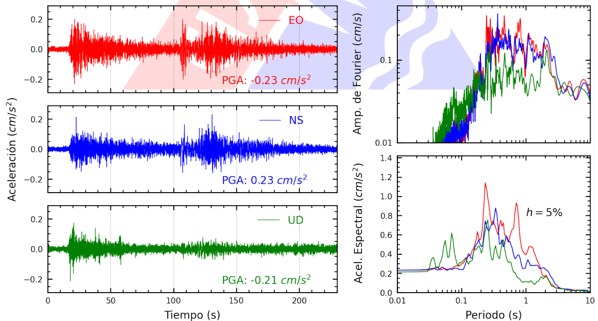
Figura A.16: Registros tiempo-historia, espectros de Fourier y de respuesta en las direcciones EO, NS y vertical de la estación ACAPU. Sismo de Esperanza, Purus - Ucayali del 2024-01-28, 04:38:50 (Hora local)
