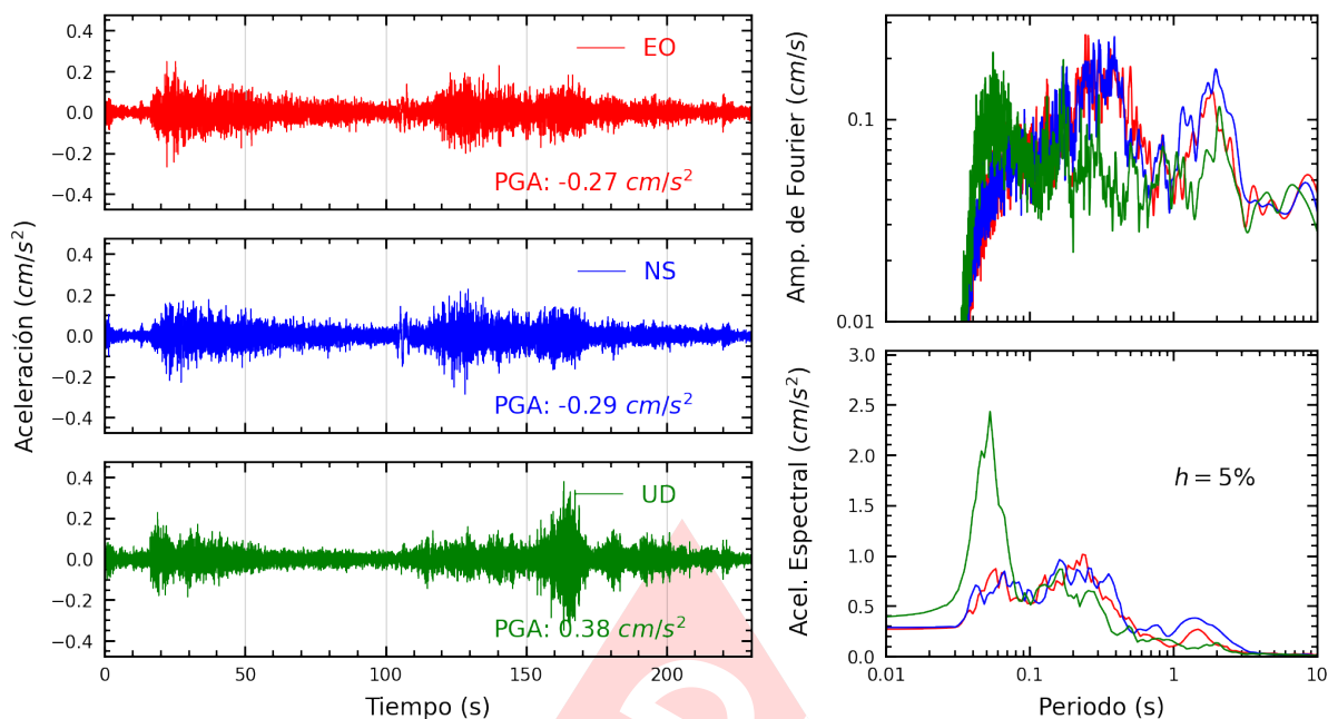
Figura A.11: Registros tiempo-historia, espectros de Fourier y de respuesta en las direcciones EO, NS y vertical de la estación ANCON. Sismo de Esperanza, Purus - Ucayali del 2024-01-28, 04:38:50 (Hora local)
