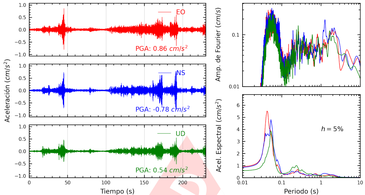
Figura A.3: Registros tiempo-historia, espectros de Fourier y de respuesta en las direcciones EO, NS y vertical de la estación PACHA. Sismo de Esperanza, Purus - Ucayali del 2024-01-28, 04:38:50 (Hora local)
