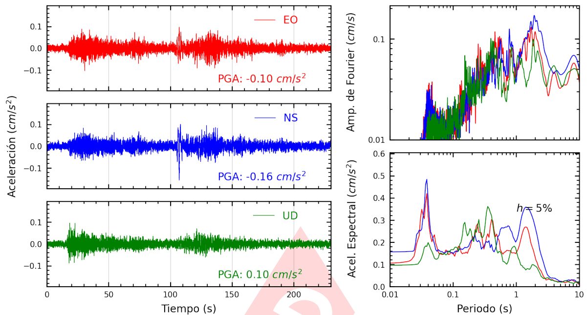
Figura A.23: Registros tiempo-historia, espectros de Fourier y de respuesta en las direcciones EO, NS y vertical de la estación CEPRE. Sismo de Esperanza, Purus - Ucayali del 2024-01-28, 04:38:50 (Hora local)
