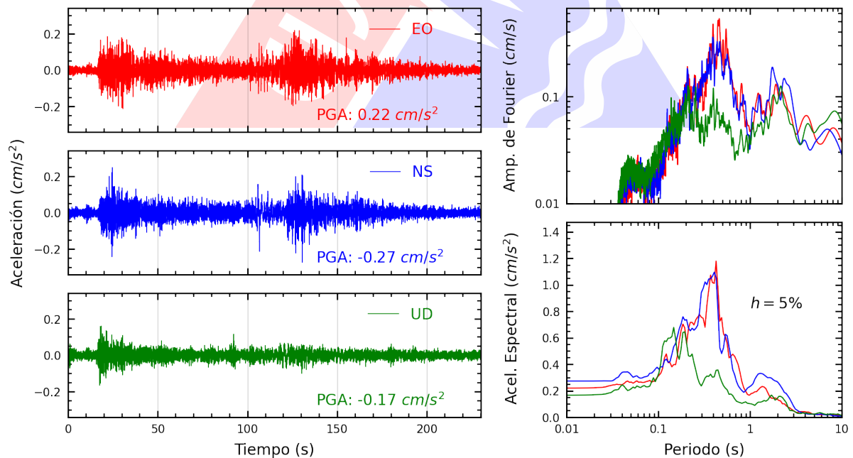
Figura A.14: Registros tiempo-historia, espectros de Fourier y de respuesta en las direcciones EO, NS y vertical de la estación VHAYA. Sismo de Esperanza, Purus - Ucayali del 2024-01-28, 04:38:50 (Hora local)
