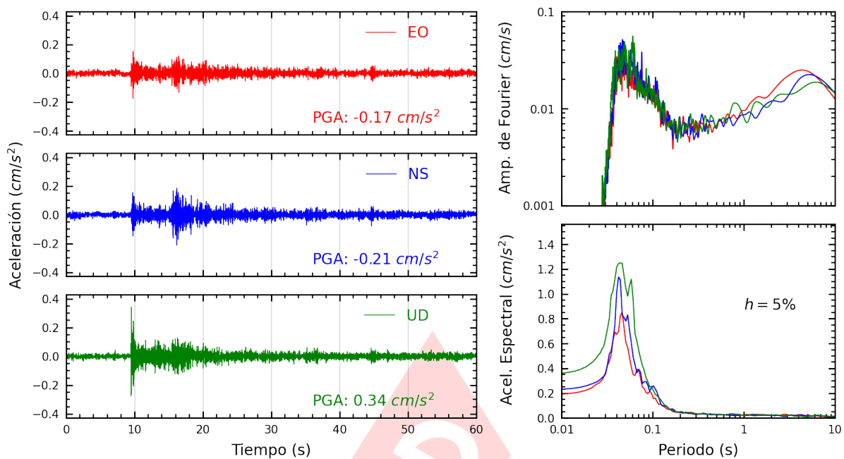
Figura A.11: Registros tiempo-historia, espectros de Fourier y de respuesta en las direcciones EO, NS y vertical de la estación SERVI. Sismo de Provincia Constitucional del Callao , Callao - Lima del 2024-03-06, 09:31:40 (Hora local)
