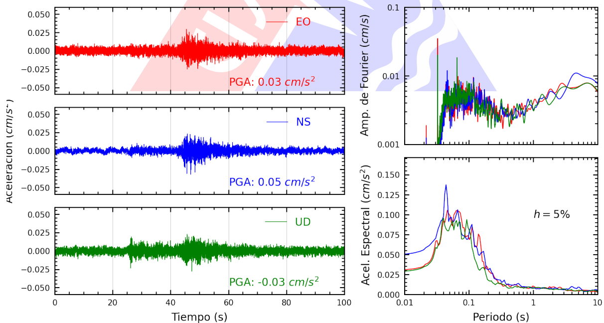
Figura A.24: Registros tiempo-historia, espectros de Fourier y de respuesta en las direcciones EO, NS y vertical de la estación CARAL. Sismo de Provincia Constitucional del Callao , Callao - Lima del 2024-03-06, 09:31:40 (Hora local)
