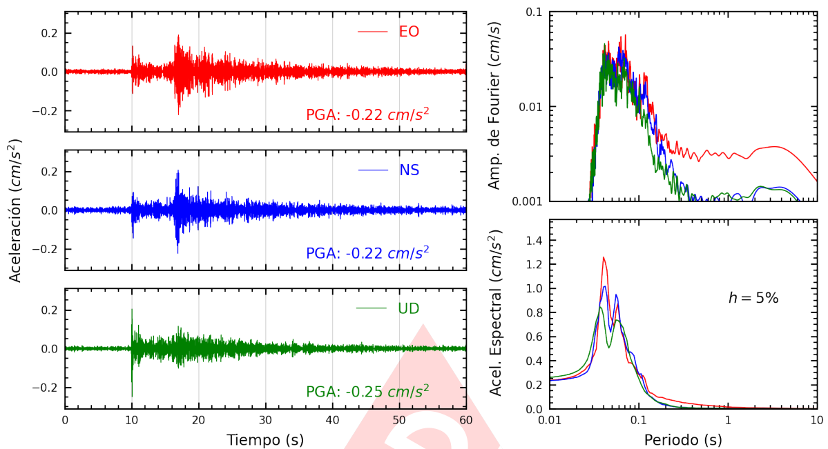
Figura A.17: Registros tiempo-historia, espectros de Fourier y de respuesta en las direcciones EO, NS y vertical de la estación ATARJ. Sismo de Provincia Constitucional del Callao , Callao - Lima del 2024-03-06, 09:31:40 (Hora local)
