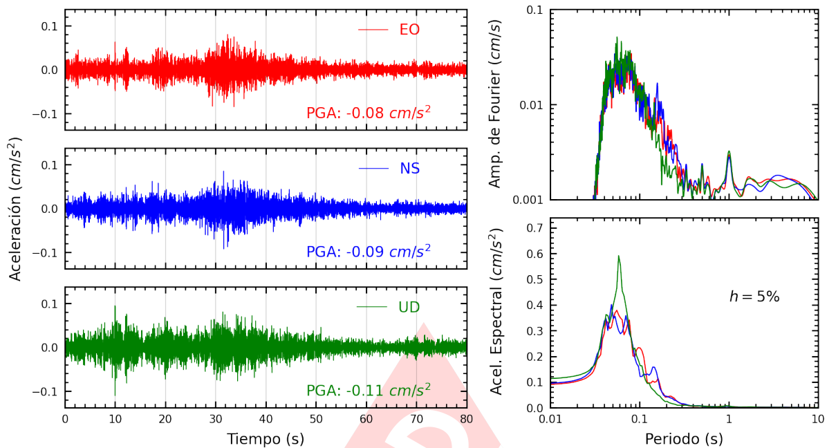
Figura A.23: Registros tiempo-historia, espectros de Fourier y de respuesta en las direcciones EO, NS y vertical de la estación ASIA. Sismo de Provincia Constitucional del Callao , Callao - Lima del 2024-03-06, 09:31:40 (Hora local)
