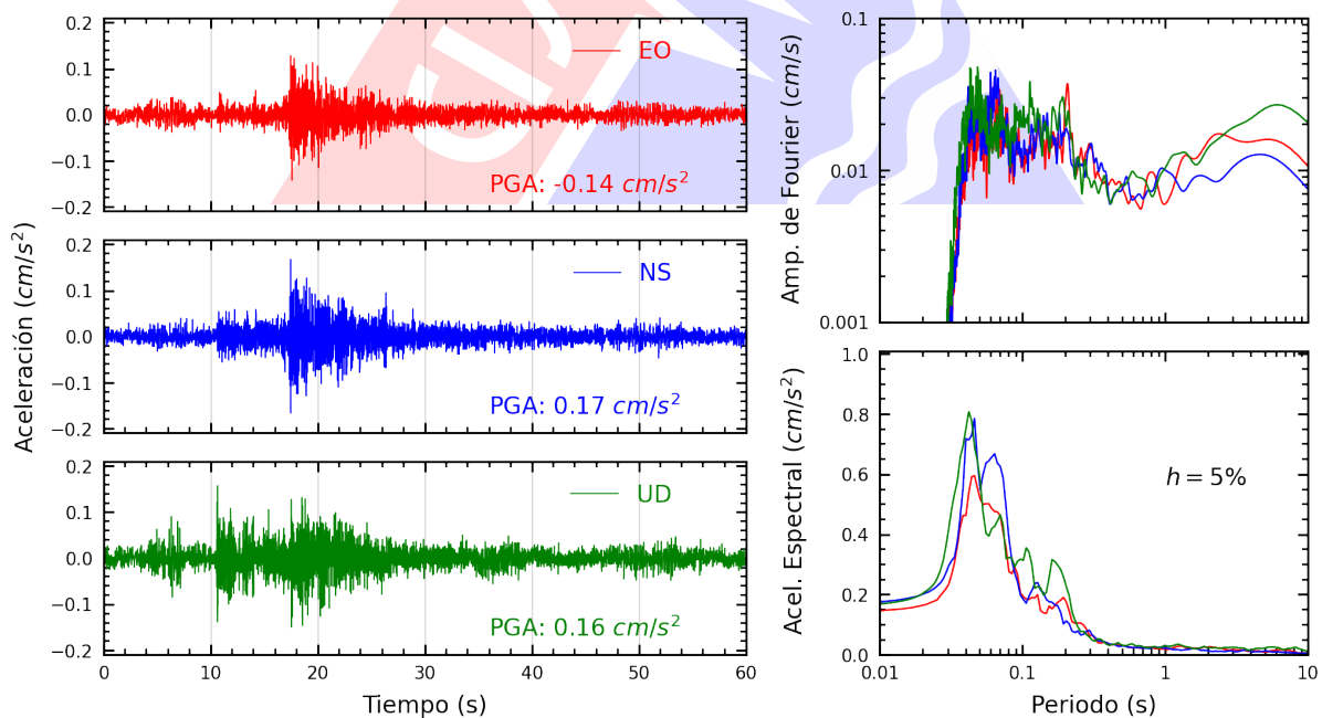
Figura A.22: Registros tiempo-historia, espectros de Fourier y de respuesta en las direcciones EO, NS y vertical de la estación VHAYA. Sismo de Provincia Constitucional del Callao , Callao - Lima del 2024-03-06, 09:31:40 (Hora local)
