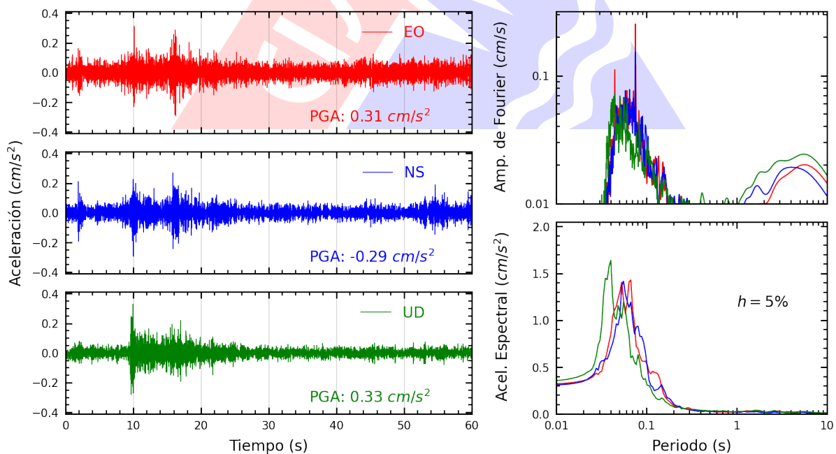
Figura A.12: Registros tiempo-historia, espectros de Fourier y de respuesta en las direcciones EO, NS y vertical de la estación UPCSM. Sismo de Provincia Constitucional del Callao , Callao - Lima del 2024-03-06, 09:31:40 (Hora local)
