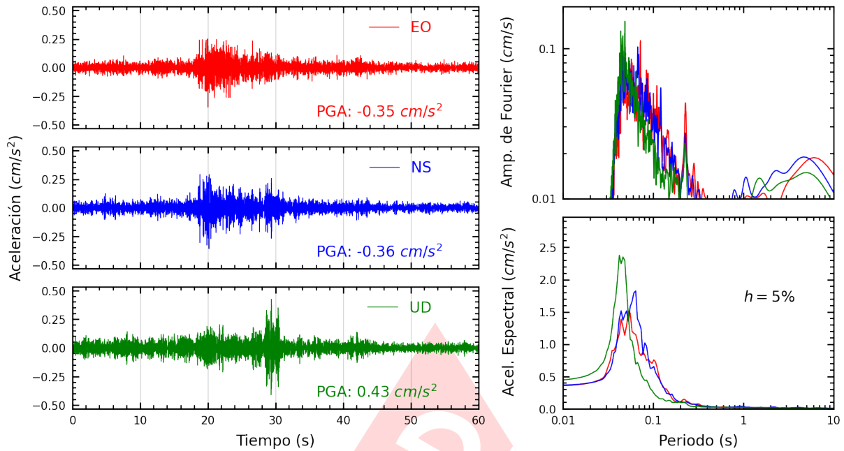
Figura A.9: Registros tiempo-historia, espectros de Fourier y de respuesta en las direcciones EO, NS y vertical de la estación DEFEN. Sismo de Provincia Constitucional del Callao , Callao - Lima del 2024-03-06, 09:31:40 (Hora local)
