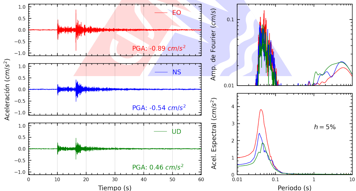
Figura A.2: Registros tiempo-historia, espectros de Fourier y de respuesta en las direcciones EO, NS y vertical de la estación UCSS. Sismo de Provincia Constitucional del Callao , Callao - Lima del 2024-03-06, 09:31:40 (Hora local)
