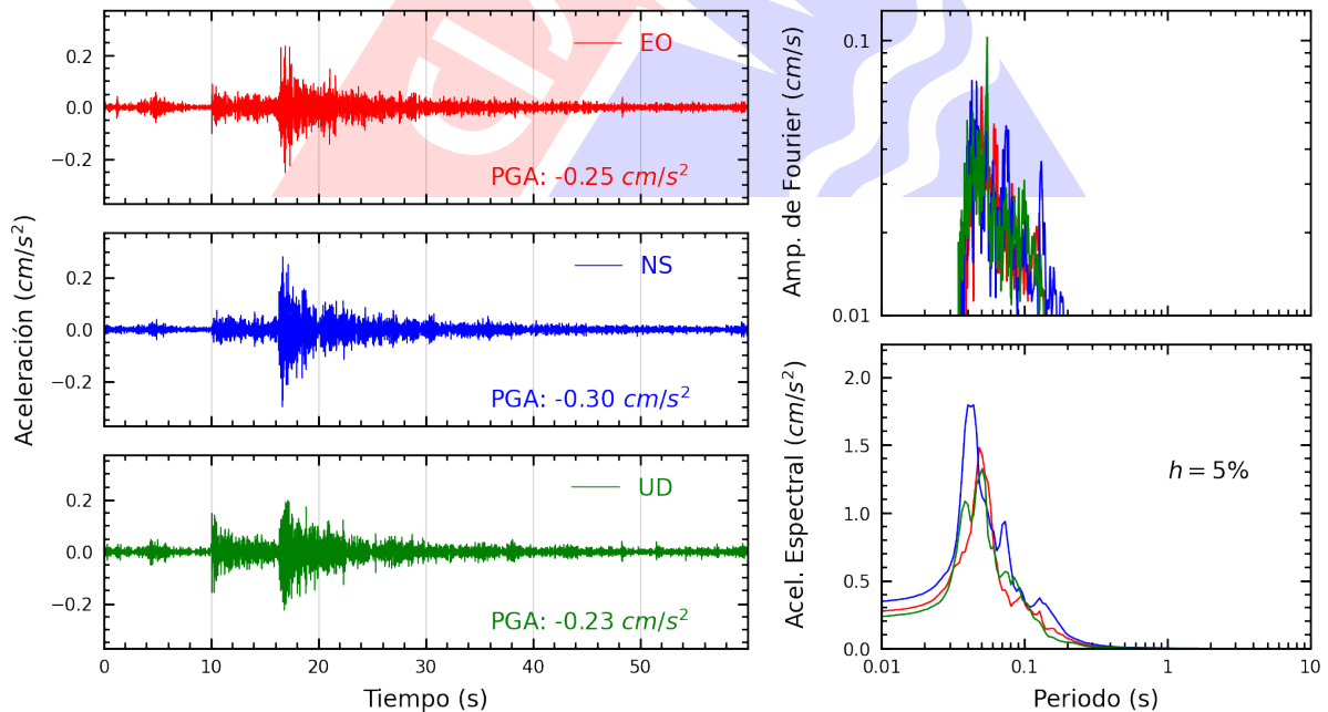
Figura A.14: Registros tiempo-historia, espectros de Fourier y de respuesta en las direcciones EO, NS y vertical de la estación JALV2. Sismo de Provincia Constitucional del Callao , Callao - Lima del 2024-03-06, 09:31:40 (Hora local)
