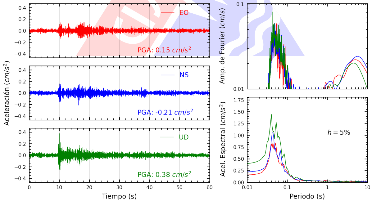
Figura A.10: Registros tiempo-historia, espectros de Fourier y de respuesta en las direcciones EO, NS y vertical de la estación CENEP. Sismo de Provincia Constitucional del Callao , Callao - Lima del 2024-03-06, 09:31:40 (Hora local)
