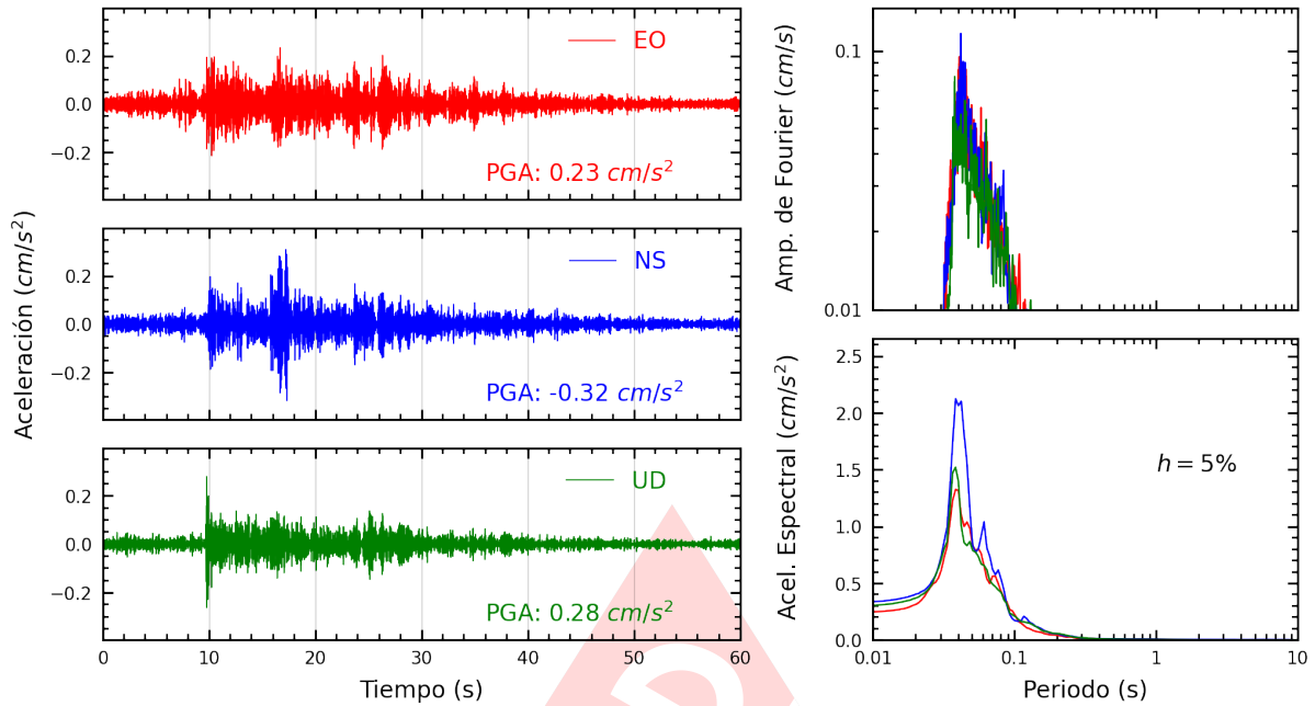
Figura A.13: Registros tiempo-historia, espectros de Fourier y de respuesta en las direcciones EO, NS y vertical de la estación BORJA. Sismo de Provincia Constitucional del Callao , Callao - Lima del 2024-03-06, 09:31:40 (Hora local)
