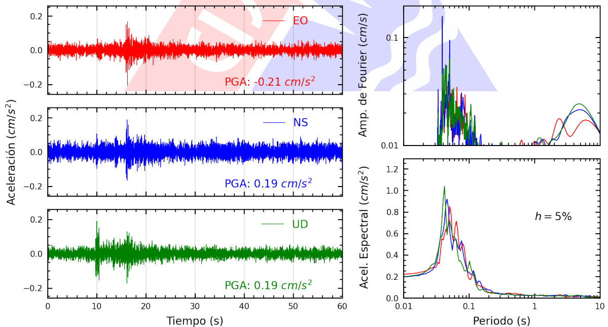
Figura A.20: Registros tiempo-historia, espectros de Fourier y de respuesta en las direcciones EO, NS y vertical de la estación BONDY. Sismo de Provincia Constitucional del Callao , Callao - Lima del 2024-03-06, 09:31:40 (Hora local)
