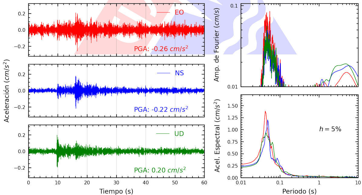
Figura A.16: Registros tiempo-historia, espectros de Fourier y de respuesta en las direcciones EO, NS y vertical de la estación INICT. Sismo de Provincia Constitucional del Callao , Callao - Lima del 2024-03-06, 09:31:40 (Hora local)
