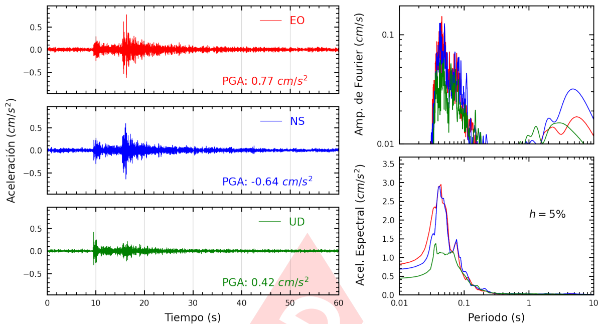
Figura A.5: Registros tiempo-historia, espectros de Fourier y de respuesta en las direcciones EO, NS y vertical de la estación CEPRE. Sismo de Provincia Constitucional del Callao , Callao - Lima del 2024-03-06, 09:31:40 (Hora local)
