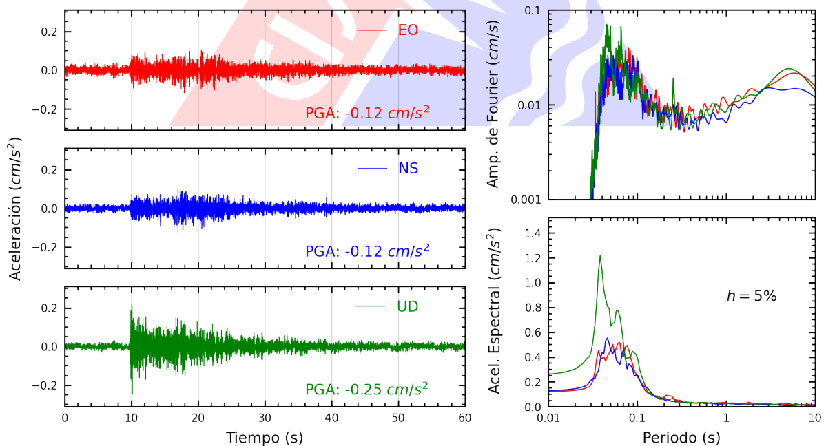
Figura A.18: Registros tiempo-historia, espectros de Fourier y de respuesta en las direcciones EO, NS y vertical de la estación USILP. Sismo de Provincia Constitucional del Callao , Callao - Lima del 2024-03-06, 09:31:40 (Hora local)
