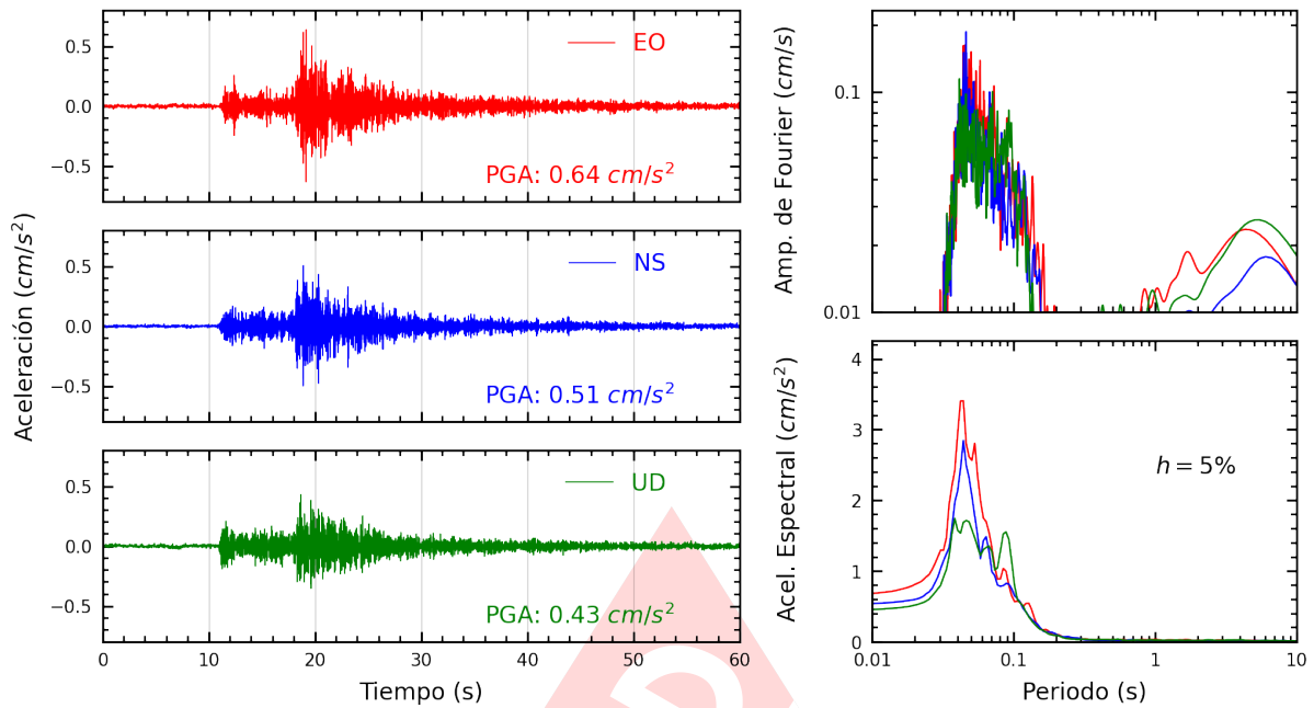
Figura A.7: Registros tiempo-historia, espectros de Fourier y de respuesta en las direcciones EO, NS y vertical de la estación AMORE. Sismo de Provincia Constitucional del Callao , Callao - Lima del 2024-03-06, 09:31:40 (Hora local)
