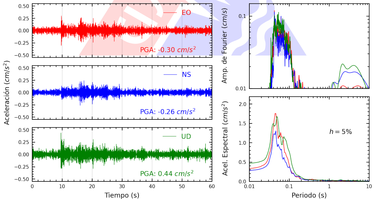
Figura A.8: Registros tiempo-historia, espectros de Fourier y de respuesta en las direcciones EO, NS y vertical de la estación URPPPE. Sismo de Provincia Constitucional del Callao , Callao - Lima del 2024-03-06, 09:31:40 (Hora local)
