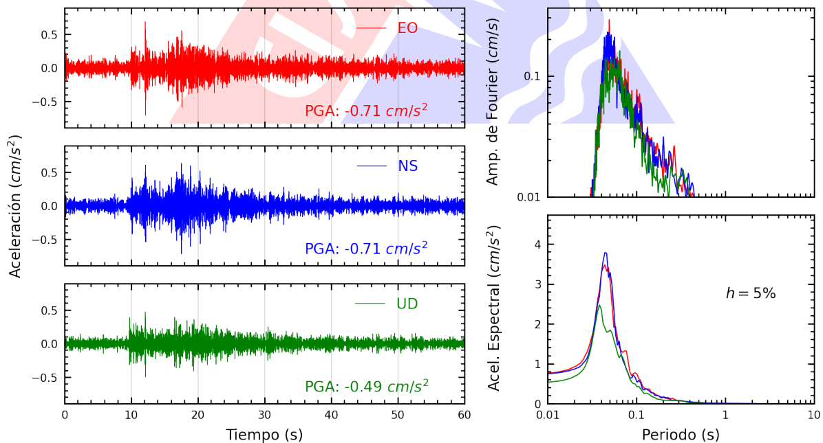
Figura A.6: Registros tiempo-historia, espectros de Fourier y de respuesta en las direcciones EO, NS y vertical de la estación UNTEL. Sismo de Provincia Constitucional del Callao , Callao - Lima del 2024-03-06, 09:31:40 (Hora local)
