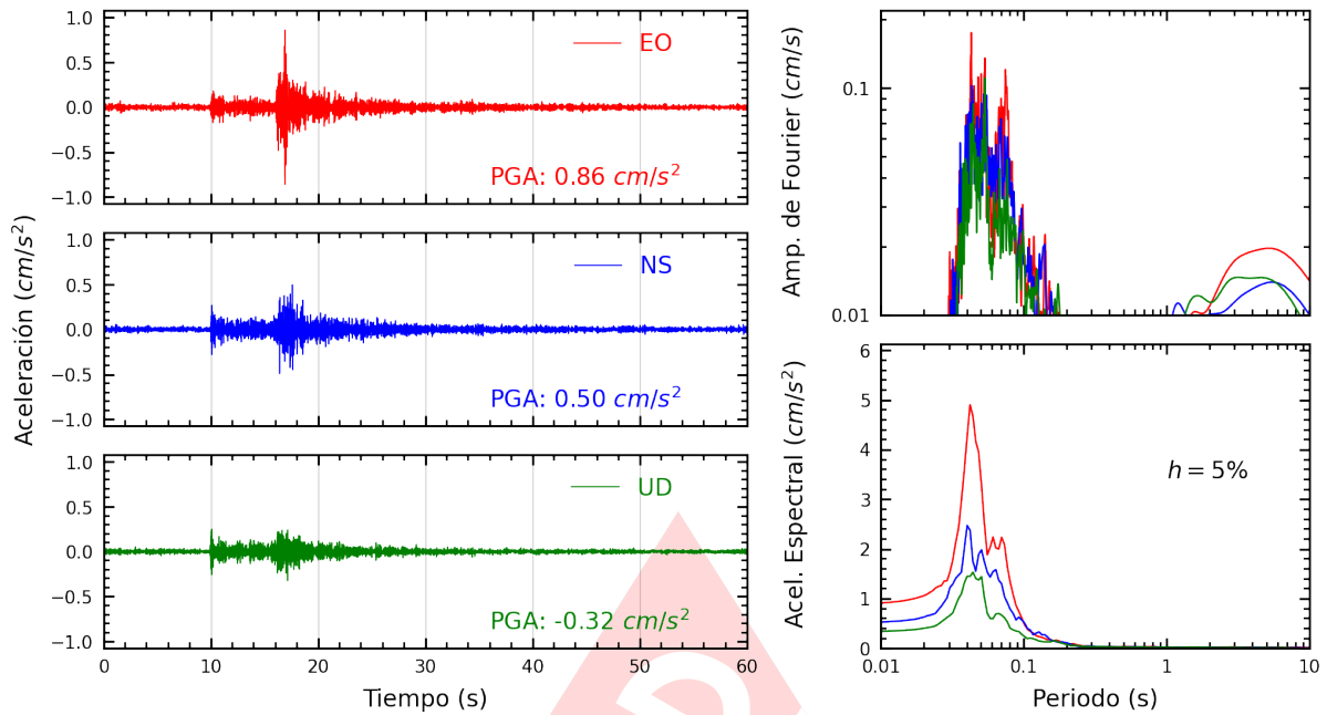
Figura A.3: Registros tiempo-historia, espectros de Fourier y de respuesta en las direcciones EO, NS y vertical de la estación FICPE. Sismo de Provincia Constitucional del Callao , Callao - Lima del 2024-03-06, 09:31:40 (Hora local)
