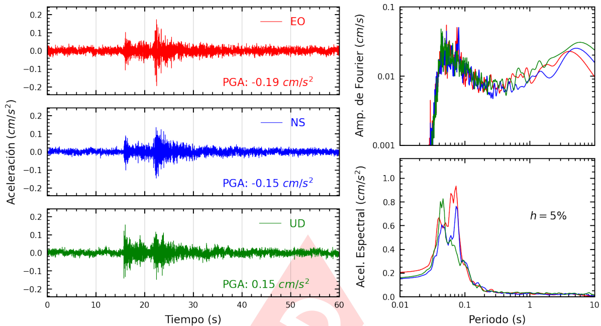
Figura A.21: Registros tiempo-historia, espectros de Fourier y de respuesta en las direcciones EO, NS y vertical de la estación UNMSM. Sismo de Provincia Constitucional del Callao , Callao - Lima del 2024-03-06, 09:31:40 (Hora local)
