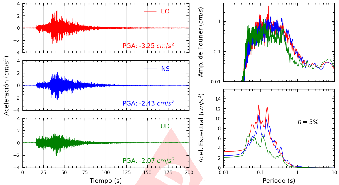
Figura A.13: Registros tiempo-historia, espectros de Fourier y de respuesta en las direcciones EO, NS y vertical de la estación USILP. Sismo de Pisco, Pisco - Ica del 2024-03-07, 11:31:59 (Hora local)
