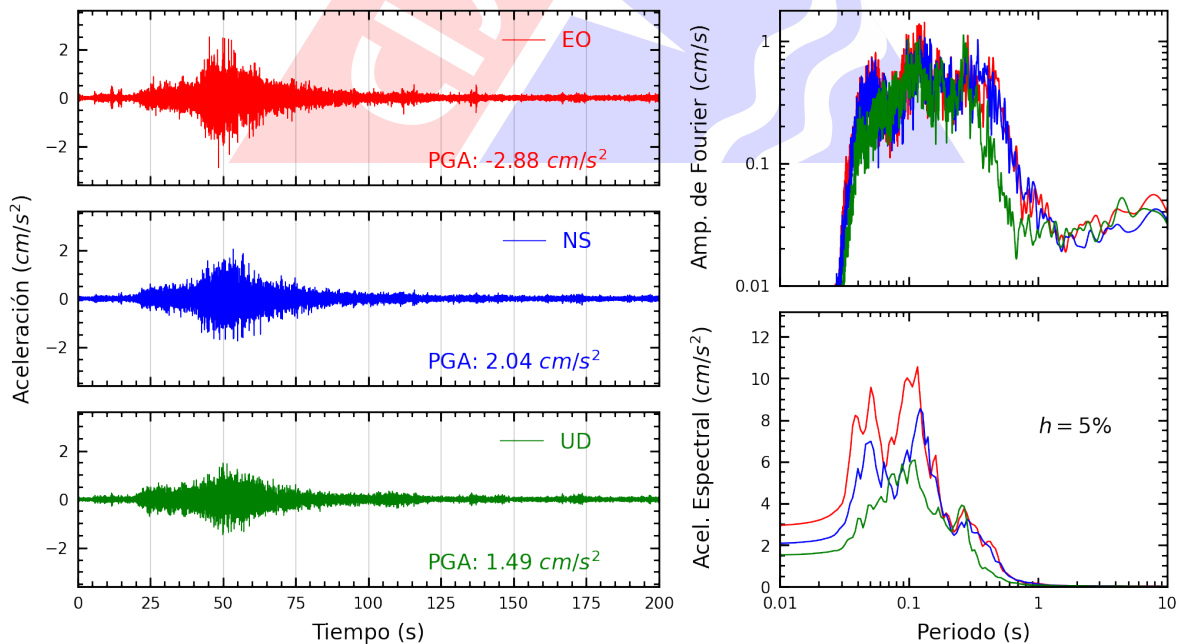
Figura A.16: Registros tiempo-historia, espectros de Fourier y de respuesta en las direcciones EO, NS y vertical de la estación OLIVO. Sismo de Pisco, Pisco - Ica del 2024-03-07, 11:31:59 (Hora local)
