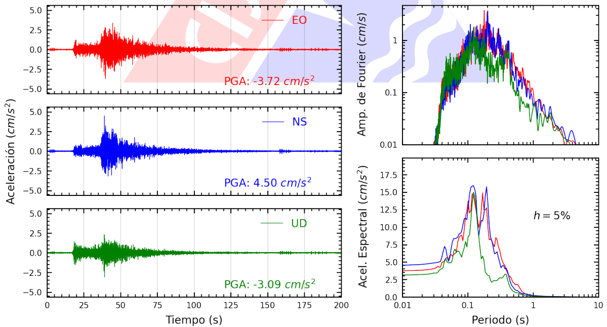
Figura A.8: Registros tiempo-historia, espectros de Fourier y de respuesta en las direcciones EO, NS y vertical de la estación SCCHO. Sismo de Pisco, Pisco - Ica del 2024-03-07, 11:31:59 (Hora local)
