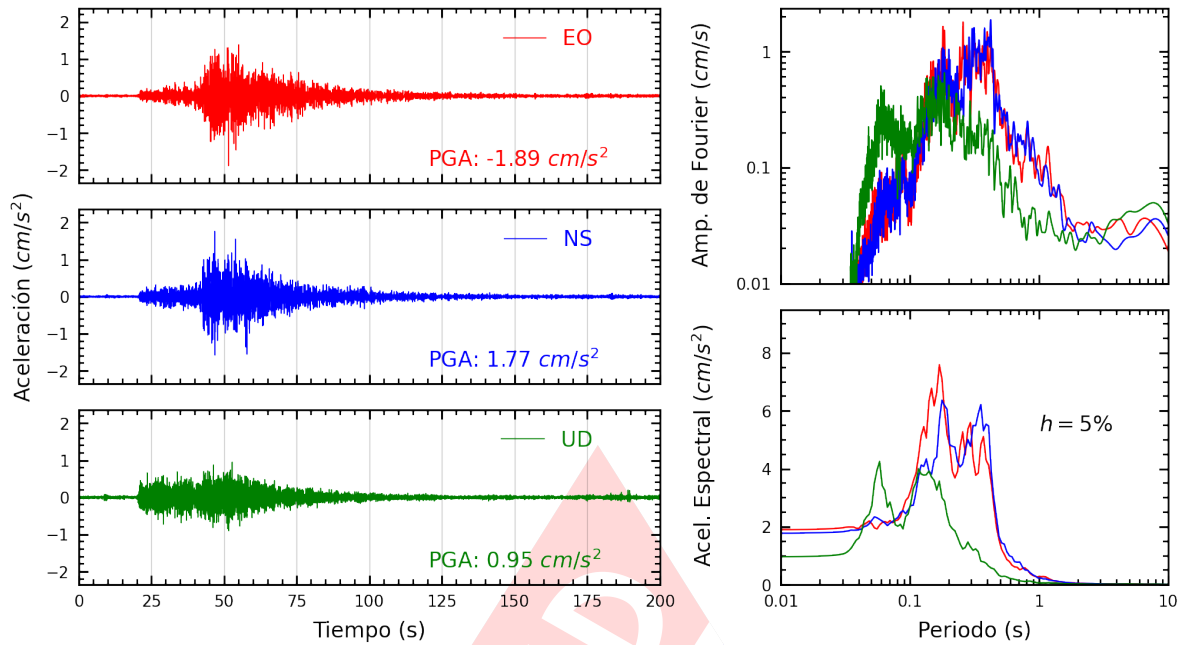
Figura A.21: Registros tiempo-historia, espectros de Fourier y de respuesta en las direcciones EO, NS y vertical de la estación ACAPU. Sismo de Pisco, Pisco - Ica del 2024-03-07, 11:31:59 (Hora local)
