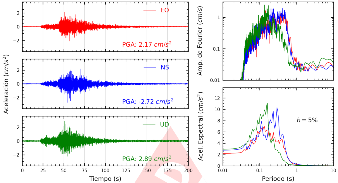
Figura A.15: Registros tiempo-historia, espectros de Fourier y de respuesta en las direcciones EO, NS y vertical de la estación MDPP. Sismo de Pisco, Pisco - Ica del 2024-03-07, 11:31:59 (Hora local)
