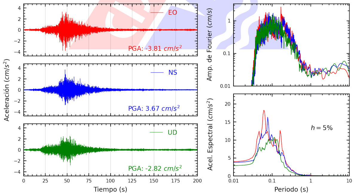
Figura A.12: Registros tiempo-historia, espectros de Fourier y de respuesta en las direcciones EO, NS y vertical de la estación INDEP. Sismo de Pisco, Pisco - Ica del 2024-03-07, 11:31:59 (Hora local)
