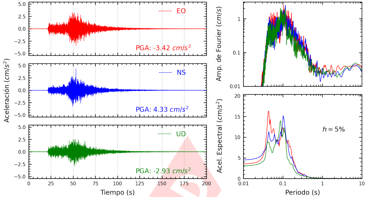
Figura A.9: Registros tiempo-historia, espectros de Fourier y de respuesta en las direcciones EO, NS y vertical de la estación AMORE. Sismo de Pisco, Pisco - Ica del 2024-03-07, 11:31:59 (Hora local)
