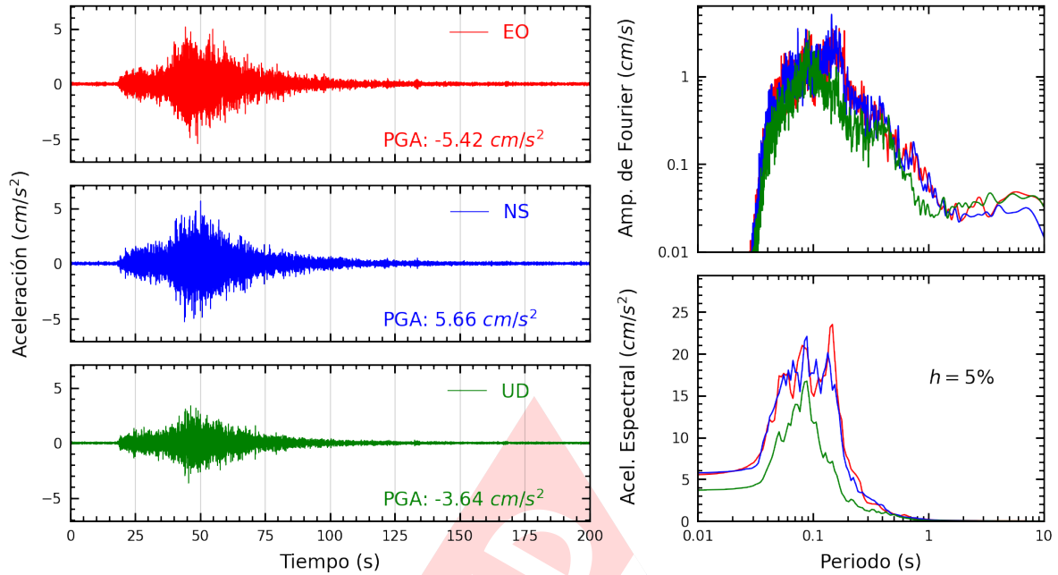
Figura A.5: Registros tiempo-historia, espectros de Fourier y de respuesta en las direcciones EO, NS y vertical de la estación USILM. Sismo de Pisco, Pisco - Ica del 2024-03-07, 11:31:59 (Hora local)
