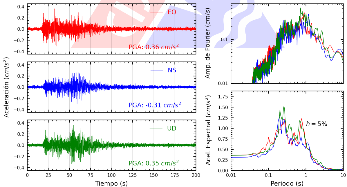
Figura A.42: Registros tiempo-historia, espectros de Fourier y de respuesta en las direcciones EO, NS y vertical de la estación UNSCH. Sismo de Pisco, Pisco - Ica del 2024-03-07, 11:31:59 (Hora local)
