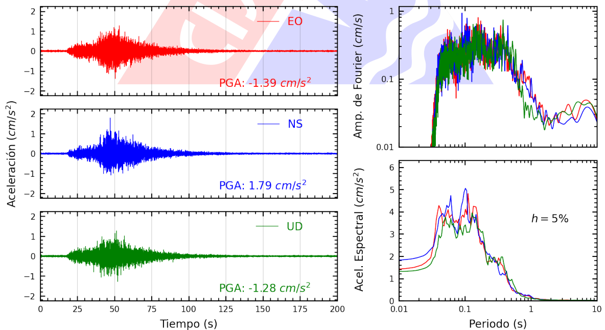
Figura A.22: Registros tiempo-historia, espectros de Fourier y de respuesta en las direcciones EO, NS y vertical de la estación IMCA. Sismo de Pisco, Pisco - Ica del 2024-03-07, 11:31:59 (Hora local)
