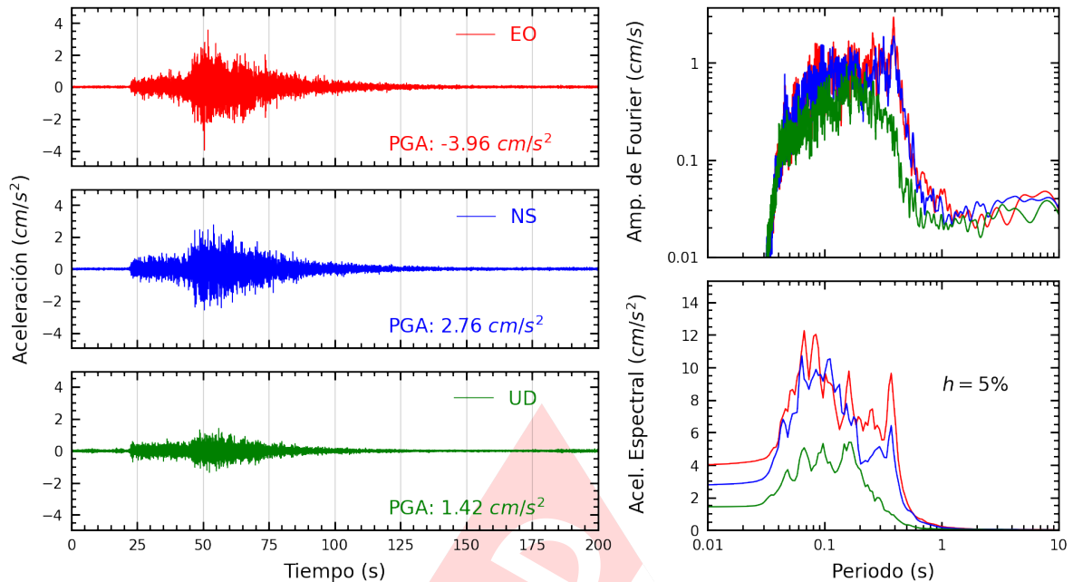
Figura A.11: Registros tiempo-historia, espectros de Fourier y de respuesta en las direcciones EO, NS y vertical de la estación DEFEN. Sismo de Pisco, Pisco - Ica del 2024-03-07, 11:31:59 (Hora local)
