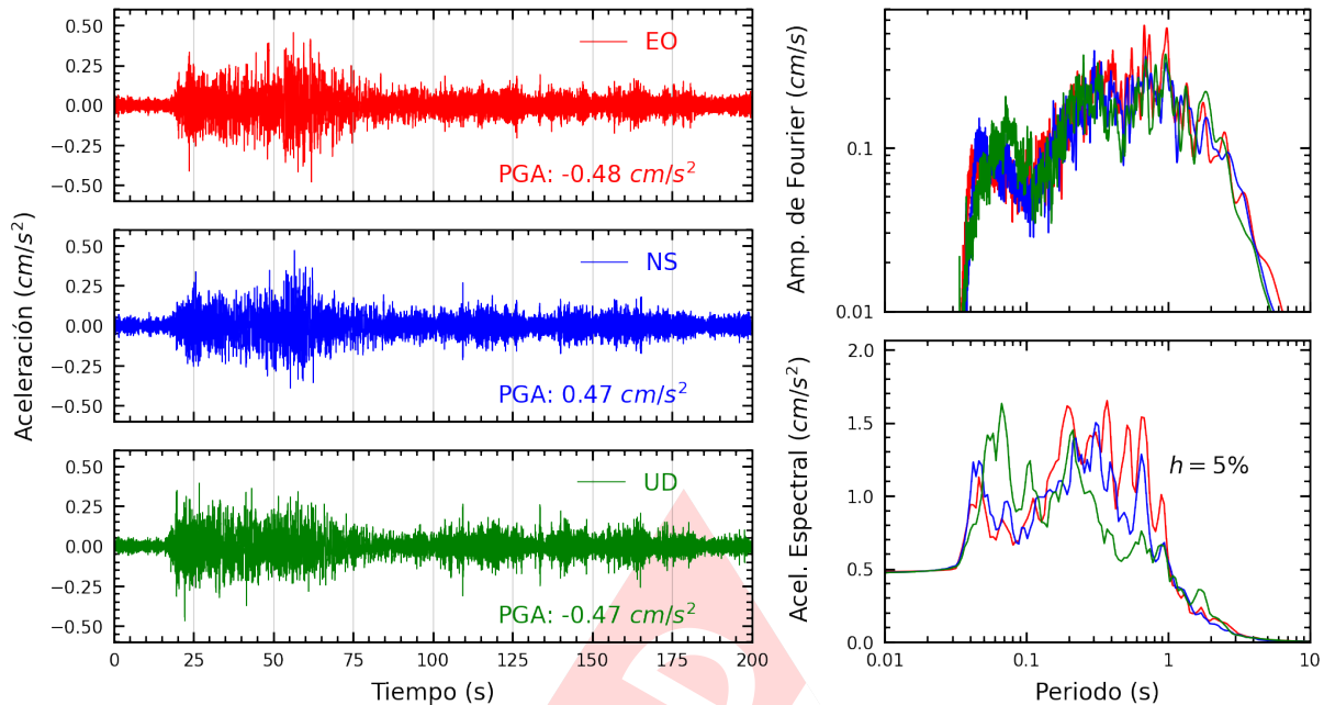
Figura A.41: Registros tiempo-historia, espectros de Fourier y de respuesta en las direcciones EO, NS y vertical de la estación SCAYA. Sismo de Pisco, Pisco - Ica del 2024-03-07, 11:31:59 (Hora local)
