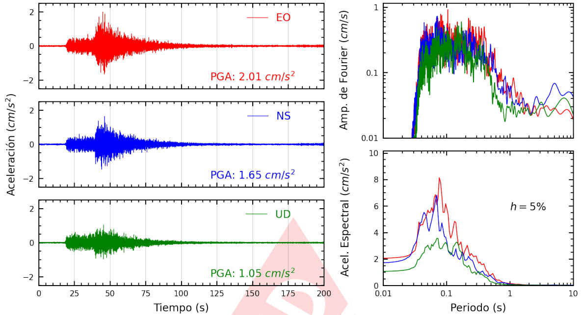
Figura A.19: Registros tiempo-historia, espectros de Fourier y de respuesta en las direcciones EO, NS y vertical de la estación CEPRE. Sismo de Pisco, Pisco - Ica del 2024-03-07, 11:31:59 (Hora local)
