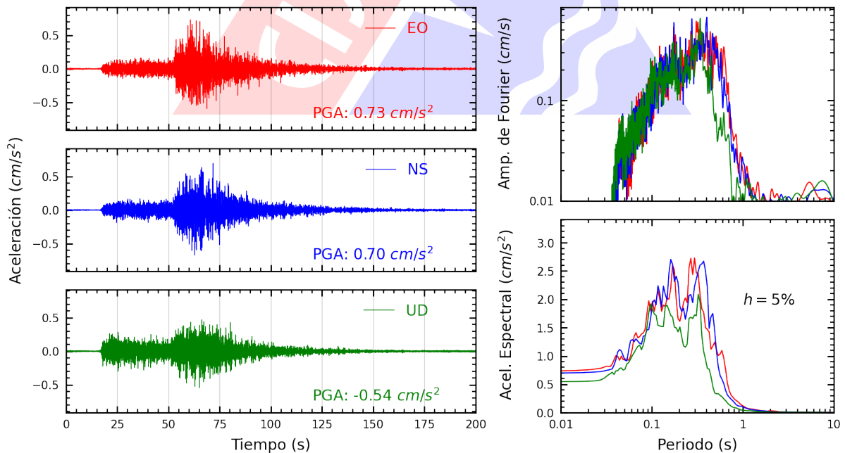
Figura A.40: Registros tiempo-historia, espectros de Fourier y de respuesta en las direcciones EO, NS y vertical de la estación CARAL. Sismo de Pisco, Pisco - Ica del 2024-03-07, 11:31:59 (Hora local)
