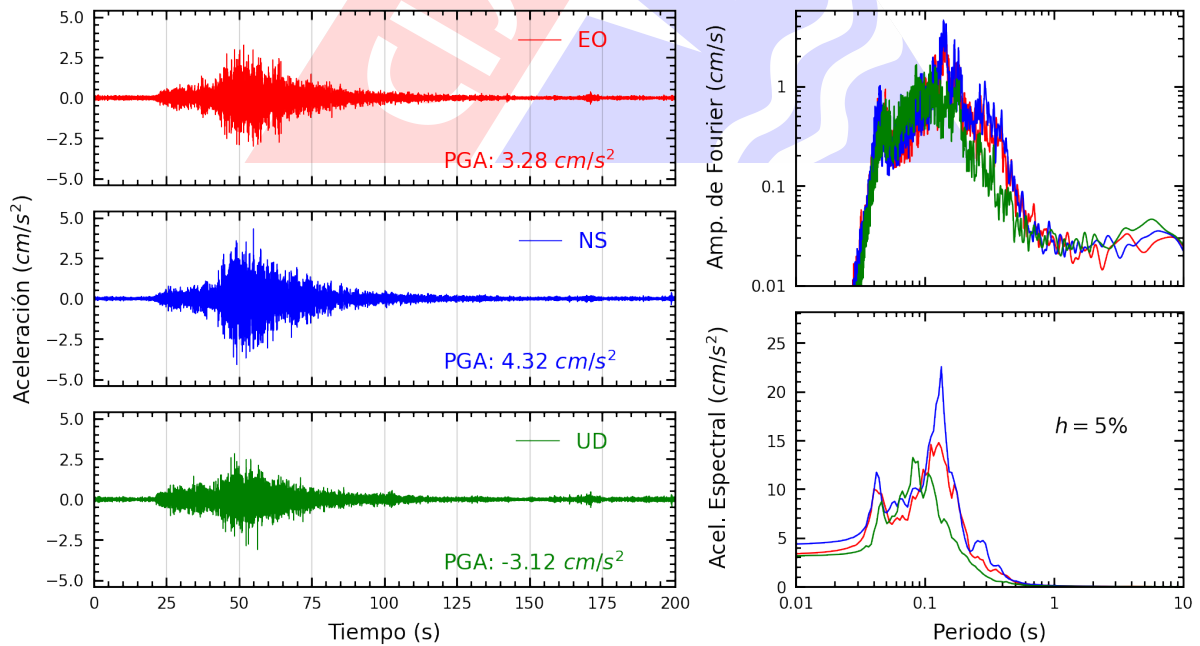
Figura A.10: Registros tiempo-historia, espectros de Fourier y de respuesta en las direcciones EO, NS y vertical de la estación CARAB. Sismo de Pisco, Pisco - Ica del 2024-03-07, 11:31:59 (Hora local)
