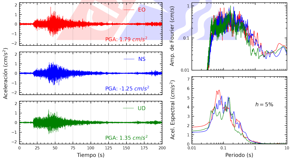
Figura A.24: Registros tiempo-historia, espectros de Fourier y de respuesta en las direcciones EO, NS y vertical de la estación UPCSM. Sismo de Pisco, Pisco - Ica del 2024-03-07, 11:31:59 (Hora local)
