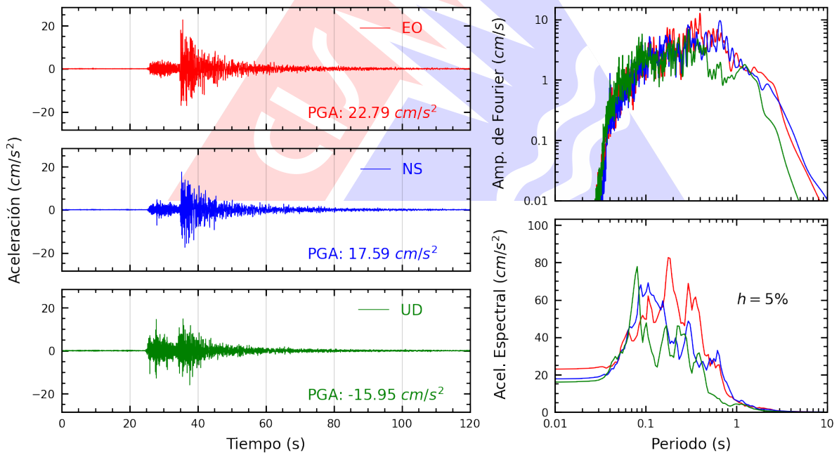
Figura A.2: Registros tiempo-historia, espectros de Fourier y de respuesta en las direcciones EO, NS y vertical de la estación SCICA. Sismo de Pisco, Pisco - Ica del 2024-03-07, 11:31:59 (Hora local)
