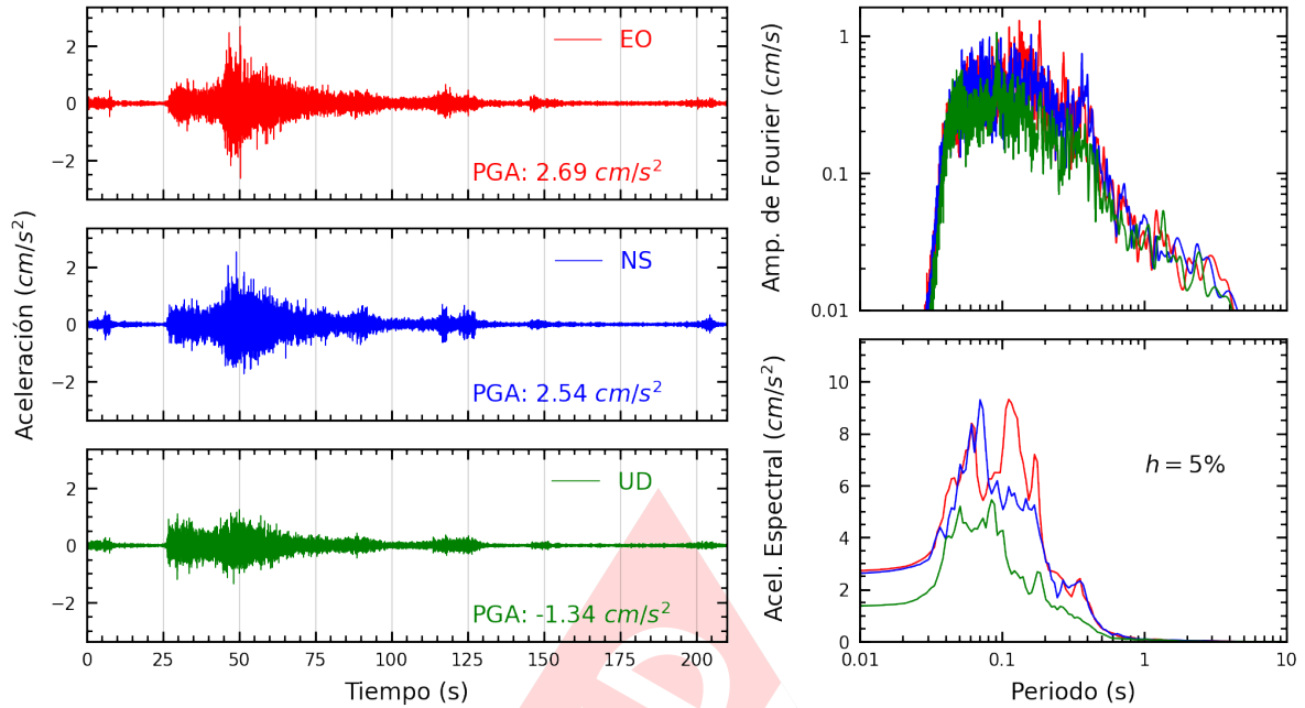
Figura A.17: Registros tiempo-historia, espectros de Fourier y de respuesta en las direcciones EO, NS y vertical de la estación PACHA. Sismo de Pisco, Pisco - Ica del 2024-03-07, 11:31:59 (Hora local)
