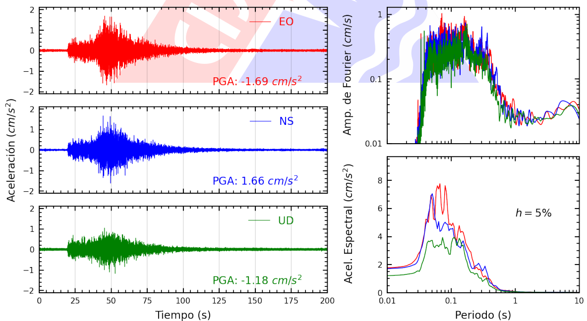
Figura A.26: Registros tiempo-historia, espectros de Fourier y de respuesta en las direcciones EO, NS y vertical de la estación FICPE. Sismo de Pisco, Pisco - Ica del 2024-03-07, 11:31:59 (Hora local)
