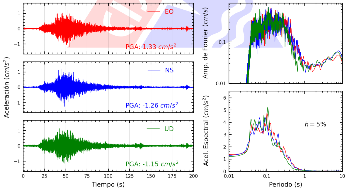
Figura A.30: Registros tiempo-historia, espectros de Fourier y de respuesta en las direcciones EO, NS y vertical de la estación USMP. Sismo de Pisco, Pisco - Ica del 2024-03-07, 11:31:59 (Hora local)
