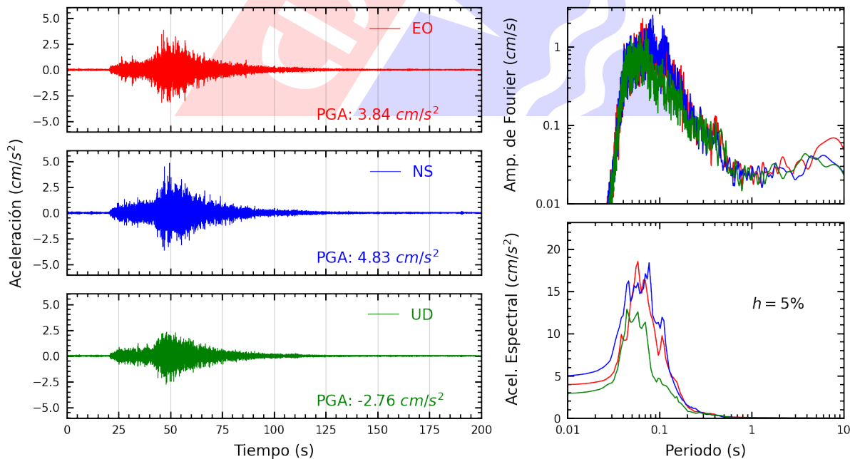
Figura A.6: Registros tiempo-historia, espectros de Fourier y de respuesta en las direcciones EO, NS y vertical de la estación JOSEO. Sismo de Pisco, Pisco - Ica del 2024-03-07, 11:31:59 (Hora local)
