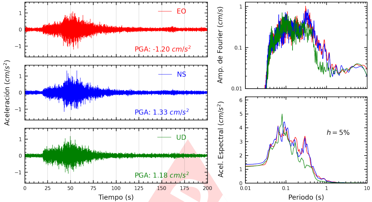
Figura A.31: Registros tiempo-historia, espectros de Fourier y de respuesta en las direcciones EO, NS y vertical de la estación MADRE. Sismo de Pisco, Pisco - Ica del 2024-03-07, 11:31:59 (Hora local)
