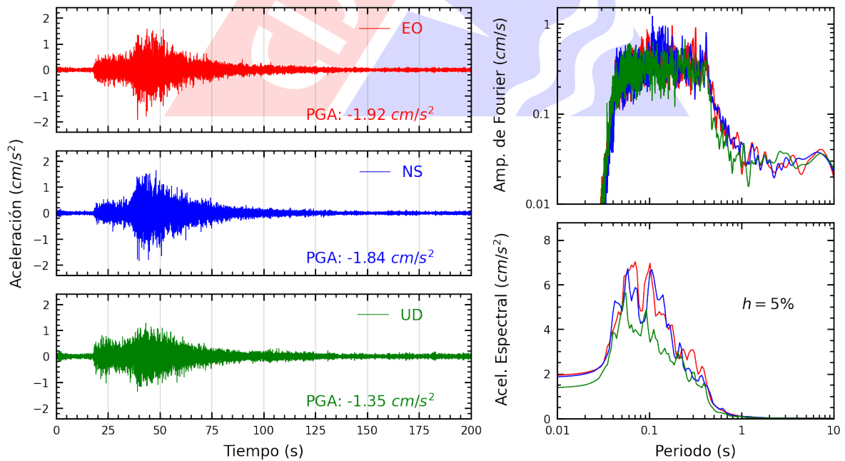
Figura A.20: Registros tiempo-historia, espectros de Fourier y de respuesta en las direcciones EO, NS y vertical de la estación URPPE. Sismo de Pisco, Pisco - Ica del 2024-03-07, 11:31:59 (Hora local)
