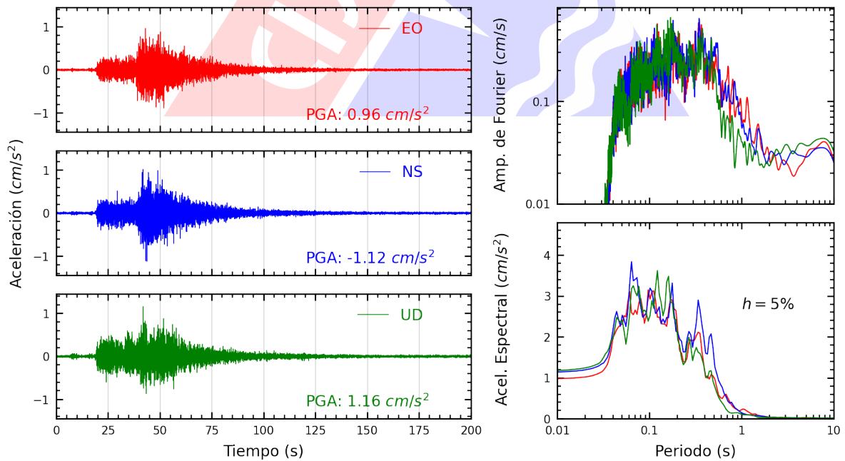
Figura A.34: Registros tiempo-historia, espectros de Fourier y de respuesta en las direcciones EO, NS y vertical de la estación UNFV. Sismo de Pisco, Pisco - Ica del 2024-03-07, 11:31:59 (Hora local)
