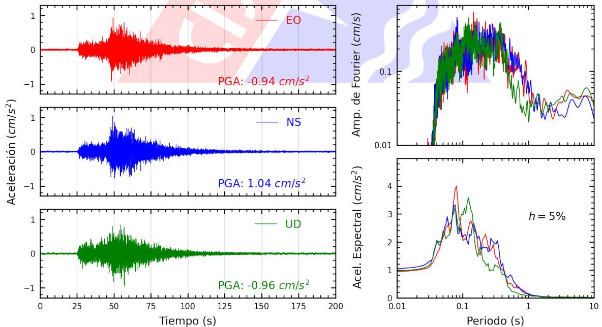
Figura A.38: Registros tiempo-historia, espectros de Fourier y de respuesta en las direcciones EO, NS y vertical de la estación UNMSM. Sismo de Pisco, Pisco - Ica del 2024-03-07, 11:31:59 (Hora local)
