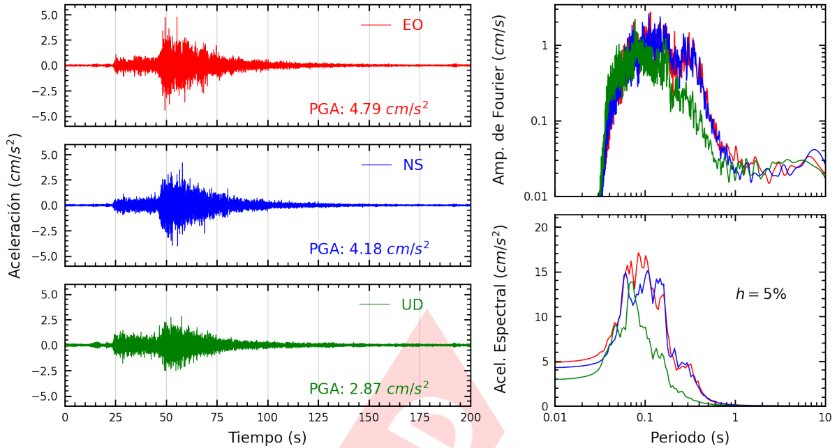
Figura A.7: Registros tiempo-historia, espectros de Fourier y de respuesta en las direcciones EO, NS y vertical de la estación ANCON. Sismo de Pisco, Pisco - Ica del 2024-03-07, 11:31:59 (Hora local)
