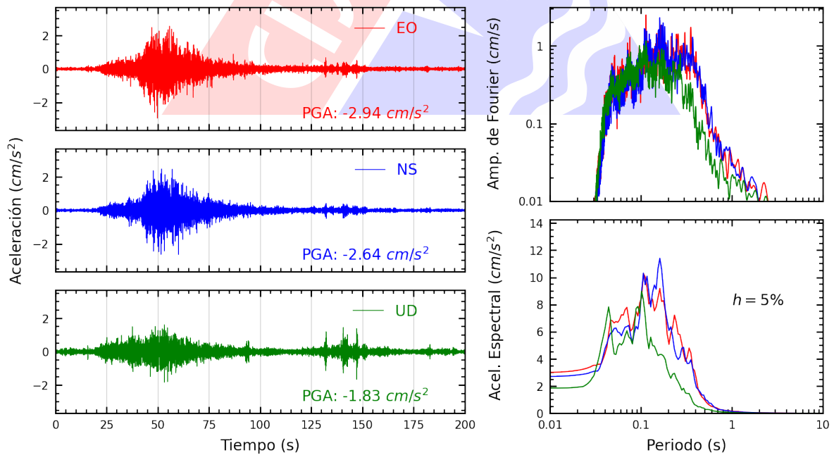
Figura A.14: Registros tiempo-historia, espectros de Fourier y de respuesta en las direcciones EO, NS y vertical de la estación SCOLI. Sismo de Pisco, Pisco - Ica del 2024-03-07, 11:31:59 (Hora local)
