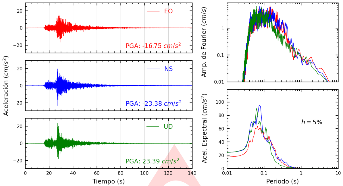
Figura A.1: Registros tiempo-historia, espectros de Fourier y de respuesta en las direcciones EO, NS y vertical de la estación ASIA. Sismo de Pisco, Pisco - Ica del 2024-03-07, 11:31:59 (Hora local)
