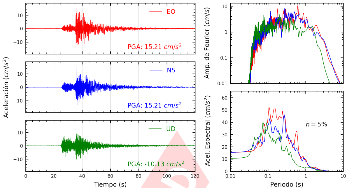
Figura A.3: Registros tiempo-historia, espectros de Fourier y de respuesta en las direcciones EO, NS y vertical de la estación UNICA. Sismo de Pisco, Pisco - Ica del 2024-03-07, 11:31:59 (Hora local)
