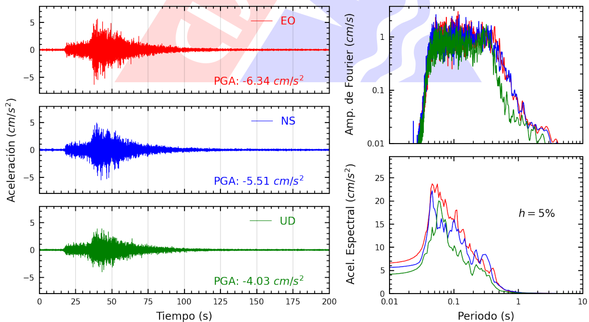
Figura A.4: Registros tiempo-historia, espectros de Fourier y de respuesta en las direcciones EO, NS y vertical de la estación UNTEL. Sismo de Pisco, Pisco - Ica del 2024-03-07, 11:31:59 (Hora local)
