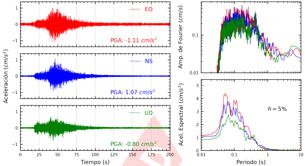
Figura A.37: Registros tiempo-historia, espectros de Fourier y de respuesta en las direcciones EO, NS y vertical de la estación INICT. Sismo de Pisco, Pisco - Ica del 2024-03-07, 11:31:59 (Hora local)
