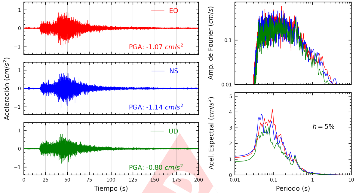
Figura A.35: Registros tiempo-historia, espectros de Fourier y de respuesta en las direcciones EO, NS y vertical de la estación BORJA. Sismo de Pisco, Pisco - Ica del 2024-03-07, 11:31:59 (Hora local)
