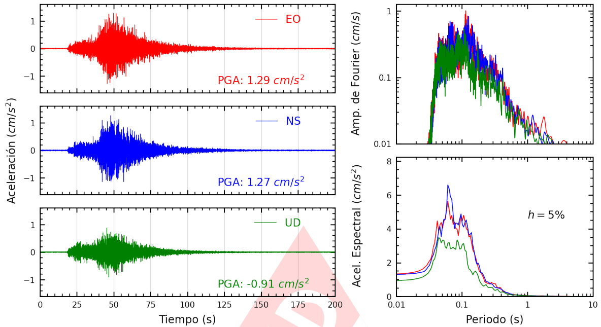
Figura A.33: Registros tiempo-historia, espectros de Fourier y de respuesta en las direcciones EO, NS y vertical de la estación ATARJ. Sismo de Pisco, Pisco - Ica del 2024-03-07, 11:31:59 (Hora local)
