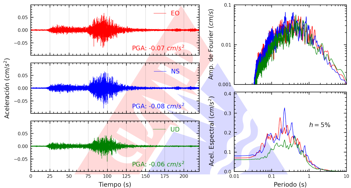
Figura A.45: Registros tiempo-historia, espectros de Fourier y de respuesta en las direcciones EO, NS y vertical de la estación UNSA. Sismo de Pisco, Pisco - Ica del 2024-03-07, 11:31:59 (Hora local)
