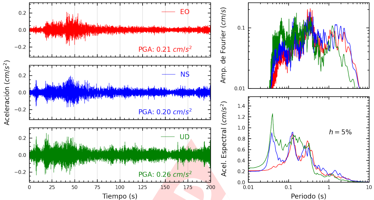
Figura A.43: Registros tiempo-historia, espectros de Fourier y de respuesta en las direcciones EO, NS y vertical de la estación SCHYO. Sismo de Pisco, Pisco - Ica del 2024-03-07, 11:31:59 (Hora local)
