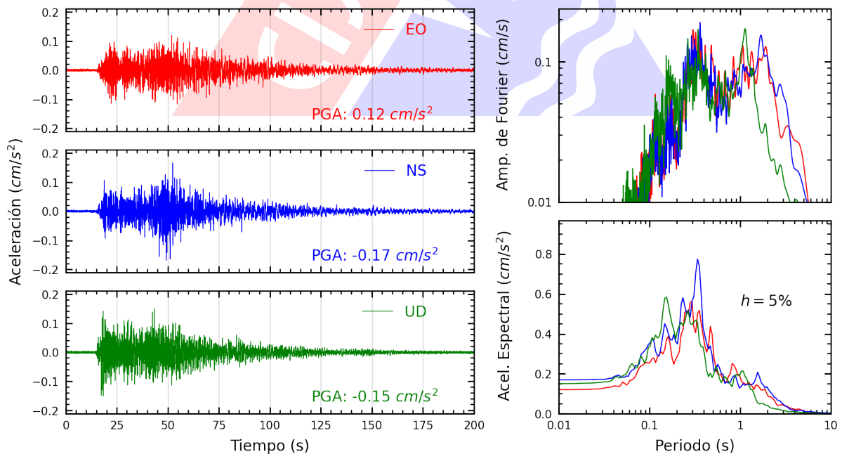
Figura A.44: Registros tiempo-historia, espectros de Fourier y de respuesta en las direcciones EO, NS y vertical de la estación UNCP. Sismo de Pisco, Pisco - Ica del 2024-03-07, 11:31:59 (Hora local)
