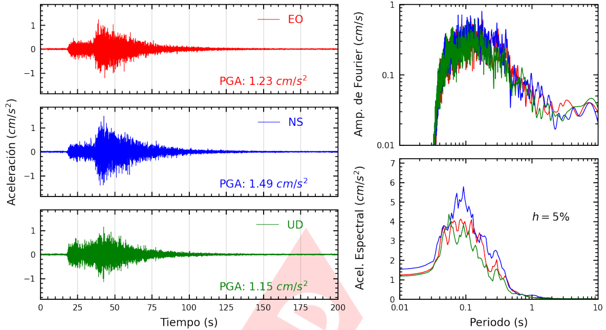
Figura A.27: Registros tiempo-historia, espectros de Fourier y de respuesta en las direcciones EO, NS y vertical de la estación SERVI. Sismo de Pisco, Pisco - Ica del 2024-03-07, 11:31:59 (Hora local)
