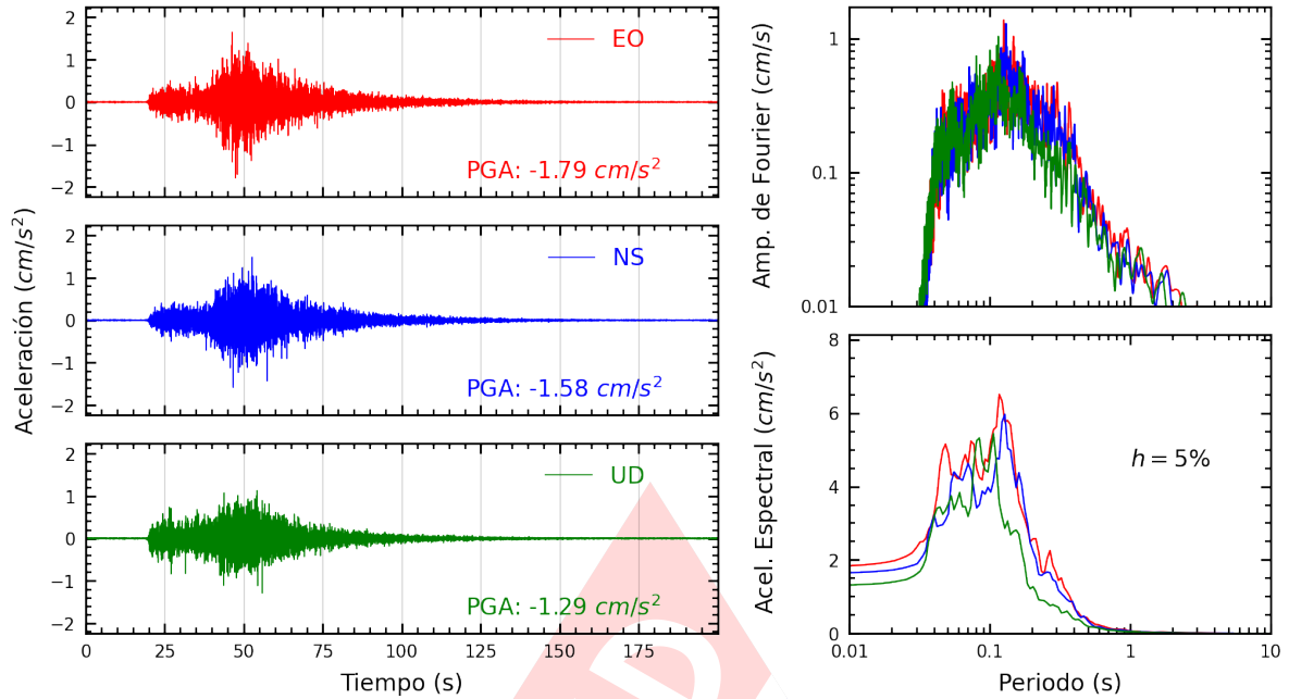
Figura A.23: Registros tiempo-historia, espectros de Fourier y de respuesta en las direcciones EO, NS y vertical de la estación JALV2. Sismo de Pisco, Pisco - Ica del 2024-03-07, 11:31:59 (Hora local)
