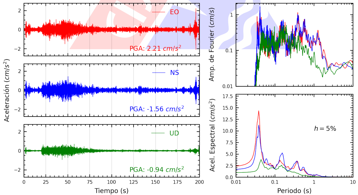
Figura A.18: Registros tiempo-historia, espectros de Fourier y de respuesta en las direcciones EO, NS y vertical de la estación DHNPE. Sismo de Pisco, Pisco - Ica del 2024-03-07, 11:31:59 (Hora local)
