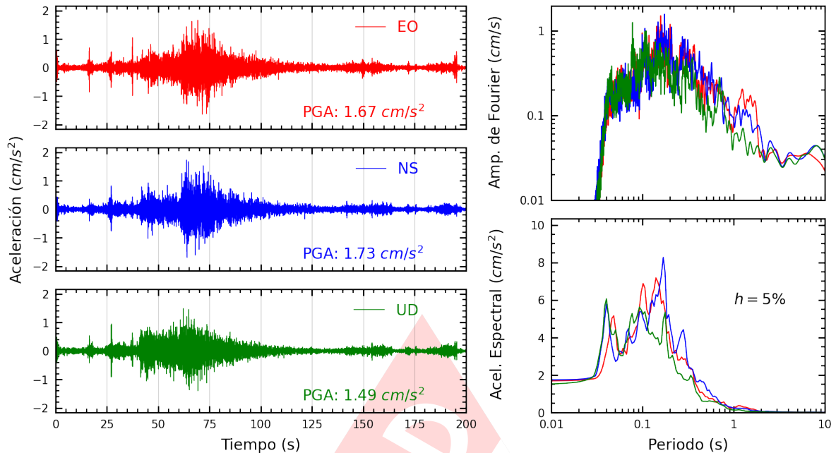
Figura A.25: Registros tiempo-historia, espectros de Fourier y de respuesta en las direcciones EO, NS y vertical de la estación PRADO. Sismo de Pisco, Pisco - Ica del 2024-03-07, 11:31:59 (Hora local)
