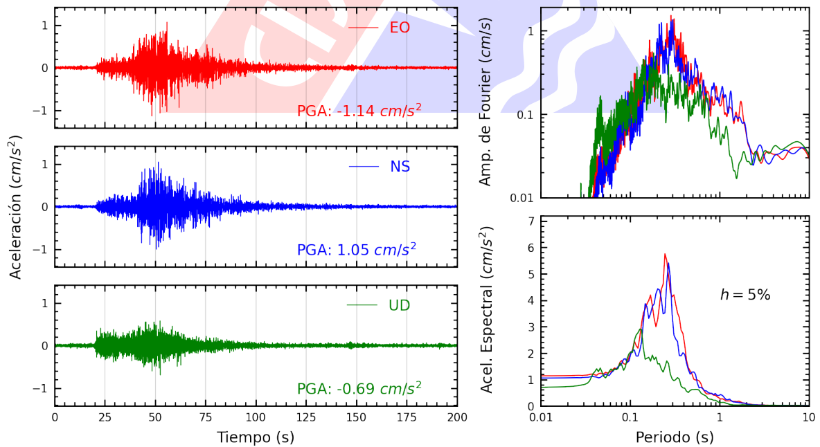
Figura A.36: Registros tiempo-historia, espectros de Fourier y de respuesta en las direcciones EO, NS y vertical de la estación DSMI. Sismo de Pisco, Pisco - Ica del 2024-03-07, 11:31:59 (Hora local)
