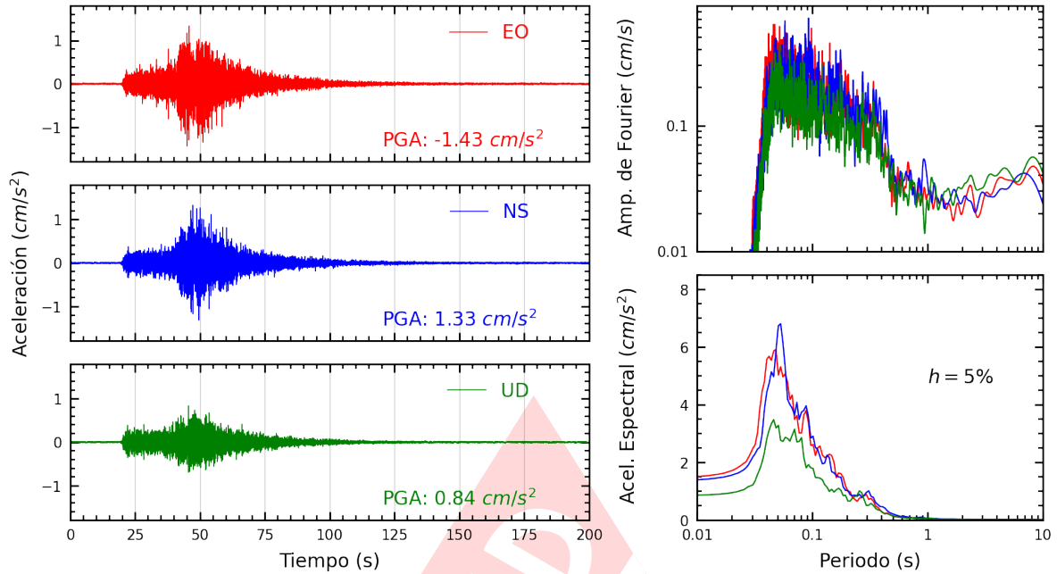
Figura A.29: Registros tiempo-historia, espectros de Fourier y de respuesta en las direcciones EO, NS y vertical de la estación UCSS. Sismo de Pisco, Pisco - Ica del 2024-03-07, 11:31:59 (Hora local)
