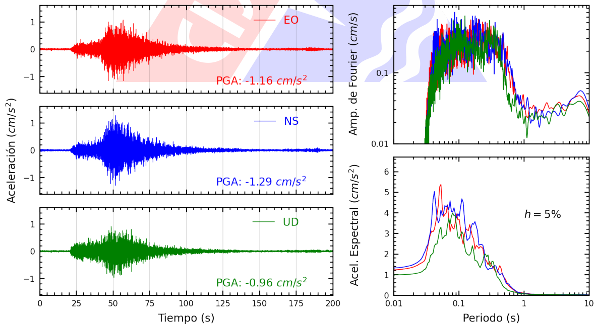
Figura A.32: Registros tiempo-historia, espectros de Fourier y de respuesta en las direcciones EO, NS y vertical de la estación COMAS. Sismo de Pisco, Pisco - Ica del 2024-03-07, 11:31:59 (Hora local)
