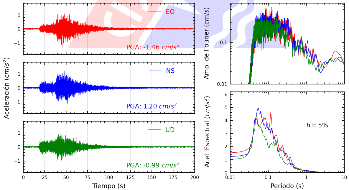
Figura A.28: Registros tiempo-historia, espectros de Fourier y de respuesta en las direcciones EO, NS y vertical de la estación CENEP. Sismo de Pisco, Pisco - Ica del 2024-03-07, 11:31:59 (Hora local)
