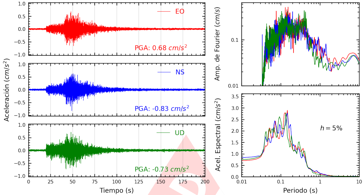
Figura A.39: Registros tiempo-historia, espectros de Fourier y de respuesta en las direcciones EO, NS y vertical de la estación BONDY. Sismo de Pisco, Pisco - Ica del 2024-03-07, 11:31:59 (Hora local)
