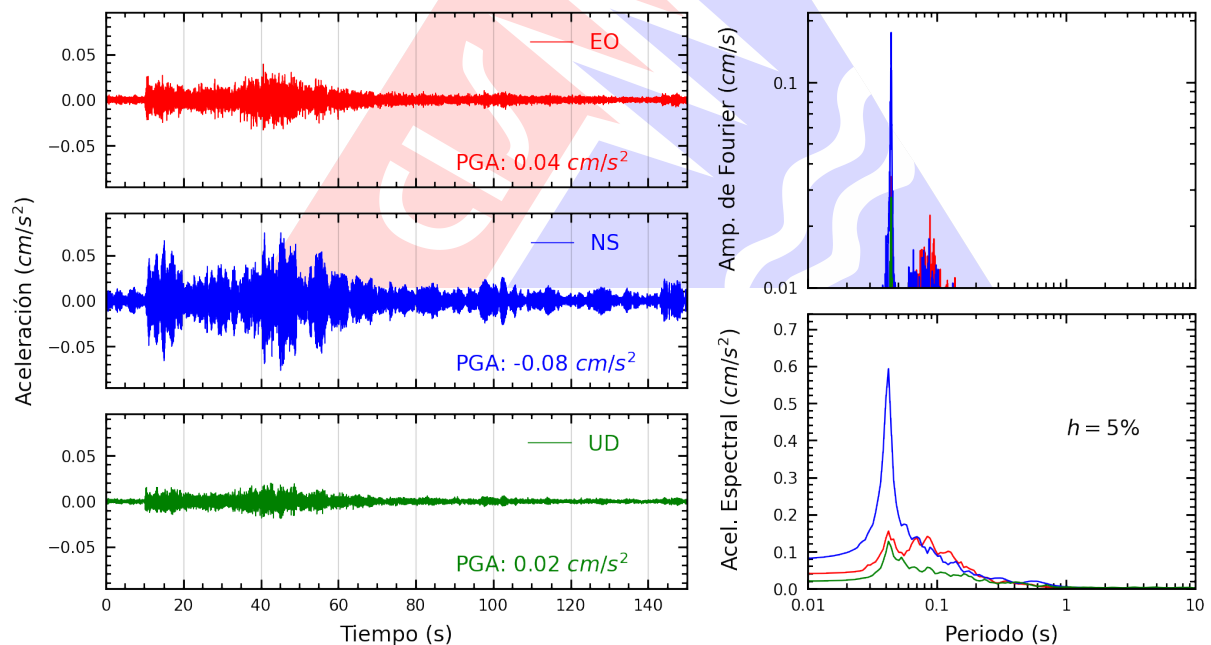
Figura A.2: Registros tiempo-historia, espectros de Fourier y de respuesta en las direcciones EO, NS y vertical de la estación UNAM. Sismo de Camana, Camana - Arequipa del 2024-03-09, 20:40:32 (Hora local)
