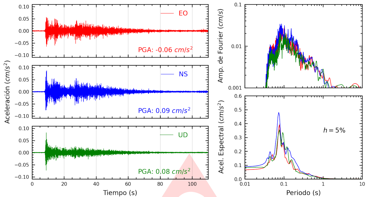
Figura A.1: Registros tiempo-historia, espectros de Fourier y de respuesta en las direcciones EO, NS y vertical de la estación UNSA. Sismo de Camana, Camana - Arequipa del 2024-03-09, 20:40:32 (Hora local)
