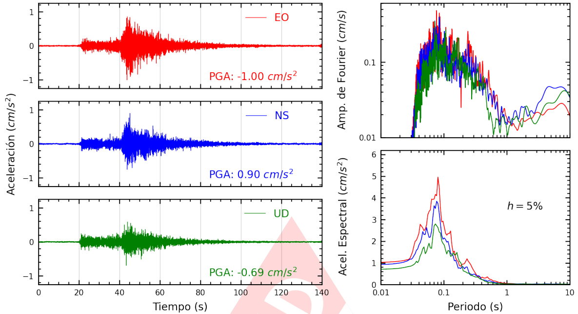
Figura A.21: Registros tiempo-historia, espectros de Fourier y de respuesta en las direcciones EO, NS y vertical de la estación CEPRE. Sismo de Pisco, Pisco - Ica del 2024-03-11, 01:29:15 (Hora local)
