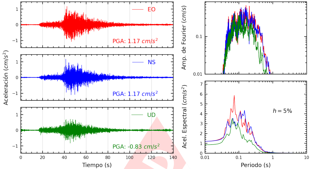
Figura A.17: Registros tiempo-historia, espectros de Fourier y de respuesta en las direcciones EO, NS y vertical de la estación SCOLI. Sismo de Pisco, Pisco - Ica del 2024-03-11, 01:29:15 (Hora local)
