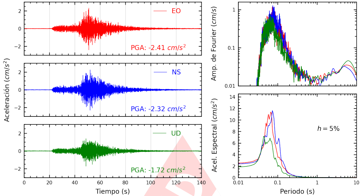
Figura A.7: Registros tiempo-historia, espectros de Fourier y de respuesta en las direcciones EO, NS y vertical de la estación JOSEO. Sismo de Pisco, Pisco - Ica del 2024-03-11, 01:29:15 (Hora local)
