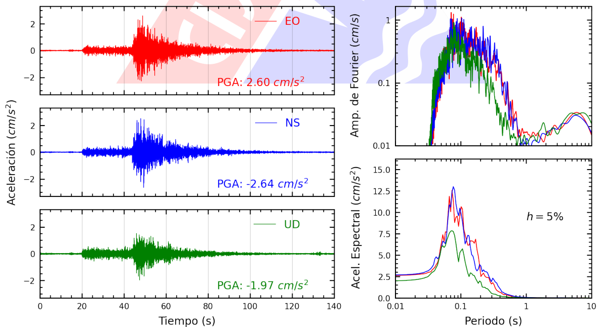
Figura A.6: Registros tiempo-historia, espectros de Fourier y de respuesta en las direcciones EO, NS y vertical de la estación ANCON. Sismo de Pisco, Pisco - Ica del 2024-03-11, 01:29:15 (Hora local)
