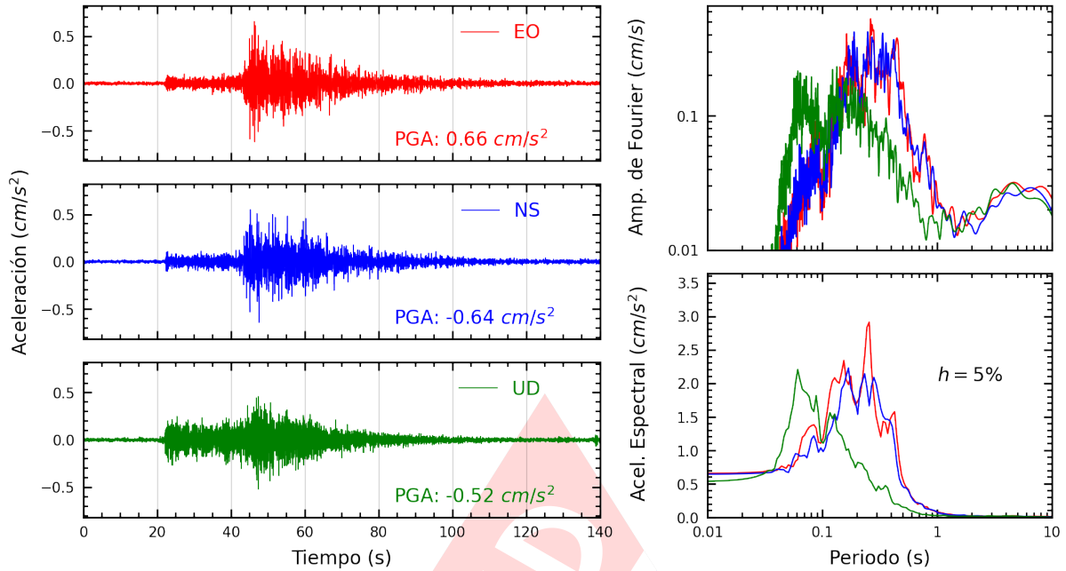
Figura A.29: Registros tiempo-historia, espectros de Fourier y de respuesta en las direcciones EO, NS y vertical de la estación ACAPU. Sismo de Pisco, Pisco - Ica del 2024-03-11, 01:29:15 (Hora local)
