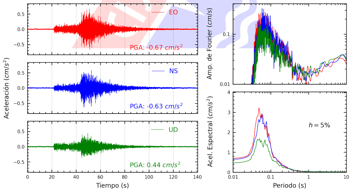
Figura A.28: Registros tiempo-historia, espectros de Fourier y de respuesta en las direcciones EO, NS y vertical de la estación UCSS. Sismo de Pisco, Pisco - Ica del 2024-03-11, 01:29:15 (Hora local)
