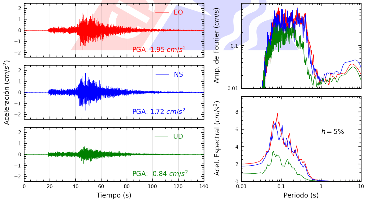
Figura A.10: Registros tiempo-historia, espectros de Fourier y de respuesta en las direcciones EO, NS y vertical de la estación DEFEN. Sismo de Pisco, Pisco - Ica del 2024-03-11, 01:29:15 (Hora local)
