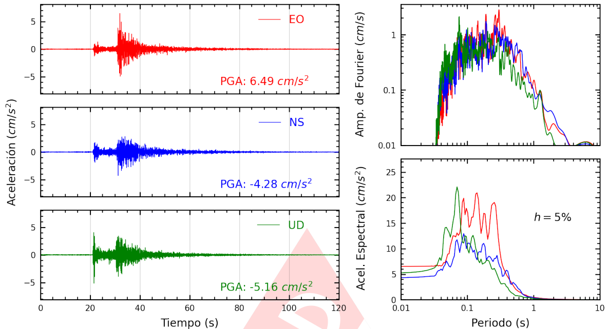
Figura A.3: Registros tiempo-historia, espectros de Fourier y de respuesta en las direcciones EO, NS y vertical de la estación UNICA. Sismo de Pisco, Pisco - Ica del 2024-03-11, 01:29:15 (Hora local)
