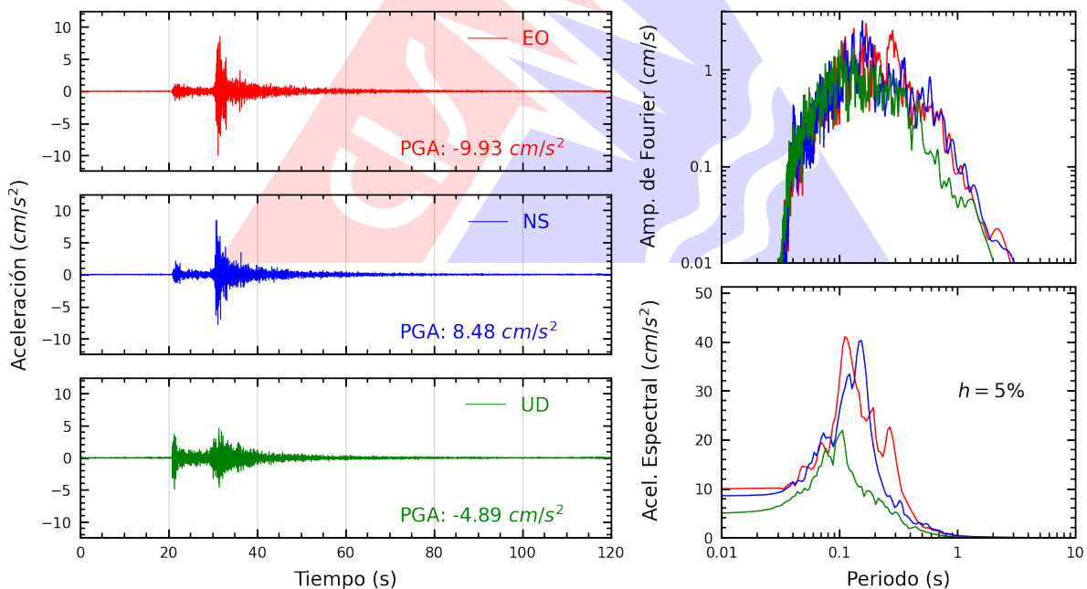
Figura A.2: Registros tiempo-historia, espectros de Fourier y de respuesta en las direcciones EO, NS y vertical de la estación SCICA. Sismo de Pisco, Pisco - Ica del 2024-03-11, 01:29:15 (Hora local)
