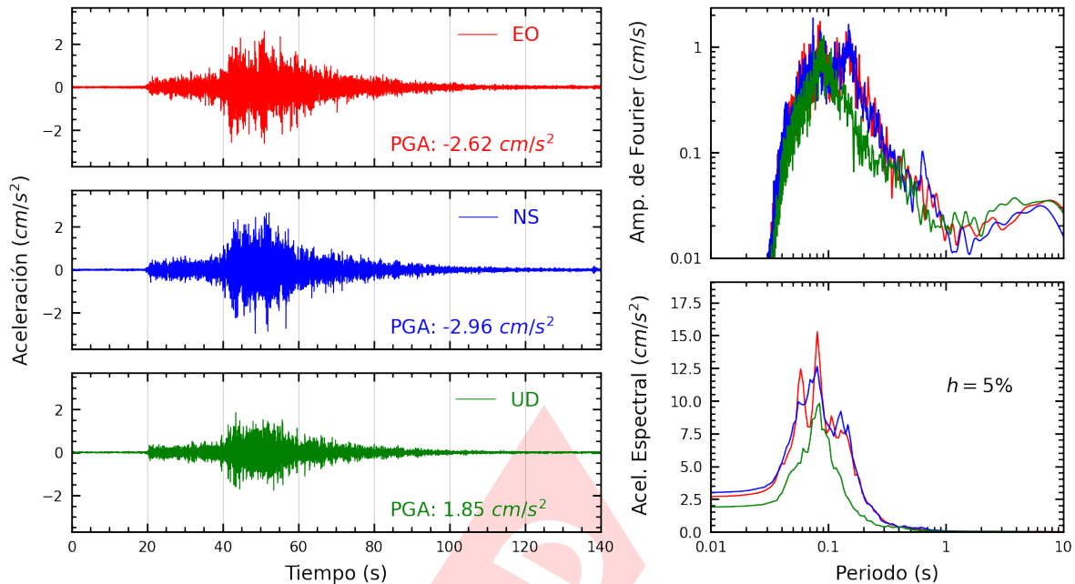
Figura A.5: Registros tiempo-historia, espectros de Fourier y de respuesta en las direcciones EO, NS y vertical de la estación USILM. Sismo de Pisco, Pisco - Ica del 2024-03-11, 01:29:15 (Hora local)
