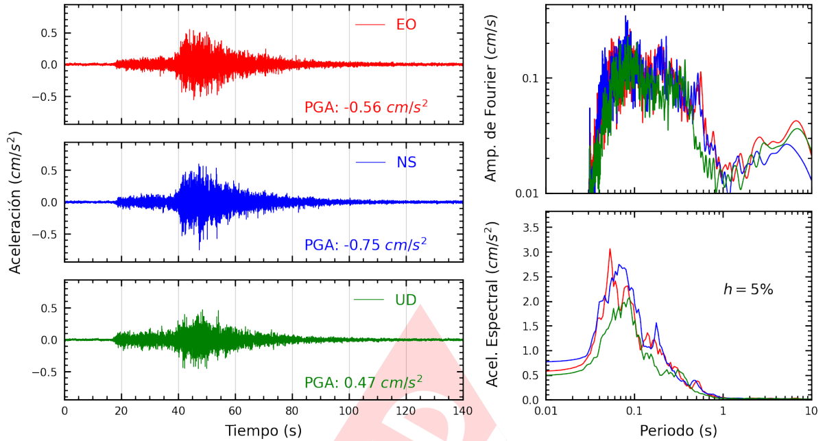
Figura A.25: Registros tiempo-historia, espectros de Fourier y de respuesta en las direcciones EO, NS y vertical de la estación COMAS. Sismo de Pisco, Pisco - Ica del 2024-03-11, 01:29:15 (Hora local)
