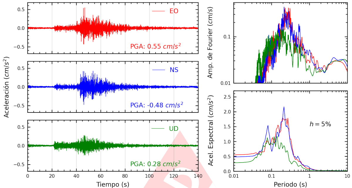
Figura A.35: Registros tiempo-historia, espectros de Fourier y de respuesta en las direcciones EO, NS y vertical de la estación DSMI. Sismo de Pisco, Pisco - Ica del 2024-03-11, 01:29:15 (Hora local)
