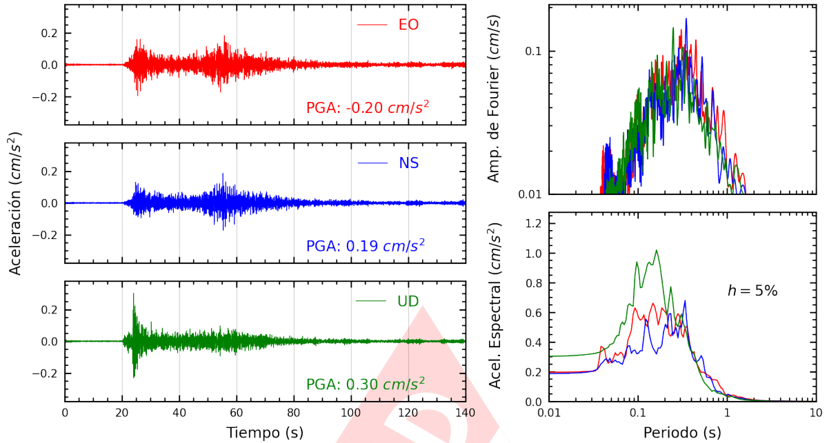
Figura A.37: Registros tiempo-historia, espectros de Fourier y de respuesta en las direcciones EO, NS y vertical de la estación SCAYA. Sismo de Pisco, Pisco - Ica del 2024-03-11, 01:29:15 (Hora local)
