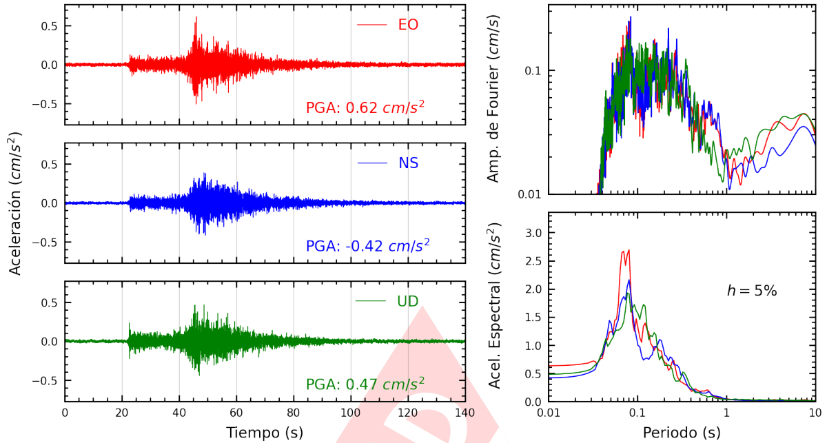
Figura A.33: Registros tiempo-historia, espectros de Fourier y de respuesta en las direcciones EO, NS y vertical de la estación UNMSM. Sismo de Pisco, Pisco - Ica del 2024-03-11, 01:29:15 (Hora local)
