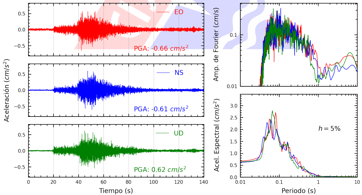
Figura A.30: Registros tiempo-historia, espectros de Fourier y de respuesta en las direcciones EO, NS y vertical de la estación IMCA. Sismo de Pisco, Pisco - Ica del 2024-03-11, 01:29:15 (Hora local)
