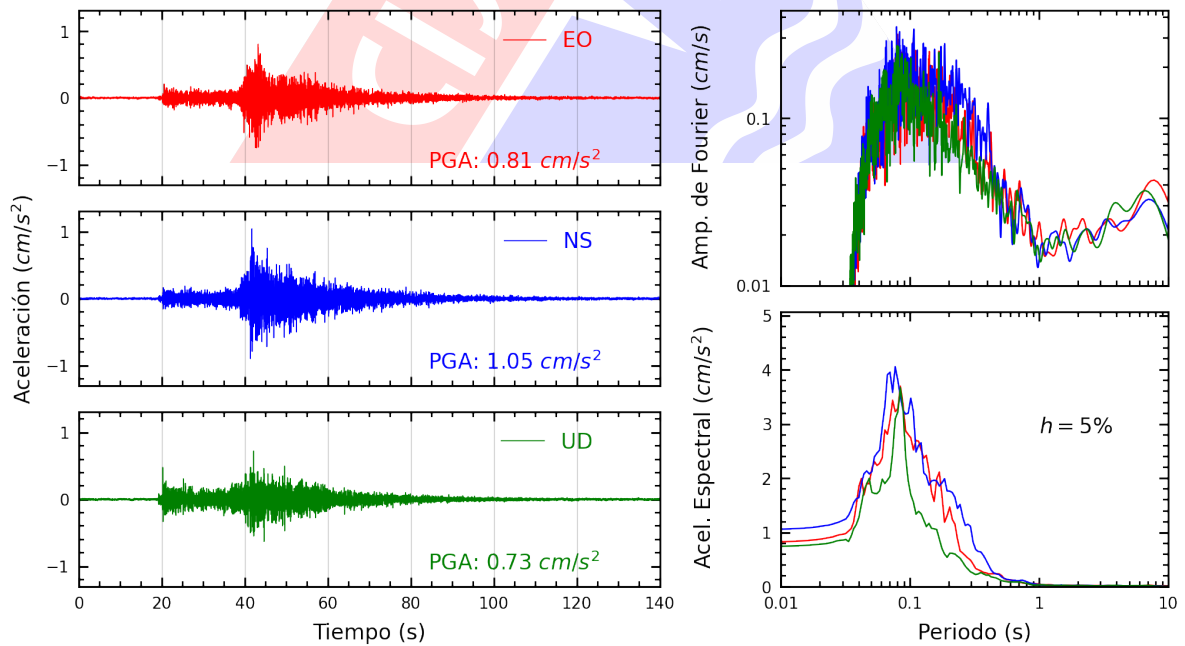
Figura A.20: Registros tiempo-historia, espectros de Fourier y de respuesta en las direcciones EO, NS y vertical de la estación SERVI. Sismo de Pisco, Pisco - Ica del 2024-03-11, 01:29:15 (Hora local)
