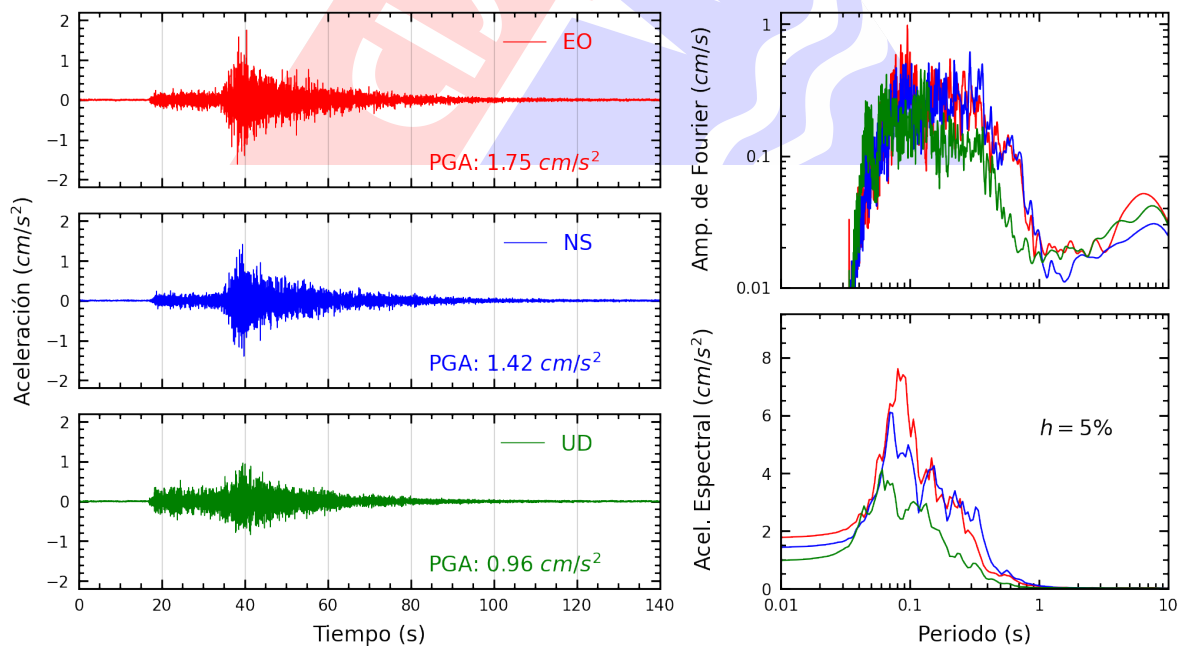
Figura A.12: Registros tiempo-historia, espectros de Fourier y de respuesta en las direcciones EO, NS y vertical de la estación USILP. Sismo de Pisco, Pisco - Ica del 2024-03-11, 01:29:15 (Hora local)
