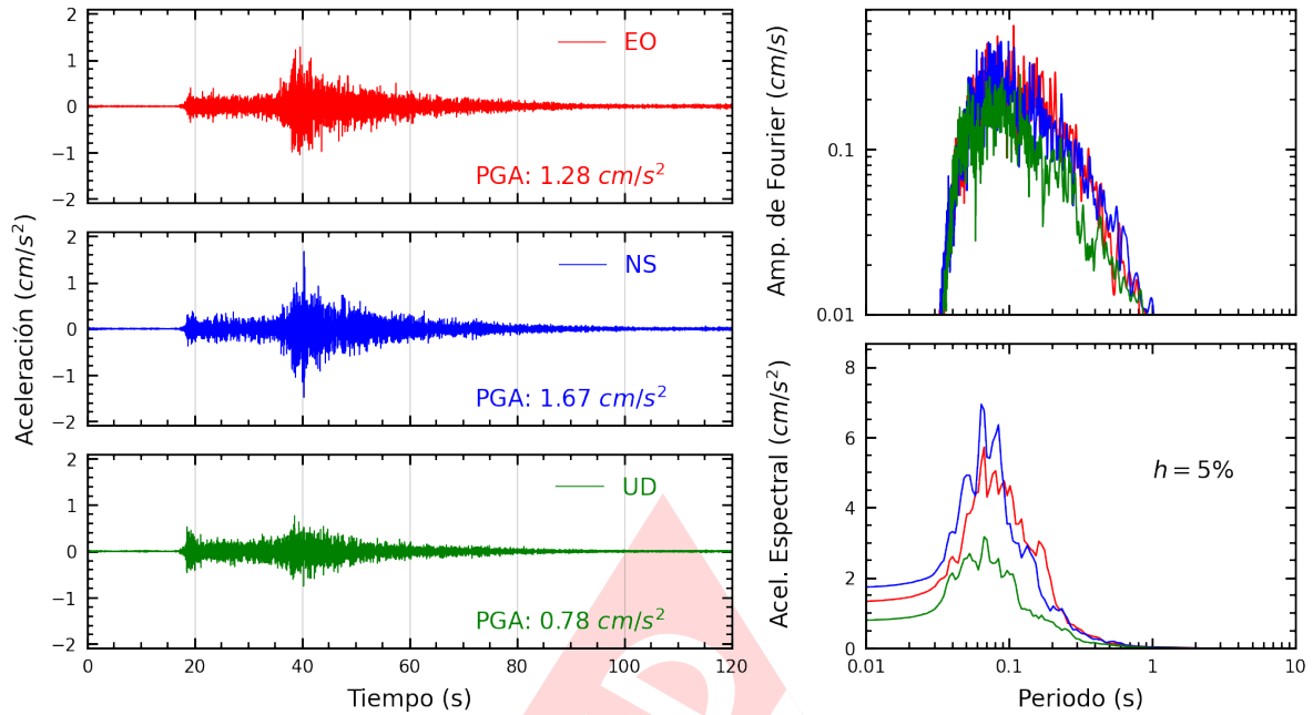
Figura A.13: Registros tiempo-historia, espectros de Fourier y de respuesta en las direcciones EO, NS y vertical de la estación PACHA. Sismo de Pisco, Pisco - Ica del 2024-03-11, 01:29:15 (Hora local)
