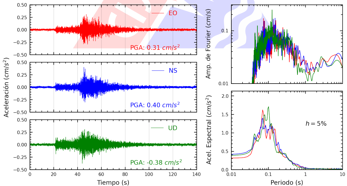
Figura A.36: Registros tiempo-historia, espectros de Fourier y de respuesta en las direcciones EO, NS y vertical de la estación BONDY. Sismo de Pisco, Pisco - Ica del 2024-03-11, 01:29:15 (Hora local)
