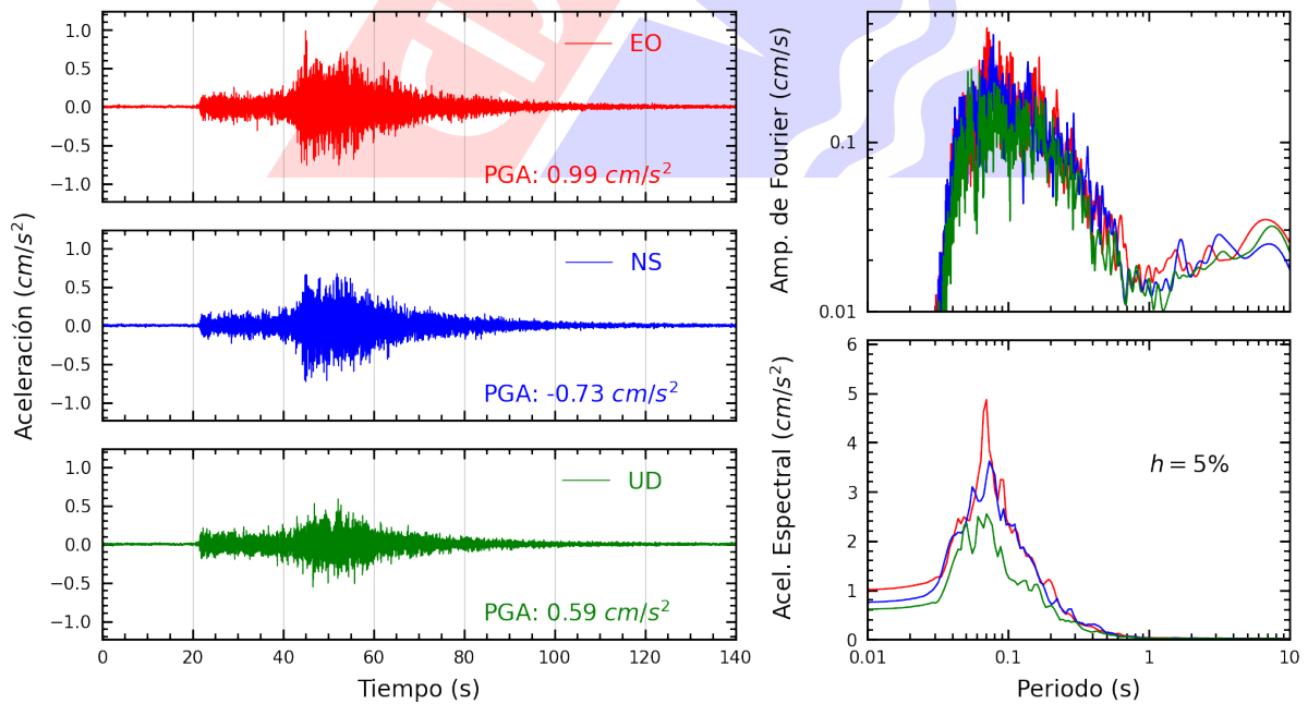
Figura A.22: Registros tiempo-historia, espectros de Fourier y de respuesta en las direcciones EO, NS y vertical de la estación FICPE. Sismo de Pisco, Pisco - Ica del 2024-03-11, 01:29:15 (Hora local)
