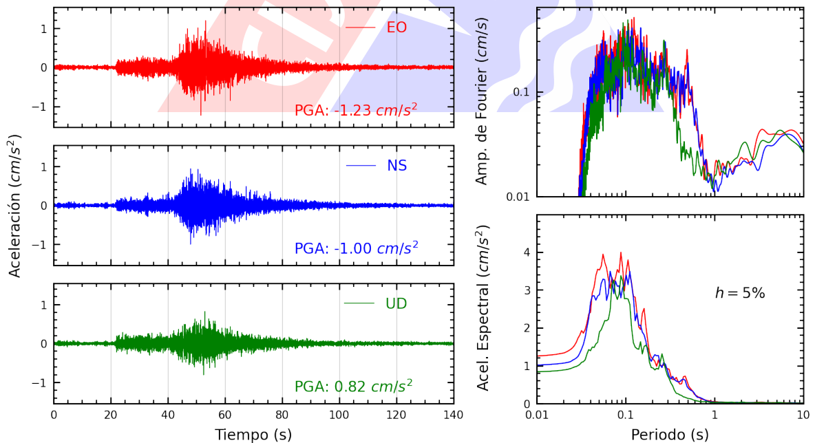
Figura A.16: Registros tiempo-historia, espectros de Fourier y de respuesta en las direcciones EO, NS y vertical de la estación OLIVO. Sismo de Pisco, Pisco - Ica del 2024-03-11, 01:29:15 (Hora local)
