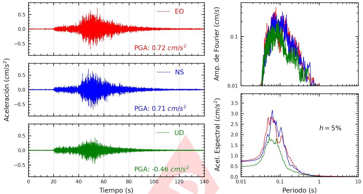
Figura A.27: Registros tiempo-historia, espectros de Fourier y de respuesta en las direcciones EO, NS y vertical de la estación ATARJ. Sismo de Pisco, Pisco - Ica del 2024-03-11, 01:29:15 (Hora local)
