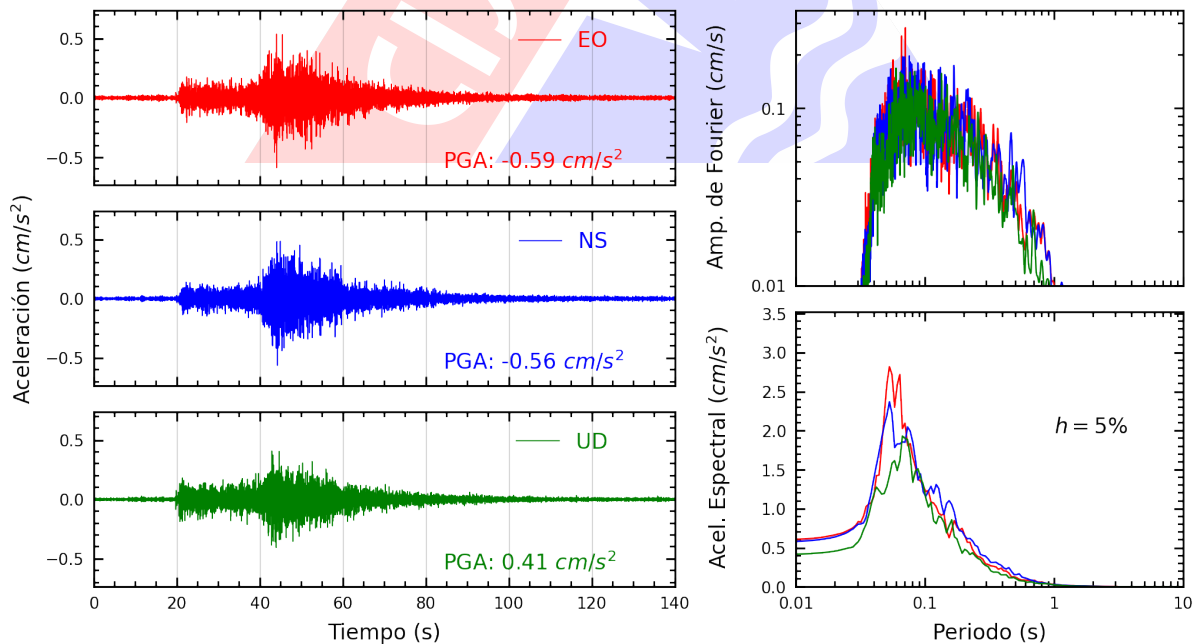
Figura A.34: Registros tiempo-historia, espectros de Fourier y de respuesta en las direcciones EO, NS y vertical de la estación BORJA. Sismo de Pisco, Pisco - Ica del 2024-03-11, 01:29:15 (Hora local)
