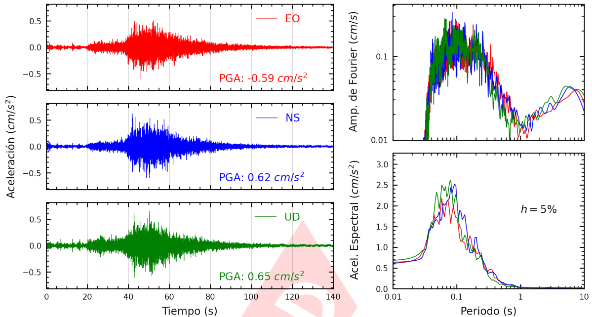
Figura A.31: Registros tiempo-historia, espectros de Fourier y de respuesta en las direcciones EO, NS y vertical de la estación USMP. Sismo de Pisco, Pisco - Ica del 2024-03-11, 01:29:15 (Hora local)
