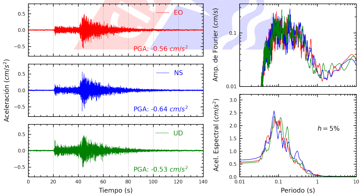
Figura A.32: Registros tiempo-historia, espectros de Fourier y de respuesta en las direcciones EO, NS y vertical de la estación UNFV. Sismo de Pisco, Pisco - Ica del 2024-03-11, 01:29:15 (Hora local)
