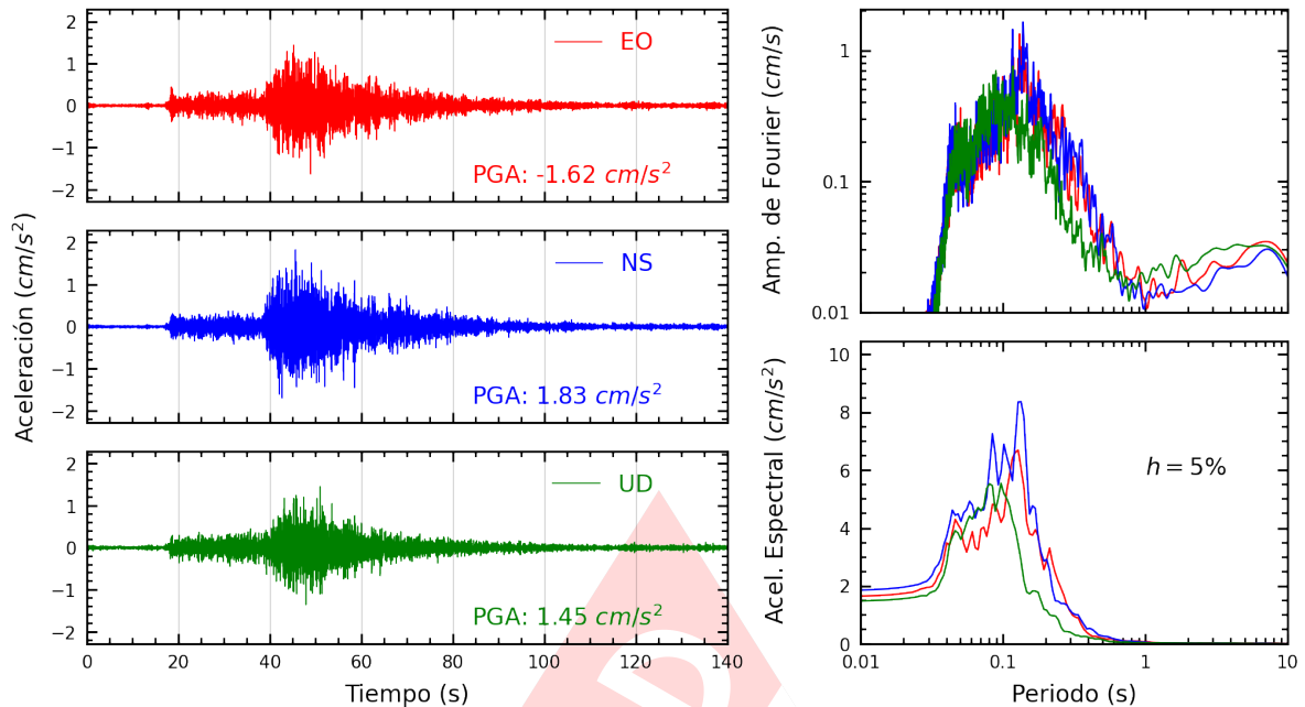
Figura A.11: Registros tiempo-historia, espectros de Fourier y de respuesta en las direcciones EO, NS y vertical de la estación CARAB. Sismo de Pisco, Pisco - Ica del 2024-03-11, 01:29:15 (Hora local)
