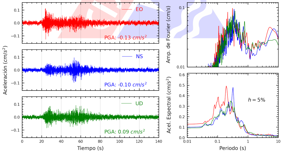
Figura A.38: Registros tiempo-historia, espectros de Fourier y de respuesta en las direcciones EO, NS y vertical de la estación UNSCH. Sismo de Pisco, Pisco - Ica del 2024-03-11, 01:29:15 (Hora local)
