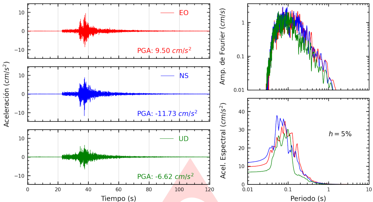
Figura A.1: Registros tiempo-historia, espectros de Fourier y de respuesta en las direcciones EO, NS y vertical de la estación ASIA. Sismo de Pisco, Pisco - Ica del 2024-03-11, 01:29:15 (Hora local)
