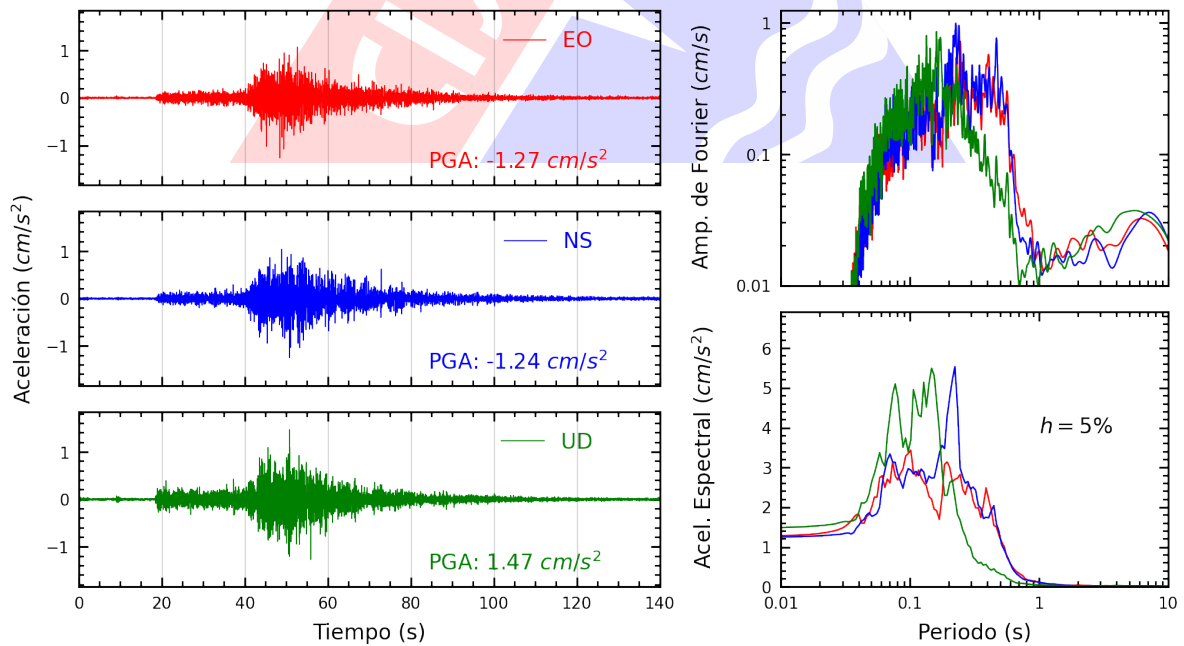
Figura A.14: Registros tiempo-historia, espectros de Fourier y de respuesta en las direcciones EO, NS y vertical de la estación MDPP. Sismo de Pisco, Pisco - Ica del 2024-03-11, 01:29:15 (Hora local)
