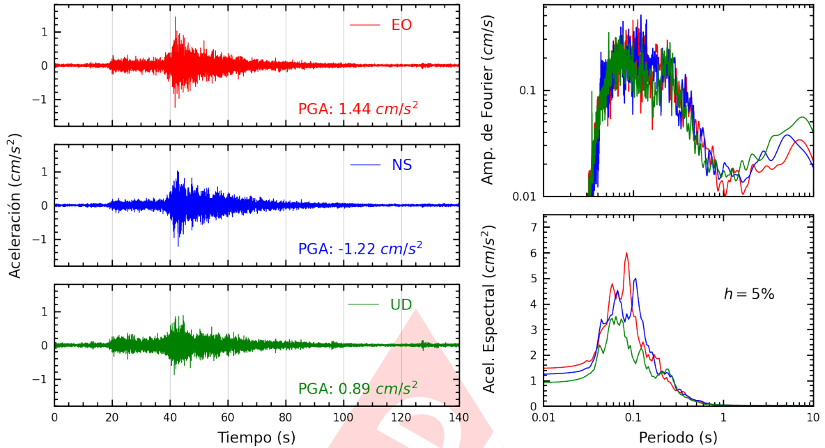
Figura A.15: Registros tiempo-historia, espectros de Fourier y de respuesta en las direcciones EO, NS y vertical de la estación URPE. Sismo de Pisco, Pisco - Ica del 2024-03-11, 01:29:15 (Hora local)
