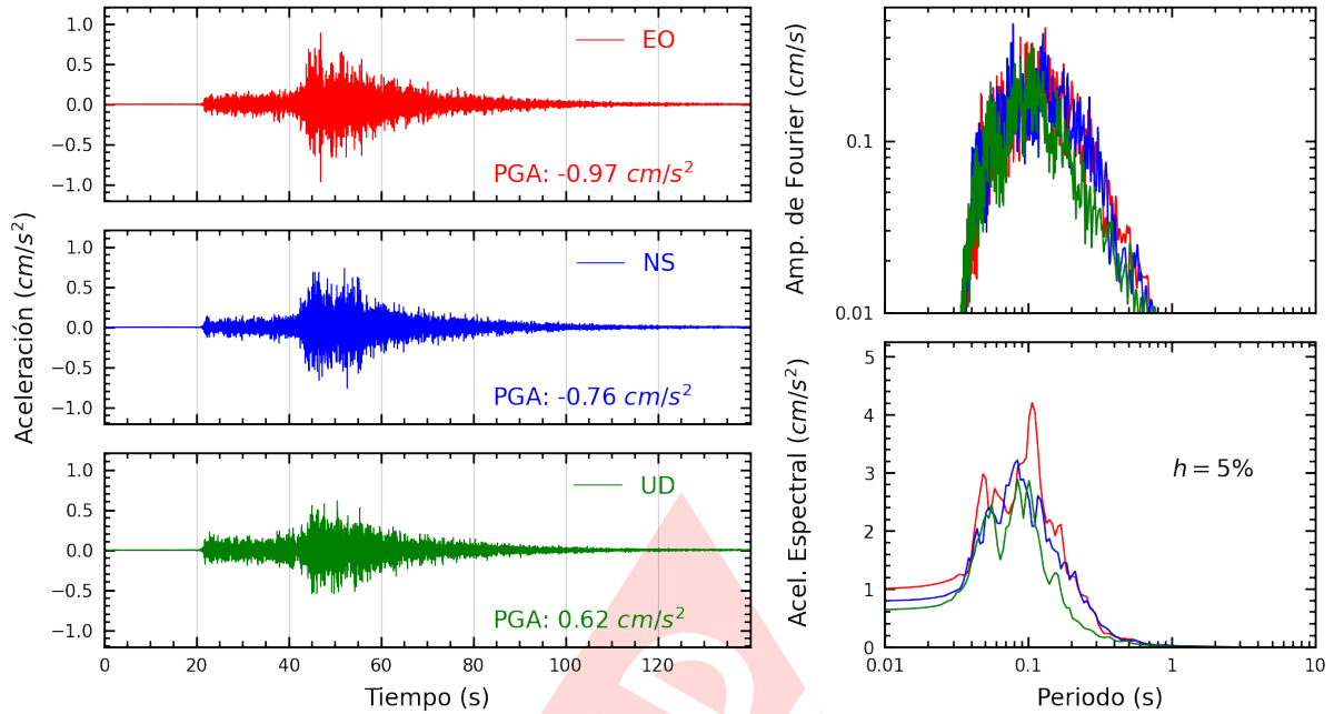
Figura A.23: Registros tiempo-historia, espectros de Fourier y de respuesta en las direcciones EO, NS y vertical de la estación JALV2. Sismo de Pisco, Pisco - Ica del 2024-03-11, 01:29:15 (Hora local)
