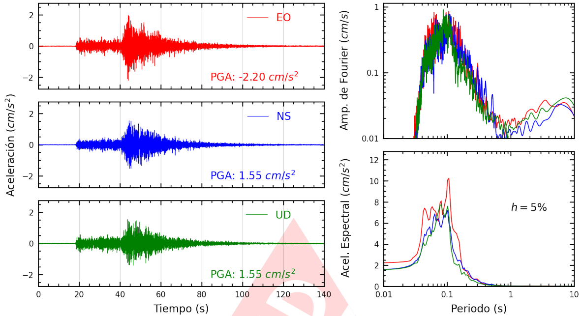
Figura A.9: Registros tiempo-historia, espectros de Fourier y de respuesta en las direcciones EO, NS y vertical de la estación AMORE. Sismo de Pisco, Pisco - Ica del 2024-03-11, 01:29:15 (Hora local)
