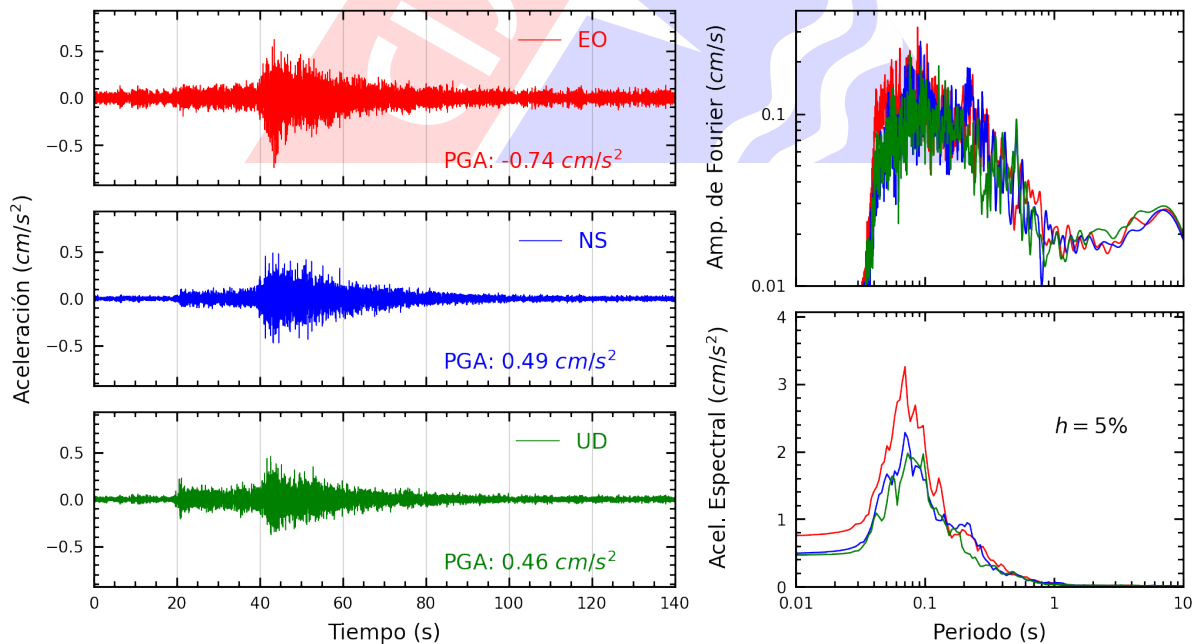
Figura A.26: Registros tiempo-historia, espectros de Fourier y de respuesta en las direcciones EO, NS y vertical de la estación INICT. Sismo de Pisco, Pisco - Ica del 2024-03-11, 01:29:15 (Hora local)
