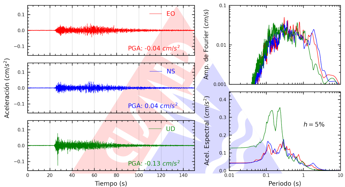
Figura A.39: Registros tiempo-historia, espectros de Fourier y de respuesta en las direcciones EO, NS y vertical de la estación UNCP. Sismo de Pisco, Pisco - Ica del 2024-03-11, 01:29:15 (Hora local)
