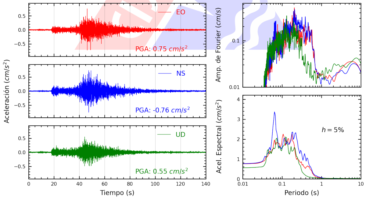
Figura A.24: Registros tiempo-historia, espectros de Fourier y de respuesta en las direcciones EO, NS y vertical de la estación VHAYA. Sismo de Pisco, Pisco - Ica del 2024-03-11, 01:29:15 (Hora local)
