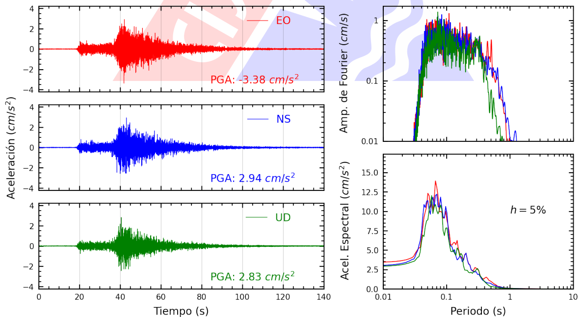
Figura A.4: Registros tiempo-historia, espectros de Fourier y de respuesta en las direcciones EO, NS y vertical de la estación UNTEL. Sismo de Pisco, Pisco - Ica del 2024-03-11, 01:29:15 (Hora local)
