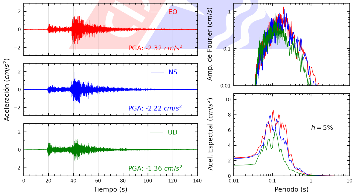
Figura A.8: Registros tiempo-historia, espectros de Fourier y de respuesta en las direcciones EO, NS y vertical de la estación SCCHO. Sismo de Pisco, Pisco - Ica del 2024-03-11, 01:29:15 (Hora local)
