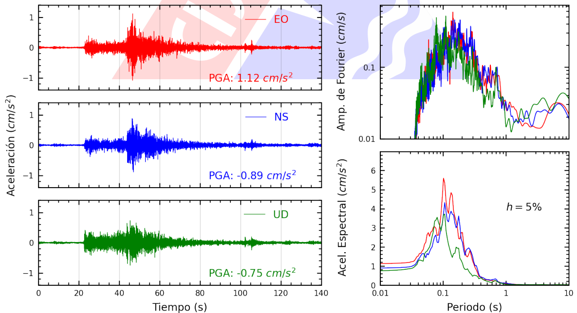
Figura A.18: Registros tiempo-historia, espectros de Fourier y de respuesta en las direcciones EO, NS y vertical de la estación PRADO. Sismo de Pisco, Pisco - Ica del 2024-03-11, 01:29:15 (Hora local)
