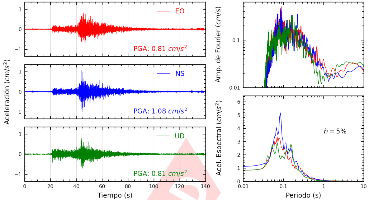
Figura A.19: Registros tiempo-historia, espectros de Fourier y de respuesta en las direcciones EO, NS y vertical de la estación UPCSM. Sismo de Pisco, Pisco - Ica del 2024-03-11, 01:29:15 (Hora local)
