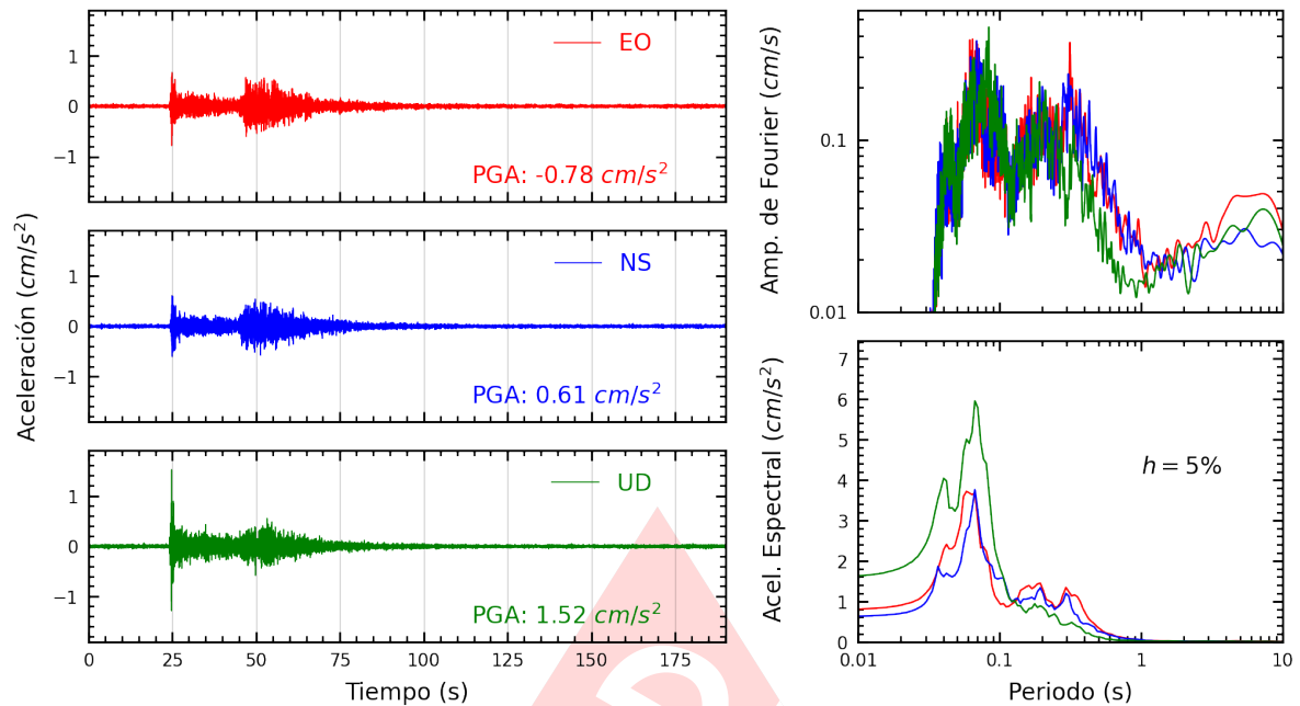
Figura A.7: Registros tiempo-historia, espectros de Fourier y de respuesta en las direcciones EO, NS y vertical de la estación MADRE. Sismo de Huarney, Huarney - Ancash del 2024-03-18, 01:45:50 (Hora local)
