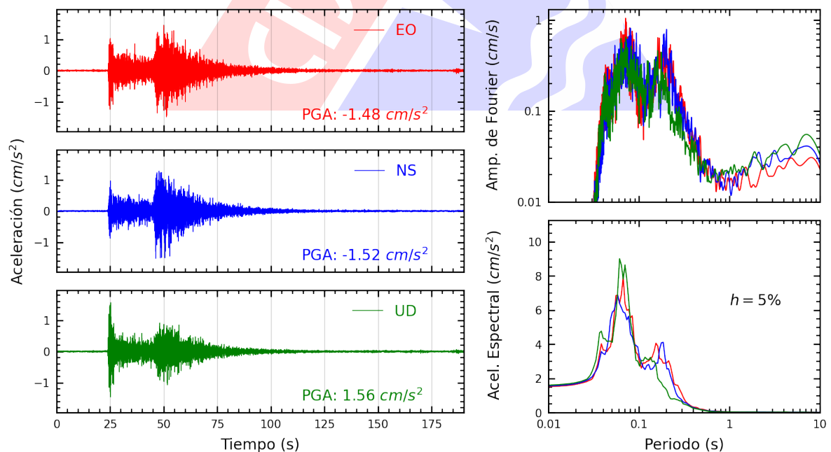
Figura A.6: Registros tiempo-historia, espectros de Fourier y de respuesta en las direcciones EO, NS y vertical de la estación INDEP. Sismo de Huarney, Huarney - Ancash del 2024-03-18, 01:45:50 (Hora local)
