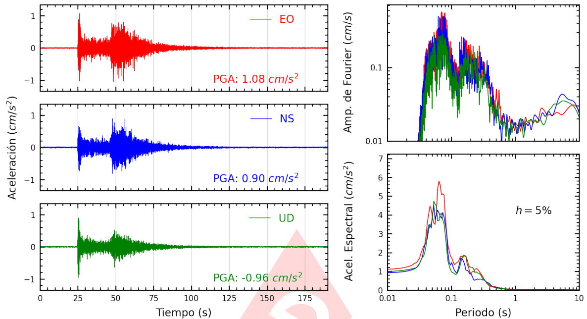
Figura A.15: Registros tiempo-historia, espectros de Fourier y de respuesta en las direcciones EO, NS y vertical de la estación FICPE. Sismo de Huarney, Huarney - Ancash del 2024-03-18, 01:45:50 (Hora local)
