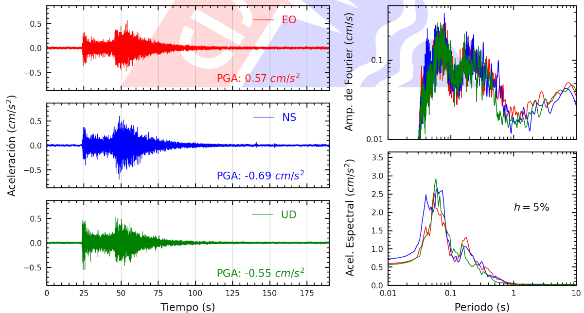
Figura A.22: Registros tiempo-historia, espectros de Fourier y de respuesta en las direcciones EO, NS y vertical de la estación COMAS. Sismo de Huarney, Huarney - Ancash del 2024-03-18, 01:45:50 (Hora local)
