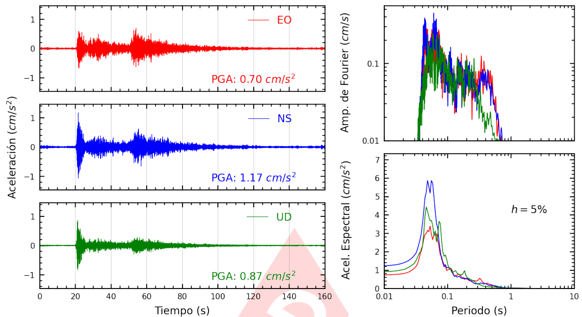
Figura A.13: Registros tiempo-historia, espectros de Fourier y de respuesta en las direcciones EO, NS y vertical de la estación SCTRU. Sismo de Huarney, Huarney - Ancash del 2024-03-18, 01:45:50 (Hora local)
