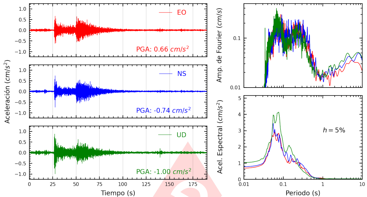
Figura A.17: Registros tiempo-historia, espectros de Fourier y de respuesta en las direcciones EO, NS y vertical de la estación URPE. Sismo de Huarney, Huarney - Ancash del 2024-03-18, 01:45:50 (Hora local)
