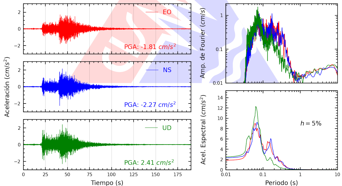
Figura A.2: Registros tiempo-historia, espectros de Fourier y de respuesta en las direcciones EO, NS y vertical de la estación ANCON. Sismo de Huarney, Huarney - Ancash del 2024-03-18, 01:45:50 (Hora local)
