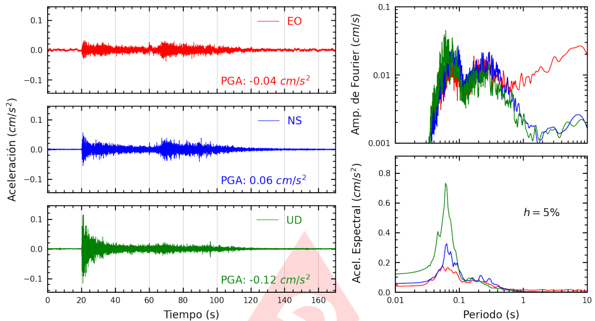
Figura A.35: Registros tiempo-historia, espectros de Fourier y de respuesta en las direcciones EO, NS y vertical de la estación SCCHL. Sismo de Huarney, Huarney - Ancash del 2024-03-18, 01:45:50 (Hora local)
