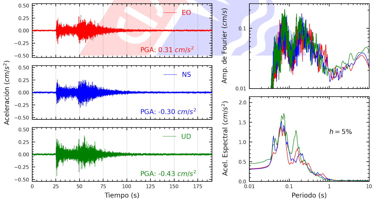
Figura A.32: Registros tiempo-historia, espectros de Fourier y de respuesta en las direcciones EO, NS y vertical de la estación UNFV. Sismo de Huarmey, Huarmey - Ancash del 2024-03-18, 01:45:50 (Hora local)
