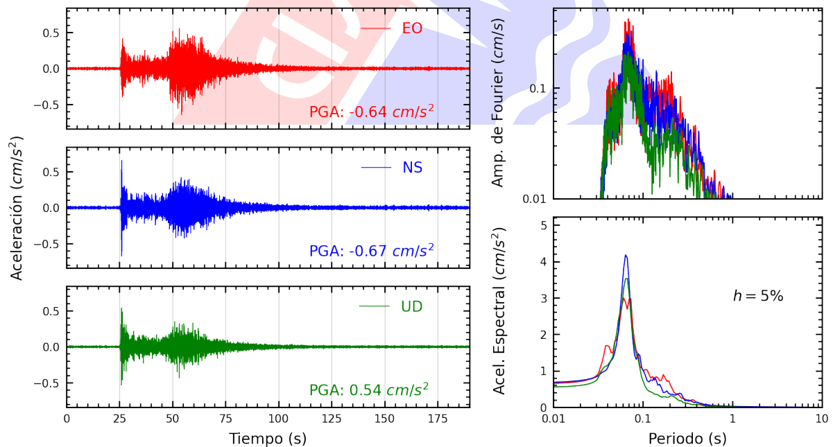
Figura A.24: Registros tiempo-historia, espectros de Fourier y de respuesta en las direcciones EO, NS y vertical de la estación ATARJ. Sismo de Huarney, Huarney - Ancash del 2024-03-18, 01:45:50 (Hora local)
