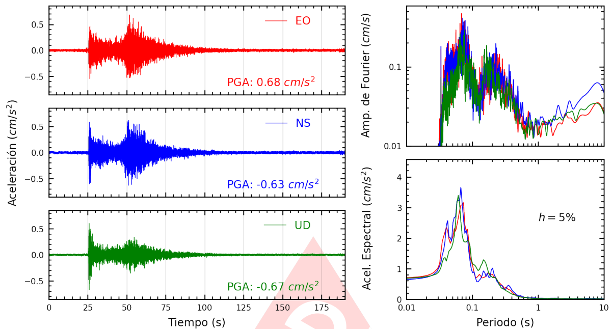
Figura A.23: Registros tiempo-historia, espectros de Fourier y de respuesta en las direcciones EO, NS y vertical de la estación CEPRE. Sismo de Huarney, Huarney - Ancash del 2024-03-18, 01:45:50 (Hora local)
