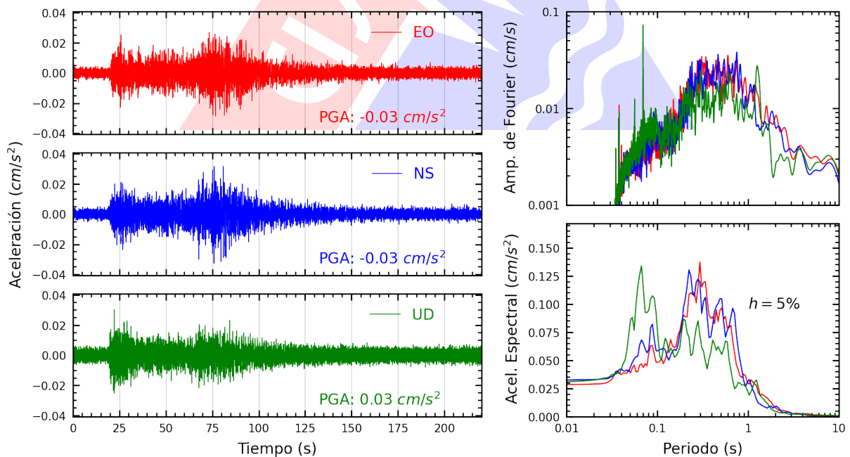
Figura A.36: Registros tiempo-historia, espectros de Fourier y de respuesta en las direcciones EO, NS y vertical de la estación UNC. Sismo de Huarney, Huarney - Ancash del 2024-03-18, 01:45:50 (Hora local)
