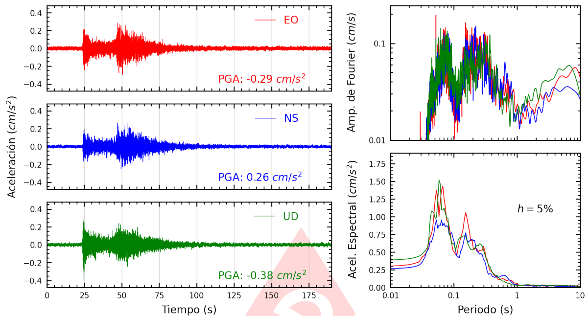
Figura A.33: Registros tiempo-historia, espectros de Fourier y de respuesta en las direcciones EO, NS y vertical de la estación UNMSM. Sismo de Huarney, Huarney - Ancash del 2024-03-18, 01:45:50 (Hora local)
