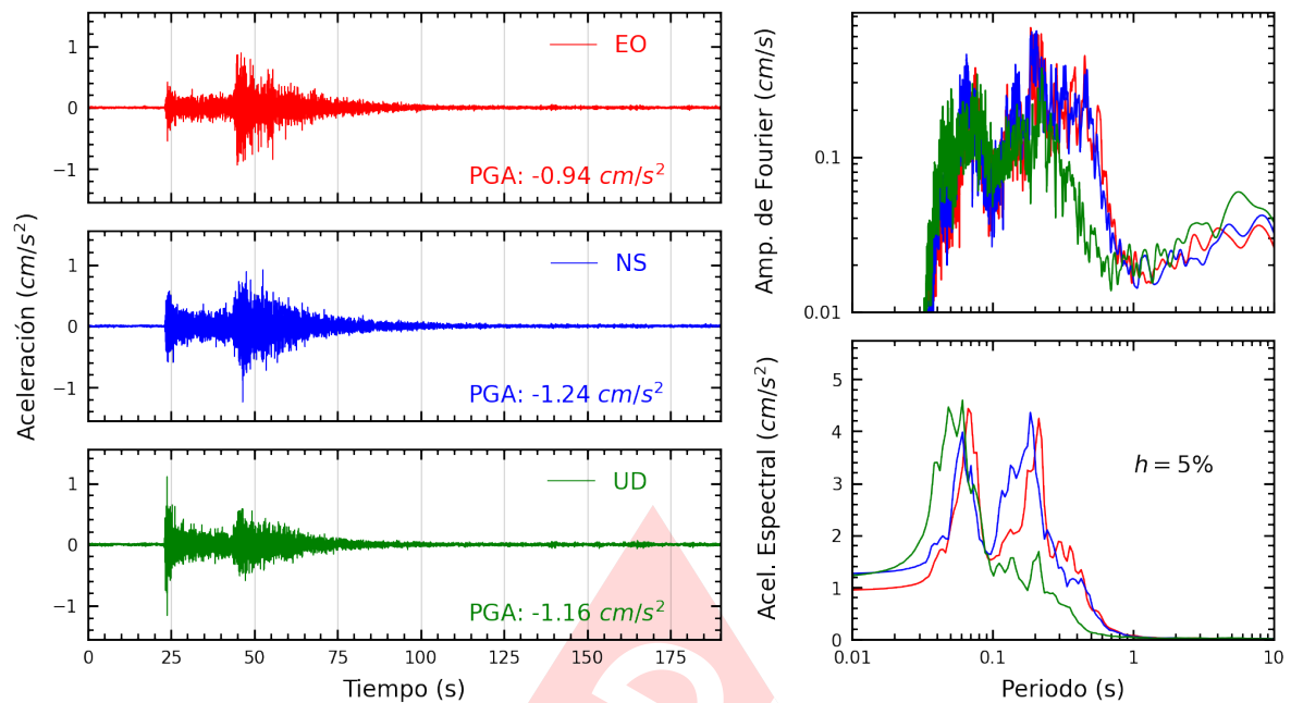
Figura A.11: Registros tiempo-historia, espectros de Fourier y de respuesta en las direcciones EO, NS y vertical de la estación VHAYA. Sismo de Huarney, Huarney - Ancash del 2024-03-18, 01:45:50 (Hora local)
