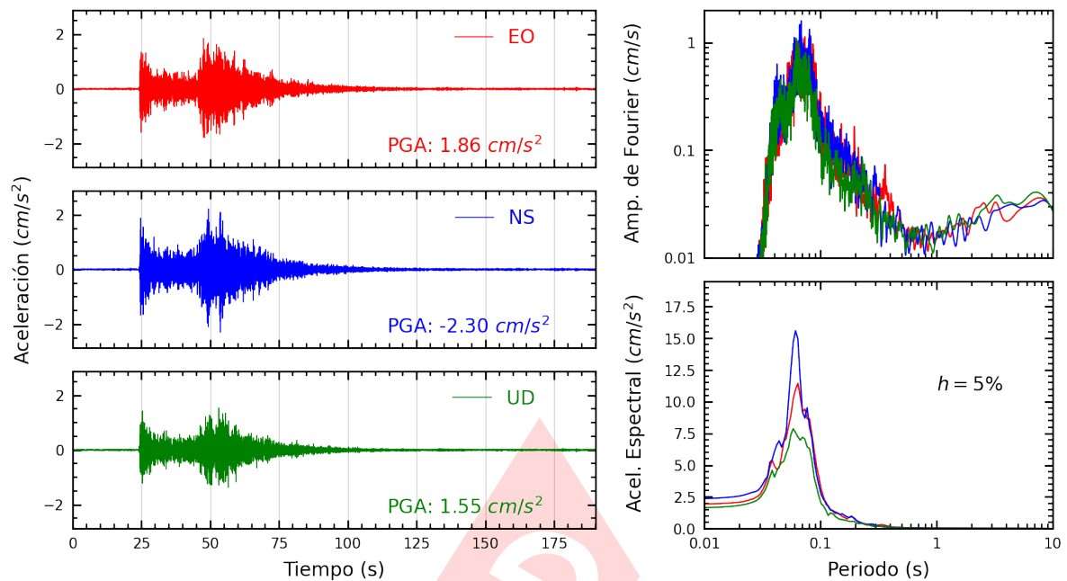
Figura A.3: Registros tiempo-historia, espectros de Fourier y de respuesta en las direcciones EO, NS y vertical de la estación JOSEO. Sismo de Huarney, Huarney - Ancash del 2024-03-18, 01:45:50 (Hora local)
