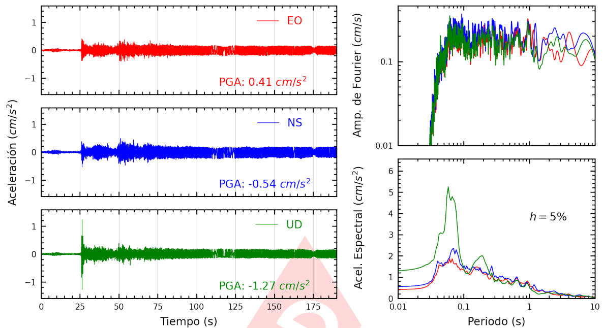
Figura A.9: Registros tiempo-historia, espectros de Fourier y de respuesta en las direcciones EO, NS y vertical de la estación CENEP. Sismo de Huarney, Huarney - Ancash del 2024-03-18, 01:45:50 (Hora local)
