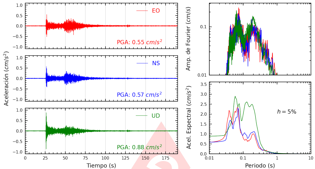
Figura A.19: Registros tiempo-historia, espectros de Fourier y de respuesta en las direcciones EO, NS y vertical de la estación BORJA. Sismo de Huarney, Huarney - Ancash del 2024-03-18, 01:45:50 (Hora local)
