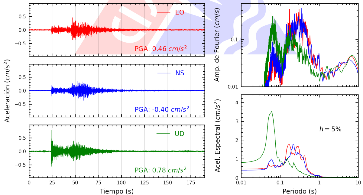
Figura A.20: Registros tiempo-historia, espectros de Fourier y de respuesta en las direcciones EO, NS y vertical de la estación ACAPU. Sismo de Huarney, Huarney - Ancash del 2024-03-18, 01:45:50 (Hora local)
