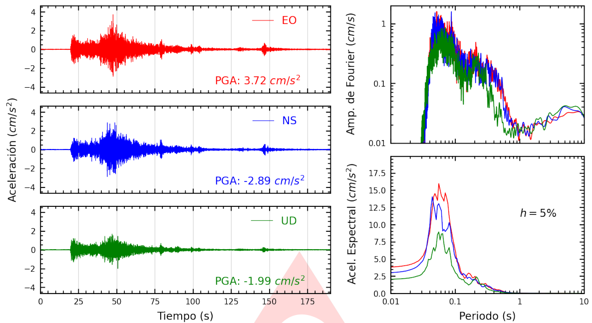
Figura A.1: Registros tiempo-historia, espectros de Fourier y de respuesta en las direcciones EO, NS y vertical de la estación USP. Sismo de Huarney, Huarney - Ancash del 2024-03-18, 01:45:50 (Hora local)
