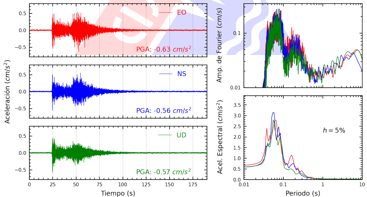
Figura A.26: Registros tiempo-historia, espectros de Fourier y de respuesta en las direcciones EO, NS y vertical de la estación UCSS. Sismo de Huarney, Huarney - Ancash del 2024-03-18, 01:45:50 (Hora local)
