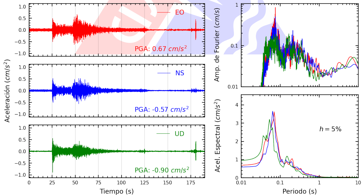
Figura A.18: Registros tiempo-historia, espectros de Fourier y de respuesta en las direcciones EO, NS y vertical de la estación UPCS. Sismo de Huarney, Huarney - Ancash del 2024-03-18, 01:45:50 (Hora local)
