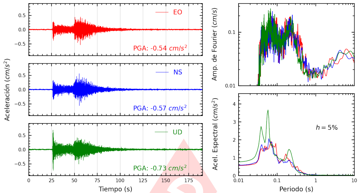
Figura A.21: Registros tiempo-historia, espectros de Fourier y de respuesta en las direcciones EO, NS y vertical de la estación USMP. Sismo de Huarney, Huarney - Ancash del 2024-03-18, 01:45:50 (Hora local)
