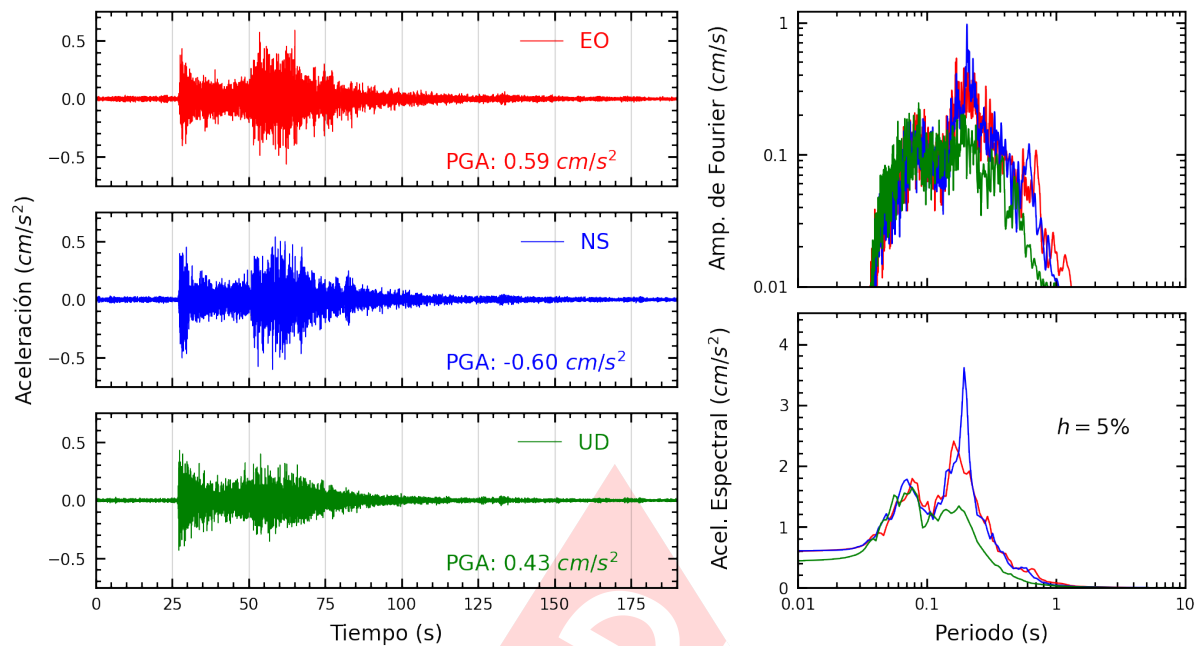
Figura A.27: Registros tiempo-historia, espectros de Fourier y de respuesta en las direcciones EO, NS y vertical de la estación SCCHO. Sismo de Huarney, Huarney - Ancash del 2024-03-18, 01:45:50 (Hora local)
