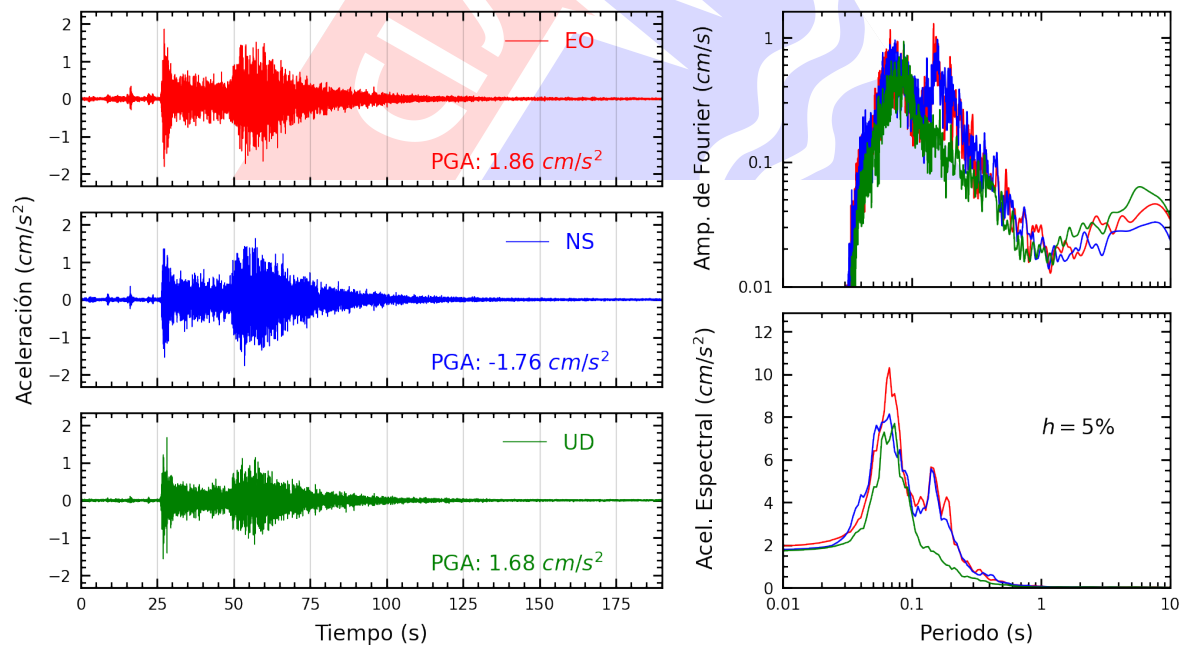
Figura A.4: Registros tiempo-historia, espectros de Fourier y de respuesta en las direcciones EO, NS y vertical de la estación USILM. Sismo de Huarney, Huarney - Ancash del 2024-03-18, 01:45:50 (Hora local)
