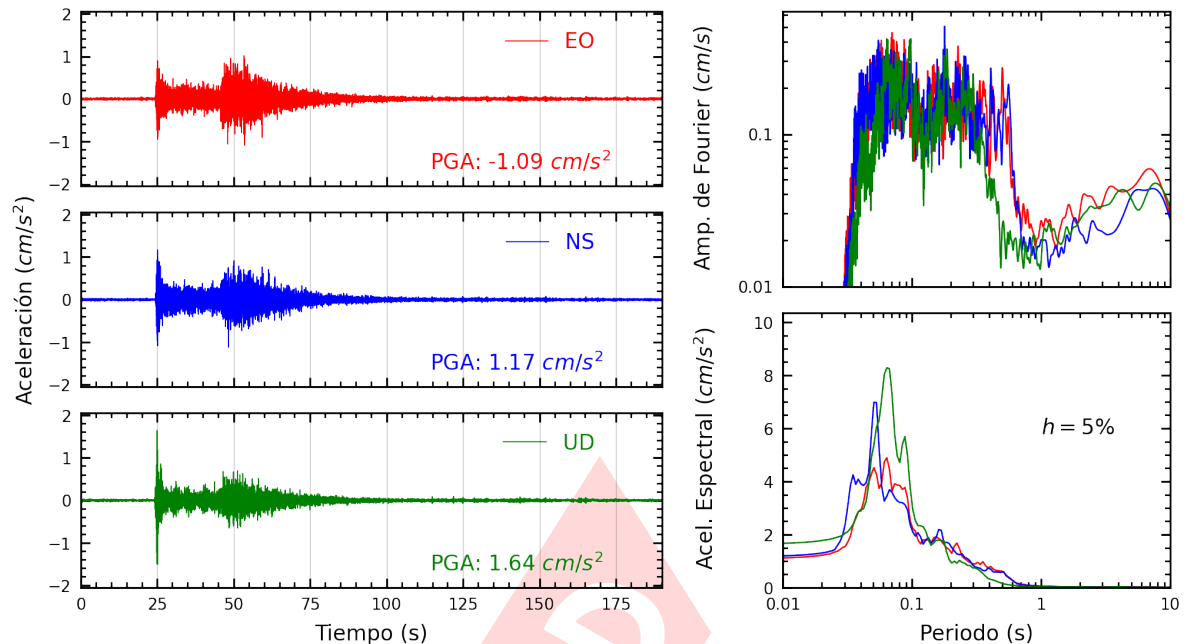
Figura A.5: Registros tiempo-historia, espectros de Fourier y de respuesta en las direcciones EO, NS y vertical de la estación OLIVO. Sismo de Huarney, Huarney - Ancash del 2024-03-18, 01:45:50 (Hora local)
