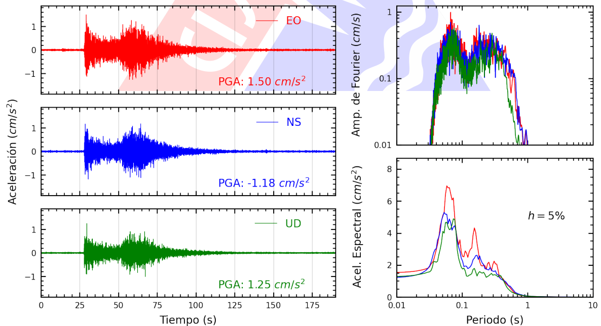
Figura A.8: Registros tiempo-historia, espectros de Fourier y de respuesta en las direcciones EO, NS y vertical de la estación UNTEL. Sismo de Huarney, Huarney - Ancash del 2024-03-18, 01:45:50 (Hora local)
