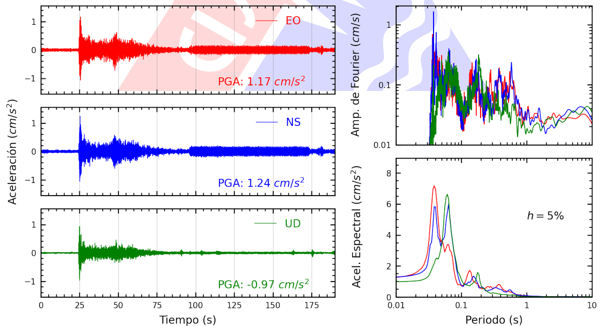
Figura A.10: Registros tiempo-historia, espectros de Fourier y de respuesta en las direcciones EO, NS y vertical de la estación DHNPE. Sismo de Huarney, Huarney - Ancash del 2024-03-18, 01:45:50 (Hora local)
