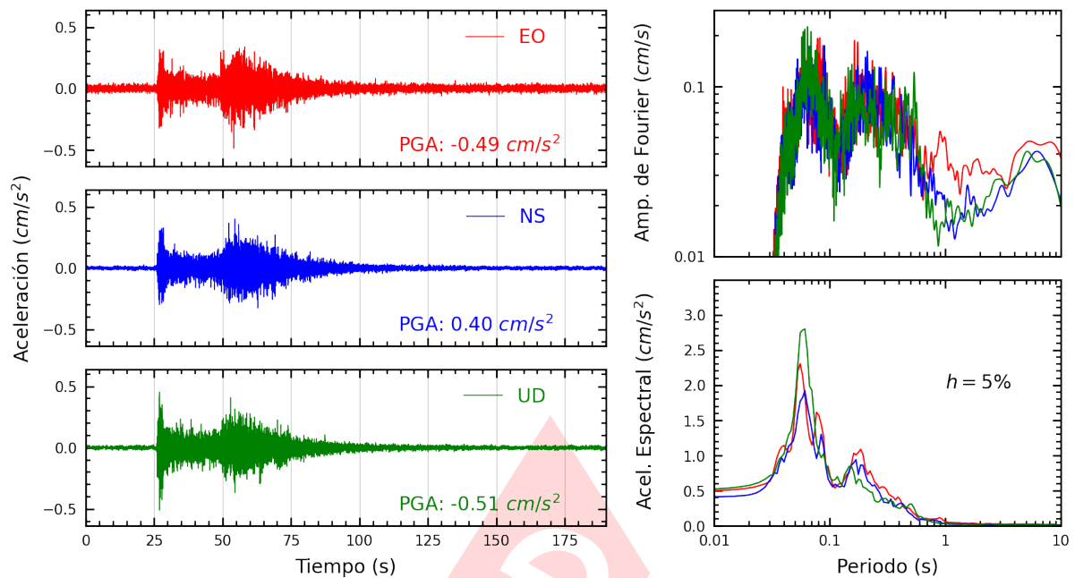
Figura A.31: Registros tiempo-historia, espectros de Fourier y de respuesta en las direcciones EO, NS y vertical de la estación IMCA. Sismo de Huarmey, Huarmey - Ancash del 2024-03-18, 01:45:50 (Hora local)
