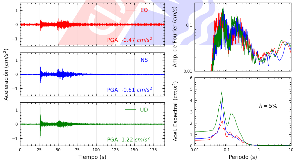
Figura A.12: Registros tiempo-historia, espectros de Fourier y de respuesta en las direcciones EO, NS y vertical de la estación INICT. Sismo de Huarney, Huarney - Ancash del 2024-03-18, 01:45:50 (Hora local)
