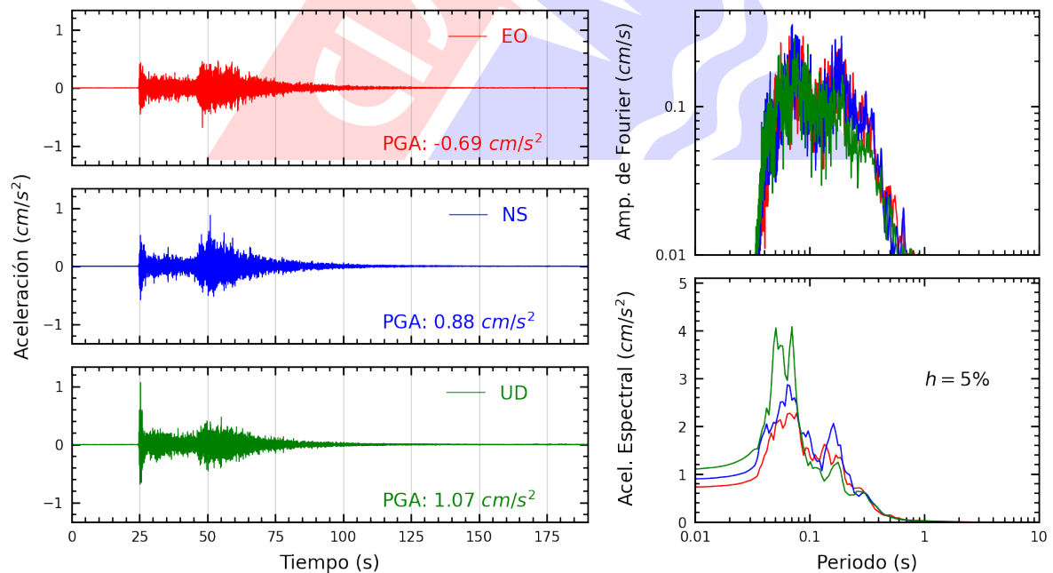
Figura A.16: Registros tiempo-historia, espectros de Fourier y de respuesta en las direcciones EO, NS y vertical de la estación JALV2. Sismo de Huarney, Huarney - Ancash del 2024-03-18, 01:45:50 (Hora local)
