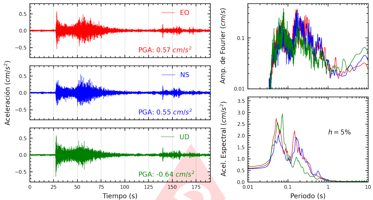
Figura A.25: Registros tiempo-historia, espectros de Fourier y de respuesta en las direcciones EO, NS y vertical de la estación PRADO. Sismo de Huarney, Huarney - Ancash del 2024-03-18, 01:45:50 (Hora local)
