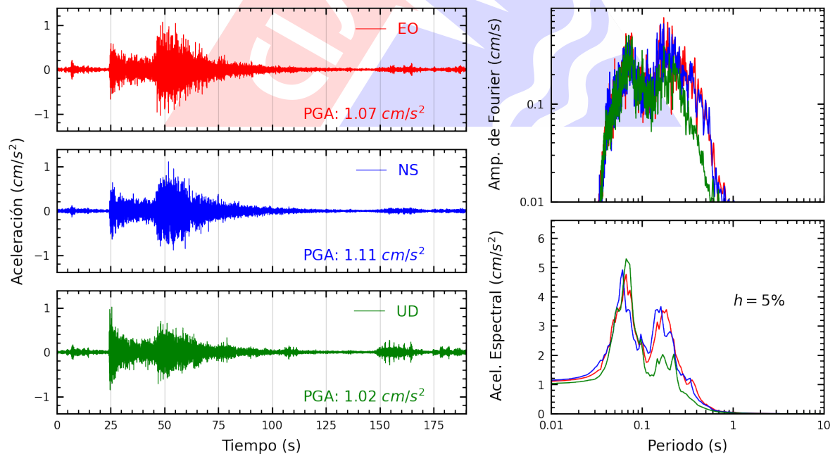
Figura A.14: Registros tiempo-historia, espectros de Fourier y de respuesta en las direcciones EO, NS y vertical de la estación SCOLI. Sismo de Huarney, Huarney - Ancash del 2024-03-18, 01:45:50 (Hora local)
