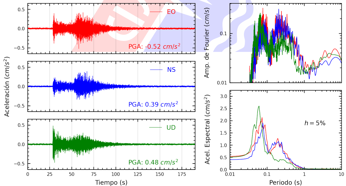
Figura A.30: Registros tiempo-historia, espectros de Fourier y de respuesta en las direcciones EO, NS y vertical de la estación USILP. Sismo de Huarmey, Huarmey - Ancash del 2024-03-18, 01:45:50 (Hora local)
