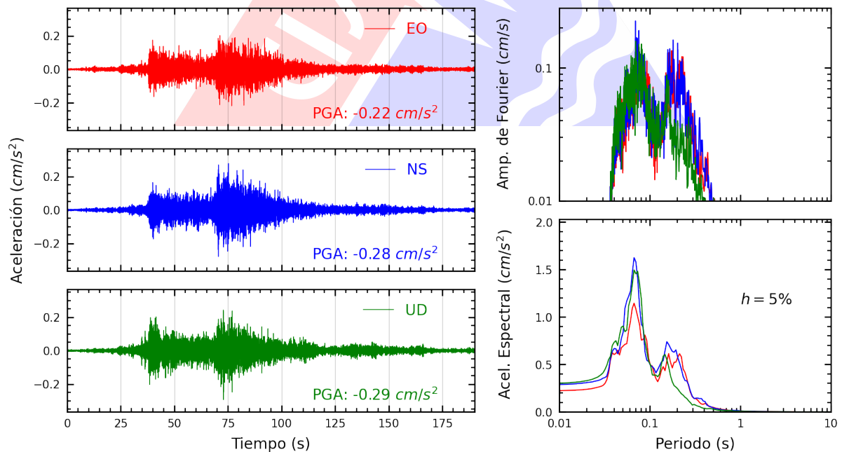
Figura A.34: Registros tiempo-historia, espectros de Fourier y de respuesta en las direcciones EO, NS y vertical de la estación ASIA. Sismo de Huarney, Huarney - Ancash del 2024-03-18, 01:45:50 (Hora local)
