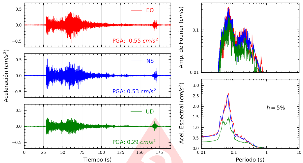
Figura A.29: Registros tiempo-historia, espectros de Fourier y de respuesta en las direcciones EO, NS y vertical de la estación PACHA. Sismo de Huarmey, Huarmey - Ancash del 2024-03-18, 01:45:50 (Hora local)
