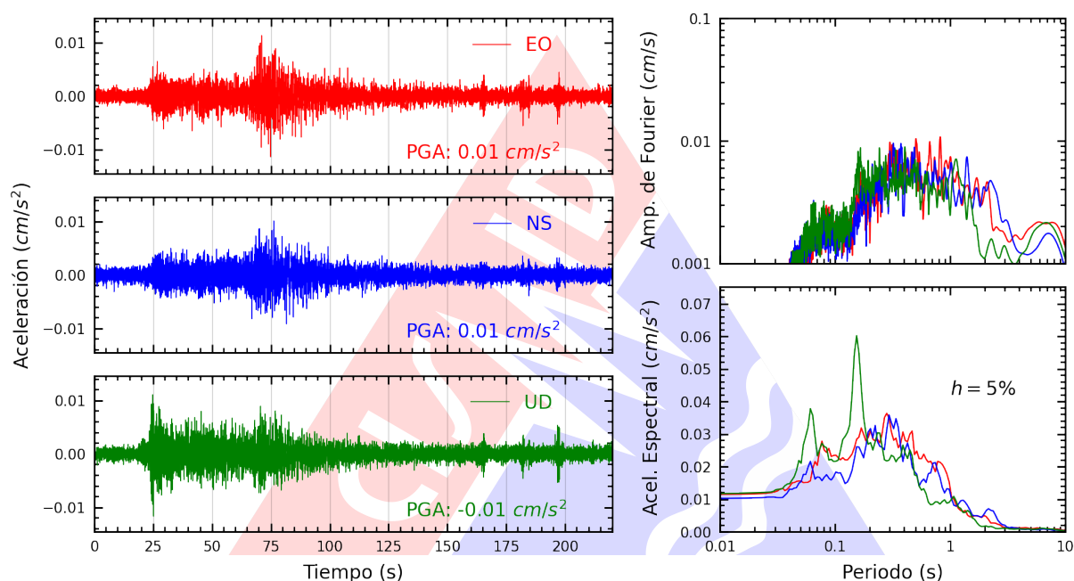
Figura A.37: Registros tiempo-historia, espectros de Fourier y de respuesta en las direcciones EO, NS y vertical de la estación UNCP. Sismo de Huaramey, Huaramey - Ancash del 2024-03-18, 01:45:50 (Hora local)
