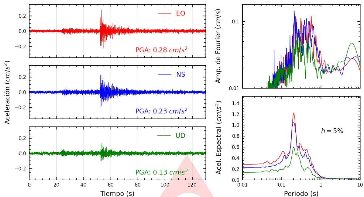
Figura A.1: Registros tiempo-historia, espectros de Fourier y de respuesta en las direcciones EO, NS y vertical de la estación UNTRM. Sismo de Lagunas, Alto Amazonas - Loreto del 2024-03-18, 18:40:55 (Hora local)
