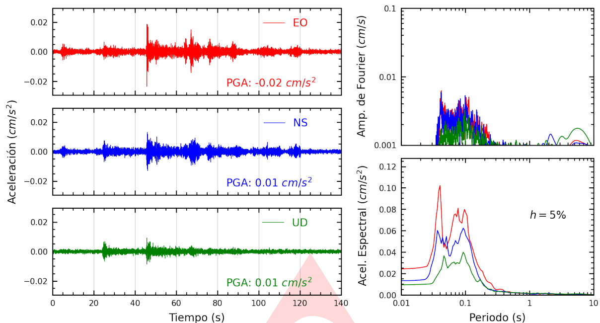
Figura A.1: Registros tiempo-historia, espectros de Fourier y de respuesta en las direcciones EO, NS y vertical de la estación UNSA. Sismo de Ichuña, General Sanchez Cerro - Moquegua del 2024-03-22, 08:04:04 (Hora local)
