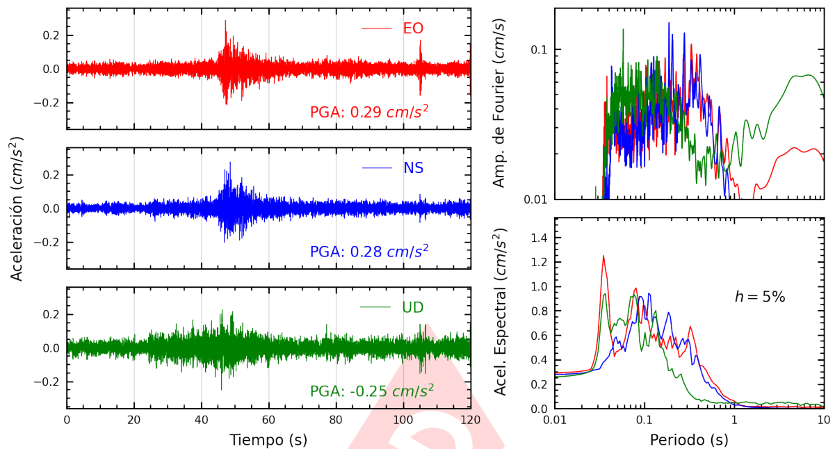
Figura A.3: Registros tiempo-historia, espectros de Fourier y de respuesta en las direcciones EO, NS y vertical de la estación SCPIU. Sismo de Zarumilla, Zarumilla - Tumbes del 2024-03-25, 10:40:01 (Hora local)
