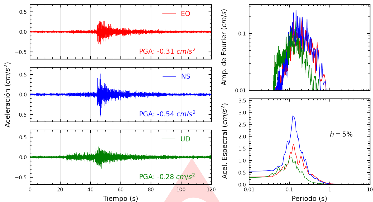
Figura A.1: Registros tiempo-historia, espectros de Fourier y de respuesta en las direcciones EO, NS y vertical de la estación UNP. Sismo de Zarumilla, Zarumilla - Tumbes del 2024-03-25, 10:40:01 (Hora local)
