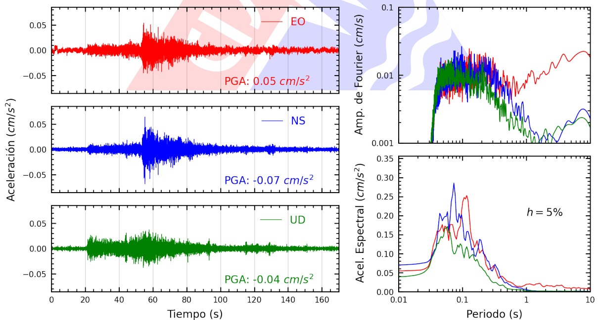
Figura A.4: Registros tiempo-historia, espectros de Fourier y de respuesta en las direcciones EO, NS y vertical de la estación SCCHI. Sismo de Zarumilla, Zarumilla - Tumbes del 2024-03-25, 10:40:01 (Hora local)
