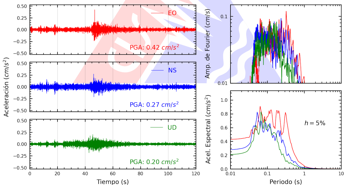
Figura A.2: Registros tiempo-historia, espectros de Fourier y de respuesta en las direcciones EO, NS y vertical de la estación UPAOP. Sismo de Zarumilla, Zarumilla - Tumbes del 2024-03-25, 10:40:01 (Hora local)
