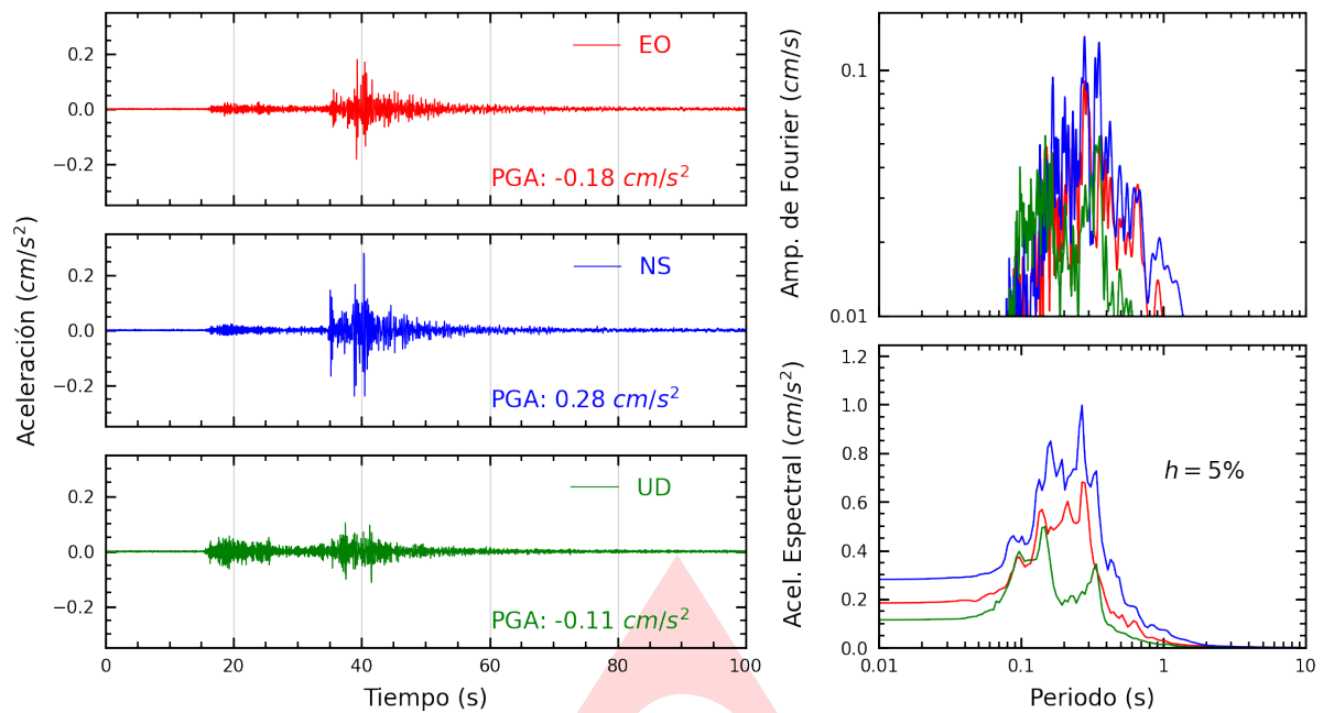
Figura A.1: Registros tiempo-historia, espectros de Fourier y de respuesta en las direcciones EO, NS y vertical de la estación UNIA. Sismo de Aguaytia, Padre Abad - Ucayali del 2024-03-28, 07:49:02 (Hora local)
