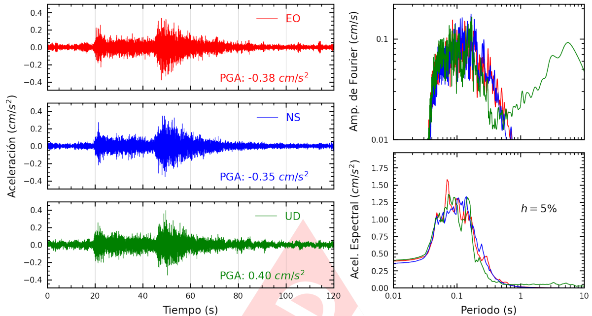
Figura A.5: Registros tiempo-historia, espectros de Fourier y de respuesta en las direcciones EO, NS y vertical de la estación SCARQ. Sismo de Tacna, Tacna - Tacna del 2024-03-29, 12:26:39 (Hora local)
