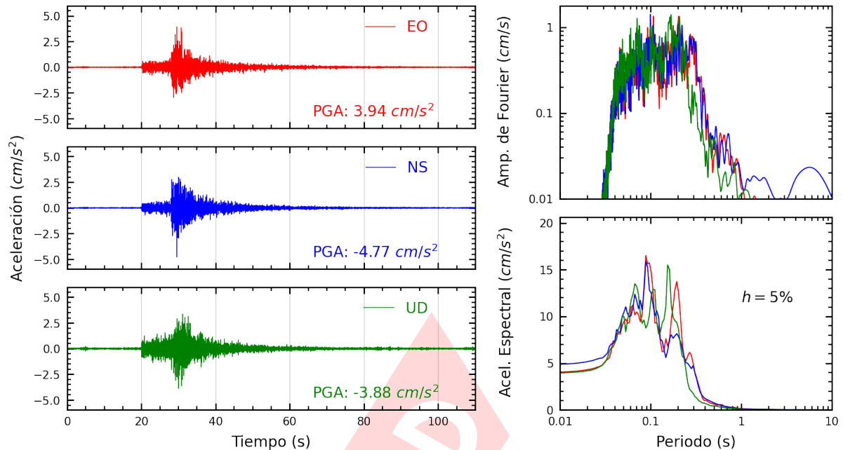
Figura A.3: Registros tiempo-historia, espectros de Fourier y de respuesta en las direcciones EO, NS y vertical de la estación SCTAC. Sismo de Tacna, Tacna - Tacna del 2024-03-29, 12:26:39 (Hora local)
