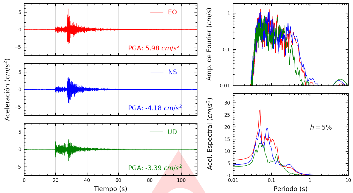
Figura A.1: Registros tiempo-historia, espectros de Fourier y de respuesta en las direcciones EO, NS y vertical de la estación CREY. Sismo de Tacna, Tacna - Tacna del 2024-03-29, 12:26:39 (Hora local)
