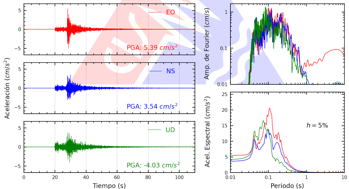
Figura A.2: Registros tiempo-historia, espectros de Fourier y de respuesta en las direcciones EO, NS y vertical de la estación UJBG3. Sismo de Tacna, Tacna - Tacna del 2024-03-29, 12:26:39 (Hora local)
