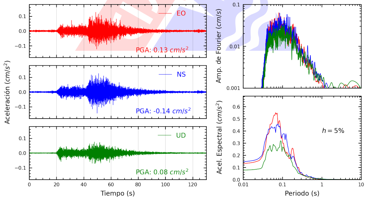
Figura A.6: Registros tiempo-historia, espectros de Fourier y de respuesta en las direcciones EO, NS y vertical de la estación UNSA. Sismo de Tacna, Tacna - Tacna del 2024-03-29, 12:26:39 (Hora local)
