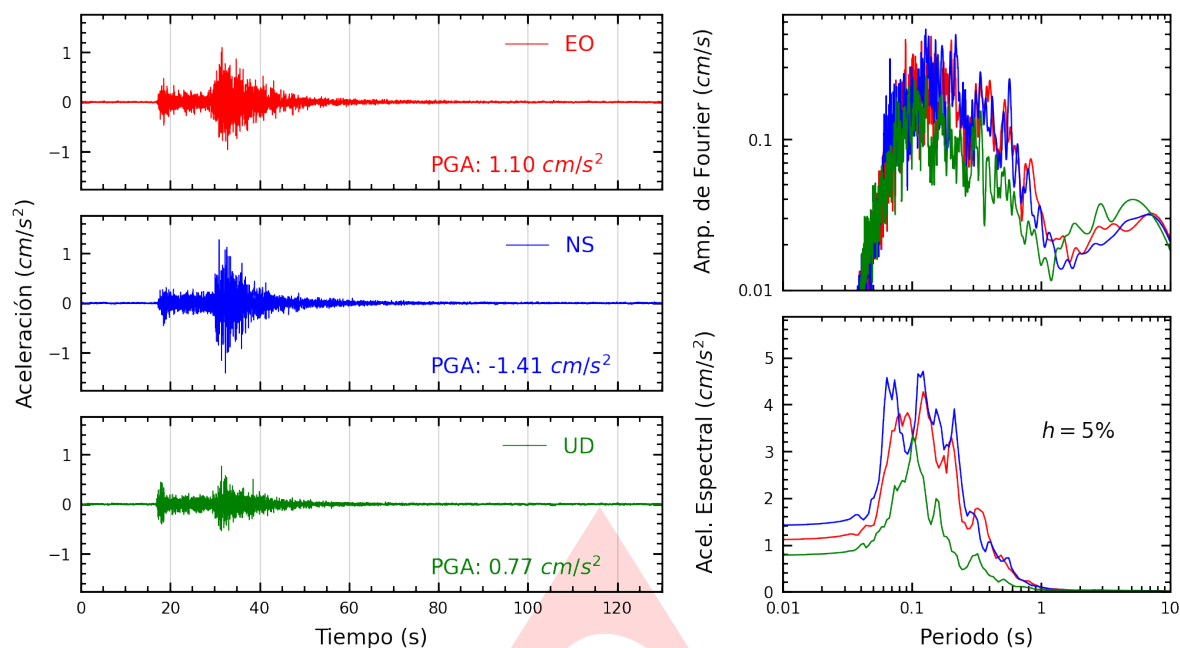
Figura A.1: Registros tiempo-historia, espectros de Fourier y de respuesta en las direcciones EO, NS y vertical de la estación UNTRM. Sismo de Jaen, Jaen - Cajamarca del 2024-03-29, 19:39:18 (Hora local)
