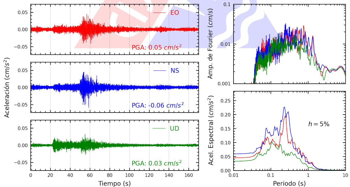
Figura A.6: Registros tiempo-historia, espectros de Fourier y de respuesta en las direcciones EO, NS y vertical de la estación UNF. Sismo de Jaen, Jaen - Cajamarca del 2024-03-29, 19:39:18 (Hora local)
