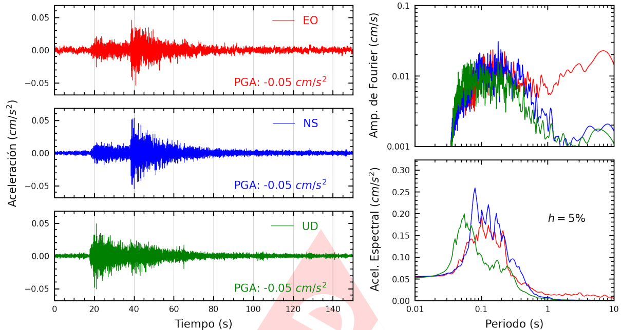
Figura A.7: Registros tiempo-historia, espectros de Fourier y de respuesta en las direcciones EO, NS y vertical de la estación SCCHI. Sismo de Jaen, Jaen - Cajamarca del 2024-03-29, 19:39:18 (Hora local)
