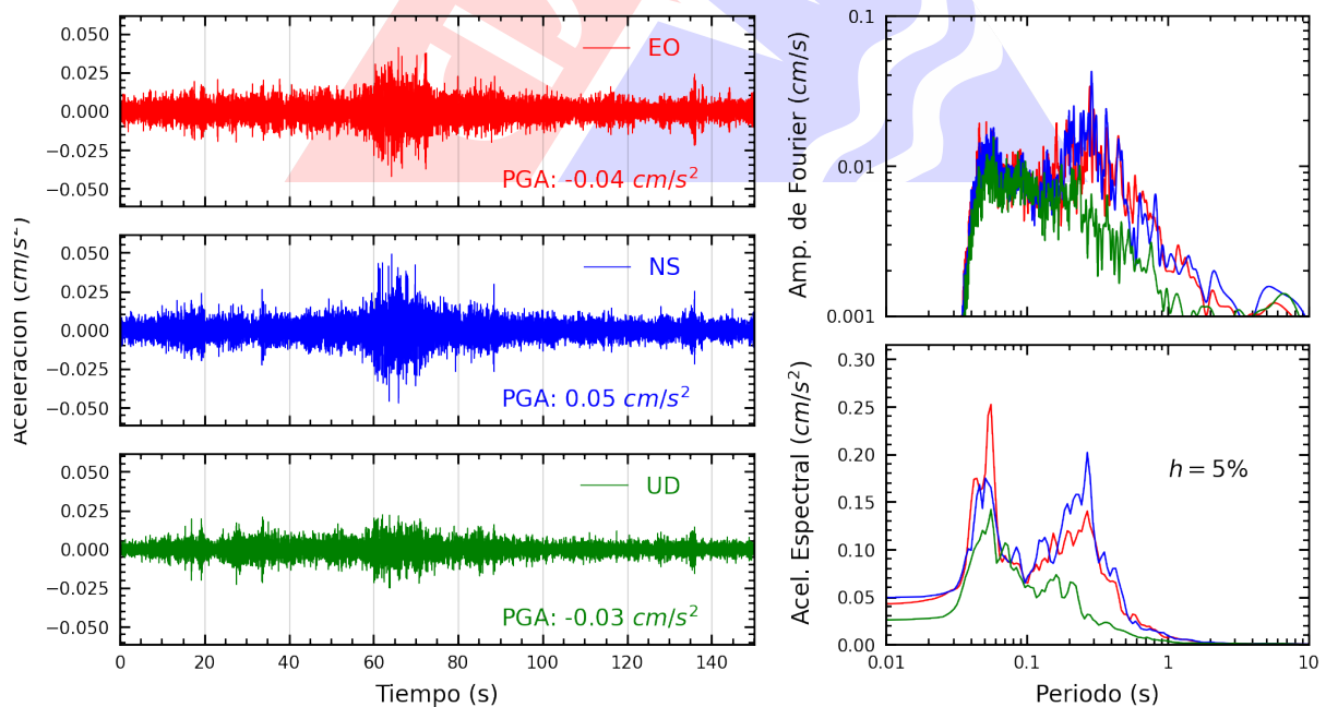
Figura A.8: Registros tiempo-historia, espectros de Fourier y de respuesta en las direcciones EO, NS y vertical de la estación UNAAA. Sismo de Jaen, Jaen - Cajamarca del 2024-03-29, 19:39:18 (Hora local)
