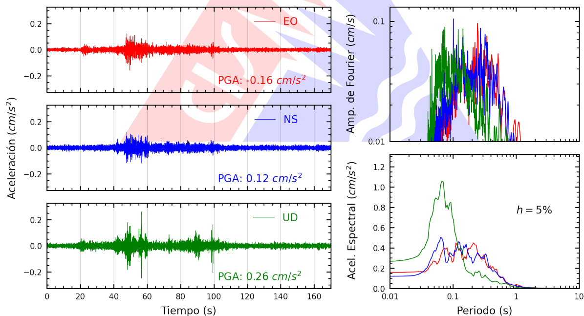
Figura A.2: Registros tiempo-historia, espectros de Fourier y de respuesta en las direcciones EO, NS y vertical de la estación UNP. Sismo de Jaen, Jaen - Cajamarca del 2024-03-29, 19:39:18 (Hora local)
