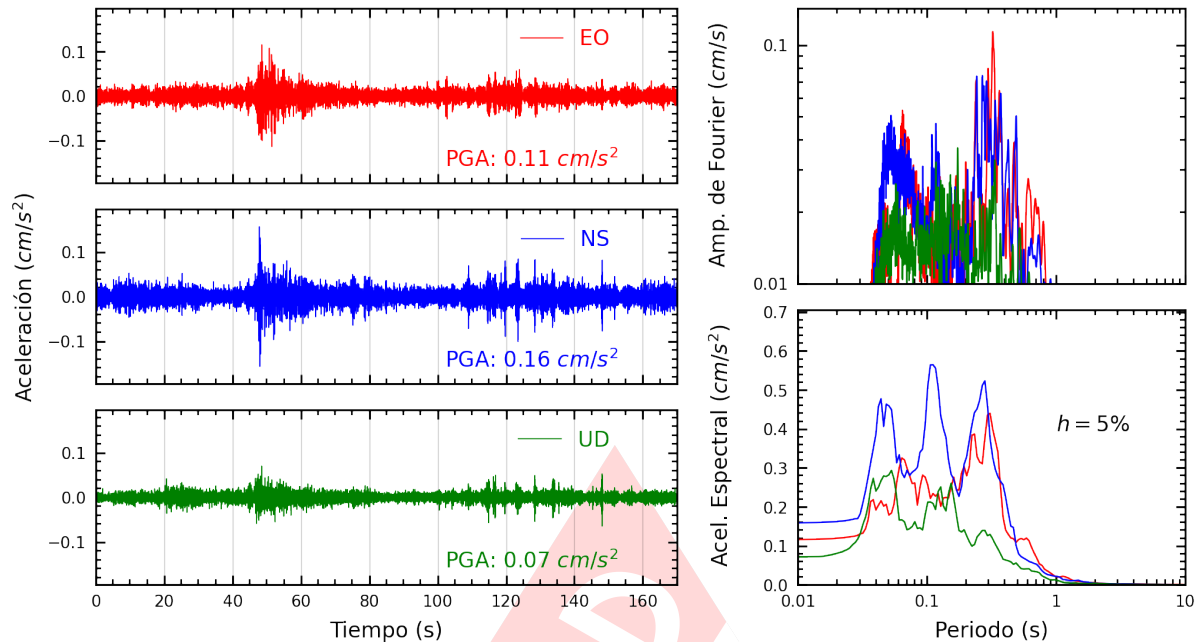
Figura A.3: Registros tiempo-historia, espectros de Fourier y de respuesta en las direcciones EO, NS y vertical de la estación UPAOP. Sismo de Jaen, Jaen - Cajamarca del 2024-03-29, 19:39:18 (Hora local)
