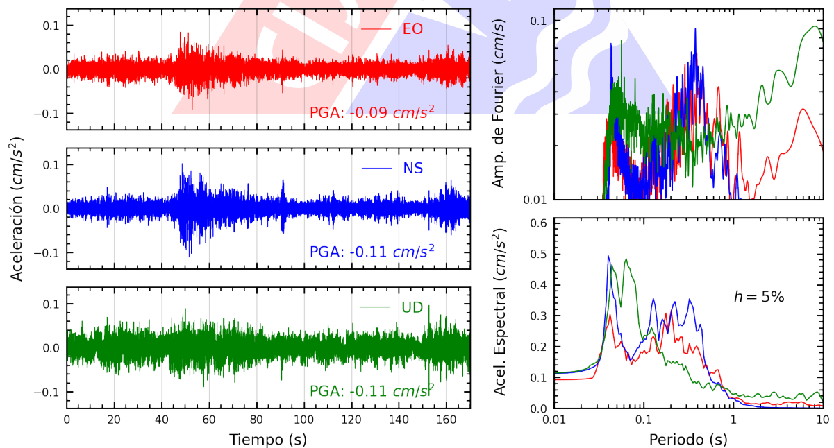
Figura A.4: Registros tiempo-historia, espectros de Fourier y de respuesta en las direcciones EO, NS y vertical de la estación SCPIU. Sismo de Jaen, Jaen - Cajamarca del 2024-03-29, 19:39:18 (Hora local)
