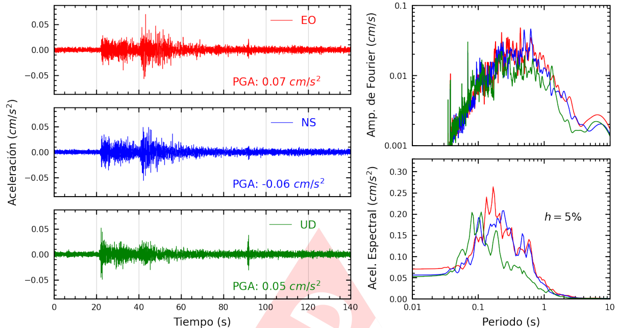
Figura A.5: Registros tiempo-historia, espectros de Fourier y de respuesta en las direcciones EO, NS y vertical de la estación UNC. Sismo de Jaen, Jaen - Cajamarca del 2024-03-29, 19:39:18 (Hora local)
