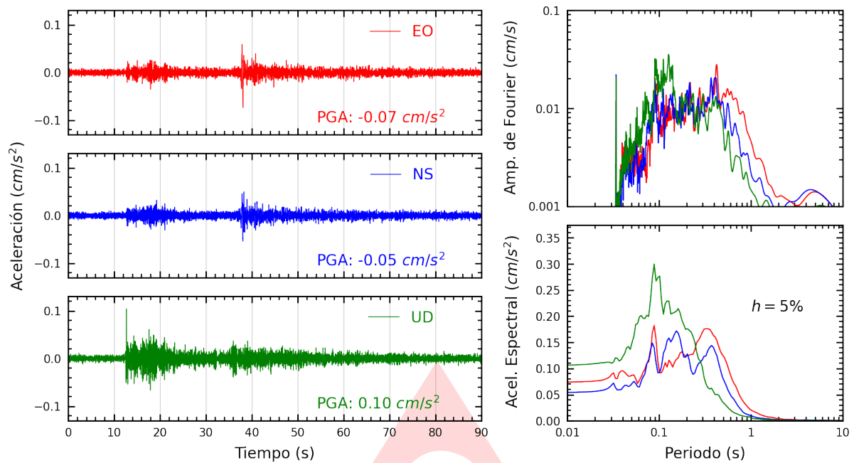
Figura A.1: Registros tiempo-historia, espectros de Fourier y de respuesta en las direcciones EO, NS y vertical de la estación UNIA. Sismo de Tocache Nuevo, Tocache - San Martín del 2024-04-12, 11:09:33 (Hora local)
