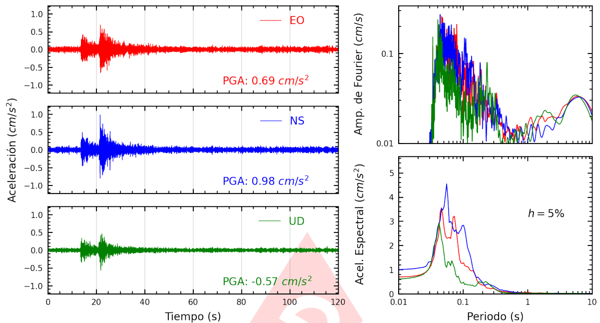
Figura A.11: Registros tiempo-historia, espectros de Fourier y de respuesta en las direcciones EO, NS y vertical de la estación UPCVI. Sismo de Chilca, Cañete - Lima del 2024-05-02, 18:09:51 (Hora local)
