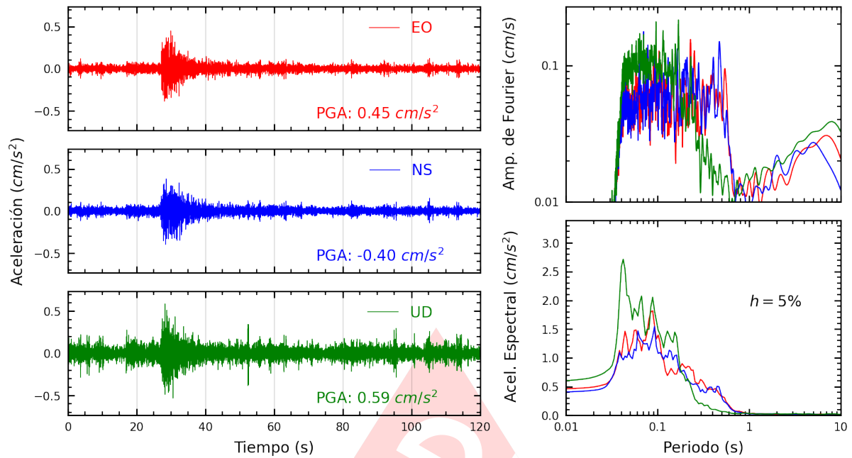
Figura A.21: Registros tiempo-historia, espectros de Fourier y de respuesta en las direcciones EO, NS y vertical de la estación MDPP. Sismo de Chilca, Cañete - Lima del 2024-05-02, 18:09:51 (Hora local)
