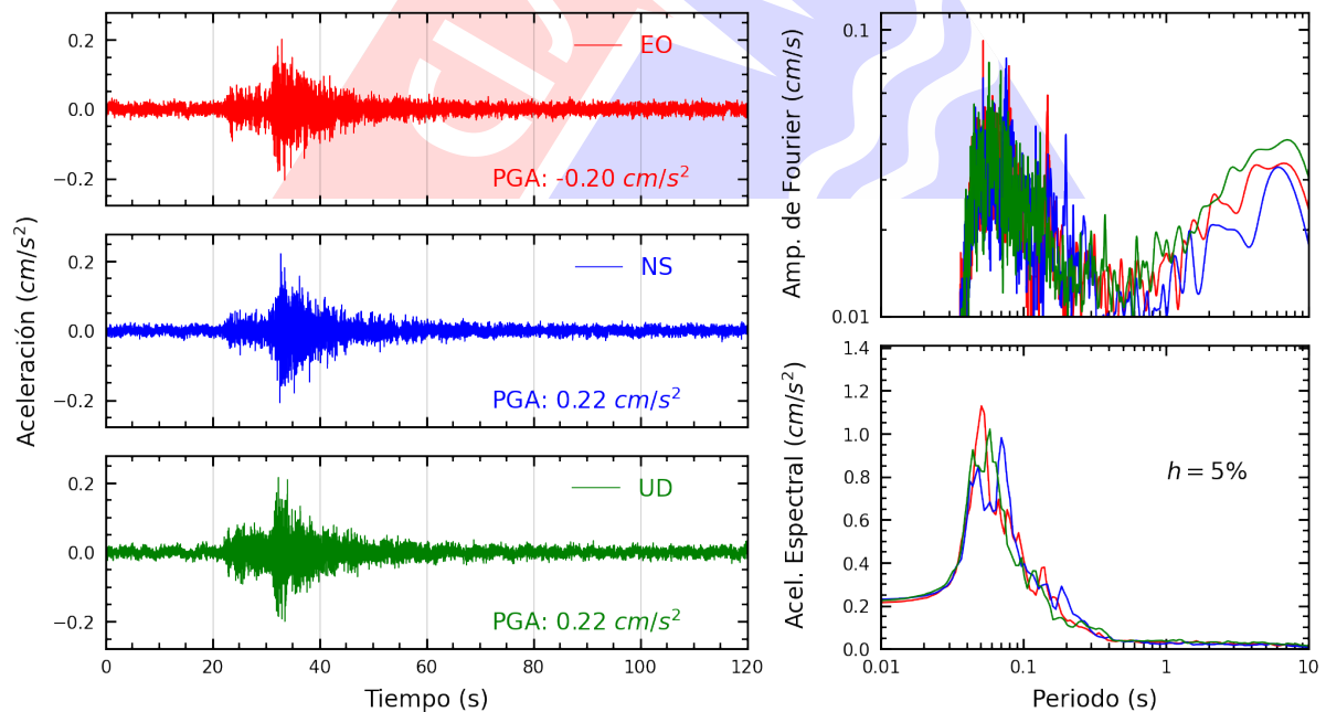
Figura A.28: Registros tiempo-historia, espectros de Fourier y de respuesta en las direcciones EO, NS y vertical de la estación UNMSM. Sismo de Chilca, Cañete - Lima del 2024-05-02, 18:09:51 (Hora local)
