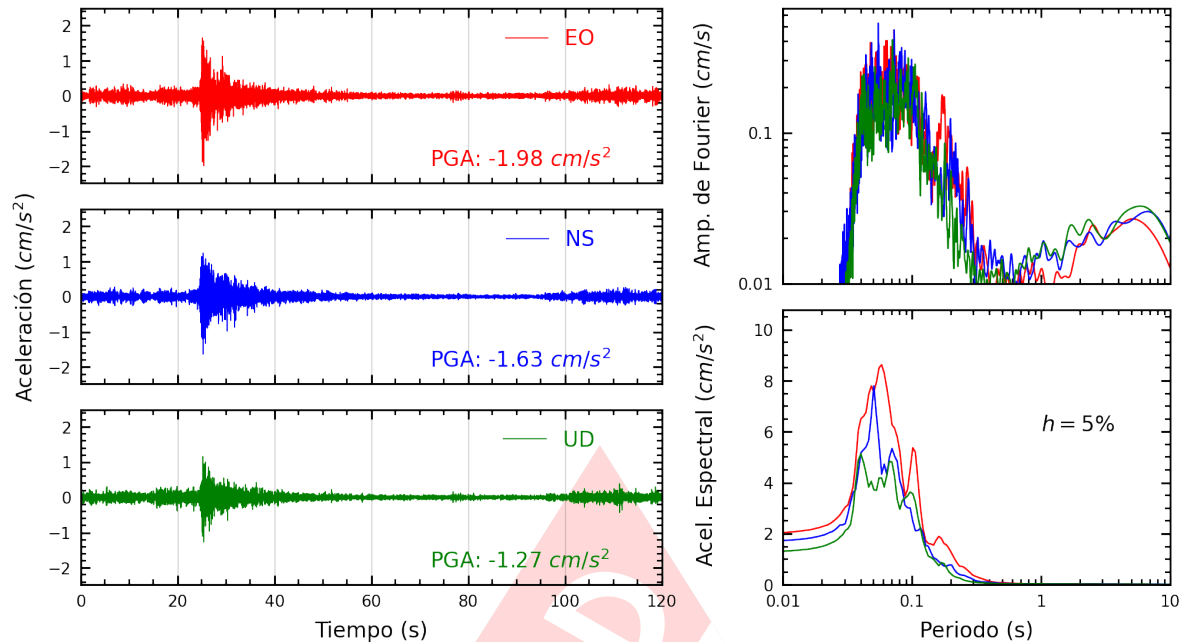
Figura A.5: Registros tiempo-historia, espectros de Fourier y de respuesta en las direcciones EO, NS y vertical de la estación INDEP. Sismo de Chilca, Cañete - Lima del 2024-05-02, 18:09:51 (Hora local)
