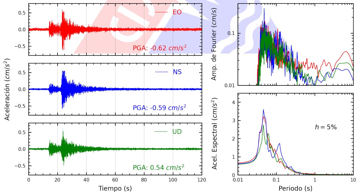
Figura A.20: Registros tiempo-historia, espectros de Fourier y de respuesta en las direcciones EO, NS y vertical de la estación IMCA. Sismo de Chilca, Cañete - Lima del 2024-05-02, 18:09:51 (Hora local)
