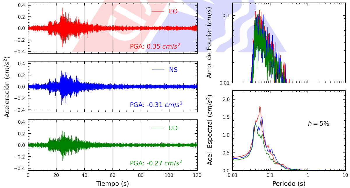
Figura A.26: Registros tiempo-historia, espectros de Fourier y de respuesta en las direcciones EO, NS y vertical de la estación BORJA. Sismo de Chilca, Cañete - Lima del 2024-05-02, 18:09:51 (Hora local)
