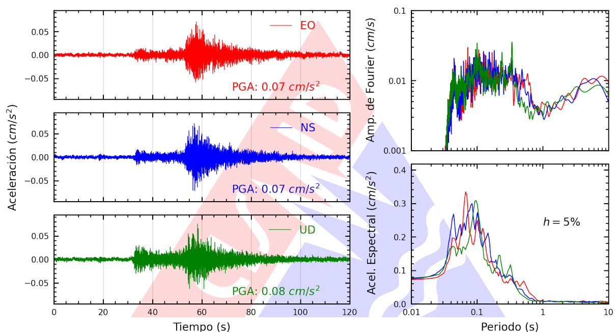
Figura A.29: Registros tiempo-historia, espectros de Fourier y de respuesta en las direcciones EO, NS y vertical de la estación CARAL. Sismo de Chilca, Cañete - Lima del 2024-05-02, 18:09:51 (Hora local)
