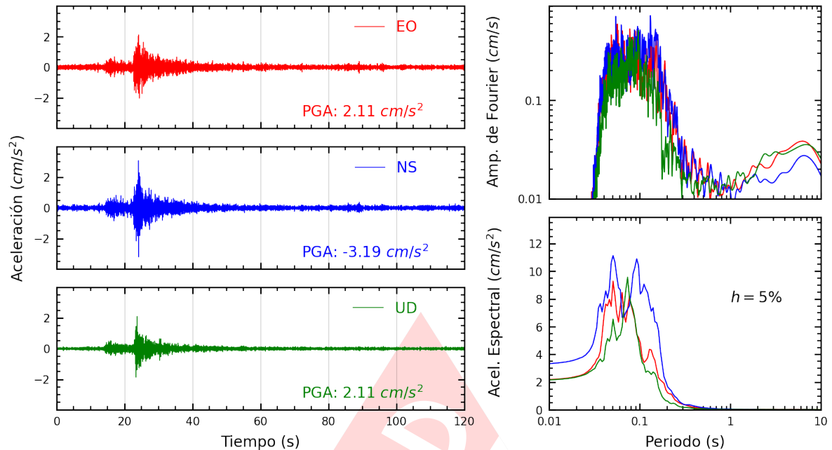
Figura A.3: Registros tiempo-historia, espectros de Fourier y de respuesta en las direcciones EO, NS y vertical de la estación USILM. Sismo de Chilca, Cañete - Lima del 2024-05-02, 18:09:51 (Hora local)
