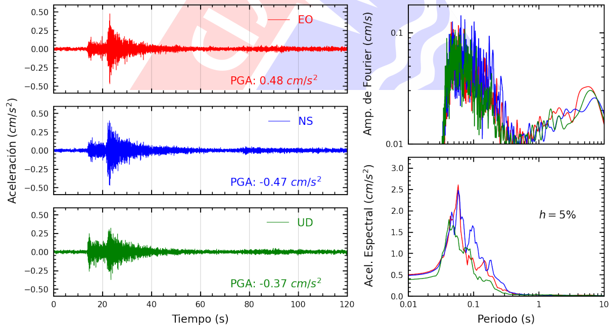
Figura A.24: Registros tiempo-historia, espectros de Fourier y de respuesta en las direcciones EO, NS y vertical de la estación SERVI. Sismo de Chilca, Cañete - Lima del 2024-05-02, 18:09:51 (Hora local)
