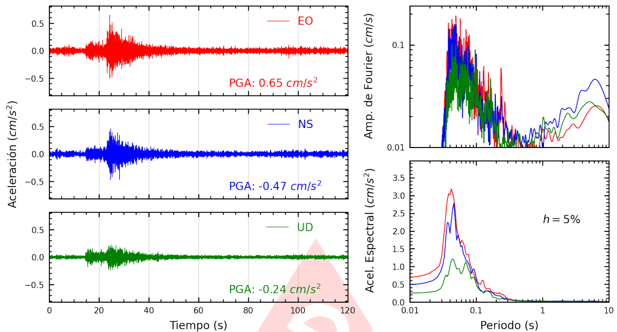
Figura A.19: Registros tiempo-historia, espectros de Fourier y de respuesta en las direcciones EO, NS y vertical de la estación CEPRE. Sismo de Chilca, Cañete - Lima del 2024-05-02, 18:09:51 (Hora local)
