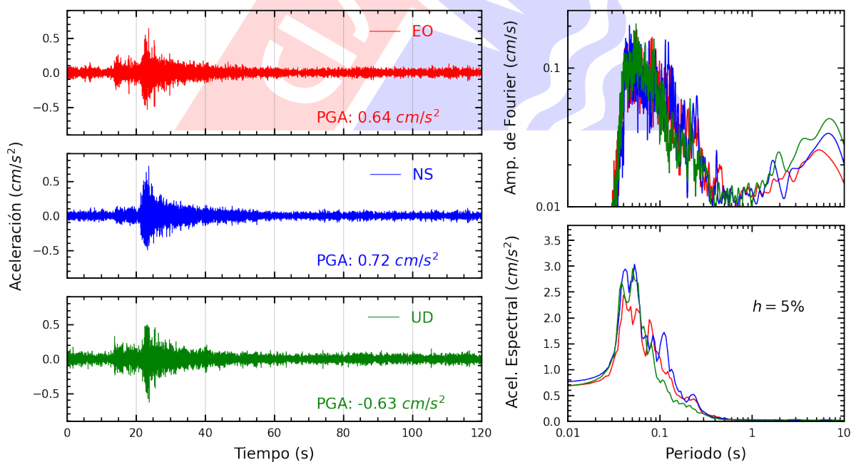
Figura A.16: Registros tiempo-historia, espectros de Fourier y de respuesta en las direcciones EO, NS y vertical de la estación URPPE. Sismo de Chilca, Cañete - Lima del 2024-05-02, 18:09:51 (Hora local)
