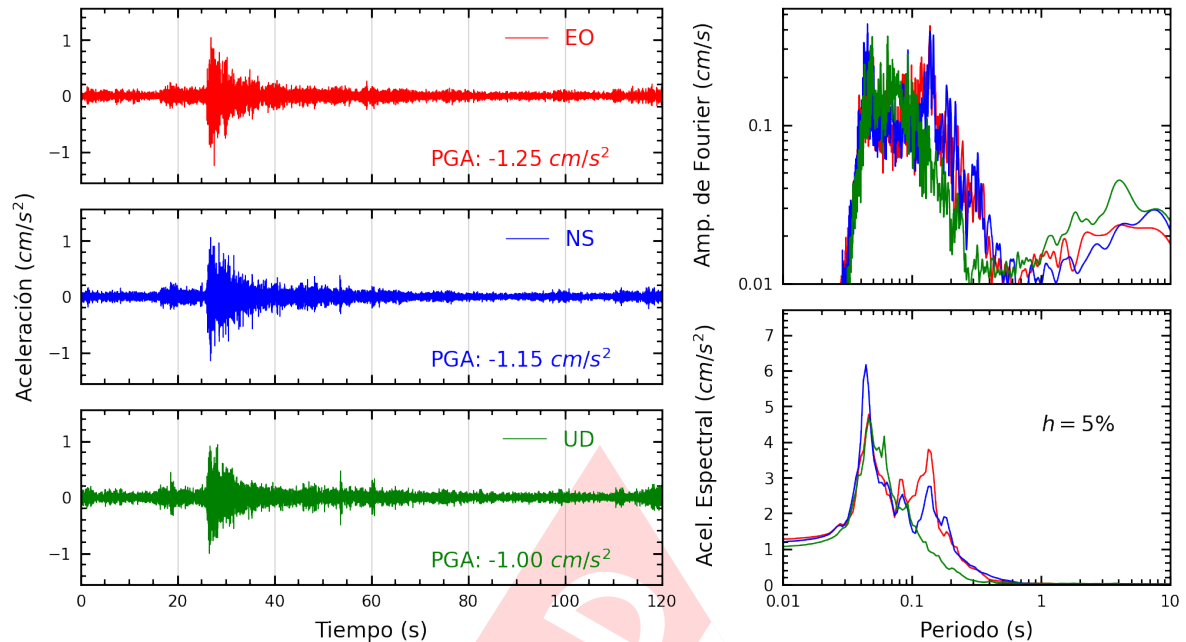
Figura A.7: Registros tiempo-historia, espectros de Fourier y de respuesta en las direcciones EO, NS y vertical de la estación CARAB. Sismo de Chilca, Cañete - Lima del 2024-05-02, 18:09:51 (Hora local)
