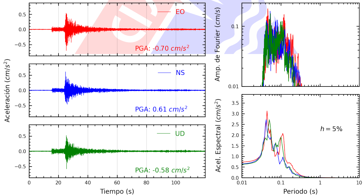
Figura A.18: Registros tiempo-historia, espectros de Fourier y de respuesta en las direcciones EO, NS y vertical de la estación JALV2. Sismo de Chilca, Cañete - Lima del 2024-05-02, 18:09:51 (Hora local)
