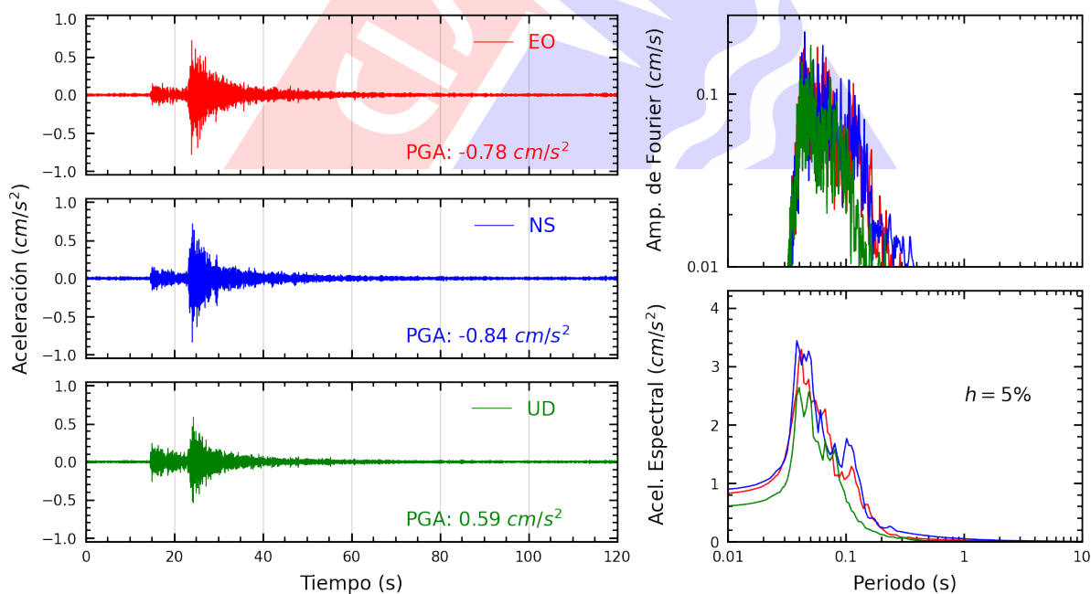
Figura A.14: Registros tiempo-historia, espectros de Fourier y de respuesta en las direcciones EO, NS y vertical de la estación ATARJ. Sismo de Chilca, Cañete - Lima del 2024-05-02, 18:09:51 (Hora local)
