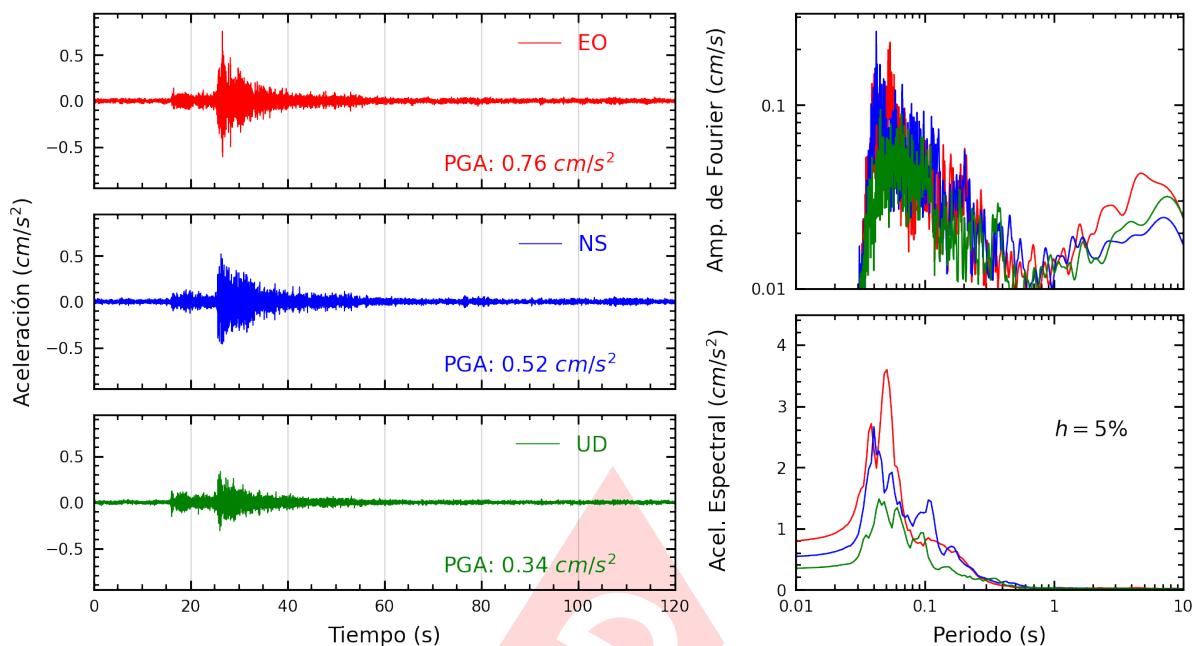
Figura A.15: Registros tiempo-historia, espectros de Fourier y de respuesta en las direcciones EO, NS y vertical de la estación COMAS. Sismo de Chilca, Cañete - Lima del 2024-05-02, 18:09:51 (Hora local)
