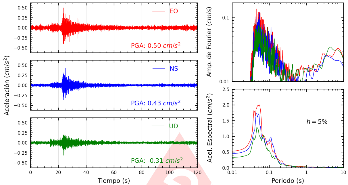
Figura A.23: Registros tiempo-historia, espectros de Fourier y de respuesta en las direcciones EO, NS y vertical de la estación INICT. Sismo de Chilca, Cañete - Lima del 2024-05-02, 18:09:51 (Hora local)
