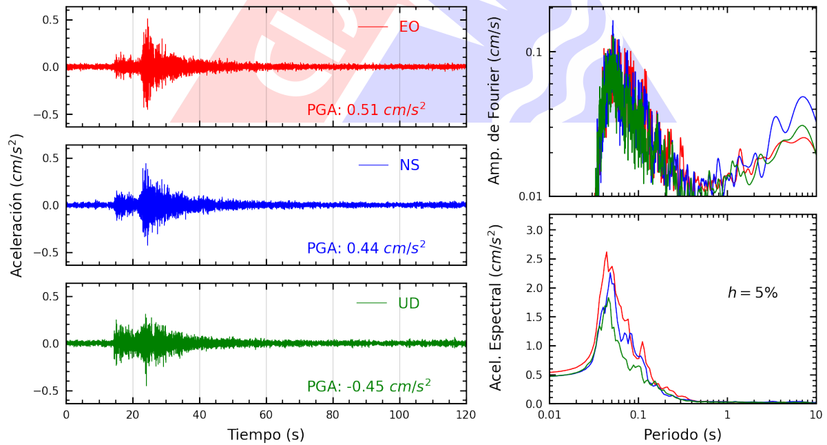
Figura A.22: Registros tiempo-historia, espectros de Fourier y de respuesta en las direcciones EO, NS y vertical de la estación CENEP. Sismo de Chilca, Cañete - Lima del 2024-05-02, 18:09:51 (Hora local)
