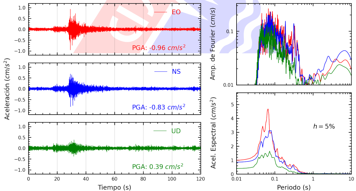
Figura A.12: Registros tiempo-historia, espectros de Fourier y de respuesta en las direcciones EO, NS y vertical de la estación DEFEN. Sismo de Chilca, Cañete - Lima del 2024-05-02, 18:09:51 (Hora local)
