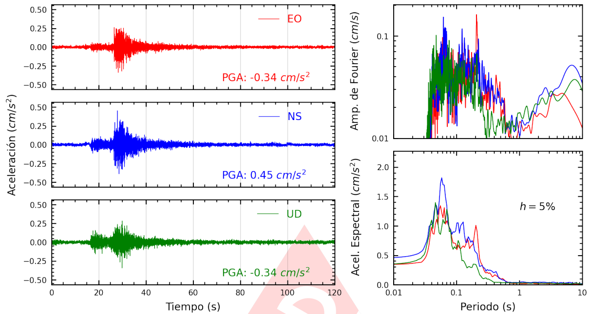
Figura A.25: Registros tiempo-historia, espectros de Fourier y de respuesta en las direcciones EO, NS y vertical de la estación VHAYA. Sismo de Chilca, Cañete - Lima del 2024-05-02, 18:09:51 (Hora local)
