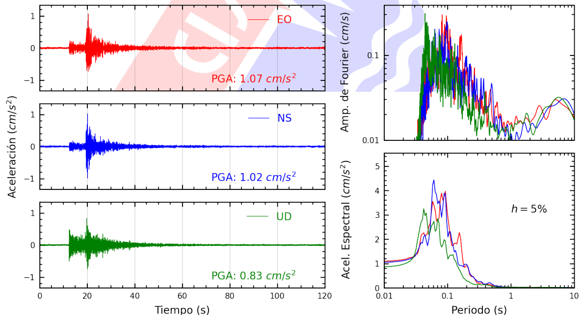
Figura A.10: Registros tiempo-historia, espectros de Fourier y de respuesta en las direcciones EO, NS y vertical de la estación USILP. Sismo de Chilca, Cañete - Lima del 2024-05-02, 18:09:51 (Hora local)
