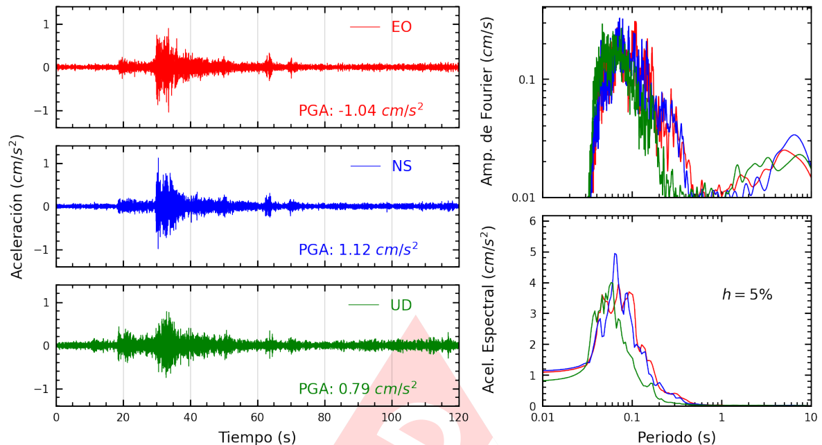
Figura A.9: Registros tiempo-historia, espectros de Fourier y de respuesta en las direcciones EO, NS y vertical de la estación ANCON. Sismo de Chilca, Cañete - Lima del 2024-05-02, 18:09:51 (Hora local)
