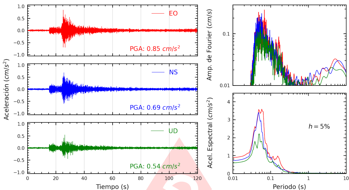
Figura A.13: Registros tiempo-historia, espectros de Fourier y de respuesta en las direcciones EO, NS y vertical de la estación FICPE. Sismo de Chilca, Cañete - Lima del 2024-05-02, 18:09:51 (Hora local)
