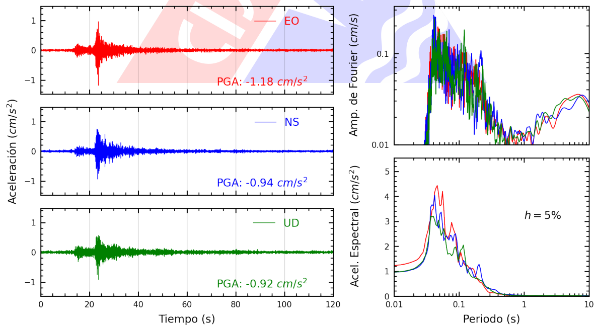
Figura A.8: Registros tiempo-historia, espectros de Fourier y de respuesta en las direcciones EO, NS y vertical de la estación USMP. Sismo de Chilca, Cañete - Lima del 2024-05-02, 18:09:51 (Hora local)
