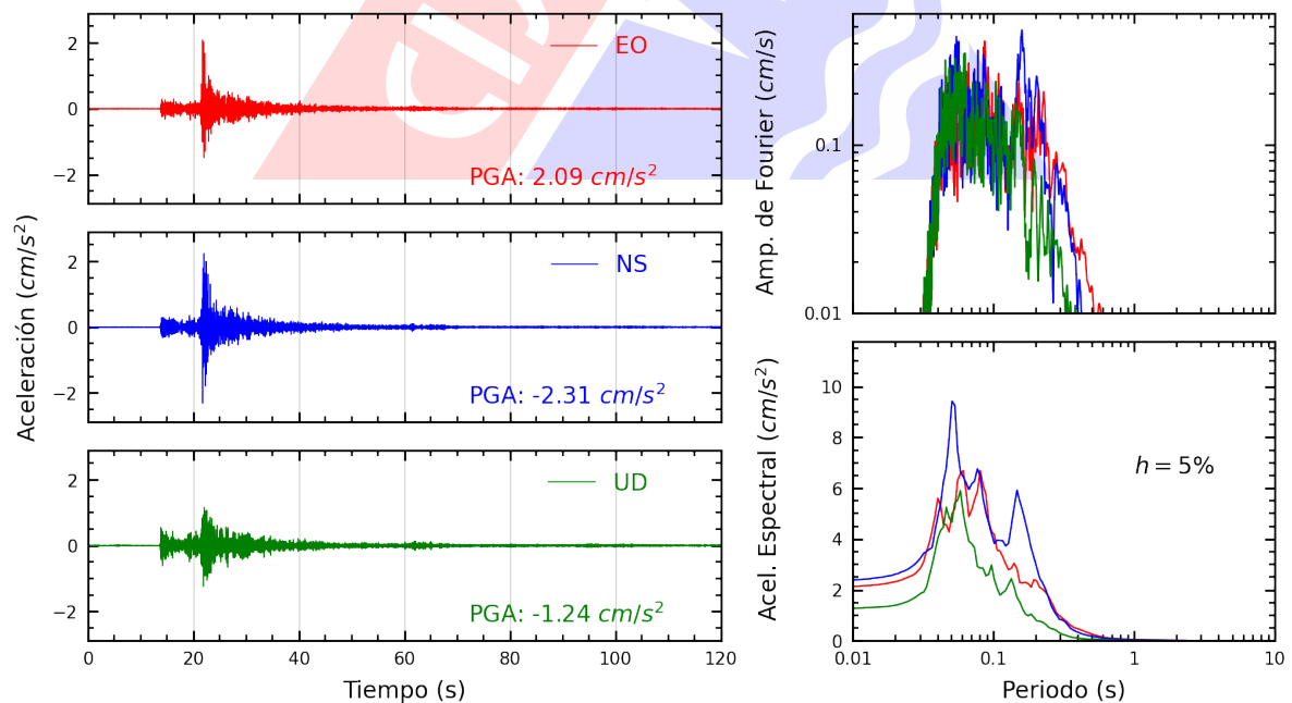
Figura A.4: Registros tiempo-historia, espectros de Fourier y de respuesta en las direcciones EO, NS y vertical de la estación ASIA. Sismo de Chilca, Cañete - Lima del 2024-05-02, 18:09:51 (Hora local)
