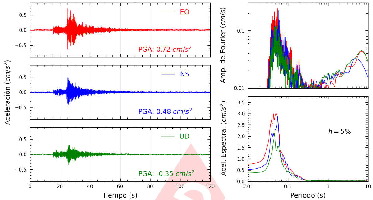
Figura A.17: Registros tiempo-historia, espectros de Fourier y de respuesta en las direcciones EO, NS y vertical de la estación UCSS. Sismo de Chilca, Cañete - Lima del 2024-05-02, 18:09:51 (Hora local)
