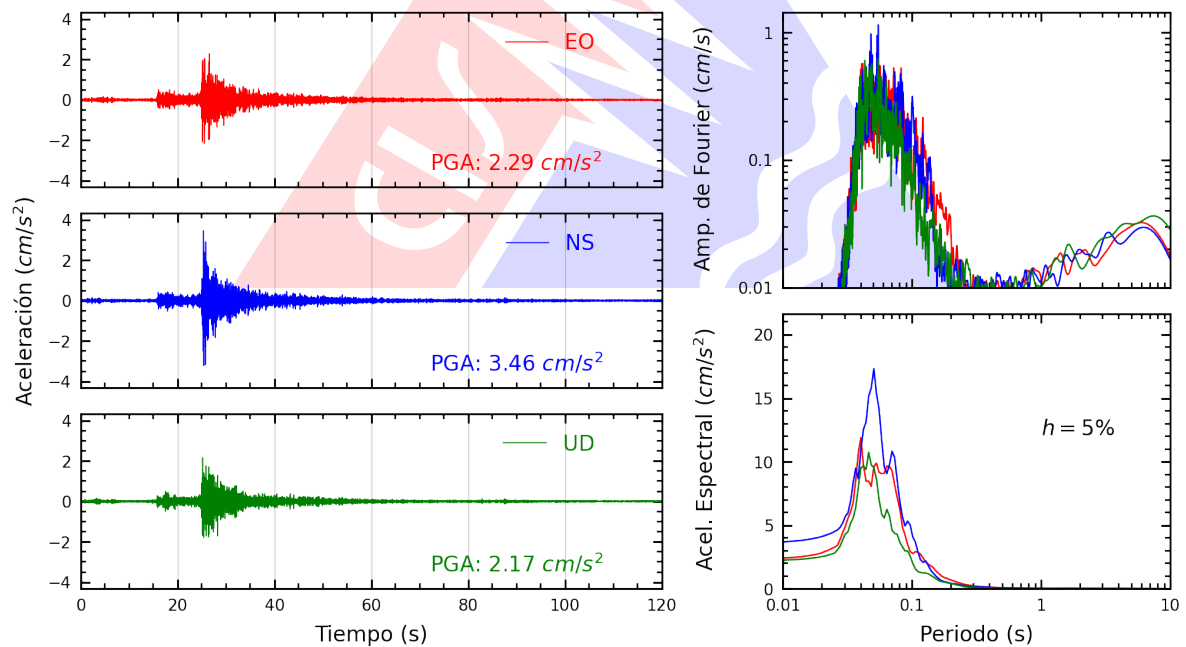
Figura A.2: Registros tiempo-historia, espectros de Fourier y de respuesta en las direcciones EO, NS y vertical de la estación JOSEO. Sismo de Chilca, Cañete - Lima del 2024-05-02, 18:09:51 (Hora local)
