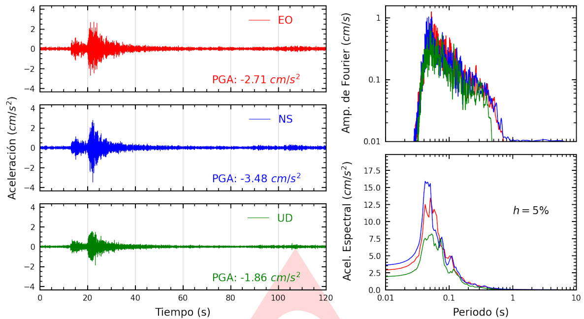
Figura A.1: Registros tiempo-historia, espectros de Fourier y de respuesta en las direcciones EO, NS y vertical de la estación UNTEL. Sismo de Chilca, Cañete - Lima del 2024-05-02, 18:09:51 (Hora local)
