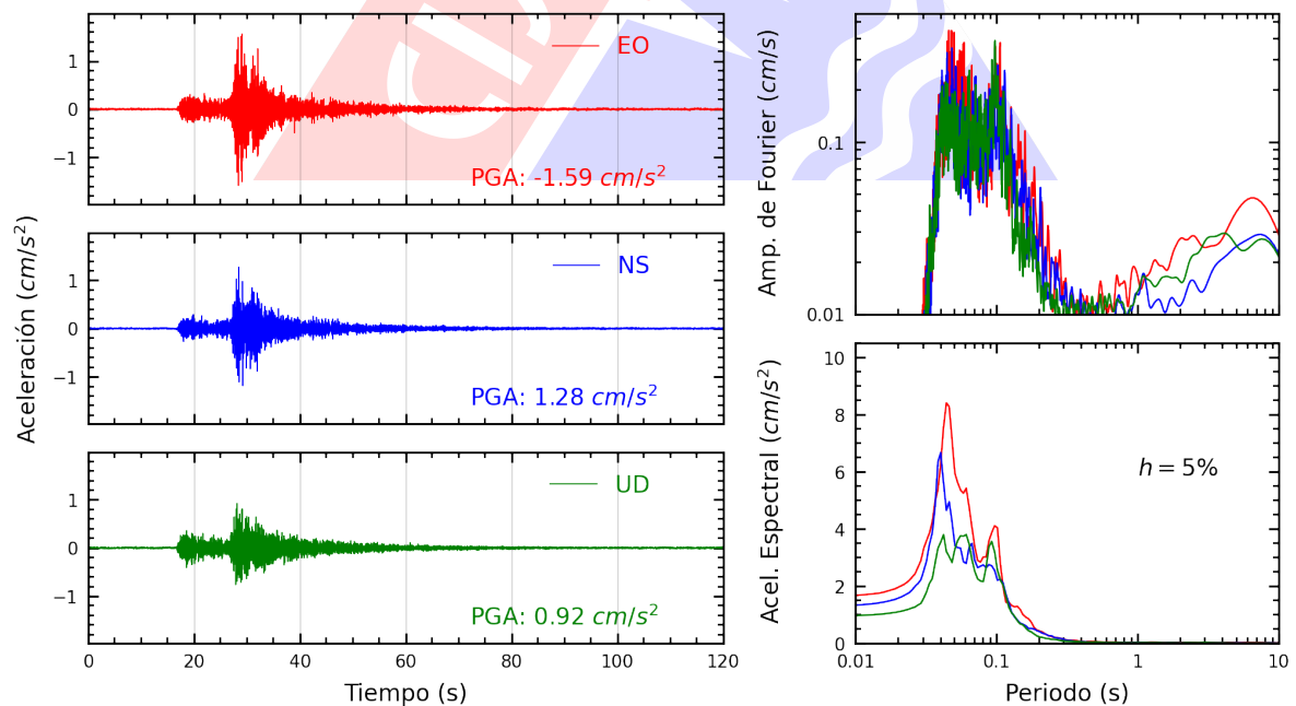
Figura A.6: Registros tiempo-historia, espectros de Fourier y de respuesta en las direcciones EO, NS y vertical de la estación AMORE. Sismo de Chilca, Cañete - Lima del 2024-05-02, 18:09:51 (Hora local)
