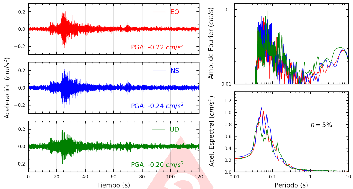
Figura A.27: Registros tiempo-historia, espectros de Fourier y de respuesta en las direcciones EO, NS y vertical de la estación UNFV. Sismo de Chilca, Cañete - Lima del 2024-05-02, 18:09:51 (Hora local)
