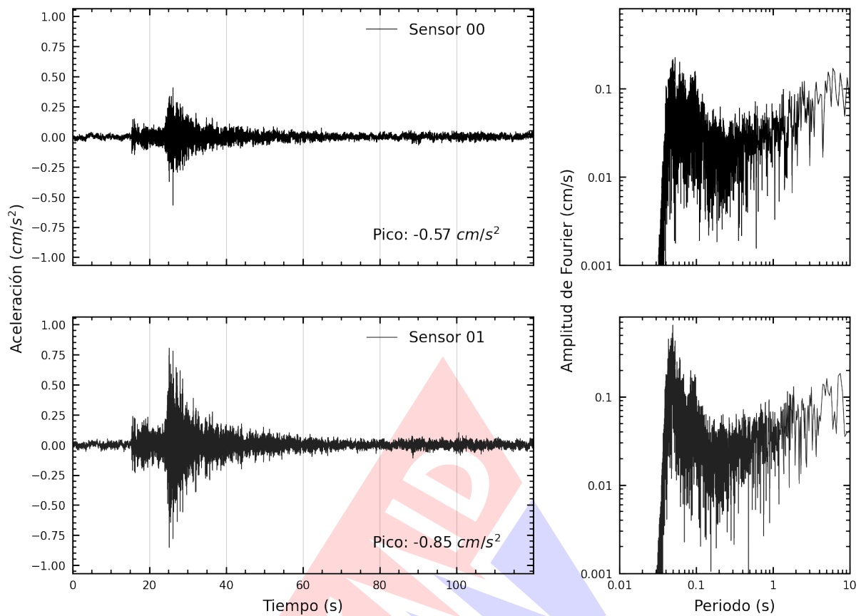
Figura A.3: Registros tiempo-historia y espectros de Fourier en la dirección vertical de la edificación Laboratorio de Estructuras del CISMID-FIC-UNI. Sismo de Chilca, Cañete - Lima del 2024-05-02, 18:09:51 (Hora local)
