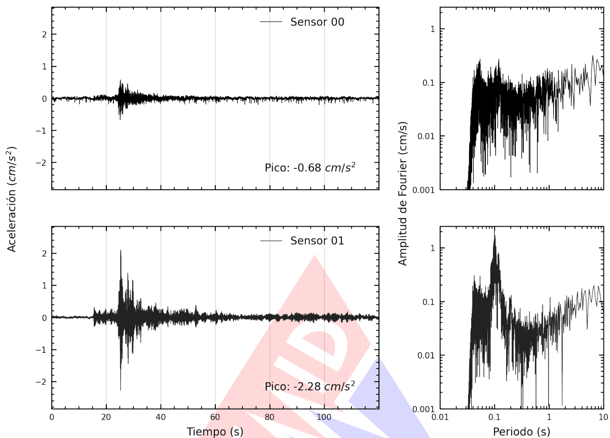
Figura A.1: Registros tiempo-historia y espectros de Fourier en la dirección EW de la edificación Laboratorio de Estructuras del CISMID-FIC-UNI. Sismo de Chilca, Cañete - Lima del 2024-05-02, 18:09:51 (Hora local)
