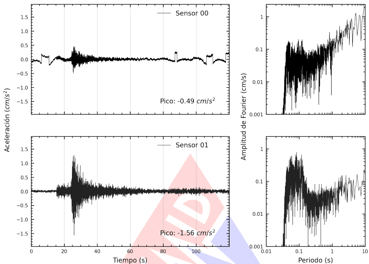
Figura A.2: Registros tiempo-historia y espectros de Fourier en la dirección NS de la edificación Laboratorio de Estructuras del CISMID-FIC-UNI. Sismo de Chilca, Cañete - Lima del 2024-05-02, 18:09:51 (Hora local)
