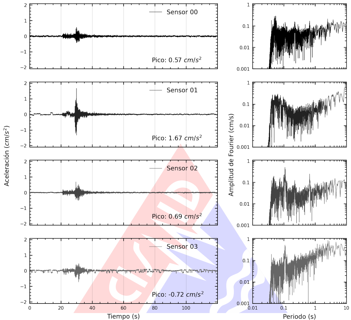
Figura A.1: Registros tiempo-historia y espectros de Fourier en la dirección EW de la edificación Centro de Información e Investigación de la FIC-UNI. Sismo de Provincia Constitucional del Callao , Callao - Lima del 2024-05-04, 22:17:27 (Hora local)
