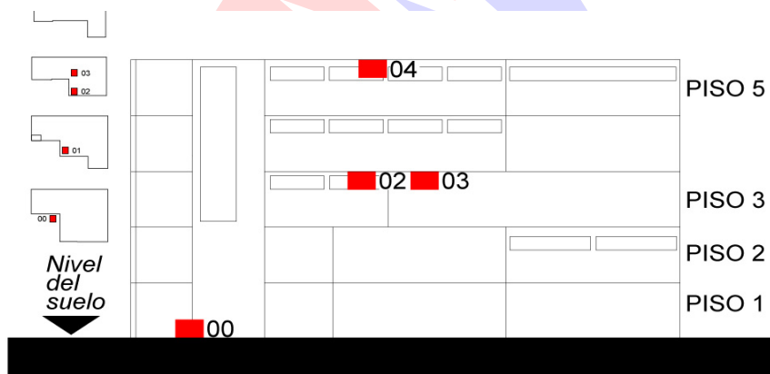
Figura 4: Distribución de sensores en la edificación monitoreada
