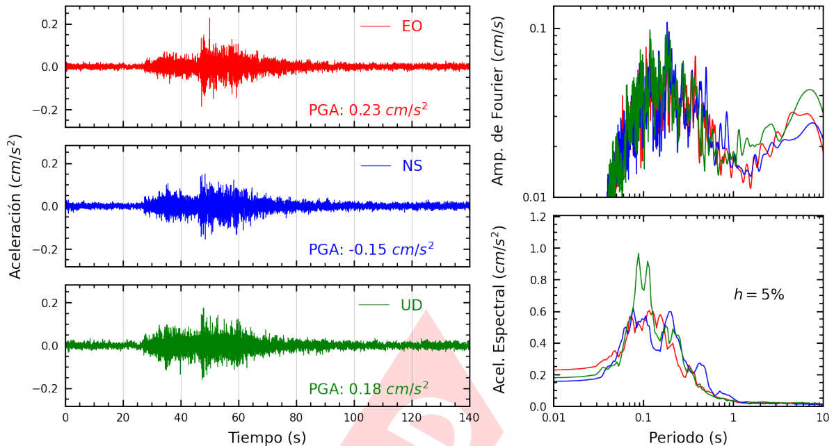
Figura A.17: Registros tiempo-historia, espectros de Fourier y de respuesta en las direcciones EO, NS y vertical de la estación UNFV. Sismo de Pisco, Pisco - Ica del 2024-05-05, 03:18:19 (Hora local)
