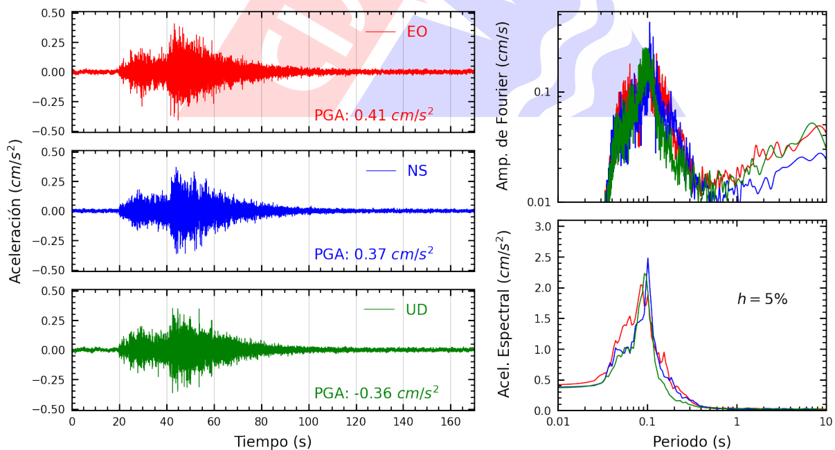
Figura A.10: Registros tiempo-historia, espectros de Fourier y de respuesta en las direcciones EO, NS y vertical de la estación AMORE. Sismo de Pisco, Pisco - Ica del 2024-05-05, 03:18:19 (Hora local)
