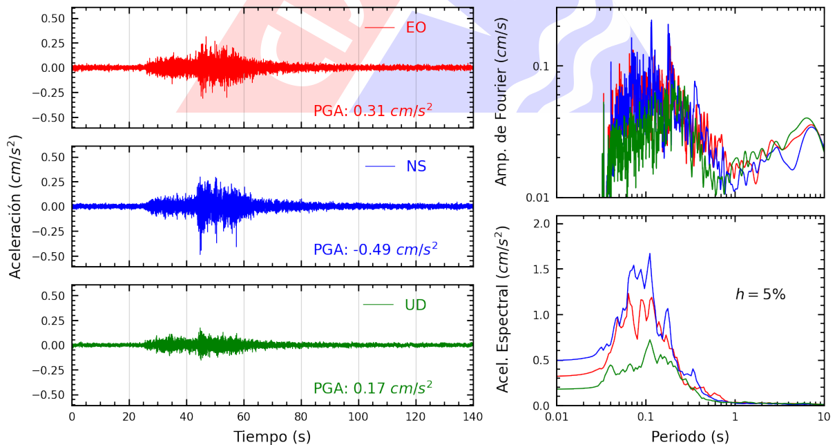
Figura A.8: Registros tiempo-historia, espectros de Fourier y de respuesta en las direcciones EO, NS y vertical de la estación UPCVI. Sismo de Pisco, Pisco - Ica del 2024-05-05, 03:18:19 (Hora local)
