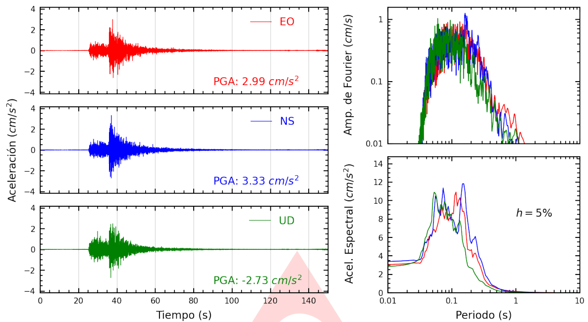
Figura A.1: Registros tiempo-historia, espectros de Fourier y de respuesta en las direcciones EO, NS y vertical de la estación ASIA. Sismo de Pisco, Pisco - Ica del 2024-05-05, 03:18:19 (Hora local)
