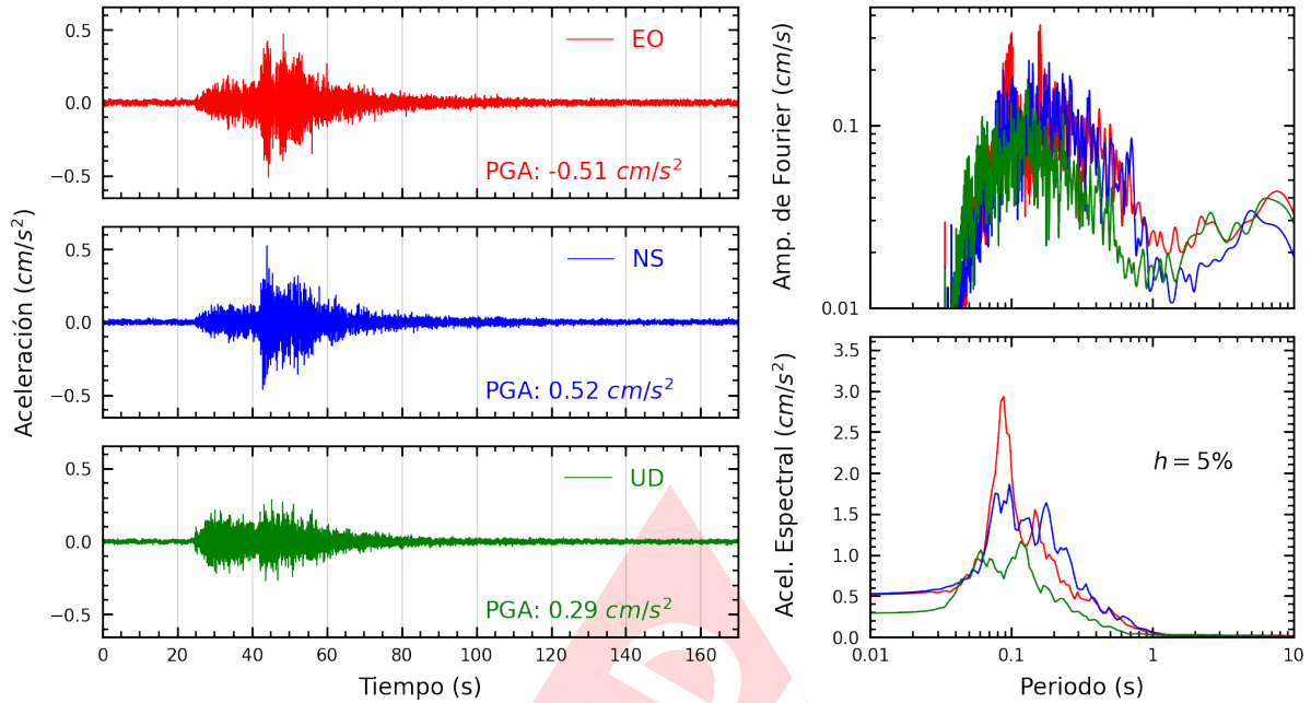
Figura A.7: Registros tiempo-historia, espectros de Fourier y de respuesta en las direcciones EO, NS y vertical de la estación USILP. Sismo de Pisco, Pisco - Ica del 2024-05-05, 03:18:19 (Hora local)
