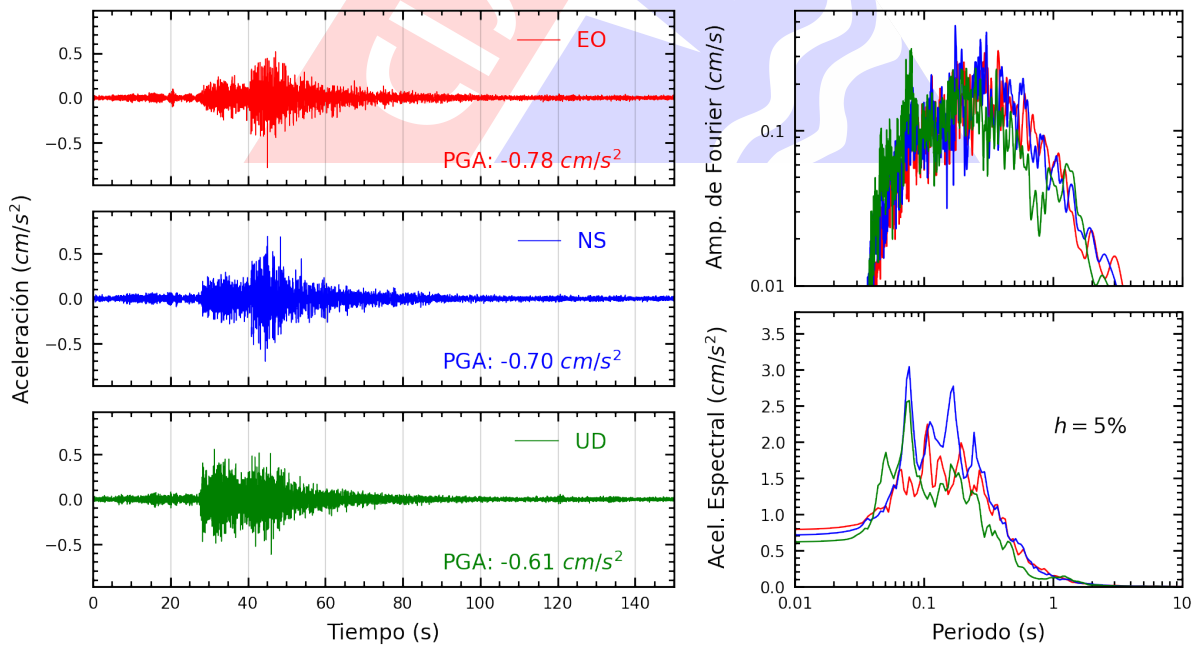
Figura A.4: Registros tiempo-historia, espectros de Fourier y de respuesta en las direcciones EO, NS y vertical de la estación UNICA. Sismo de Pisco, Pisco - Ica del 2024-05-05, 03:18:19 (Hora local)
