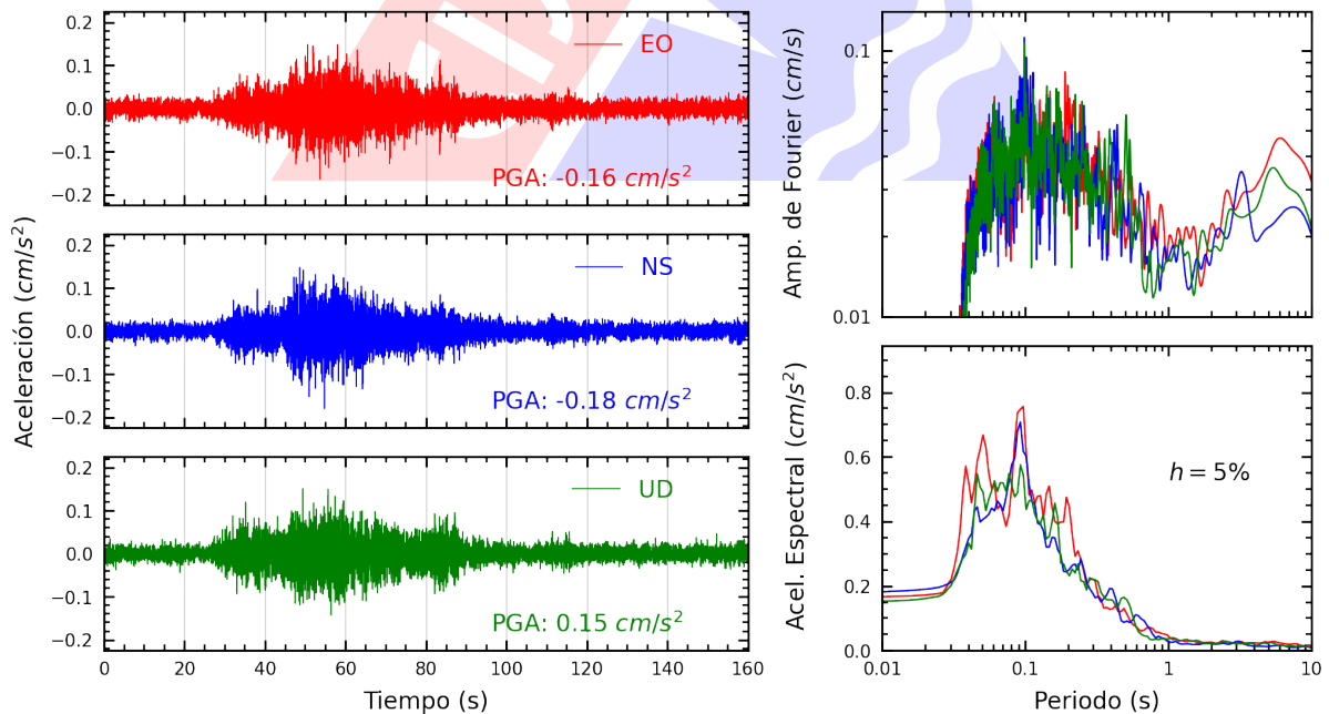
Figura A.22: Registros tiempo-historia, espectros de Fourier y de respuesta en las direcciones EO, NS y vertical de la estación IMCA. Sismo de Pisco, Pisco - Ica del 2024-05-05, 03:18:19 (Hora local)
