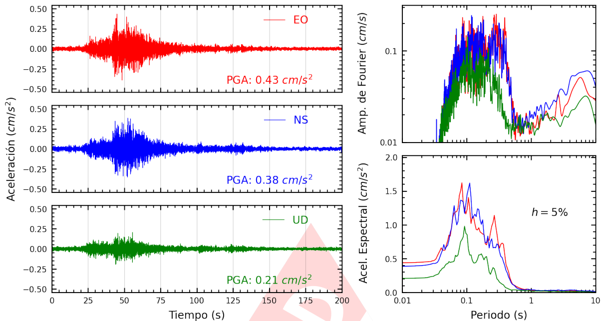
Figura A.9: Registros tiempo-historia, espectros de Fourier y de respuesta en las direcciones EO, NS y vertical de la estación DEFEN. Sismo de Pisco, Pisco - Ica del 2024-05-05, 03:18:19 (Hora local)
