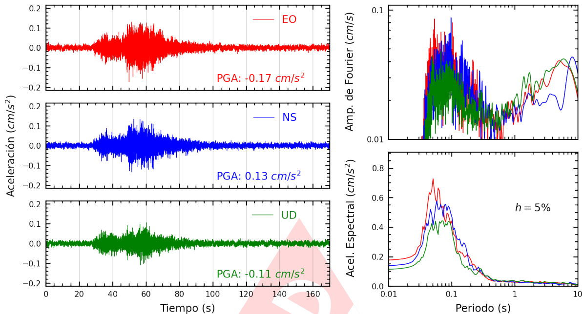
Figura A.23: Registros tiempo-historia, espectros de Fourier y de respuesta en las direcciones EO, NS y vertical de la estación UCSS. Sismo de Pisco, Pisco - Ica del 2024-05-05, 03:18:19 (Hora local)
