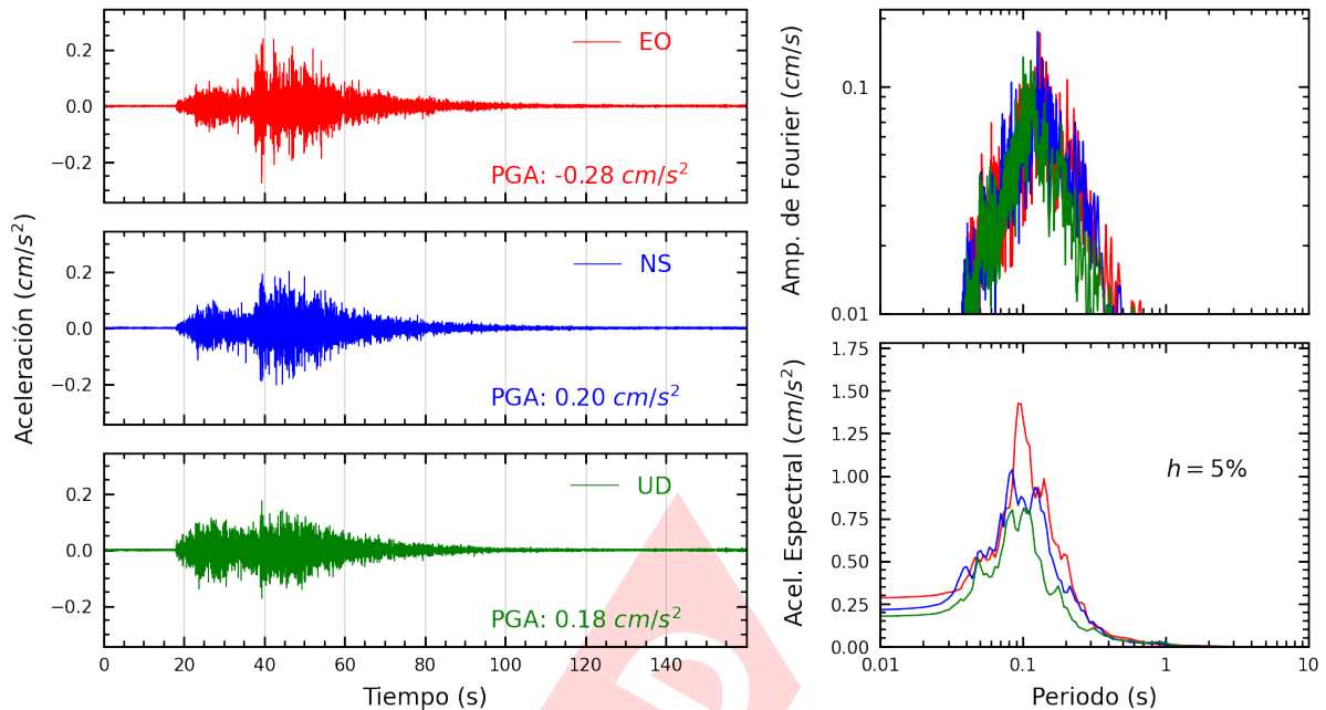
Figura A.15: Registros tiempo-historia, espectros de Fourier y de respuesta en las direcciones EO, NS y vertical de la estación JALV2. Sismo de Pisco, Pisco - Ica del 2024-05-05, 03:18:19 (Hora local)
