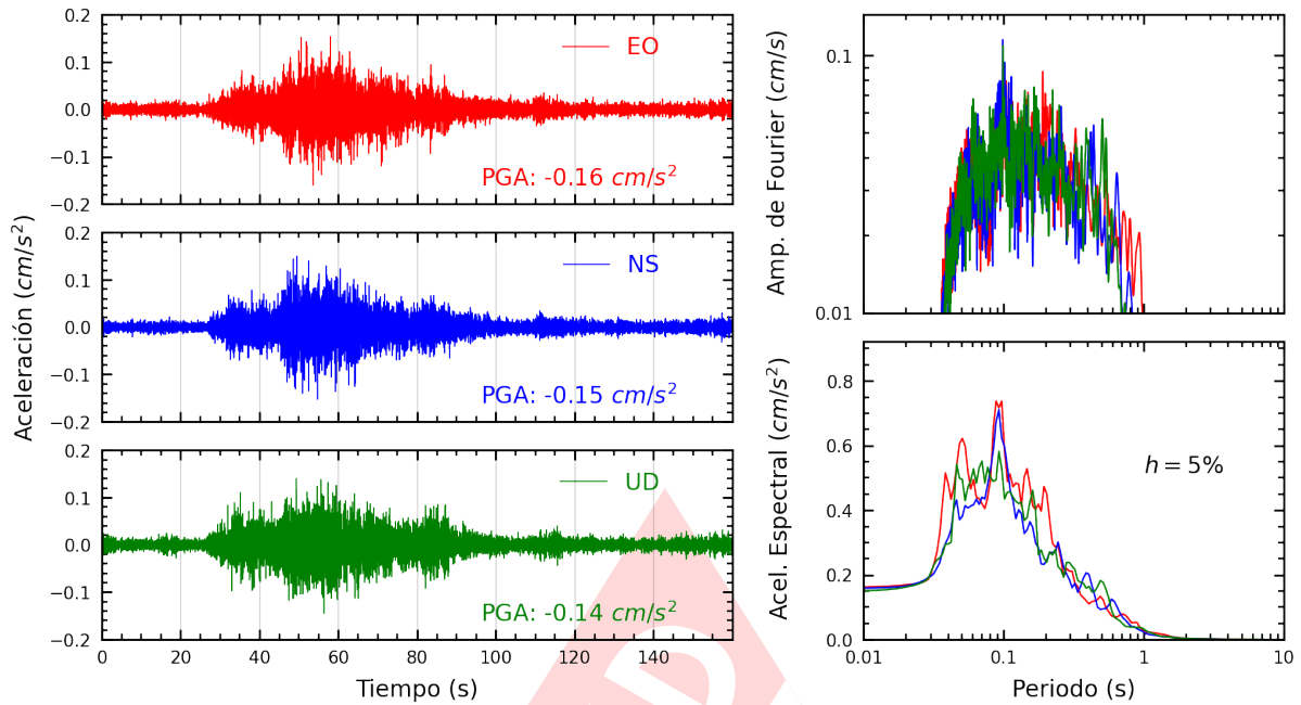
Figura A.25: Registros tiempo-historia, espectros de Fourier y de respuesta en las direcciones EO, NS y vertical de la estación IMCA2. Sismo de Pisco, Pisco - Ica del 2024-05-05, 03:18:19 (Hora local)
