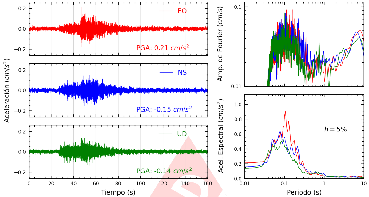
Figura A.19: Registros tiempo-historia, espectros de Fourier y de respuesta en las direcciones EO, NS y vertical de la estación CENEP. Sismo de Pisco, Pisco - Ica del 2024-05-05, 03:18:19 (Hora local)
