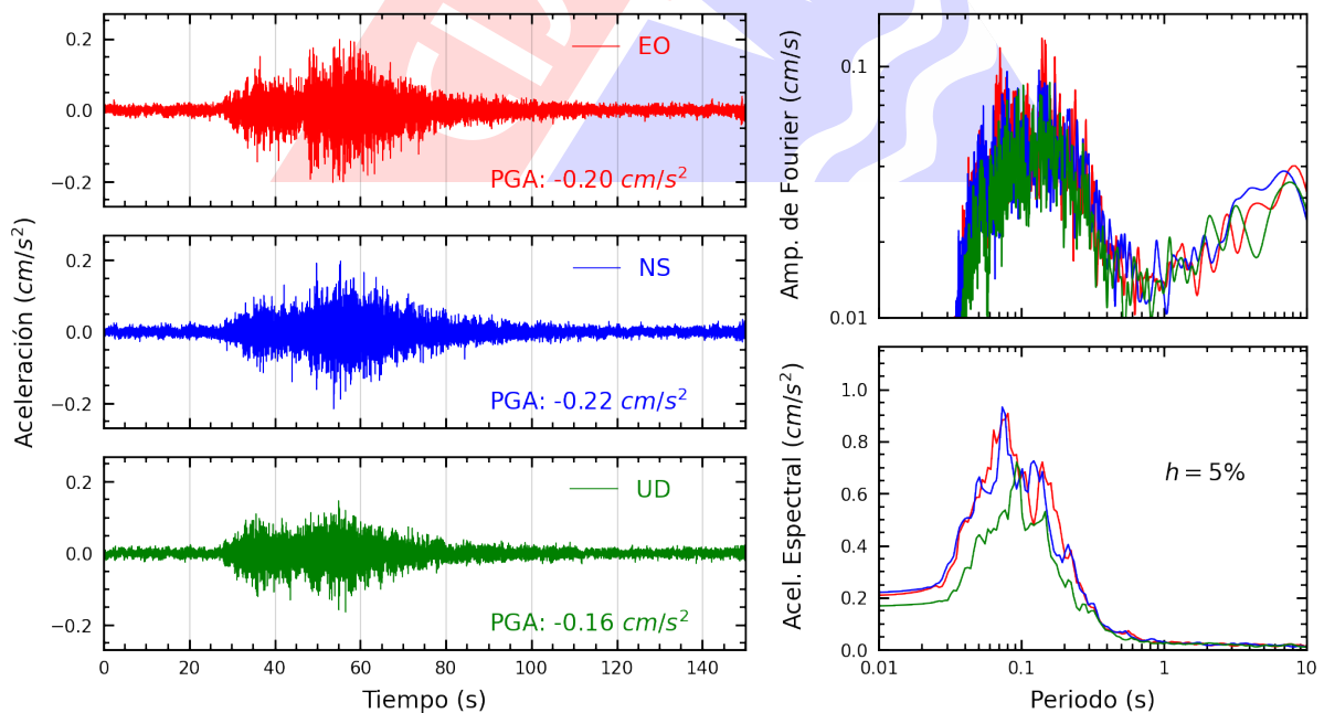
Figura A.18: Registros tiempo-historia, espectros de Fourier y de respuesta en las direcciones EO, NS y vertical de la estación FICPE. Sismo de Pisco, Pisco - Ica del 2024-05-05, 03:18:19 (Hora local)
