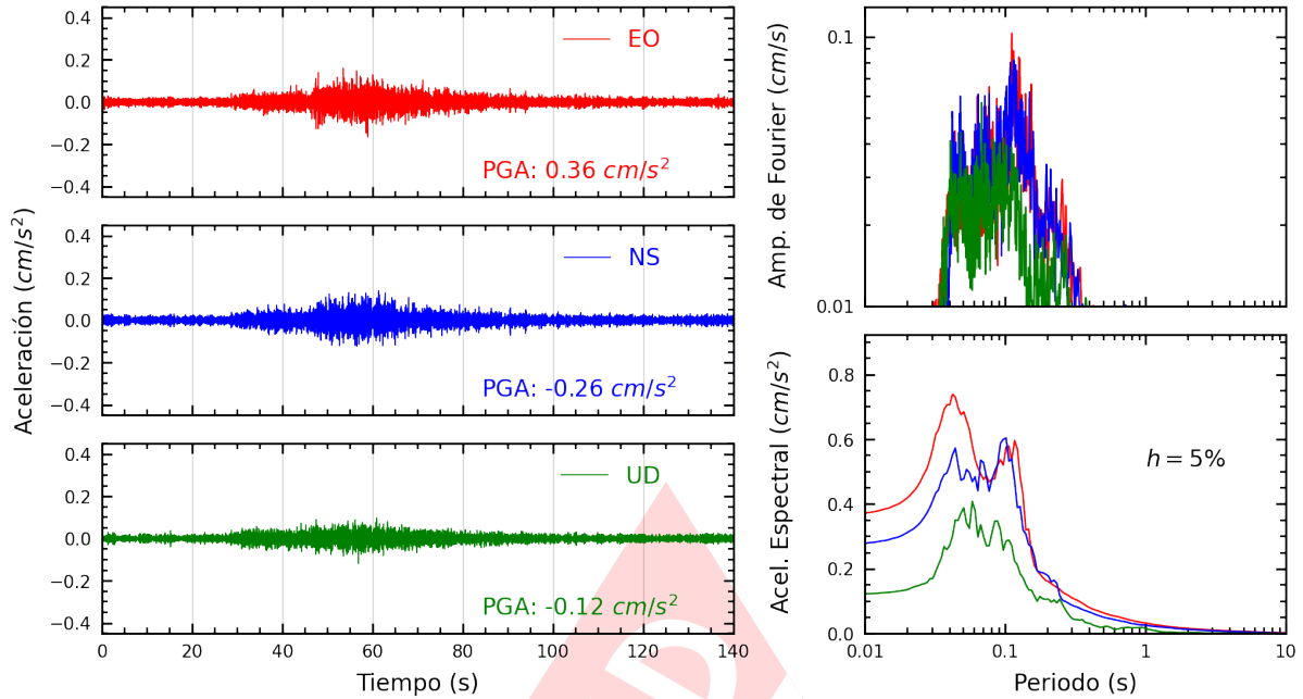
Figura A.11: Registros tiempo-historia, espectros de Fourier y de respuesta en las direcciones EO, NS y vertical de la estación ATARJ. Sismo de Pisco, Pisco - Ica del 2024-05-05, 03:18:19 (Hora local)
