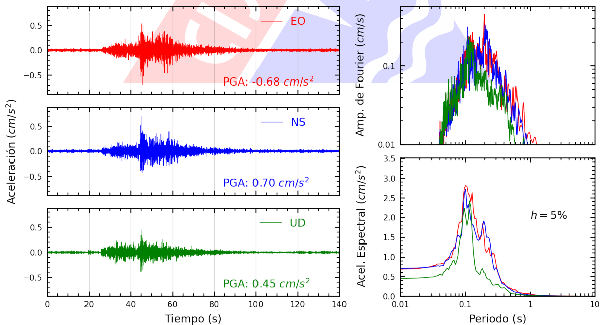
Figura A.6: Registros tiempo-historia, espectros de Fourier y de respuesta en las direcciones EO, NS y vertical de la estación SCCHO. Sismo de Pisco, Pisco - Ica del 2024-05-05, 03:18:19 (Hora local)
