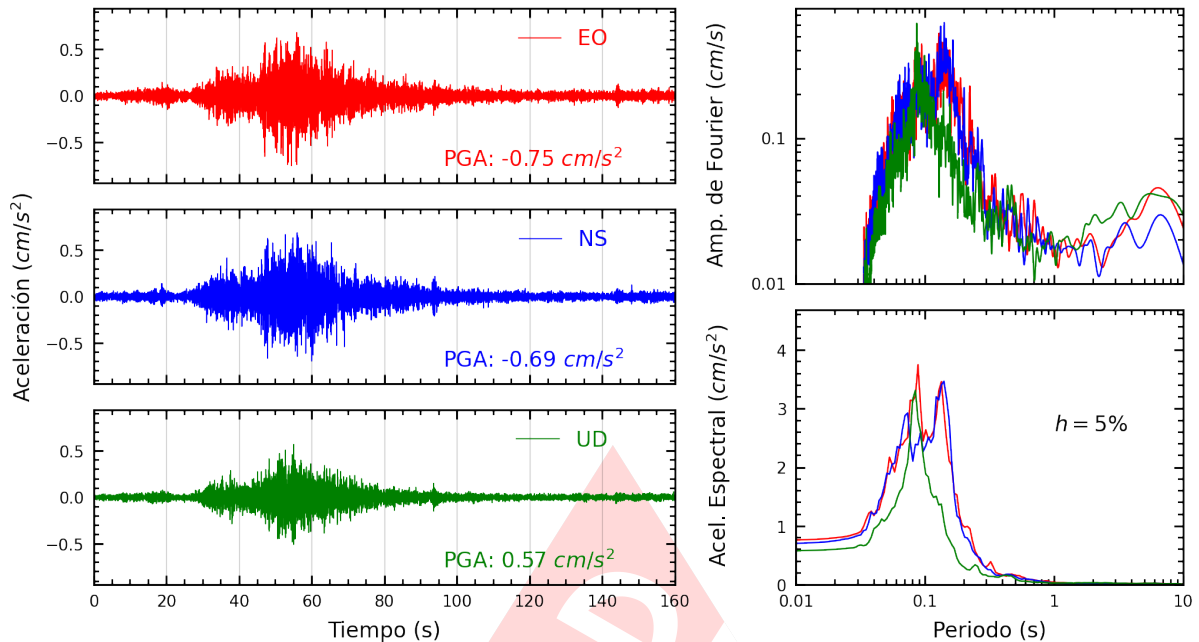
Figura A.5: Registros tiempo-historia, espectros de Fourier y de respuesta en las direcciones EO, NS y vertical de la estación USILM. Sismo de Pisco, Pisco - Ica del 2024-05-05, 03:18:19 (Hora local)
