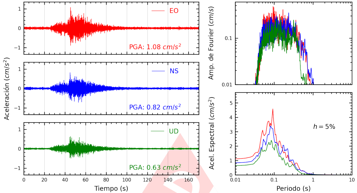
Figura A.3: Registros tiempo-historia, espectros de Fourier y de respuesta en las direcciones EO, NS y vertical de la estación UNTEL. Sismo de Pisco, Pisco - Ica del 2024-05-05, 03:18:19 (Hora local)
