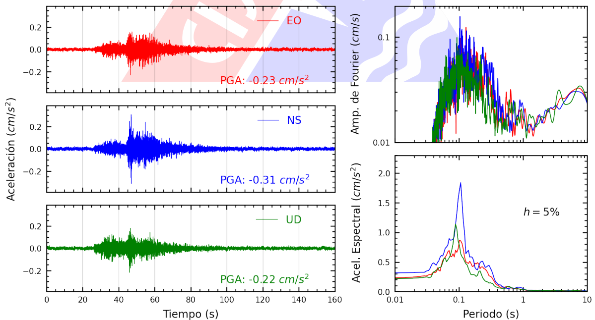
Figura A.14: Registros tiempo-historia, espectros de Fourier y de respuesta en las direcciones EO, NS y vertical de la estación SERVI. Sismo de Pisco, Pisco - Ica del 2024-05-05, 03:18:19 (Hora local)
