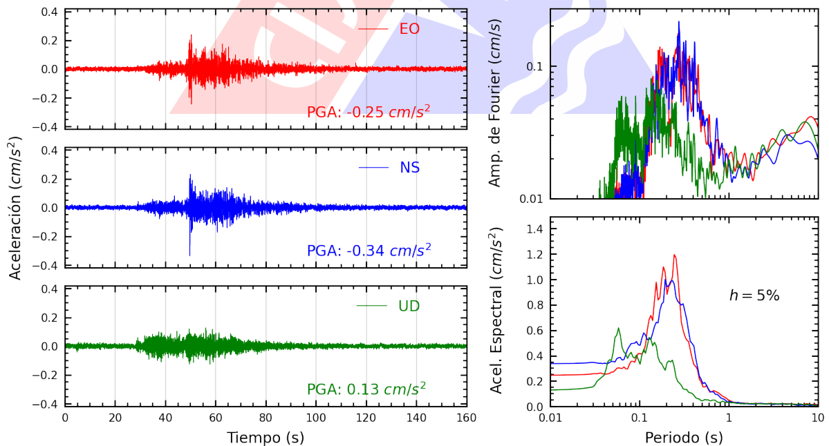
Figura A.12: Registros tiempo-historia, espectros de Fourier y de respuesta en las direcciones EO, NS y vertical de la estación ACAPU. Sismo de Pisco, Pisco - Ica del 2024-05-05, 03:18:19 (Hora local)
