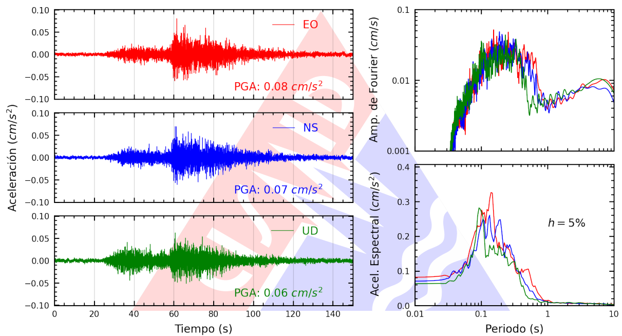
Figura A.27: Registros tiempo-historia, espectros de Fourier y de respuesta en las direcciones EO, NS y vertical de la estación CARAL. Sismo de Pisco, Pisco - Ica del 2024-05-05, 03:18:19 (Hora local)
