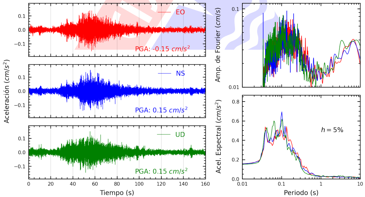
Figura A.26: Registros tiempo-historia, espectros de Fourier y de respuesta en las direcciones EO, NS y vertical de la estación USMP. Sismo de Pisco, Pisco - Ica del 2024-05-05, 03:18:19 (Hora local)
