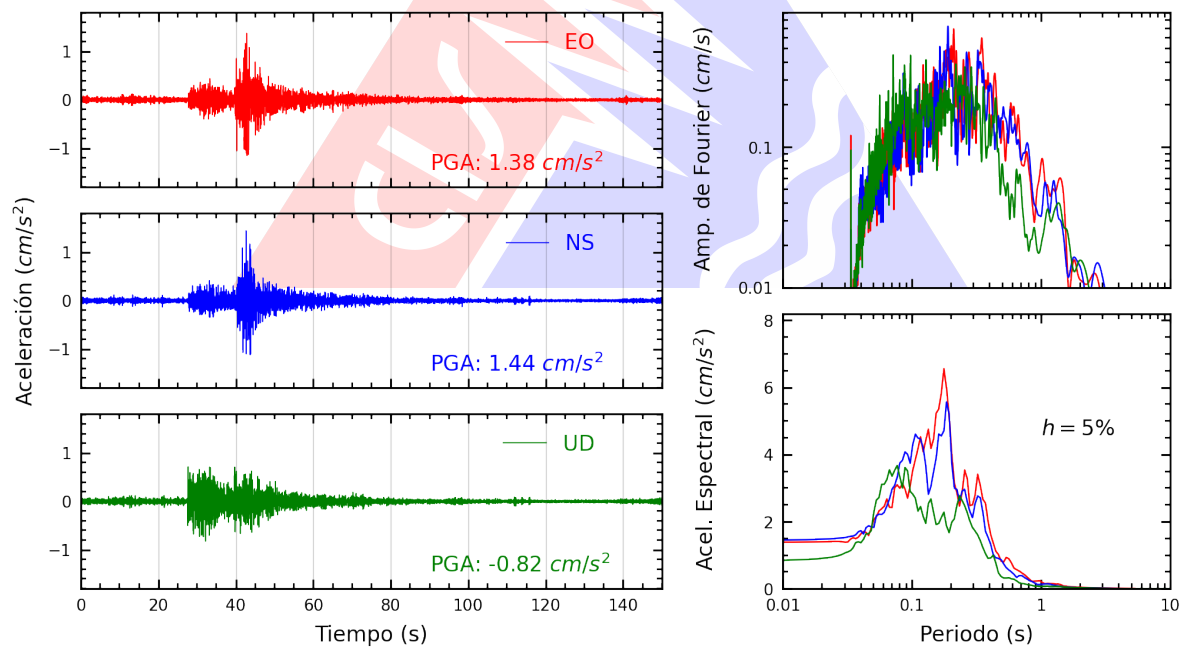
Figura A.2: Registros tiempo-historia, espectros de Fourier y de respuesta en las direcciones EO, NS y vertical de la estación SCICA. Sismo de Pisco, Pisco - Ica del 2024-05-05, 03:18:19 (Hora local)
