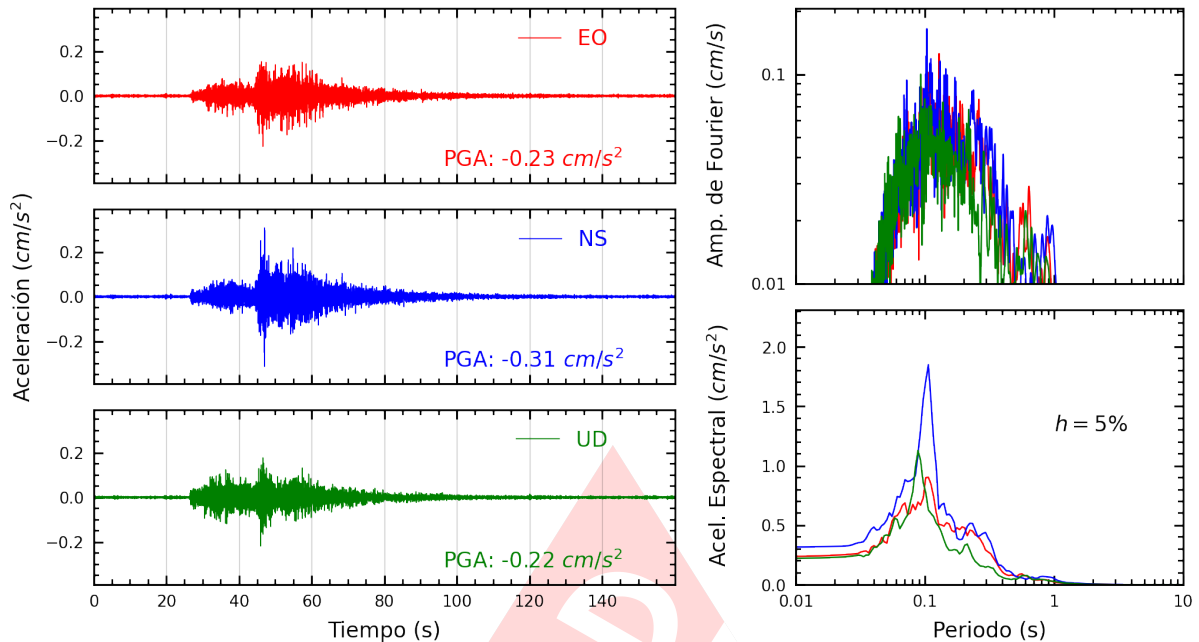
Figura A.13: Registros tiempo-historia, espectros de Fourier y de respuesta en las direcciones EO, NS y vertical de la estación SERV2. Sismo de Pisco, Pisco - Ica del 2024-05-05, 03:18:19 (Hora local)
