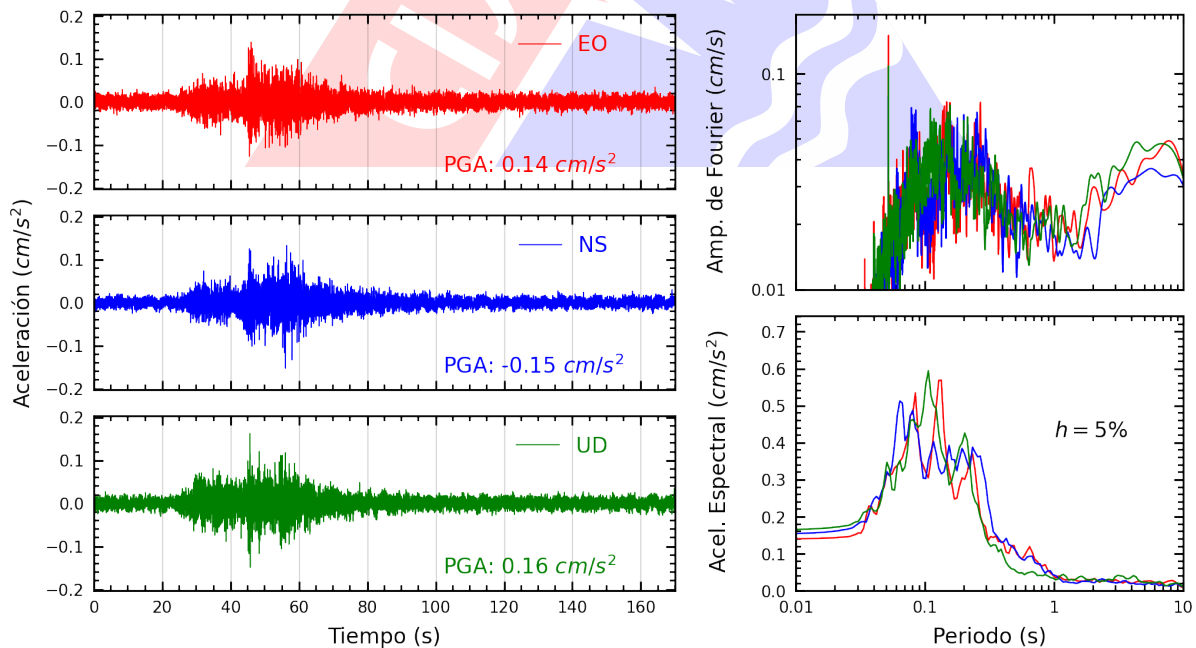
Figura A.24: Registros tiempo-historia, espectros de Fourier y de respuesta en las direcciones EO, NS y vertical de la estación UNMSM. Sismo de Pisco, Pisco - Ica del 2024-05-05, 03:18:19 (Hora local)
