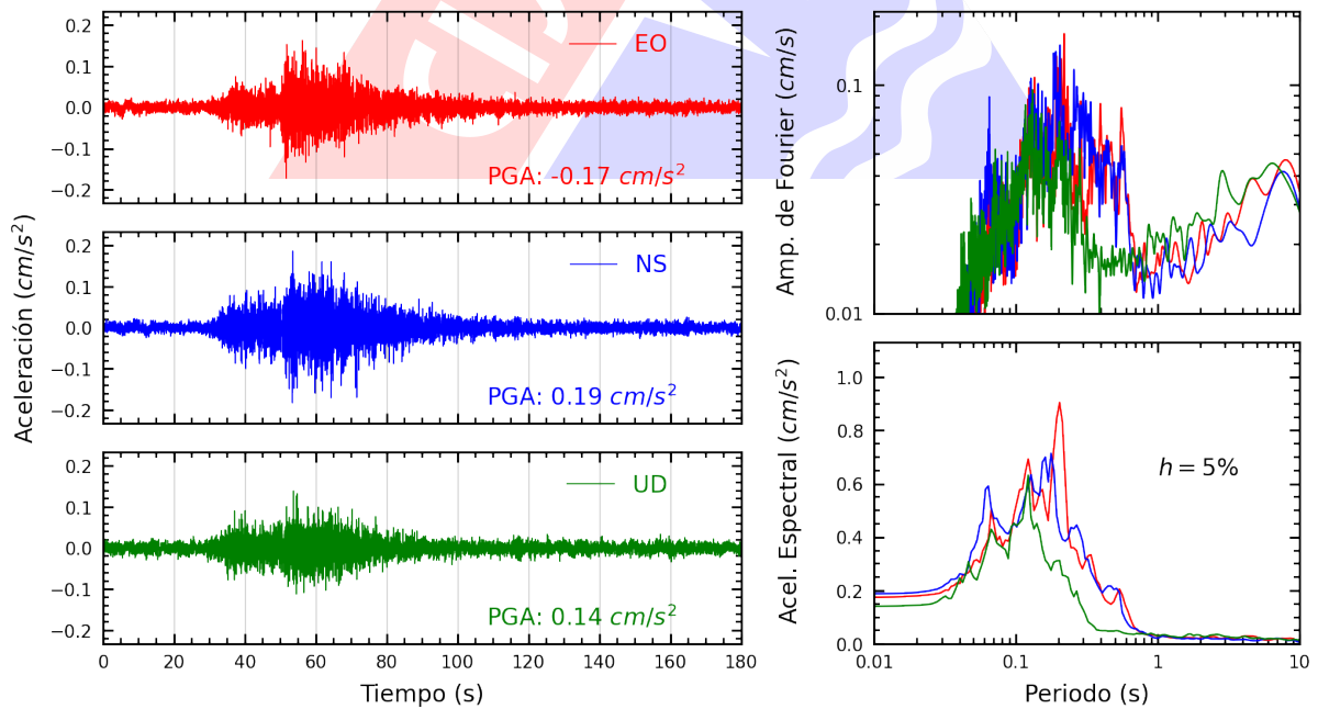
Figura A.20: Registros tiempo-historia, espectros de Fourier y de respuesta en las direcciones EO, NS y vertical de la estación VHAYA. Sismo de Pisco, Pisco - Ica del 2024-05-05, 03:18:19 (Hora local)
