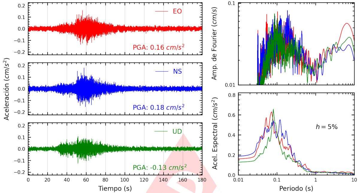
Figura A.21: Registros tiempo-historia, espectros de Fourier y de respuesta en las direcciones EO, NS y vertical de la estación COMAS. Sismo de Pisco, Pisco - Ica del 2024-05-05, 03:18:19 (Hora local)
