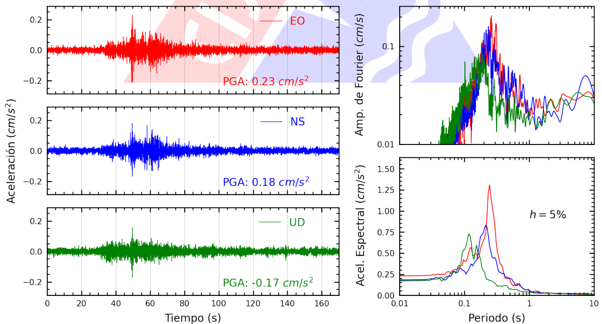
Figura A.16: Registros tiempo-historia, espectros de Fourier y de respuesta en las direcciones EO, NS y vertical de la estación DSMI. Sismo de Pisco, Pisco - Ica del 2024-05-05, 03:18:19 (Hora local)
