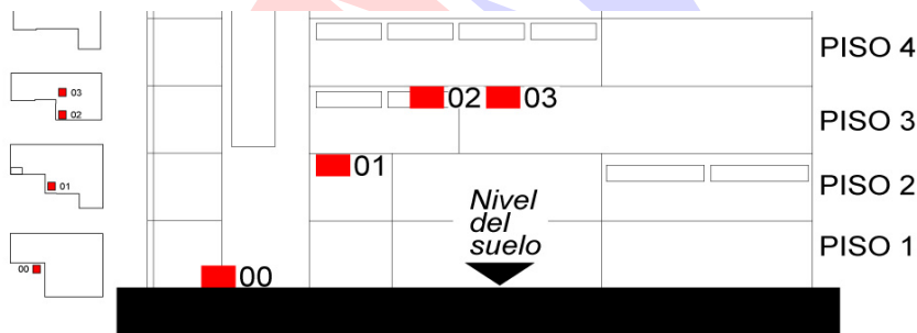
Figura 4: Distribución de sensores en la edificación monitoreada
