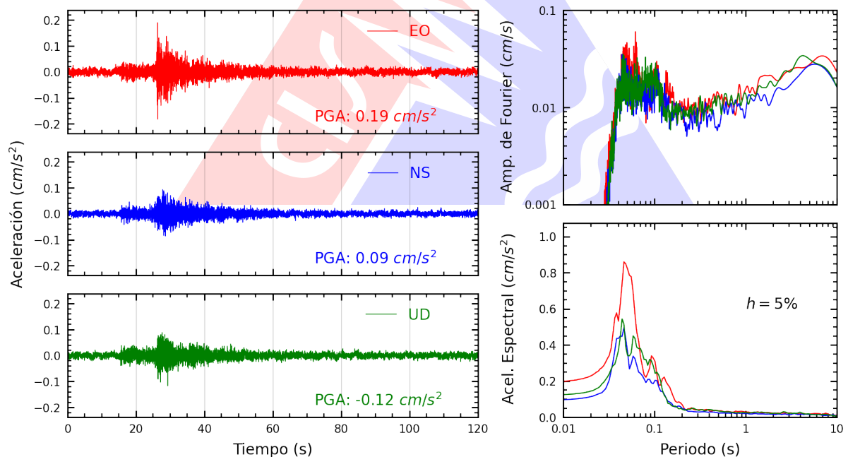
Figura A.2: Registros tiempo-historia, espectros de Fourier y de respuesta en las direcciones EO, NS y vertical de la estación AMORE. Sismo de Calango, Cañete - Lima del 2024-05-05, 15:43:11 (Hora local)
