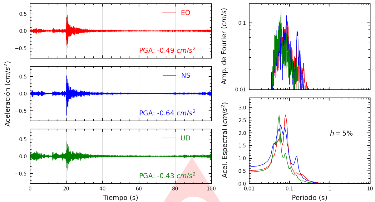
Figura A.1: Registros tiempo-historia, espectros de Fourier y de respuesta en las direcciones EO, NS y vertical de la estación ASIA. Sismo de Calango, Cañete - Lima del 2024-05-05, 15:43:11 (Hora local)
