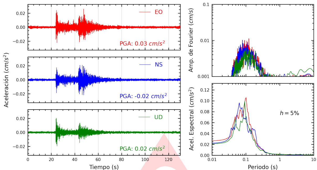
Figura A.1: Registros tiempo-historia, espectros de Fourier y de respuesta en las direcciones EO, NS y vertical de la estación UNSA. Sismo de Chivay, Caylloma - Arequipa del 2024-05-05, 20:36:36 (Hora local)
