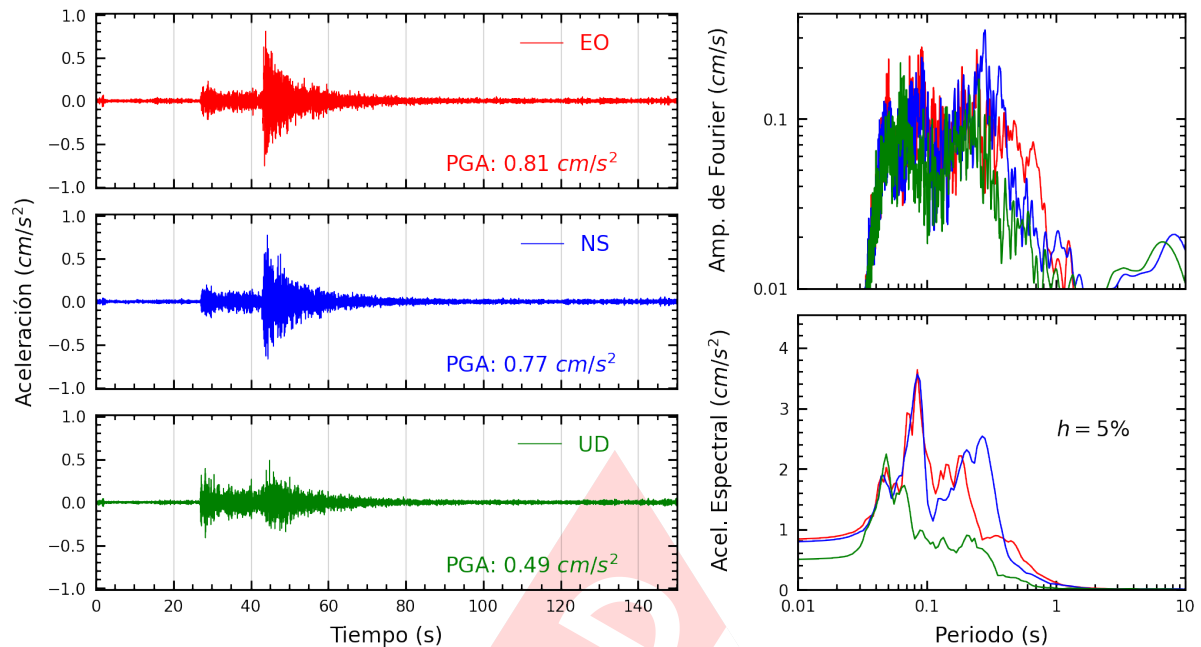
Figura A.3: Registros tiempo-historia, espectros de Fourier y de respuesta en las direcciones EO, NS y vertical de la estación CREY. Sismo de Calana, Tacna - Tacna del 2024-05-09, 08:40:44 (Hora local)
