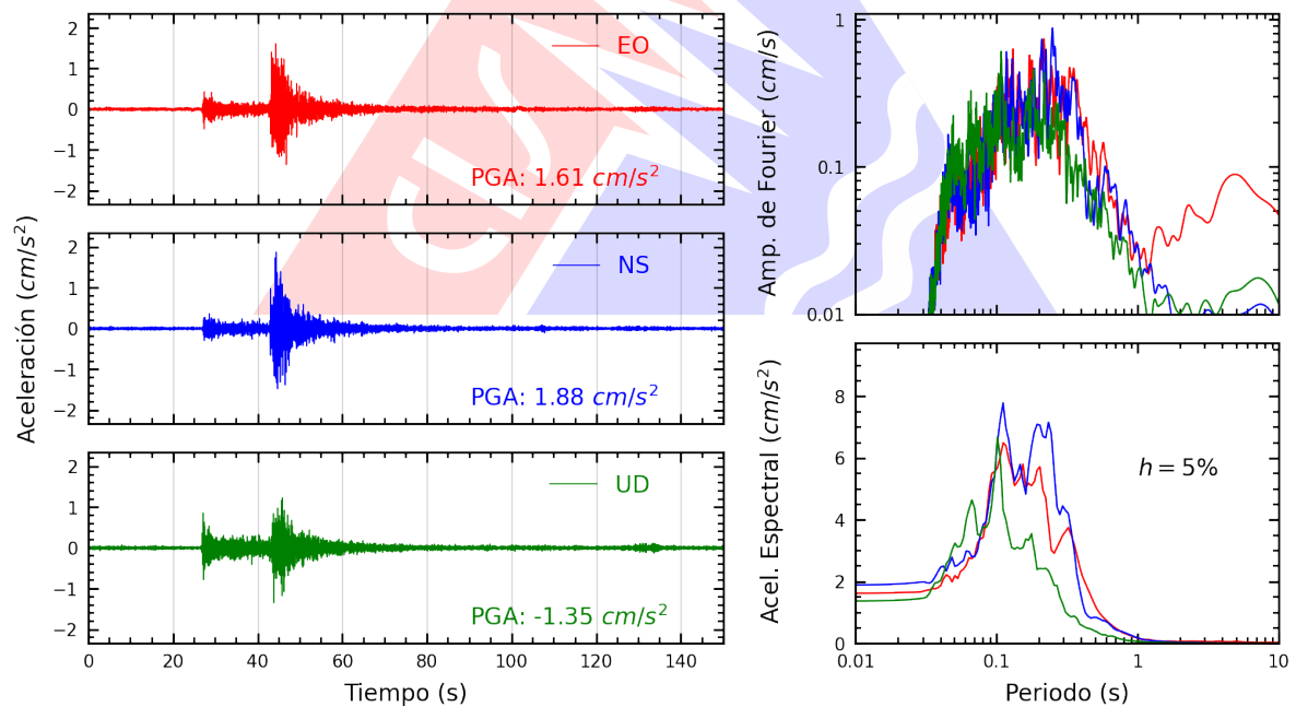
Figura A.2: Registros tiempo-historia, espectros de Fourier y de respuesta en las direcciones EO, NS y vertical de la estación UJBG3. Sismo de Calana, Tacna - Tacna del 2024-05-09, 08:40:44 (Hora local)
