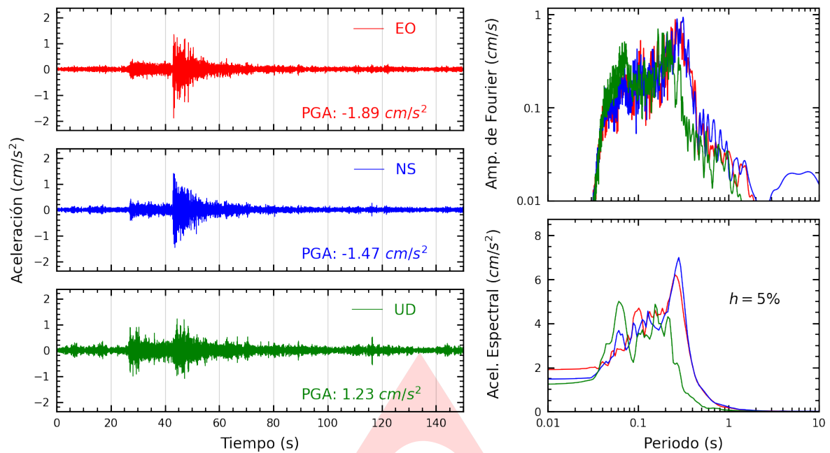
Figura A.1: Registros tiempo-historia, espectros de Fourier y de respuesta en las direcciones EO, NS y vertical de la estación SCTAC. Sismo de Calana, Tacna - Tacna del 2024-05-09, 08:40:44 (Hora local)
