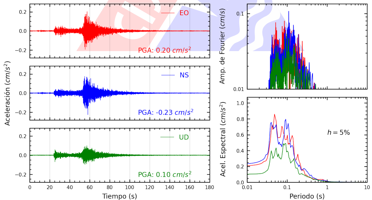
Figura A.4: Registros tiempo-historia, espectros de Fourier y de respuesta en las direcciones EO, NS y vertical de la estación UNSA. Sismo de Calana, Tacna - Tacna del 2024-05-09, 08:40:44 (Hora local)
