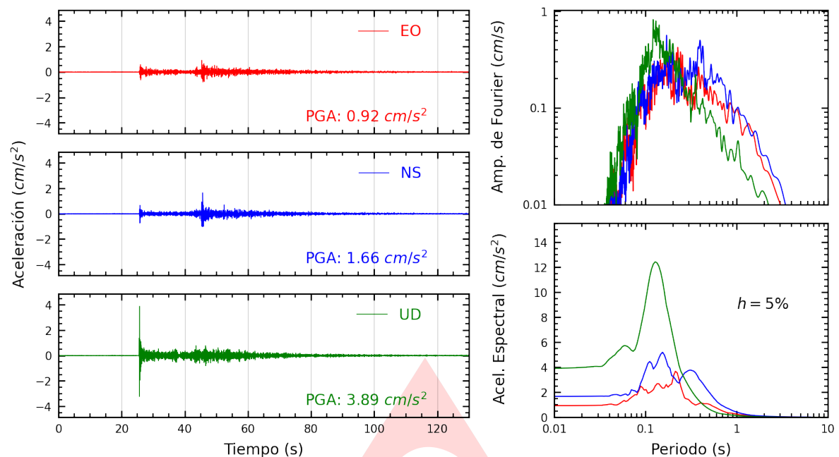
Figura A.1: Registros tiempo-historia, espectros de Fourier y de respuesta en las direcciones EO, NS y vertical de la estación UNIA. Sismo de Aguaytia, Padre Abad - Ucayali del 2024-05-10, 07:34:48 (Hora local)
