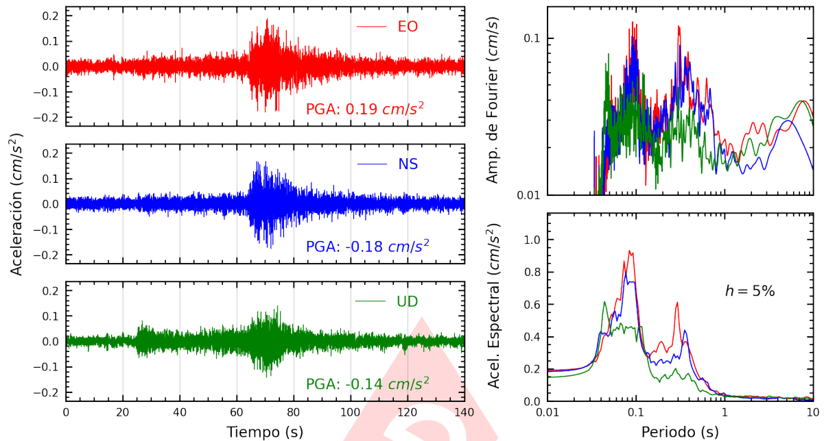
Figura A.9: Registros tiempo-historia, espectros de Fourier y de respuesta en las direcciones EO, NS y vertical de la estación USILP. Sismo de Aguaytia, Padre Abad - Ucayali del 2024-05-10, 07:34:48 (Hora local)
