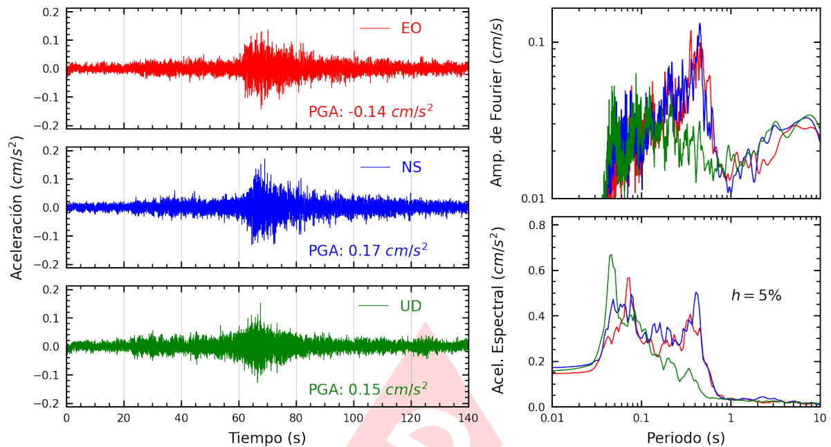
Figura A.11: Registros tiempo-historia, espectros de Fourier y de respuesta en las direcciones EO, NS y vertical de la estación VHAYA. Sismo de Aguaytia, Padre Abad - Ucayali del 2024-05-10, 07:34:48 (Hora local)
