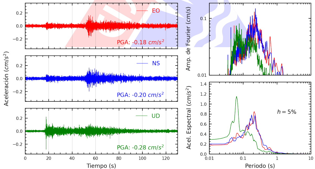
Figura A.6: Registros tiempo-historia, espectros de Fourier y de respuesta en las direcciones EO, NS y vertical de la estación UNAAA. Sismo de Aguaytia, Padre Abad - Ucayali del 2024-05-10, 07:34:48 (Hora local)
