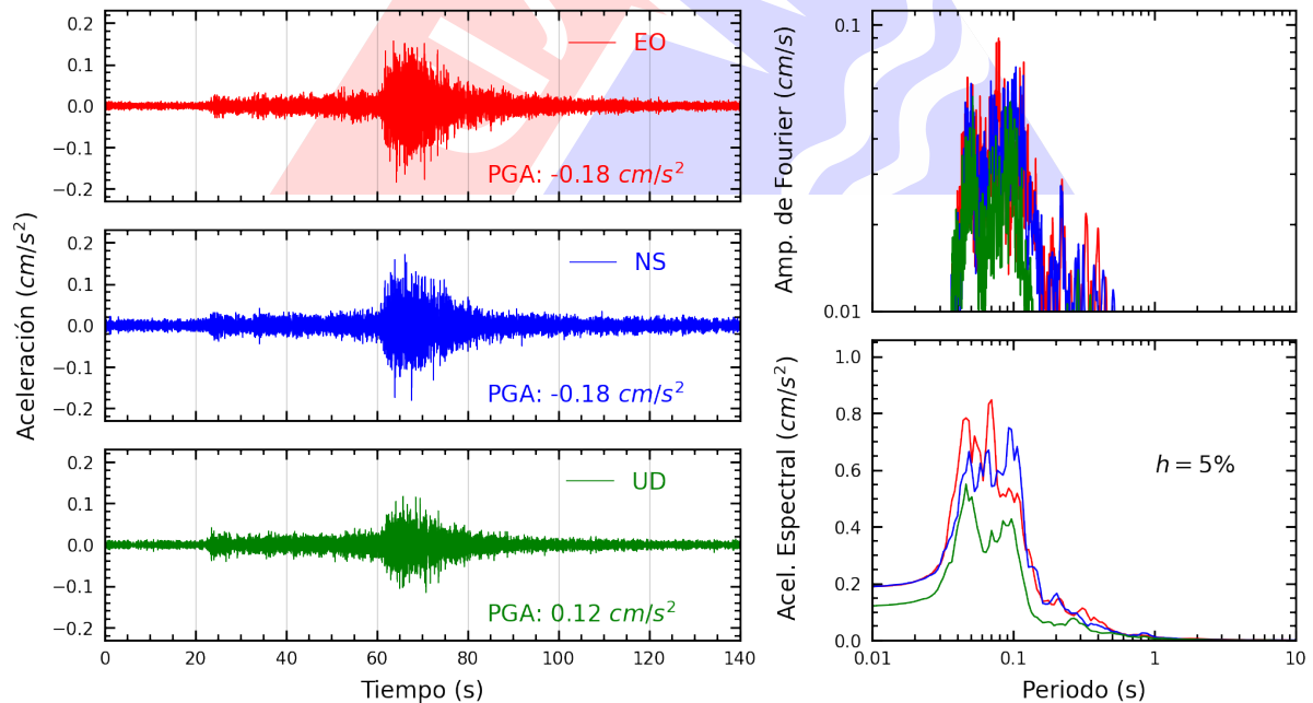
Figura A.10: Registros tiempo-historia, espectros de Fourier y de respuesta en las direcciones EO, NS y vertical de la estación ATARJ. Sismo de Aguaytia, Padre Abad - Ucayali del 2024-05-10, 07:34:48 (Hora local)
