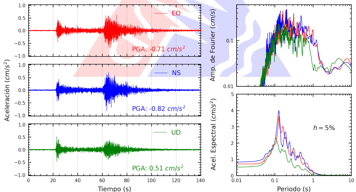
Figura A.2: Registros tiempo-historia, espectros de Fourier y de respuesta en las direcciones EO, NS y vertical de la estación UNTRM. Sismo de Aguaytia, Padre Abad - Ucayali del 2024-05-10, 07:34:48 (Hora local)
