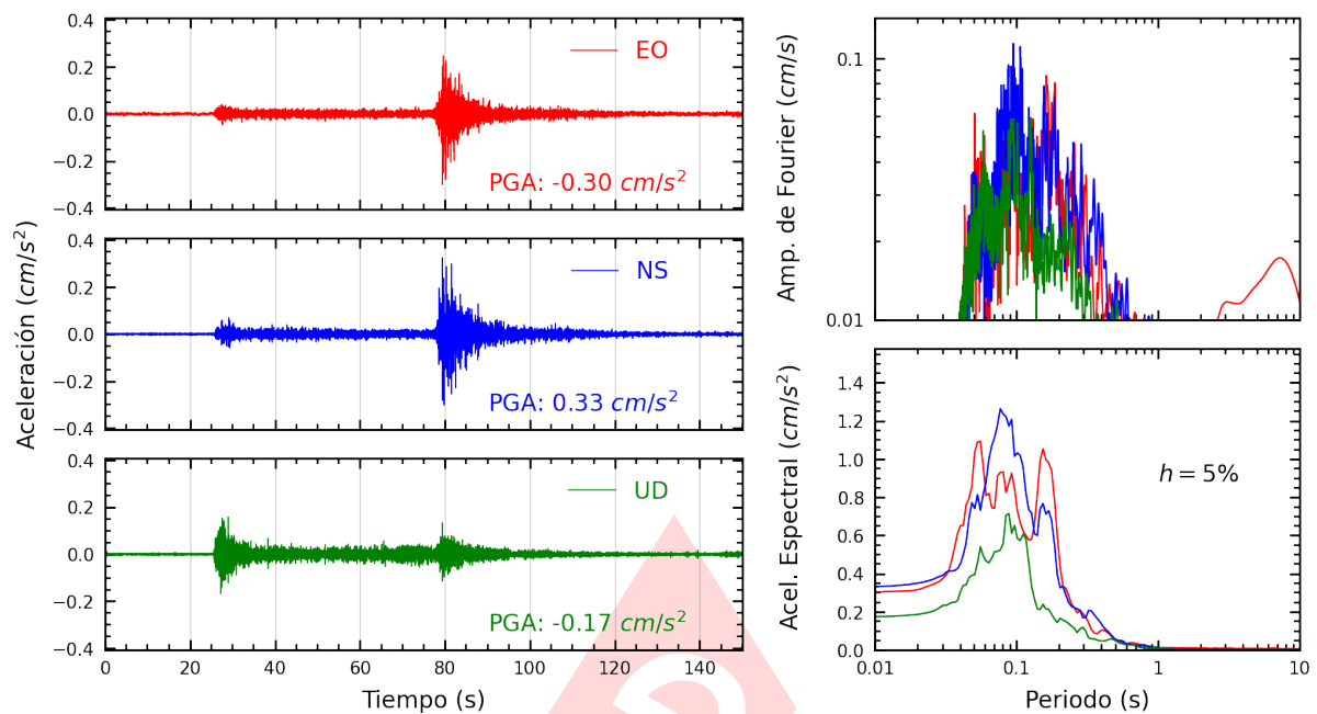
Figura A.5: Registros tiempo-historia, espectros de Fourier y de respuesta en las direcciones EO, NS y vertical de la estación SCCHI. Sismo de Aguaytia, Padre Abad - Ucayali del 2024-05-10, 07:34:48 (Hora local)
