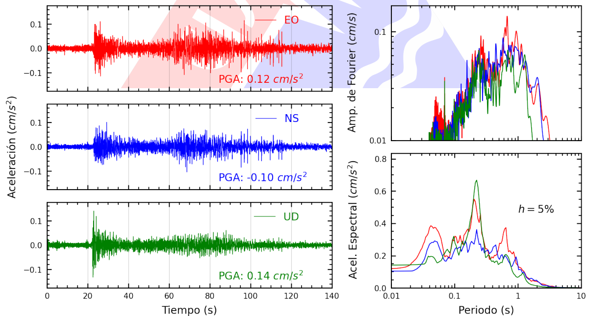
Figura A.12: Registros tiempo-historia, espectros de Fourier y de respuesta en las direcciones EO, NS y vertical de la estación UNC. Sismo de Aguaytia, Padre Abad - Ucayali del 2024-05-10, 07:34:48 (Hora local)
