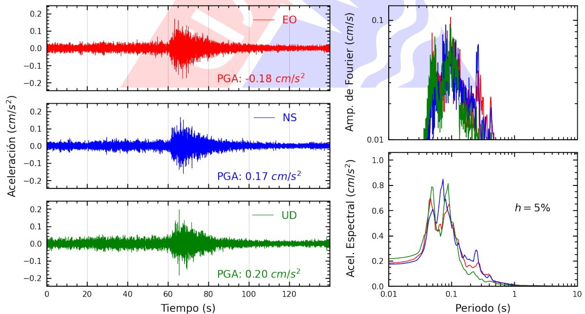
Figura A.8: Registros tiempo-historia, espectros de Fourier y de respuesta en las direcciones EO, NS y vertical de la estación JALV2. Sismo de Aguaytia, Padre Abad - Ucayali del 2024-05-10, 07:34:48 (Hora local)
