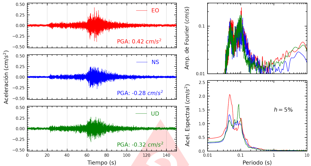
Figura A.3: Registros tiempo-historia, espectros de Fourier y de respuesta en las direcciones EO, NS y vertical de la estación AMORE. Sismo de Aguaytia, Padre Abad - Ucayali del 2024-05-10, 07:34:48 (Hora local)
