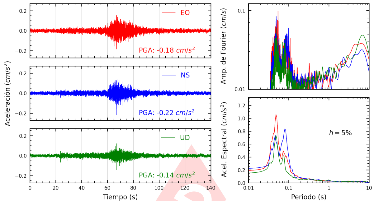
Figura A.7: Registros tiempo-historia, espectros de Fourier y de respuesta en las direcciones EO, NS y vertical de la estación UCSS. Sismo de Aguaytia, Padre Abad - Ucayali del 2024-05-10, 07:34:48 (Hora local)
