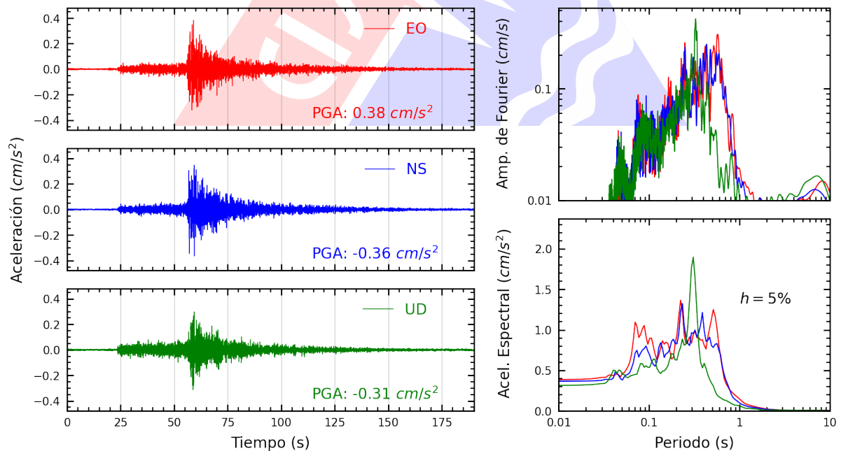
Figura A.4: Registros tiempo-historia, espectros de Fourier y de respuesta en las direcciones EO, NS y vertical de la estación CARAL. Sismo de Aguaytia, Padre Abad - Ucayali del 2024-05-10, 07:34:48 (Hora local)
