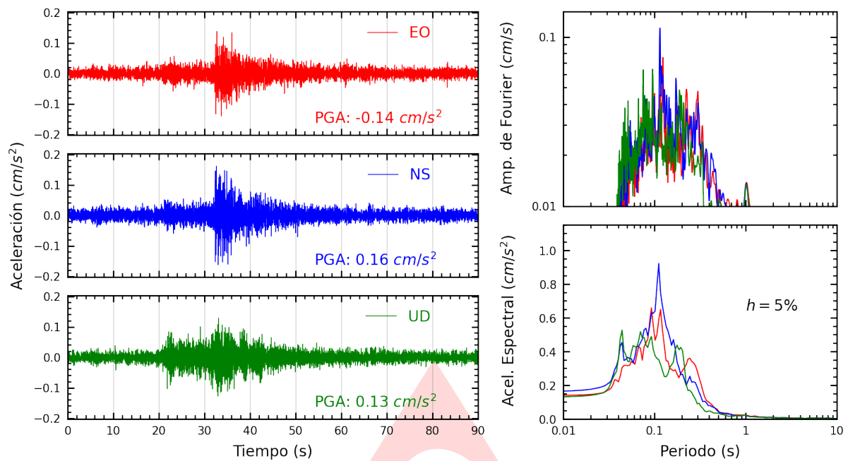
Figura A.1: Registros tiempo-historia, espectros de Fourier y de respuesta en las direcciones EO, NS y vertical de la estación UNICA. Sismo de Palpa, Palpa - Ica del 2024-05-11, 04:15:57 (Hora local)
