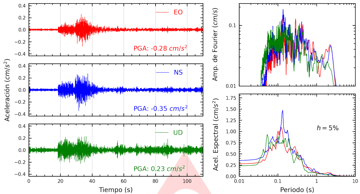
Figura A.1: Registros tiempo-historia, espectros de Fourier y de respuesta en las direcciones EO, NS y vertical de la estación SCHYO. Sismo de La Oroya, Yauli - Junin del 2024-05-12, 14:58:01 (Hora local)
