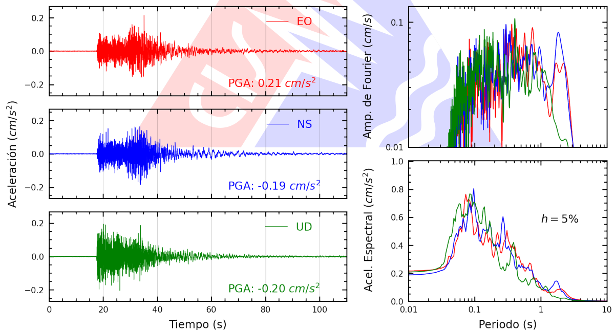
Figura A.2: Registros tiempo-historia, espectros de Fourier y de respuesta en las direcciones EO, NS y vertical de la estación UNCP. Sismo de La Oroya, Yauli - Junin del 2024-05-12, 14:58:01 (Hora local)
