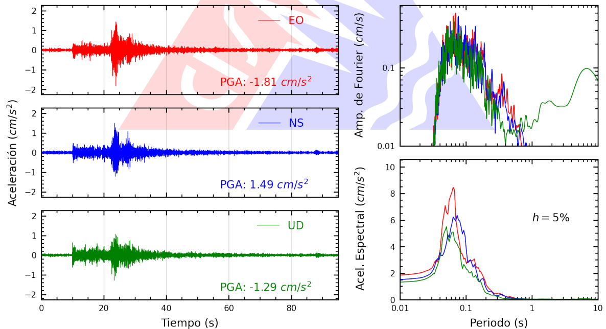
Figura A.2: Registros tiempo-historia, espectros de Fourier y de respuesta en las direcciones EO, NS y vertical de la estación SCARQ. Sismo de Punta De Bombon, Islay - Arequipa del 2024-05-13, 17:09:21 (Hora local)
