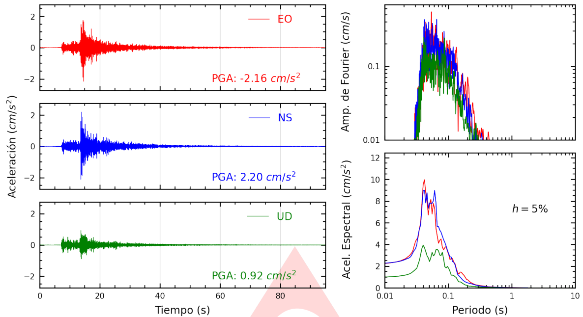
Figura A.1: Registros tiempo-historia, espectros de Fourier y de respuesta en las direcciones EO, NS y vertical de la estación UNSA. Sismo de Punta De Bombon, Islay - Arequipa del 2024-05-13, 17:09:21 (Hora local)
