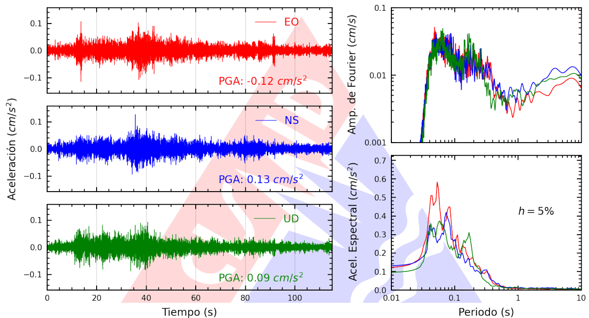
Figura A.5: Registros tiempo-historia, espectros de Fourier y de respuesta en las direcciones EO, NS y vertical de la estación CREY. Sismo de Punta De Bombon, Islay - Arequipa del 2024-05-13, 17:09:21 (Hora local)
