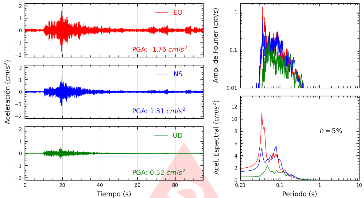
Figura A.3: Registros tiempo-historia, espectros de Fourier y de respuesta en las direcciones EO, NS y vertical de la estación UNAM. Sismo de Punta De Bombon, Islay - Arequipa del 2024-05-13, 17:09:21 (Hora local)
