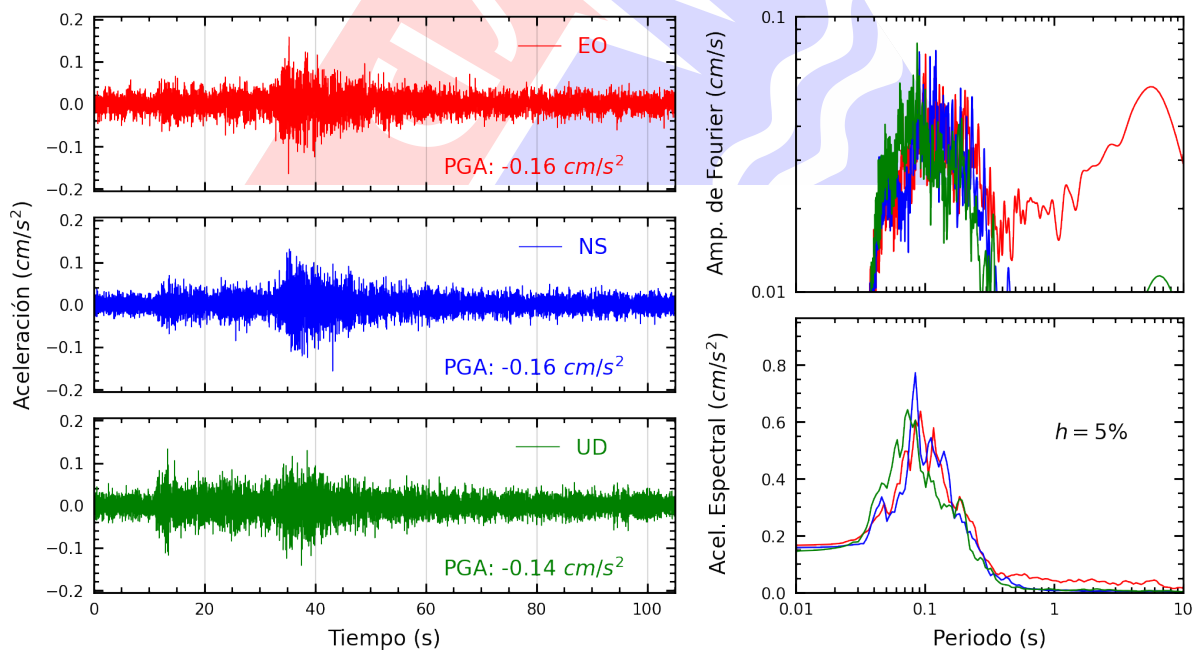
Figura A.4: Registros tiempo-historia, espectros de Fourier y de respuesta en las direcciones EO, NS y vertical de la estación UJBG3. Sismo de Punta De Bombon, Islay - Arequipa del 2024-05-13, 17:09:21 (Hora local)
