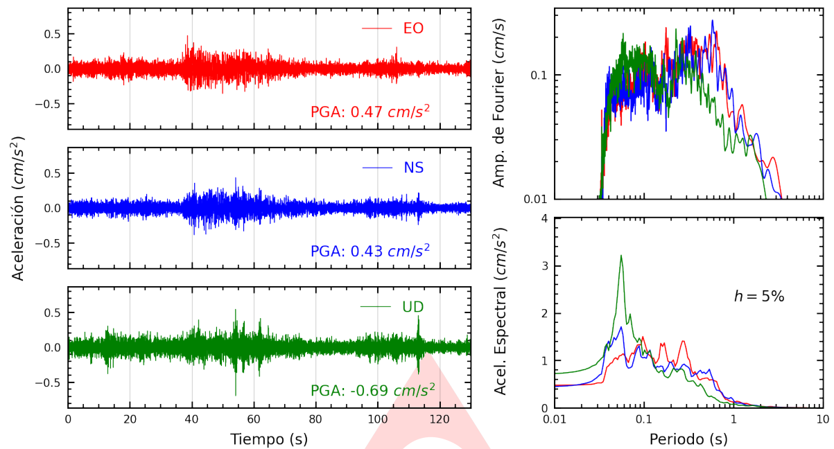
Figura A.1: Registros tiempo-historia, espectros de Fourier y de respuesta en las direcciones EO, NS y vertical de la estación SCICA. Sismo de Pampamarca, Parinacochas - Ayacucho del 2024-05-20, 12:23:43 (Hora local)
