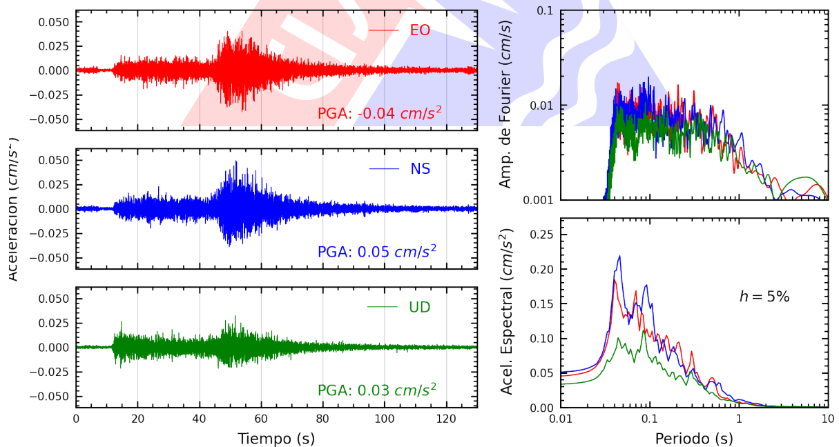
Figura A.4: Registros tiempo-historia, espectros de Fourier y de respuesta en las direcciones EO, NS y vertical de la estación UNSA. Sismo de Pampamarca, Parinacochas - Ayacucho del 2024-05-20, 12:23:43 (Hora local)
