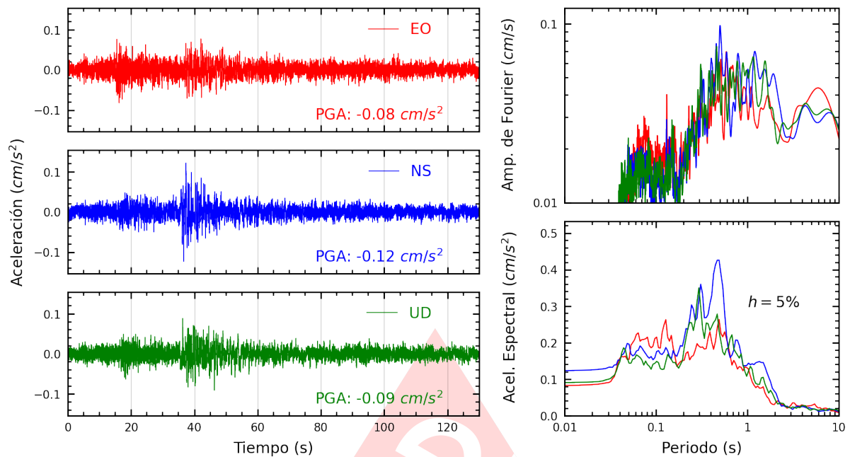
Figura A.3: Registros tiempo-historia, espectros de Fourier y de respuesta en las direcciones EO, NS y vertical de la estación UNSCH. Sismo de Pampamarca, Parinacochas - Ayacucho del 2024-05-20, 12:23:43 (Hora local)
