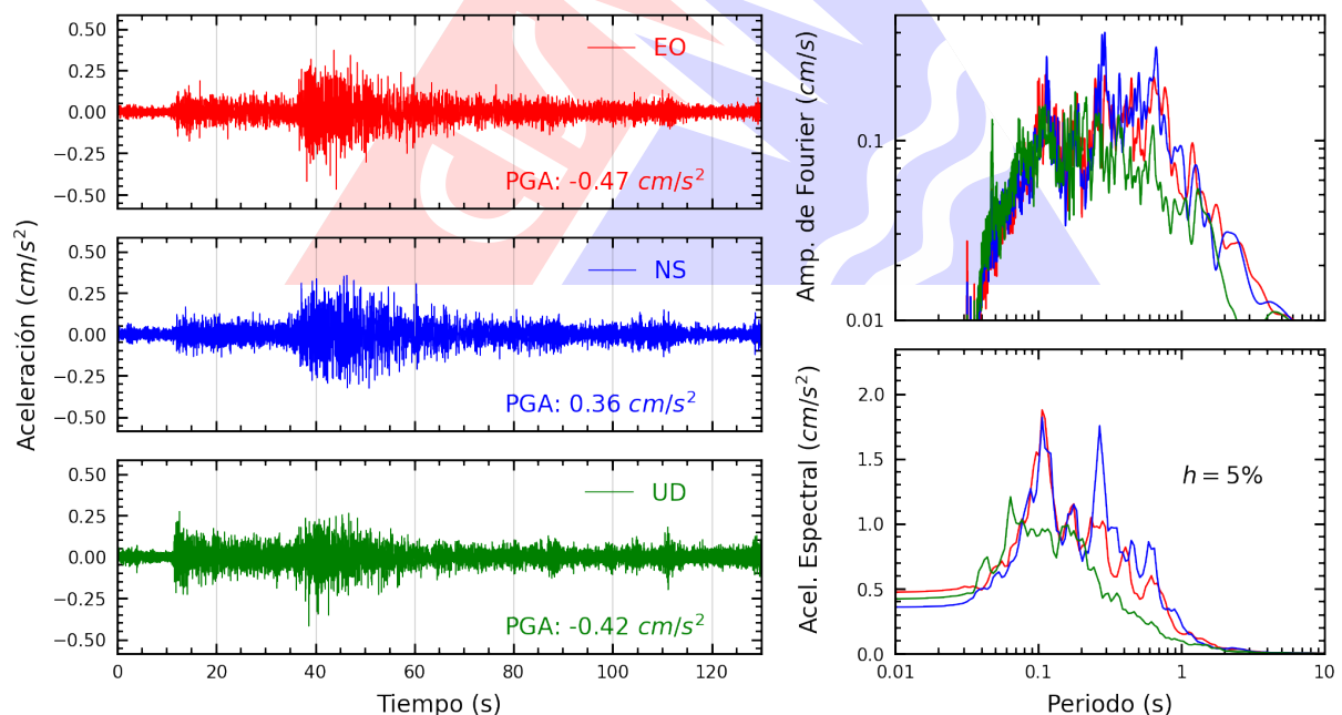
Figura A.2: Registros tiempo-historia, espectros de Fourier y de respuesta en las direcciones EO, NS y vertical de la estación UNICA. Sismo de Pampamarca, Parinacochas - Ayacucho del 2024-05-20, 12:23:43 (Hora local)
