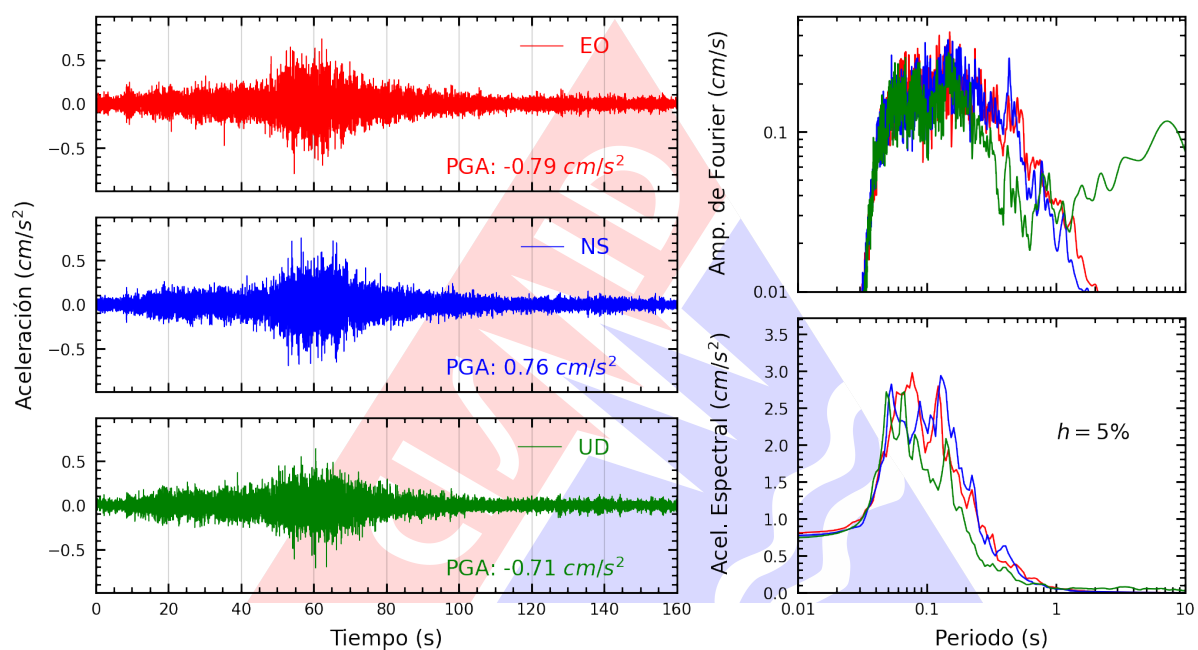
Figura A.5: Registros tiempo-historia, espectros de Fourier y de respuesta en las direcciones EO, NS y vertical de la estación SCARQ. Sismo de Azangaro, Azangaro - Puno del 2024-05-20, 18:53:48 (Hora local)
