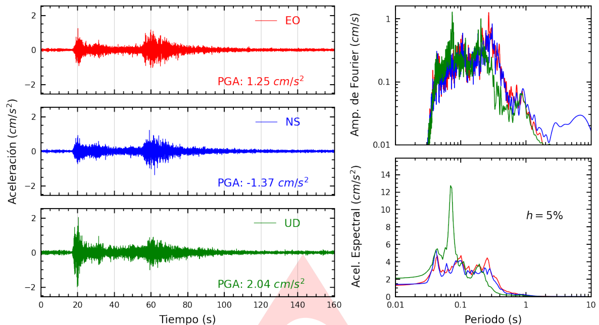
Figura A.1: Registros tiempo-historia, espectros de Fourier y de respuesta en las direcciones EO, NS y vertical de la estación SCTAC. Sismo de Azangaro, Azangaro - Puno del 2024-05-20, 18:53:48 (Hora local)
