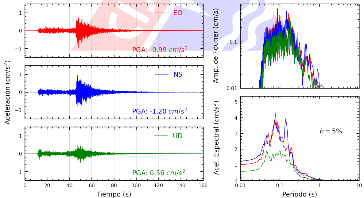
Figura A.4: Registros tiempo-historia, espectros de Fourier y de respuesta en las direcciones EO, NS y vertical de la estación UNSA. Sismo de Azangaro, Azangaro - Puno del 2024-05-20, 18:53:48 (Hora local)
