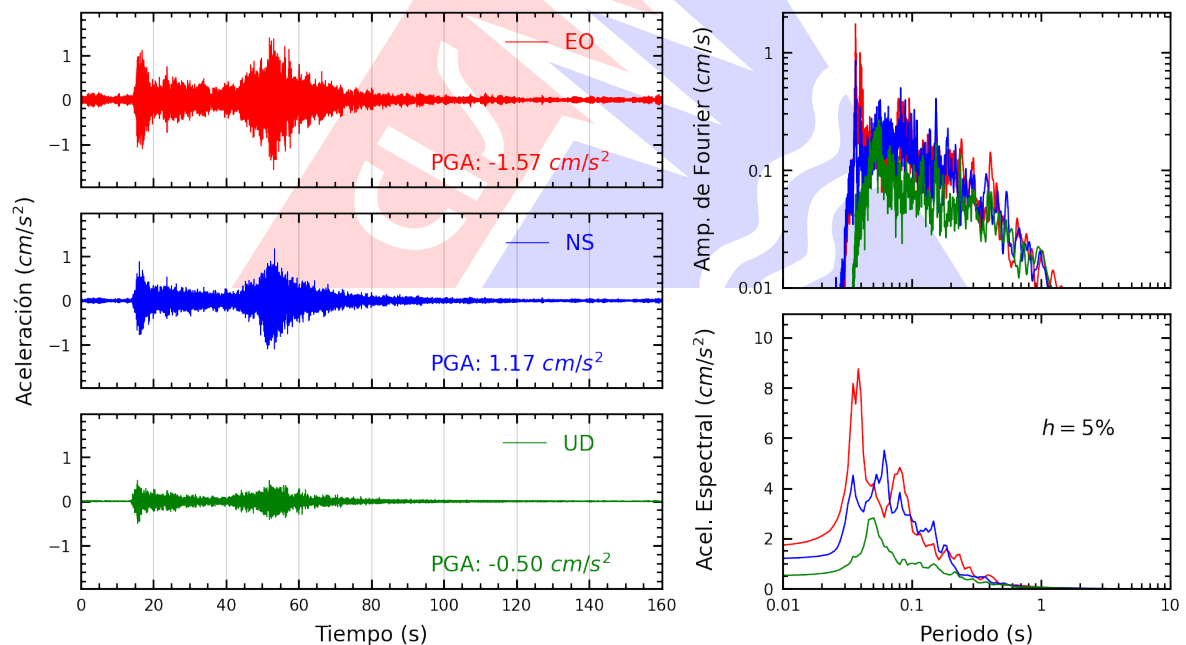
Figura A.2: Registros tiempo-historia, espectros de Fourier y de respuesta en las direcciones EO, NS y vertical de la estación UNAM. Sismo de Azangaro, Azangaro - Puno del 2024-05-20, 18:53:48 (Hora local)
