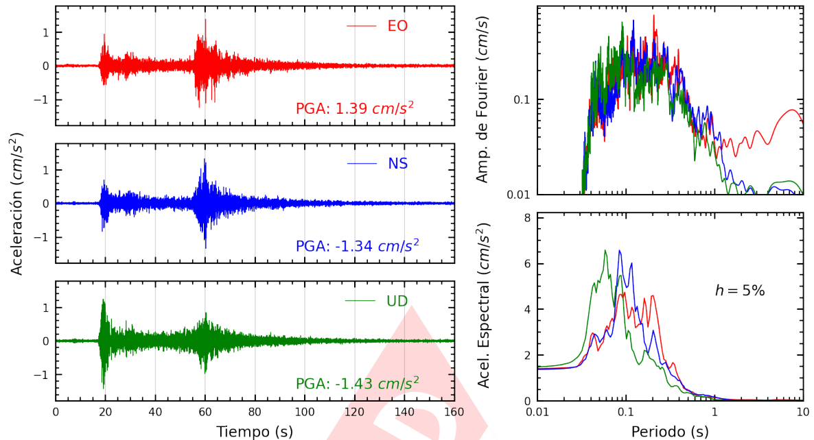
Figura A.3: Registros tiempo-historia, espectros de Fourier y de respuesta en las direcciones EO, NS y vertical de la estación UJBG3. Sismo de Azangaro, Azangaro - Puno del 2024-05-20, 18:53:48 (Hora local)
