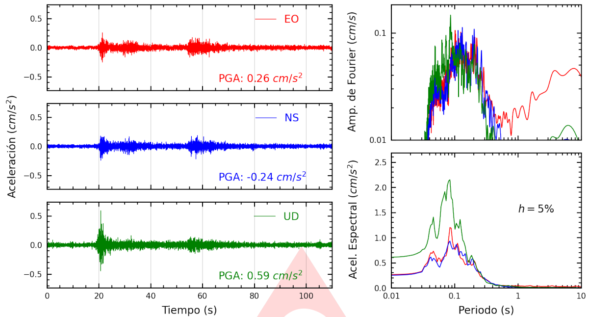
Figura A.1: Registros tiempo-historia, espectros de Fourier y de respuesta en las direcciones EO, NS y vertical de la estación UJBG3. Sismo de Juliaca, San Roman - Puno del 2024-05-22, 11:38:52 (Hora local)
