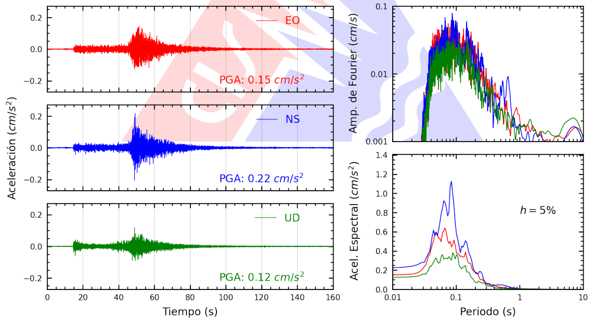
Figura A.2: Registros tiempo-historia, espectros de Fourier y de respuesta en las direcciones EO, NS y vertical de la estación UNSA. Sismo de Juliaca, San Roman - Puno del 2024-05-22, 11:38:52 (Hora local)
