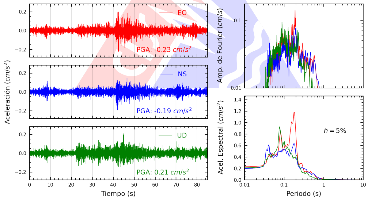
Figura A.2: Registros tiempo-historia, espectros de Fourier y de respuesta en las direcciones EO, NS y vertical de la estación SCICA. Sismo de Nazca, Nazca - Ica del 2024-05-24, 00:28:32 (Hora local)
