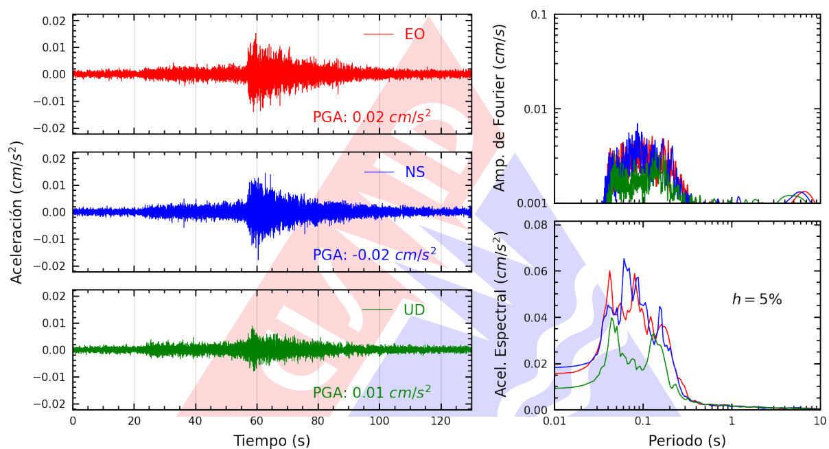
Figura A.3: Registros tiempo-historia, espectros de Fourier y de respuesta en las direcciones EO, NS y vertical de la estación UNSA. Sismo de Nazca, Nazca - Ica del 2024-05-24, 00:28:32 (Hora local)
