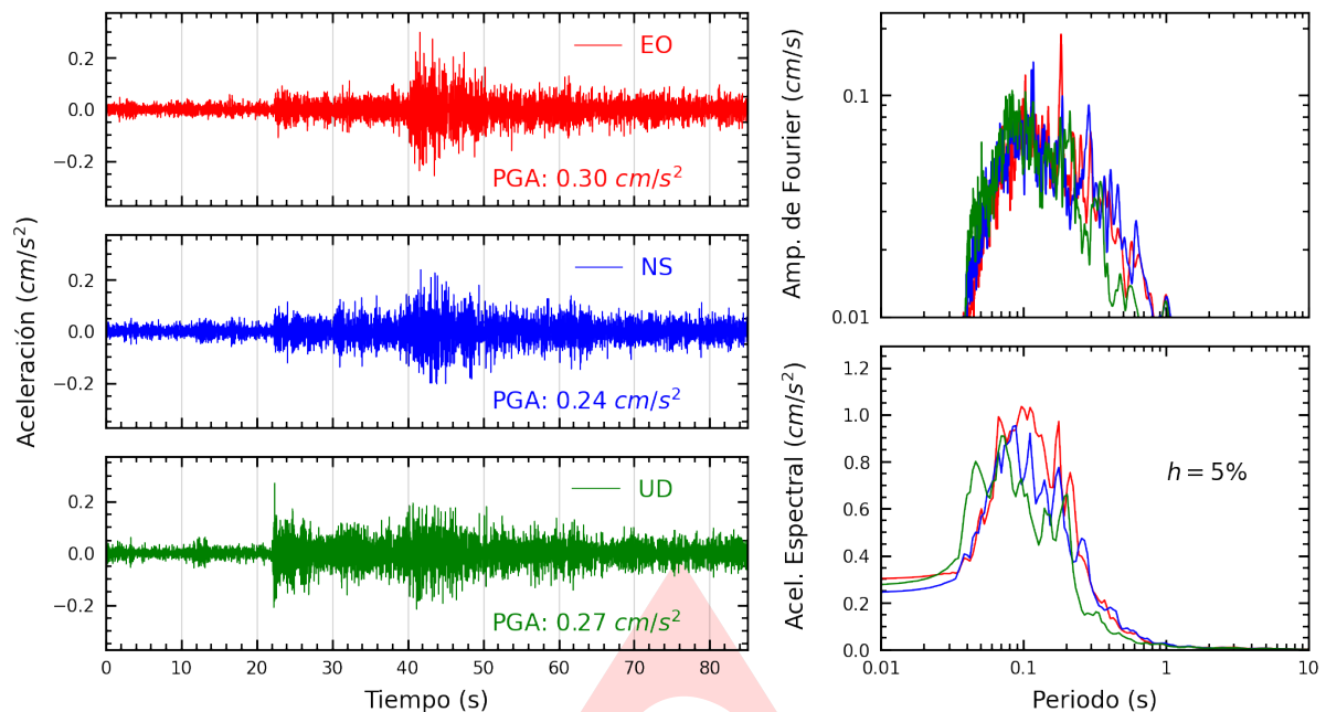
Figura A.1: Registros tiempo-historia, espectros de Fourier y de respuesta en las direcciones EO, NS y vertical de la estación UNICA. Sismo de Nazca, Nazca - Ica del 2024-05-24, 00:28:32 (Hora local)
